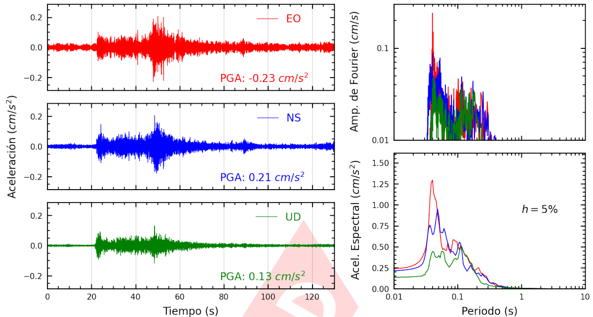
Figura A.3: Registros tiempo-historia, espectros de Fourier y de respuesta en las direcciones EO, NS y vertical de la estación UPTAC. Sismo de Conduriri, El Collao - Puno del 2025-01-03, 23:59:47 (Hora local)
