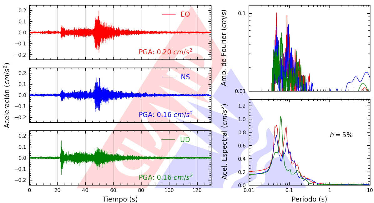
Figura A.5: Registros tiempo-historia, espectros de Fourier y de respuesta en las direcciones EO, NS y vertical de la estación CREY. Sismo de Conduriri, El Collao - Puno del 2025-01-03, 23:59:47 (Hora local)
