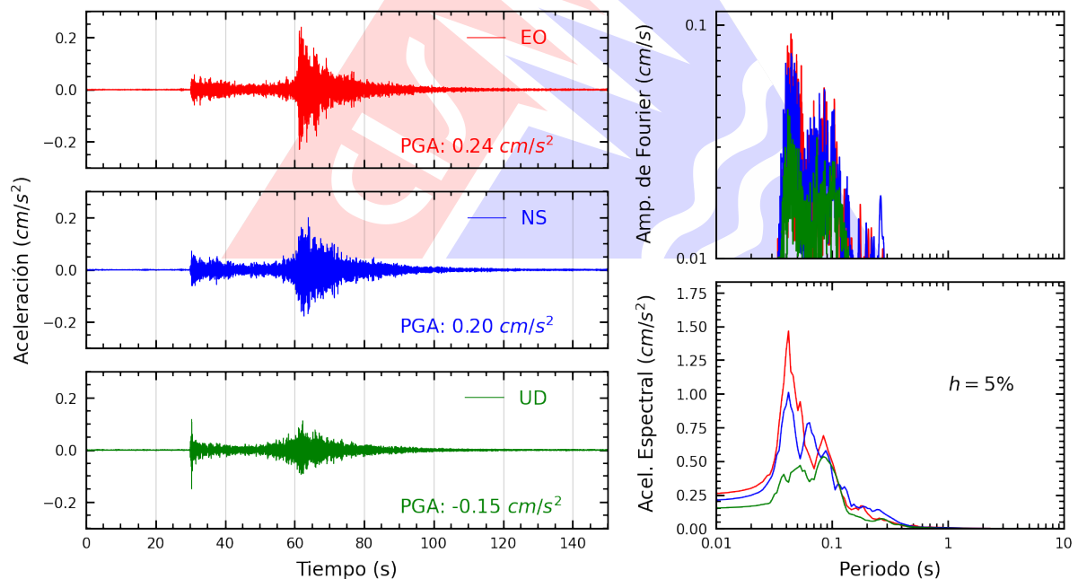
Figura A.2: Registros tiempo-historia, espectros de Fourier y de respuesta en las direcciones EO, NS y vertical de la estación UNSA2. Sismo de Conduriri, El Collao - Puno del 2025-01-03, 23:59:47 (Hora local)
