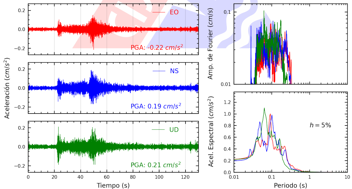
Figura A.4: Registros tiempo-historia, espectros de Fourier y de respuesta en las direcciones EO, NS y vertical de la estación UJBG4. Sismo de Conduriri, El Collao - Puno del 2025-01-03, 23:59:47 (Hora local)
