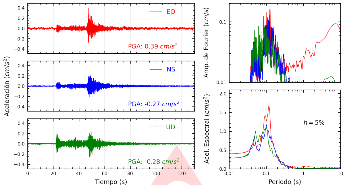
Figura A.1: Registros tiempo-historia, espectros de Fourier y de respuesta en las direcciones EO, NS y vertical de la estación UJBG3. Sismo de Conduriri, El Collao - Puno del 2025-01-03, 23:59:47 (Hora local)
