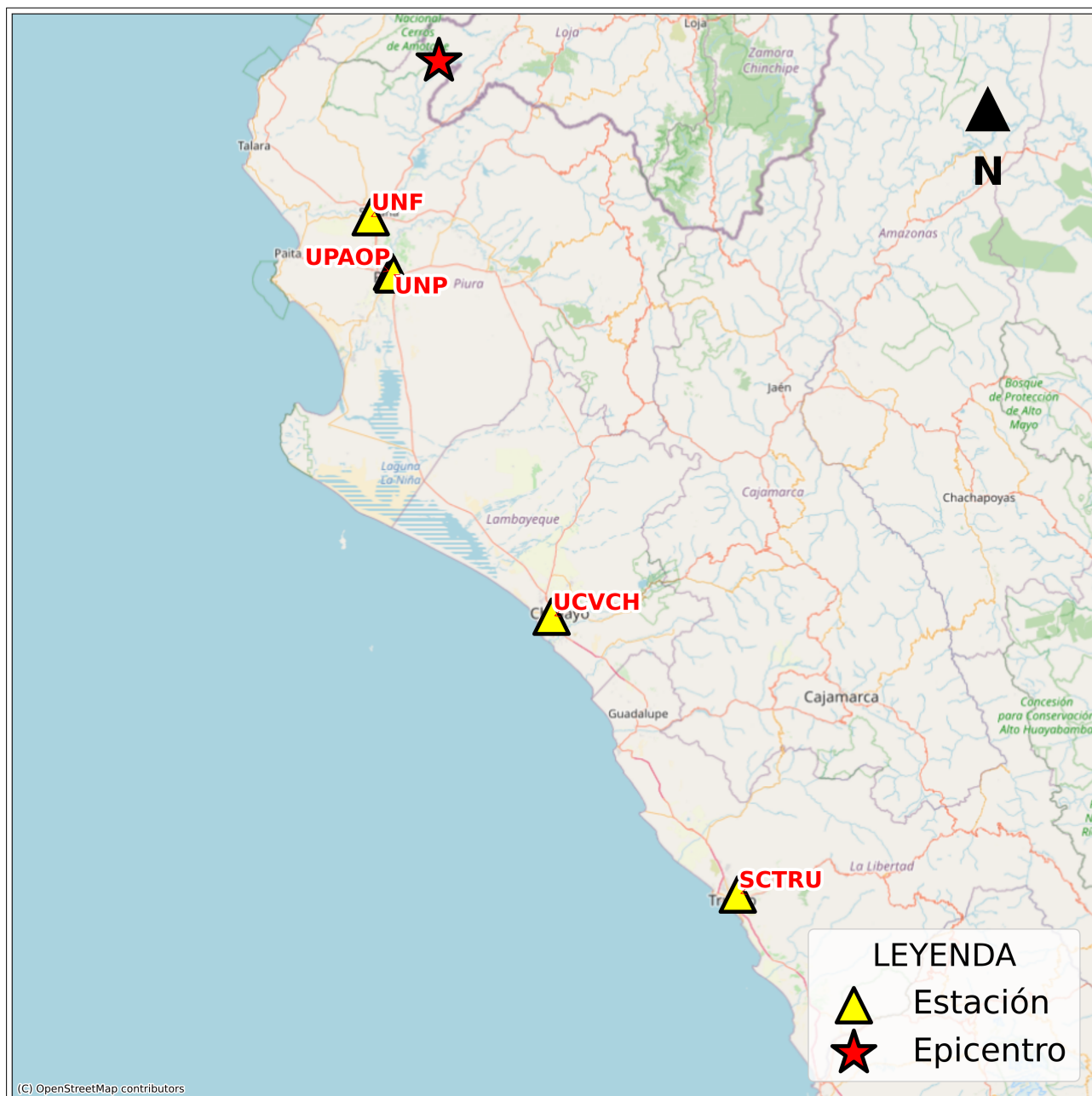
Figura 2: Mapa de ubicación de la(s) estación(es) acelerográfica(s) correspondiente(s) al Sismo de Zorritos, Contralmirante Villar - Tumbes del 05 de enero de 2025 a las 03:19:52 (hora local)
