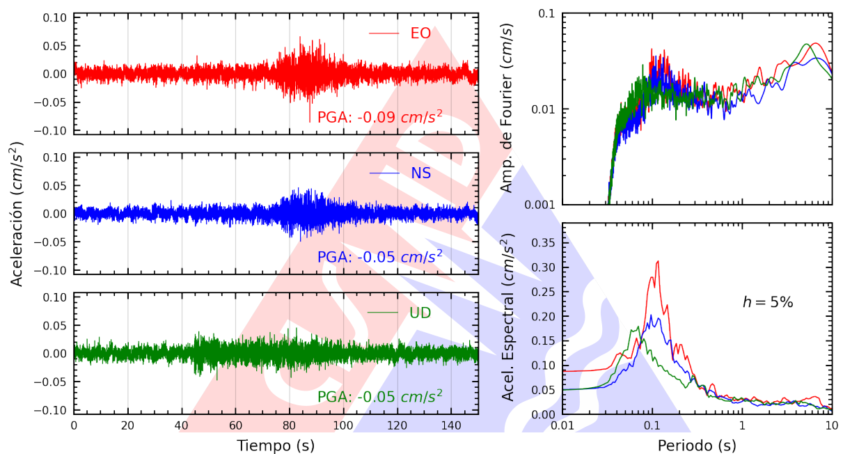
Figura A.5: Registros tiempo-historia, espectros de Fourier y de respuesta en las direcciones EO, NS y vertical de la estación UCVCH. Sismo de Zorritos, Contralmirante Villar - Tumbes del 2025-01-05, 03:19:52 (Hora local)
