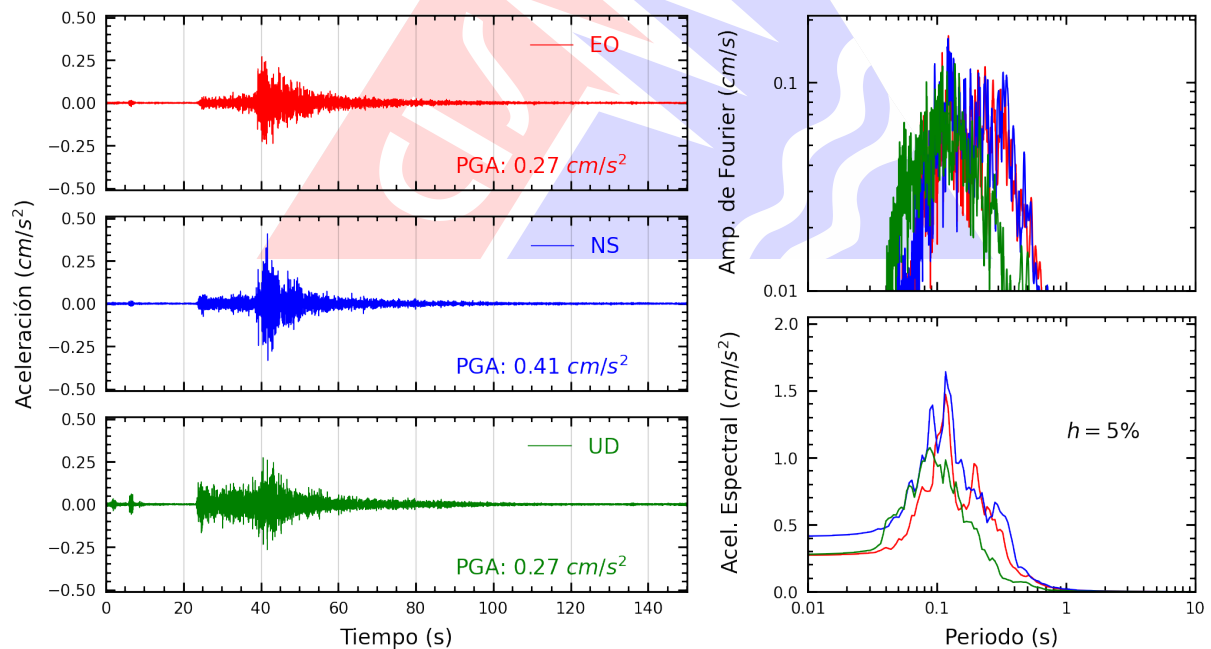
Figura A.2: Registros tiempo-historia, espectros de Fourier y de respuesta en las direcciones EO, NS y vertical de la estación UNP. Sismo de Zorritos, Contralmirante Villar - Tumbes del 2025-01-05, 03:19:52 (Hora local)
