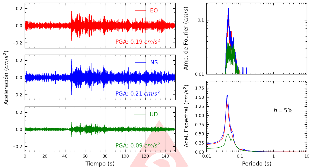
Figura A.3: Registros tiempo-historia, espectros de Fourier y de respuesta en las direcciones EO, NS y vertical de la estación SCTRU. Sismo de Zorritos, Contralmirante Villar - Tumbes del 2025-01-05, 03:19:52 (Hora local)
