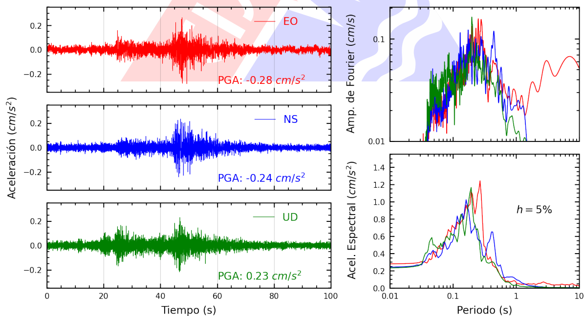
Figura A.6: Registros tiempo-historia, espectros de Fourier y de respuesta en las direcciones EO, NS y vertical de la estación UJBG3. Sismo de Ilo, Ilo - Moquegua del 2025-03-06, 13:13:35 (Hora local)
