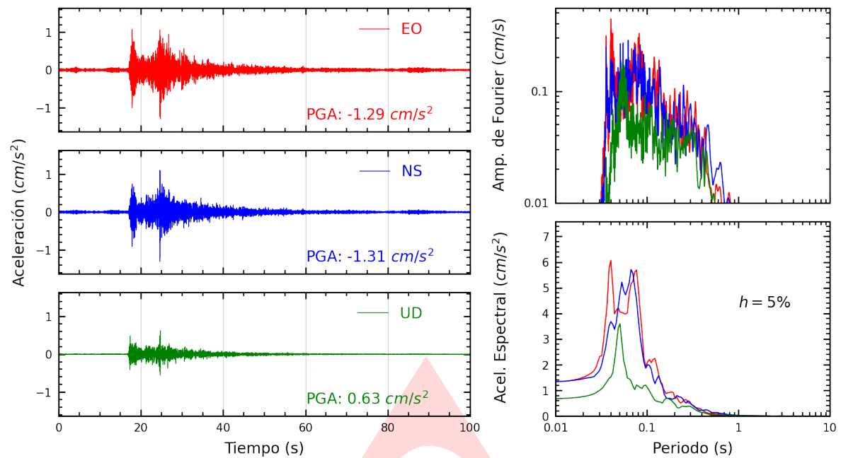
Figura A.1: Registros tiempo-historia, espectros de Fourier y de respuesta en las direcciones EO, NS y vertical de la estación UNAM. Sismo de Ilo, Ilo - Moquegua del 2025-03-06, 13:13:35 (Hora local)
