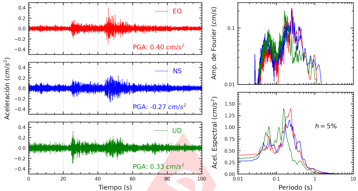
Figura A.3: Registros tiempo-historia, espectros de Fourier y de respuesta en las direcciones EO, NS y vertical de la estación UJBG4. Sismo de Ilo, Ilo - Moquegua del 2025-03-06, 13:13:35 (Hora local)
