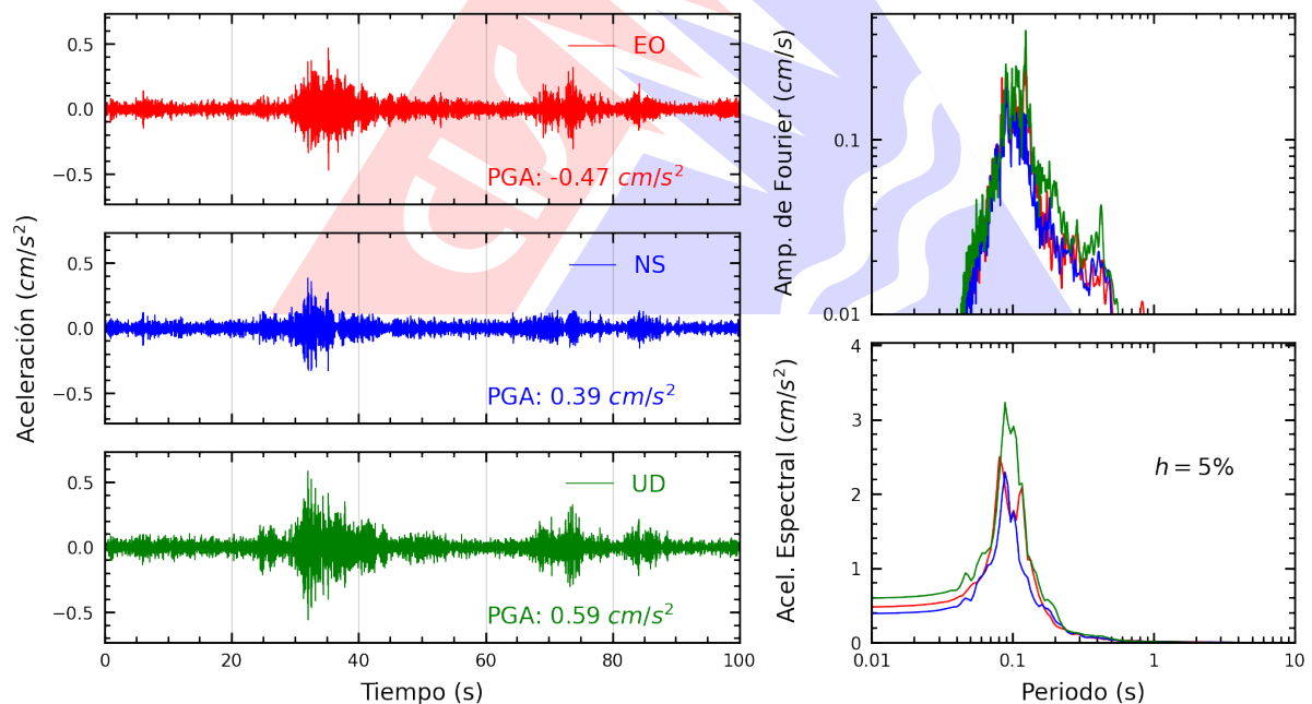
Figura A.2: Registros tiempo-historia, espectros de Fourier y de respuesta en las direcciones EO, NS y vertical de la estación UANCV. Sismo de Ilo, Ilo - Moquegua del 2025-03-06, 13:13:35 (Hora local)
