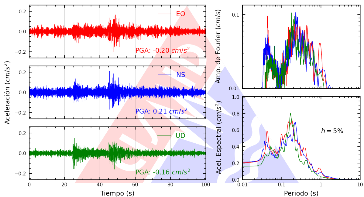
Figura A.7: Registros tiempo-historia, espectros de Fourier y de respuesta en las direcciones EO, NS y vertical de la estación UPTAC. Sismo de Ilo, Ilo - Moquegua del 2025-03-06, 13:13:35 (Hora local)
