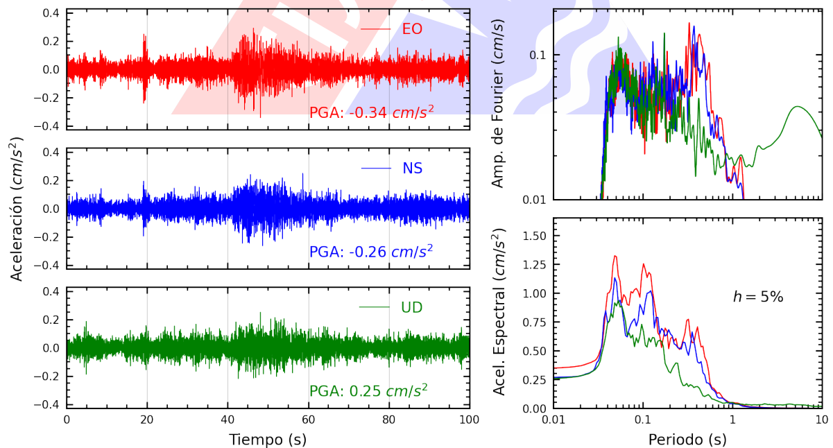
Figura A.4: Registros tiempo-historia, espectros de Fourier y de respuesta en las direcciones EO, NS y vertical de la estación SCARQ. Sismo de Ilo, Ilo - Moquegua del 2025-03-06, 13:13:35 (Hora local)
