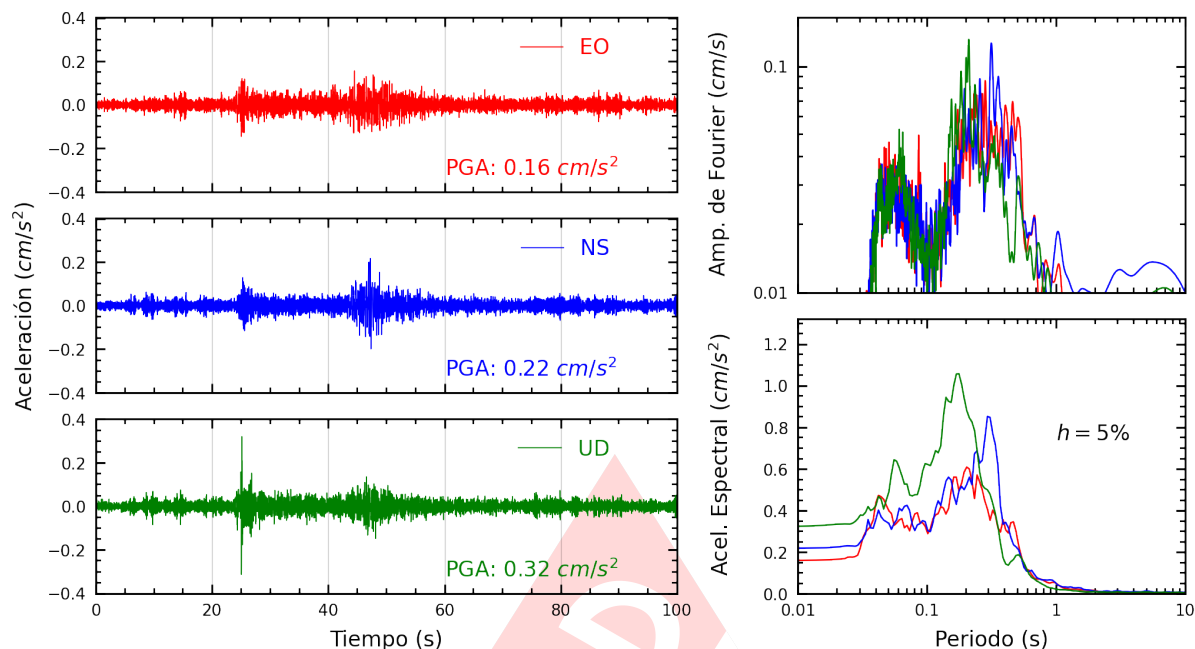
Figura A.5: Registros tiempo-historia, espectros de Fourier y de respuesta en las direcciones EO, NS y vertical de la estación CREY. Sismo de Ilo, Ilo - Moquegua del 2025-03-06, 13:13:35 (Hora local)
