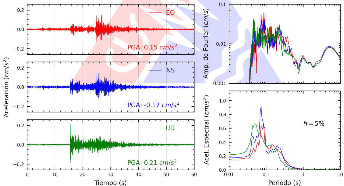
Figura A.2: Registros tiempo-historia, espectros de Fourier y de respuesta en las direcciones EO, NS y vertical de la estación UNF. Sismo de Sechura, Sechura - Piura del 2025-04-01, 03:45:02 (Hora local)
