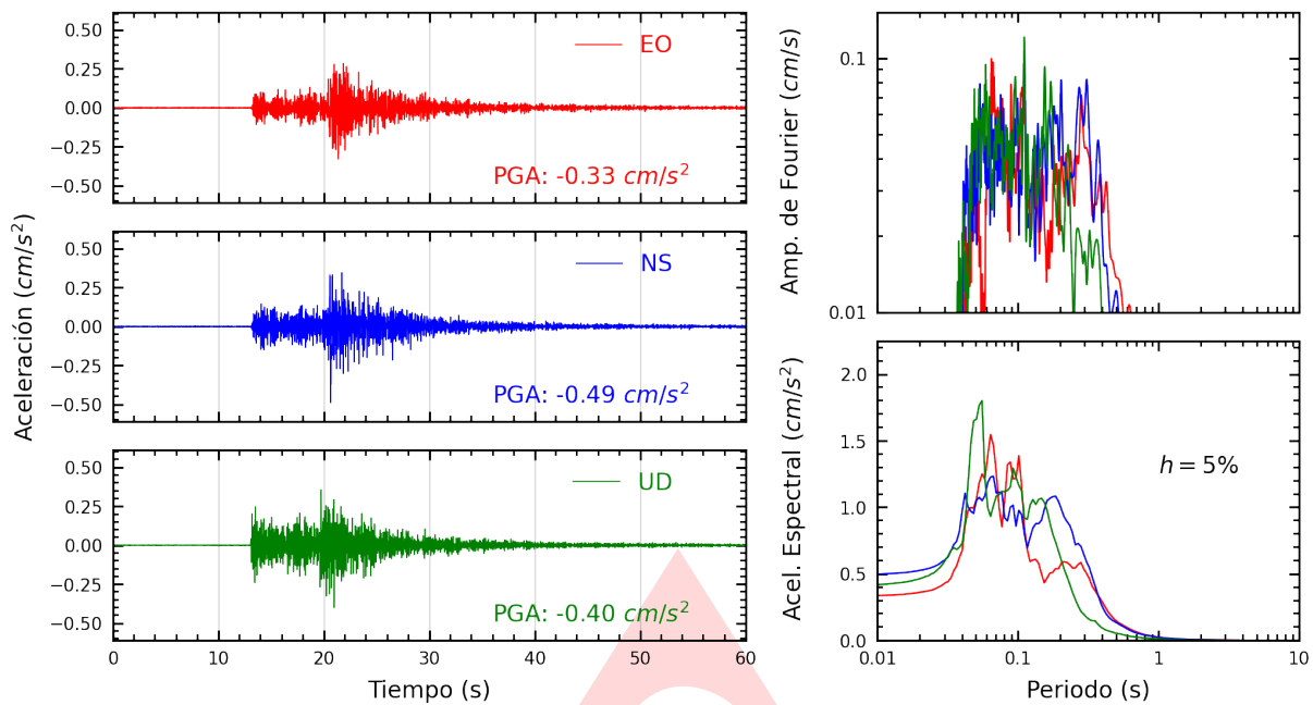
Figura A.1: Registros tiempo-historia, espectros de Fourier y de respuesta en las direcciones EO, NS y vertical de la estación UPAOP. Sismo de Sechura, Sechura - Piura del 2025-04-01, 03:45:02 (Hora local)
