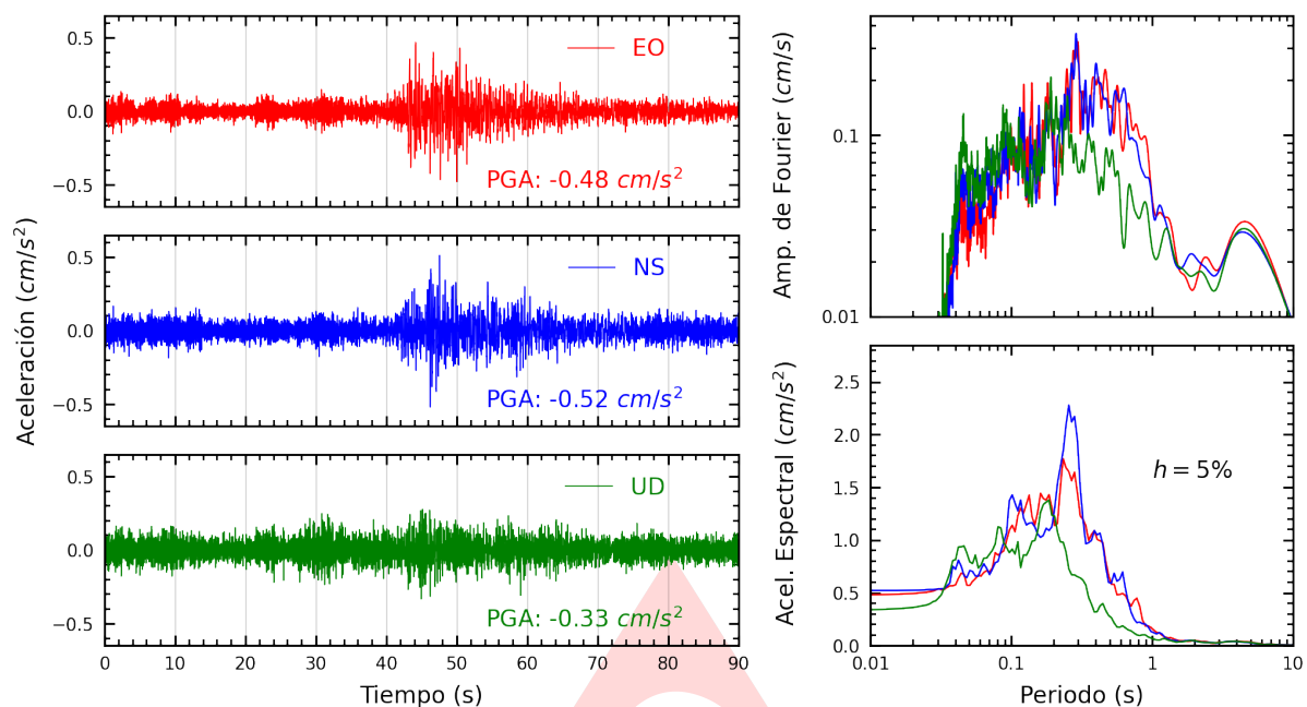
Figura A.1: Registros tiempo-historia, espectros de Fourier y de respuesta en las direcciones EO, NS y vertical de la estación UNICA. Sismo de Marcona, Nazca - Ica del 2025-04-03, 08:03:47 (Hora local)
