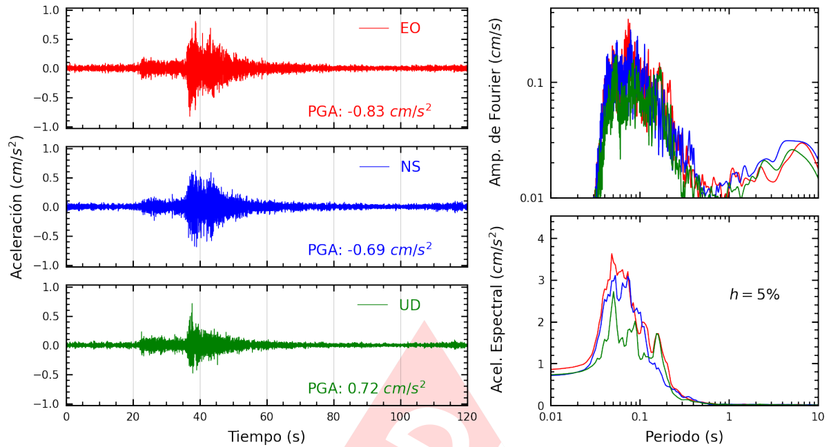
Figura A.25: Registros tiempo-historia, espectros de Fourier y de respuesta en las direcciones EO, NS y vertical de la estación FICPE. Sismo de Calango, Cañete - Lima del 2025-04-07, 10:24:02 (Hora local)
