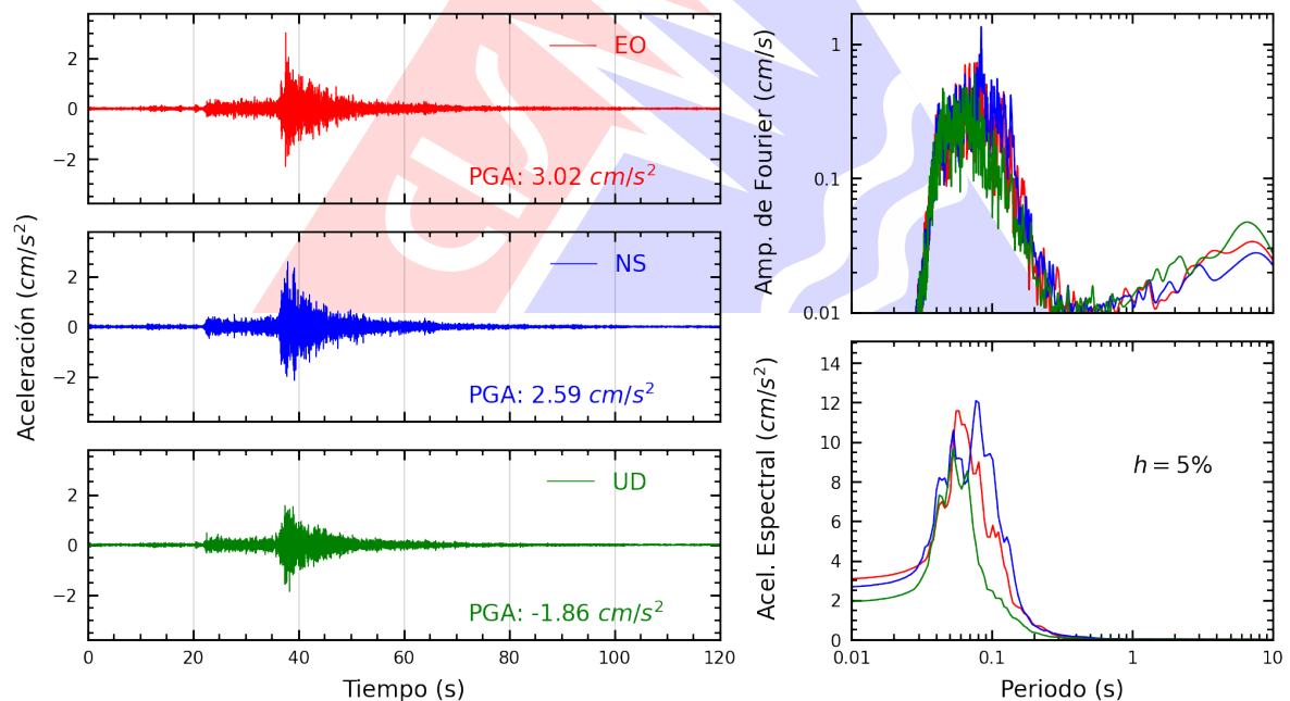
Figura A.2: Registros tiempo-historia, espectros de Fourier y de respuesta en las direcciones EO, NS y vertical de la estación JOSEO. Sismo de Calango, Cañete - Lima del 2025-04-07, 10:24:02 (Hora local)
