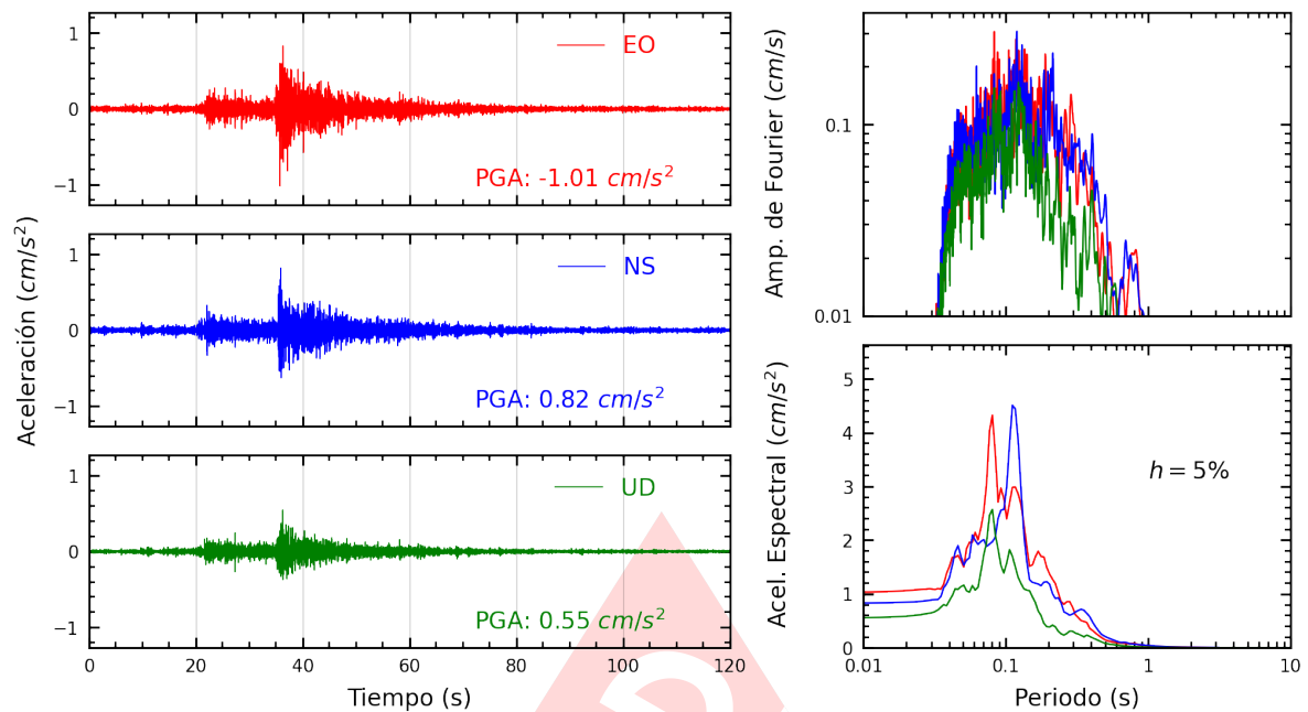
Figura A.19: Registros tiempo-historia, espectros de Fourier y de respuesta en las direcciones EO, NS y vertical de la estación BRISA. Sismo de Calango, Cañete - Lima del 2025-04-07, 10:24:02 (Hora local)
