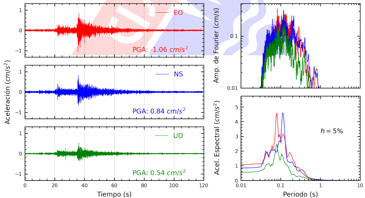
Figura A.18: Registros tiempo-historia, espectros de Fourier y de respuesta en las direcciones EO, NS y vertical de la estación BRIS2. Sismo de Calango, Cañete - Lima del 2025-04-07, 10:24:02 (Hora local)
