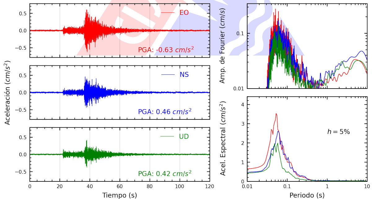
Figura A.28: Registros tiempo-historia, espectros de Fourier y de respuesta en las direcciones EO, NS y vertical de la estación UCSS. Sismo de Calango, Cañete - Lima del 2025-04-07, 10:24:02 (Hora local)
