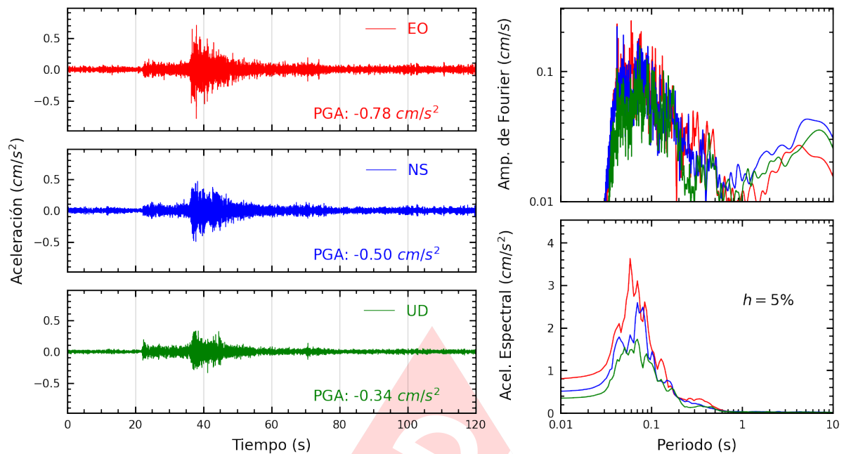
Figura A.27: Registros tiempo-historia, espectros de Fourier y de respuesta en las direcciones EO, NS y vertical de la estación CEPRE. Sismo de Calango, Cañete - Lima del 2025-04-07, 10:24:02 (Hora local)
