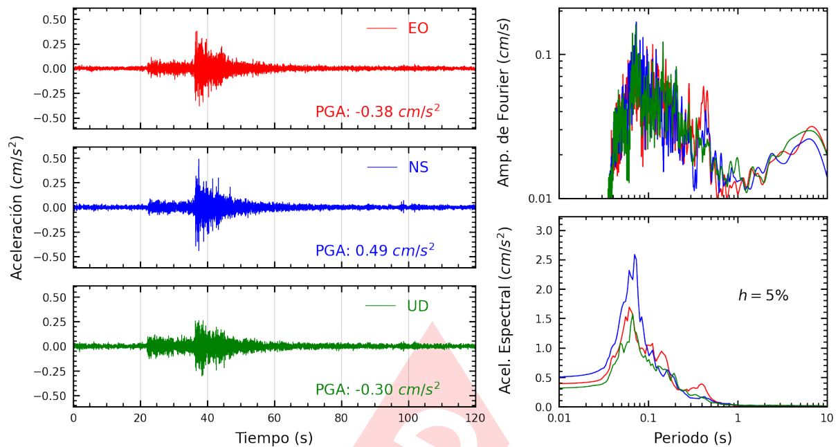
Figura A.31: Registros tiempo-historia, espectros de Fourier y de respuesta en las direcciones EO, NS y vertical de la estación UNFV. Sismo de Calango, Cañete - Lima del 2025-04-07, 10:24:02 (Hora local)
