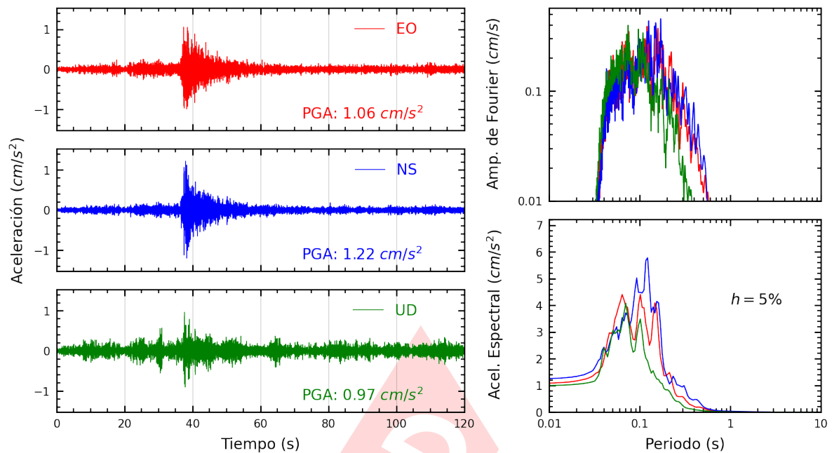
Figura A.15: Registros tiempo-historia, espectros de Fourier y de respuesta en las direcciones EO, NS y vertical de la estación SCOLI. Sismo de Calango, Cañete - Lima del 2025-04-07, 10:24:02 (Hora local)
