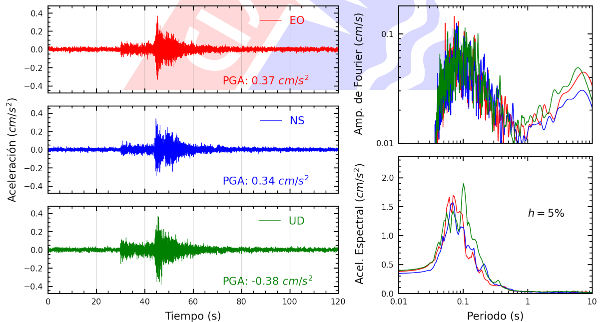
Figura A.32: Registros tiempo-historia, espectros de Fourier y de respuesta en las direcciones EO, NS y vertical de la estación UNMSM. Sismo de Calango, Cañete - Lima del 2025-04-07, 10:24:02 (Hora local)
