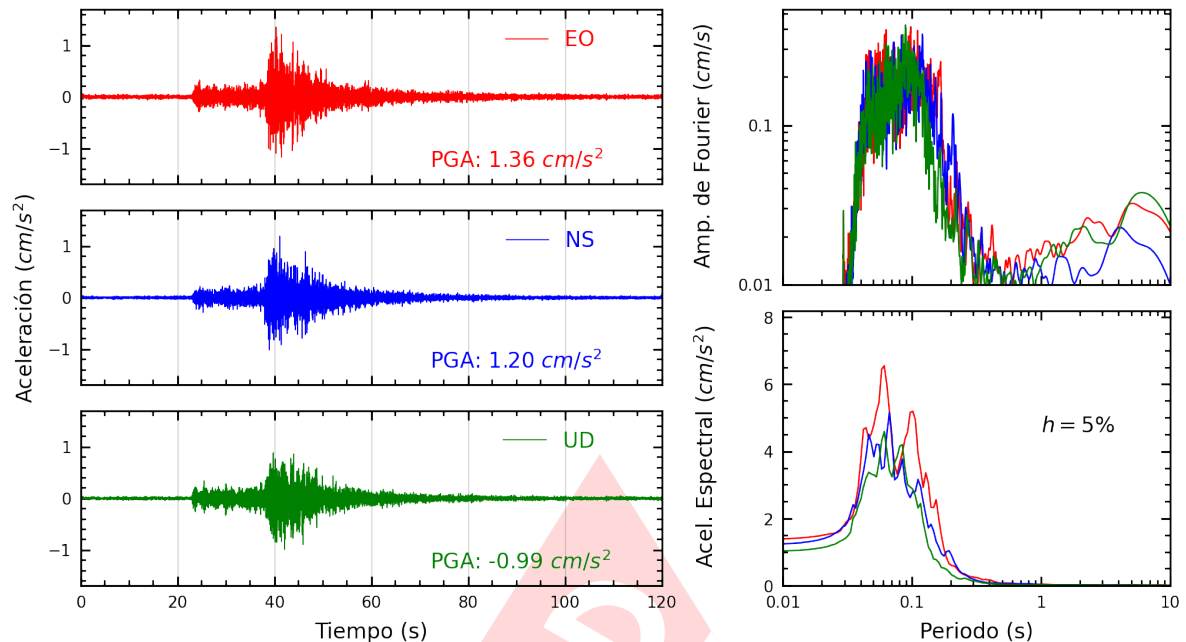
Figura A.9: Registros tiempo-historia, espectros de Fourier y de respuesta en las direcciones EO, NS y vertical de la estación AMORE. Sismo de Calango, Cañete - Lima del 2025-04-07, 10:24:02 (Hora local)
