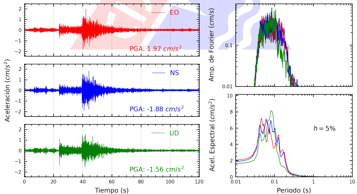
Figura A.4: Registros tiempo-historia, espectros de Fourier y de respuesta en las direcciones EO, NS y vertical de la estación SROS2. Sismo de Calango, Cañete - Lima del 2025-04-07, 10:24:02 (Hora local)
