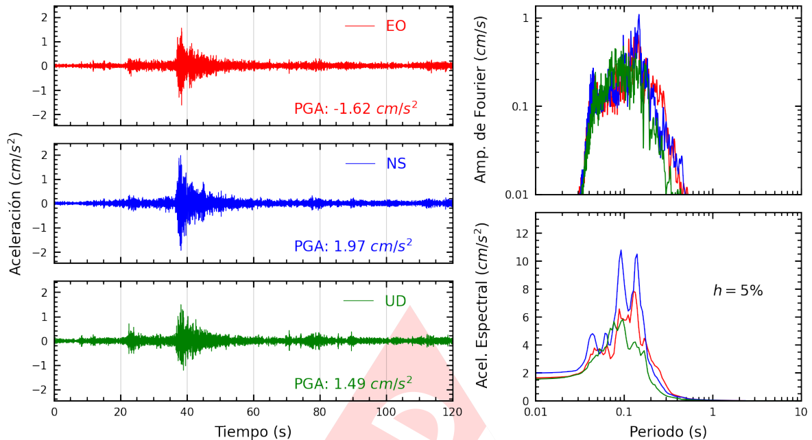
Figura A.5: Registros tiempo-historia, espectros de Fourier y de respuesta en las direcciones EO, NS y vertical de la estación CARA2. Sismo de Calango, Cañete - Lima del 2025-04-07, 10:24:02 (Hora local)
