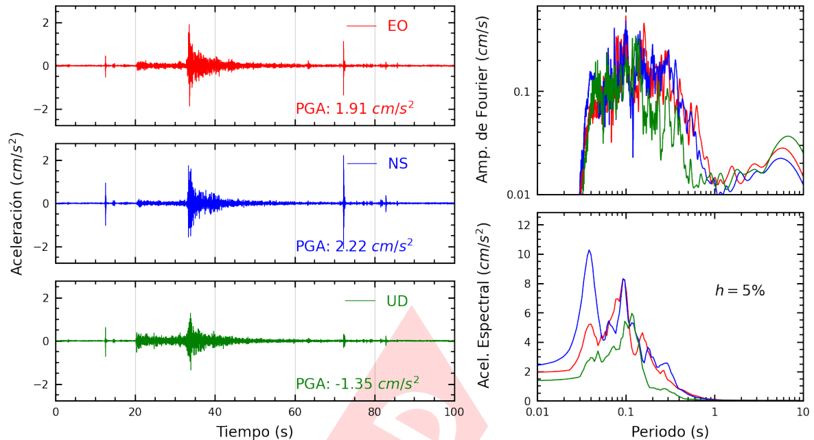
Figura A.3: Registros tiempo-historia, espectros de Fourier y de respuesta en las direcciones EO, NS y vertical de la estación USILP. Sismo de Calango, Cañete - Lima del 2025-04-07, 10:24:02 (Hora local)
