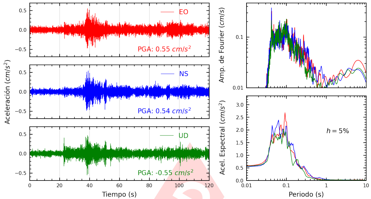
Figura A.29: Registros tiempo-historia, espectros de Fourier y de respuesta en las direcciones EO, NS y vertical de la estación MADRE. Sismo de Calango, Cañete - Lima del 2025-04-07, 10:24:02 (Hora local)
