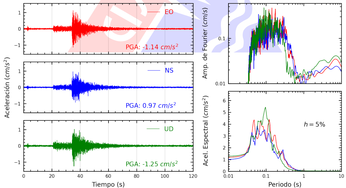
Figura A.14: Registros tiempo-historia, espectros de Fourier y de respuesta en las direcciones EO, NS y vertical de la estación SOVES. Sismo de Calango, Cañete - Lima del 2025-04-07, 10:24:02 (Hora local)
