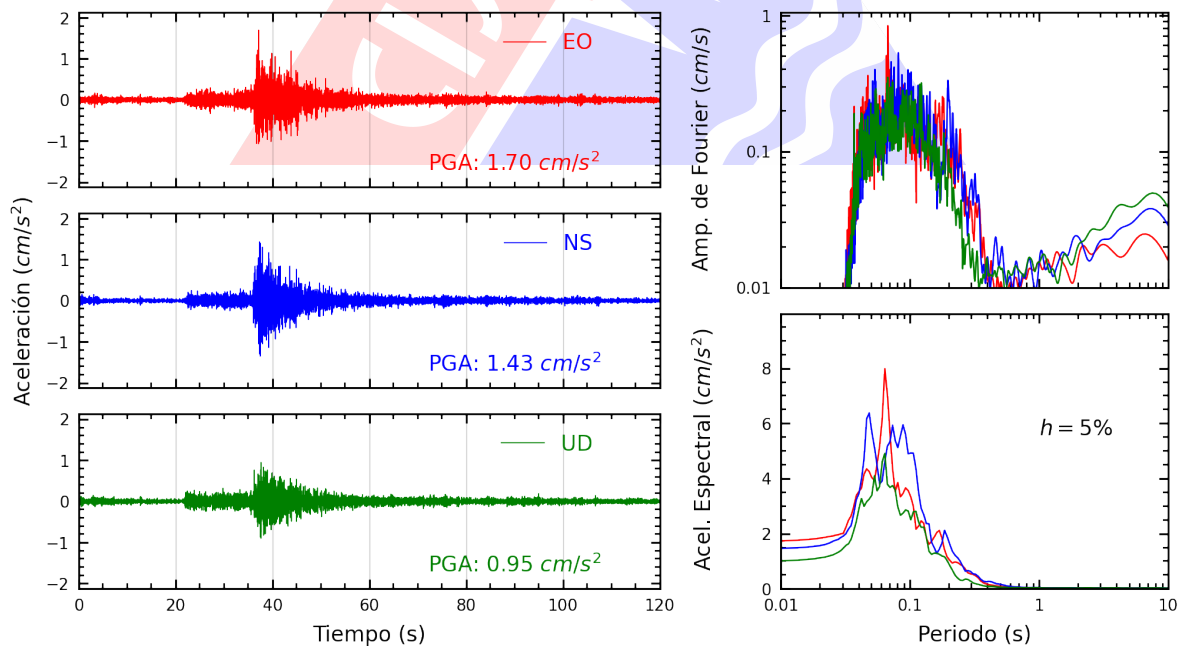
Figura A.6: Registros tiempo-historia, espectros de Fourier y de respuesta en las direcciones EO, NS y vertical de la estación INDEP. Sismo de Calango, Cañete - Lima del 2025-04-07, 10:24:02 (Hora local)
