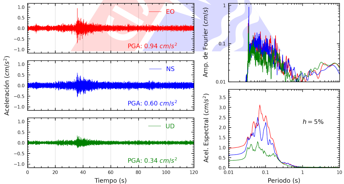
Figura A.20: Registros tiempo-historia, espectros de Fourier y de respuesta en las direcciones EO, NS y vertical de la estación UPCVI. Sismo de Calango, Cañete - Lima del 2025-04-07, 10:24:02 (Hora local)
