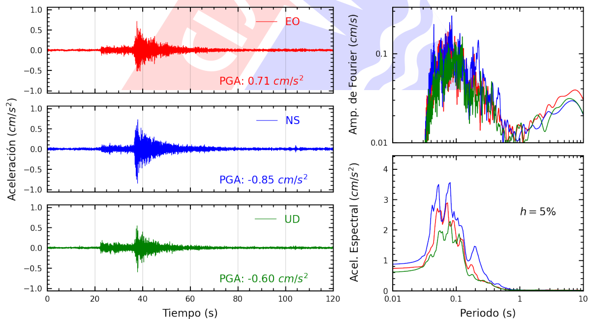
Figura A.24: Registros tiempo-historia, espectros de Fourier y de respuesta en las direcciones EO, NS y vertical de la estación COMAS. Sismo de Calango, Cañete - Lima del 2025-04-07, 10:24:02 (Hora local)
