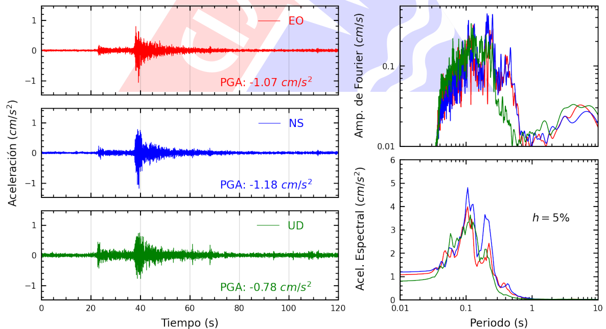
Figura A.16: Registros tiempo-historia, espectros de Fourier y de respuesta en las direcciones EO, NS y vertical de la estación MDPP. Sismo de Calango, Cañete - Lima del 2025-04-07, 10:24:02 (Hora local)
