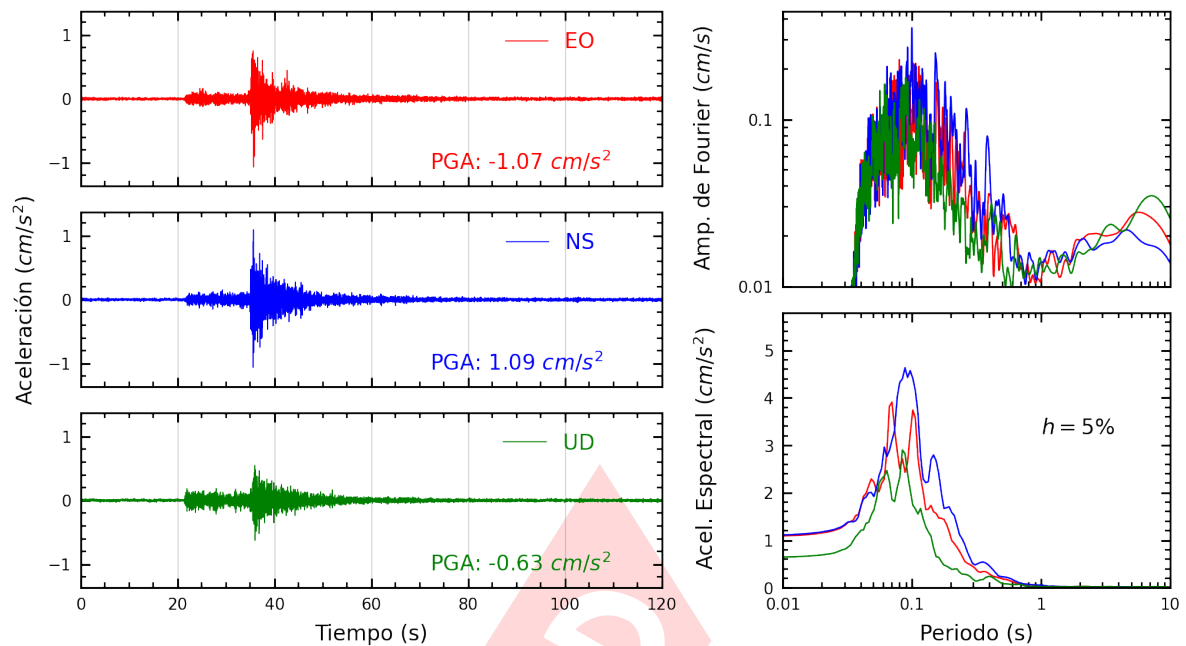
Figura A.17: Registros tiempo-historia, espectros de Fourier y de respuesta en las direcciones EO, NS y vertical de la estación SERVI. Sismo de Calango, Cañete - Lima del 2025-04-07, 10:24:02 (Hora local)
