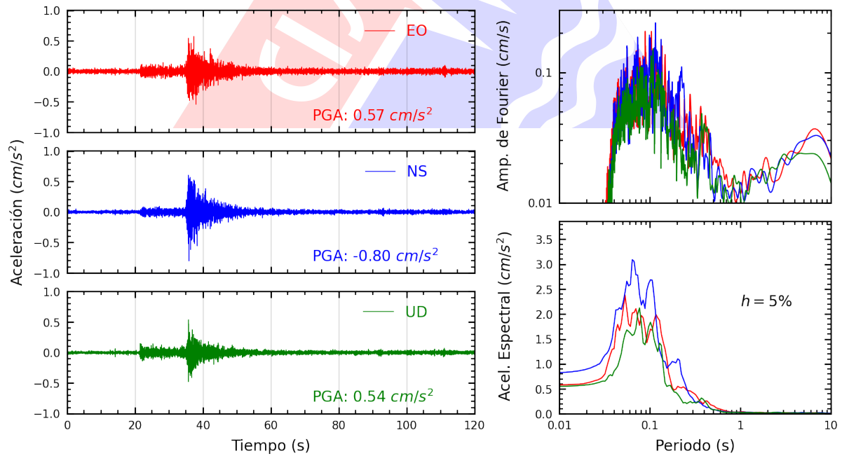
Figura A.26: Registros tiempo-historia, espectros de Fourier y de respuesta en las direcciones EO, NS y vertical de la estación INICT. Sismo de Calango, Cañete - Lima del 2025-04-07, 10:24:02 (Hora local)
