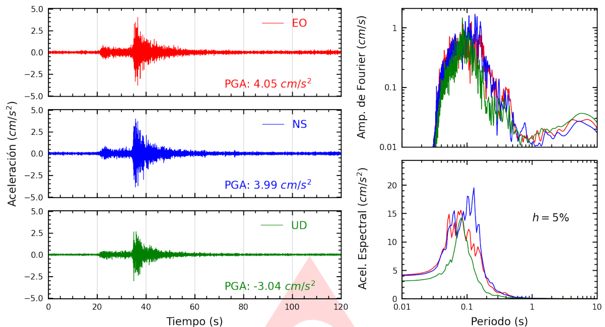
Figura A.1: Registros tiempo-historia, espectros de Fourier y de respuesta en las direcciones EO, NS y vertical de la estación USILM. Sismo de Calango, Cañete - Lima del 2025-04-07, 10:24:02 (Hora local)
