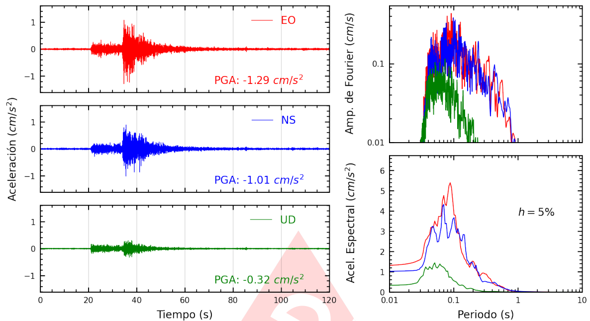
Figura A.13: Registros tiempo-historia, espectros de Fourier y de respuesta en las direcciones EO, NS y vertical de la estación UCVA2. Sismo de Calango, Cañete - Lima del 2025-04-07, 10:24:02 (Hora local)
