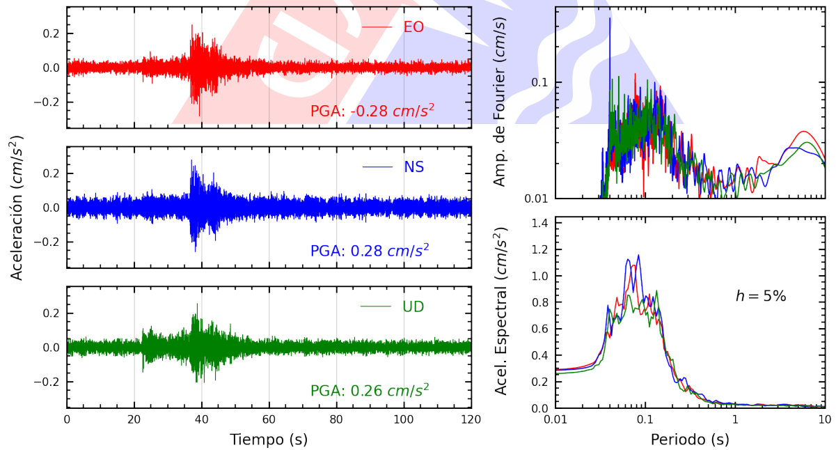
Figura A.34: Registros tiempo-historia, espectros de Fourier y de respuesta en las direcciones EO, NS y vertical de la estación BONDY. Sismo de Calango, Cañete - Lima del 2025-04-07, 10:24:02 (Hora local)
