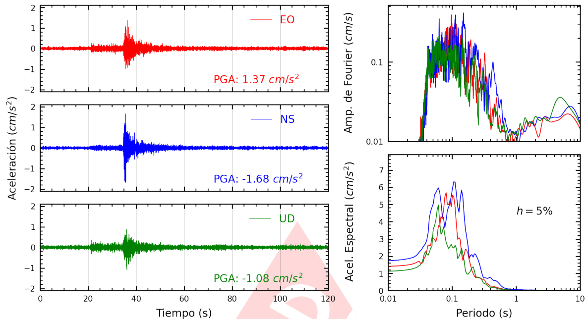
Figura A.7: Registros tiempo-historia, espectros de Fourier y de respuesta en las direcciones EO, NS y vertical de la estación URPE. Sismo de Calango, Cañete - Lima del 2025-04-07, 10:24:02 (Hora local)
