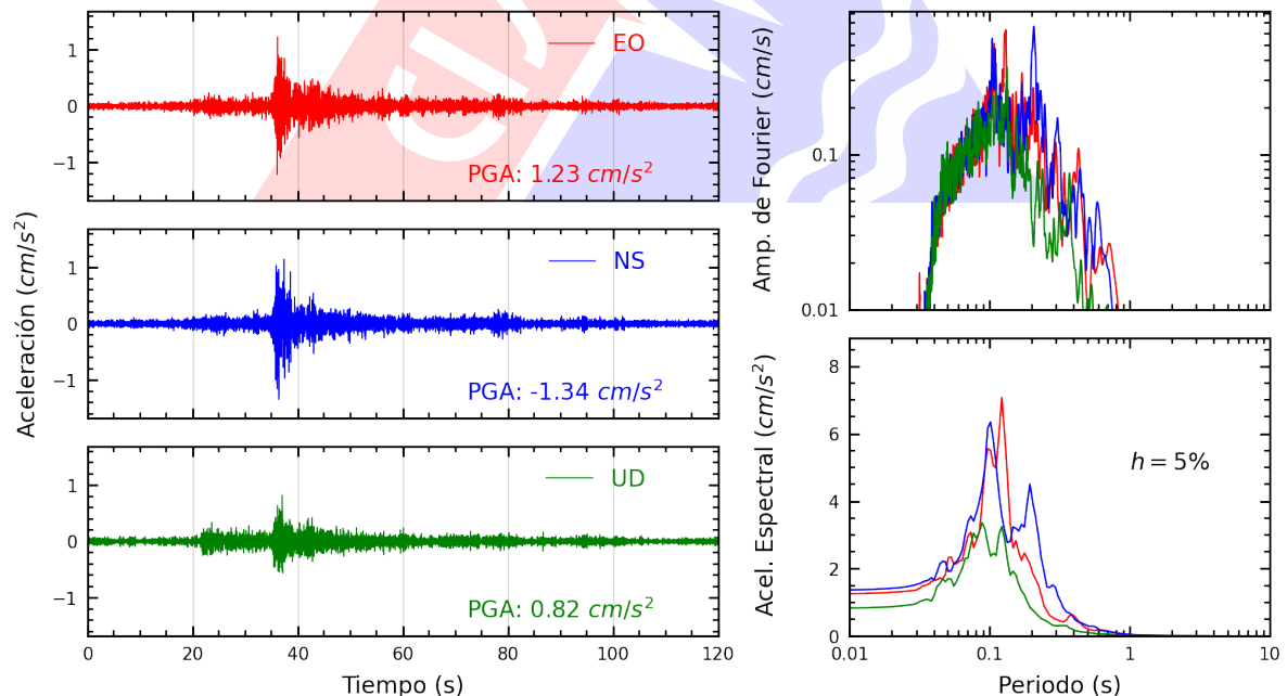
Figura A.10: Registros tiempo-historia, espectros de Fourier y de respuesta en las direcciones EO, NS y vertical de la estación SCCHO. Sismo de Calango, Cañete - Lima del 2025-04-07, 10:24:02 (Hora local)
