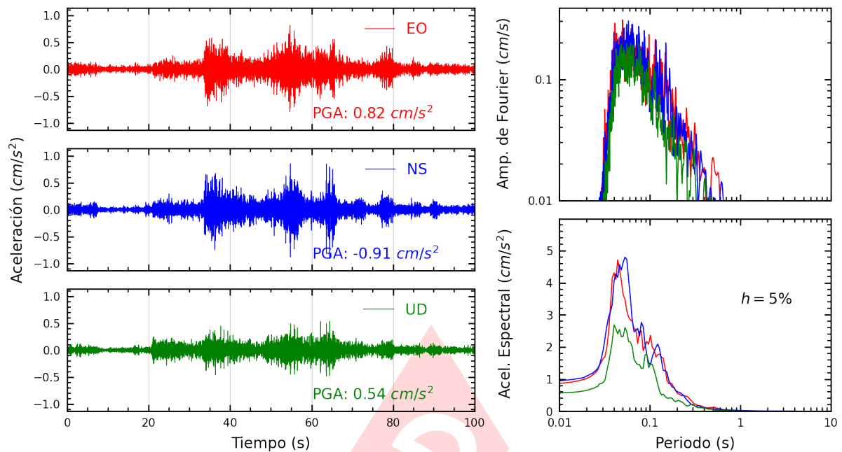
Figura A.21: Registros tiempo-historia, espectros de Fourier y de respuesta en las direcciones EO, NS y vertical de la estación PACHA. Sismo de Calango, Cañete - Lima del 2025-04-07, 10:24:02 (Hora local)
