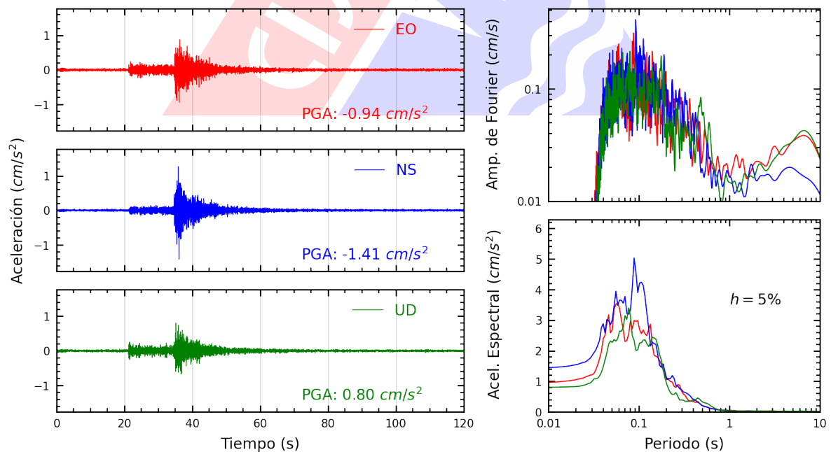
Figura A.8: Registros tiempo-historia, espectros de Fourier y de respuesta en las direcciones EO, NS y vertical de la estación IMCA. Sismo de Calango, Cañete - Lima del 2025-04-07, 10:24:02 (Hora local)
