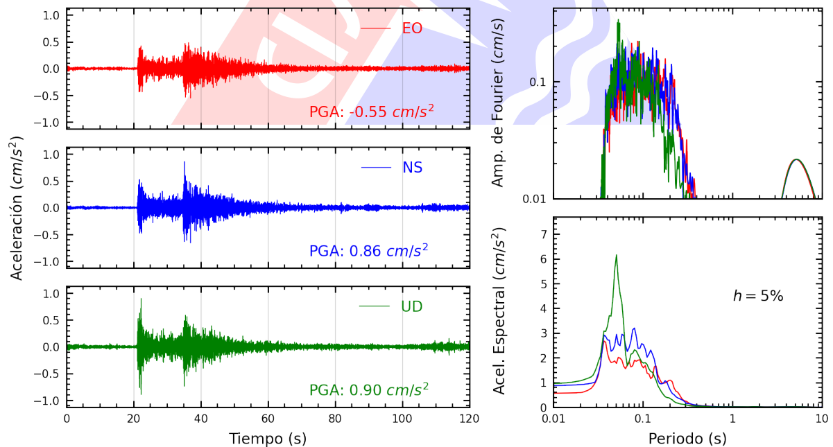
Figura A.22: Registros tiempo-historia, espectros de Fourier y de respuesta en las direcciones EO, NS y vertical de la estación ASIA. Sismo de Calango, Cañete - Lima del 2025-04-07, 10:24:02 (Hora local)
