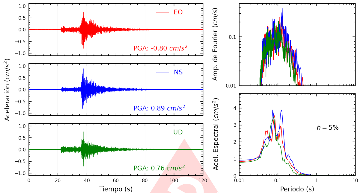
Figura A.23: Registros tiempo-historia, espectros de Fourier y de respuesta en las direcciones EO, NS y vertical de la estación JALV2. Sismo de Calango, Cañete - Lima del 2025-04-07, 10:24:02 (Hora local)
