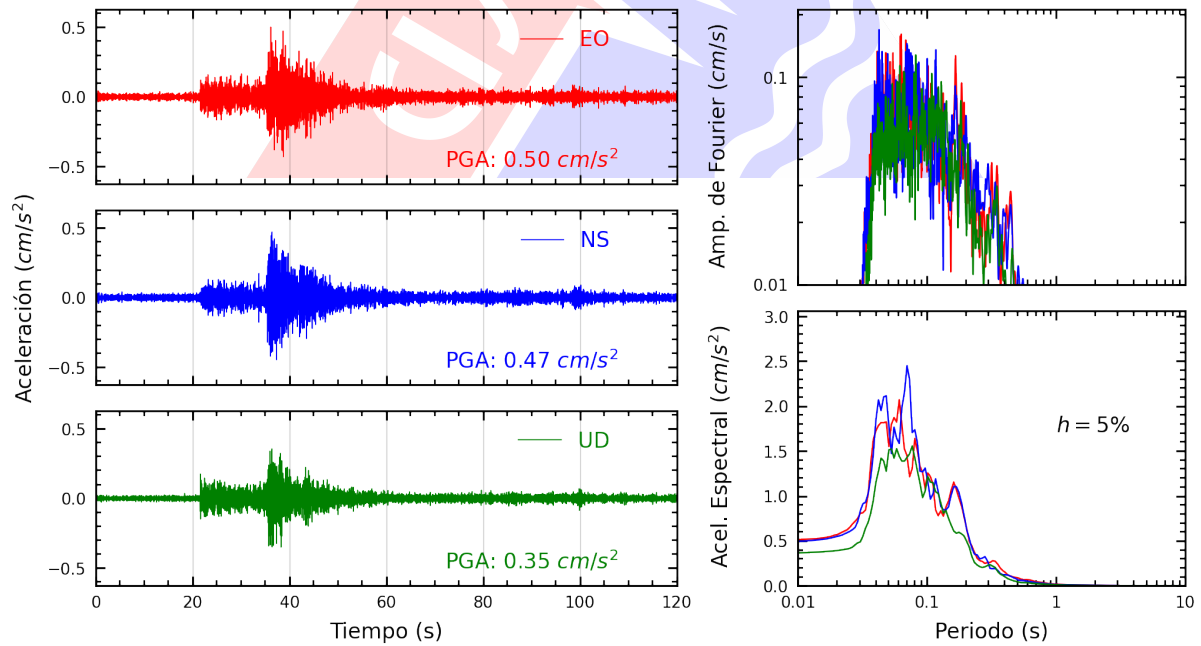
Figura A.30: Registros tiempo-historia, espectros de Fourier y de respuesta en las direcciones EO, NS y vertical de la estación BORJA. Sismo de Calango, Cañete - Lima del 2025-04-07, 10:24:02 (Hora local)
