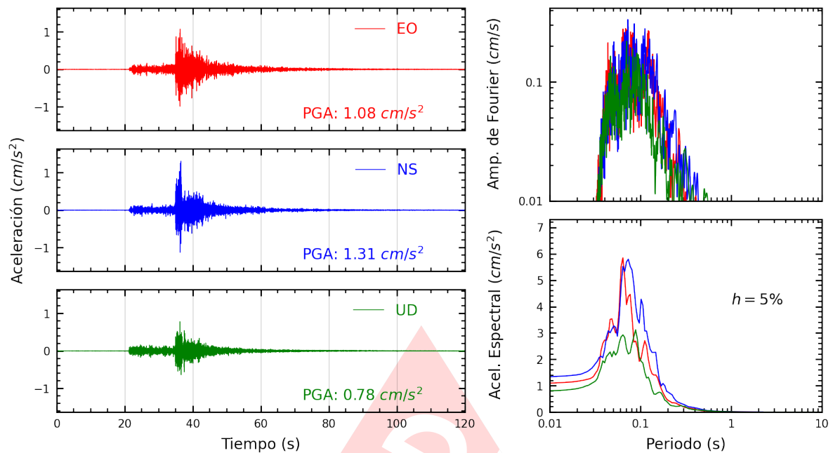
Figura A.11: Registros tiempo-historia, espectros de Fourier y de respuesta en las direcciones EO, NS y vertical de la estación ATARJ. Sismo de Calango, Cañete - Lima del 2025-04-07, 10:24:02 (Hora local)
