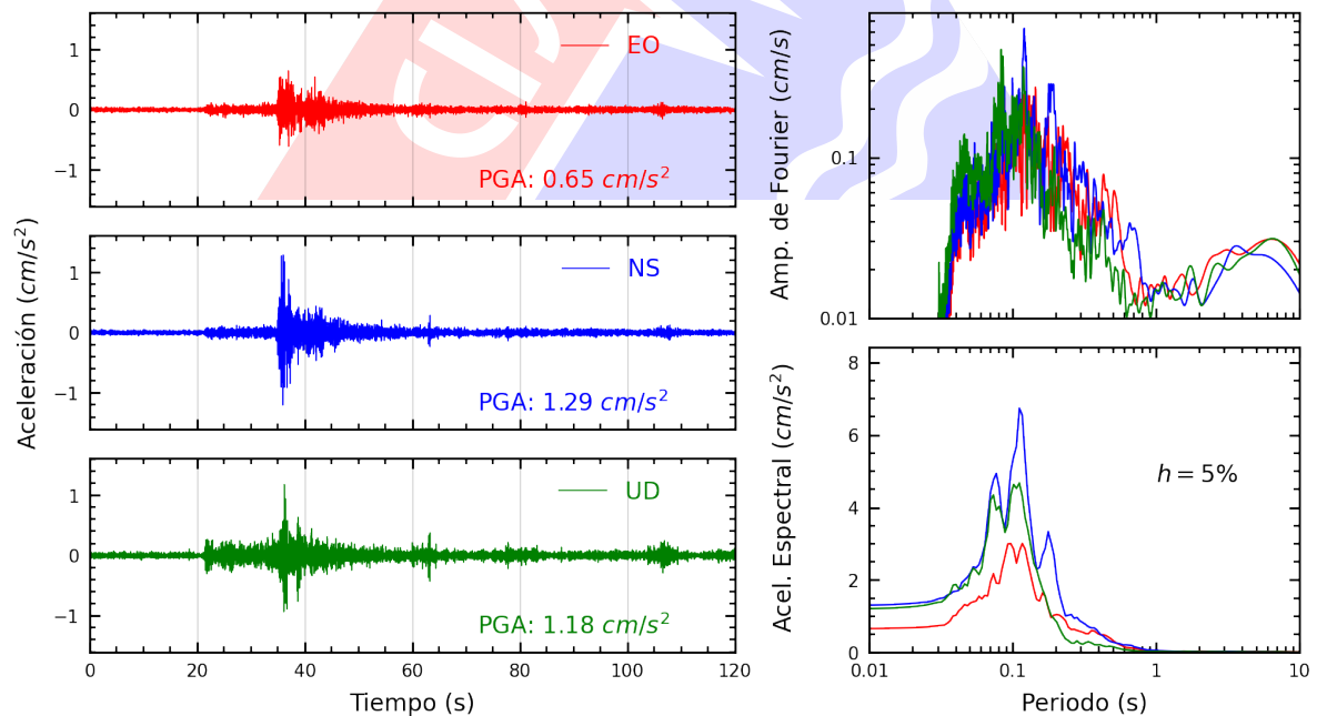
Figura A.12: Registros tiempo-historia, espectros de Fourier y de respuesta en las direcciones EO, NS y vertical de la estación SOCHO. Sismo de Calango, Cañete - Lima del 2025-04-07, 10:24:02 (Hora local)
