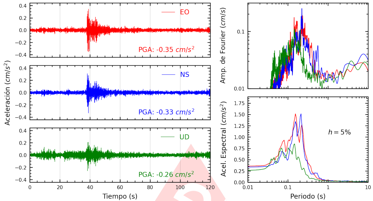
Figura A.33: Registros tiempo-historia, espectros de Fourier y de respuesta en las direcciones EO, NS y vertical de la estación DSML. Sismo de Calango, Cañete - Lima del 2025-04-07, 10:24:02 (Hora local)
