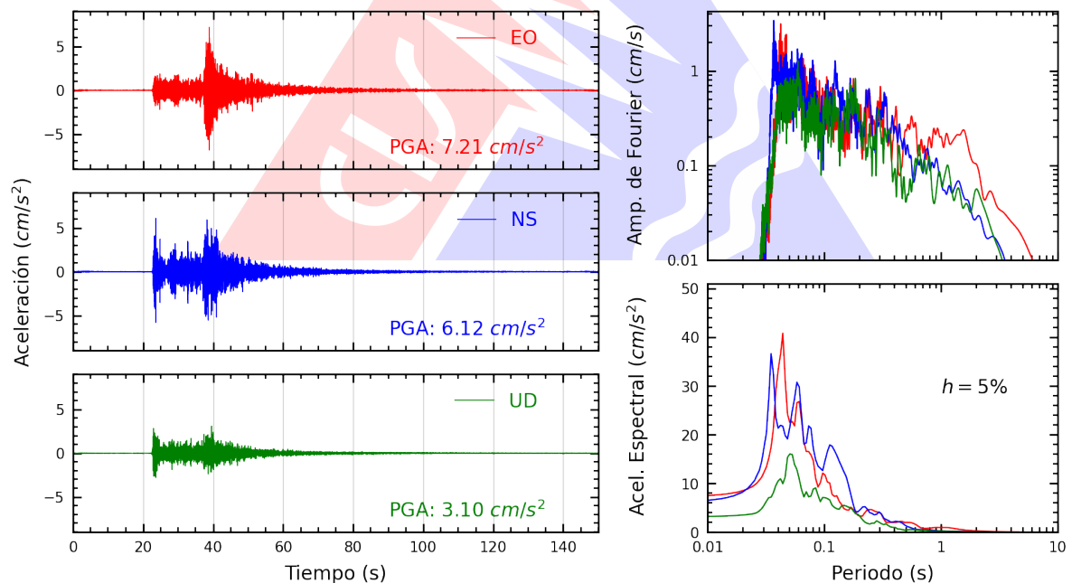
Figura A.2: Registros tiempo-historia, espectros de Fourier y de respuesta en las direcciones EO, NS y vertical de la estación UPTAC. Sismo de Calana, Tacna - Tacna del 2025-04-08, 05:28:41 (Hora local)
