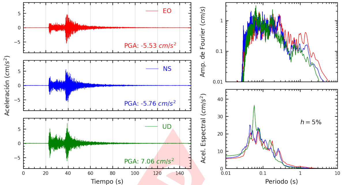
Figura A.3: Registros tiempo-historia, espectros de Fourier y de respuesta en las direcciones EO, NS y vertical de la estación UJBG4. Sismo de Calana, Tacna - Tacna del 2025-04-08, 05:28:41 (Hora local)
