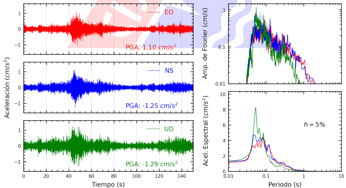
Figura A.6: Registros tiempo-historia, espectros de Fourier y de respuesta en las direcciones EO, NS y vertical de la estación SCAR2. Sismo de Calana, Tacna - Tacna del 2025-04-08, 05:28:41 (Hora local)
