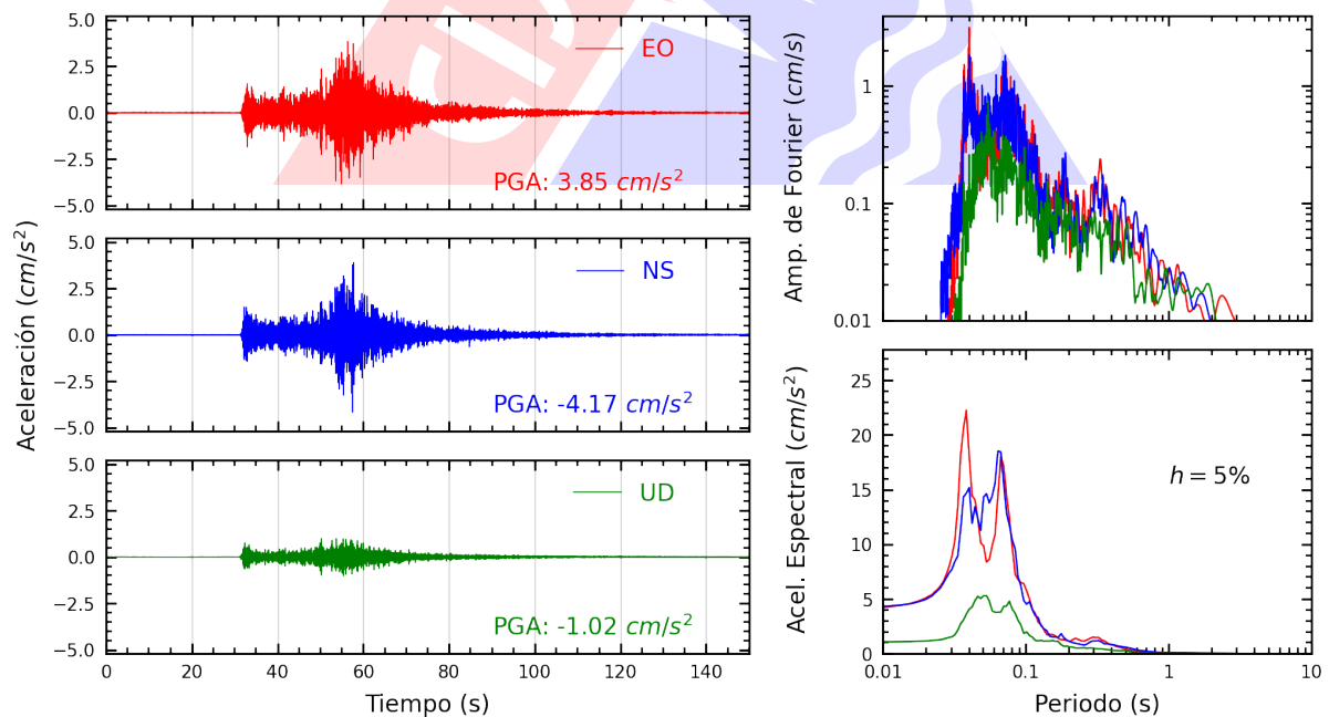
Figura A.4: Registros tiempo-historia, espectros de Fourier y de respuesta en las direcciones EO, NS y vertical de la estación UNAM. Sismo de Calana, Tacna - Tacna del 2025-04-08, 05:28:41 (Hora local)
