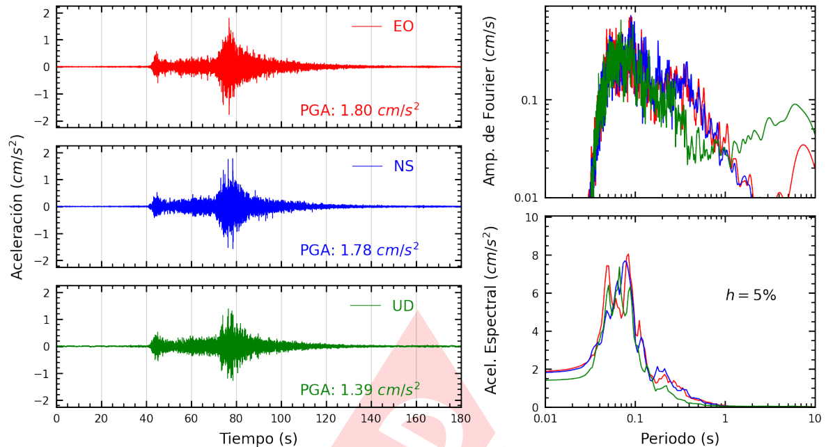
Figura A.5: Registros tiempo-historia, espectros de Fourier y de respuesta en las direcciones EO, NS y vertical de la estación SCARQ. Sismo de Calana, Tacna - Tacna del 2025-04-08, 05:28:41 (Hora local)
