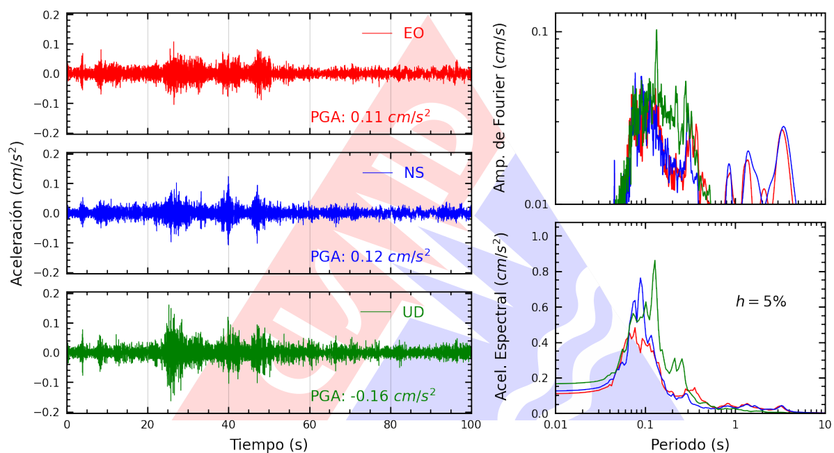
Figura A.7: Registros tiempo-historia, espectros de Fourier y de respuesta en las direcciones EO, NS y vertical de la estación UANCV. Sismo de Calana, Tacna - Tacna del 2025-04-08, 05:28:41 (Hora local)
