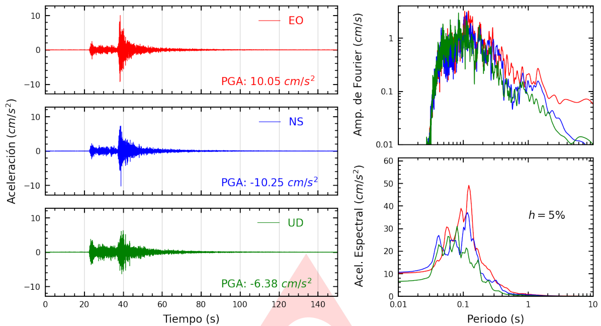
Figura A.1: Registros tiempo-historia, espectros de Fourier y de respuesta en las direcciones EO, NS y vertical de la estación UJBG3. Sismo de Calana, Tacna - Tacna del 2025-04-08, 05:28:41 (Hora local)
