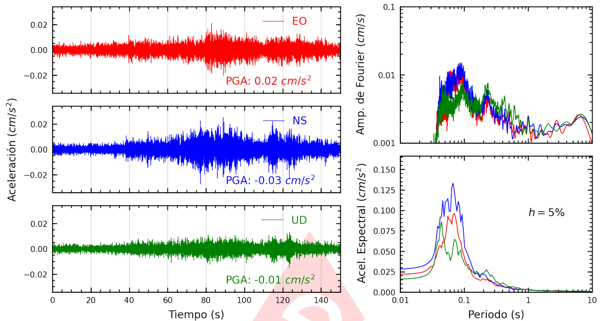
Figura A.9: Registros tiempo-historia, espectros de Fourier y de respuesta en las direcciones EO, NS y vertical de la estación UNF. Sismo de Bellavista, Bellavista - San Martín del 2025-04-08, 22:07:32 (Hora local)
