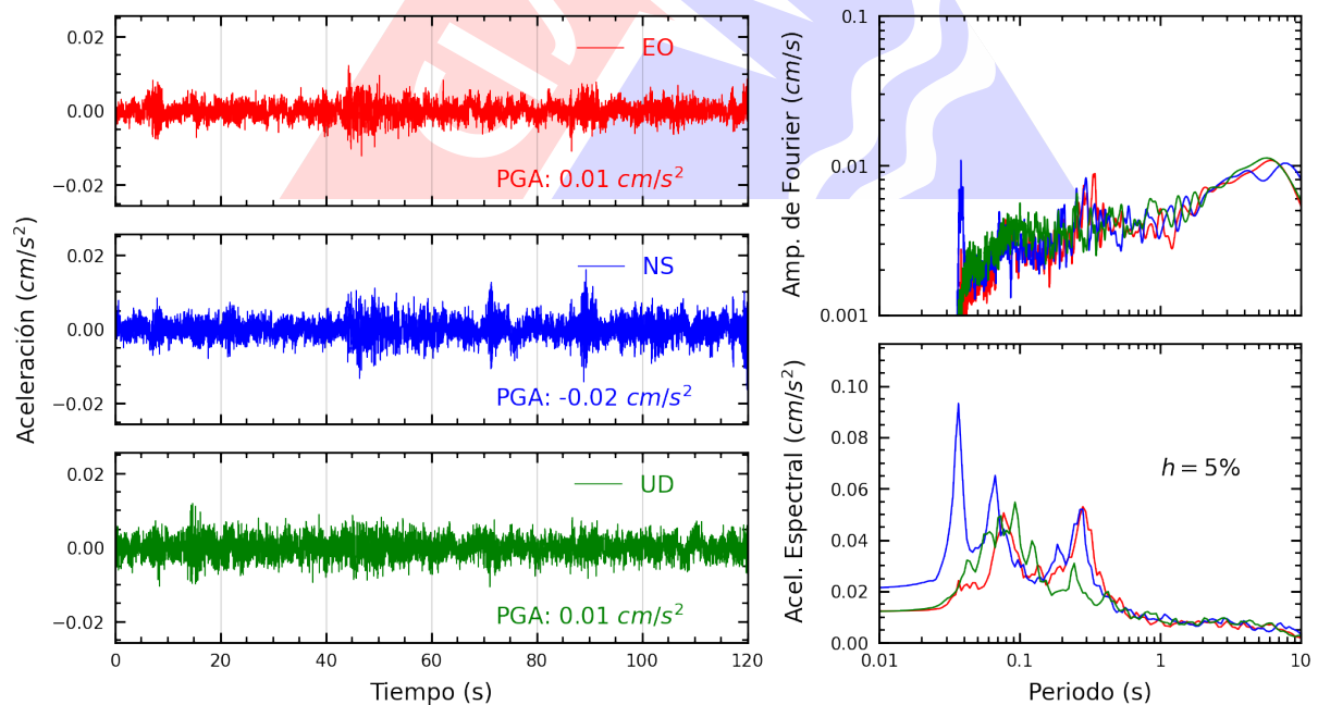
Figura A.10: Registros tiempo-historia, espectros de Fourier y de respuesta en las direcciones EO, NS y vertical de la estación UNJ. Sismo de Bellavista, Bellavista - San Martín del 2025-04-08, 22:07:32 (Hora local)
