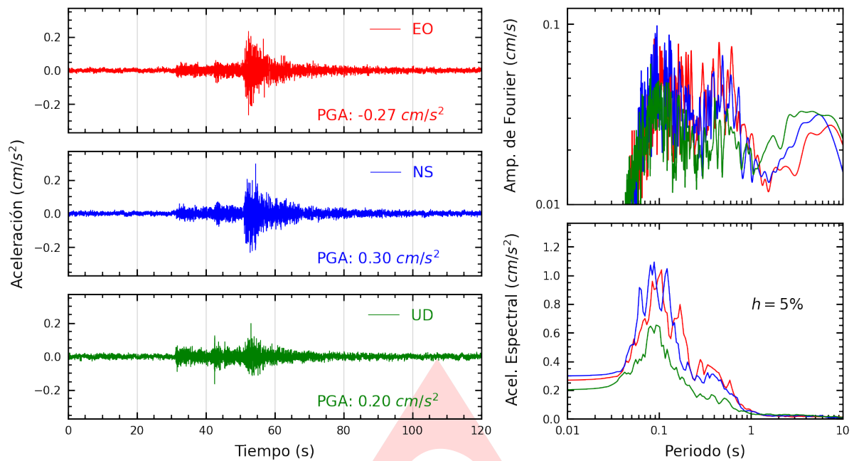
Figura A.1: Registros tiempo-historia, espectros de Fourier y de respuesta en las direcciones EO, NS y vertical de la estación UNTRM. Sismo de Bellavista, Bellavista - San Martín del 2025-04-08, 22:07:32 (Hora local)
