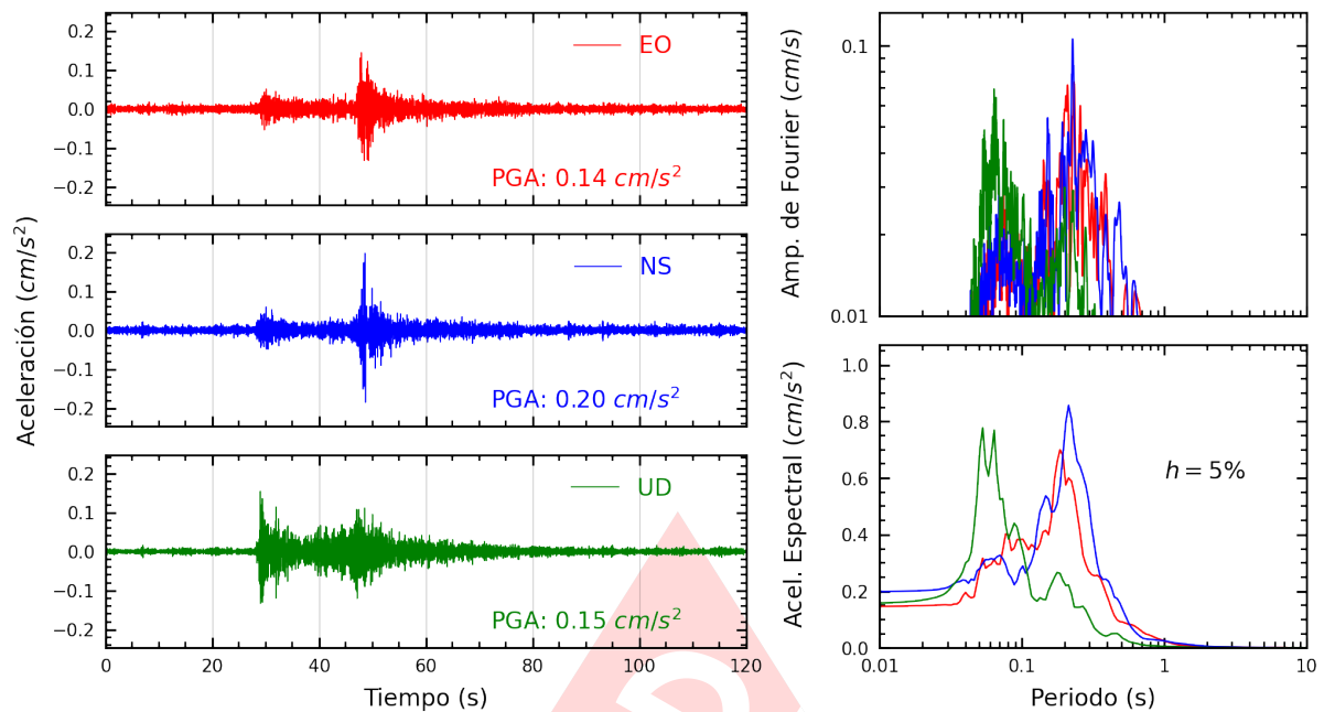
Figura A.3: Registros tiempo-historia, espectros de Fourier y de respuesta en las direcciones EO, NS y vertical de la estación UNAAA. Sismo de Bellavista, Bellavista - San Martín del 2025-04-08, 22:07:32 (Hora local)
