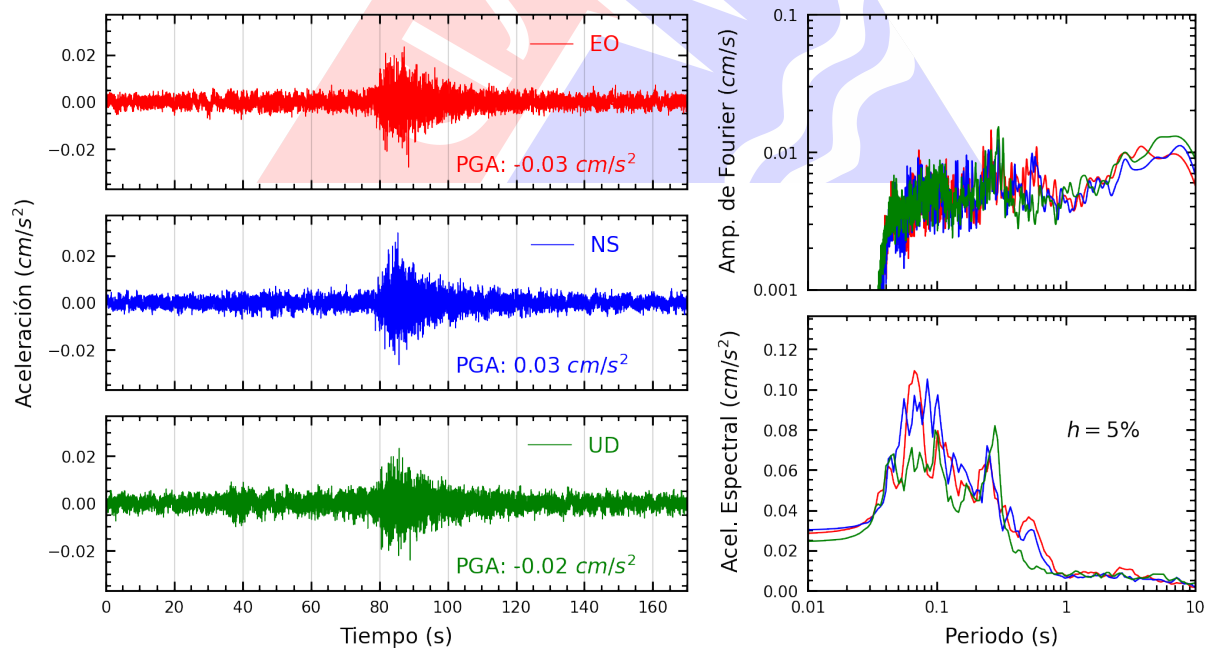
Figura A.8: Registros tiempo-historia, espectros de Fourier y de respuesta en las direcciones EO, NS y vertical de la estación CARAL. Sismo de Bellavista, Bellavista - San Martín del 2025-04-08, 22:07:32 (Hora local)
