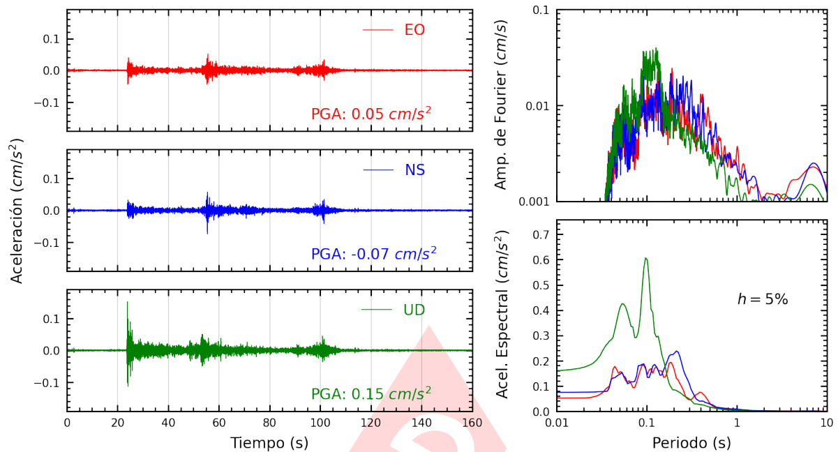
Figura A.5: Registros tiempo-historia, espectros de Fourier y de respuesta en las direcciones EO, NS y vertical de la estación UNIA. Sismo de Bellavista, Bellavista - San Martín del 2025-04-08, 22:07:32 (Hora local)
