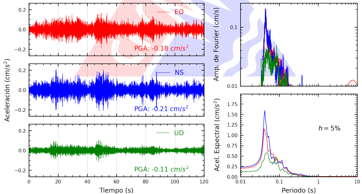
Figura A.2: Registros tiempo-historia, espectros de Fourier y de respuesta en las direcciones EO, NS y vertical de la estación SCTRU. Sismo de Bellavista, Bellavista - San Martín del 2025-04-08, 22:07:32 (Hora local)
