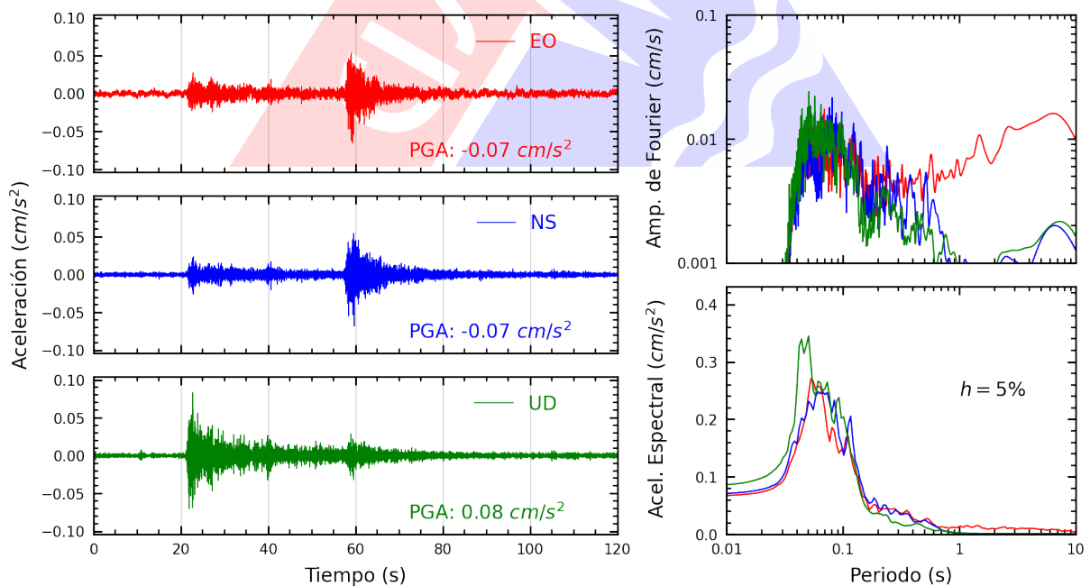
Figura A.6: Registros tiempo-historia, espectros de Fourier y de respuesta en las direcciones EO, NS y vertical de la estación SCCHI. Sismo de Bellavista, Bellavista - San Martín del 2025-04-08, 22:07:32 (Hora local)
