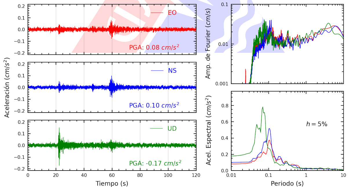
Figura A.4: Registros tiempo-historia, espectros de Fourier y de respuesta en las direcciones EO, NS y vertical de la estación UCVCH. Sismo de Bellavista, Bellavista - San Martín del 2025-04-08, 22:07:32 (Hora local)
