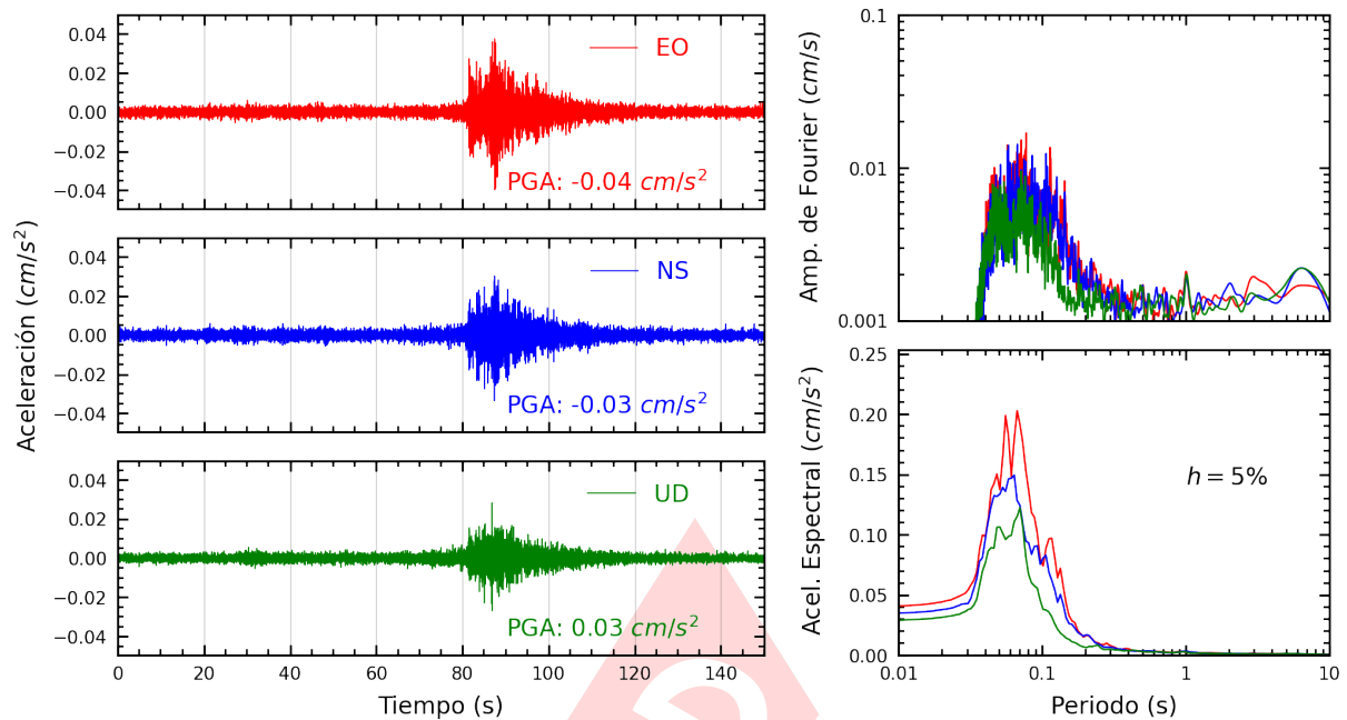
Figura A.7: Registros tiempo-historia, espectros de Fourier y de respuesta en las direcciones EO, NS y vertical de la estación ATARJ. Sismo de Bellavista, Bellavista - San Martín del 2025-04-08, 22:07:32 (Hora local)
