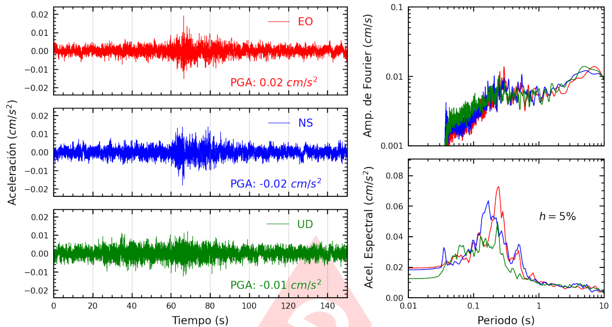
Figura A.9: Registros tiempo-historia, espectros de Fourier y de respuesta en las direcciones EO, NS y vertical de la estación UNJ. Sismo de Yurimaguas, Alto Amazonas - Loreto del 2025-04-10, 01:24:03 (Hora local)
