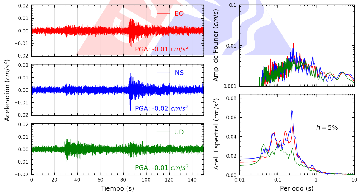
Figura A.10: Registros tiempo-historia, espectros de Fourier y de respuesta en las direcciones EO, NS y vertical de la estación UNF. Sismo de Yurimaguas, Alto Amazonas - Loreto del 2025-04-10, 01:24:03 (Hora local)
