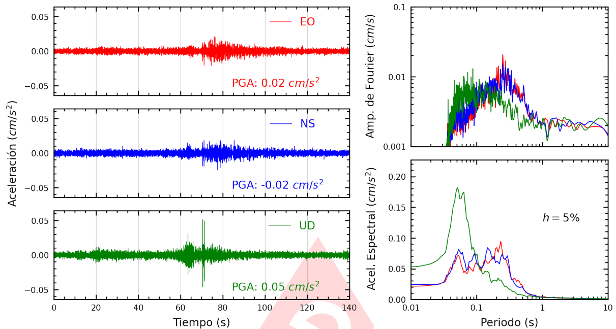
Figura A.7: Registros tiempo-historia, espectros de Fourier y de respuesta en las direcciones EO, NS y vertical de la estación UNP. Sismo de Yurimaguas, Alto Amazonas - Loreto del 2025-04-10, 01:24:03 (Hora local)
