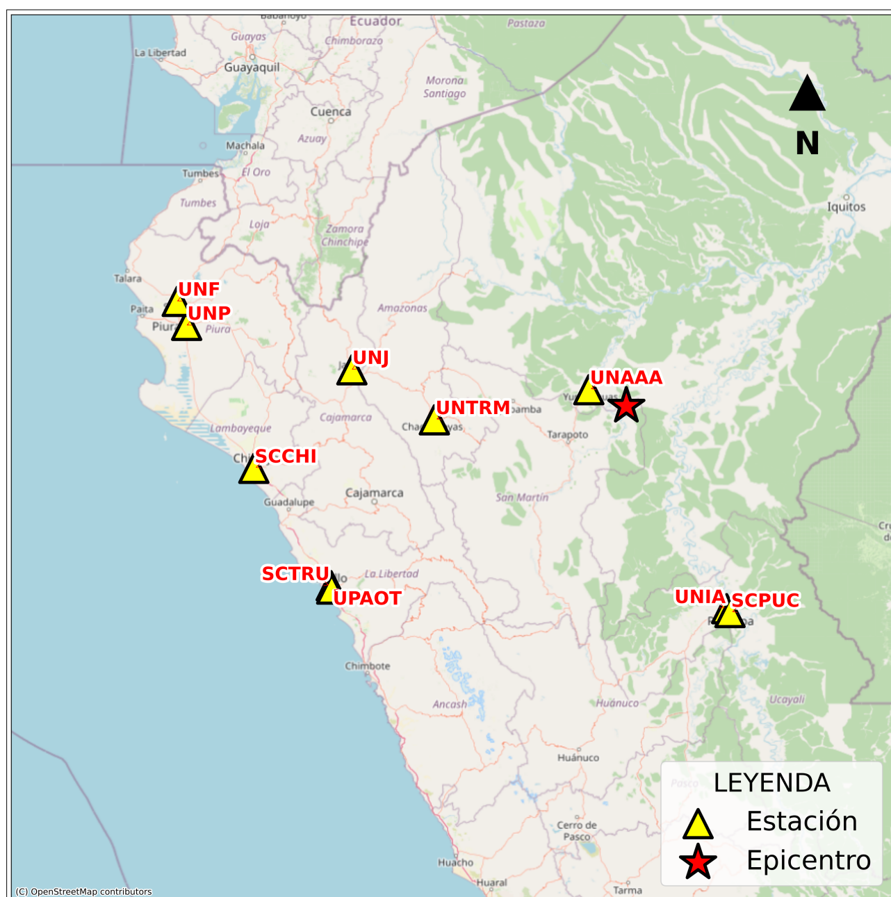
Figura 2: Mapa de ubicación de la(s) estación(es) acelerográfica(s) correspondiente(s) al Sismo de Yurimaguas, Alto Amazonas - Loreto del 10 de abril de 2025 a las 01:24:03 (hora local)
