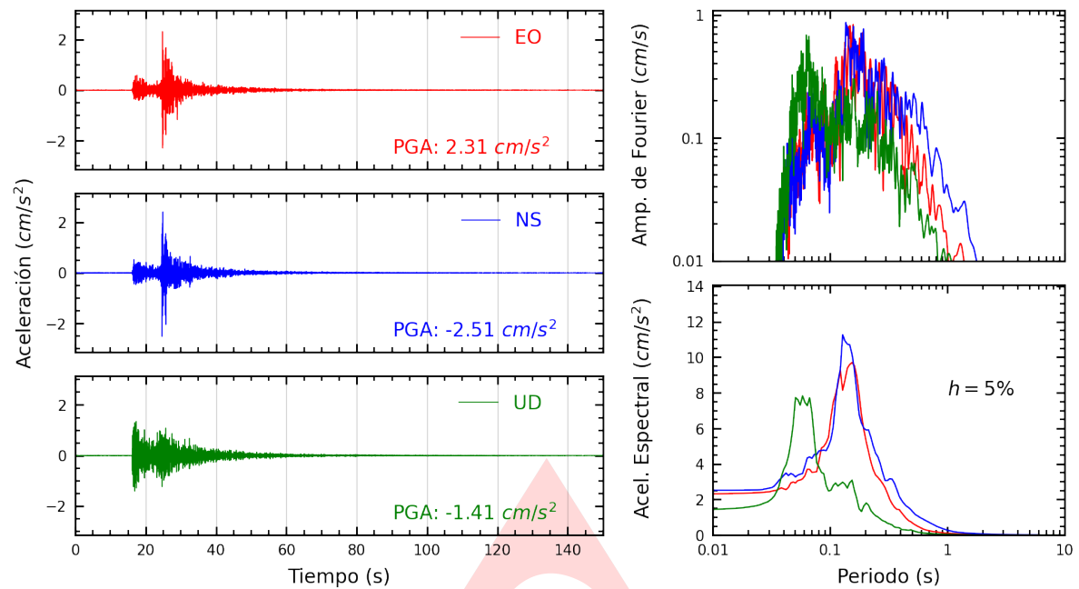
Figura A.1: Registros tiempo-historia, espectros de Fourier y de respuesta en las direcciones EO, NS y vertical de la estación UNAAA. Sismo de Yurimaguas, Alto Amazonas - Loreto del 2025-04-10, 01:24:03 (Hora local)
