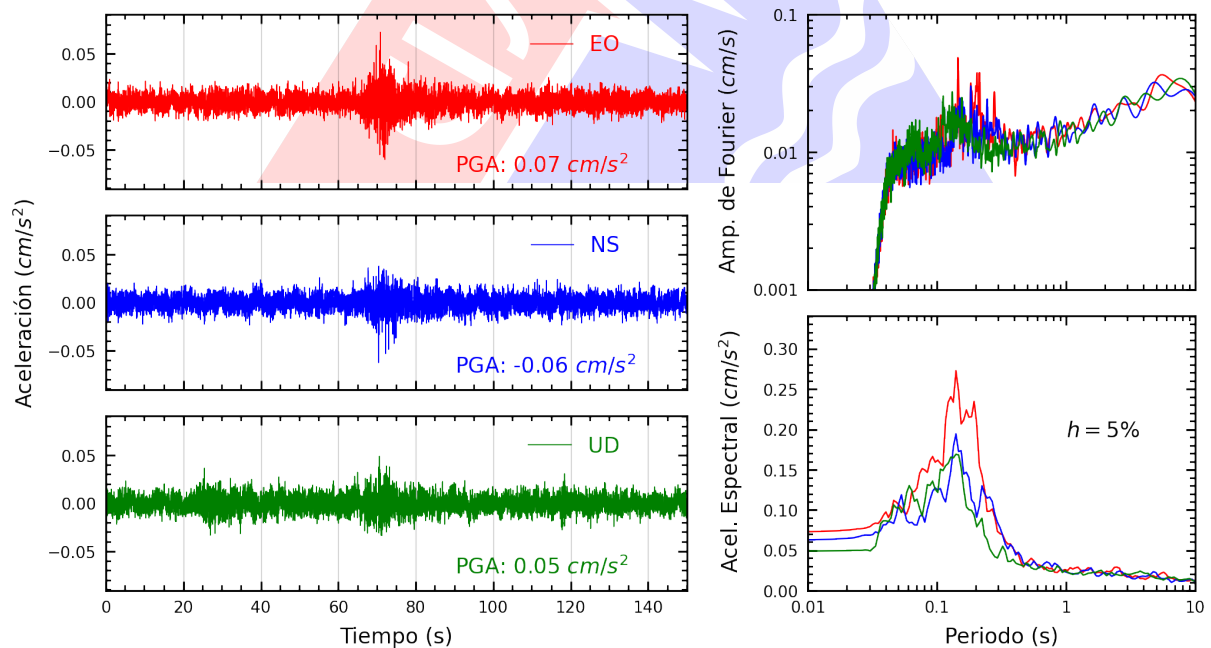
Figura A.6: Registros tiempo-historia, espectros de Fourier y de respuesta en las direcciones EO, NS y vertical de la estación UPAOT. Sismo de Yurimaguas, Alto Amazonas - Loreto del 2025-04-10, 01:24:03 (Hora local)
