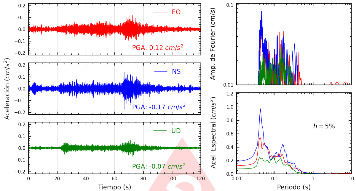
Figura A.3: Registros tiempo-historia, espectros de Fourier y de respuesta en las direcciones EO, NS y vertical de la estación SCTRU. Sismo de Yurimaguas, Alto Amazonas - Loreto del 2025-04-10, 01:24:03 (Hora local)
