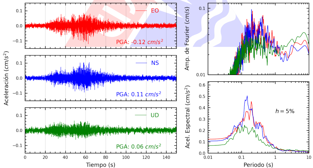
Figura A.4: Registros tiempo-historia, espectros de Fourier y de respuesta en las direcciones EO, NS y vertical de la estación UNTRM. Sismo de Yurimaguas, Alto Amazonas - Loreto del 2025-04-10, 01:24:03 (Hora local)
