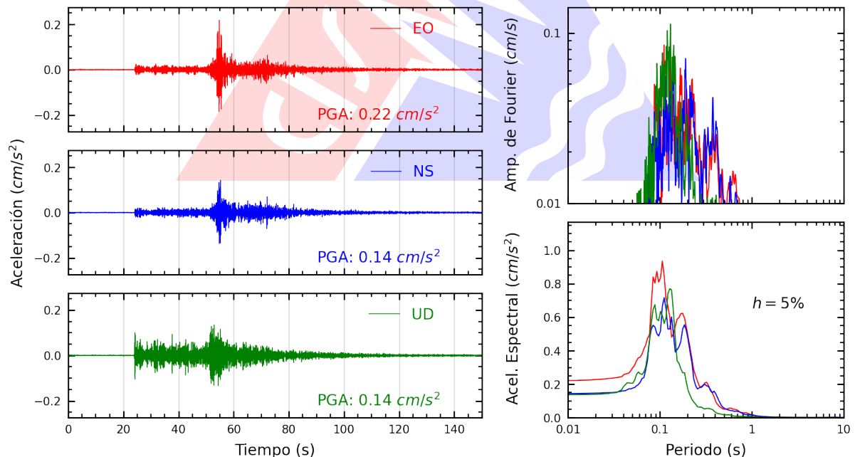
Figura A.2: Registros tiempo-historia, espectros de Fourier y de respuesta en las direcciones EO, NS y vertical de la estación UNIA. Sismo de Yurimaguas, Alto Amazonas - Loreto del 2025-04-10, 01:24:03 (Hora local)
