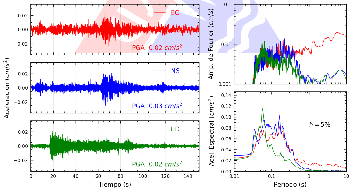
Figura A.8: Registros tiempo-historia, espectros de Fourier y de respuesta en las direcciones EO, NS y vertical de la estación SCCHI. Sismo de Yurimaguas, Alto Amazonas - Loreto del 2025-04-10, 01:24:03 (Hora local)
