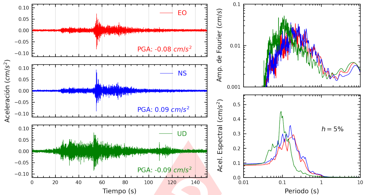
Figura A.5: Registros tiempo-historia, espectros de Fourier y de respuesta en las direcciones EO, NS y vertical de la estación SCPUC. Sismo de Yurimaguas, Alto Amazonas - Loreto del 2025-04-10, 01:24:03 (Hora local)
