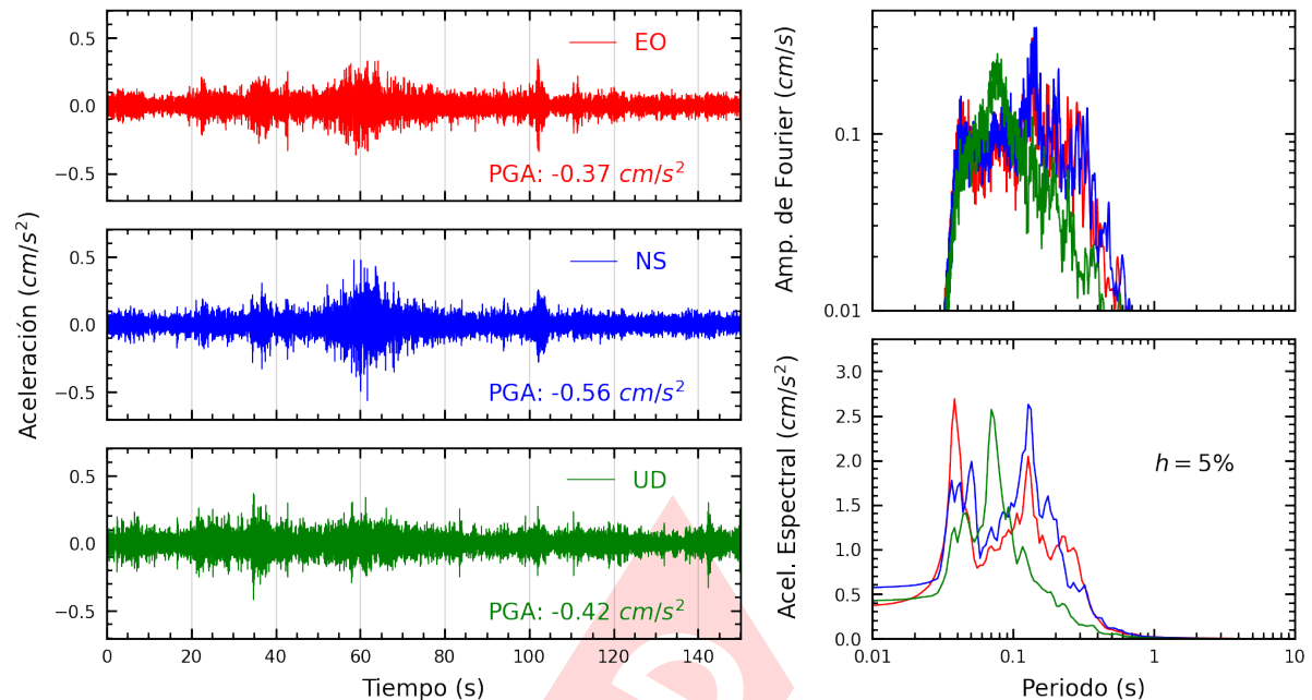
Figura A.5: Registros tiempo-historia, espectros de Fourier y de respuesta en las direcciones EO, NS y vertical de la estación CARA2. Sismo de Chuschi, Cangallo - Ayacucho del 2025-04-10, 12:13:14 (Hora local)
