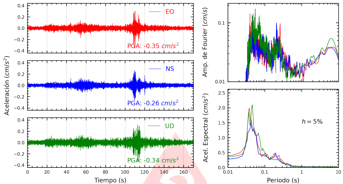
Figura A.13: Registros tiempo-historia, espectros de Fourier y de respuesta en las direcciones EO, NS y vertical de la estación USMP. Sismo de Chuschi, Cangallo - Ayacucho del 2025-04-10, 12:13:14 (Hora local)
