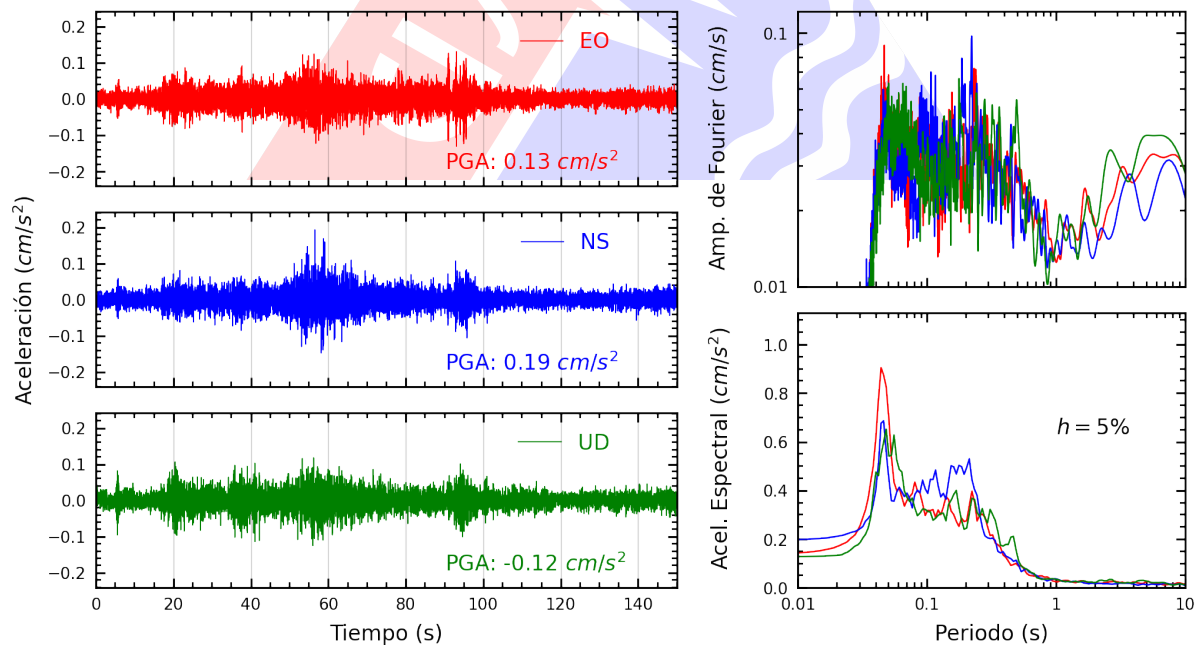
Figura A.20: Registros tiempo-historia, espectros de Fourier y de respuesta en las direcciones EO, NS y vertical de la estación IMCA. Sismo de Chuschi, Cangallo - Ayacucho del 2025-04-10, 12:13:14 (Hora local)
