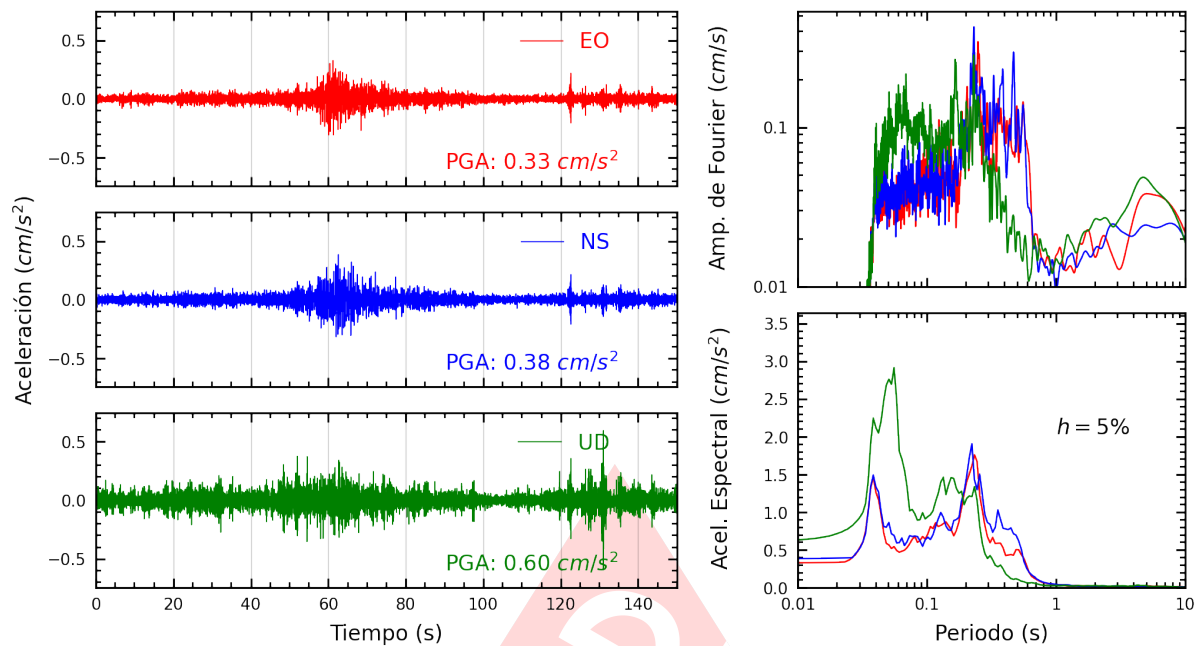
Figura A.3: Registros tiempo-historia, espectros de Fourier y de respuesta en las direcciones EO, NS y vertical de la estación MDPP. Sismo de Chuschi, Cangallo - Ayacucho del 2025-04-10, 12:13:14 (Hora local)
