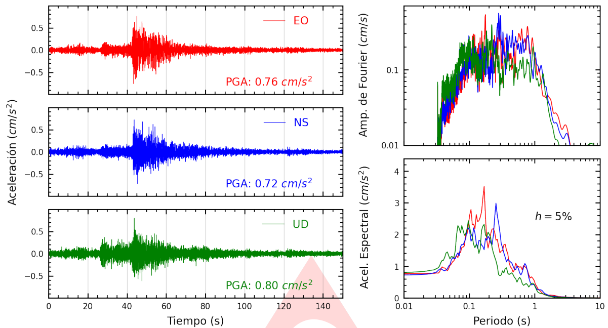
Figura A.1: Registros tiempo-historia, espectros de Fourier y de respuesta en las direcciones EO, NS y vertical de la estación UNICA. Sismo de Chuschi, Cangallo - Ayacucho del 2025-04-10, 12:13:14 (Hora local)
