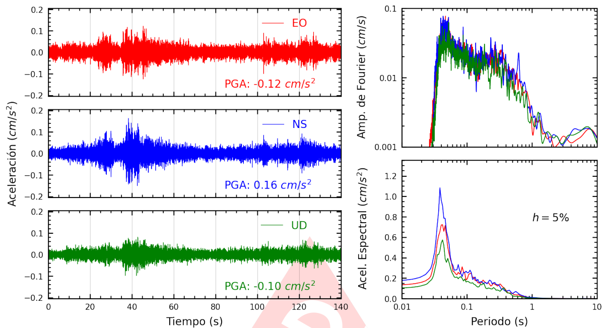
Figura A.23: Registros tiempo-historia, espectros de Fourier y de respuesta en las direcciones EO, NS y vertical de la estación BORJA. Sismo de Chuschi, Cangallo - Ayacucho del 2025-04-10, 12:13:14 (Hora local)
