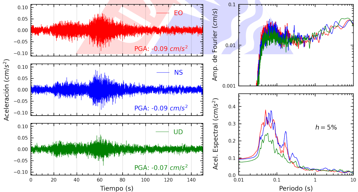
Figura A.28: Registros tiempo-historia, espectros de Fourier y de respuesta en las direcciones EO, NS y vertical de la estación UCSS. Sismo de Chuschi, Cangallo - Ayacucho del 2025-04-10, 12:13:14 (Hora local)
