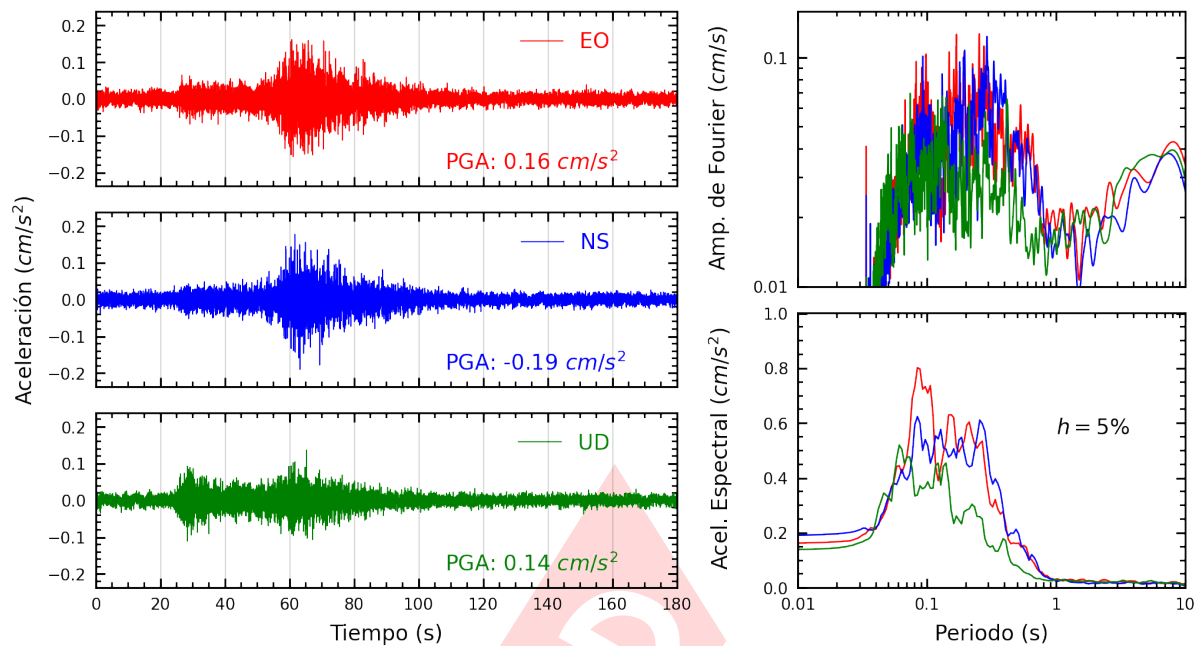
Figura A.21: Registros tiempo-historia, espectros de Fourier y de respuesta en las direcciones EO, NS y vertical de la estación USILP. Sismo de Chuschi, Cangallo - Ayacucho del 2025-04-10, 12:13:14 (Hora local)
