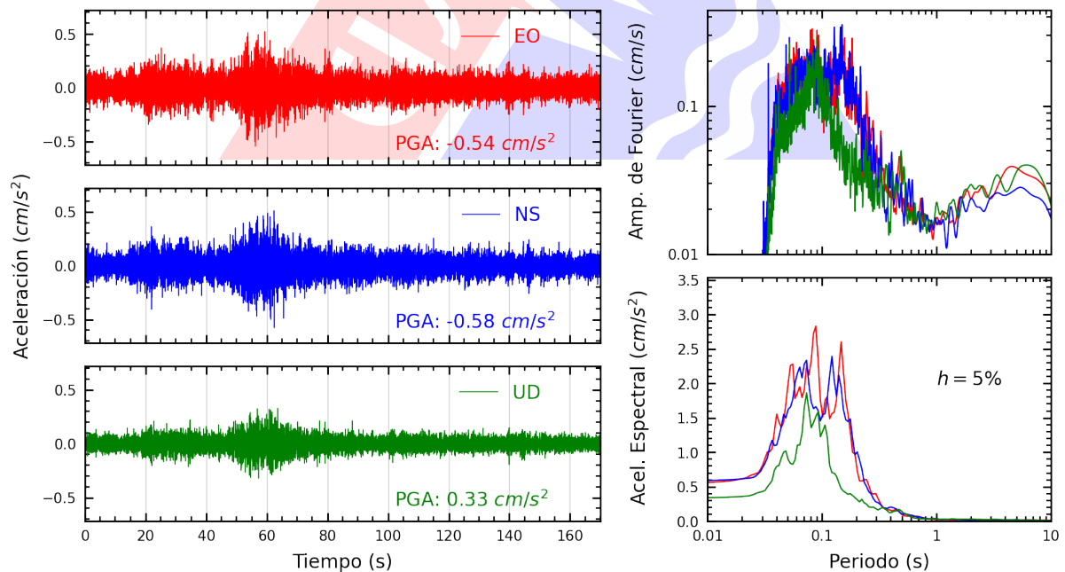
Figura A.4: Registros tiempo-historia, espectros de Fourier y de respuesta en las direcciones EO, NS y vertical de la estación USILM. Sismo de Chuschi, Cangallo - Ayacucho del 2025-04-10, 12:13:14 (Hora local)
