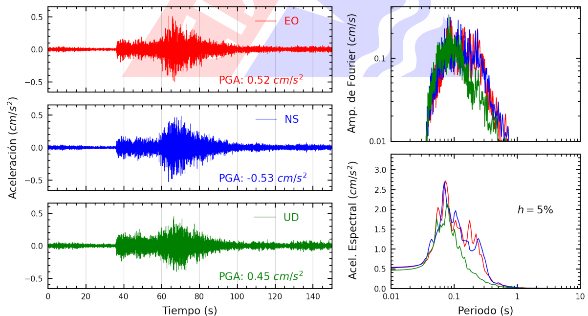
Figura A.6: Registros tiempo-historia, espectros de Fourier y de respuesta en las direcciones EO, NS y vertical de la estación ASIA. Sismo de Chuschi, Cangallo - Ayacucho del 2025-04-10, 12:13:14 (Hora local)
