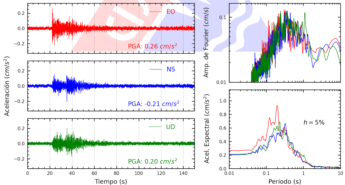
Figura A.18: Registros tiempo-historia, espectros de Fourier y de respuesta en las direcciones EO, NS y vertical de la estación UNSCH. Sismo de Chuschi, Cangallo - Ayacucho del 2025-04-10, 12:13:14 (Hora local)
