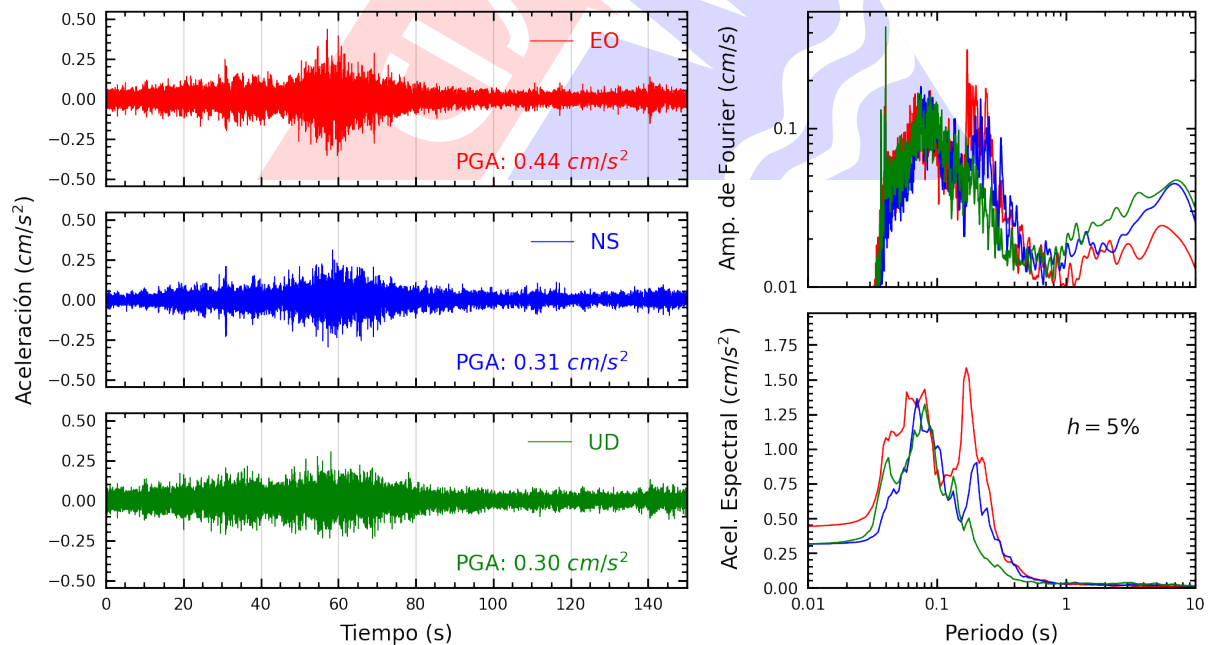
Figura A.10: Registros tiempo-historia, espectros de Fourier y de respuesta en las direcciones EO, NS y vertical de la estación INDEP. Sismo de Chuschi, Cangallo - Ayacucho del 2025-04-10, 12:13:14 (Hora local)
