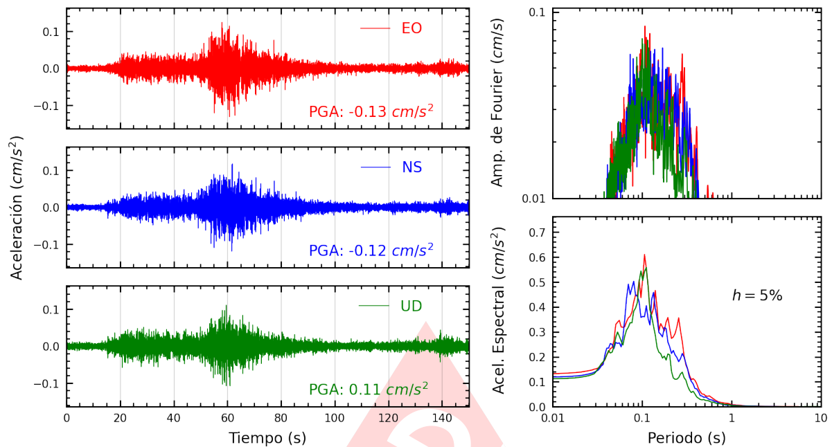
Figura A.27: Registros tiempo-historia, espectros de Fourier y de respuesta en las direcciones EO, NS y vertical de la estación JALV2. Sismo de Chuschi, Cangallo - Ayacucho del 2025-04-10, 12:13:14 (Hora local)
