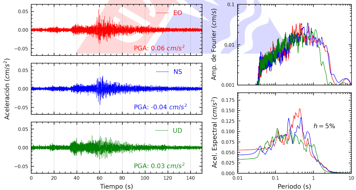
Figura A.30: Registros tiempo-historia, espectros de Fourier y de respuesta en las direcciones EO, NS y vertical de la estación UNCP. Sismo de Chuschi, Cangallo - Ayacucho del 2025-04-10, 12:13:14 (Hora local)
