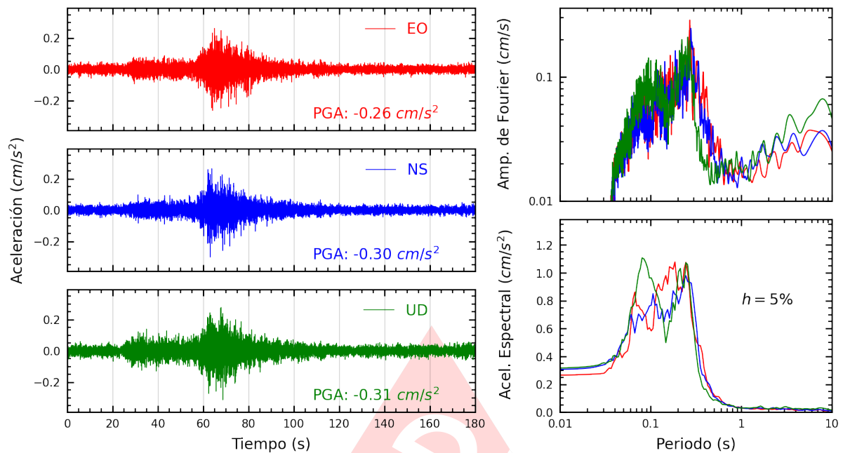
Figura A.15: Registros tiempo-historia, espectros de Fourier y de respuesta en las direcciones EO, NS y vertical de la estación SOVES. Sismo de Chuschi, Cangallo - Ayacucho del 2025-04-10, 12:13:14 (Hora local)
