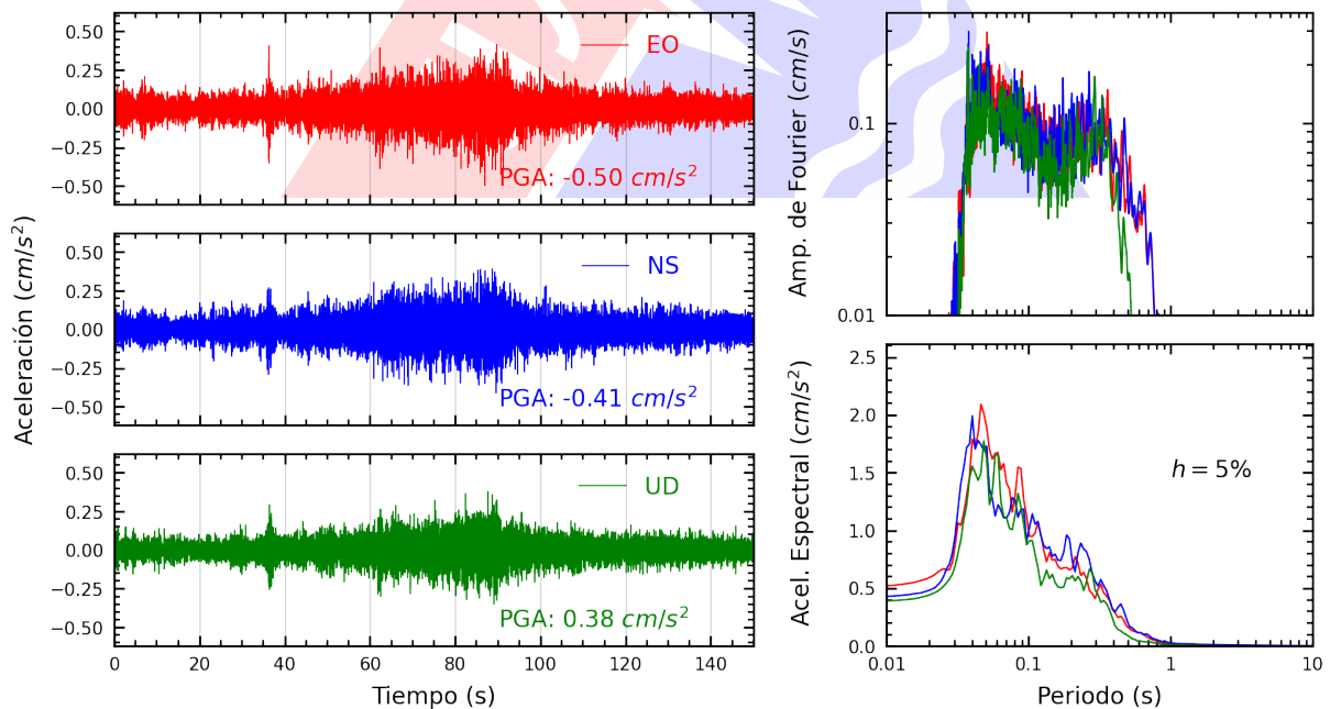
Figura A.8: Registros tiempo-historia, espectros de Fourier y de respuesta en las direcciones EO, NS y vertical de la estación UNTEL. Sismo de Chuschi, Cangallo - Ayacucho del 2025-04-10, 12:13:14 (Hora local)
