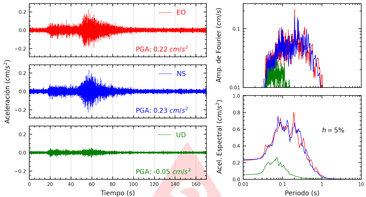
Figura A.19: Registros tiempo-historia, espectros de Fourier y de respuesta en las direcciones EO, NS y vertical de la estación UCVA2. Sismo de Chuschi, Cangallo - Ayacucho del 2025-04-10, 12:13:14 (Hora local)
