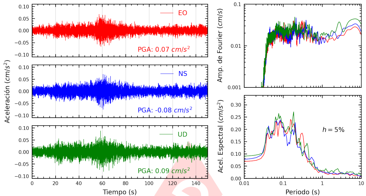
Figura A.29: Registros tiempo-historia, espectros de Fourier y de respuesta en las direcciones EO, NS y vertical de la estación UNFV. Sismo de Chuschi, Cangallo - Ayacucho del 2025-04-10, 12:13:14 (Hora local)
