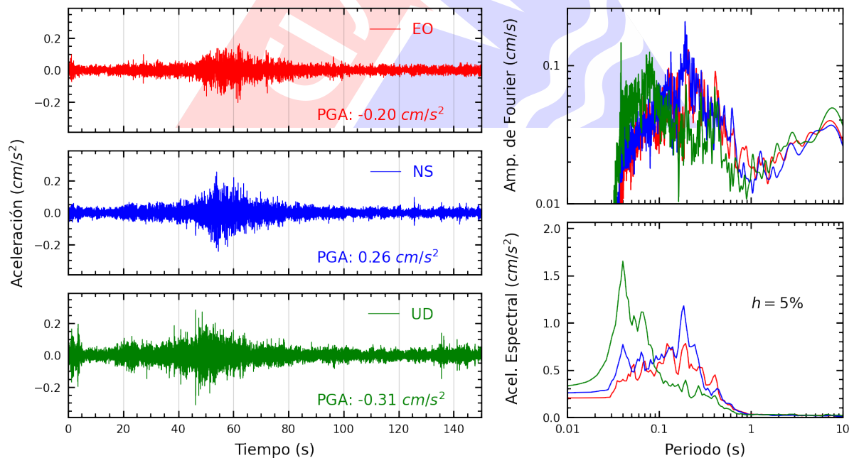
Figura A.16: Registros tiempo-historia, espectros de Fourier y de respuesta en las direcciones EO, NS y vertical de la estación SOCHO. Sismo de Chuschi, Cangallo - Ayacucho del 2025-04-10, 12:13:14 (Hora local)
