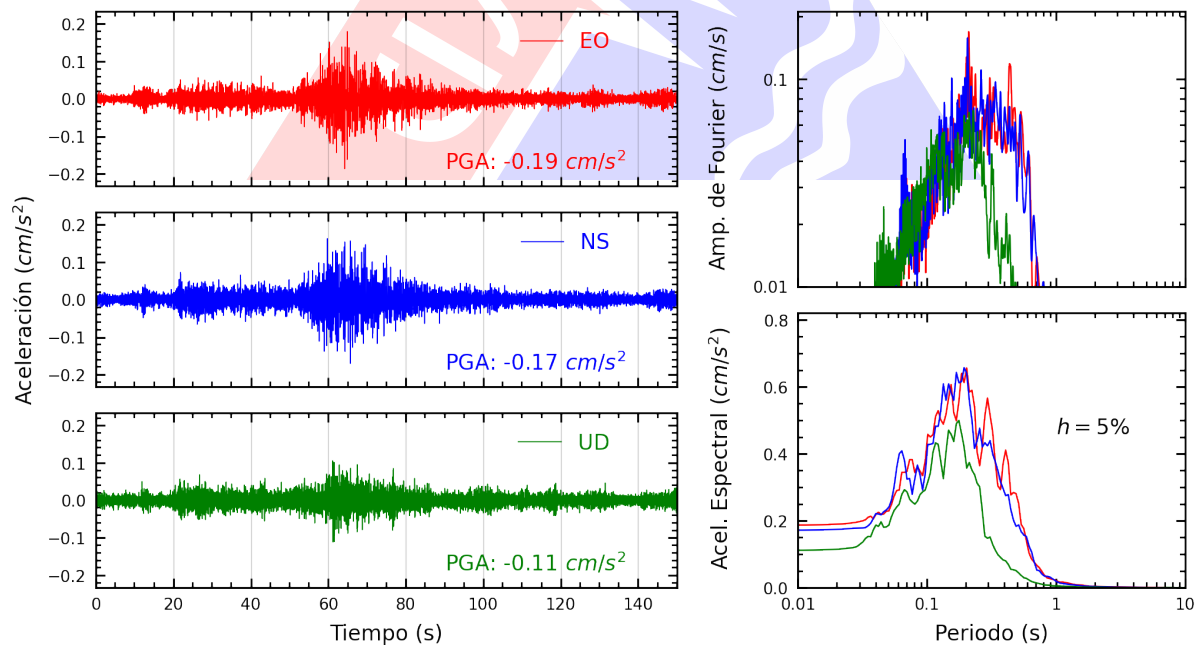
Figura A.22: Registros tiempo-historia, espectros de Fourier y de respuesta en las direcciones EO, NS y vertical de la estación VHAY2. Sismo de Chuschi, Cangallo - Ayacucho del 2025-04-10, 12:13:14 (Hora local)
