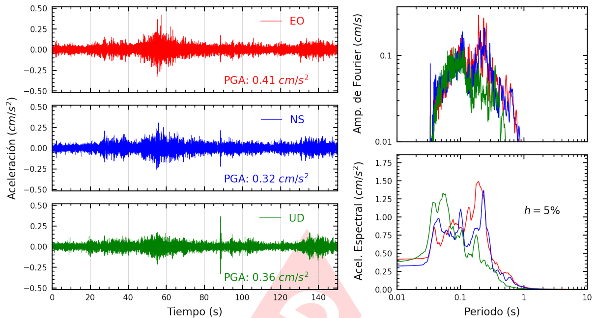
Figura A.11: Registros tiempo-historia, espectros de Fourier y de respuesta en las direcciones EO, NS y vertical de la estación SCCHO. Sismo de Chuschi, Cangallo - Ayacucho del 2025-04-10, 12:13:14 (Hora local)
