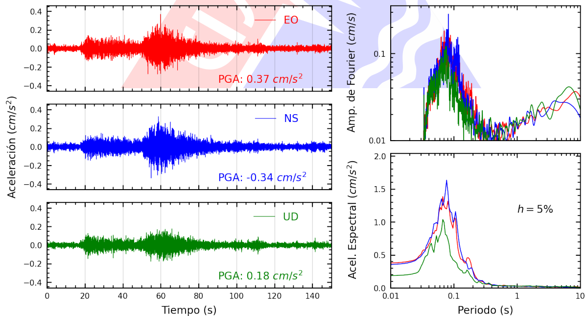
Figura A.12: Registros tiempo-historia, espectros de Fourier y de respuesta en las direcciones EO, NS y vertical de la estación JOSEO. Sismo de Chuschi, Cangallo - Ayacucho del 2025-04-10, 12:13:14 (Hora local)
