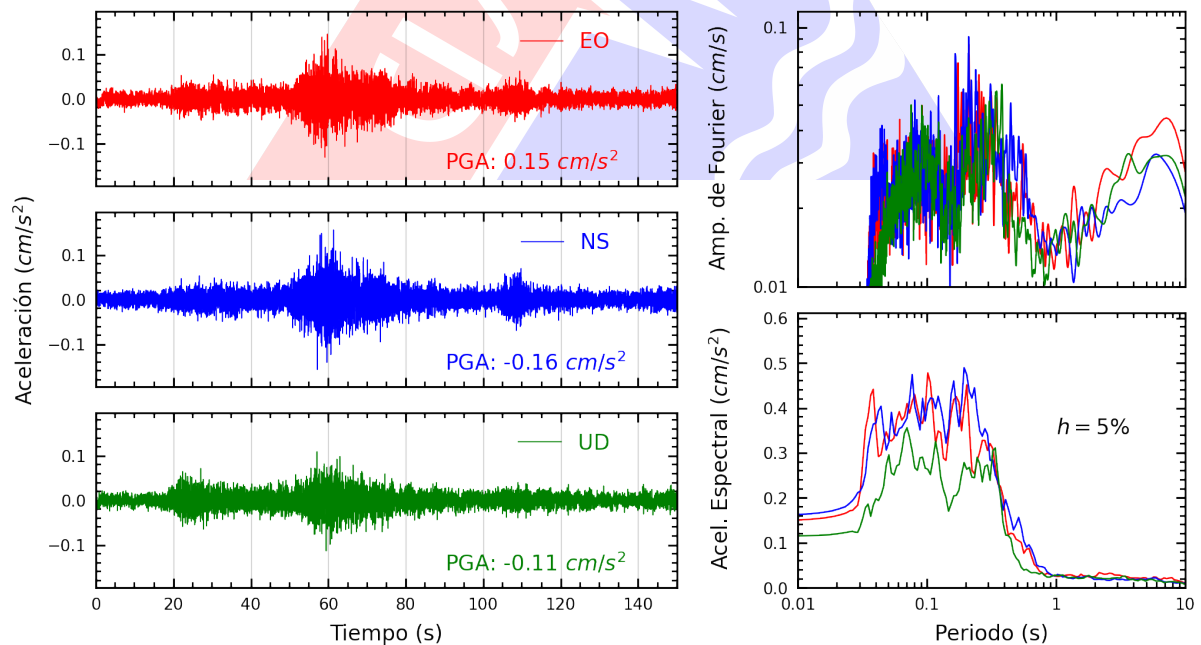
Figura A.24: Registros tiempo-historia, espectros de Fourier y de respuesta en las direcciones EO, NS y vertical de la estación COMAS. Sismo de Chuschi, Cangallo - Ayacucho del 2025-04-10, 12:13:14 (Hora local)
