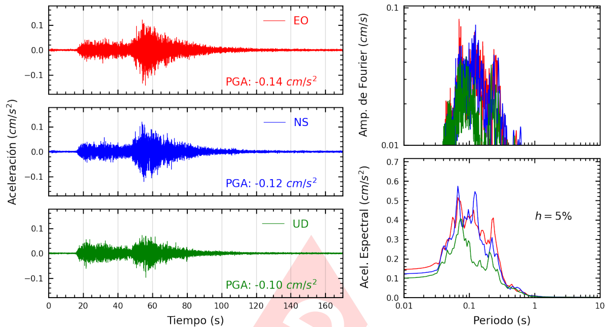
Figura A.25: Registros tiempo-historia, espectros de Fourier y de respuesta en las direcciones EO, NS y vertical de la estación ATARJ. Sismo de Chuschi, Cangallo - Ayacucho del 2025-04-10, 12:13:14 (Hora local)
