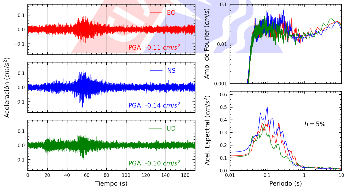
Figura A.26: Registros tiempo-historia, espectros de Fourier y de respuesta en las direcciones EO, NS y vertical de la estación SERVI. Sismo de Chuschi, Cangallo - Ayacucho del 2025-04-10, 12:13:14 (Hora local)
