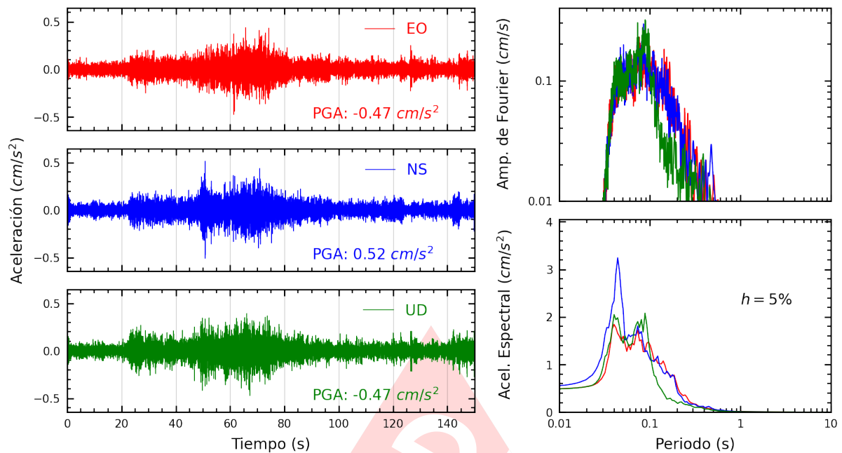
Figura A.7: Registros tiempo-historia, espectros de Fourier y de respuesta en las direcciones EO, NS y vertical de la estación SROS2. Sismo de Chuschi, Cangallo - Ayacucho del 2025-04-10, 12:13:14 (Hora local)
