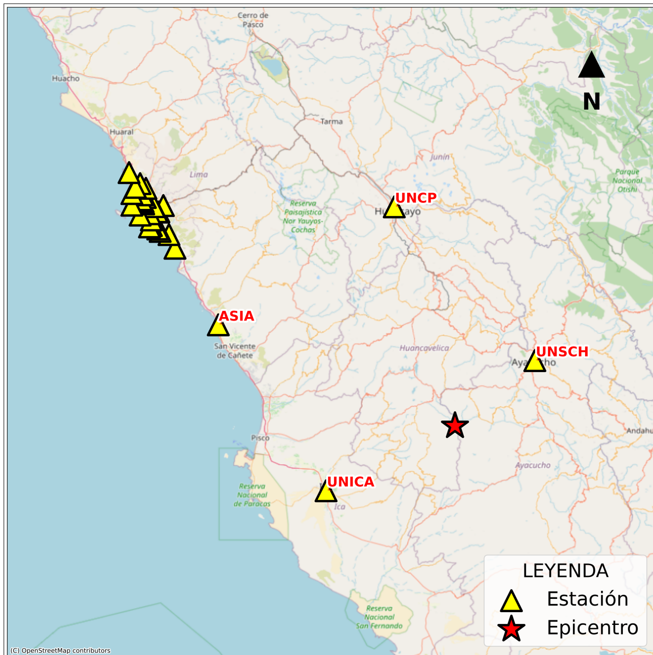
Figura 2: Mapa de ubicación de la(s) estación(es) acelerográfica(s) a nivel nacional correspondiente(s) al Sismo de Chuschi, Cangallo - Ayacucho del 10 de abril de 2025 a las 12:13:14 (hora local)
