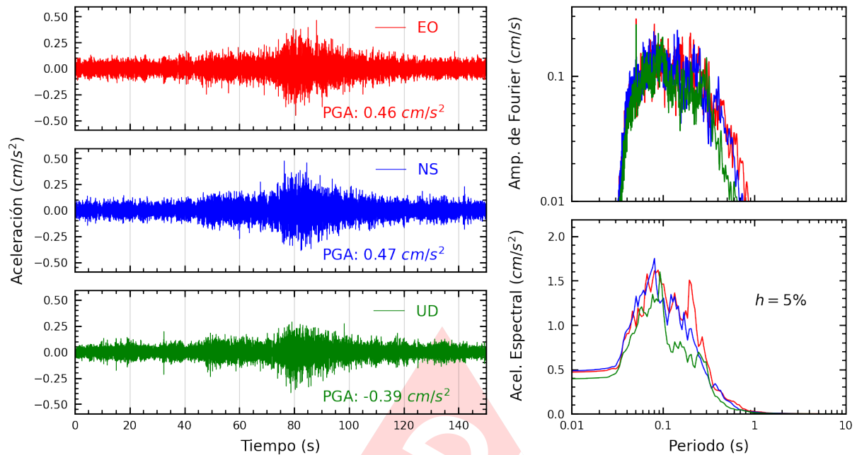
Figura A.9: Registros tiempo-historia, espectros de Fourier y de respuesta en las direcciones EO, NS y vertical de la estación PHER2. Sismo de Chuschi, Cangallo - Ayacucho del 2025-04-10, 12:13:14 (Hora local)
