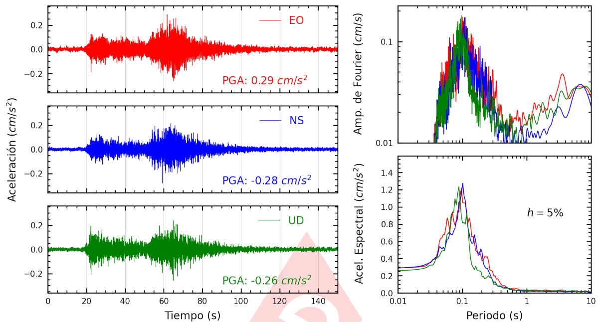
Figura A.17: Registros tiempo-historia, espectros de Fourier y de respuesta en las direcciones EO, NS y vertical de la estación AMORE. Sismo de Chuschi, Cangallo - Ayacucho del 2025-04-10, 12:13:14 (Hora local)
