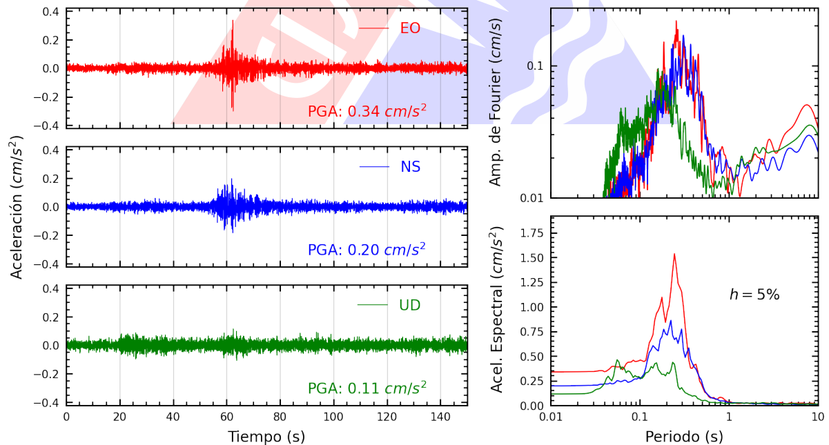
Figura A.14: Registros tiempo-historia, espectros de Fourier y de respuesta en las direcciones EO, NS y vertical de la estación ACAPU. Sismo de Chuschi, Cangallo - Ayacucho del 2025-04-10, 12:13:14 (Hora local)
