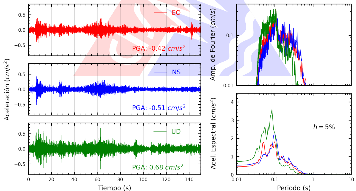
Figura A.2: Registros tiempo-historia, espectros de Fourier y de respuesta en las direcciones EO, NS y vertical de la estación SCOLI. Sismo de Chuschi, Cangallo - Ayacucho del 2025-04-10, 12:13:14 (Hora local)
