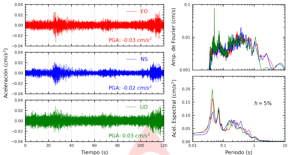
Figura A.1: Registros tiempo-historia, espectros de Fourier y de respuesta en las direcciones EO, NS y vertical de la estación UNCP. Sismo de Oxapampa, Oxapampa - Pasco del 2025-04-10, 14:20:28 (Hora local)
