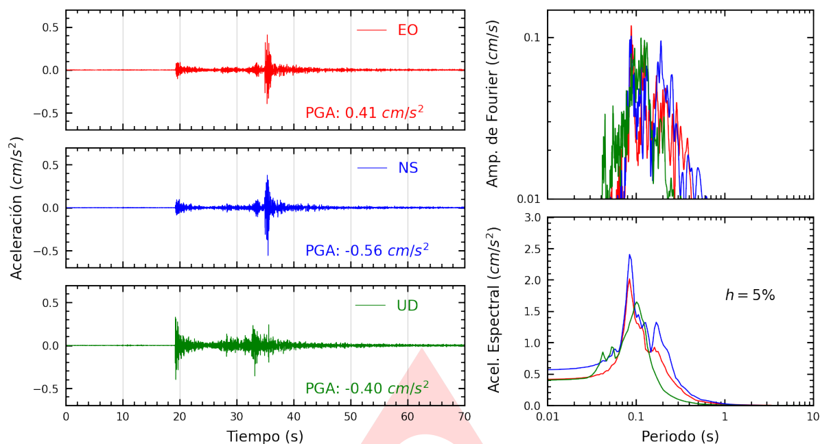
Figura A.1: Registros tiempo-historia, espectros de Fourier y de respuesta en las direcciones EO, NS y vertical de la estación UNIA. Sismo de Curimana, Padre Abad - Ucayali del 2025-04-12, 20:58:59 (Hora local)
