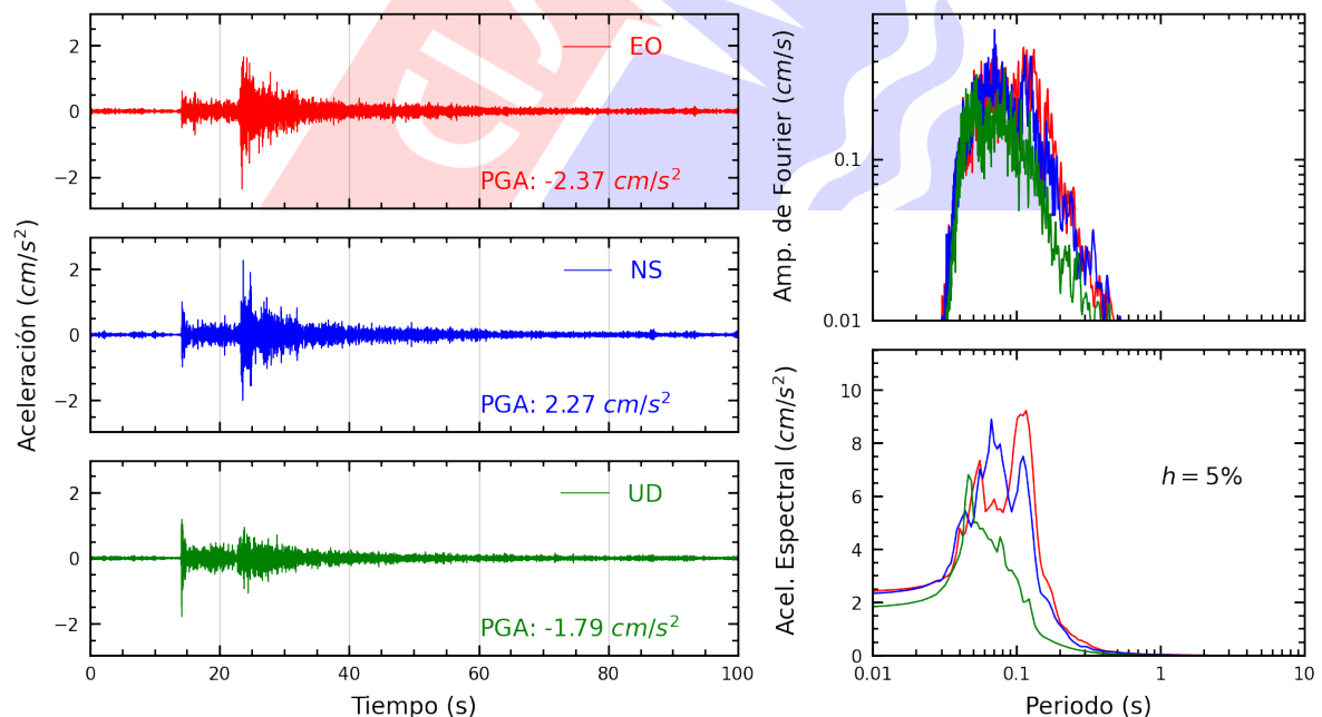
Figura A.10: Registros tiempo-historia, espectros de Fourier y de respuesta en las direcciones EO, NS y vertical de la estación PACHA. Sismo de Mala, Cañete - Lima del 2025-04-12, 22:47:00 (Hora local)
