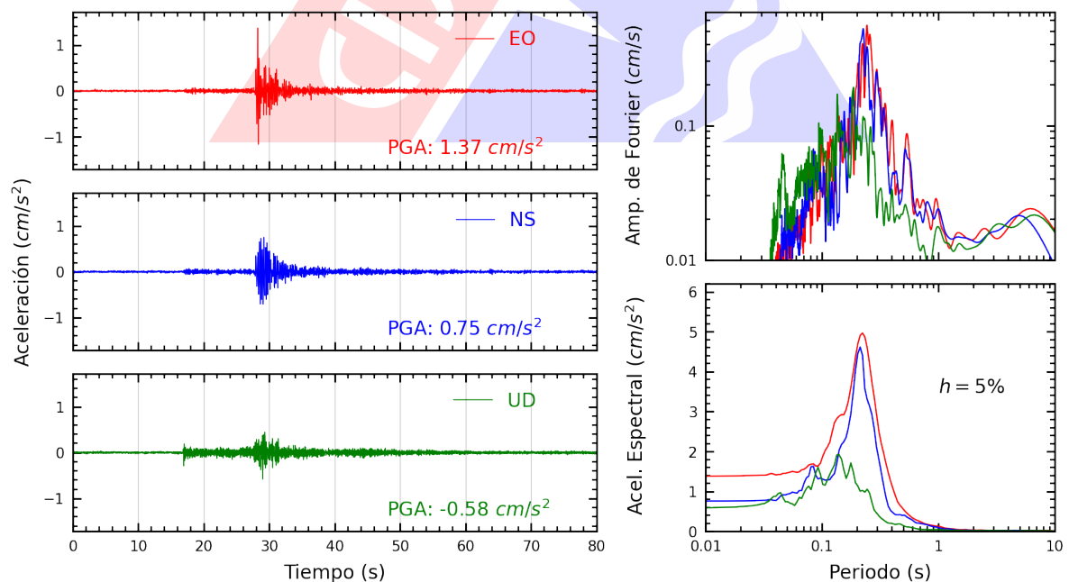
Figura A.22: Registros tiempo-historia, espectros de Fourier y de respuesta en las direcciones EO, NS y vertical de la estación DSMI. Sismo de Mala, Cañete - Lima del 2025-04-12, 22:47:00 (Hora local)
