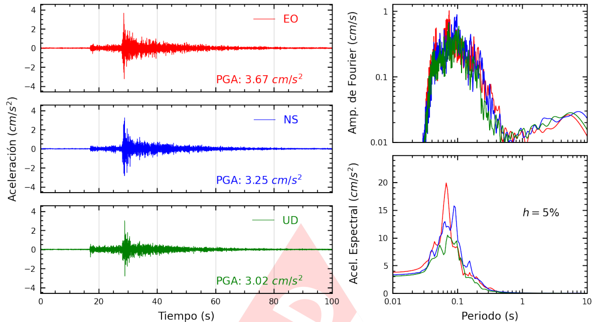
Figura A.3: Registros tiempo-historia, espectros de Fourier y de respuesta en las direcciones EO, NS y vertical de la estación INDEP. Sismo de Mala, Cañete - Lima del 2025-04-12, 22:47:00 (Hora local)
