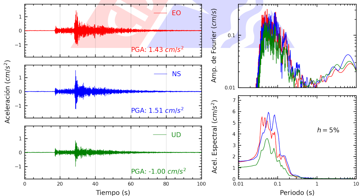
Figura A.20: Registros tiempo-historia, espectros de Fourier y de respuesta en las direcciones EO, NS y vertical de la estación UCSS. Sismo de Mala, Cañete - Lima del 2025-04-12, 22:47:00 (Hora local)
