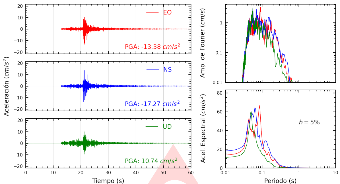
Figura A.1: Registros tiempo-historia, espectros de Fourier y de respuesta en las direcciones EO, NS y vertical de la estación ASIA. Sismo de Mala, Cañete - Lima del 2025-04-12, 22:47:00 (Hora local)
