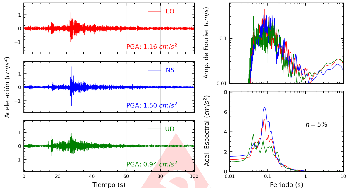
Figura A.21: Registros tiempo-historia, espectros de Fourier y de respuesta en las direcciones EO, NS y vertical de la estación UPCSM. Sismo de Mala, Cañete - Lima del 2025-04-12, 22:47:00 (Hora local)
