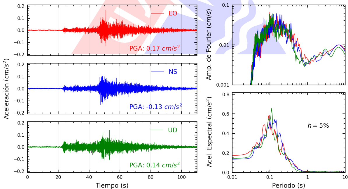
Figura A.34: Registros tiempo-historia, espectros de Fourier y de respuesta en las direcciones EO, NS y vertical de la estación CARAL. Sismo de Mala, Cañete - Lima del 2025-04-12, 22:47:00 (Hora local)
