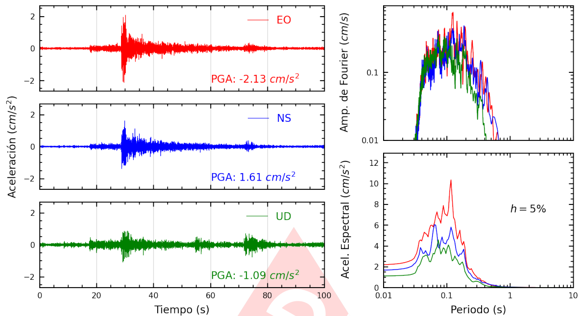
Figura A.11: Registros tiempo-historia, espectros de Fourier y de respuesta en las direcciones EO, NS y vertical de la estación SCOLI. Sismo de Mala, Cañete - Lima del 2025-04-12, 22:47:00 (Hora local)
