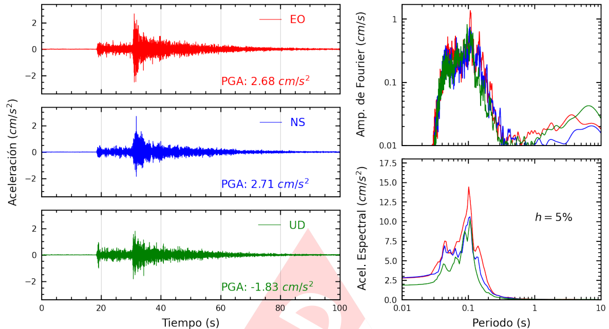
Figura A.7: Registros tiempo-historia, espectros de Fourier y de respuesta en las direcciones EO, NS y vertical de la estación AMORE. Sismo de Mala, Cañete - Lima del 2025-04-12, 22:47:00 (Hora local)
