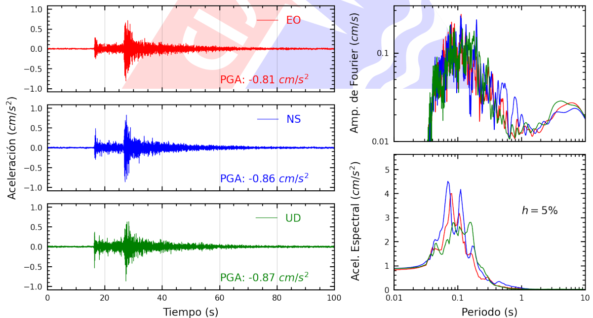
Figura A.26: Registros tiempo-historia, espectros de Fourier y de respuesta en las direcciones EO, NS y vertical de la estación UNFV. Sismo de Mala, Cañete - Lima del 2025-04-12, 22:47:00 (Hora local)
