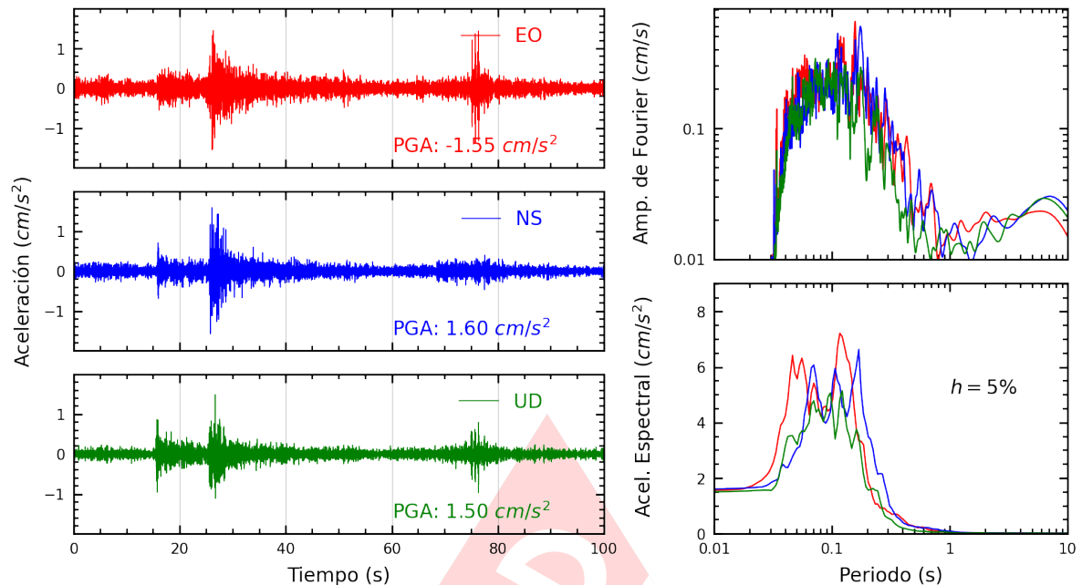
Figura A.19: Registros tiempo-historia, espectros de Fourier y de respuesta en las direcciones EO, NS y vertical de la estación SOBAR. Sismo de Mala, Cañete - Lima del 2025-04-12, 22:47:00 (Hora local)
