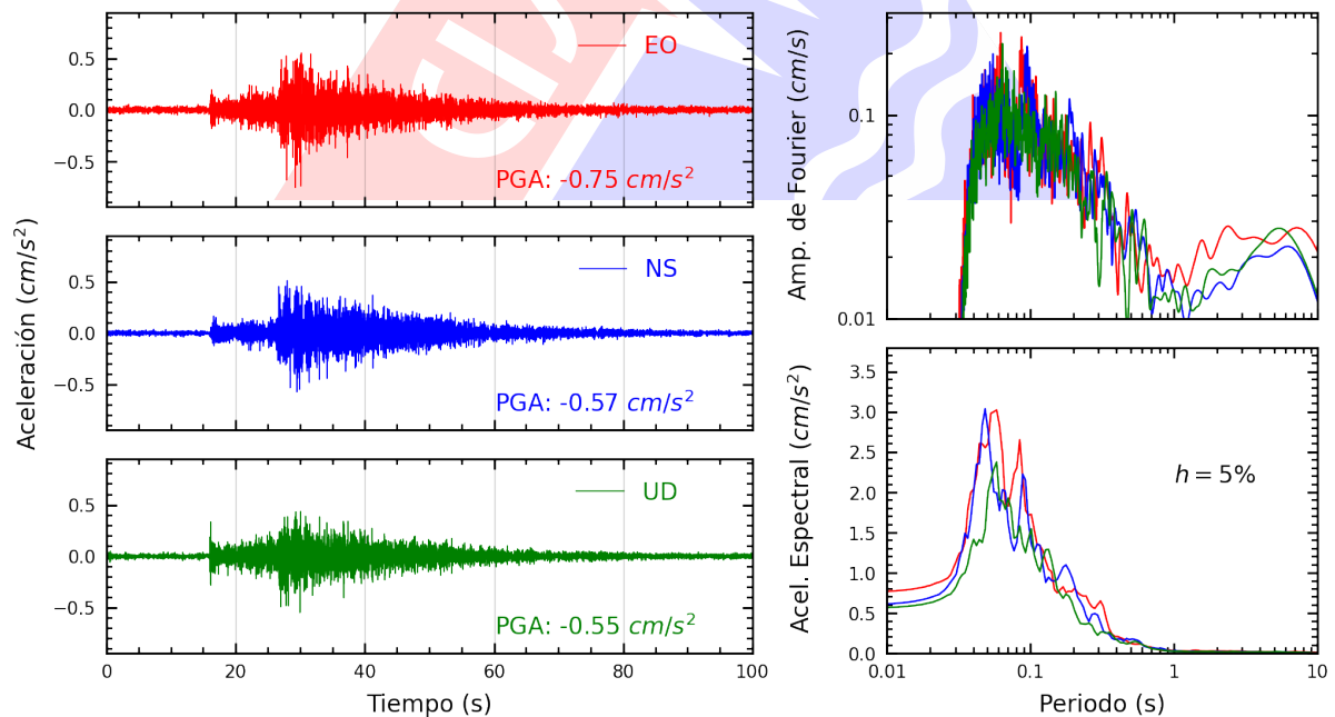
Figura A.28: Registros tiempo-historia, espectros de Fourier y de respuesta en las direcciones EO, NS y vertical de la estación IMCA. Sismo de Mala, Cañete - Lima del 2025-04-12, 22:47:00 (Hora local)
