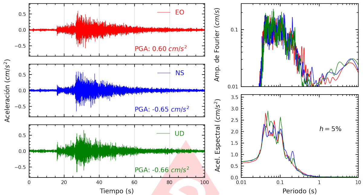
Figura A.31: Registros tiempo-historia, espectros de Fourier y de respuesta en las direcciones EO, NS y vertical de la estación USMP. Sismo de Mala, Cañete - Lima del 2025-04-12, 22:47:00 (Hora local)
