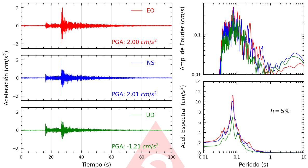
Figura A.15: Registros tiempo-historia, espectros de Fourier y de respuesta en las direcciones EO, NS y vertical de la estación CEPRE. Sismo de Mala, Cañete - Lima del 2025-04-12, 22:47:00 (Hora local)
