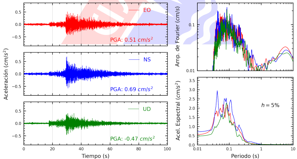
Figura A.30: Registros tiempo-historia, espectros de Fourier y de respuesta en las direcciones EO, NS y vertical de la estación COMAS. Sismo de Mala, Cañete - Lima del 2025-04-12, 22:47:00 (Hora local)
