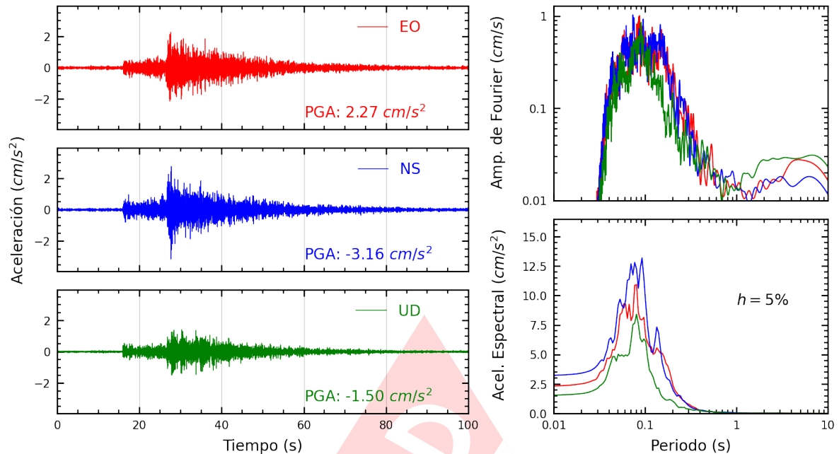
Figura A.5: Registros tiempo-historia, espectros de Fourier y de respuesta en las direcciones EO, NS y vertical de la estación USILM. Sismo de Mala, Cañete - Lima del 2025-04-12, 22:47:00 (Hora local)
