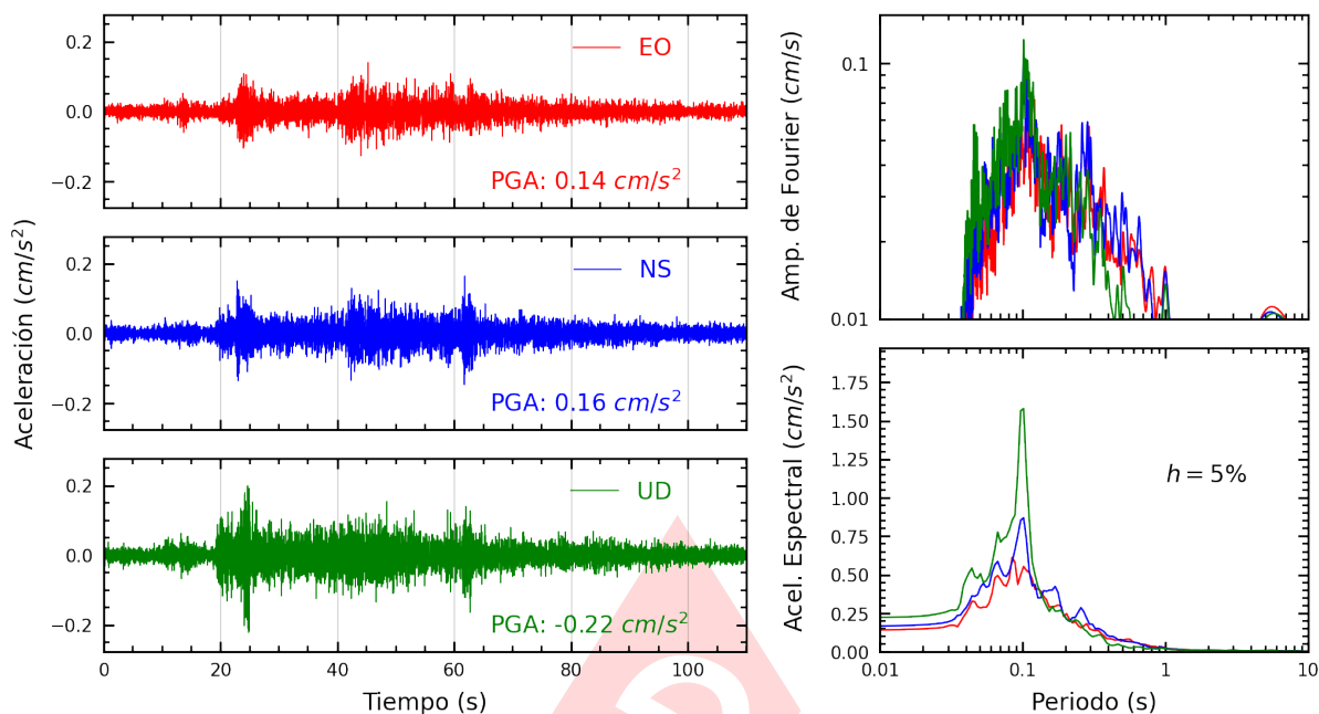
Figura A.33: Registros tiempo-historia, espectros de Fourier y de respuesta en las direcciones EO, NS y vertical de la estación UNICA. Sismo de Mala, Cañete - Lima del 2025-04-12, 22:47:00 (Hora local)
