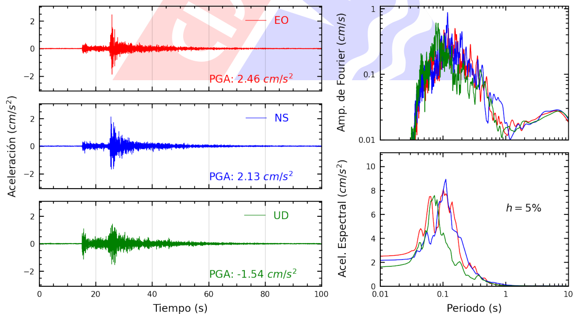
Figura A.8: Registros tiempo-historia, espectros de Fourier y de respuesta en las direcciones EO, NS y vertical de la estación SOCHO. Sismo de Mala, Cañete - Lima del 2025-04-12, 22:47:00 (Hora local)
