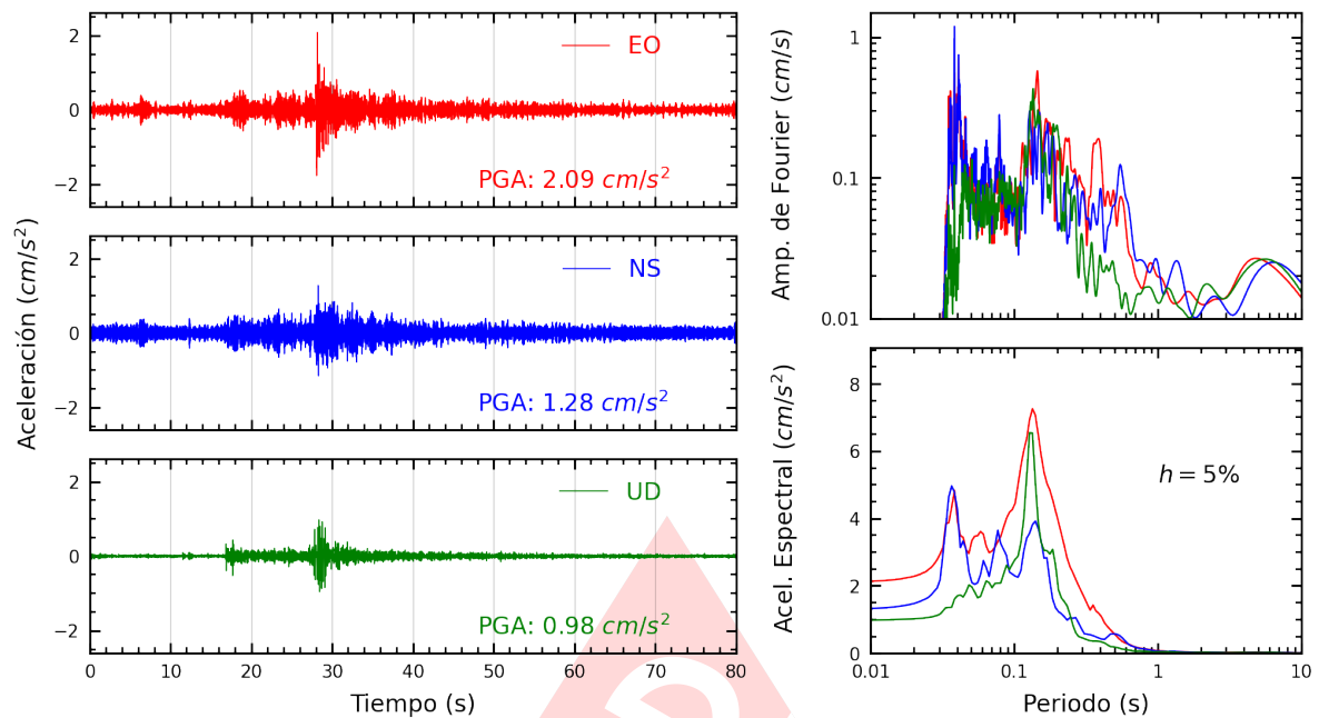
Figura A.13: Registros tiempo-historia, espectros de Fourier y de respuesta en las direcciones EO, NS y vertical de la estación DHNPE. Sismo de Mala, Cañete - Lima del 2025-04-12, 22:47:00 (Hora local)
