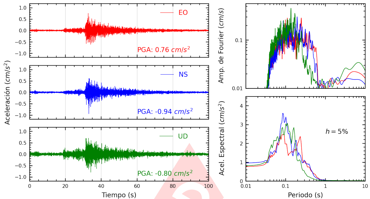
Figura A.25: Registros tiempo-historia, espectros de Fourier y de respuesta en las direcciones EO, NS y vertical de la estación MDPP. Sismo de Mala, Cañete - Lima del 2025-04-12, 22:47:00 (Hora local)
