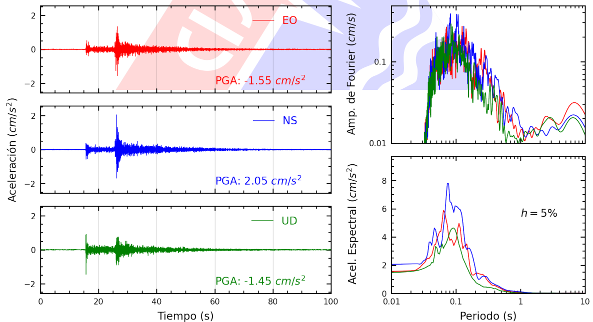
Figura A.14: Registros tiempo-historia, espectros de Fourier y de respuesta en las direcciones EO, NS y vertical de la estación SERVI. Sismo de Mala, Cañete - Lima del 2025-04-12, 22:47:00 (Hora local)
