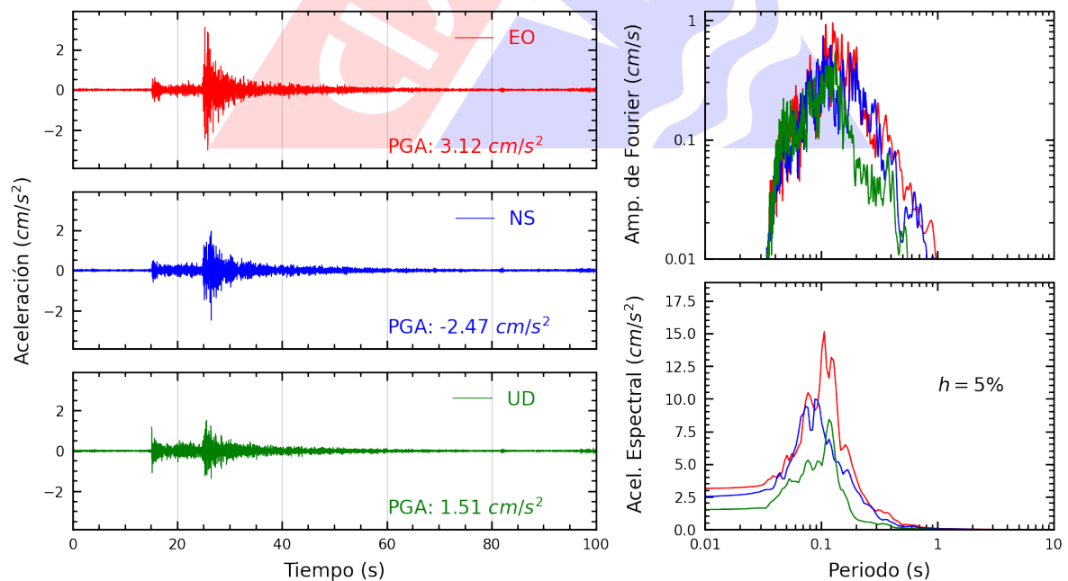
Figura A.6: Registros tiempo-historia, espectros de Fourier y de respuesta en las direcciones EO, NS y vertical de la estación SCCHO. Sismo de Mala, Cañete - Lima del 2025-04-12, 22:47:00 (Hora local)
