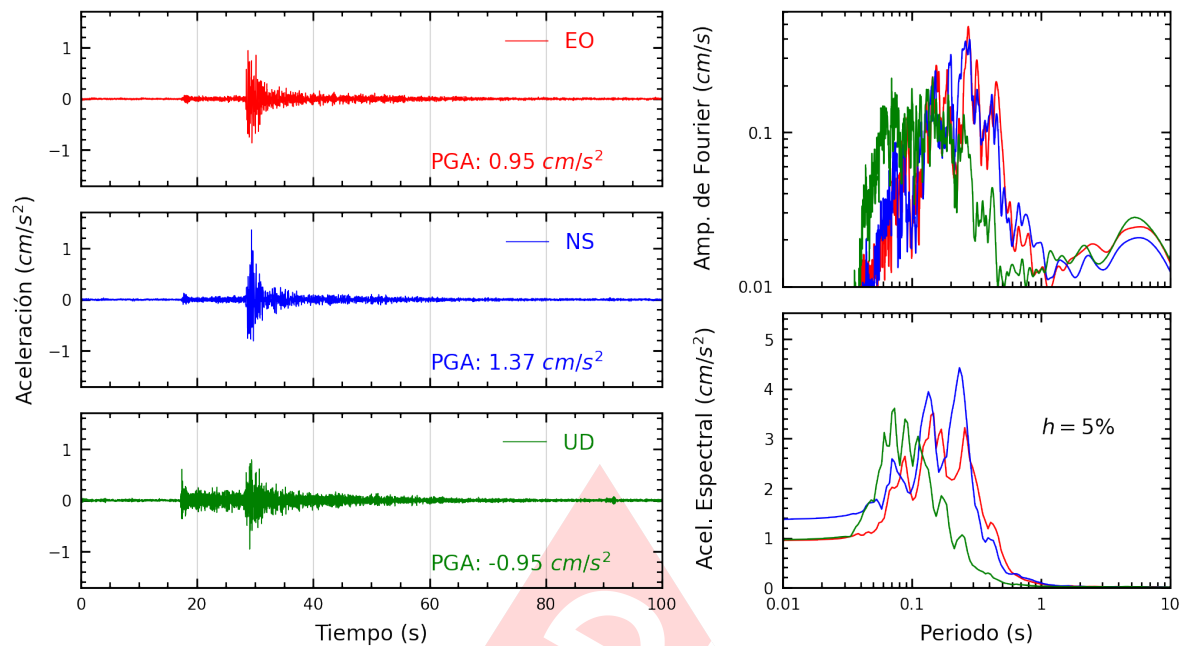
Figura A.23: Registros tiempo-historia, espectros de Fourier y de respuesta en las direcciones EO, NS y vertical de la estación ACAPU. Sismo de Mala, Cañete - Lima del 2025-04-12, 22:47:00 (Hora local)
