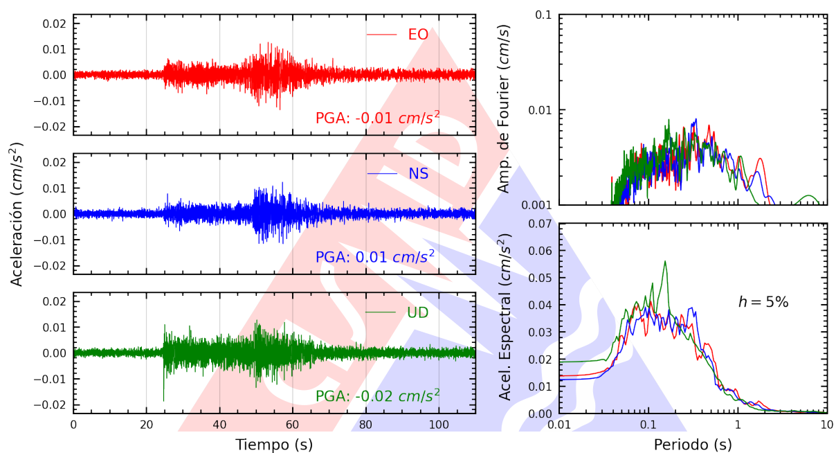
Figura A.35: Registros tiempo-historia, espectros de Fourier y de respuesta en las direcciones EO, NS y vertical de la estación UNCP. Sismo de Mala, Cañete - Lima del 2025-04-12, 22:47:00 (Hora local)
