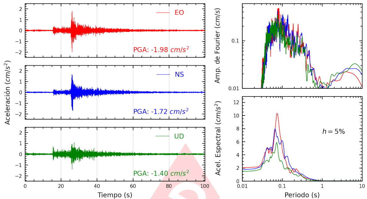
Figura A.17: Registros tiempo-historia, espectros de Fourier y de respuesta en las direcciones EO, NS y vertical de la estación URPPE. Sismo de Mala, Cañete - Lima del 2025-04-12, 22:47:00 (Hora local)
