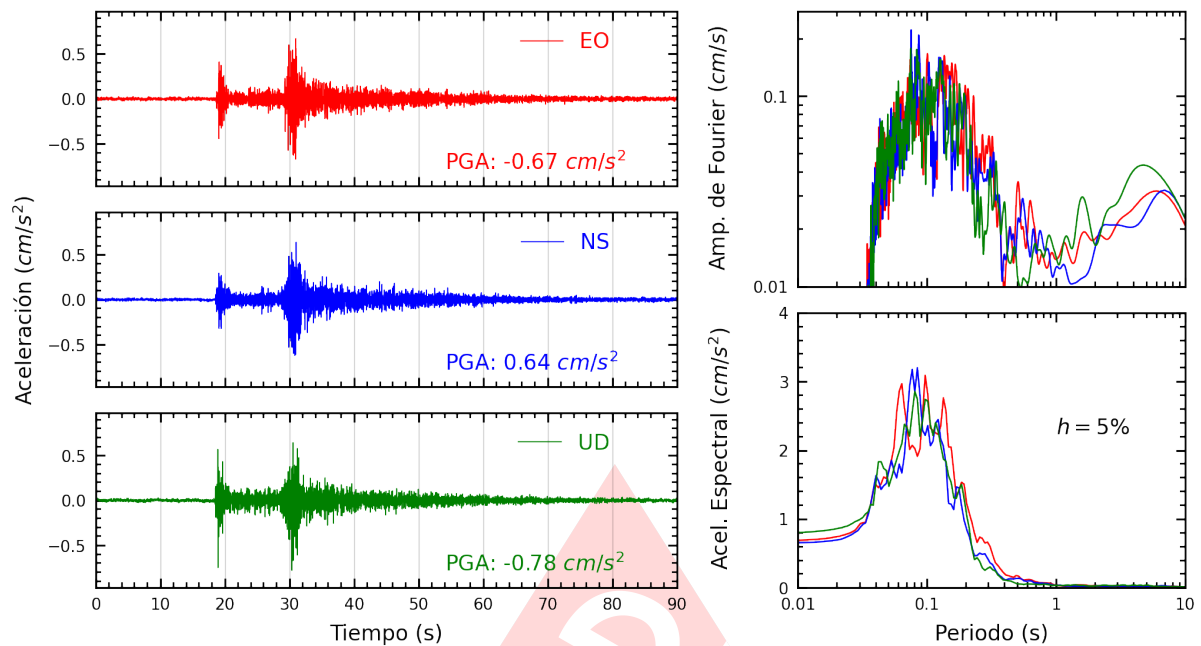
Figura A.27: Registros tiempo-historia, espectros de Fourier y de respuesta en las direcciones EO, NS y vertical de la estación UNMSM. Sismo de Mala, Cañete - Lima del 2025-04-12, 22:47:00 (Hora local)
