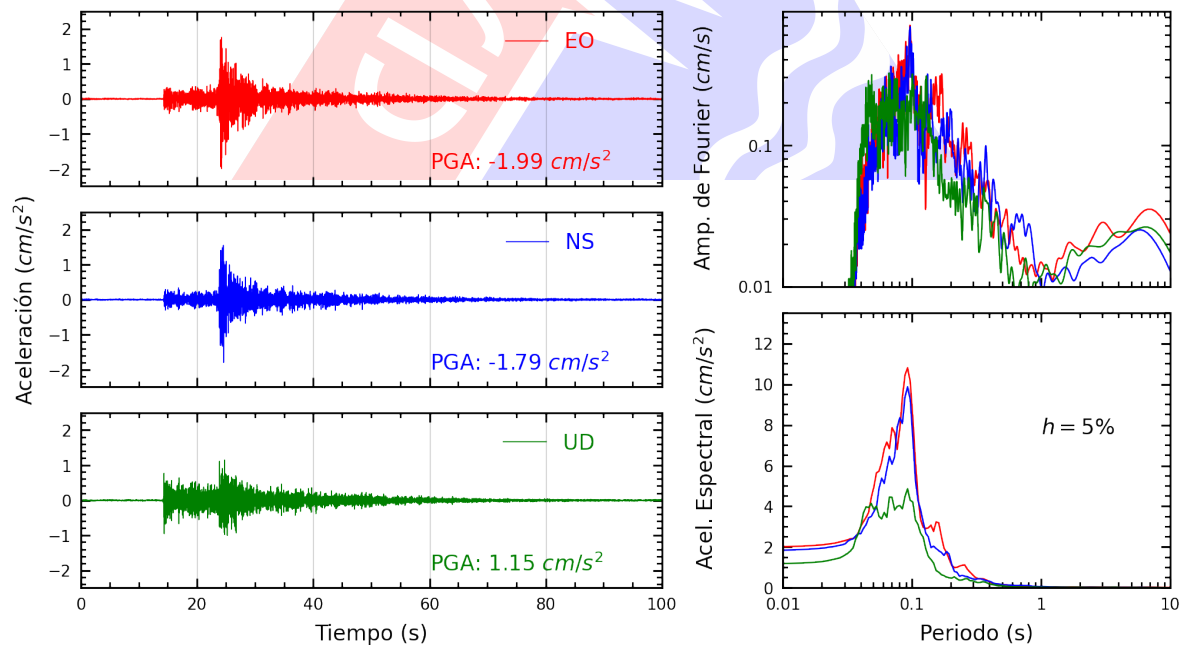
Figura A.16: Registros tiempo-historia, espectros de Fourier y de respuesta en las direcciones EO, NS y vertical de la estación USILP. Sismo de Mala, Cañete - Lima del 2025-04-12, 22:47:00 (Hora local)
