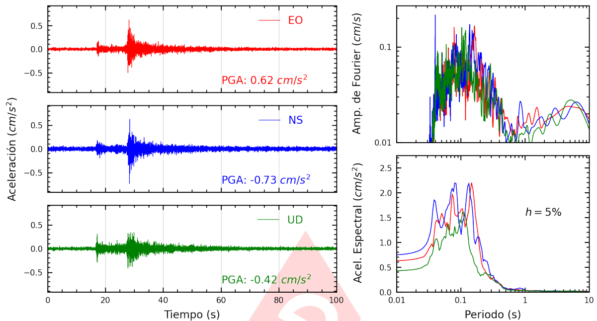
Figura A.29: Registros tiempo-historia, espectros de Fourier y de respuesta en las direcciones EO, NS y vertical de la estación BONDY. Sismo de Mala, Cañete - Lima del 2025-04-12, 22:47:00 (Hora local)
