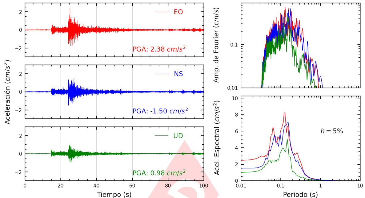
Figura A.9: Registros tiempo-historia, espectros de Fourier y de respuesta en las direcciones EO, NS y vertical de la estación BRISA. Sismo de Mala, Cañete - Lima del 2025-04-12, 22:47:00 (Hora local)
