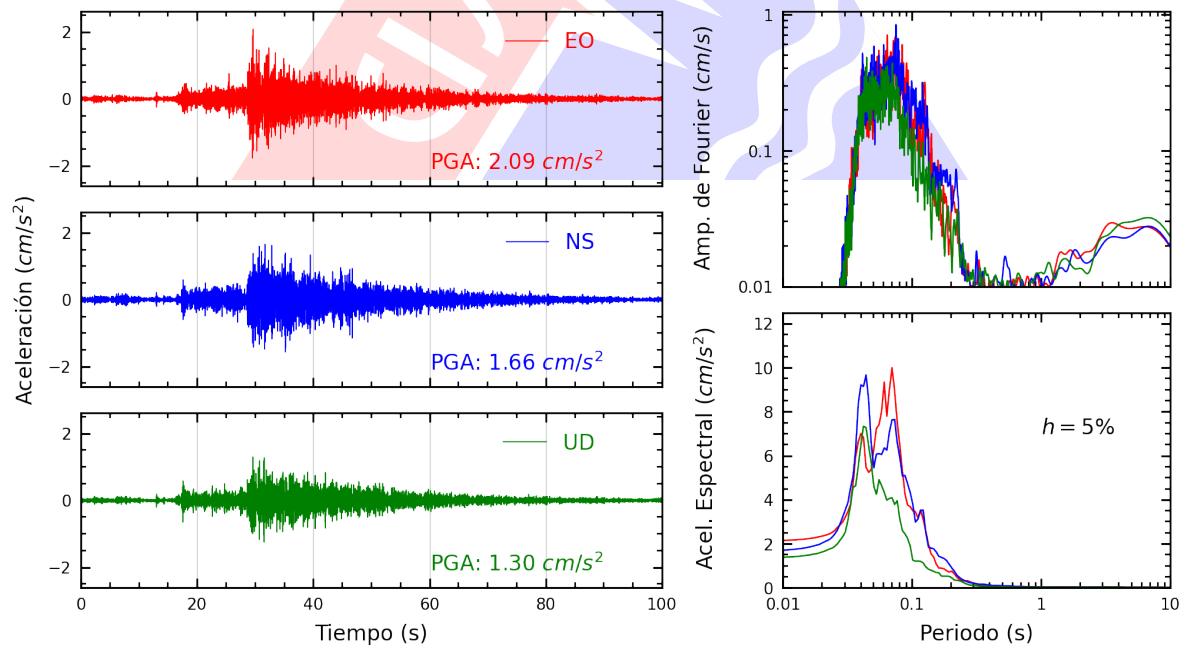
Figura A.12: Registros tiempo-historia, espectros de Fourier y de respuesta en las direcciones EO, NS y vertical de la estación JOSEO. Sismo de Mala, Cañete - Lima del 2025-04-12, 22:47:00 (Hora local)
