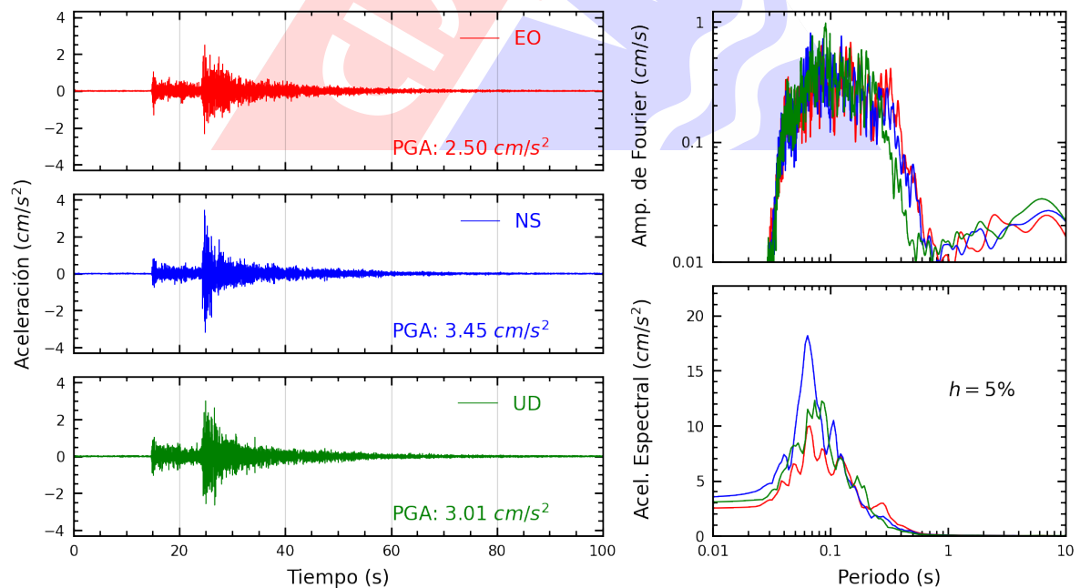
Figura A.4: Registros tiempo-historia, espectros de Fourier y de respuesta en las direcciones EO, NS y vertical de la estación SOVES. Sismo de Mala, Cañete - Lima del 2025-04-12, 22:47:00 (Hora local)
