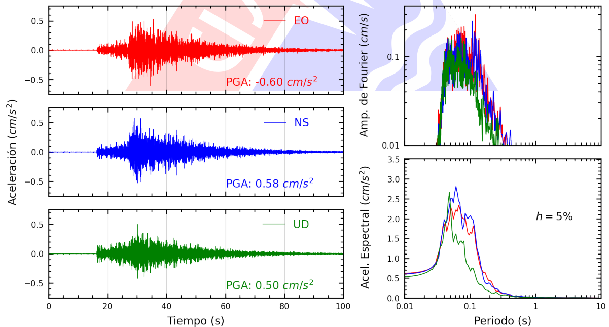
Figura A.32: Registros tiempo-historia, espectros de Fourier y de respuesta en las direcciones EO, NS y vertical de la estación ATARJ. Sismo de Mala, Cañete - Lima del 2025-04-12, 22:47:00 (Hora local)
