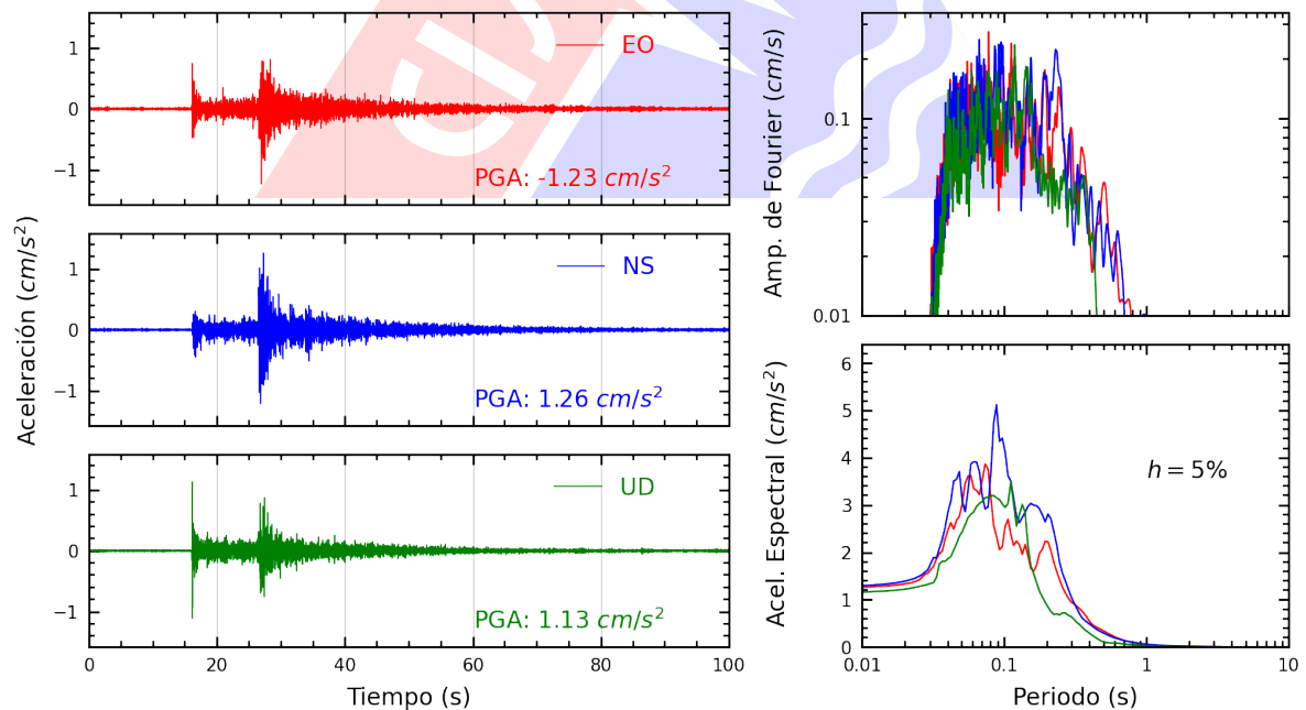
Figura A.24: Registros tiempo-historia, espectros de Fourier y de respuesta en las direcciones EO, NS y vertical de la estación BORJA. Sismo de Mala, Cañete - Lima del 2025-04-12, 22:47:00 (Hora local)
