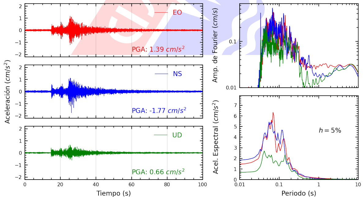
Figura A.18: Registros tiempo-historia, espectros de Fourier y de respuesta en las direcciones EO, NS y vertical de la estación UPCVI. Sismo de Mala, Cañete - Lima del 2025-04-12, 22:47:00 (Hora local)
