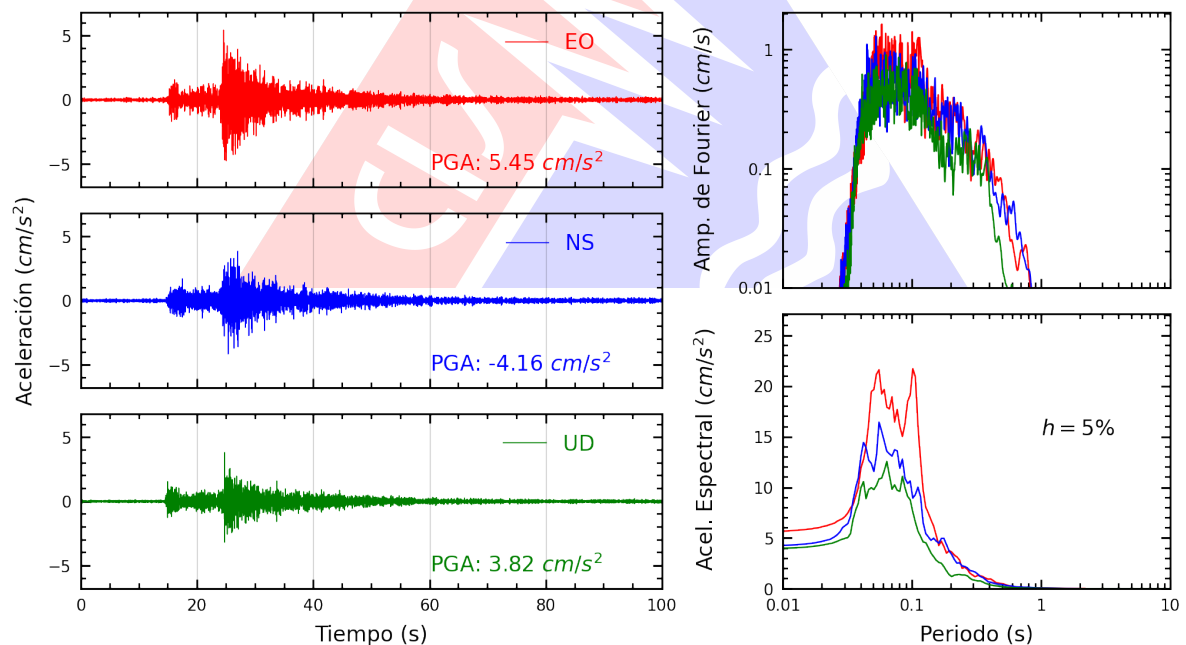
Figura A.2: Registros tiempo-historia, espectros de Fourier y de respuesta en las direcciones EO, NS y vertical de la estación UNTEL. Sismo de Mala, Cañete - Lima del 2025-04-12, 22:47:00 (Hora local)
