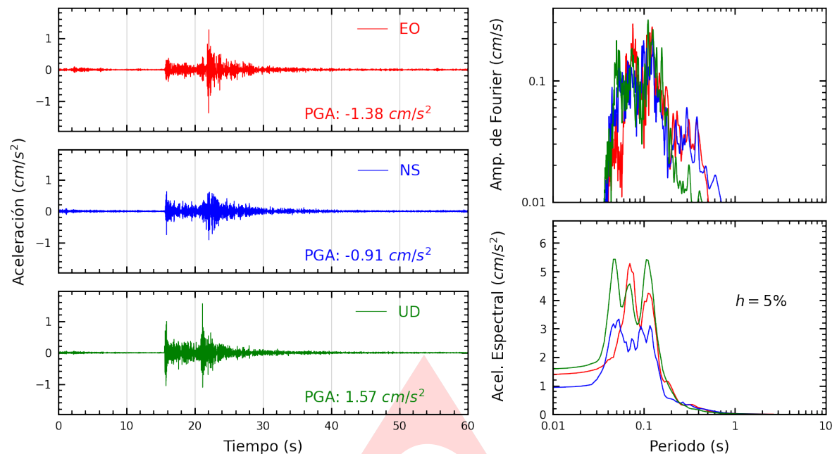
Figura A.1: Registros tiempo-historia, espectros de Fourier y de respuesta en las direcciones EO, NS y vertical de la estación UPAOP. Sismo de Sullana, Sullana - Piura del 2025-04-13, 07:52:56 (Hora local)
