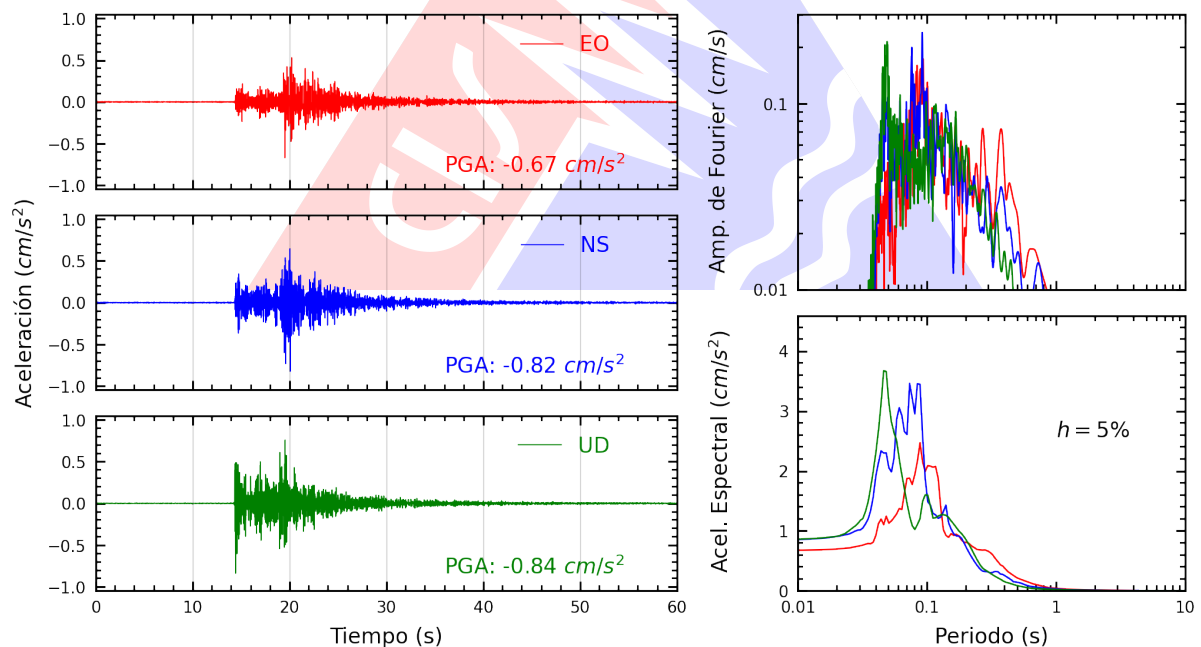
Figura A.2: Registros tiempo-historia, espectros de Fourier y de respuesta en las direcciones EO, NS y vertical de la estación UNF. Sismo de Sullana, Sullana - Piura del 2025-04-13, 07:52:56 (Hora local)
