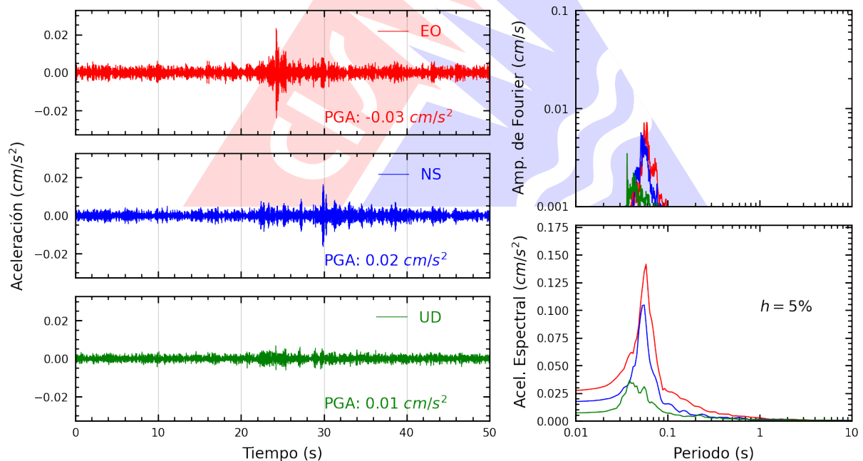
Figura A.2: Registros tiempo-historia, espectros de Fourier y de respuesta en las direcciones EO, NS y vertical de la estación UNMBA. Sismo de Chala, Caraveli - Arequipa del 2025-04-15, 00:54:56 (Hora local)
