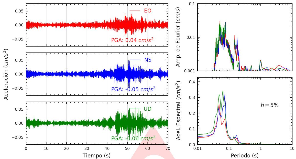
Figura A.1: Registros tiempo-historia, espectros de Fourier y de respuesta en las direcciones EO, NS y vertical de la estación ASIA. Sismo de Chala, Caraveli - Arequipa del 2025-04-15, 00:54:56 (Hora local)
