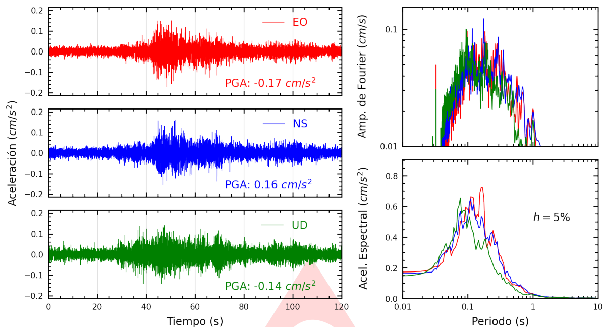
Figura A.1: Registros tiempo-historia, espectros de Fourier y de respuesta en las direcciones EO, NS y vertical de la estación UNICA. Sismo de Marcona, Nazca - Ica del 2025-04-15, 14:37:16 (Hora local)
