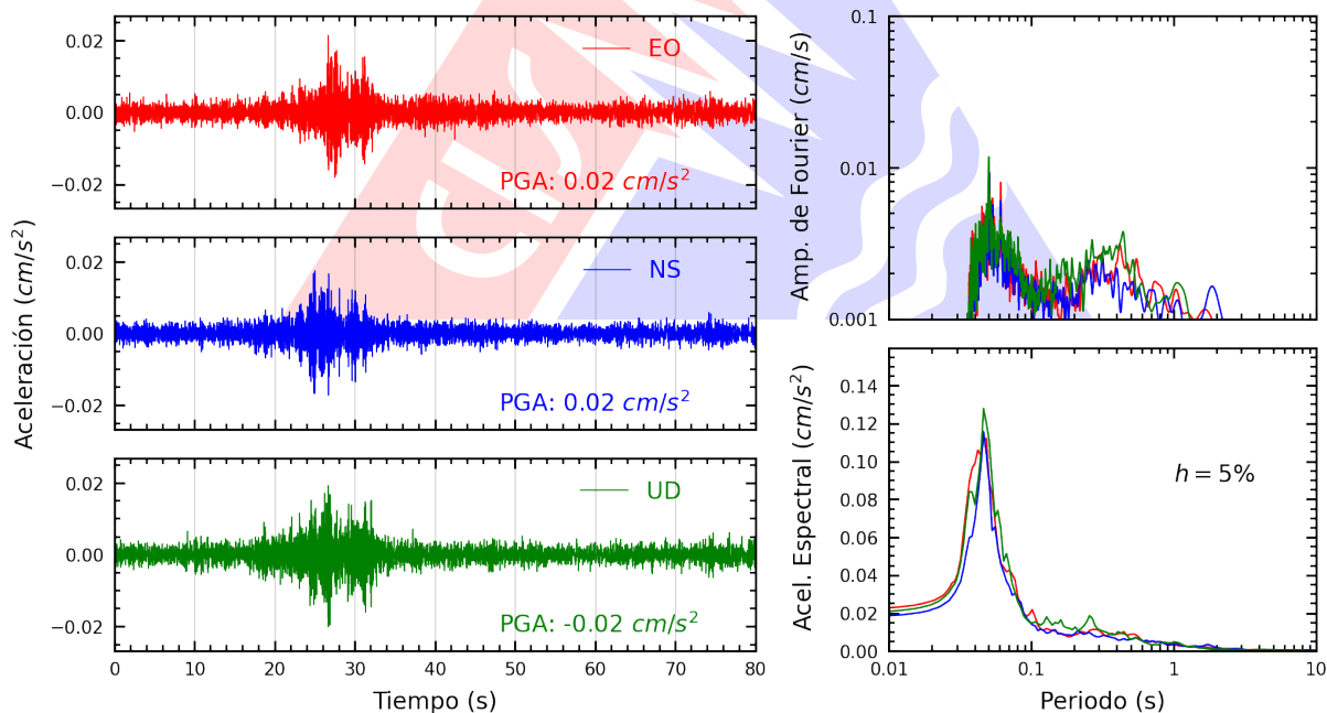
Figura A.2: Registros tiempo-historia, espectros de Fourier y de respuesta en las direcciones EO, NS y vertical de la estación UNCP. Sismo de Marcona, Nazca - Ica del 2025-04-15, 14:37:16 (Hora local)
