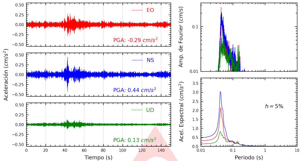
Figura A.1: Registros tiempo-historia, espectros de Fourier y de respuesta en las direcciones EO, NS y vertical de la estación SCTRU. Sismo de Tocache Nuevo, Tocache - San Martín del 2025-04-18, 06:19:38 (Hora local)
