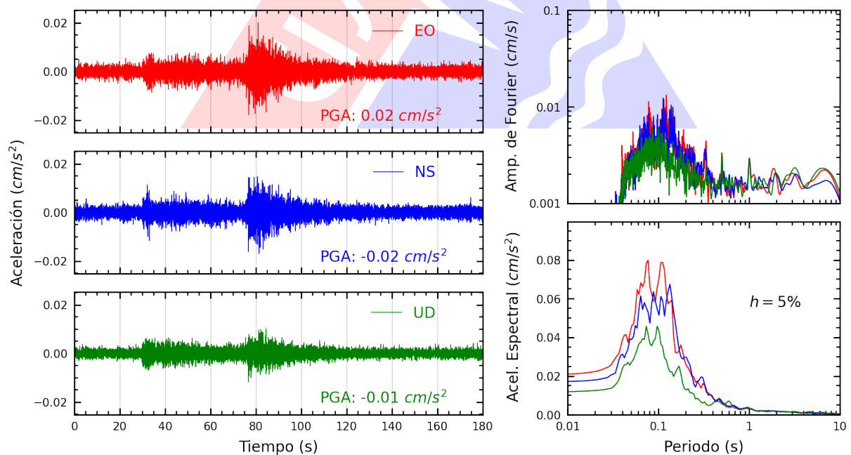
Figura A.8: Registros tiempo-historia, espectros de Fourier y de respuesta en las direcciones EO, NS y vertical de la estación ATARJ. Sismo de Tocache Nuevo, Tocache - San Martín del 2025-04-18, 06:19:38 (Hora local)
