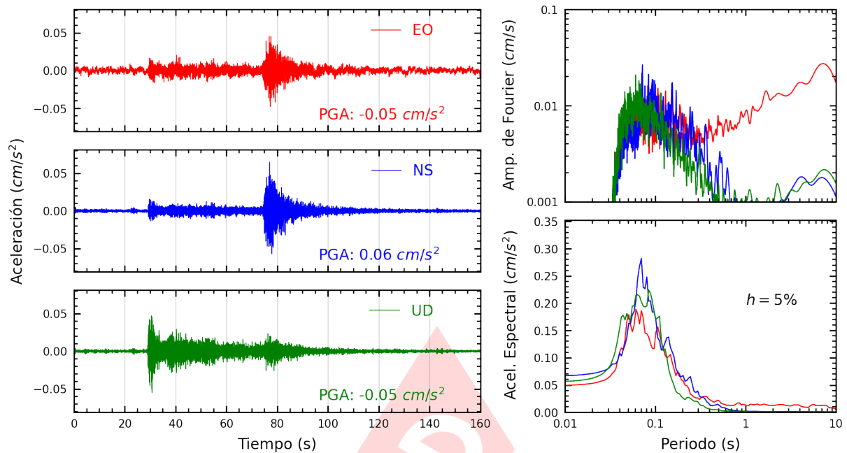
Figura A.7: Registros tiempo-historia, espectros de Fourier y de respuesta en las direcciones EO, NS y vertical de la estación SCCHI. Sismo de Tocache Nuevo, Tocache - San Martín del 2025-04-18, 06:19:38 (Hora local)
