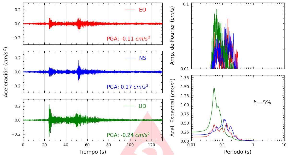
Figura A.5: Registros tiempo-historia, espectros de Fourier y de respuesta en las direcciones EO, NS y vertical de la estación UNAAA. Sismo de Tocache Nuevo, Tocache - San Martín del 2025-04-18, 06:19:38 (Hora local)
