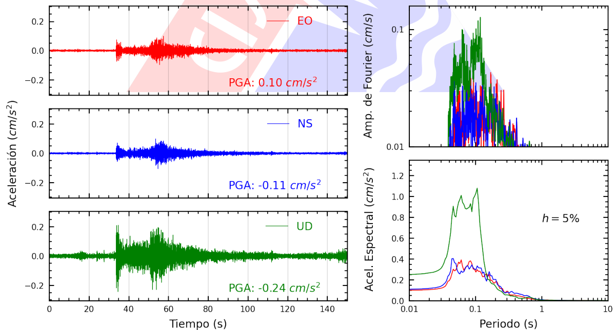
Figura A.4: Registros tiempo-historia, espectros de Fourier y de respuesta en las direcciones EO, NS y vertical de la estación SCPUC. Sismo de Tocache Nuevo, Tocache - San Martín del 2025-04-18, 06:19:38 (Hora local)
