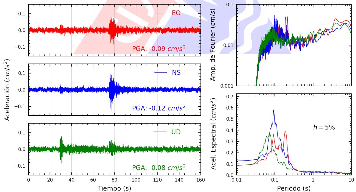
Figura A.6: Registros tiempo-historia, espectros de Fourier y de respuesta en las direcciones EO, NS y vertical de la estación UCVCH. Sismo de Tocache Nuevo, Tocache - San Martín del 2025-04-18, 06:19:38 (Hora local)
