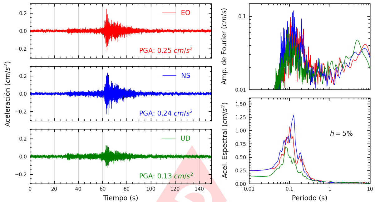
Figura A.3: Registros tiempo-historia, espectros de Fourier y de respuesta en las direcciones EO, NS y vertical de la estación UNTRM. Sismo de Tocache Nuevo, Tocache - San Martín del 2025-04-18, 06:19:38 (Hora local)
