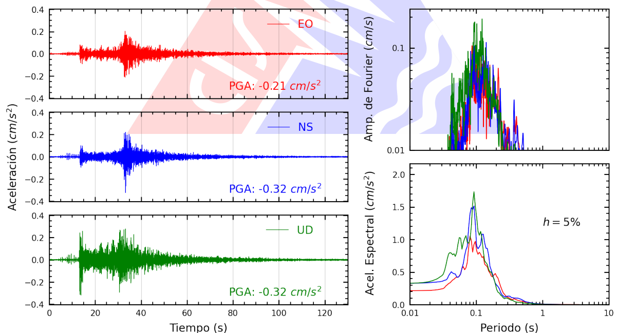
Figura A.2: Registros tiempo-historia, espectros de Fourier y de respuesta en las direcciones EO, NS y vertical de la estación UNIA. Sismo de Tocache Nuevo, Tocache - San Martín del 2025-04-18, 06:19:38 (Hora local)
