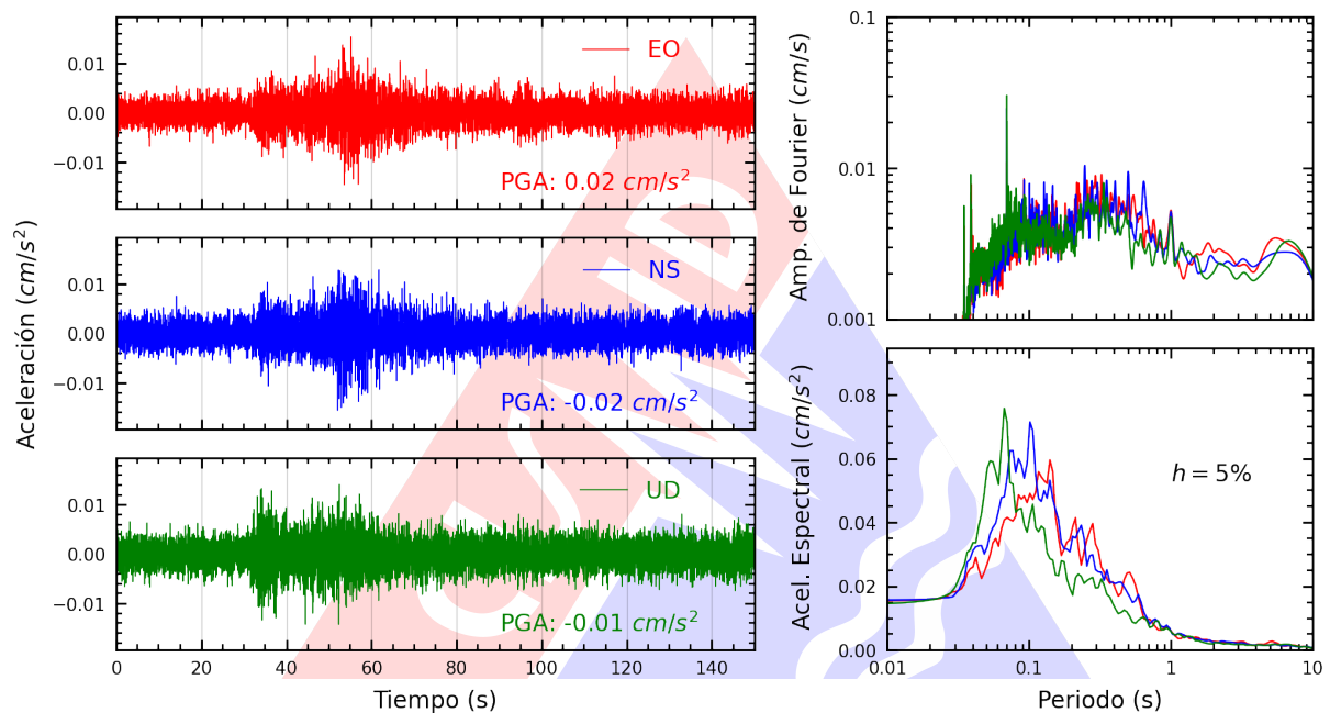
Figura A.5: Registros tiempo-historia, espectros de Fourier y de respuesta en las direcciones EO, NS y vertical de la estación UNC. Sismo de San Pedro De Lloc, Pacasmayo - La Libertad del 2025-04-19, 01:13:44 (Hora local)
