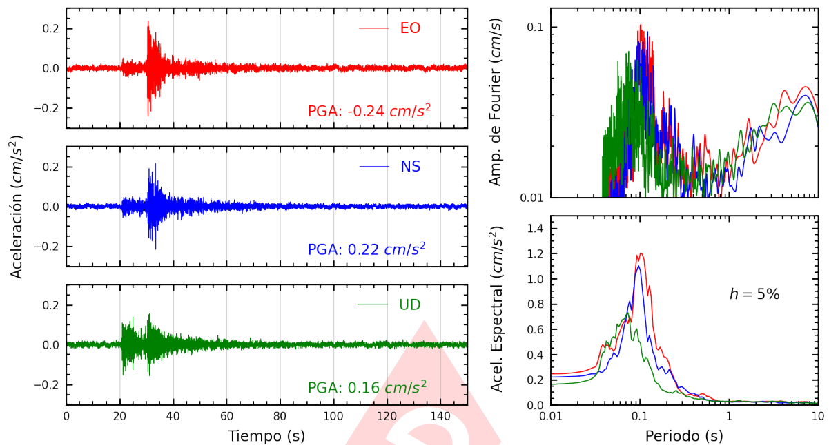
Figura A.3: Registros tiempo-historia, espectros de Fourier y de respuesta en las direcciones EO, NS y vertical de la estación UCVCH. Sismo de San Pedro De Lloc, Pacasmayo - La Libertad del 2025-04-19, 01:13:44 (Hora local)
