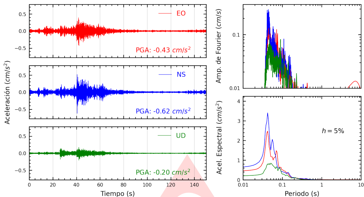
Figura A.1: Registros tiempo-historia, espectros de Fourier y de respuesta en las direcciones EO, NS y vertical de la estación SCTR. Sismo de San Pedro De Lloc, Pacasmayo - La Libertad del 2025-04-19, 01:13:44 (Hora local)
