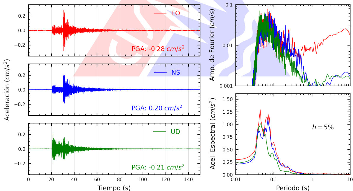
Figura A.2: Registros tiempo-historia, espectros de Fourier y de respuesta en las direcciones EO, NS y vertical de la estación SCCHI. Sismo de San Pedro De Lloc, Pacasmayo - La Libertad del 2025-04-19, 01:13:44 (Hora local)
