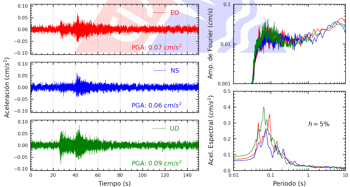
Figura A.4: Registros tiempo-historia, espectros de Fourier y de respuesta en las direcciones EO, NS y vertical de la estación UPAOT. Sismo de San Pedro De Lloc, Pacasmayo - La Libertad del 2025-04-19, 01:13:44 (Hora local)
