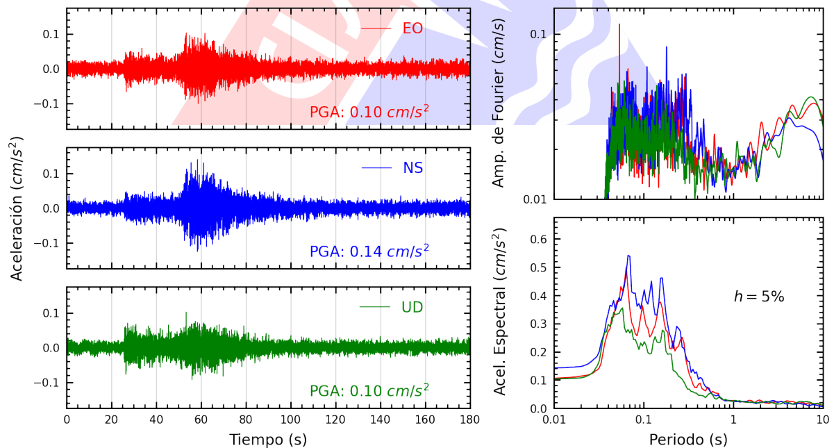
Figura A.18: Registros tiempo-historia, espectros de Fourier y de respuesta en las direcciones EO, NS y vertical de la estación SERVI. Sismo de La Tinguña, Ica - Ica del 2025-04-20, 17:03:32 (Hora local)
