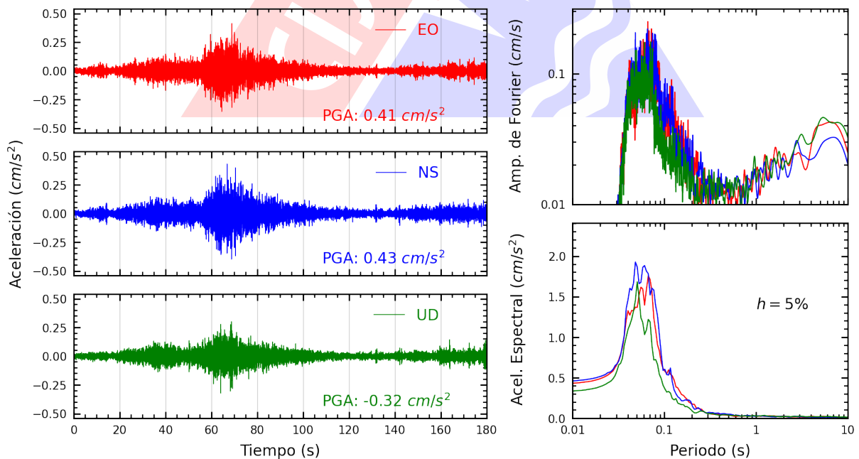
Figura A.6: Registros tiempo-historia, espectros de Fourier y de respuesta en las direcciones EO, NS y vertical de la estación JOSEO. Sismo de La Tinguña, Ica - Ica del 2025-04-20, 17:03:32 (Hora local)
