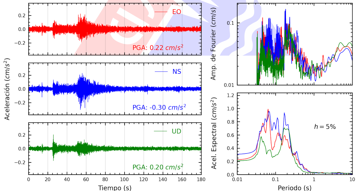
Figura A.10: Registros tiempo-historia, espectros de Fourier y de respuesta en las direcciones EO, NS y vertical de la estación UPCVI. Sismo de La Tinguña, Ica - Ica del 2025-04-20, 17:03:32 (Hora local)
