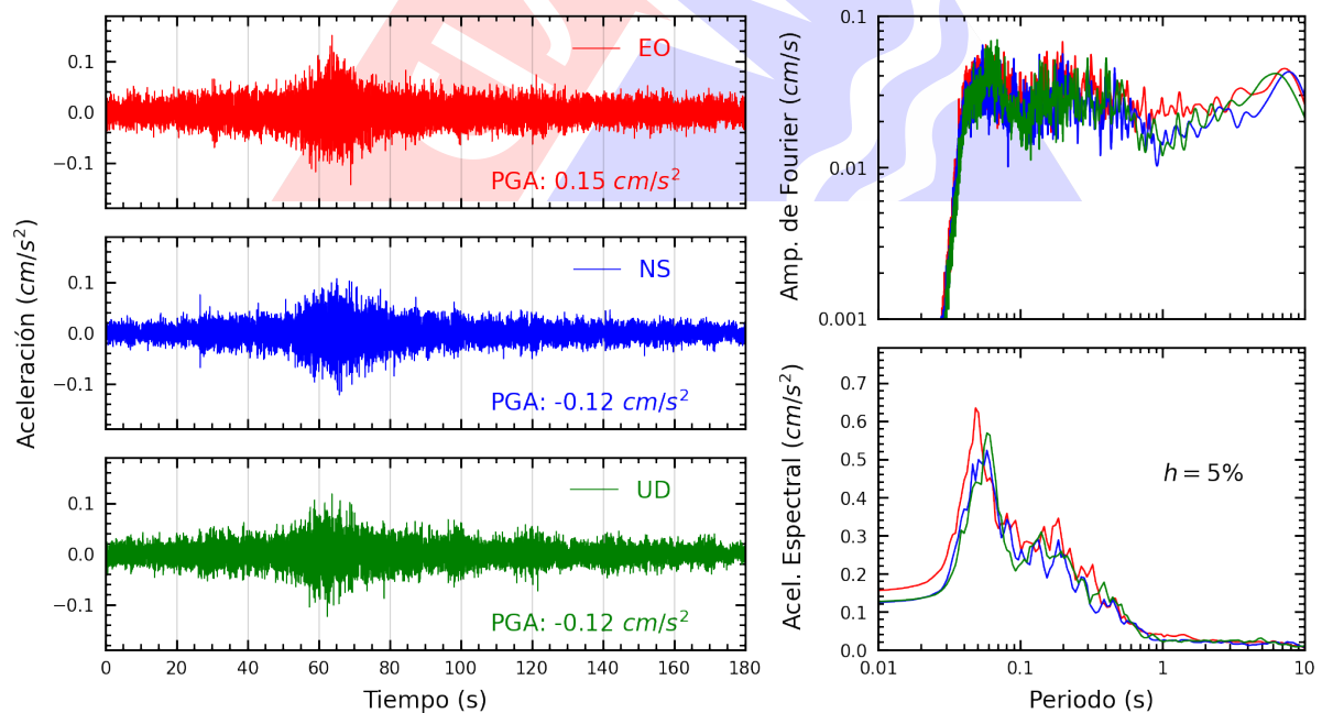
Figura A.16: Registros tiempo-historia, espectros de Fourier y de respuesta en las direcciones EO, NS y vertical de la estación IMCA. Sismo de La Tinguña, Ica - Ica del 2025-04-20, 17:03:32 (Hora local)
