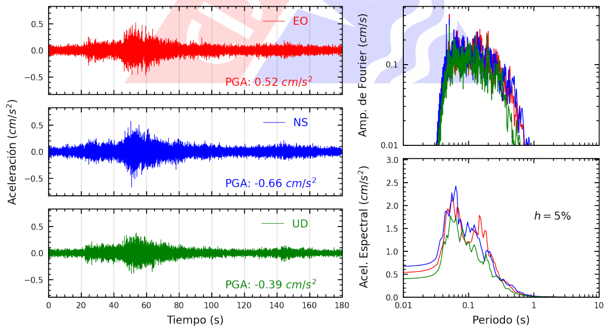
Figura A.4: Registros tiempo-historia, espectros de Fourier y de respuesta en las direcciones EO, NS y vertical de la estación PHER2. Sismo de La Tinguña, Ica - Ica del 2025-04-20, 17:03:32 (Hora local)
