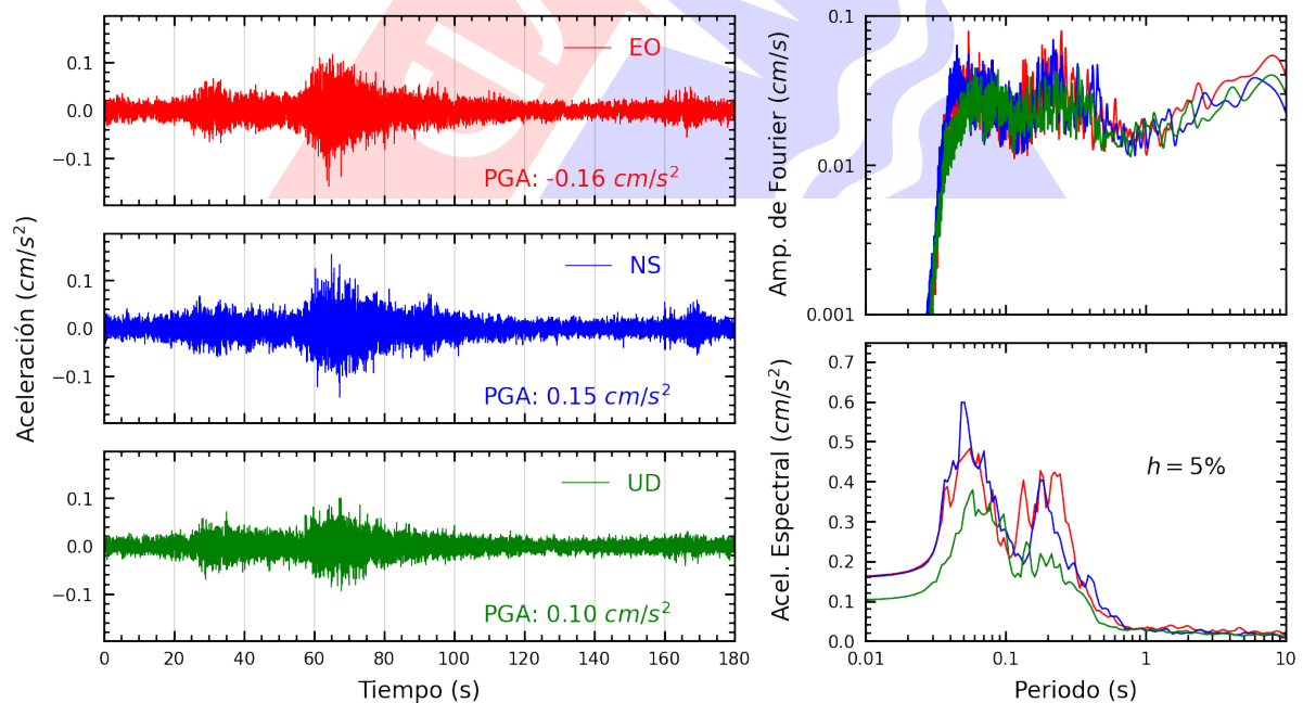
Figura A.14: Registros tiempo-historia, espectros de Fourier y de respuesta en las direcciones EO, NS y vertical de la estación COMAS. Sismo de La Tinguña, Ica - Ica del 2025-04-20, 17:03:32 (Hora local)
