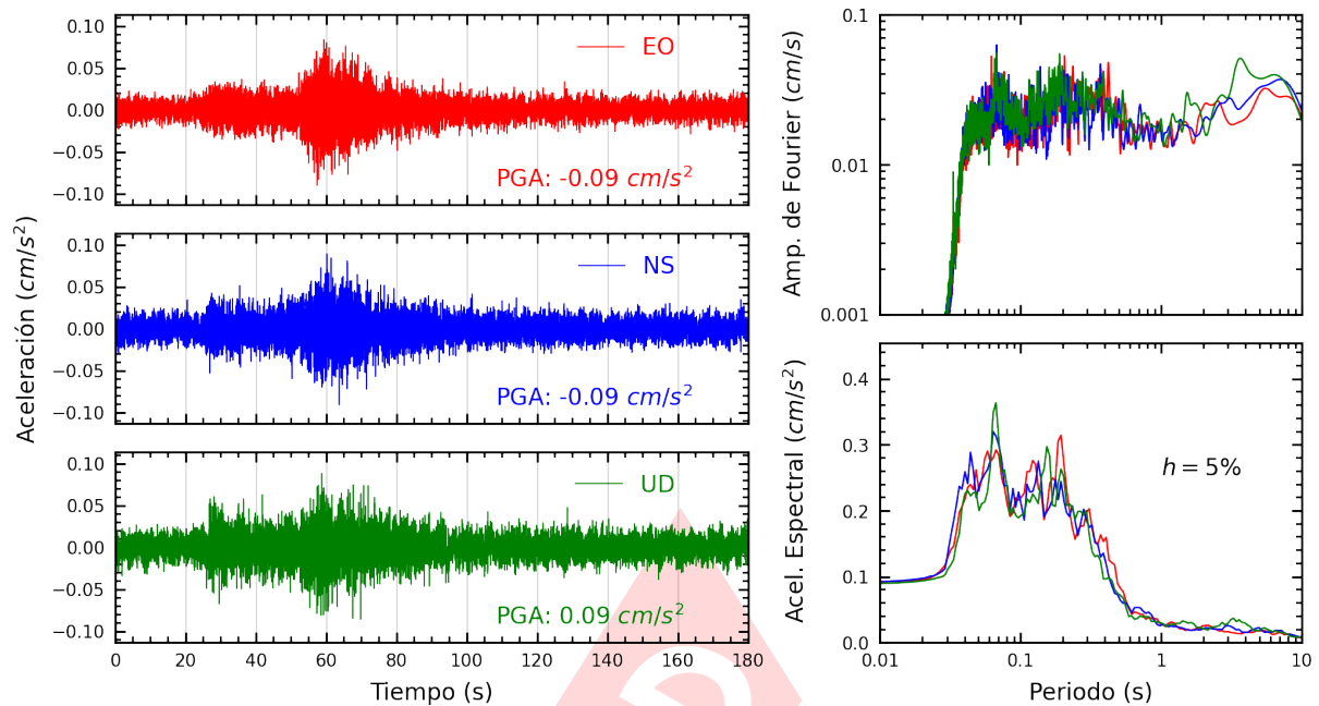
Figura A.19: Registros tiempo-historia, espectros de Fourier y de respuesta en las direcciones EO, NS y vertical de la estación UNFV. Sismo de La Tinguña, Ica - Ica del 2025-04-20, 17:03:32 (Hora local)
