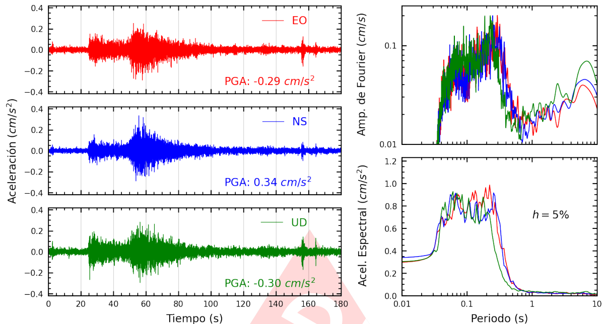
Figura A.9: Registros tiempo-historia, espectros de Fourier y de respuesta en las direcciones EO, NS y vertical de la estación SOVES. Sismo de La Tinguña, Ica - Ica del 2025-04-20, 17:03:32 (Hora local)
