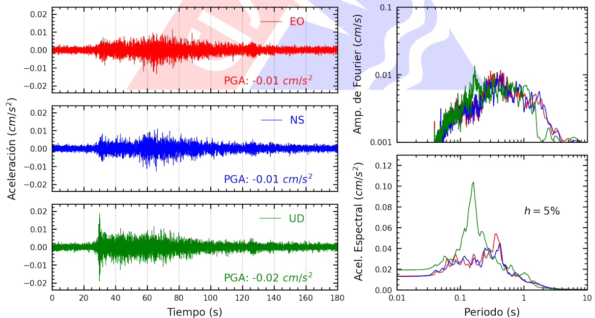
Figura A.20: Registros tiempo-historia, espectros de Fourier y de respuesta en las direcciones EO, NS y vertical de la estación UNCP. Sismo de La Tinguña, Ica - Ica del 2025-04-20, 17:03:32 (Hora local)
