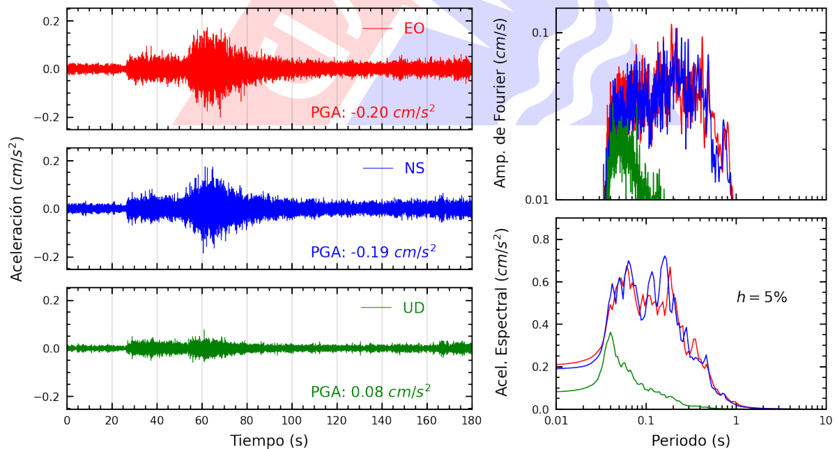
Figura A.12: Registros tiempo-historia, espectros de Fourier y de respuesta en las direcciones EO, NS y vertical de la estación UCVA2. Sismo de La Tinguña, Ica - Ica del 2025-04-20, 17:03:32 (Hora local)
