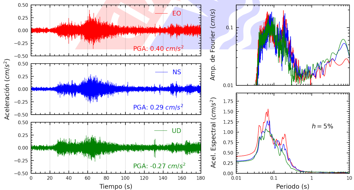
Figura A.8: Registros tiempo-historia, espectros de Fourier y de respuesta en las direcciones EO, NS y vertical de la estación INDEP. Sismo de La Tinguña, Ica - Ica del 2025-04-20, 17:03:32 (Hora local)
