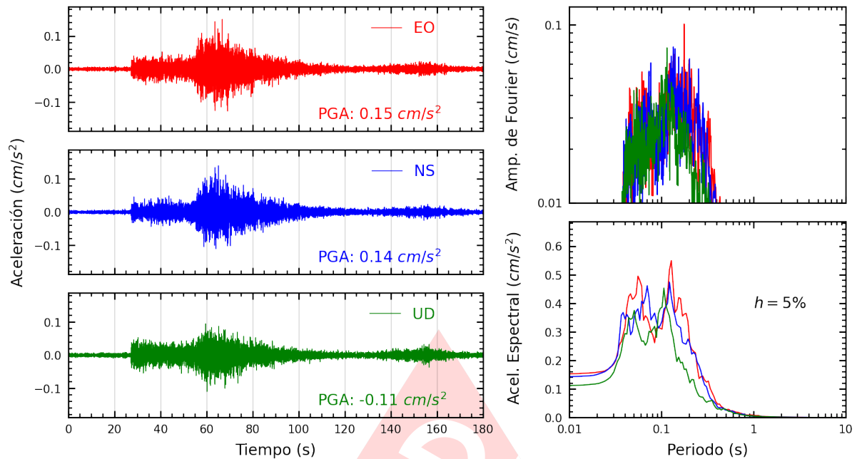
Figura A.17: Registros tiempo-historia, espectros de Fourier y de respuesta en las direcciones EO, NS y vertical de la estación JALV2. Sismo de La Tinguña, Ica - Ica del 2025-04-20, 17:03:32 (Hora local)
