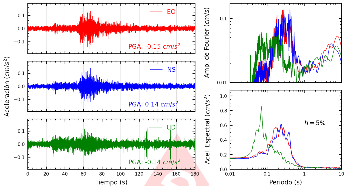
Figura A.15: Registros tiempo-historia, espectros de Fourier y de respuesta en las direcciones EO, NS y vertical de la estación ACAPU. Sismo de La Tinguña, Ica - Ica del 2025-04-20, 17:03:32 (Hora local)
