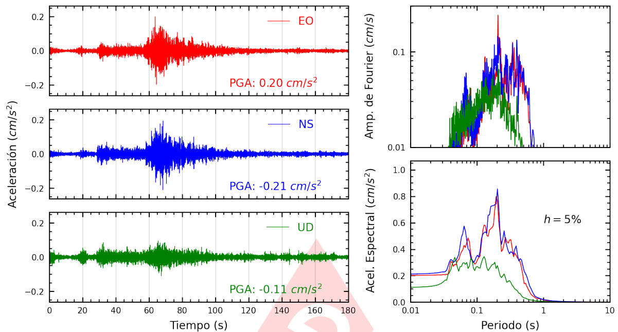
Figura A.11: Registros tiempo-historia, espectros de Fourier y de respuesta en las direcciones EO, NS y vertical de la estación VHAY2. Sismo de La Tinguña, Ica - Ica del 2025-04-20, 17:03:32 (Hora local)
