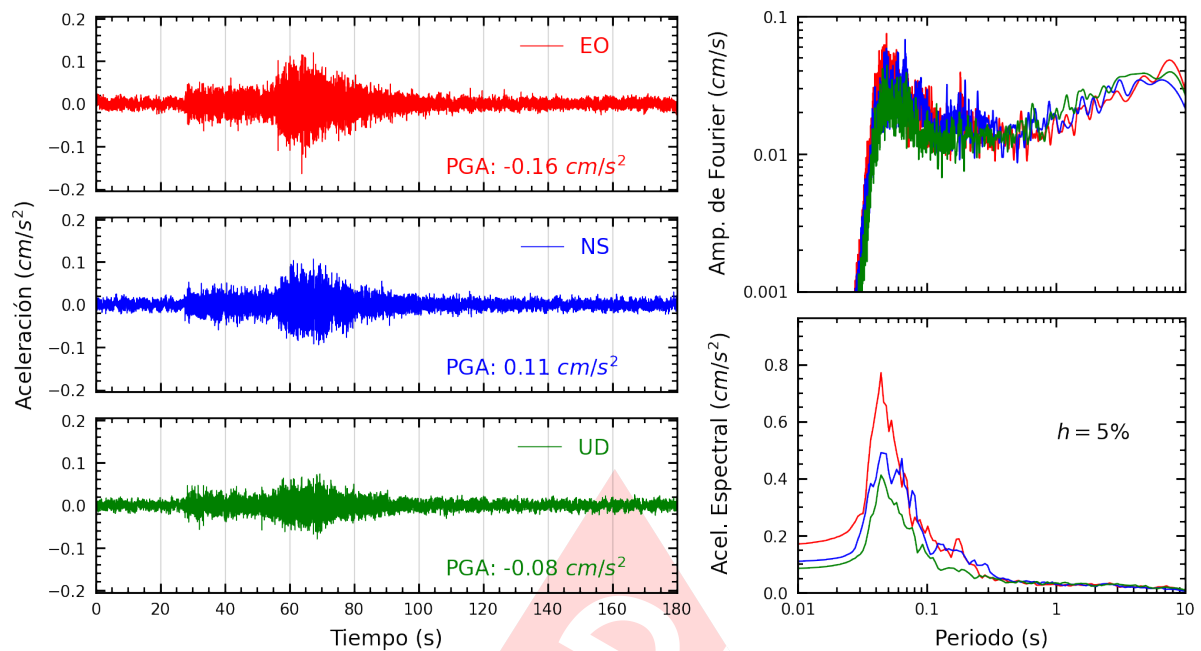
Figura A.13: Registros tiempo-historia, espectros de Fourier y de respuesta en las direcciones EO, NS y vertical de la estación UCSS. Sismo de La Tinguña, Ica - Ica del 2025-04-20, 17:03:32 (Hora local)
