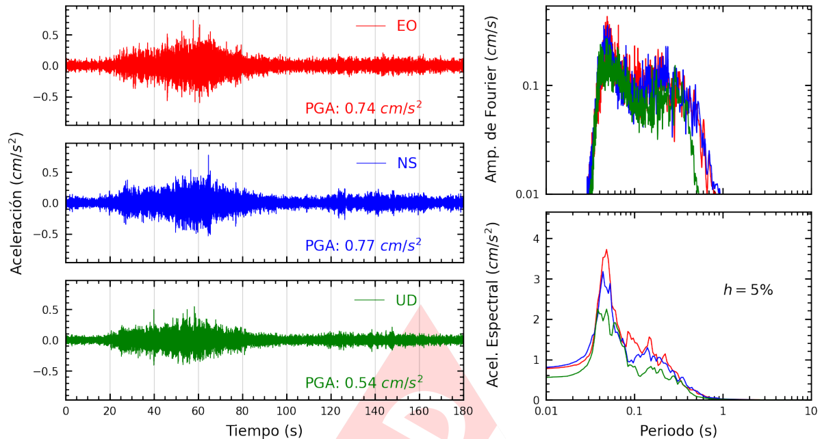
Figura A.3: Registros tiempo-historia, espectros de Fourier y de respuesta en las direcciones EO, NS y vertical de la estación UNTEL. Sismo de La Tinguña, Ica - Ica del 2025-04-20, 17:03:32 (Hora local)
