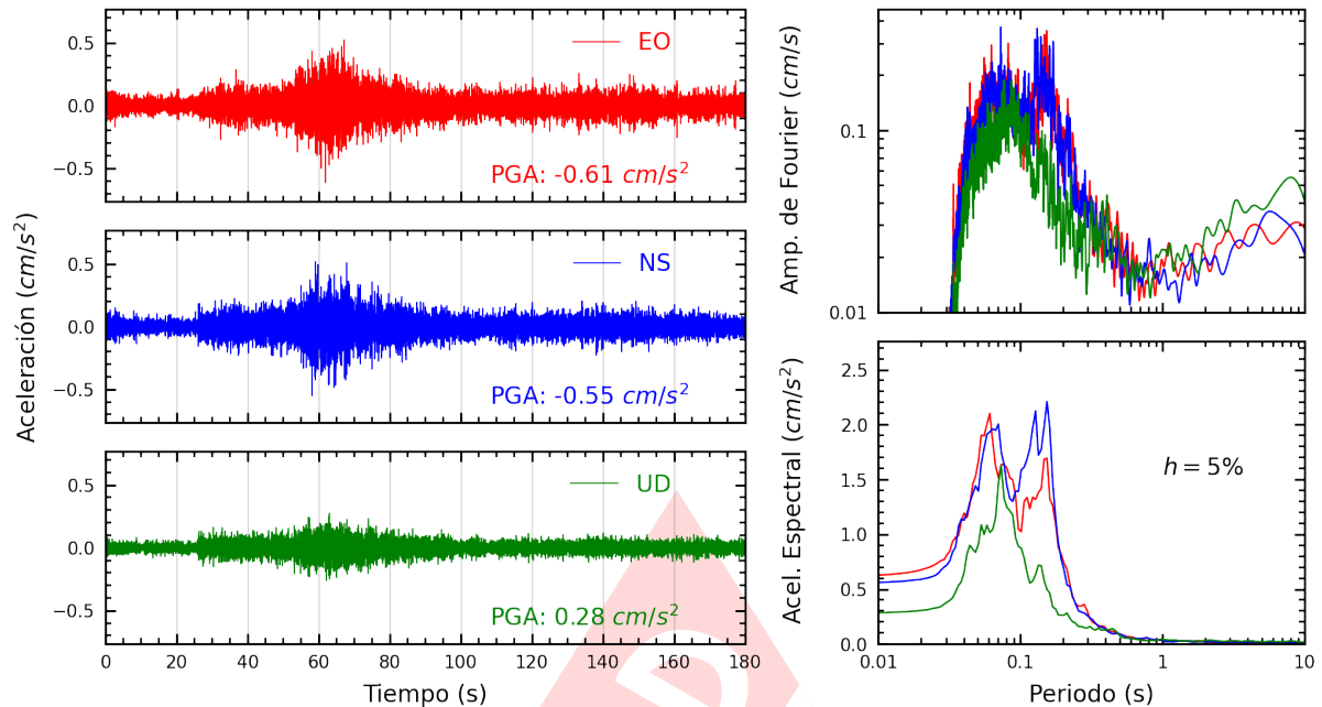
Figura A.5: Registros tiempo-historia, espectros de Fourier y de respuesta en las direcciones EO, NS y vertical de la estación USILM. Sismo de La Tinguña, Ica - Ica del 2025-04-20, 17:03:32 (Hora local)
