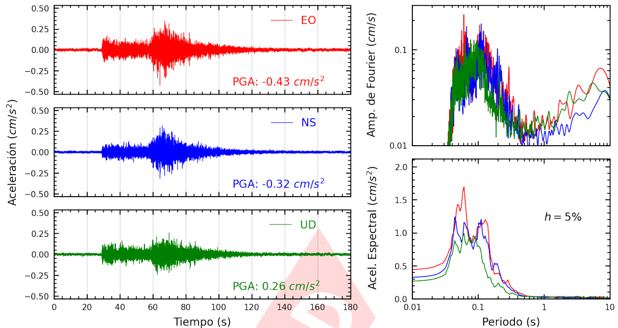
Figura A.7: Registros tiempo-historia, espectros de Fourier y de respuesta en las direcciones EO, NS y vertical de la estación AMORE. Sismo de La Tinguña, Ica - Ica del 2025-04-20, 17:03:32 (Hora local)
