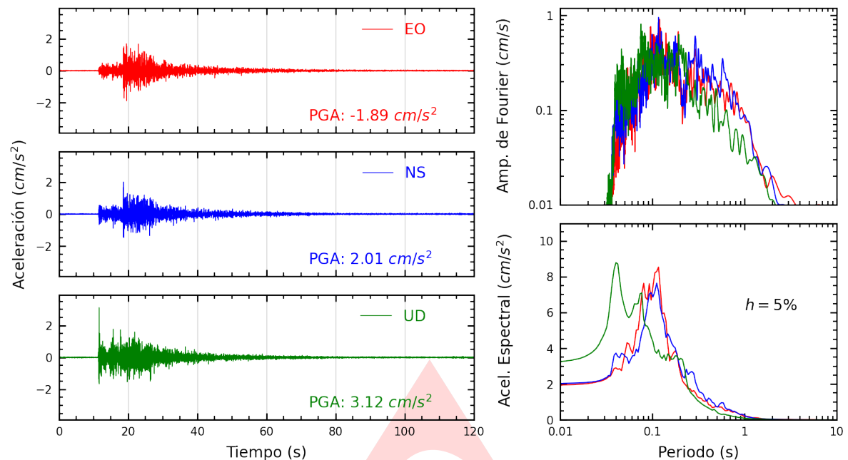
Figura A.1: Registros tiempo-historia, espectros de Fourier y de respuesta en las direcciones EO, NS y vertical de la estación UNICA. Sismo de La Tinguña, Ica - Ica del 2025-04-20, 17:03:32 (Hora local)
