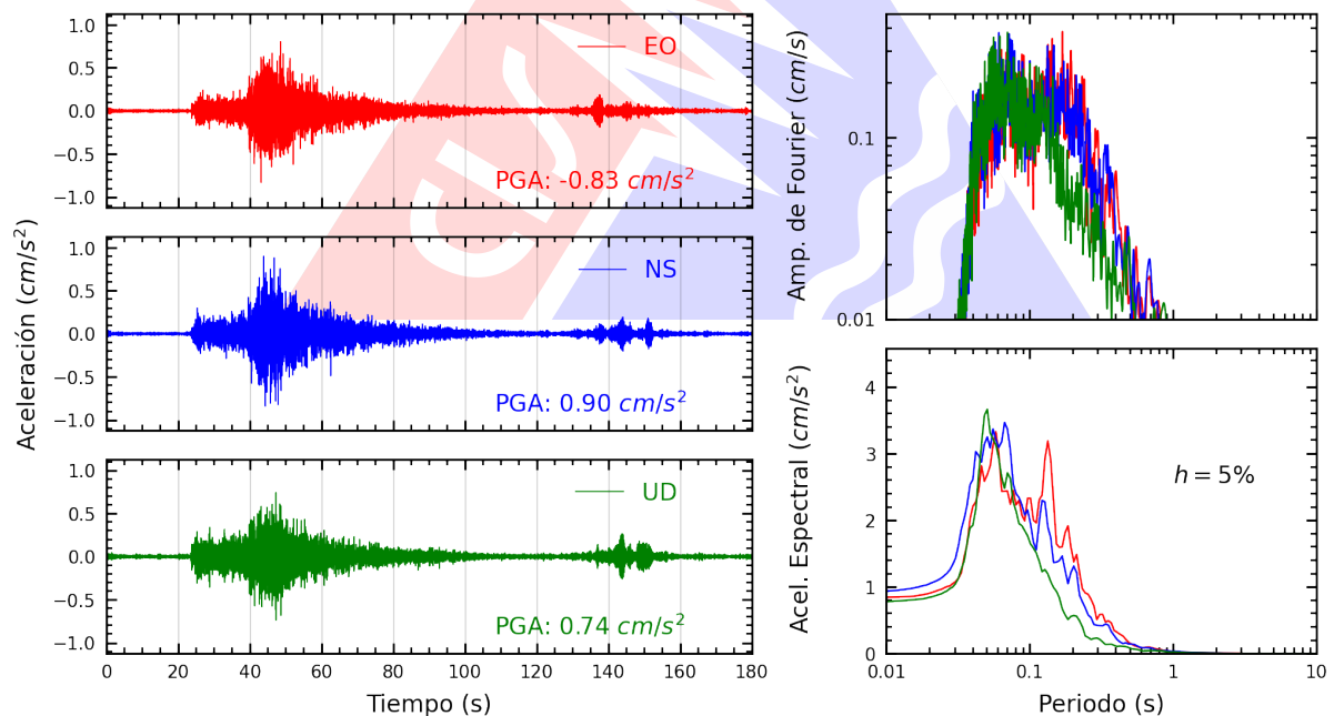
Figura A.2: Registros tiempo-historia, espectros de Fourier y de respuesta en las direcciones EO, NS y vertical de la estación ASIA. Sismo de La Tinguña, Ica - Ica del 2025-04-20, 17:03:32 (Hora local)
