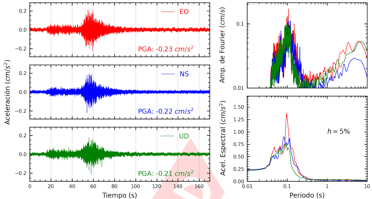
Figura A.9: Registros tiempo-historia, espectros de Fourier y de respuesta en las direcciones EO, NS y vertical de la estación AMORE. Sismo de Ica, Ica - Ica del 2025-04-21, 05:13:45 (Hora local)
