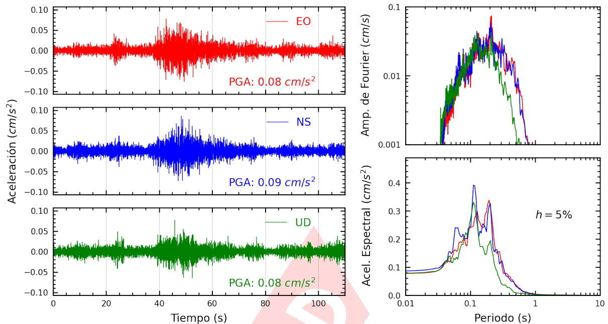
Figura A.17: Registros tiempo-historia, espectros de Fourier y de respuesta en las direcciones EO, NS y vertical de la estación VHAY2. Sismo de Ica, Ica - Ica del 2025-04-21, 05:13:45 (Hora local)
