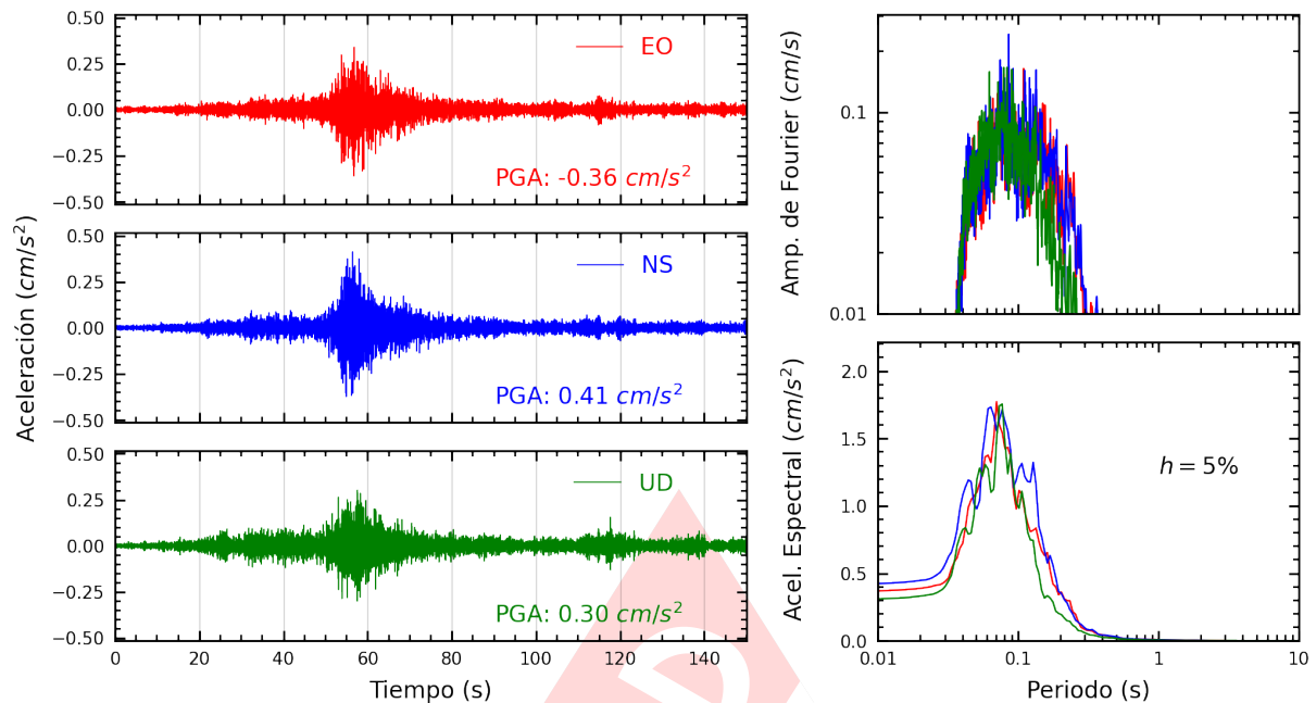
Figura A.3: Registros tiempo-historia, espectros de Fourier y de respuesta en las direcciones EO, NS y vertical de la estación ASIA. Sismo de Ica, Ica - Ica del 2025-04-21, 05:13:45 (Hora local)
