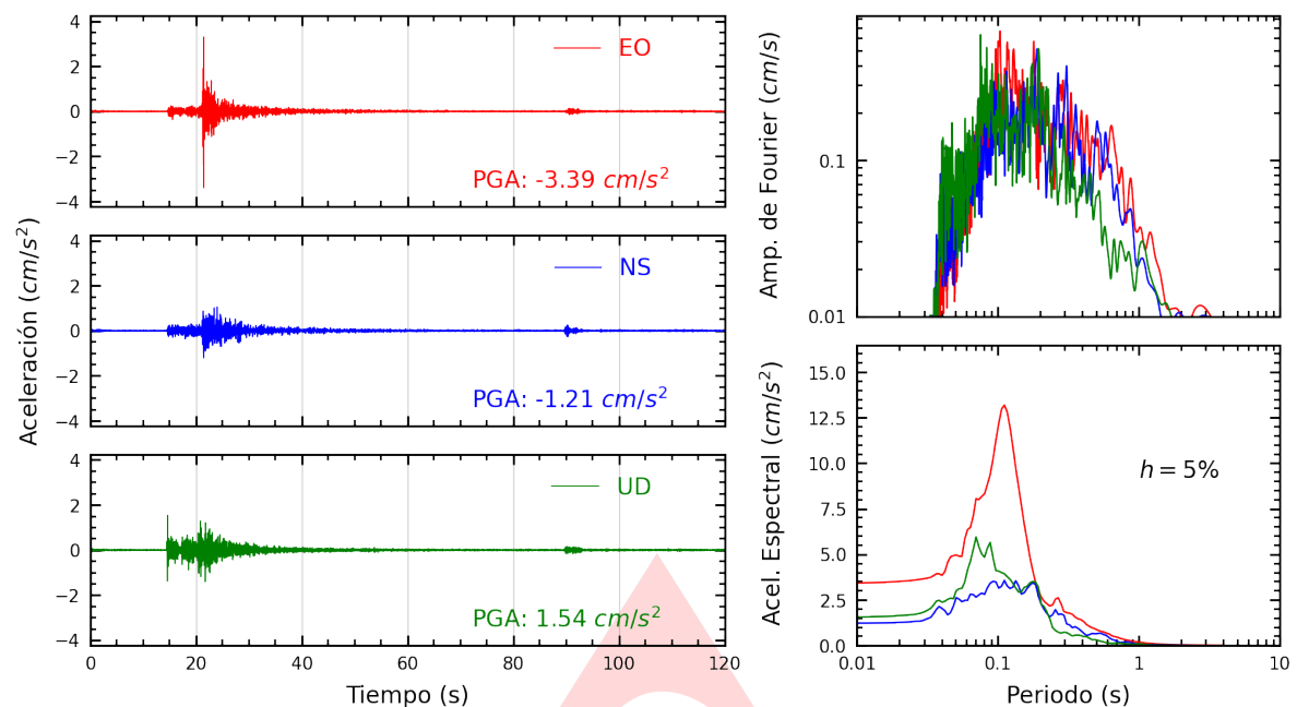
Figura A.1: Registros tiempo-historia, espectros de Fourier y de respuesta en las direcciones EO, NS y vertical de la estación UNICA. Sismo de Ica, Ica - Ica del 2025-04-21, 05:13:45 (Hora local)
