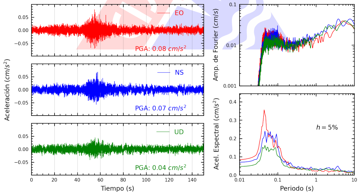
Figura A.18: Registros tiempo-historia, espectros de Fourier y de respuesta en las direcciones EO, NS y vertical de la estación UCSS. Sismo de Ica, Ica - Ica del 2025-04-21, 05:13:45 (Hora local)
