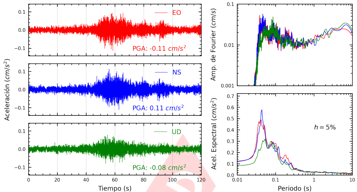
Figura A.15: Registros tiempo-historia, espectros de Fourier y de respuesta en las direcciones EO, NS y vertical de la estación COMAS. Sismo de Ica, Ica - Ica del 2025-04-21, 05:13:45 (Hora local)
