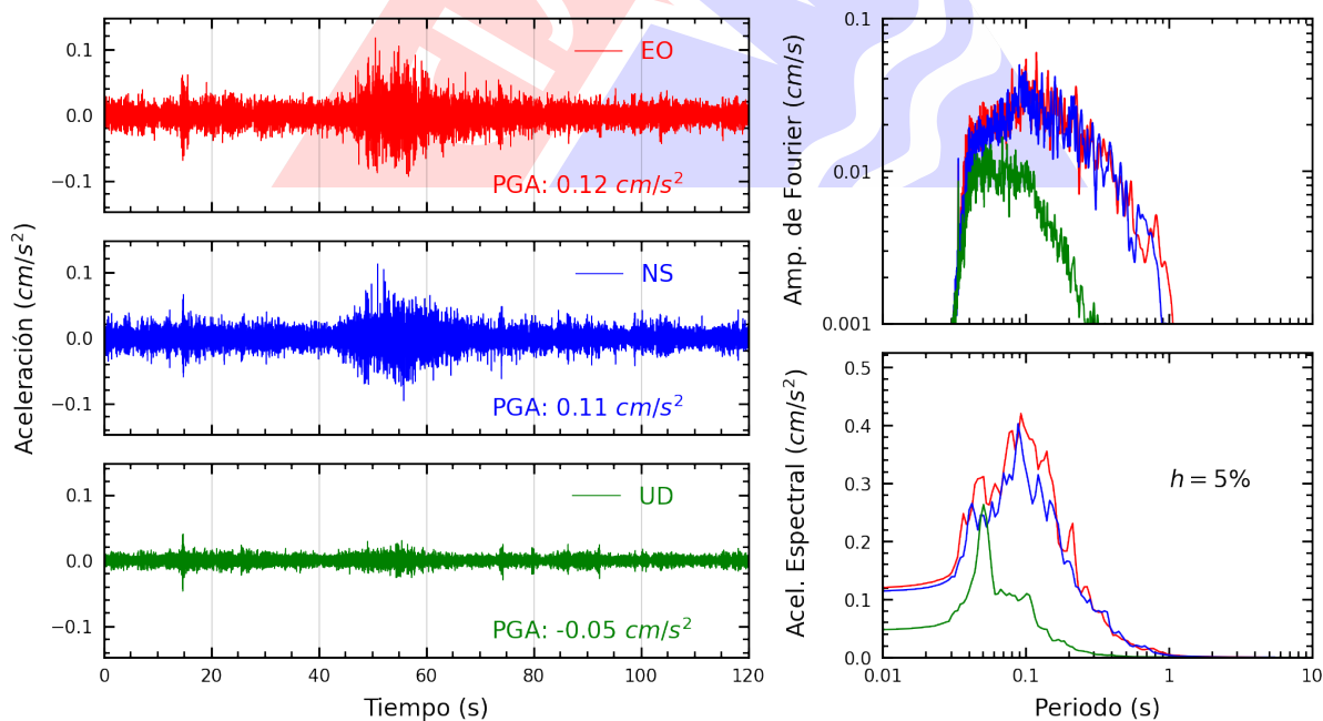
Figura A.14: Registros tiempo-historia, espectros de Fourier y de respuesta en las direcciones EO, NS y vertical de la estación UCVA2. Sismo de Ica, Ica - Ica del 2025-04-21, 05:13:45 (Hora local)
