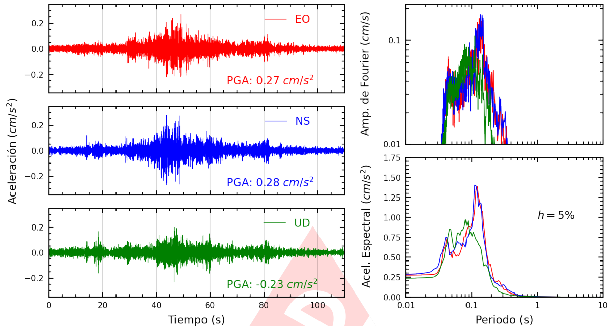
Figura A.7: Registros tiempo-historia, espectros de Fourier y de respuesta en las direcciones EO, NS y vertical de la estación CARA2. Sismo de Ica, Ica - Ica del 2025-04-21, 05:13:45 (Hora local)
