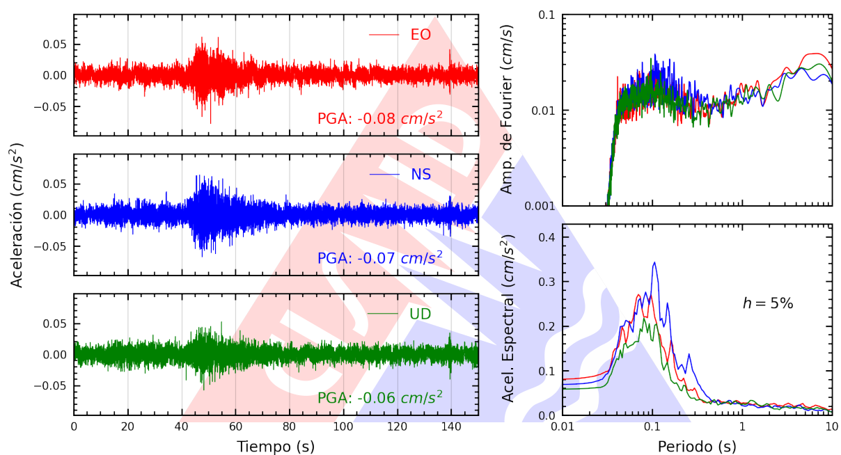
Figura A.19: Registros tiempo-historia, espectros de Fourier y de respuesta en las direcciones EO, NS y vertical de la estación SERVI. Sismo de Ica, Ica - Ica del 2025-04-21, 05:13:45 (Hora local)
