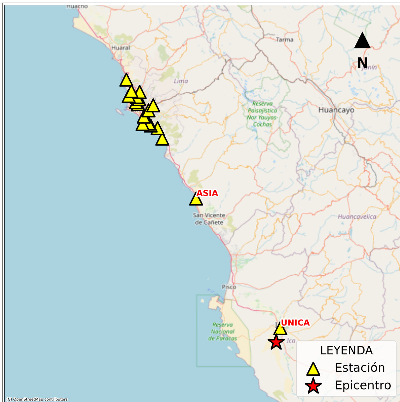
Figura 2: Mapa de ubicación de la(s) estación(es) acelerográfica(s) a nivel nacional correspondiente(s) al Sismo de Ica, Ica - Ica del 21 de abril de 2025 a las 05:13:45 (hora local)
