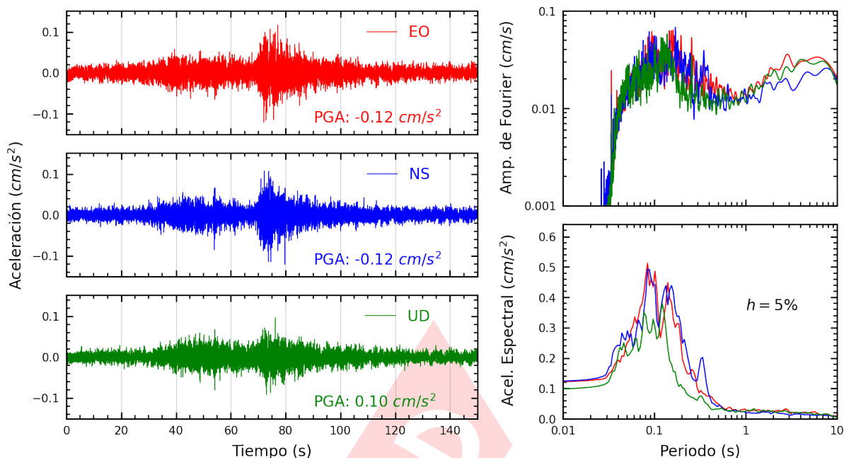
Figura A.13: Registros tiempo-historia, espectros de Fourier y de respuesta en las direcciones EO, NS y vertical de la estación USILP. Sismo de Ica, Ica - Ica del 2025-04-21, 05:13:45 (Hora local)
