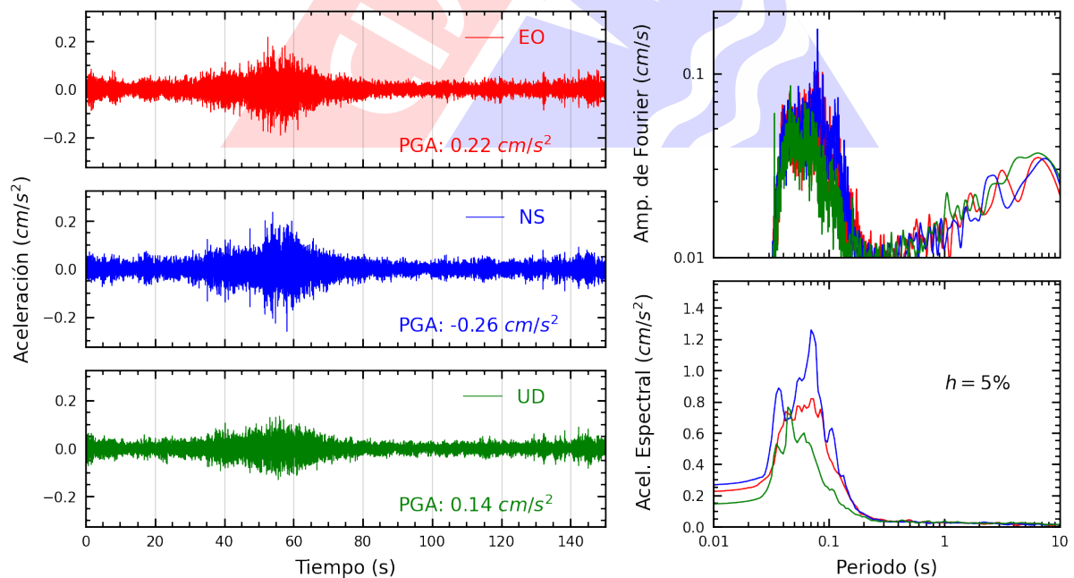
Figura A.8: Registros tiempo-historia, espectros de Fourier y de respuesta en las direcciones EO, NS y vertical de la estación JOSEO. Sismo de Ica, Ica - Ica del 2025-04-21, 05:13:45 (Hora local)
