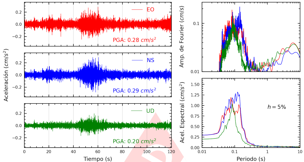
Figura A.5: Registros tiempo-historia, espectros de Fourier y de respuesta en las direcciones EO, NS y vertical de la estación USILM. Sismo de Ica, Ica - Ica del 2025-04-21, 05:13:45 (Hora local)
