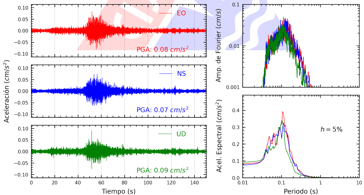
Figura A.16: Registros tiempo-historia, espectros de Fourier y de respuesta en las direcciones EO, NS y vertical de la estación JALV2. Sismo de Ica, Ica - Ica del 2025-04-21, 05:13:45 (Hora local)
