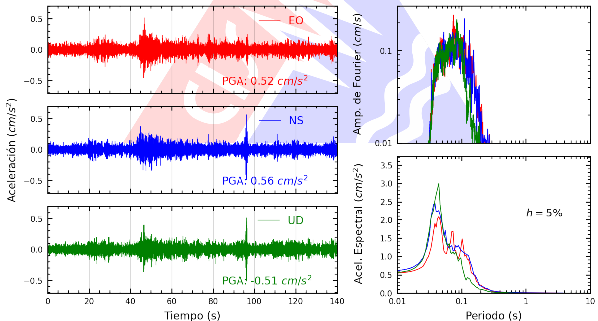
Figura A.2: Registros tiempo-historia, espectros de Fourier y de respuesta en las direcciones EO, NS y vertical de la estación SROS2. Sismo de Ica, Ica - Ica del 2025-04-21, 05:13:45 (Hora local)
