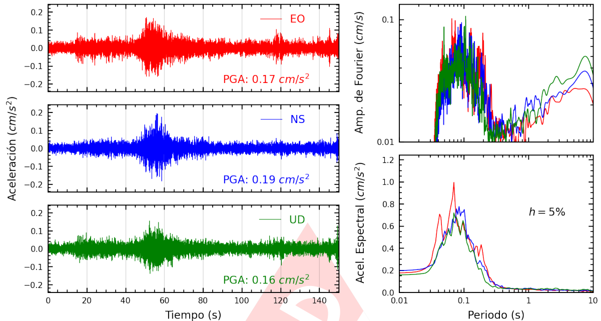
Figura A.11: Registros tiempo-historia, espectros de Fourier y de respuesta en las direcciones EO, NS y vertical de la estación INDEP. Sismo de Ica, Ica - Ica del 2025-04-21, 05:13:45 (Hora local)
