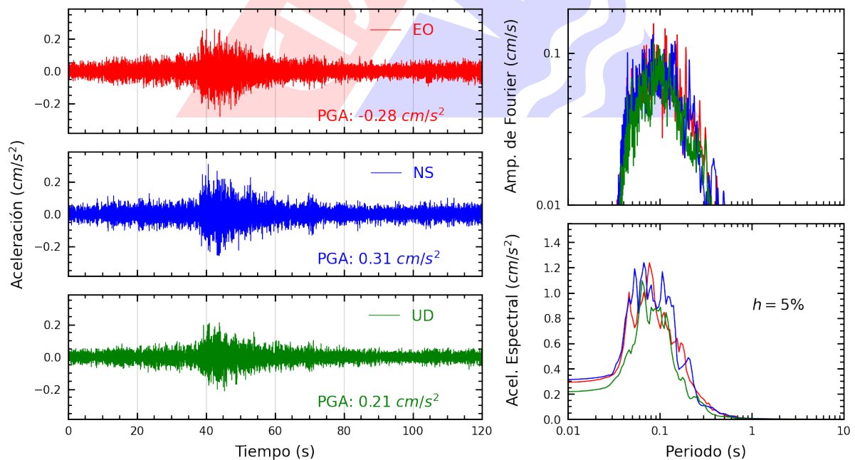
Figura A.4: Registros tiempo-historia, espectros de Fourier y de respuesta en las direcciones EO, NS y vertical de la estación PHER2. Sismo de Ica, Ica - Ica del 2025-04-21, 05:13:45 (Hora local)
