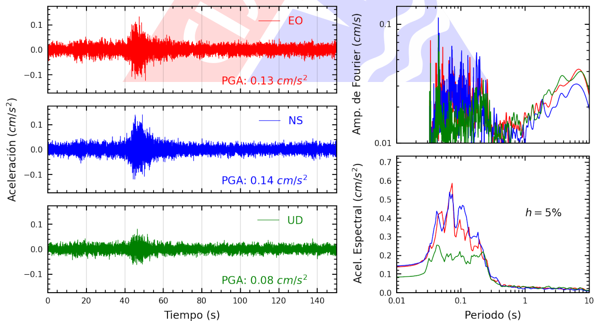
Figura A.12: Registros tiempo-historia, espectros de Fourier y de respuesta en las direcciones EO, NS y vertical de la estación UPCVI. Sismo de Ica, Ica - Ica del 2025-04-21, 05:13:45 (Hora local)
