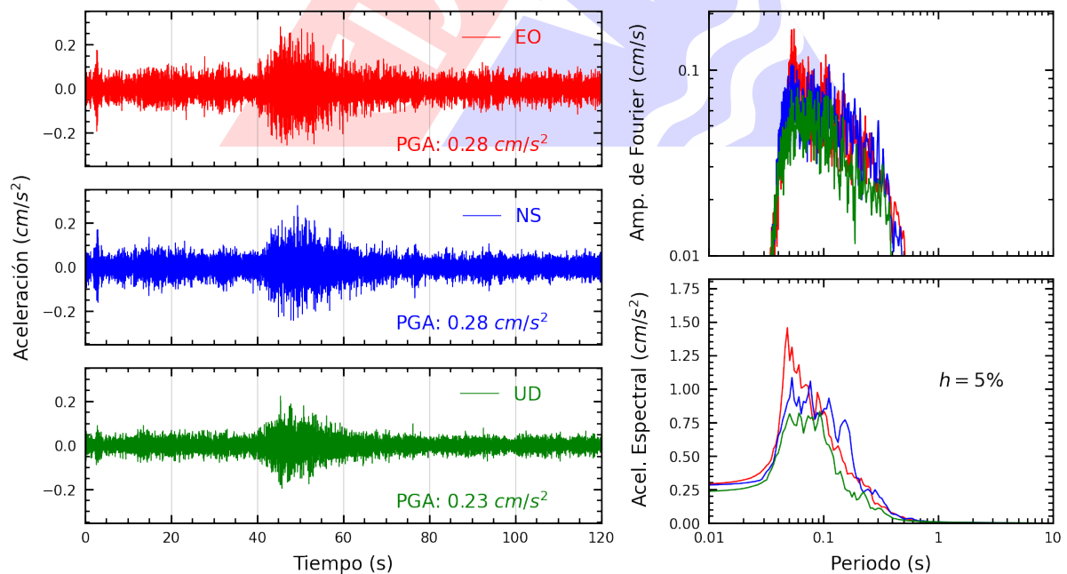
Figura A.6: Registros tiempo-historia, espectros de Fourier y de respuesta en las direcciones EO, NS y vertical de la estación UNTEL. Sismo de Ica, Ica - Ica del 2025-04-21, 05:13:45 (Hora local)
