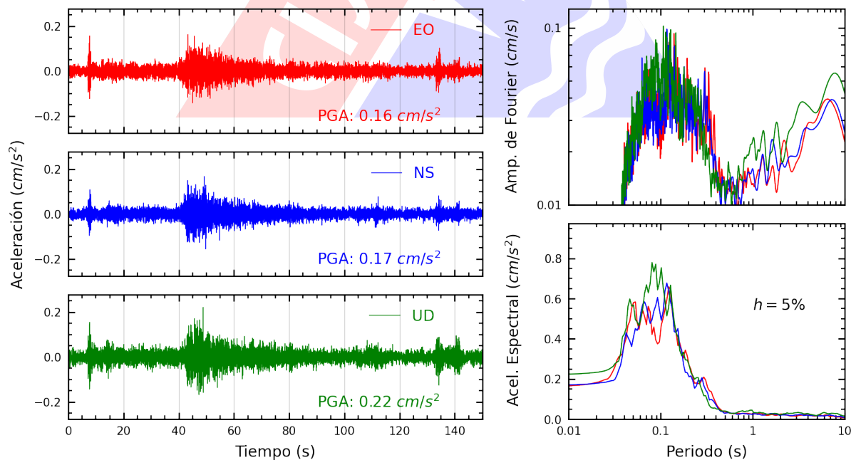
Figura A.10: Registros tiempo-historia, espectros de Fourier y de respuesta en las direcciones EO, NS y vertical de la estación SOVES. Sismo de Ica, Ica - Ica del 2025-04-21, 05:13:45 (Hora local)
