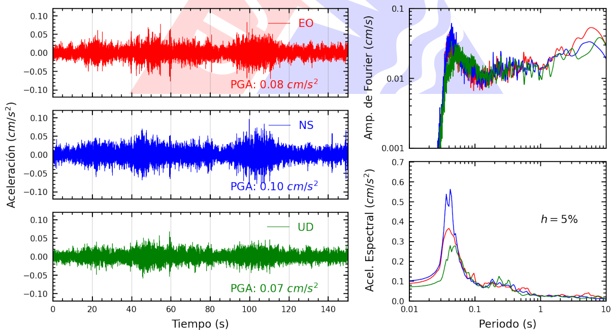
Figura A.4: Registros tiempo-historia, espectros de Fourier y de respuesta en las direcciones EO, NS y vertical de la estación COMAS. Sismo de Tingo Maria, Leoncio Prado - Huanuco del 2025-04-21, 19:35:25 (Hora local)
