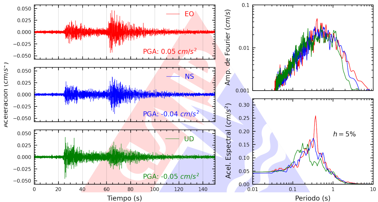
Figura A.5: Registros tiempo-historia, espectros de Fourier y de respuesta en las direcciones EO, NS y vertical de la estación UNCP. Sismo de Tingo Maria, Leoncio Prado - Huanuco del 2025-04-21, 19:35:25 (Hora local)
