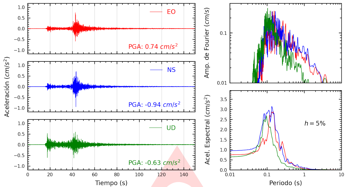
Figura A.1: Registros tiempo-historia, espectros de Fourier y de respuesta en las direcciones EO, NS y vertical de la estación UNIA. Sismo de Tingo Maria, Leoncio Prado - Huanuco del 2025-04-21, 19:35:25 (Hora local)
