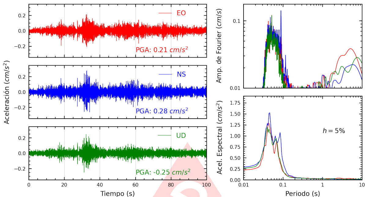
Figura A.3: Registros tiempo-historia, espectros de Fourier y de respuesta en las direcciones EO, NS y vertical de la estación JOSEO. Sismo de Tingo Maria, Leoncio Prado - Huanuco del 2025-04-21, 19:35:25 (Hora local)
