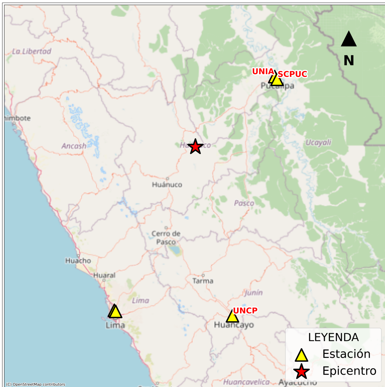
Figura 2: Mapa de ubicación de la(s) estación(es) acelerográfica(s) a nivel nacional correspondiente(s) al Sismo de Tingo Maria, Leoncio Prado - Huanuco del 21 de abril de 2025 a las 19:35:25 (hora local)
