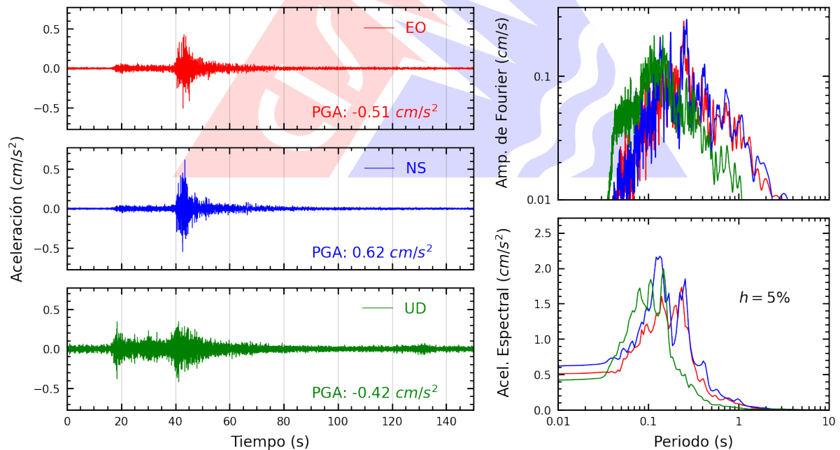
Figura A.2: Registros tiempo-historia, espectros de Fourier y de respuesta en las direcciones EO, NS y vertical de la estación SCPUC. Sismo de Tingo Maria, Leoncio Prado - Huanuco del 2025-04-21, 19:35:25 (Hora local)
