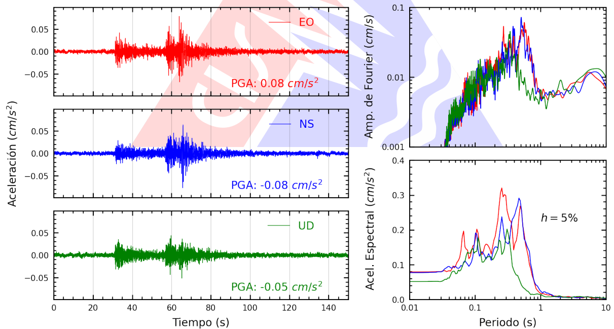
Figura A.2: Registros tiempo-historia, espectros de Fourier y de respuesta en las direcciones EO, NS y vertical de la estación CARAL. Sismo de Pozuzo, Oxapampa - Pasco del 2025-04-25, 06:15:54 (Hora local)
