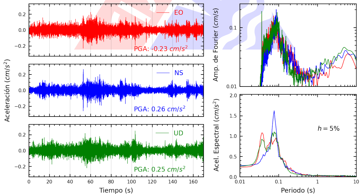
Figura A.4: Registros tiempo-historia, espectros de Fourier y de respuesta en las direcciones EO, NS y vertical de la estación INDEP. Sismo de Chimbote, Santa - Ancash del 2025-04-25, 14:24:59 (Hora local)
