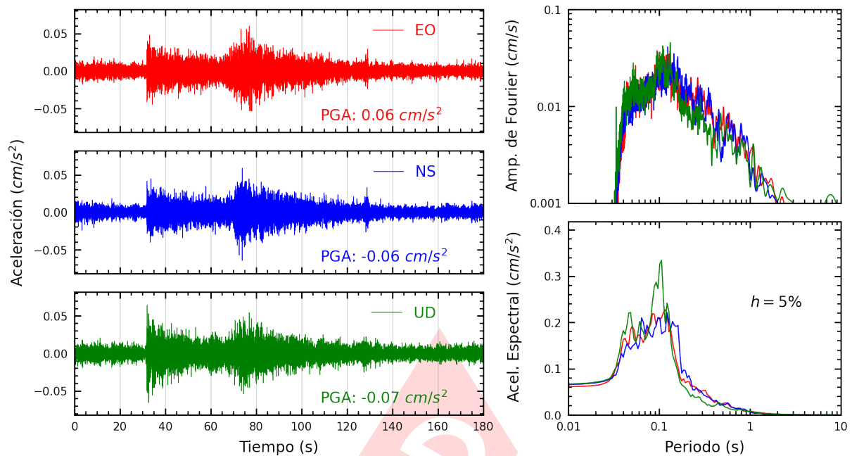
Figura A.11: Registros tiempo-historia, espectros de Fourier y de respuesta en las direcciones EO, NS y vertical de la estación JALV2. Sismo de Chimbote, Santa - Ancash del 2025-04-25, 14:24:59 (Hora local)
