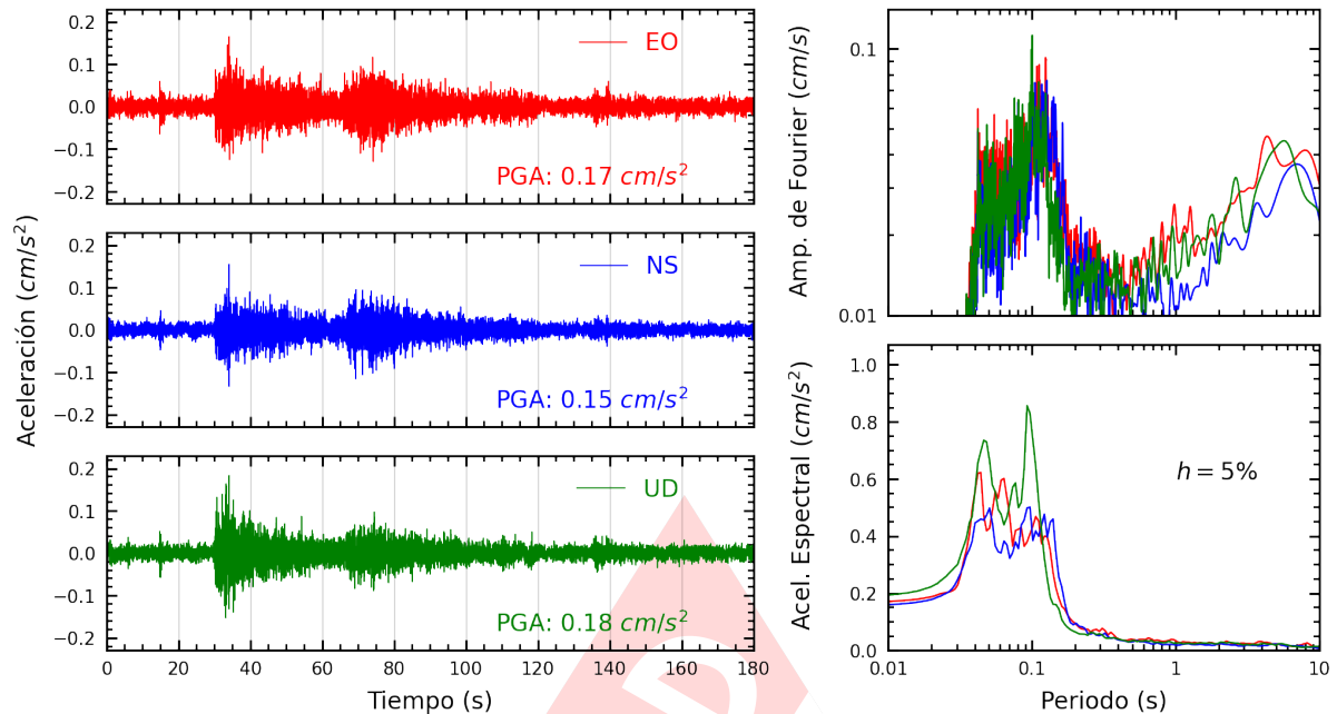
Figura A.7: Registros tiempo-historia, espectros de Fourier y de respuesta en las direcciones EO, NS y vertical de la estación AMORE. Sismo de Chimbote, Santa - Ancash del 2025-04-25, 14:24:59 (Hora local)
