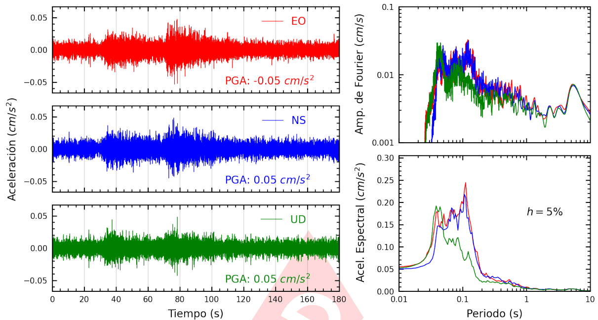
Figura A.13: Registros tiempo-historia, espectros de Fourier y de respuesta en las direcciones EO, NS y vertical de la estación ATARJ. Sismo de Chimbote, Santa - Ancash del 2025-04-25, 14:24:59 (Hora local)
