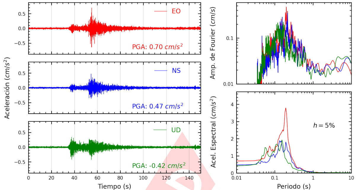
Figura A.3: Registros tiempo-historia, espectros de Fourier y de respuesta en las direcciones EO, NS y vertical de la estación UPAOT. Sismo de Chimbote, Santa - Ancash del 2025-04-25, 14:24:59 (Hora local)
