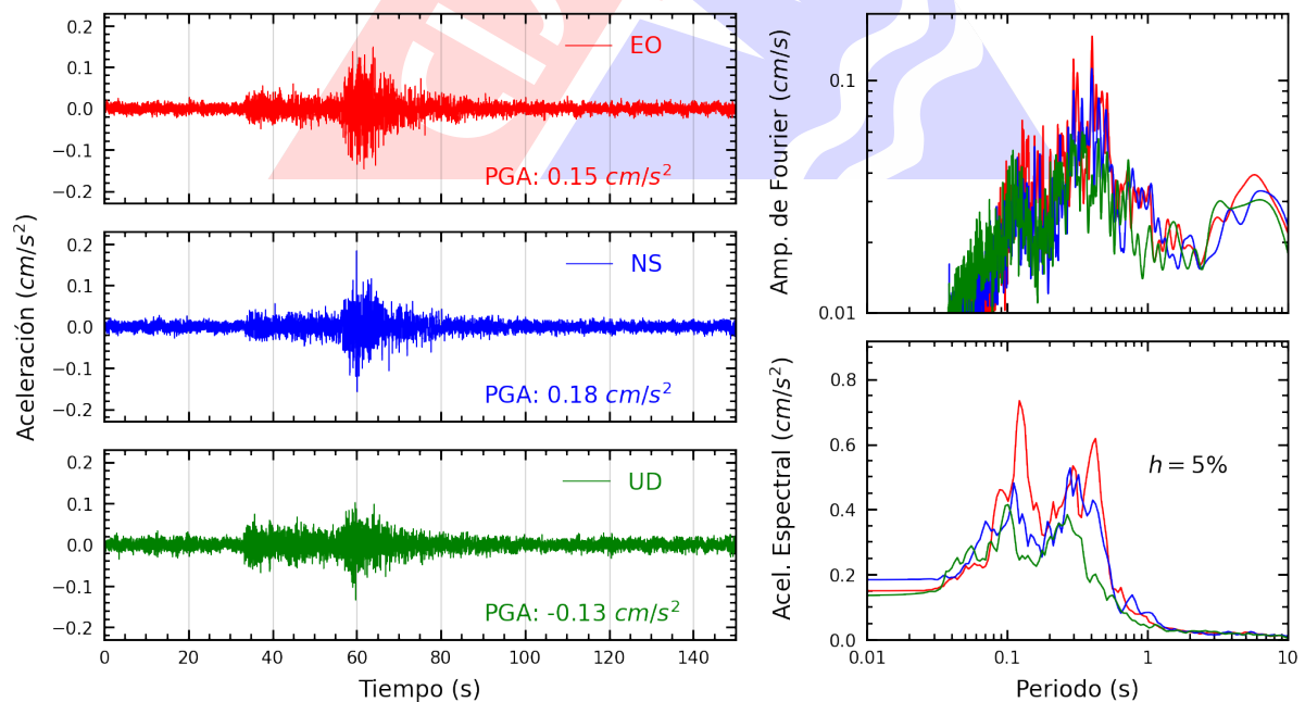
Figura A.6: Registros tiempo-historia, espectros de Fourier y de respuesta en las direcciones EO, NS y vertical de la estación UNASA. Sismo de Chimbote, Santa - Ancash del 2025-04-25, 14:24:59 (Hora local)
