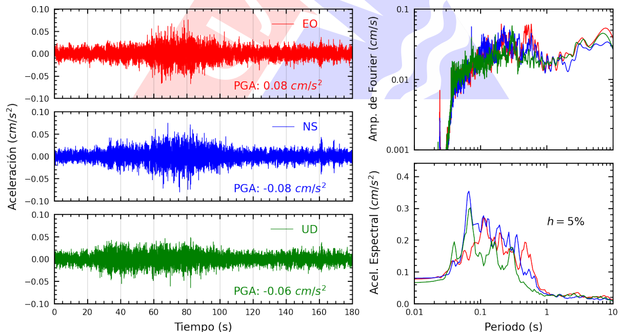
Figura A.10: Registros tiempo-historia, espectros de Fourier y de respuesta en las direcciones EO, NS y vertical de la estación UCVCH. Sismo de Chimbote, Santa - Ancash del 2025-04-25, 14:24:59 (Hora local)
