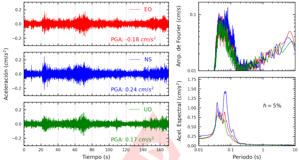
Figura A.5: Registros tiempo-historia, espectros de Fourier y de respuesta en las direcciones EO, NS y vertical de la estación JOSEO. Sismo de Chimbote, Santa - Ancash del 2025-04-25, 14:24:59 (Hora local)
