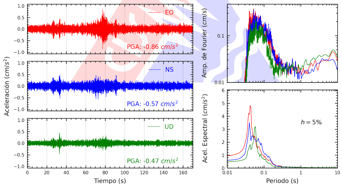
Figura A.2: Registros tiempo-historia, espectros de Fourier y de respuesta en las direcciones EO, NS y vertical de la estación USILM. Sismo de Chimbote, Santa - Ancash del 2025-04-25, 14:24:59 (Hora local)
