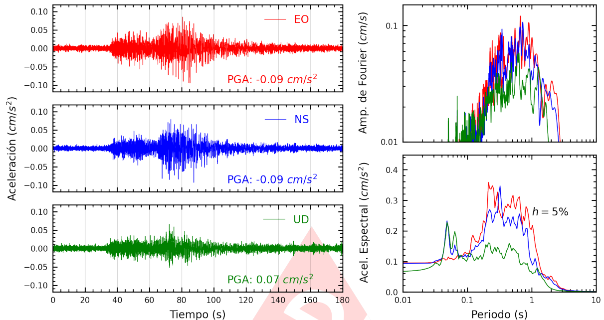
Figura A.9: Registros tiempo-historia, espectros de Fourier y de respuesta en las direcciones EO, NS y vertical de la estación UNC. Sismo de Chimbote, Santa - Ancash del 2025-04-25, 14:24:59 (Hora local)
