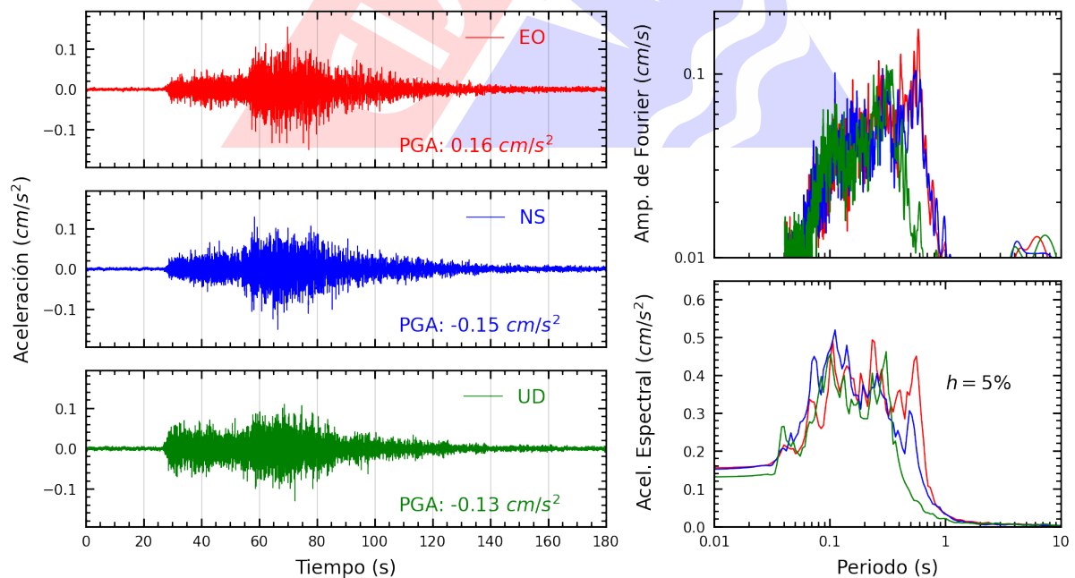
Figura A.8: Registros tiempo-historia, espectros de Fourier y de respuesta en las direcciones EO, NS y vertical de la estación CARAL. Sismo de Chimbote, Santa - Ancash del 2025-04-25, 14:24:59 (Hora local)
