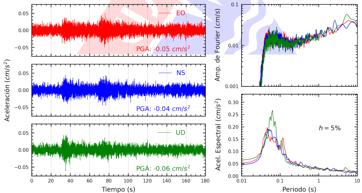
Figura A.12: Registros tiempo-historia, espectros de Fourier y de respuesta en las direcciones EO, NS y vertical de la estación UCSS. Sismo de Chimbote, Santa - Ancash del 2025-04-25, 14:24:59 (Hora local)
