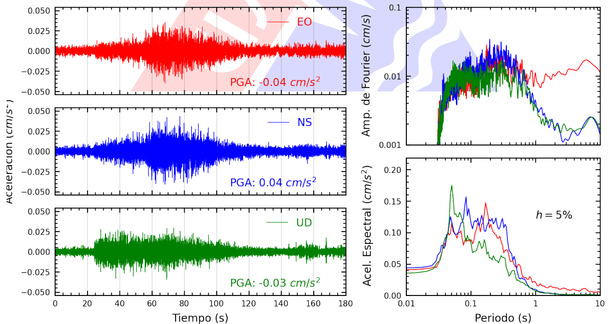
Figura A.14: Registros tiempo-historia, espectros de Fourier y de respuesta en las direcciones EO, NS y vertical de la estación SCCHI. Sismo de Chimbote, Santa - Ancash del 2025-04-25, 14:24:59 (Hora local)
