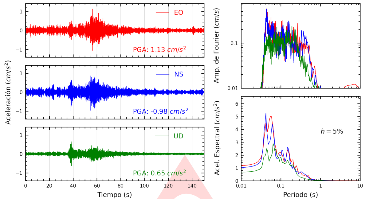
Figura A.1: Registros tiempo-historia, espectros de Fourier y de respuesta en las direcciones EO, NS y vertical de la estación SCTRU. Sismo de Chimbote, Santa - Ancash del 2025-04-25, 14:24:59 (Hora local)
