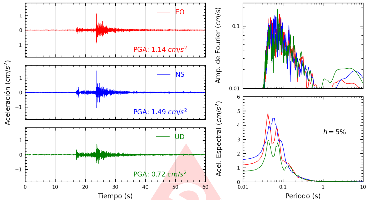
Figura A.25: Registros tiempo-historia, espectros de Fourier y de respuesta en las direcciones EO, NS y vertical de la estación UNFV. Sismo de Chilca, Cañete - Lima del 2025-04-25, 16:21:07 (Hora local)
