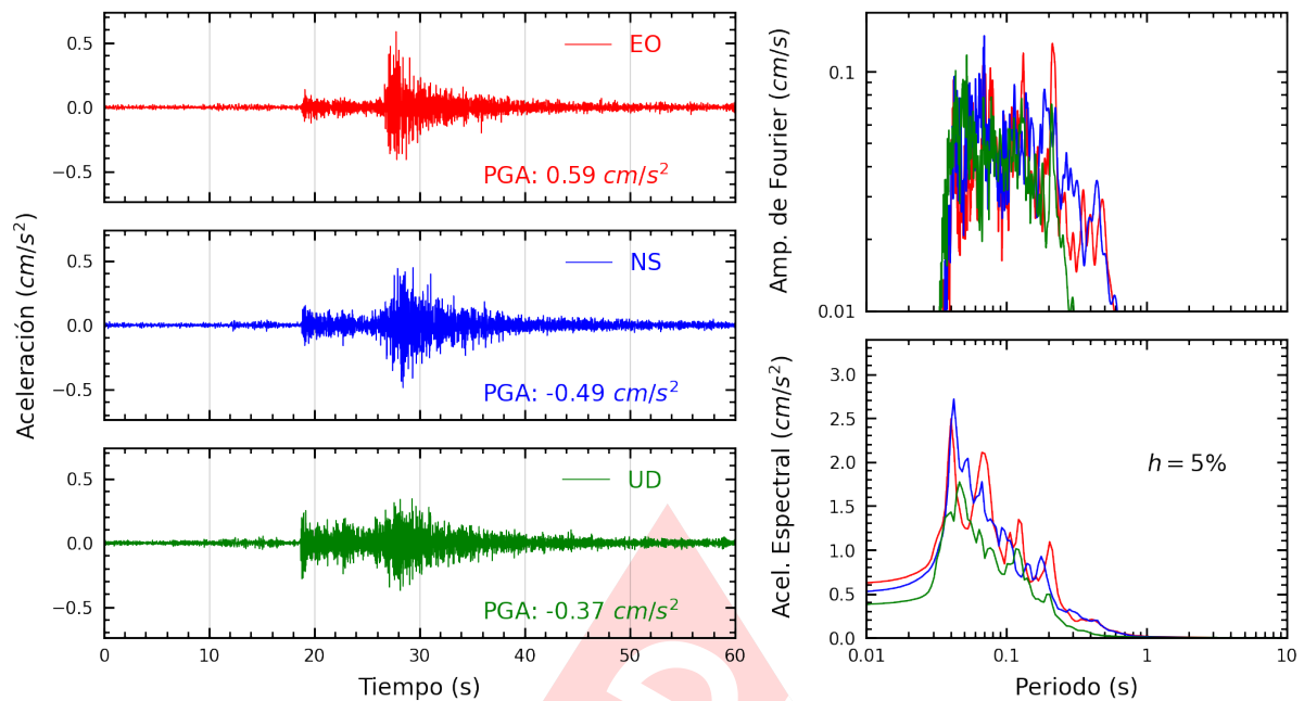
Figura A.39: Registros tiempo-historia, espectros de Fourier y de respuesta en las direcciones EO, NS y vertical de la estación VHAY2. Sismo de Chilca, Cañete - Lima del 2025-04-25, 16:21:07 (Hora local)
