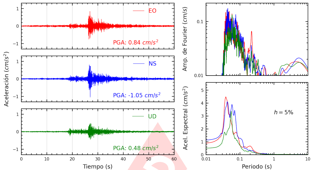
Figura A.31: Registros tiempo-historia, espectros de Fourier y de respuesta en las direcciones EO, NS y vertical de la estación COMAS. Sismo de Chilca, Cañete - Lima del 2025-04-25, 16:21:07 (Hora local)
