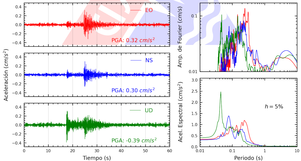
Figura A.40: Registros tiempo-historia, espectros de Fourier y de respuesta en las direcciones EO, NS y vertical de la estación DSMI. Sismo de Chilca, Cañete - Lima del 2025-04-25, 16:21:07 (Hora local)
