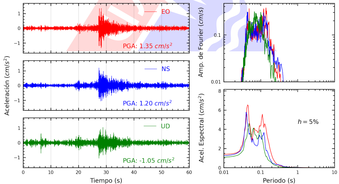
Figura A.26: Registros tiempo-historia, espectros de Fourier y de respuesta en las direcciones EO, NS y vertical de la estación CARA2. Sismo de Chilca, Cañete - Lima del 2025-04-25, 16:21:07 (Hora local)
