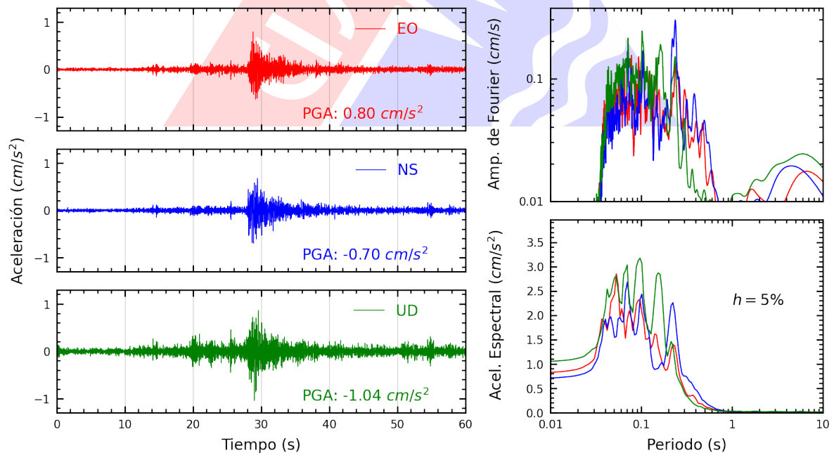
Figura A.32: Registros tiempo-historia, espectros de Fourier y de respuesta en las direcciones EO, NS y vertical de la estación MDPP. Sismo de Chilca, Cañete - Lima del 2025-04-25, 16:21:07 (Hora local)
