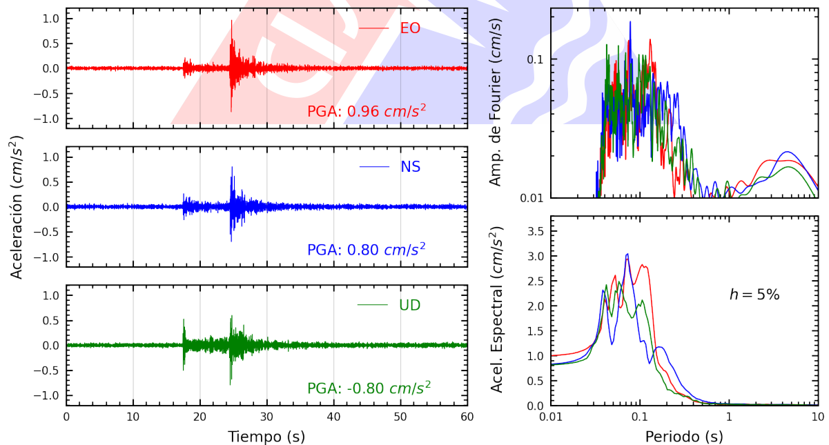
Figura A.34: Registros tiempo-historia, espectros de Fourier y de respuesta en las direcciones EO, NS y vertical de la estación BONDY. Sismo de Chilca, Cañete - Lima del 2025-04-25, 16:21:07 (Hora local)
