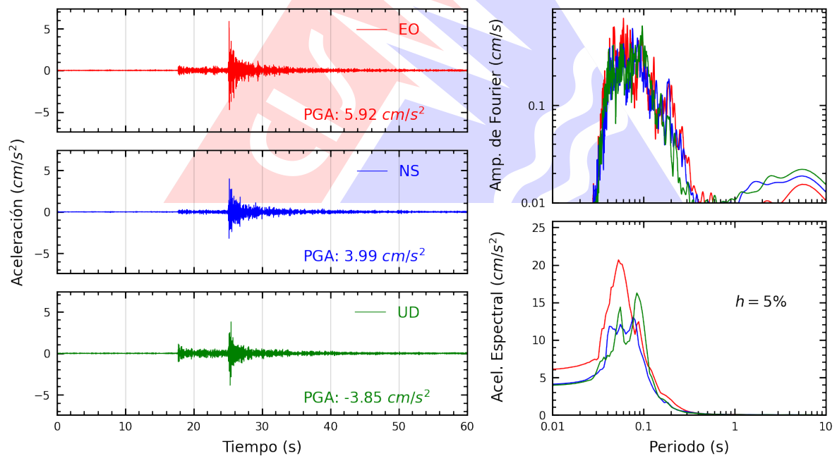
Figura A.2: Registros tiempo-historia, espectros de Fourier y de respuesta en las direcciones EO, NS y vertical de la estación INDEP. Sismo de Chilca, Cañete - Lima del 2025-04-25, 16:21:07 (Hora local)
