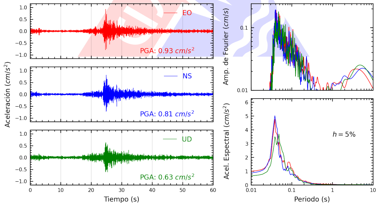
Figura A.36: Registros tiempo-historia, espectros de Fourier y de respuesta en las direcciones EO, NS y vertical de la estación USMP. Sismo de Chilca, Cañete - Lima del 2025-04-25, 16:21:07 (Hora local)
