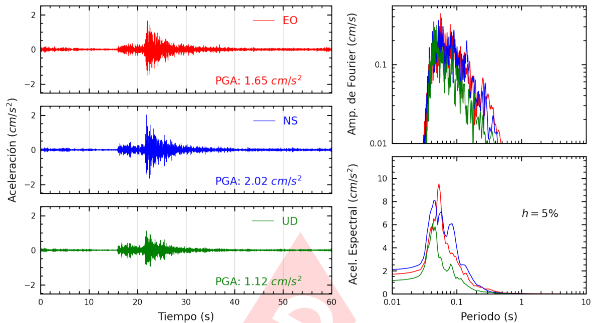
Figura A.15: Registros tiempo-historia, espectros de Fourier y de respuesta en las direcciones EO, NS y vertical de la estación PACHA. Sismo de Chilca, Cañete - Lima del 2025-04-25, 16:21:07 (Hora local)
