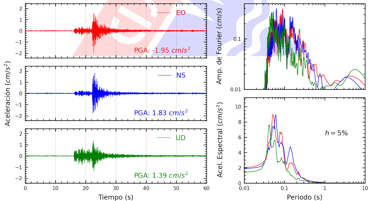
Figura A.16: Registros tiempo-historia, espectros de Fourier y de respuesta en las direcciones EO, NS y vertical de la estación USILP. Sismo de Chilca, Cañete - Lima del 2025-04-25, 16:21:07 (Hora local)
