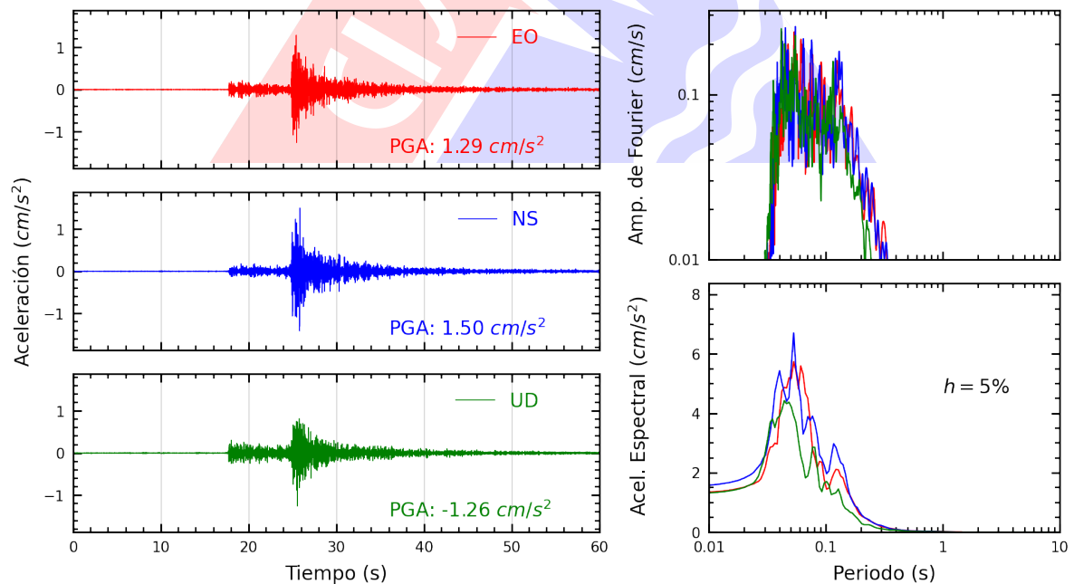
Figura A.24: Registros tiempo-historia, espectros de Fourier y de respuesta en las direcciones EO, NS y vertical de la estación JALV2. Sismo de Chilca, Cañete - Lima del 2025-04-25, 16:21:07 (Hora local)
