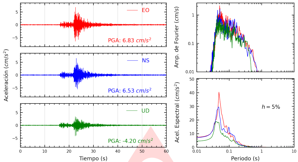
Figura A.1: Registros tiempo-historia, espectros de Fourier y de respuesta en las direcciones EO, NS y vertical de la estación UNTEL. Sismo de Chilca, Cañete - Lima del 2025-04-25, 16:21:07 (Hora local)
