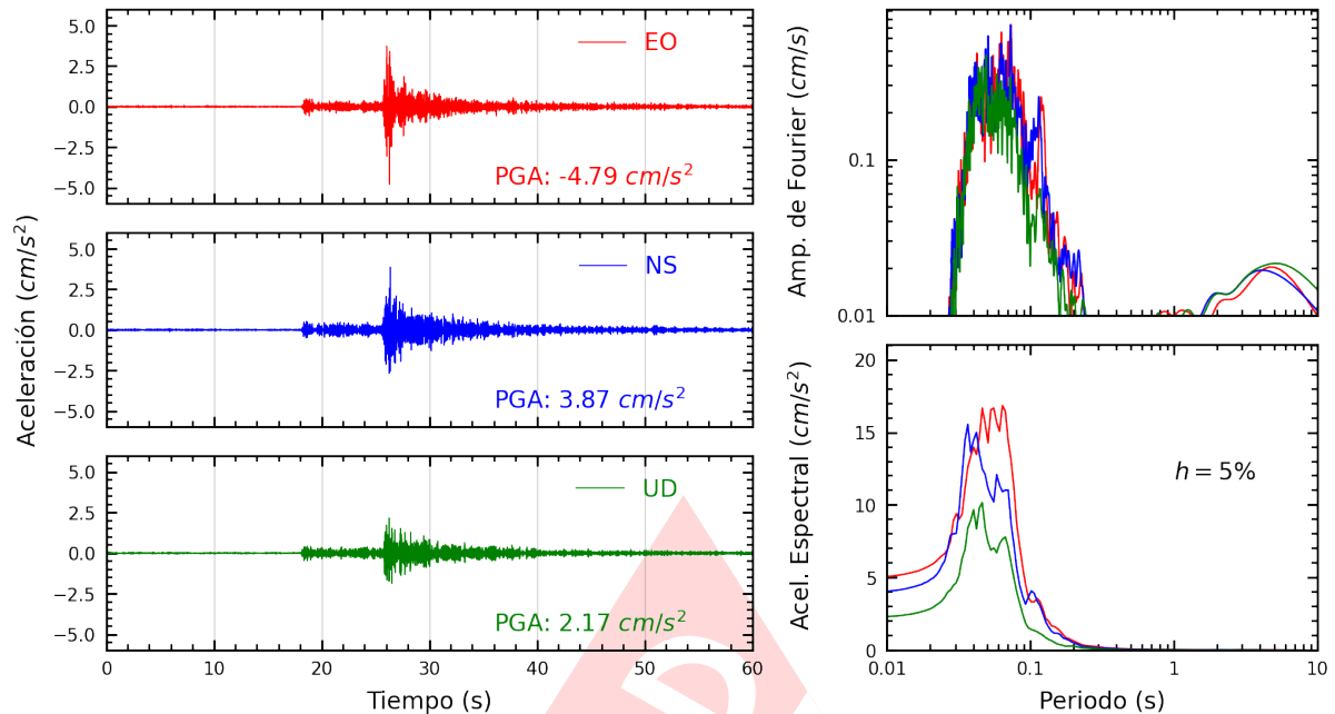
Figura A.3: Registros tiempo-historia, espectros de Fourier y de respuesta en las direcciones EO, NS y vertical de la estación JOSEO. Sismo de Chilca, Cañete - Lima del 2025-04-25, 16:21:07 (Hora local)
