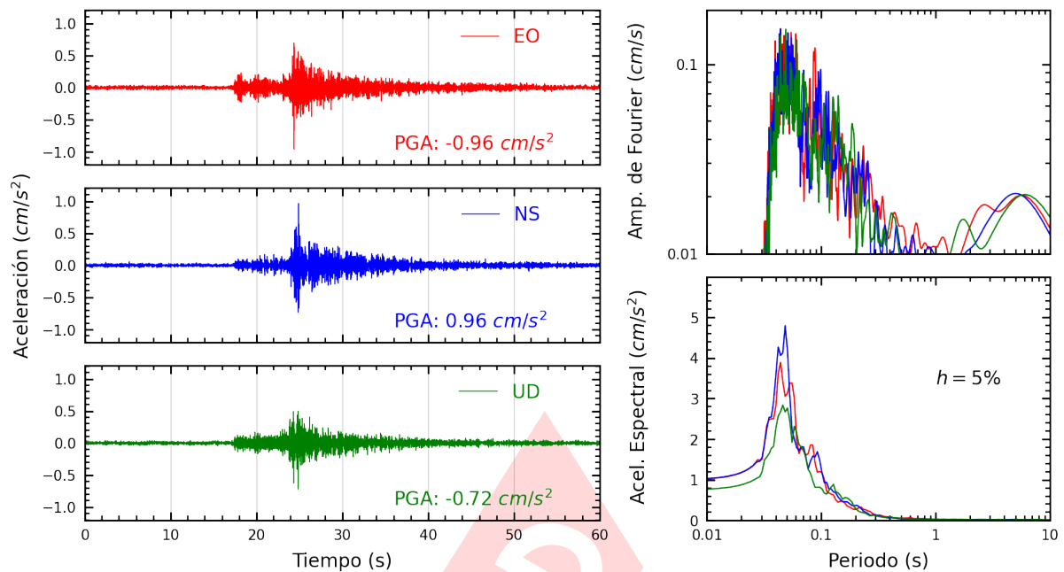
Figura A.33: Registros tiempo-historia, espectros de Fourier y de respuesta en las direcciones EO, NS y vertical de la estación IMCA. Sismo de Chilca, Cañete - Lima del 2025-04-25, 16:21:07 (Hora local)
