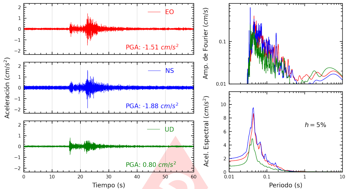
Figura A.17: Registros tiempo-historia, espectros de Fourier y de respuesta en las direcciones EO, NS y vertical de la estación UPCVI. Sismo de Chilca, Cañete - Lima del 2025-04-25, 16:21:07 (Hora local)
