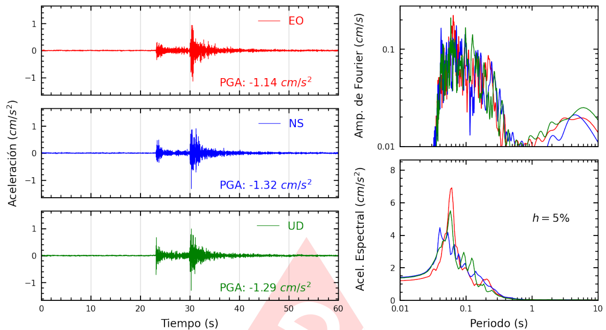
Figura A.27: Registros tiempo-historia, espectros de Fourier y de respuesta en las direcciones EO, NS y vertical de la estación UNMSM. Sismo de Chilca, Cañete - Lima del 2025-04-25, 16:21:07 (Hora local)
