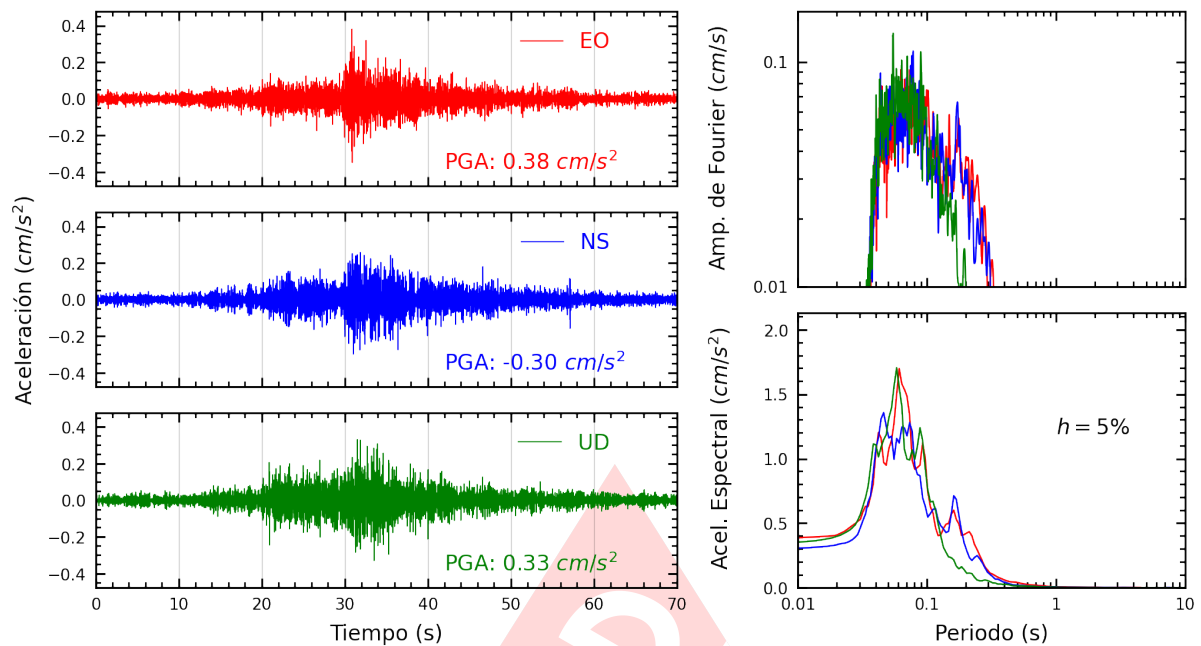
Figura A.41: Registros tiempo-historia, espectros de Fourier y de respuesta en las direcciones EO, NS y vertical de la estación ASIA. Sismo de Chilca, Cañete - Lima del 2025-04-25, 16:21:07 (Hora local)
