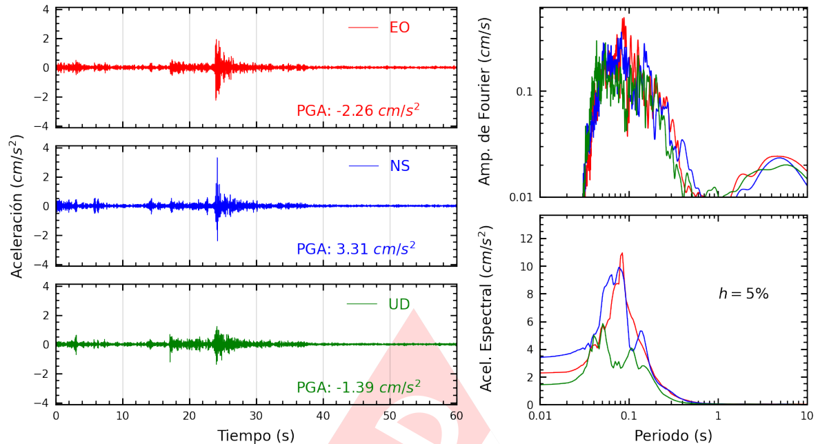
Figura A.7: Registros tiempo-historia, espectros de Fourier y de respuesta en las direcciones EO, NS y vertical de la estación UPCSM. Sismo de Chilca, Cañete - Lima del 2025-04-25, 16:21:07 (Hora local)
