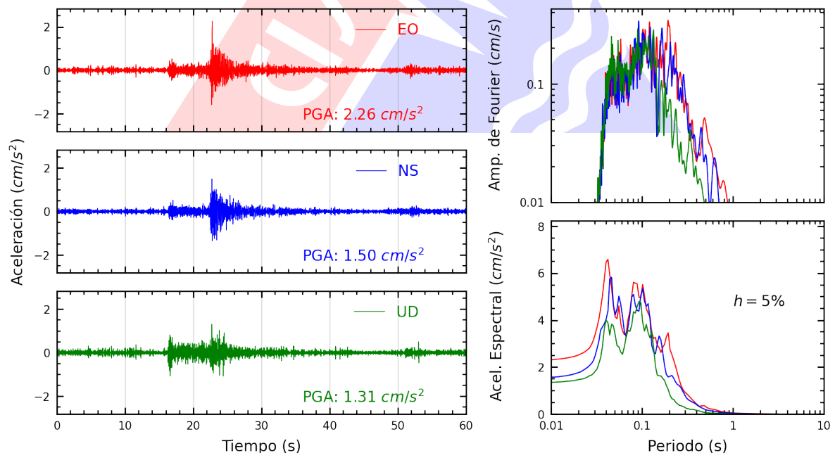
Figura A.10: Registros tiempo-historia, espectros de Fourier y de respuesta en las direcciones EO, NS y vertical de la estación SCCHO. Sismo de Chilca, Cañete - Lima del 2025-04-25, 16:21:07 (Hora local)
