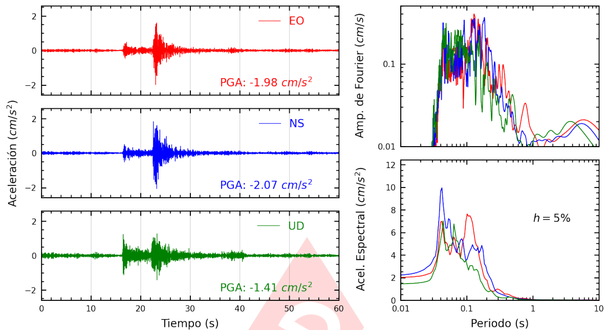
Figura A.13: Registros tiempo-historia, espectros de Fourier y de respuesta en las direcciones EO, NS y vertical de la estación SOCHO. Sismo de Chilca, Cañete - Lima del 2025-04-25, 16:21:07 (Hora local)
