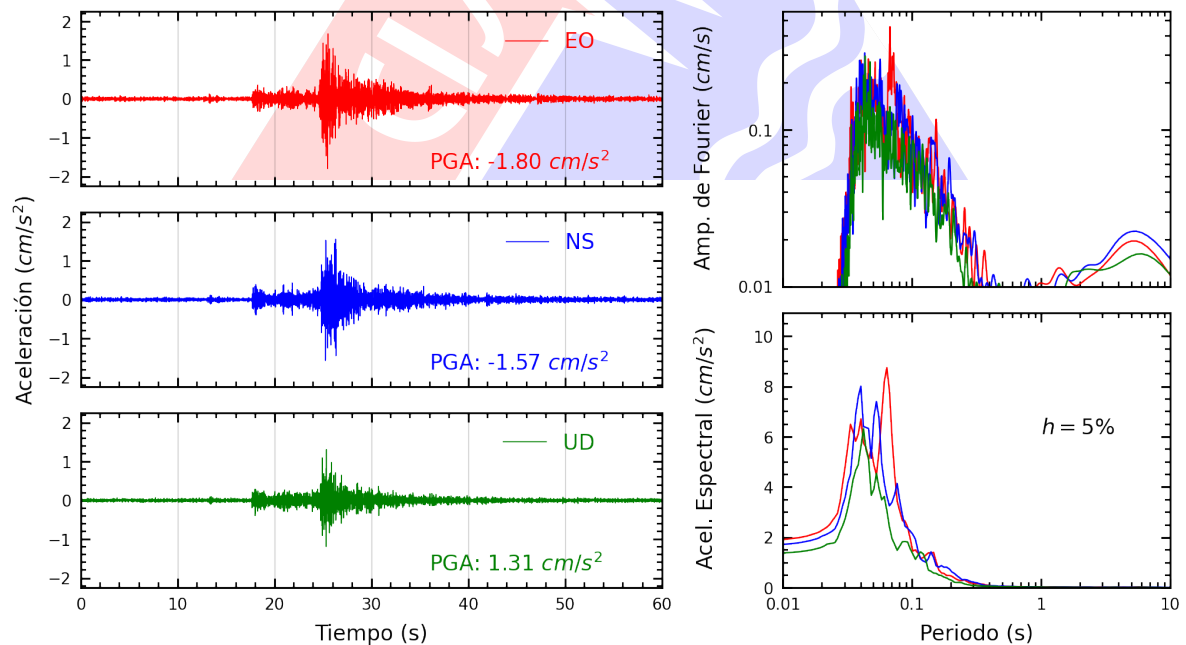
Figura A.20: Registros tiempo-historia, espectros de Fourier y de respuesta en las direcciones EO, NS y vertical de la estación FICPE. Sismo de Chilca, Cañete - Lima del 2025-04-25, 16:21:07 (Hora local)
