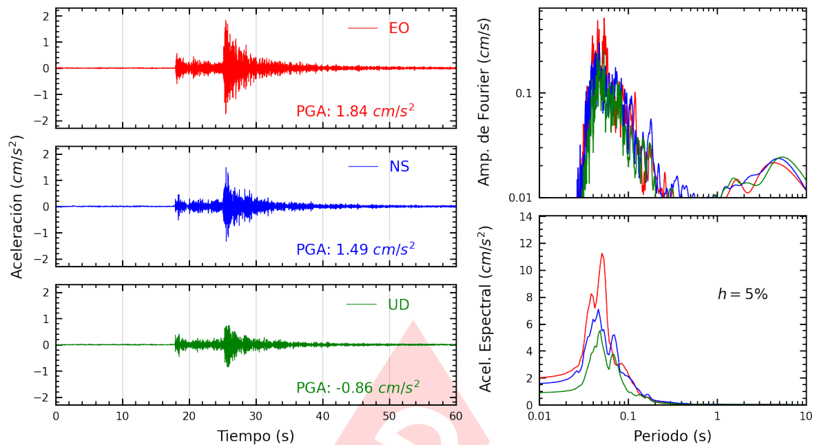
Figura A.19: Registros tiempo-historia, espectros de Fourier y de respuesta en las direcciones EO, NS y vertical de la estación UCSS. Sismo de Chilca, Cañete - Lima del 2025-04-25, 16:21:07 (Hora local)
