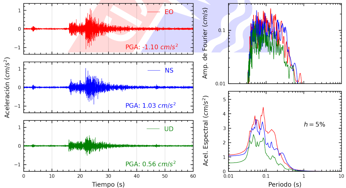
Figura A.30: Registros tiempo-historia, espectros de Fourier y de respuesta en las direcciones EO, NS y vertical de la estación BRISA. Sismo de Chilca, Cañete - Lima del 2025-04-25, 16:21:07 (Hora local)
