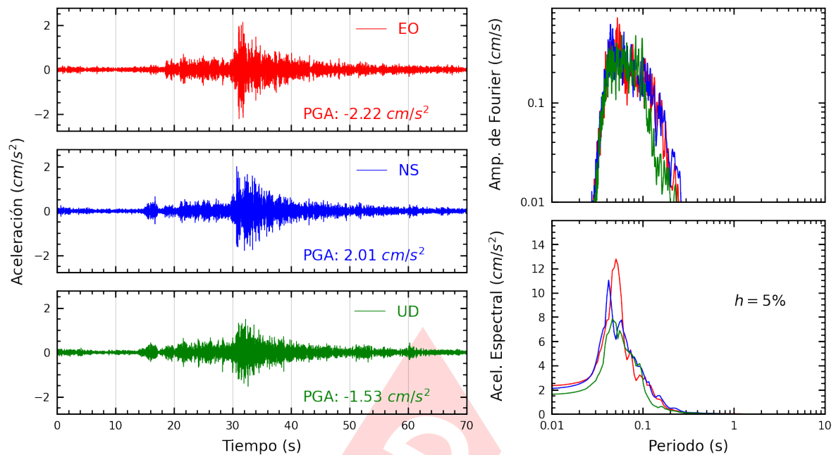
Figura A.11: Registros tiempo-historia, espectros de Fourier y de respuesta en las direcciones EO, NS y vertical de la estación SROS2. Sismo de Chilca, Cañete - Lima del 2025-04-25, 16:21:07 (Hora local)
