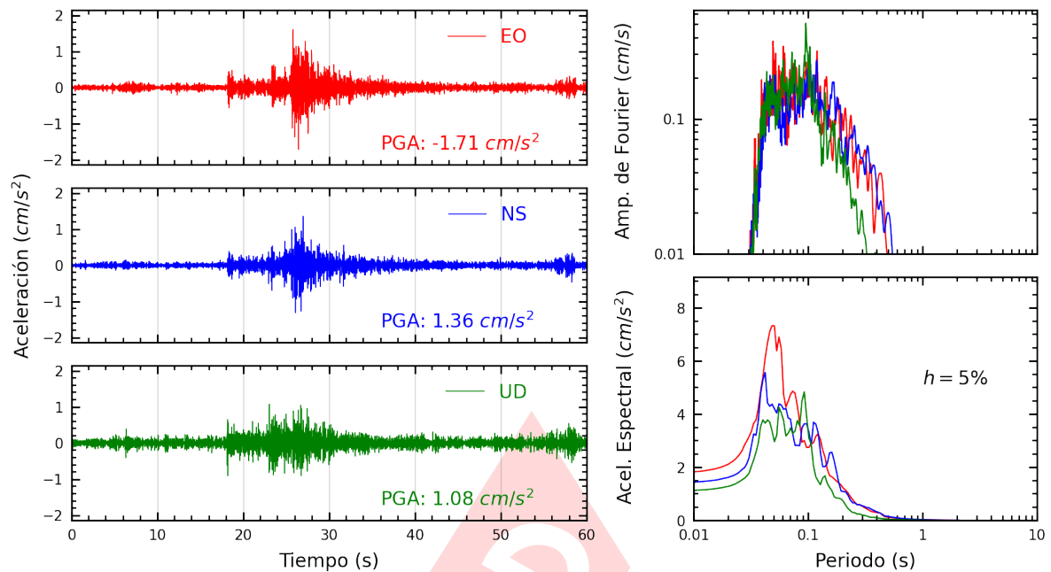
Figura A.23: Registros tiempo-historia, espectros de Fourier y de respuesta en las direcciones EO, NS y vertical de la estación SCOLI. Sismo de Chilca, Cañete - Lima del 2025-04-25, 16:21:07 (Hora local)
