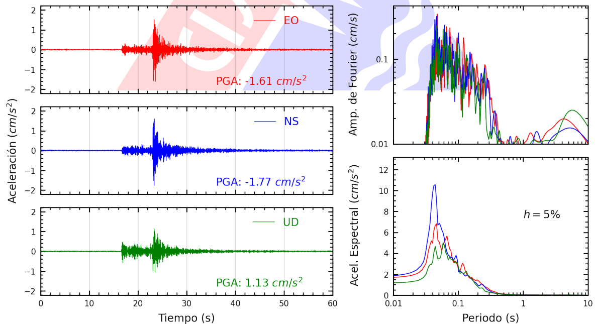
Figura A.22: Registros tiempo-historia, espectros de Fourier y de respuesta en las direcciones EO, NS y vertical de la estación SERVI. Sismo de Chilca, Cañete - Lima del 2025-04-25, 16:21:07 (Hora local)
