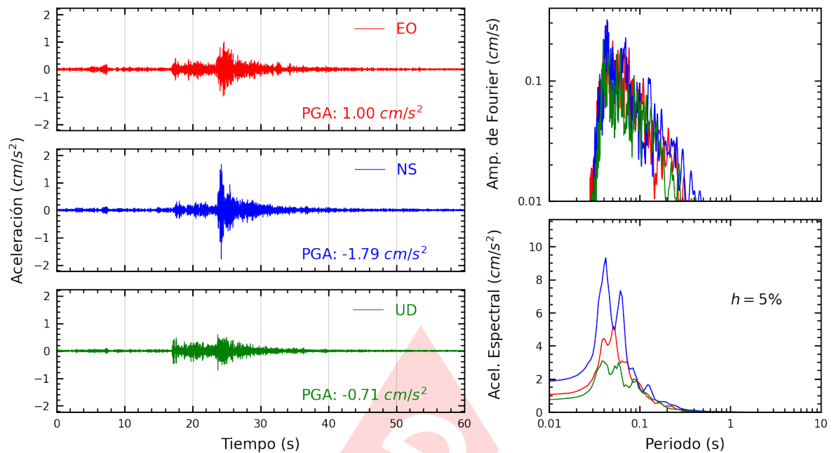
Figura A.21: Registros tiempo-historia, espectros de Fourier y de respuesta en las direcciones EO, NS y vertical de la estación BORJA. Sismo de Chilca, Cañete - Lima del 2025-04-25, 16:21:07 (Hora local)
