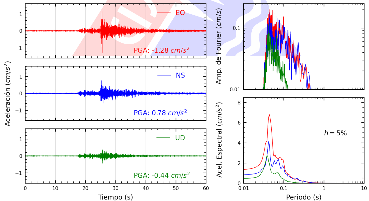
Figura A.28: Registros tiempo-historia, espectros de Fourier y de respuesta en las direcciones EO, NS y vertical de la estación UCVA2. Sismo de Chilca, Cañete - Lima del 2025-04-25, 16:21:07 (Hora local)
