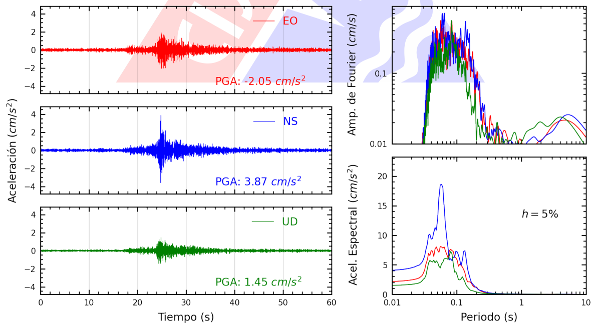
Figura A.6: Registros tiempo-historia, espectros de Fourier y de respuesta en las direcciones EO, NS y vertical de la estación USILM. Sismo de Chilca, Cañete - Lima del 2025-04-25, 16:21:07 (Hora local)
