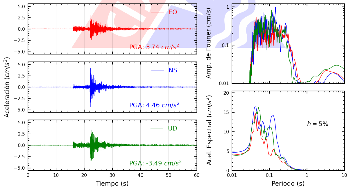
Figura A.4: Registros tiempo-historia, espectros de Fourier y de respuesta en las direcciones EO, NS y vertical de la estación SOVES. Sismo de Chilca, Cañete - Lima del 2025-04-25, 16:21:07 (Hora local)
