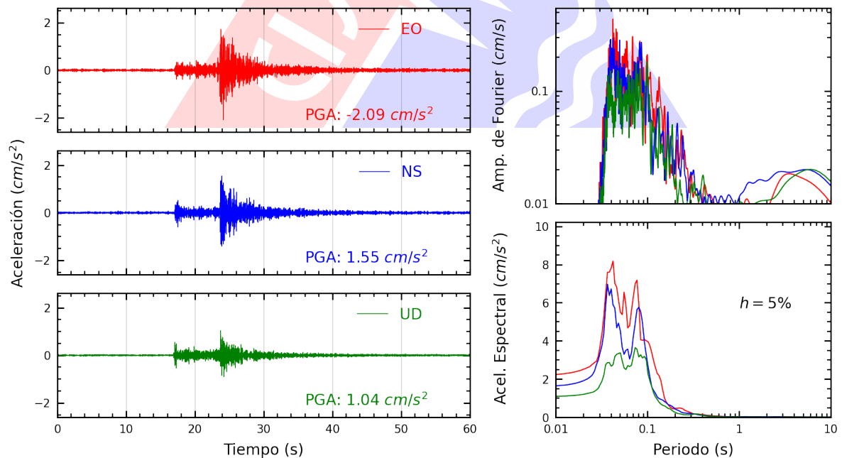
Figura A.12: Registros tiempo-historia, espectros de Fourier y de respuesta en las direcciones EO, NS y vertical de la estación CEPRE. Sismo de Chilca, Cañete - Lima del 2025-04-25, 16:21:07 (Hora local)
