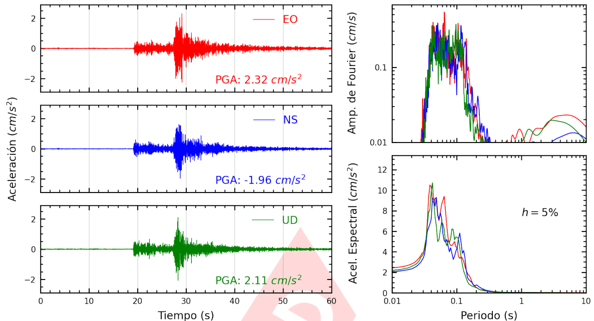
Figura A.9: Registros tiempo-historia, espectros de Fourier y de respuesta en las direcciones EO, NS y vertical de la estación AMORE. Sismo de Chilca, Cañete - Lima del 2025-04-25, 16:21:07 (Hora local)
