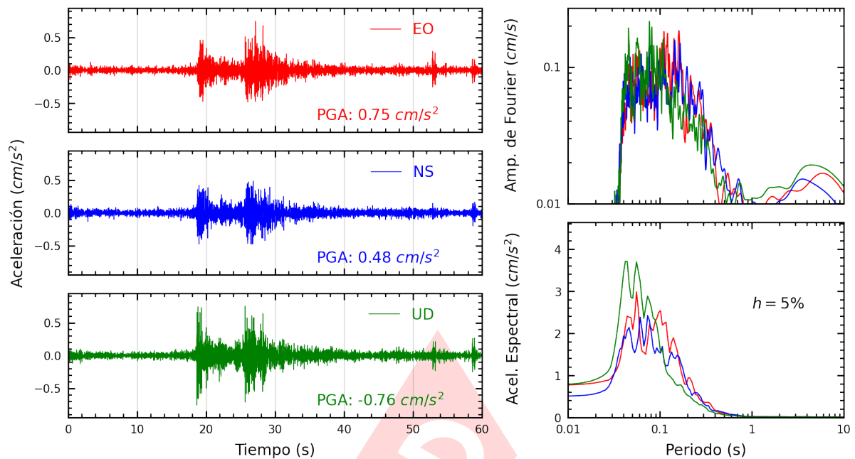
Figura A.37: Registros tiempo-historia, espectros de Fourier y de respuesta en las direcciones EO, NS y vertical de la estación PRADO. Sismo de Chilca, Cañete - Lima del 2025-04-25, 16:21:07 (Hora local)
