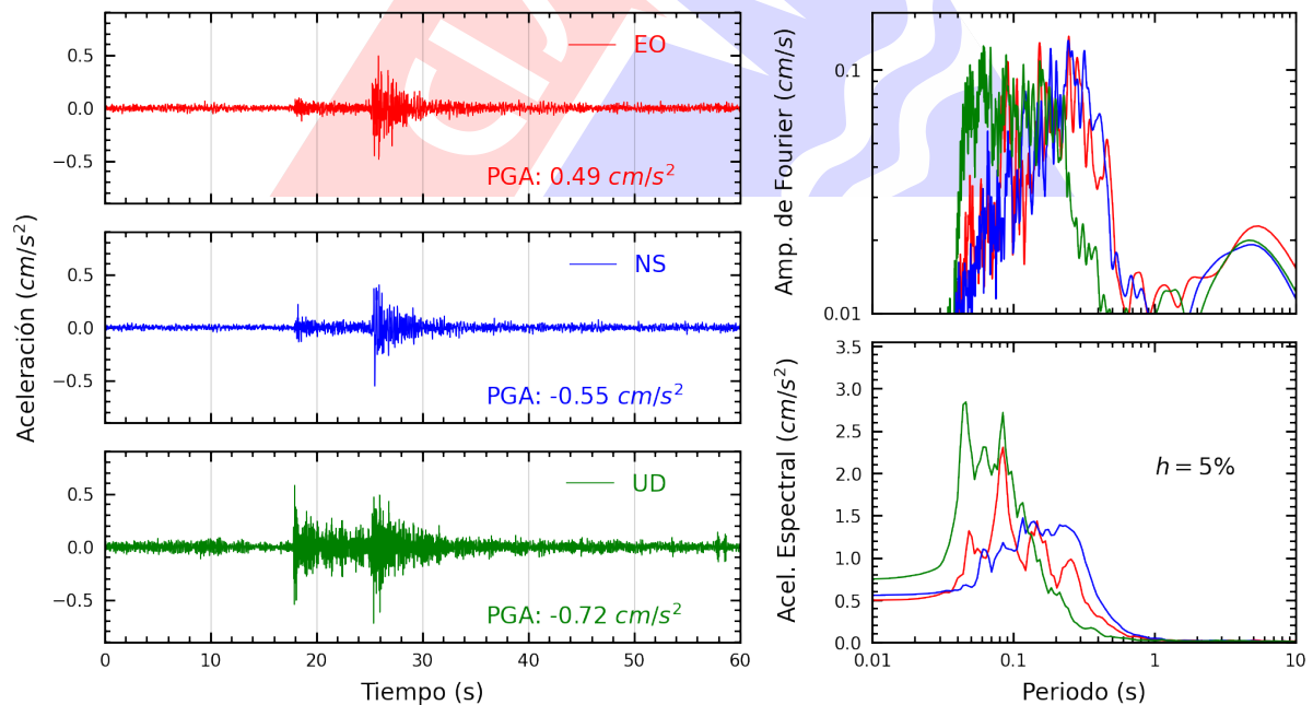
Figura A.38: Registros tiempo-historia, espectros de Fourier y de respuesta en las direcciones EO, NS y vertical de la estación ACAPU. Sismo de Chilca, Cañete - Lima del 2025-04-25, 16:21:07 (Hora local)
