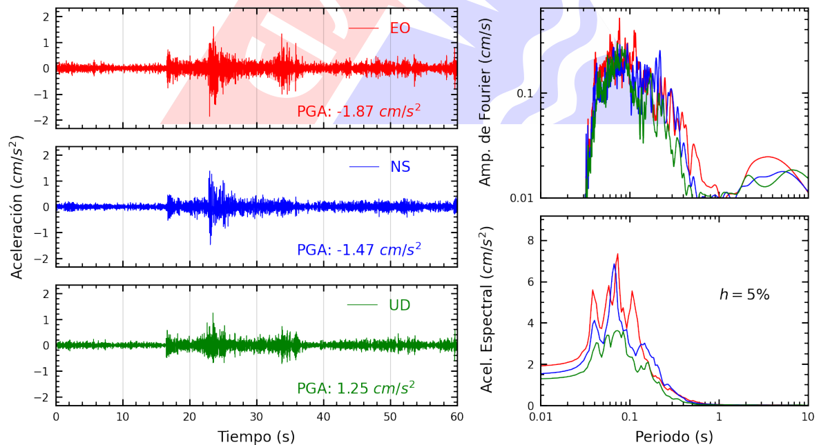
Figura A.18: Registros tiempo-historia, espectros de Fourier y de respuesta en las direcciones EO, NS y vertical de la estación SOBAR. Sismo de Chilca, Cañete - Lima del 2025-04-25, 16:21:07 (Hora local)
