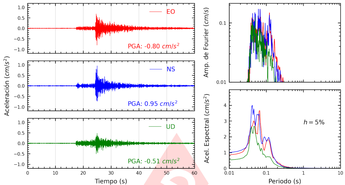
Figura A.35: Registros tiempo-historia, espectros de Fourier y de respuesta en las direcciones EO, NS y vertical de la estación ATARJ. Sismo de Chilca, Cañete - Lima del 2025-04-25, 16:21:07 (Hora local)
