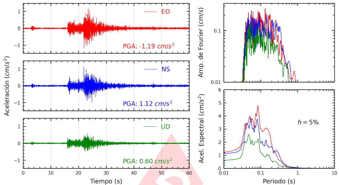
Figura A.29: Registros tiempo-historia, espectros de Fourier y de respuesta en las direcciones EO, NS y vertical de la estación BRIS2. Sismo de Chilca, Cañete - Lima del 2025-04-25, 16:21:07 (Hora local)
