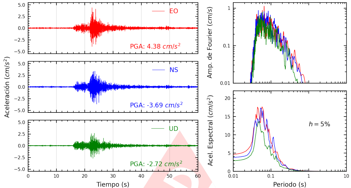
Figura A.5: Registros tiempo-historia, espectros de Fourier y de respuesta en las direcciones EO, NS y vertical de la estación PHER2. Sismo de Chilca, Cañete - Lima del 2025-04-25, 16:21:07 (Hora local)
