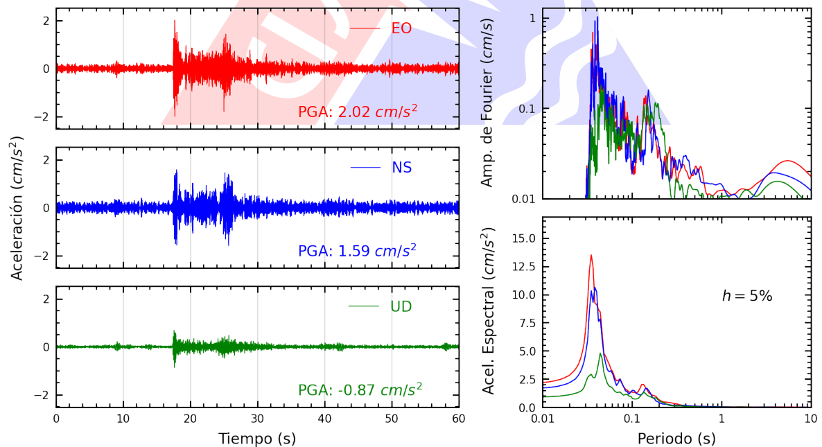
Figura A.14: Registros tiempo-historia, espectros de Fourier y de respuesta en las direcciones EO, NS y vertical de la estación DHNPE. Sismo de Chilca, Cañete - Lima del 2025-04-25, 16:21:07 (Hora local)
