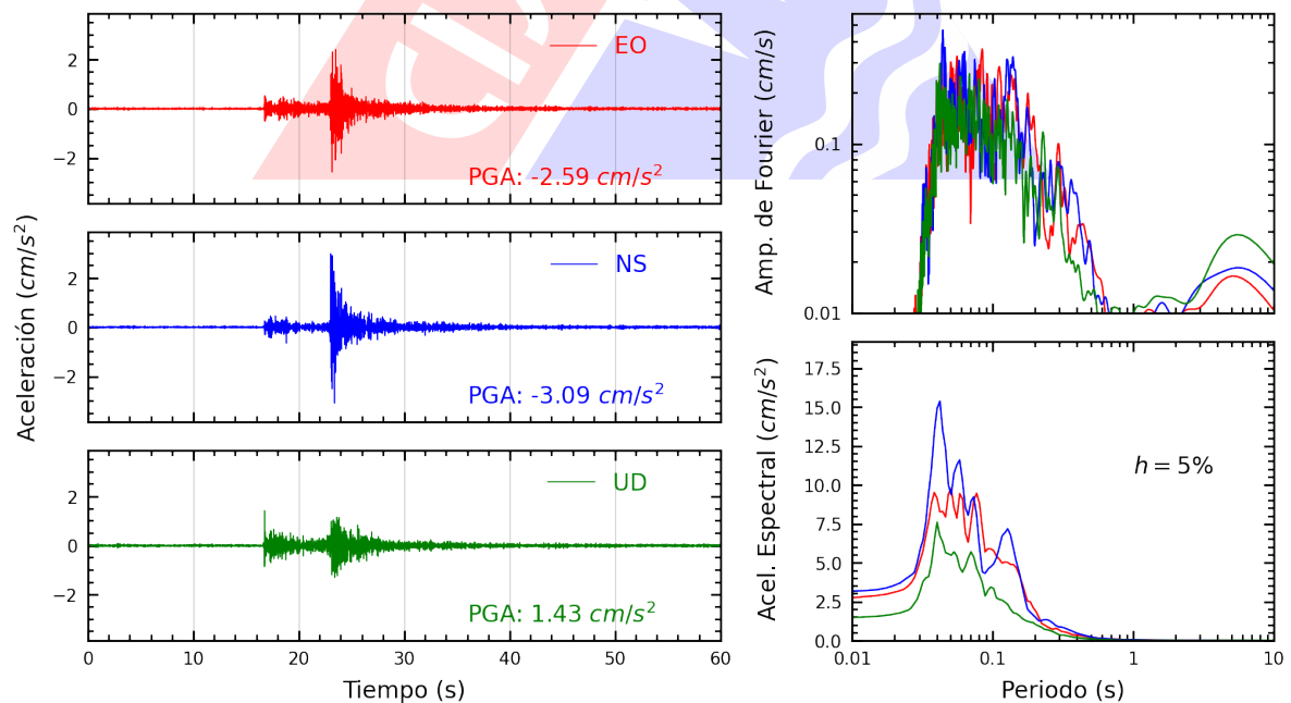
Figura A.8: Registros tiempo-historia, espectros de Fourier y de respuesta en las direcciones EO, NS y vertical de la estación URPPE. Sismo de Chilca, Cañete - Lima del 2025-04-25, 16:21:07 (Hora local)
