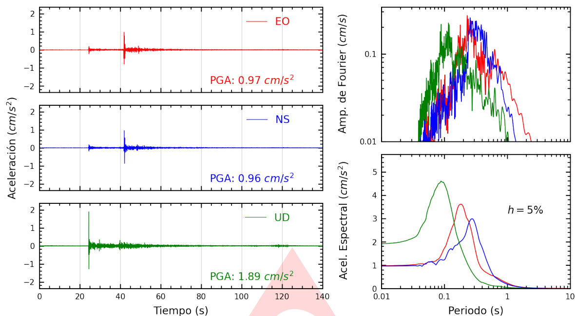
Figura A.1: Registros tiempo-historia, espectros de Fourier y de respuesta en las direcciones EO, NS y vertical de la estación SCPUC. Sismo de Pucallpa, Coronel Portillo - Ucayali del 2025-04-27, 04:38:38 (Hora local)
