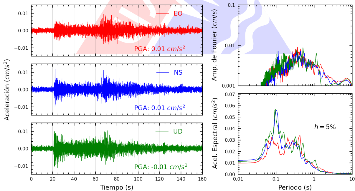
Figura A.8: Registros tiempo-historia, espectros de Fourier y de respuesta en las direcciones EO, NS y vertical de la estación UNCP. Sismo de Pucallpa, Coronel Portillo - Ucayali del 2025-04-27, 04:38:38 (Hora local)
