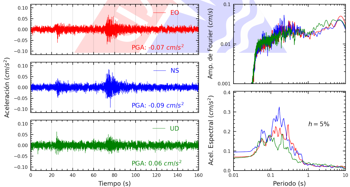
Figura A.6: Registros tiempo-historia, espectros de Fourier y de respuesta en las direcciones EO, NS y vertical de la estación UNTRM. Sismo de Pucallpa, Coronel Portillo - Ucayali del 2025-04-27, 04:38:38 (Hora local)
