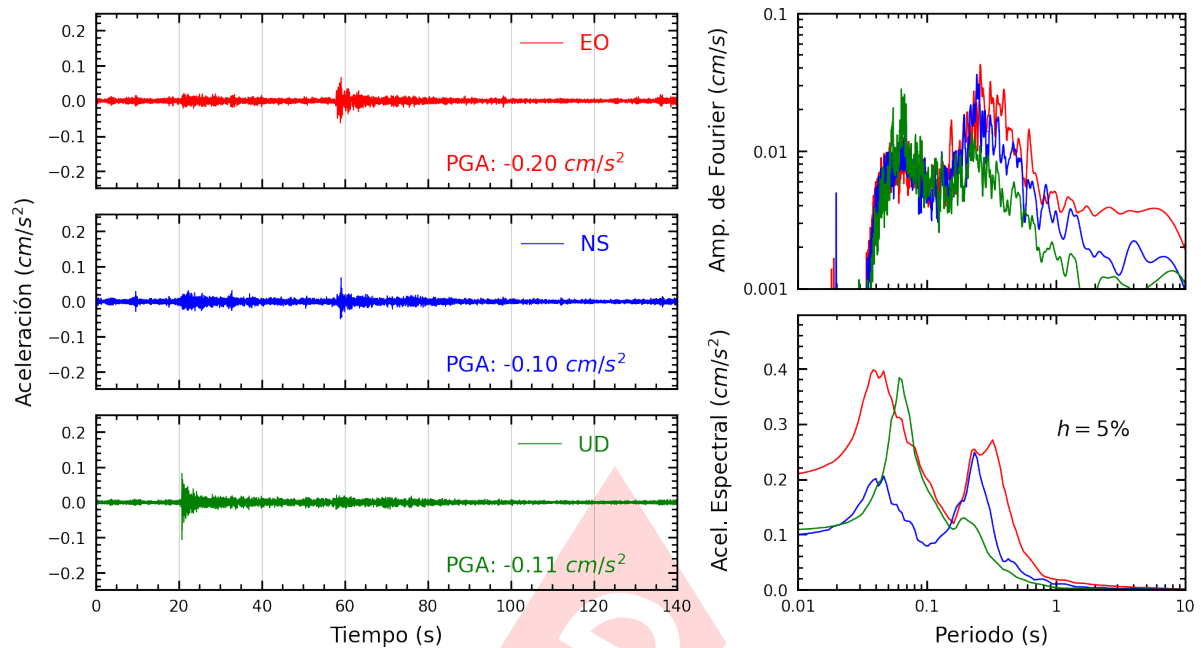
Figura A.3: Registros tiempo-historia, espectros de Fourier y de respuesta en las direcciones EO, NS y vertical de la estación UNAAA. Sismo de Pucallpa, Coronel Portillo - Ucayali del 2025-04-27, 04:38:38 (Hora local)
