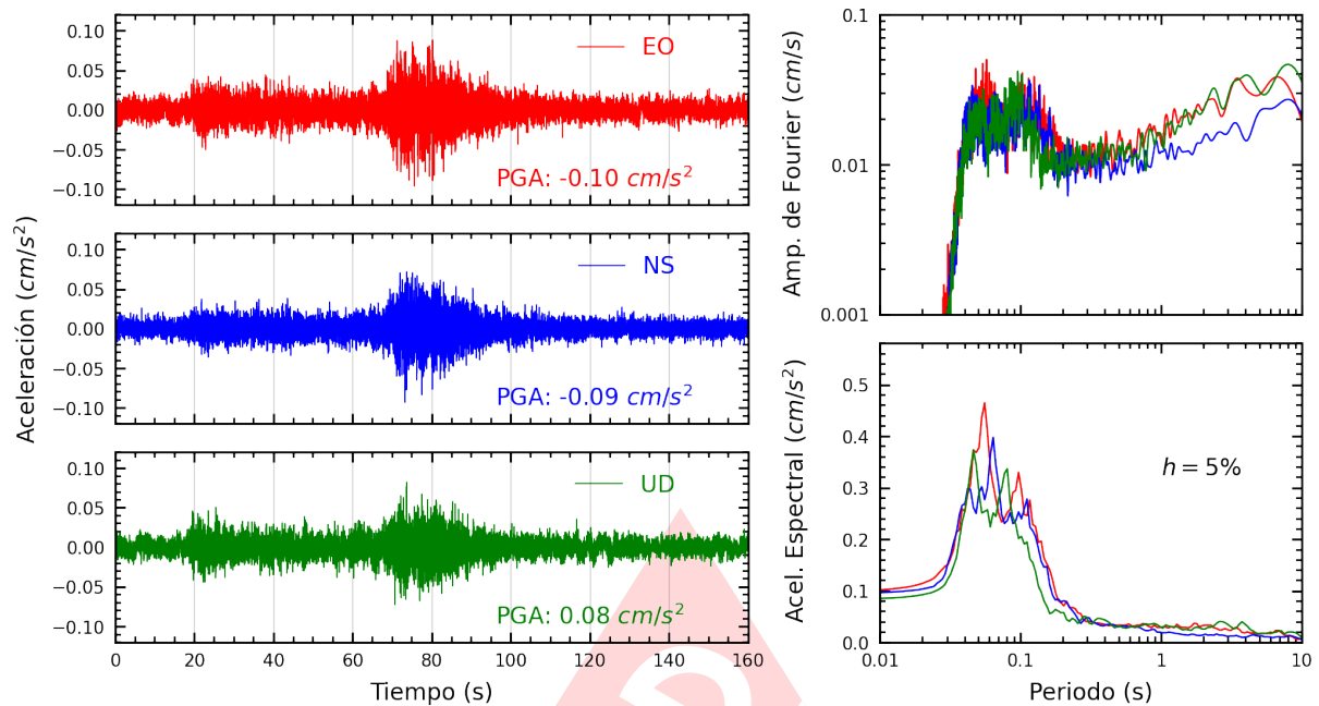
Figura A.5: Registros tiempo-historia, espectros de Fourier y de respuesta en las direcciones EO, NS y vertical de la estación AMORE. Sismo de Pucallpa, Coronel Portillo - Ucayali del 2025-04-27, 04:38:38 (Hora local)
