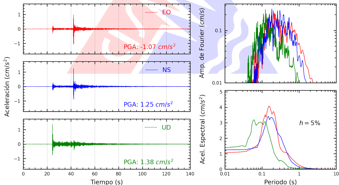
Figura A.2: Registros tiempo-historia, espectros de Fourier y de respuesta en las direcciones EO, NS y vertical de la estación UNIA. Sismo de Pucallpa, Coronel Portillo - Ucayali del 2025-04-27, 04:38:38 (Hora local)
