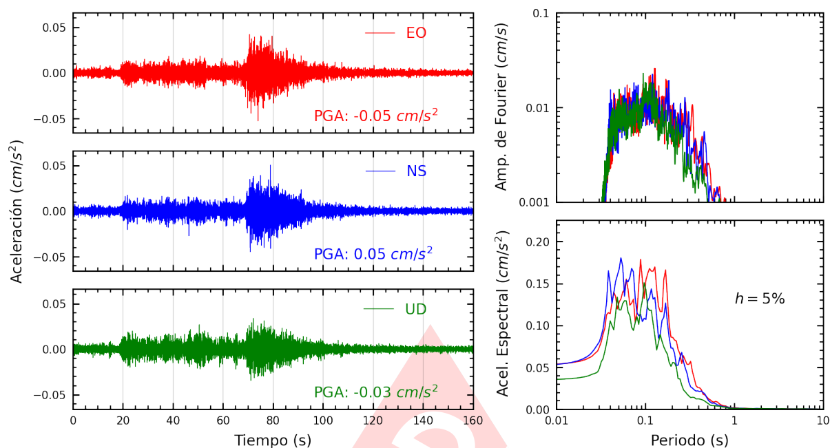
Figura A.7: Registros tiempo-historia, espectros de Fourier y de respuesta en las direcciones EO, NS y vertical de la estación JALV2. Sismo de Pucallpa, Coronel Portillo - Ucayali del 2025-04-27, 04:38:38 (Hora local)
