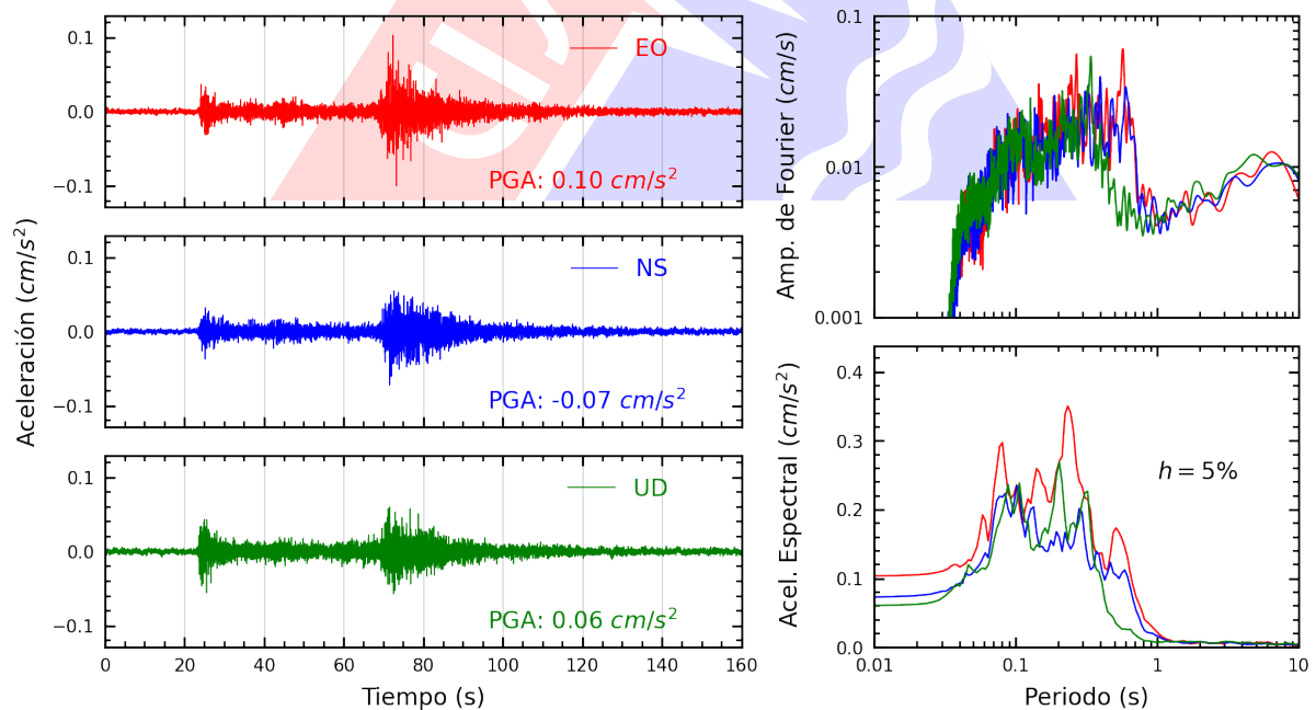
Figura A.4: Registros tiempo-historia, espectros de Fourier y de respuesta en las direcciones EO, NS y vertical de la estación CARAL. Sismo de Pucallpa, Coronel Portillo - Ucayali del 2025-04-27, 04:38:38 (Hora local)
