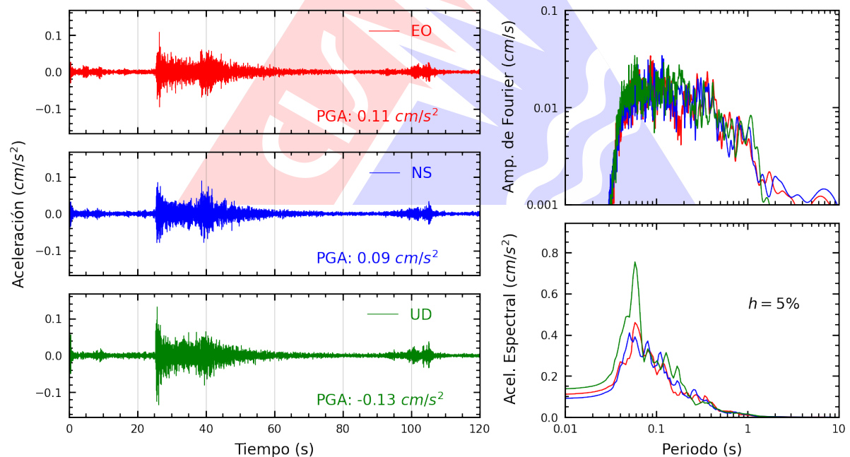
Figura A.2: Registros tiempo-historia, espectros de Fourier y de respuesta en las direcciones EO, NS y vertical de la estación UNCP. Sismo de Satipo, Satipo - Junin del 2025-04-28, 09:02:48 (Hora local)
