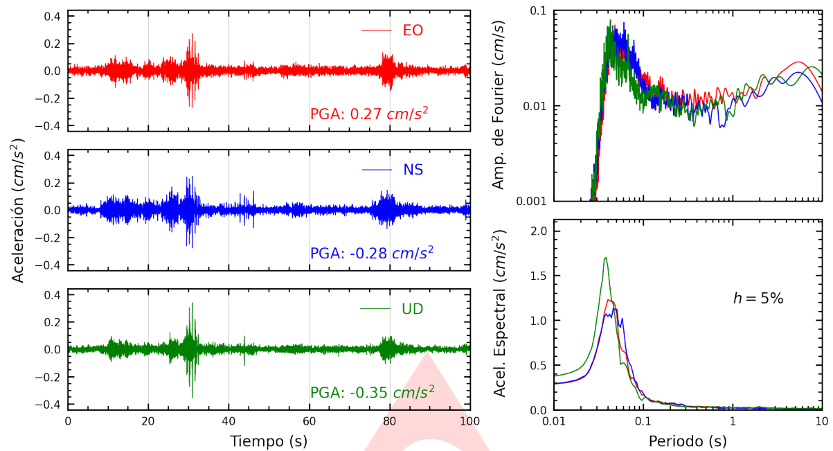
Figura A.1: Registros tiempo-historia, espectros de Fourier y de respuesta en las direcciones EO, NS y vertical de la estación USILP. Sismo de Satipo, Satipo - Junin del 2025-04-28, 09:02:48 (Hora local)
