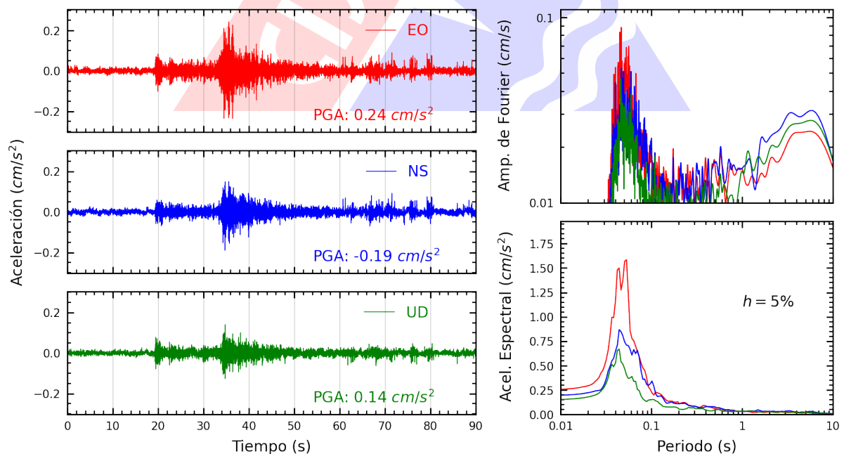
Figura A.18: Registros tiempo-historia, espectros de Fourier y de respuesta en las direcciones EO, NS y vertical de la estación UCSS. Sismo de Mala, Cañete - Lima del 2025-04-30, 07:34:49 (Hora local)
