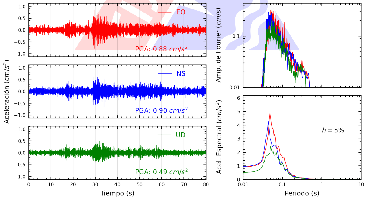
Figura A.4: Registros tiempo-historia, espectros de Fourier y de respuesta en las direcciones EO, NS y vertical de la estación UNTEL. Sismo de Mala, Cañete - Lima del 2025-04-30, 07:34:49 (Hora local)
