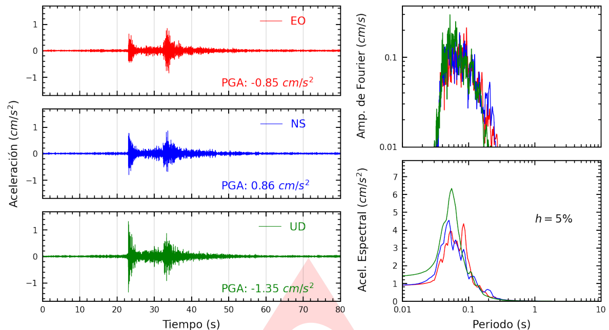
Figura A.1: Registros tiempo-historia, espectros de Fourier y de respuesta en las direcciones EO, NS y vertical de la estación ASIA. Sismo de Mala, Cañete - Lima del 2025-04-30, 07:34:49 (Hora local)
