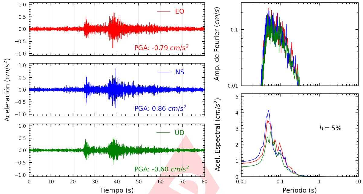
Figura A.5: Registros tiempo-historia, espectros de Fourier y de respuesta en las direcciones EO, NS y vertical de la estación PHER2. Sismo de Mala, Cañete - Lima del 2025-04-30, 07:34:49 (Hora local)
