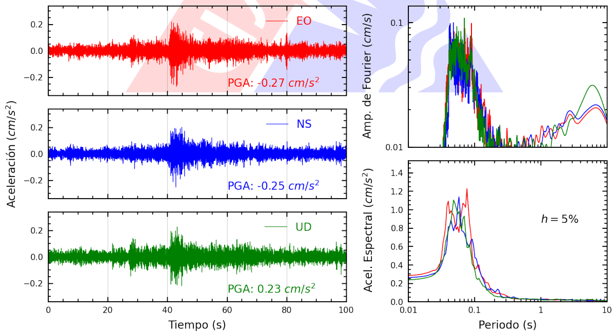
Figura A.16: Registros tiempo-historia, espectros de Fourier y de respuesta en las direcciones EO, NS y vertical de la estación URPE. Sismo de Mala, Cañete - Lima del 2025-04-30, 07:34:49 (Hora local)
