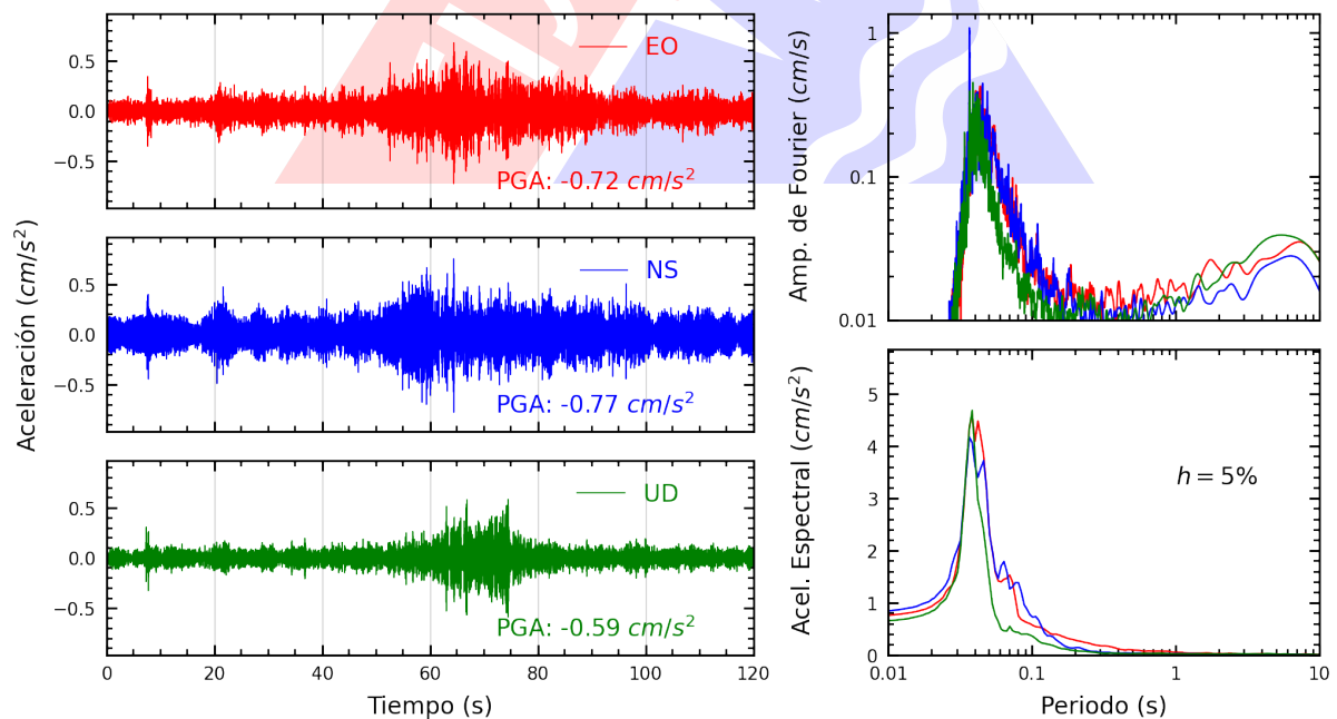
Figura A.8: Registros tiempo-historia, espectros de Fourier y de respuesta en las direcciones EO, NS y vertical de la estación UPCVI. Sismo de Mala, Cañete - Lima del 2025-04-30, 07:34:49 (Hora local)
