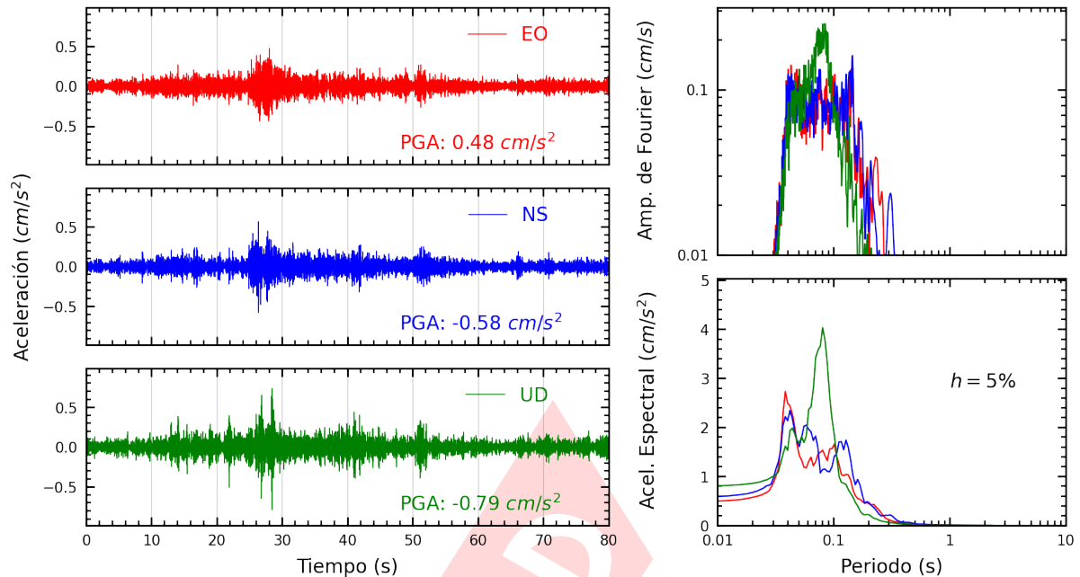
Figura A.7: Registros tiempo-historia, espectros de Fourier y de respuesta en las direcciones EO, NS y vertical de la estación CARA2. Sismo de Mala, Cañete - Lima del 2025-04-30, 07:34:49 (Hora local)
