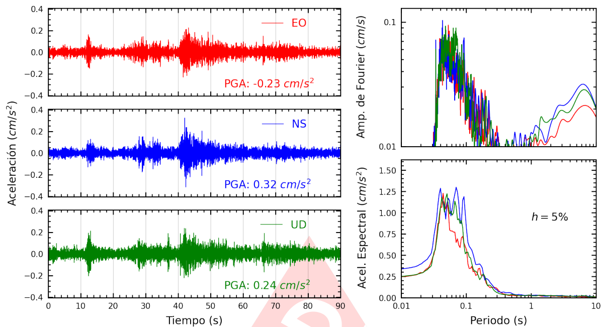
Figura A.13: Registros tiempo-historia, espectros de Fourier y de respuesta en las direcciones EO, NS y vertical de la estación USMP. Sismo de Mala, Cañete - Lima del 2025-04-30, 07:34:49 (Hora local)
