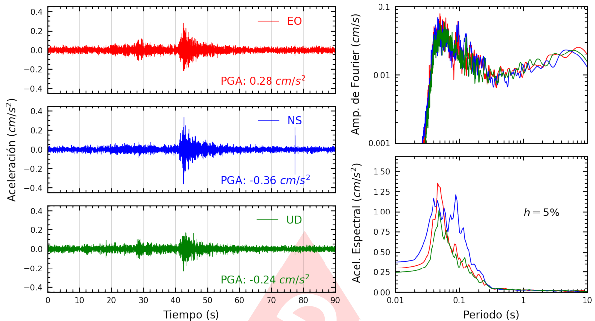
Figura A.11: Registros tiempo-historia, espectros de Fourier y de respuesta en las direcciones EO, NS y vertical de la estación IMCA. Sismo de Mala, Cañete - Lima del 2025-04-30, 07:34:49 (Hora local)
