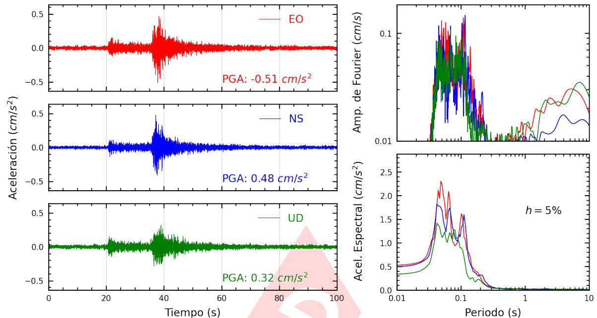
Figura A.9: Registros tiempo-historia, espectros de Fourier y de respuesta en las direcciones EO, NS y vertical de la estación AMORE. Sismo de Mala, Cañete - Lima del 2025-04-30, 07:34:49 (Hora local)
