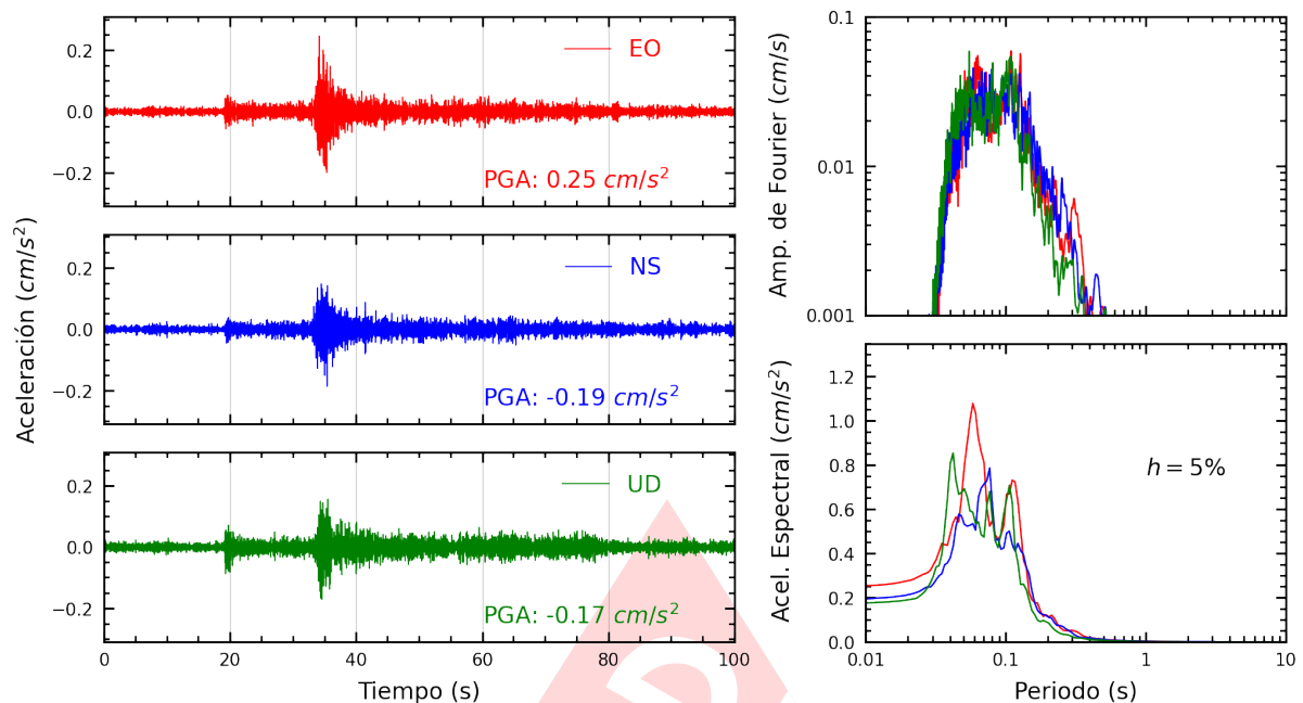
Figura A.17: Registros tiempo-historia, espectros de Fourier y de respuesta en las direcciones EO, NS y vertical de la estación JALV2. Sismo de Mala, Cañete - Lima del 2025-04-30, 07:34:49 (Hora local)
