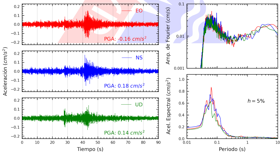
Figura A.20: Registros tiempo-historia, espectros de Fourier y de respuesta en las direcciones EO, NS y vertical de la estación SERVI. Sismo de Mala, Cañete - Lima del 2025-04-30, 07:34:49 (Hora local)
