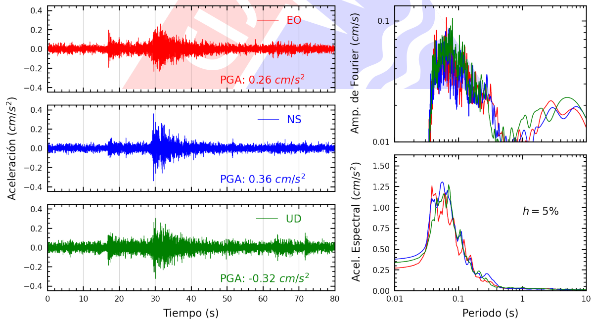
Figura A.12: Registros tiempo-historia, espectros de Fourier y de respuesta en las direcciones EO, NS y vertical de la estación SOVES. Sismo de Mala, Cañete - Lima del 2025-04-30, 07:34:49 (Hora local)
