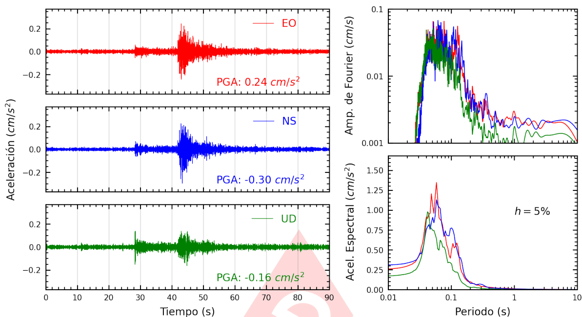
Figura A.15: Registros tiempo-historia, espectros de Fourier y de respuesta en las direcciones EO, NS y vertical de la estación ATARJ. Sismo de Mala, Cañete - Lima del 2025-04-30, 07:34:49 (Hora local)
