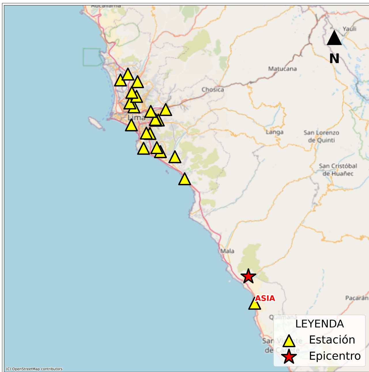
Figura 2: Mapa de ubicación de la(s) estación(es) acelerográfica(s) a nivel nacional correspondiente(s) al Sismo de Mala, Cañete - Lima del 30 de abril de 2025 a las 07:34:49 (hora local)
