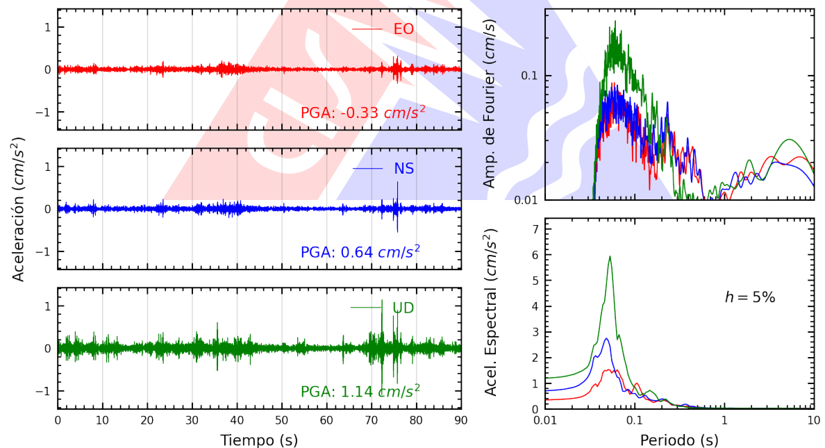
Figura A.2: Registros tiempo-historia, espectros de Fourier y de respuesta en las direcciones EO, NS y vertical de la estación MDPP. Sismo de Mala, Cañete - Lima del 2025-04-30, 07:34:49 (Hora local)
