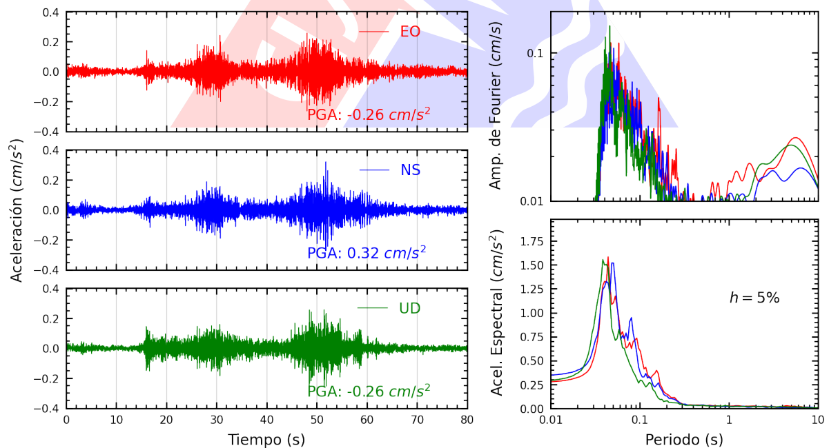
Figura A.14: Registros tiempo-historia, espectros de Fourier y de respuesta en las direcciones EO, NS y vertical de la estación USILP. Sismo de Mala, Cañete - Lima del 2025-04-30, 07:34:49 (Hora local)
