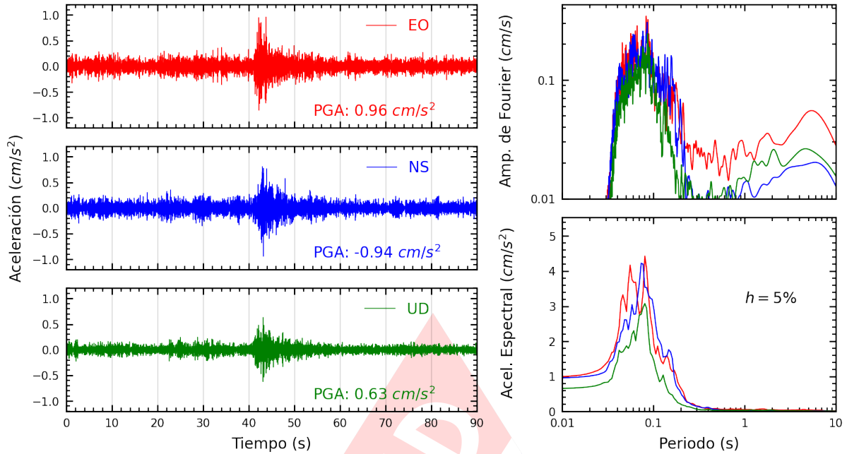
Figura A.3: Registros tiempo-historia, espectros de Fourier y de respuesta en las direcciones EO, NS y vertical de la estación USILM. Sismo de Mala, Cañete - Lima del 2025-04-30, 07:34:49 (Hora local)
