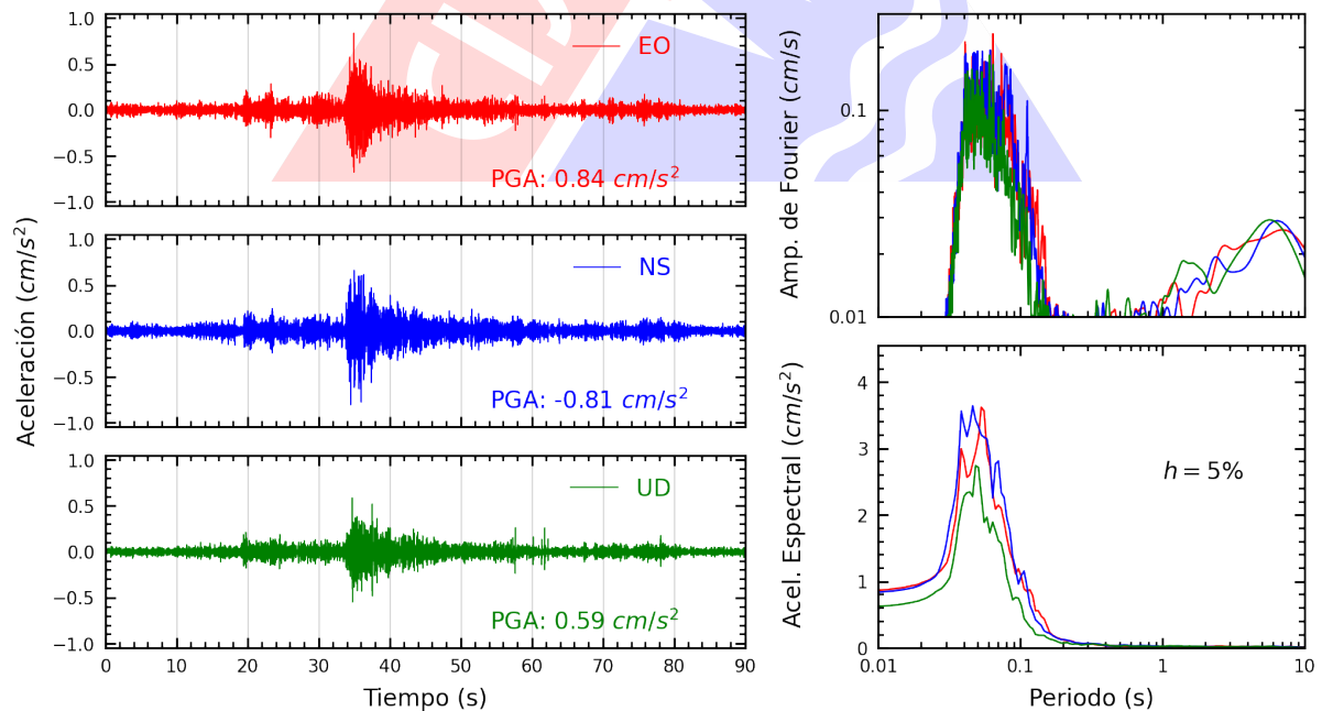
Figura A.6: Registros tiempo-historia, espectros de Fourier y de respuesta en las direcciones EO, NS y vertical de la estación JOSEO. Sismo de Mala, Cañete - Lima del 2025-04-30, 07:34:49 (Hora local)
