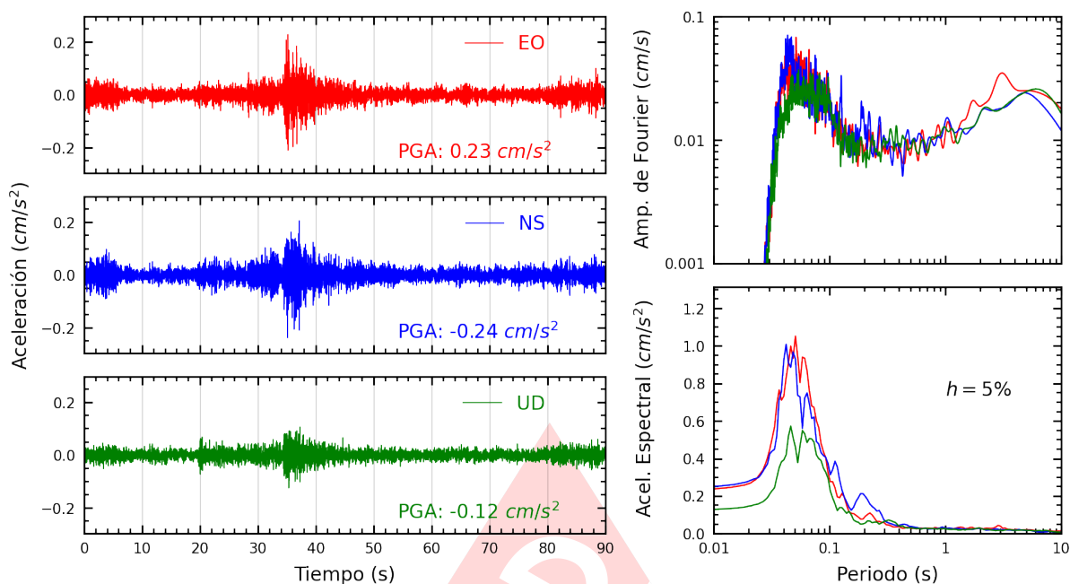
Figura A.19: Registros tiempo-historia, espectros de Fourier y de respuesta en las direcciones EO, NS y vertical de la estación COMAS. Sismo de Mala, Cañete - Lima del 2025-04-30, 07:34:49 (Hora local)
