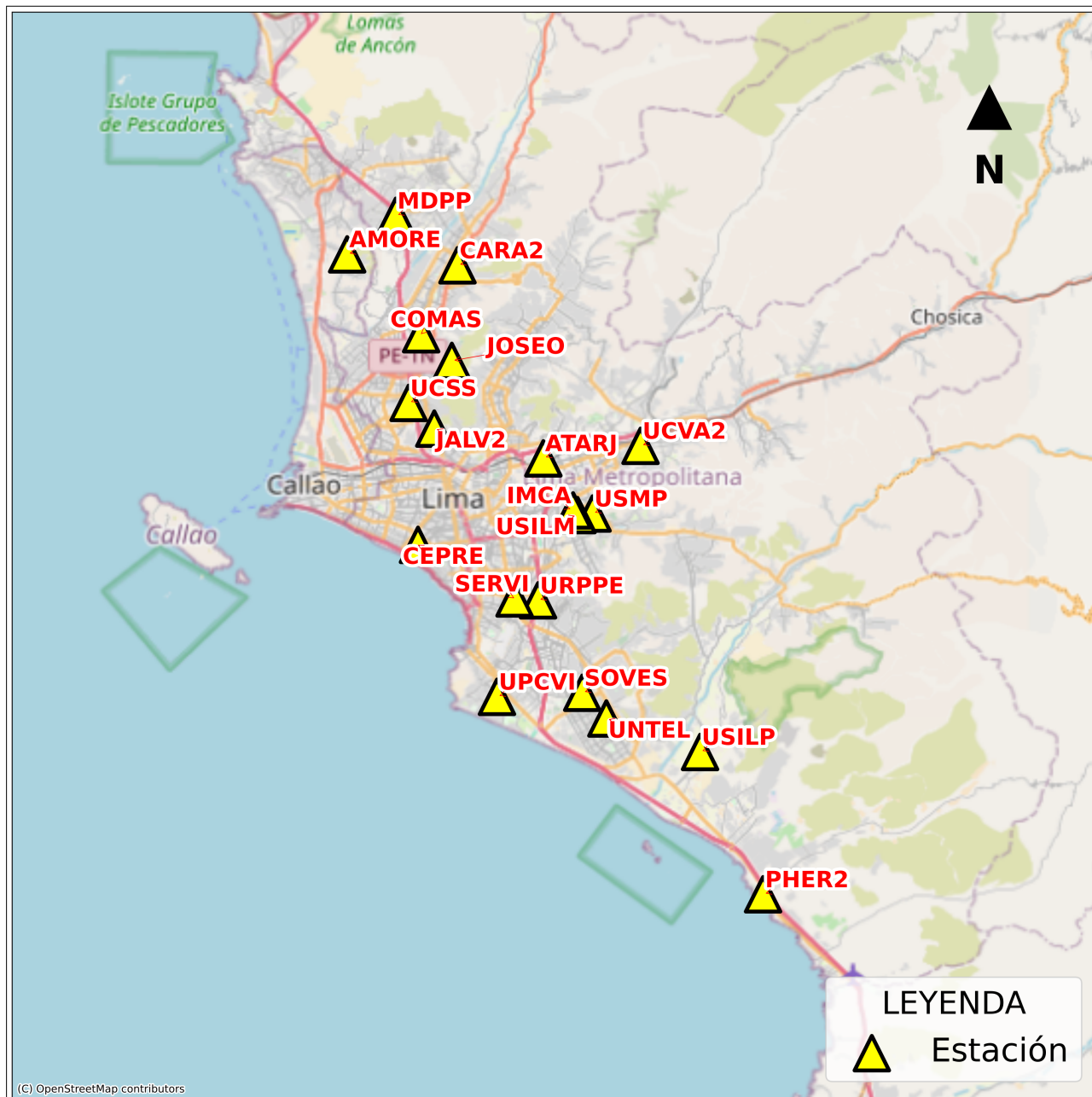
Figura 3: Mapa de ubicación de la(s) estación(es) acelerográfica(s) en Lima Metropolitana correspondiente(s) al Sismo de Mala, Cañete - Lima del 30 de abril de 2025 a las 07:34:49 (hora local)
