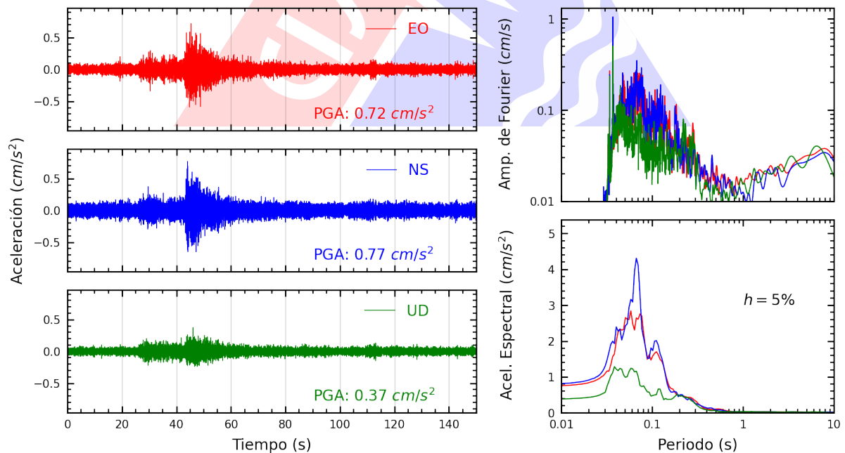
Figura A.12: Registros tiempo-historia, espectros de Fourier y de respuesta en las direcciones EO, NS y vertical de la estación UPCVI. Sismo de Chincha Alta, Chincha - Ica del 2025-04-26, 13:56:02 (Hora local)
