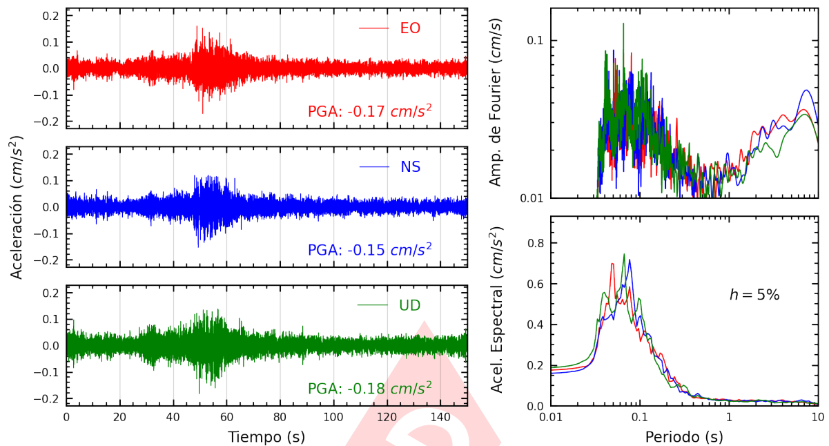
Figura A.35: Registros tiempo-historia, espectros de Fourier y de respuesta en las direcciones EO, NS y vertical de la estación BONDY. Sismo de Chinchá Alta, Chinchá - Ica del 2025-04-26, 13:56:02 (Hora local)
