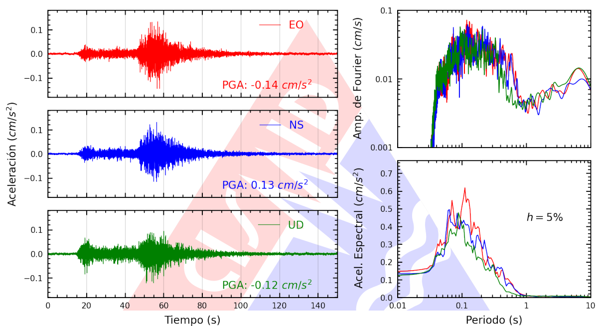
Figura A.37: Registros tiempo-historia, espectros de Fourier y de respuesta en las direcciones EO, NS y vertical de la estación CARAL. Sismo de Chincha Alta, Chincha - Ica del 2025-04-26, 13:56:02 (Hora local)
