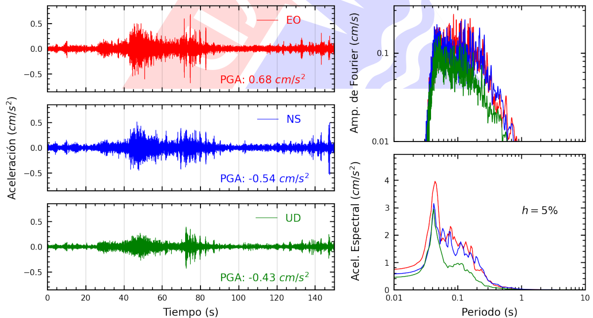
Figura A.16: Registros tiempo-historia, espectros de Fourier y de respuesta en las direcciones EO, NS y vertical de la estación BRISA. Sismo de Chinchá Alta, Chinchá - Ica del 2025-04-26, 13:56:02 (Hora local)
