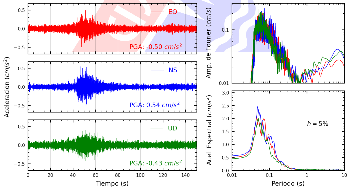
Figura A.22: Registros tiempo-historia, espectros de Fourier y de respuesta en las direcciones EO, NS y vertical de la estación URPPE. Sismo de Chinchá Alta, Chinchá - Ica del 2025-04-26, 13:56:02 (Hora local)
