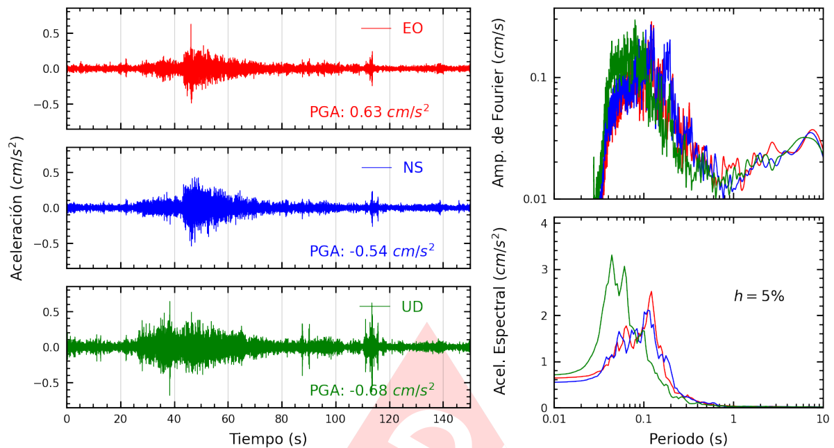
Figura A.17: Registros tiempo-historia, espectros de Fourier y de respuesta en las direcciones EO, NS y vertical de la estación SOCHO. Sismo de Chincha Alta, Chincha - Ica del 2025-04-26, 13:56:02 (Hora local)
