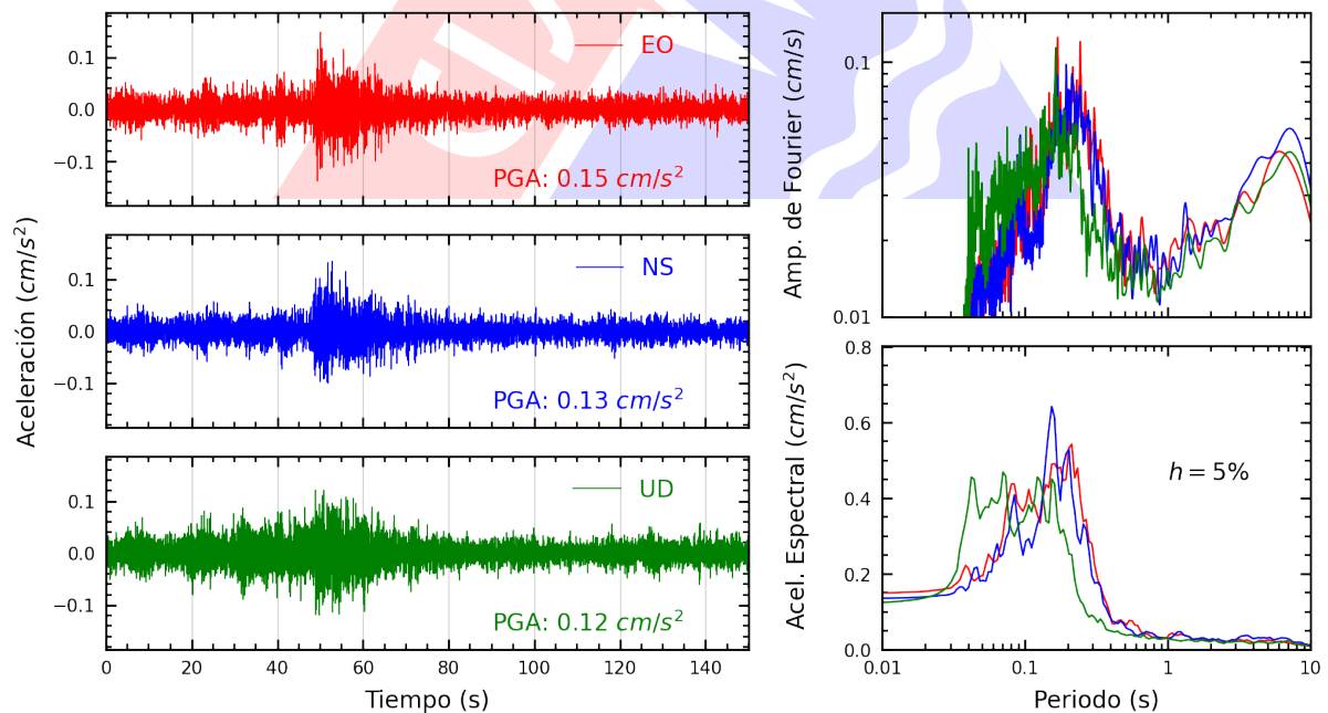
Figura A.36: Registros tiempo-historia, espectros de Fourier y de respuesta en las direcciones EO, NS y vertical de la estación DSMI. Sismo de Chinchá Alta, Chinchá - Ica del 2025-04-26, 13:56:02 (Hora local)
