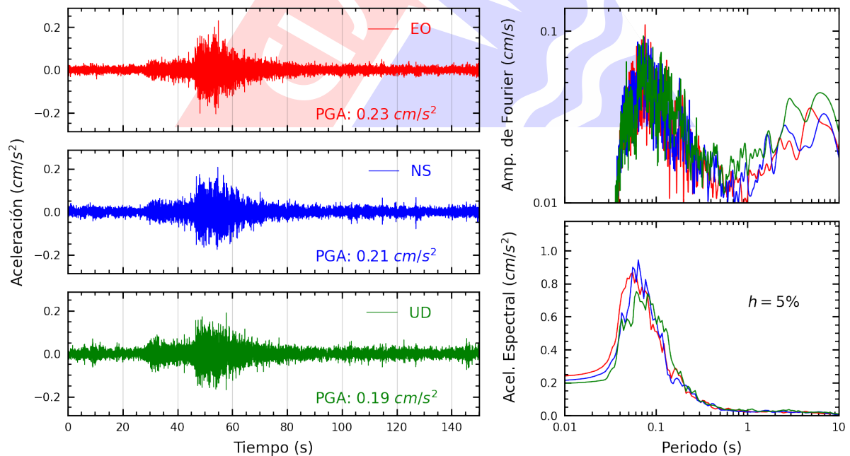
Figura A.34: Registros tiempo-historia, espectros de Fourier y de respuesta en las direcciones EO, NS y vertical de la estación UNFV. Sismo de Chincha Alta, Chincha - Ica del 2025-04-26, 13:56:02 (Hora local)
