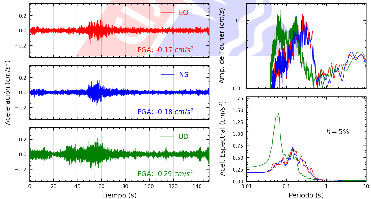
Figura A.32: Registros tiempo-historia, espectros de Fourier y de respuesta en las direcciones EO, NS y vertical de la estación ACAPU. Sismo de Chinchá Alta, Chinchá - Ica del 2025-04-26, 13:56:02 (Hora local)
