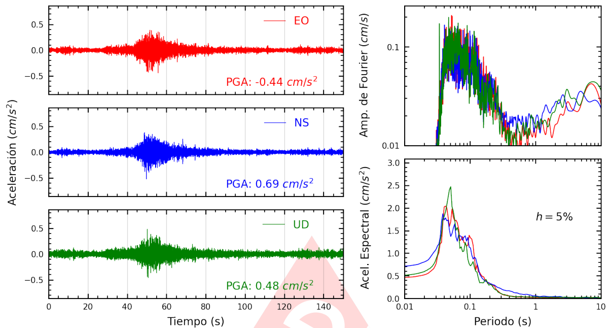
Figura A.15: Registros tiempo-historia, espectros de Fourier y de respuesta en las direcciones EO, NS y vertical de la estación USMP. Sismo de Chinchá Alta, Chinchá - Ica del 2025-04-26, 13:56:02 (Hora local)
