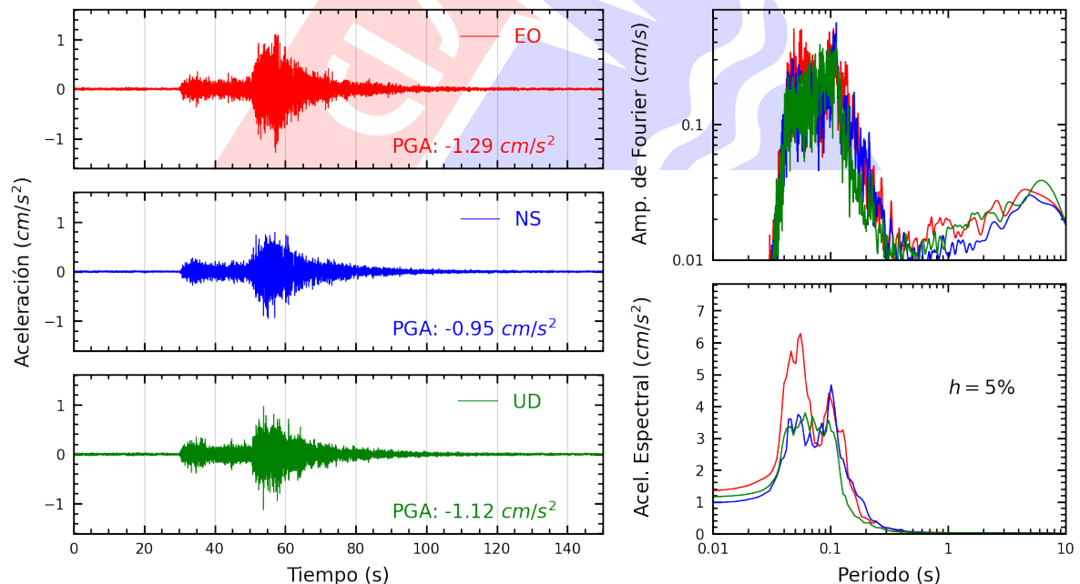
Figura A.8: Registros tiempo-historia, espectros de Fourier y de respuesta en las direcciones EO, NS y vertical de la estación AMORE. Sismo de Chinchá Alta, Chinchá - Ica del 2025-04-26, 13:56:02 (Hora local)
