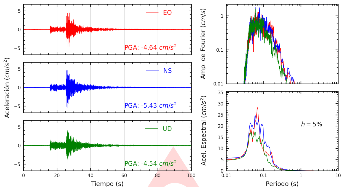
Figura A.1: Registros tiempo-historia, espectros de Fourier y de respuesta en las direcciones EO, NS y vertical de la estación ASIA. Sismo de Chinchá Alta, Chinchá - Ica del 2025-04-26, 13:56:02 (Hora local)
