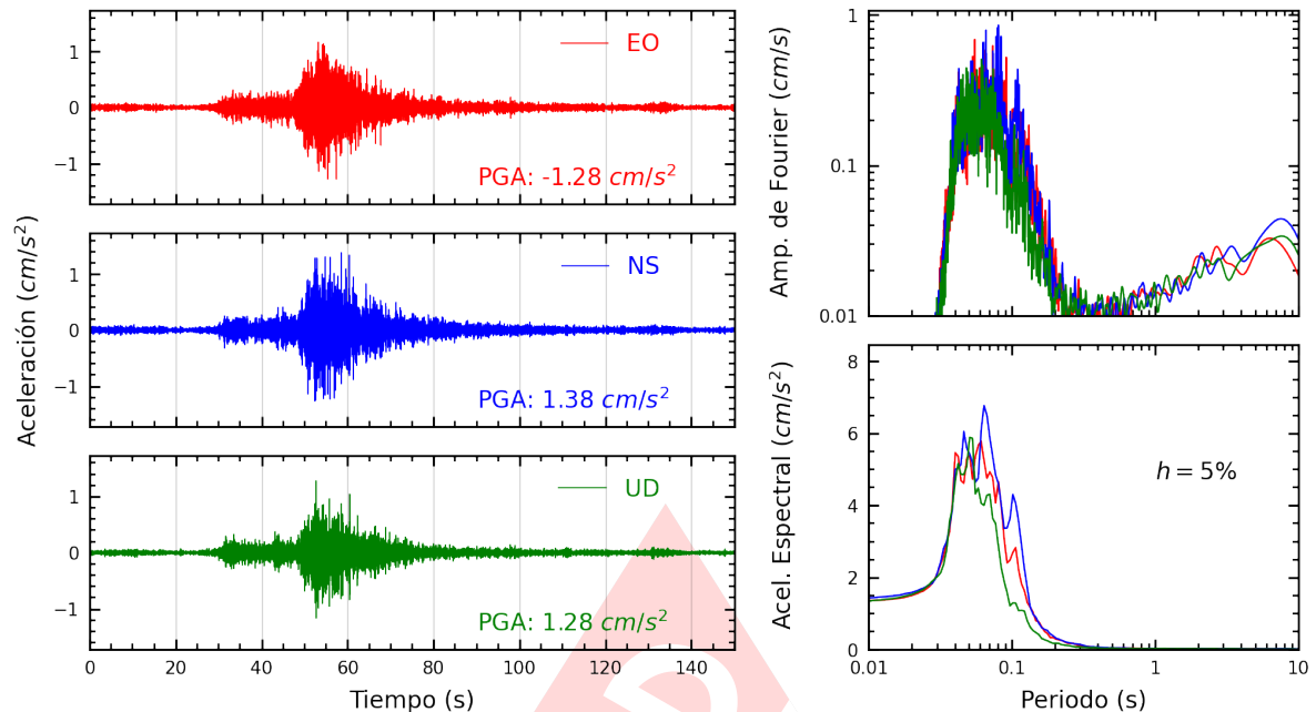
Figura A.7: Registros tiempo-historia, espectros de Fourier y de respuesta en las direcciones EO, NS y vertical de la estación JOSEO. Sismo de Chinchá Alta, Chinchá - Ica del 2025-04-26, 13:56:02 (Hora local)
