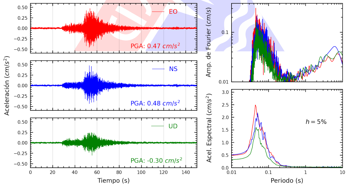
Figura A.26: Registros tiempo-historia, espectros de Fourier y de respuesta en las direcciones EO, NS y vertical de la estación UCSS. Sismo de Chinchá Alta, Chinchá - Ica del 2025-04-26, 13:56:02 (Hora local)
