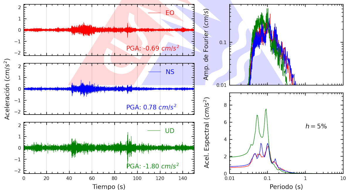
Figura A.2: Registros tiempo-historia, espectros de Fourier y de respuesta en las direcciones EO, NS y vertical de la estación SCOLI. Sismo de Chinchá Alta, Chinchá - Ica del 2025-04-26, 13:56:02 (Hora local)
