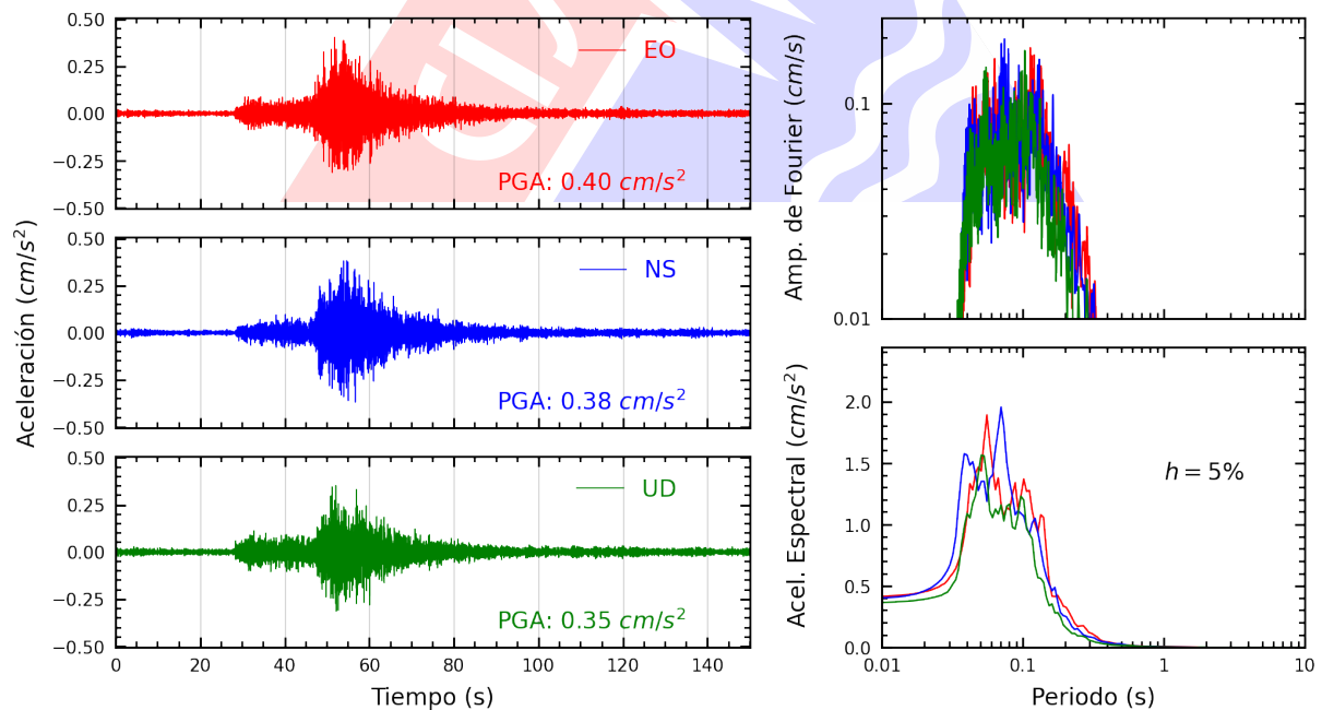
Figura A.28: Registros tiempo-historia, espectros de Fourier y de respuesta en las direcciones EO, NS y vertical de la estación JALV2. Sismo de Chinchá Alta, Chinchá - Ica del 2025-04-26, 13:56:02 (Hora local)
