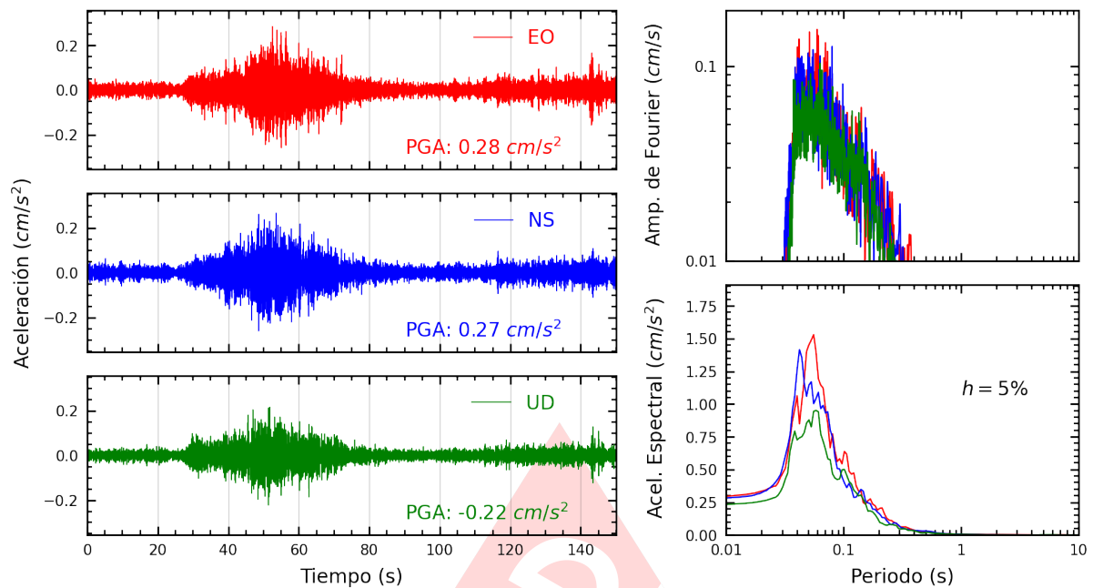
Figura A.33: Registros tiempo-historia, espectros de Fourier y de respuesta en las direcciones EO, NS y vertical de la estación BORJA. Sismo de Chincha Alta, Chincha - Ica del 2025-04-26, 13:56:02 (Hora local)
