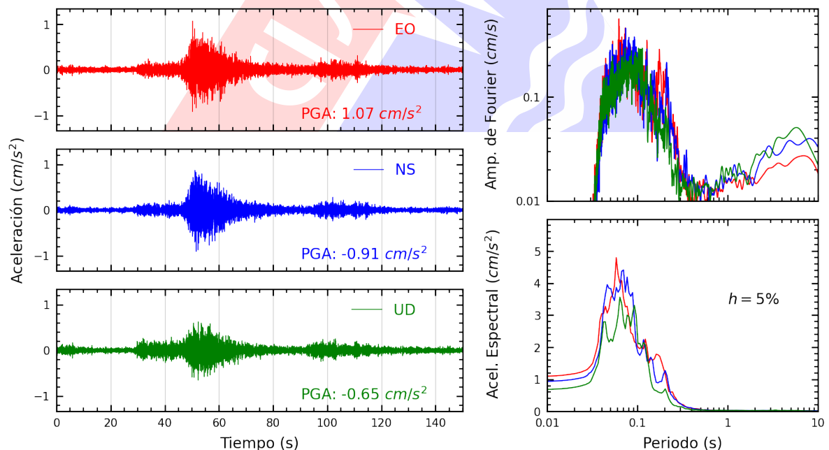
Figura A.10: Registros tiempo-historia, espectros de Fourier y de respuesta en las direcciones EO, NS y vertical de la estación INDEP. Sismo de Chinchá Alta, Chinchá - Ica del 2025-04-26, 13:56:02 (Hora local)
