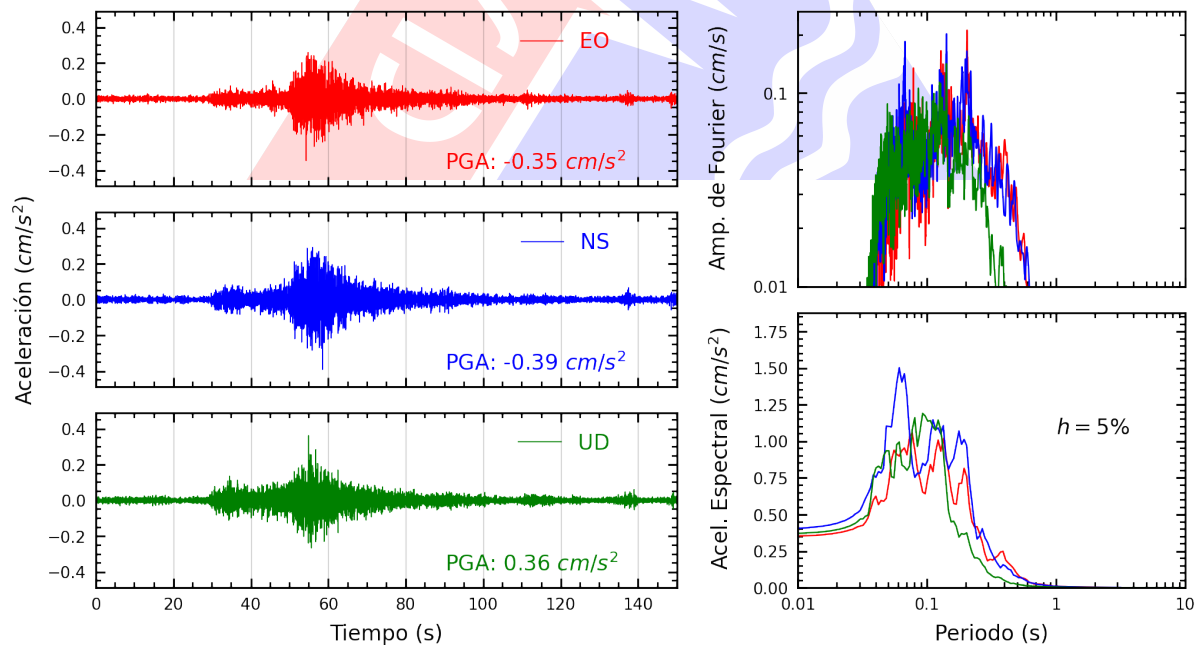
Figura A.30: Registros tiempo-historia, espectros de Fourier y de respuesta en las direcciones EO, NS y vertical de la estación VHAY2. Sismo de Chinchá Alta, Chinchá - Ica del 2025-04-26, 13:56:02 (Hora local)
