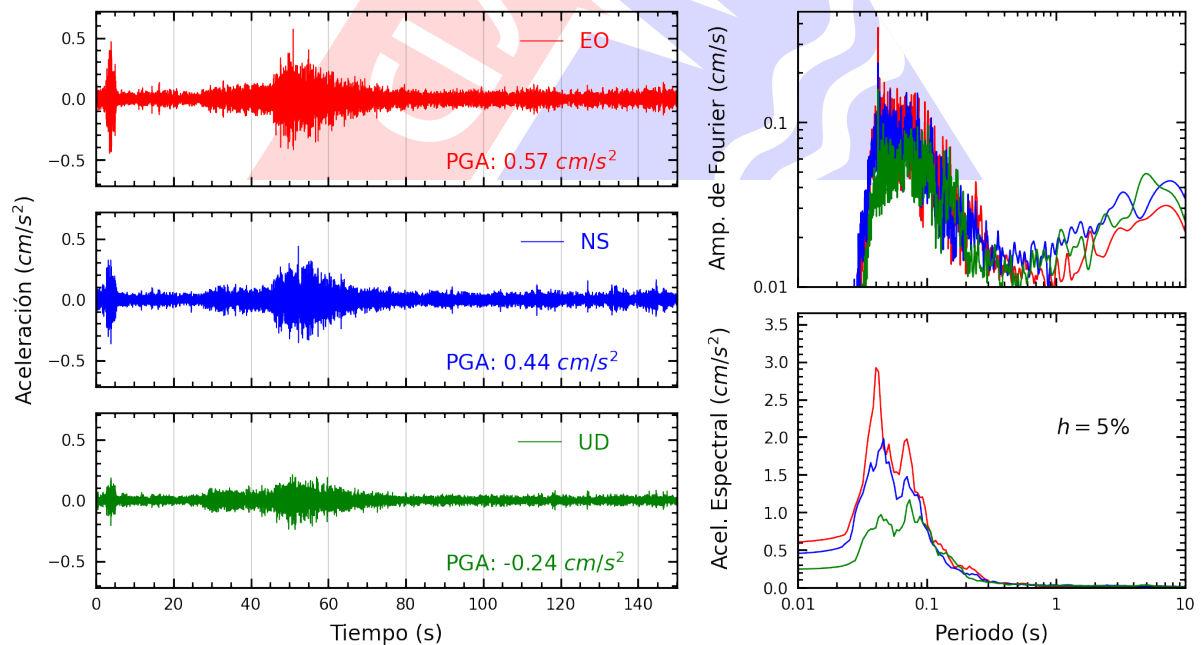
Figura A.20: Registros tiempo-historia, espectros de Fourier y de respuesta en las direcciones EO, NS y vertical de la estación CEPRE. Sismo de Chinchá Alta, Chinchá - Ica del 2025-04-26, 13:56:02 (Hora local)
