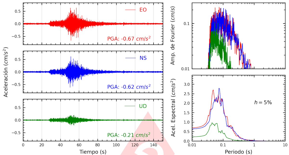
Figura A.19: Registros tiempo-historia, espectros de Fourier y de respuesta en las direcciones EO, NS y vertical de la estación UCVA2. Sismo de Chinchá Alta, Chinchá - Ica del 2025-04-26, 13:56:02 (Hora local)
