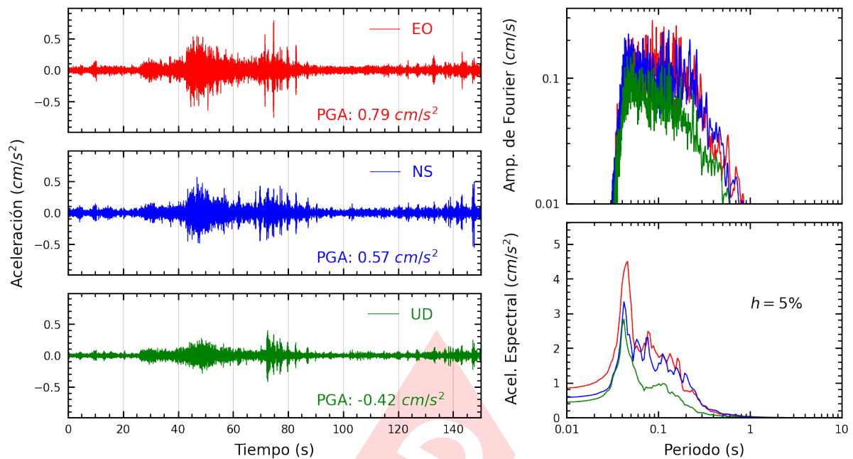
Figura A.11: Registros tiempo-historia, espectros de Fourier y de respuesta en las direcciones EO, NS y vertical de la estación BRIS2. Sismo de Chincha Alta, Chincha - Ica del 2025-04-26, 13:56:02 (Hora local)
