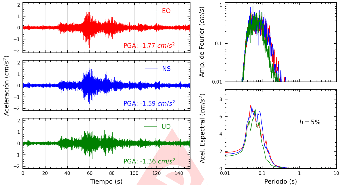
Figura A.3: Registros tiempo-historia, espectros de Fourier y de respuesta en las direcciones EO, NS y vertical de la estación SROS2. Sismo de Chinchá Alta, Chinchá - Ica del 2025-04-26, 13:56:02 (Hora local)
