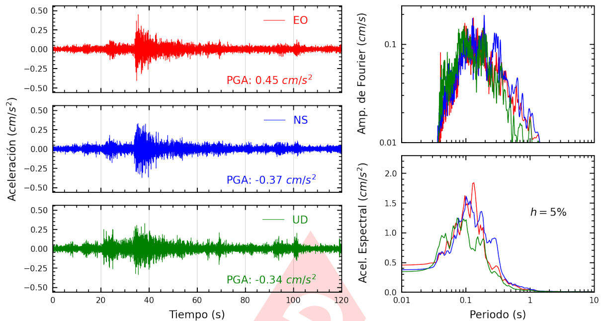
Figura A.27: Registros tiempo-historia, espectros de Fourier y de respuesta en las direcciones EO, NS y vertical de la estación UNICA. Sismo de Chinchá Alta, Chinchá - Ica del 2025-04-26, 13:56:02 (Hora local)
