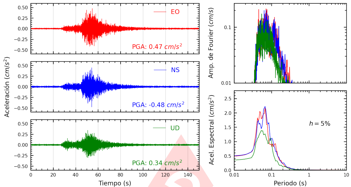
Figura A.25: Registros tiempo-historia, espectros de Fourier y de respuesta en las direcciones EO, NS y vertical de la estación ATARJ. Sismo de Chinchá Alta, Chinchá - Ica del 2025-04-26, 13:56:02 (Hora local)
