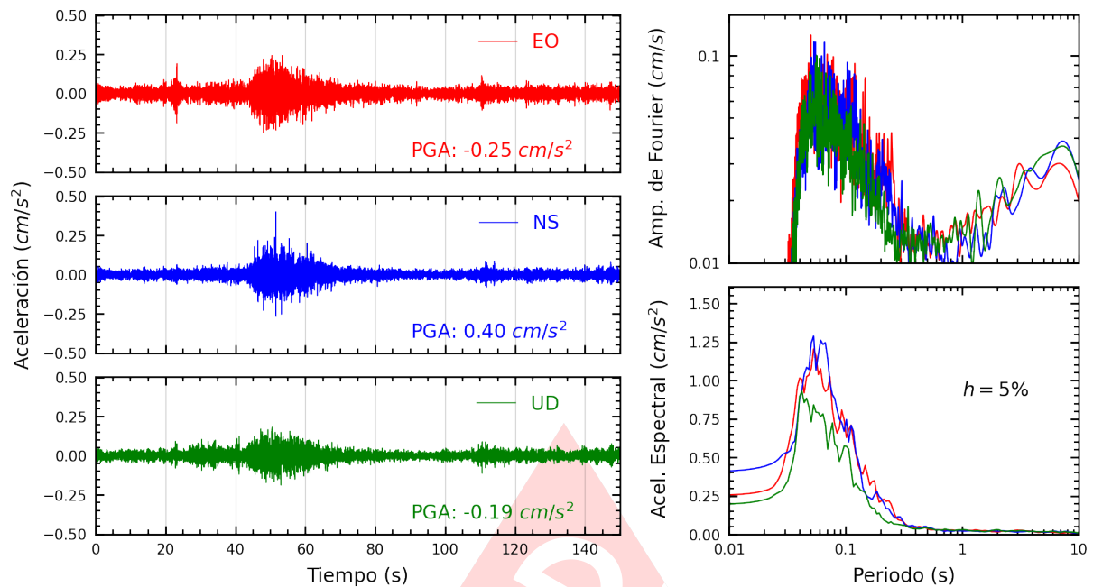
Figura A.29: Registros tiempo-historia, espectros de Fourier y de respuesta en las direcciones EO, NS y vertical de la estación INICT. Sismo de Chinchá Alta, Chinchá - Ica del 2025-04-26, 13:56:02 (Hora local)
