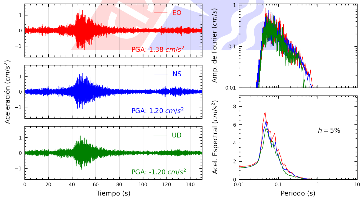
Figura A.6: Registros tiempo-historia, espectros de Fourier y de respuesta en las direcciones EO, NS y vertical de la estación UNTEL. Sismo de Chinchá Alta, Chinchá - Ica del 2025-04-26, 13:56:02 (Hora local)
