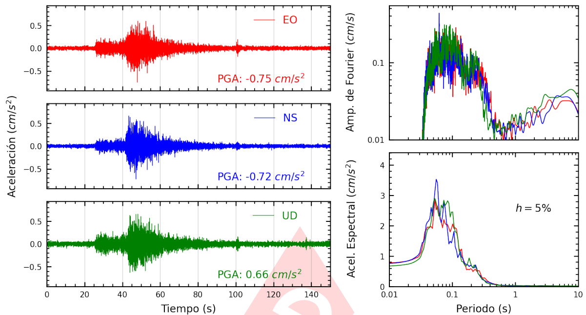
Figura A.13: Registros tiempo-historia, espectros de Fourier y de respuesta en las direcciones EO, NS y vertical de la estación SOVES. Sismo de Chinchá Alta, Chinchá - Ica del 2025-04-26, 13:56:02 (Hora local)
