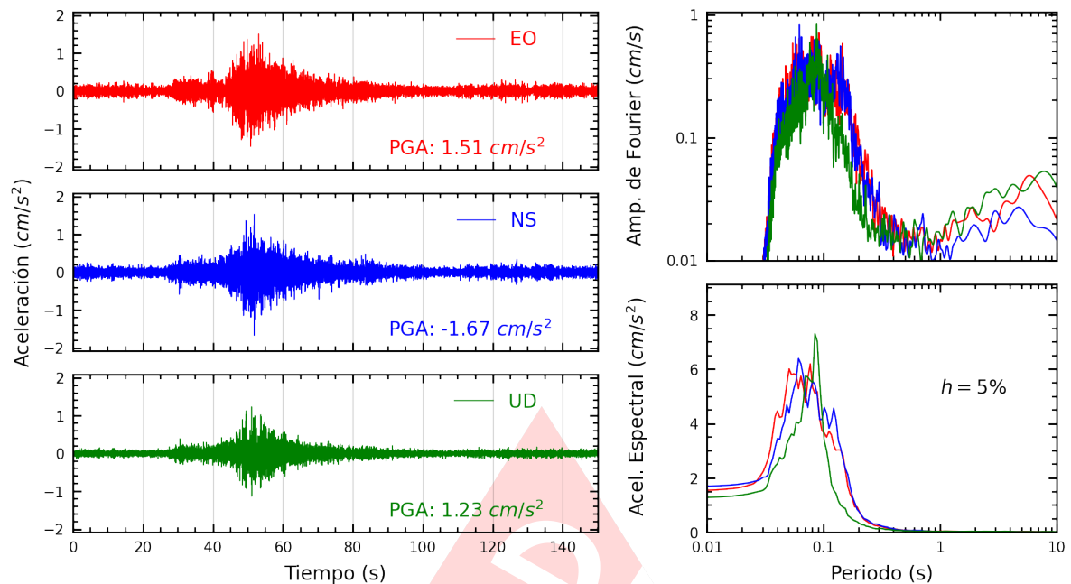
Figura A.5: Registros tiempo-historia, espectros de Fourier y de respuesta en las direcciones EO, NS y vertical de la estación USILM. Sismo de Chinchá Alta, Chinchá - Ica del 2025-04-26, 13:56:02 (Hora local)
