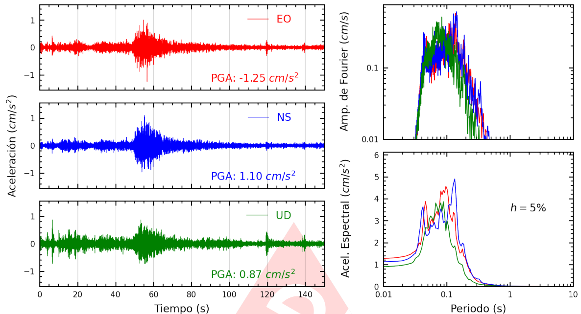
Figura A.9: Registros tiempo-historia, espectros de Fourier y de respuesta en las direcciones EO, NS y vertical de la estación CARA2. Sismo de Chinchá Alta, Chinchá - Ica del 2025-04-26, 13:56:02 (Hora local)
