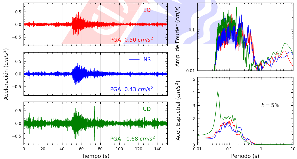
Figura A.18: Registros tiempo-historia, espectros de Fourier y de respuesta en las direcciones EO, NS y vertical de la estación MDPP. Sismo de Chincha Alta, Chincha - Ica del 2025-04-26, 13:56:02 (Hora local)
