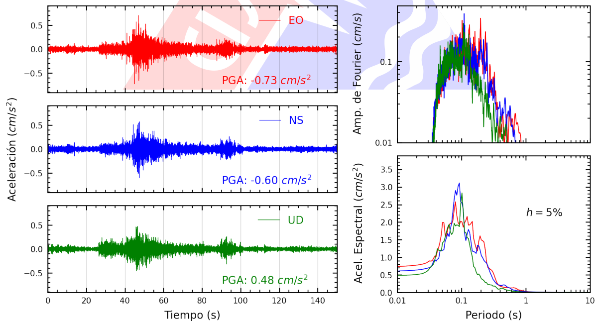
Figura A.14: Registros tiempo-historia, espectros de Fourier y de respuesta en las direcciones EO, NS y vertical de la estación SCCHO. Sismo de Chinchá Alta, Chinchá - Ica del 2025-04-26, 13:56:02 (Hora local)
