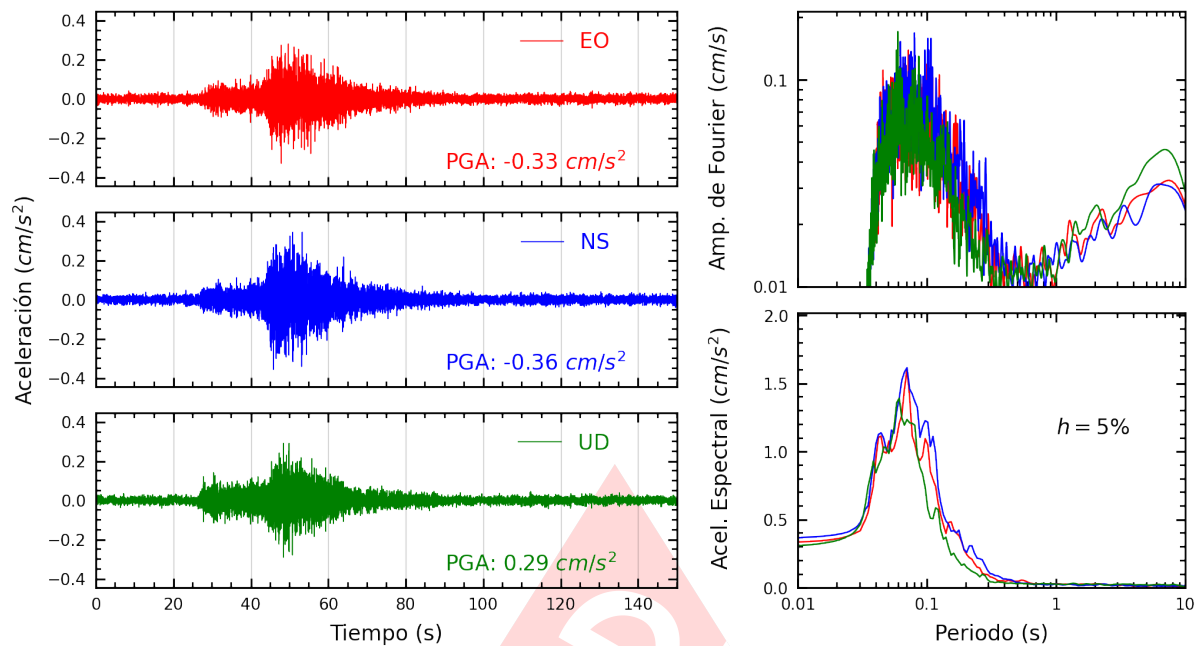
Figura A.31: Registros tiempo-historia, espectros de Fourier y de respuesta en las direcciones EO, NS y vertical de la estación SERVI. Sismo de Chinchá Alta, Chinchá - Ica del 2025-04-26, 13:56:02 (Hora local)
