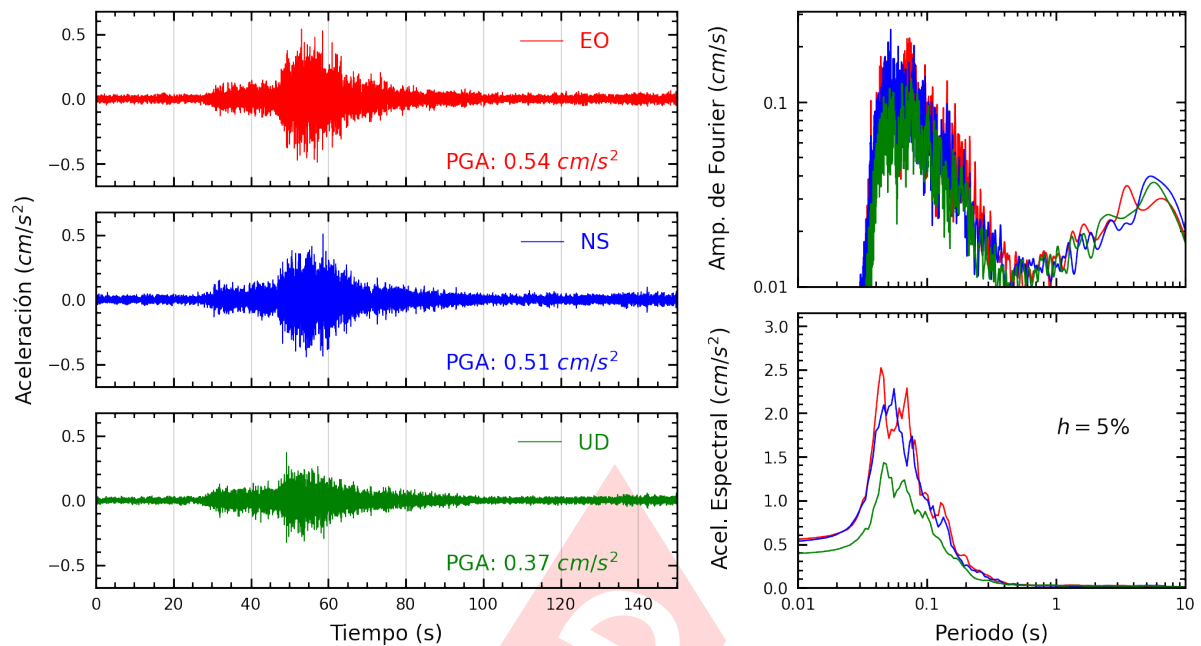
Figura A.23: Registros tiempo-historia, espectros de Fourier y de respuesta en las direcciones EO, NS y vertical de la estación FICPE. Sismo de Chinchá Alta, Chinchá - Ica del 2025-04-26, 13:56:02 (Hora local)
