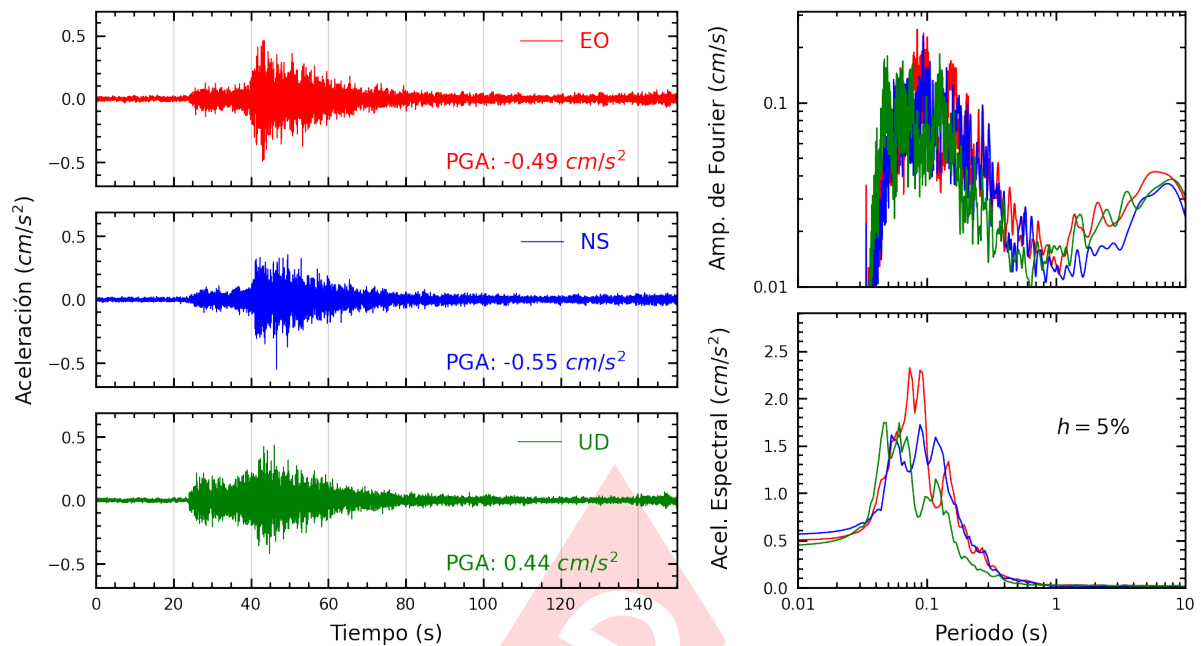
Figura A.21: Registros tiempo-historia, espectros de Fourier y de respuesta en las direcciones EO, NS y vertical de la estación USILP. Sismo de Chinchá Alta, Chinchá - Ica del 2025-04-26, 13:56:02 (Hora local)
