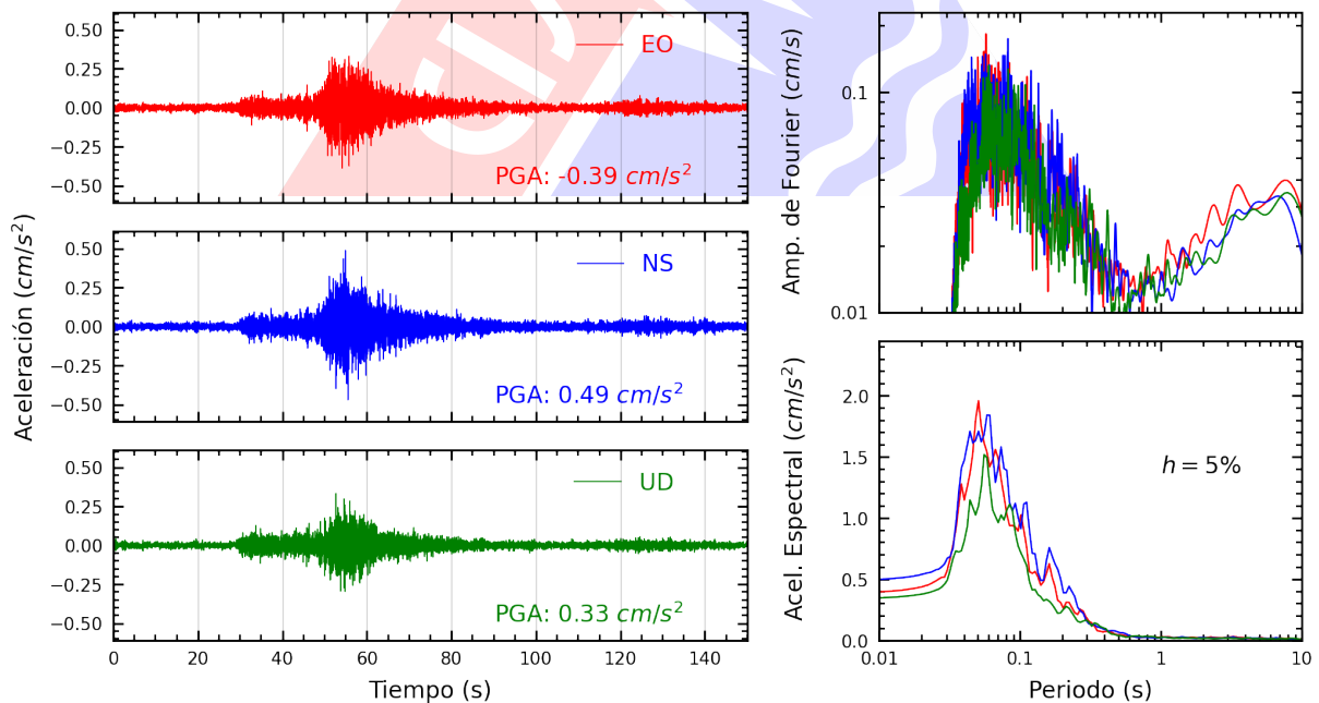
Figura A.24: Registros tiempo-historia, espectros de Fourier y de respuesta en las direcciones EO, NS y vertical de la estación COMAS. Sismo de Chinchá Alta, Chinchá - Ica del 2025-04-26, 13:56:02 (Hora local)
