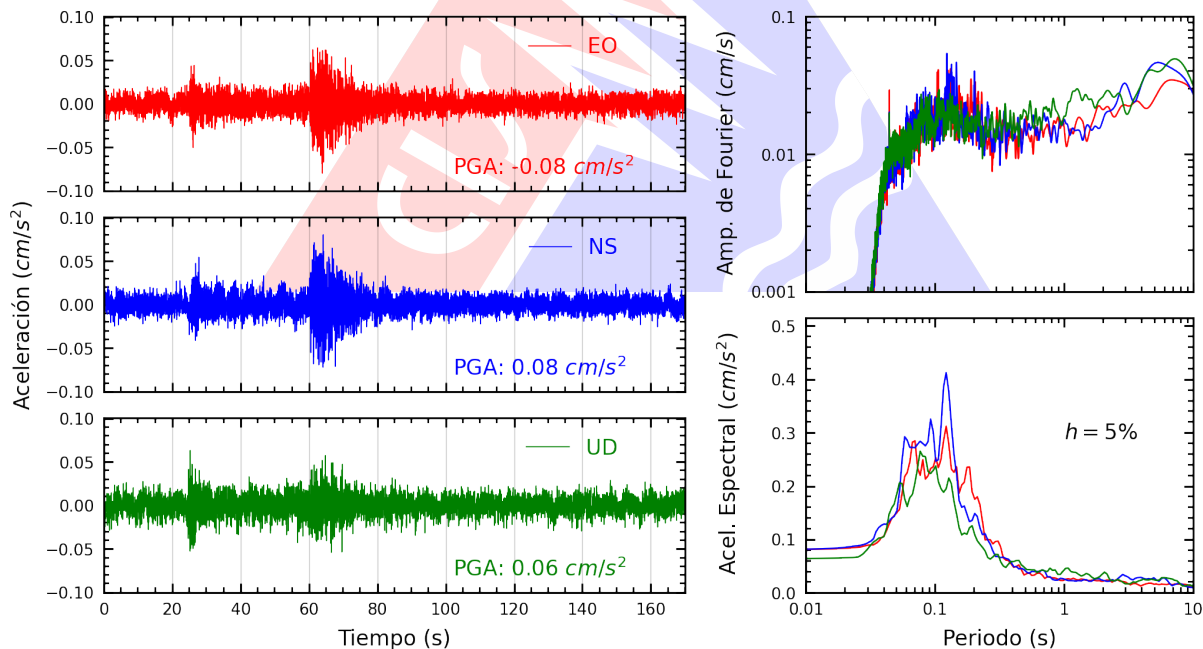
Figura A.2: Registros tiempo-historia, espectros de Fourier y de respuesta en las direcciones EO, NS y vertical de la estación UNTRM. Sismo de Contamana, Ucayali - Loreto del 2025-04-30, 18:53:54 (Hora local)
