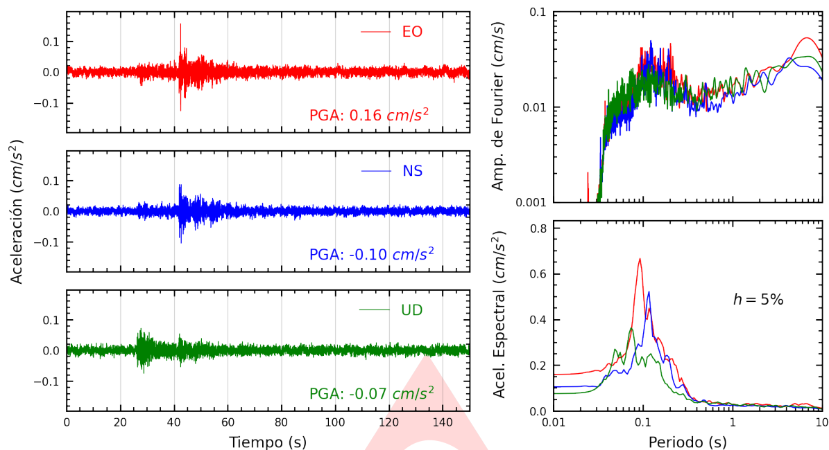
Figura A.1: Registros tiempo-historia, espectros de Fourier y de respuesta en las direcciones EO, NS y vertical de la estación UCVCH. Sismo de Cutervo, Cutervo - Cajamarca del 2025-05-02, 14:37:05 (Hora local)
