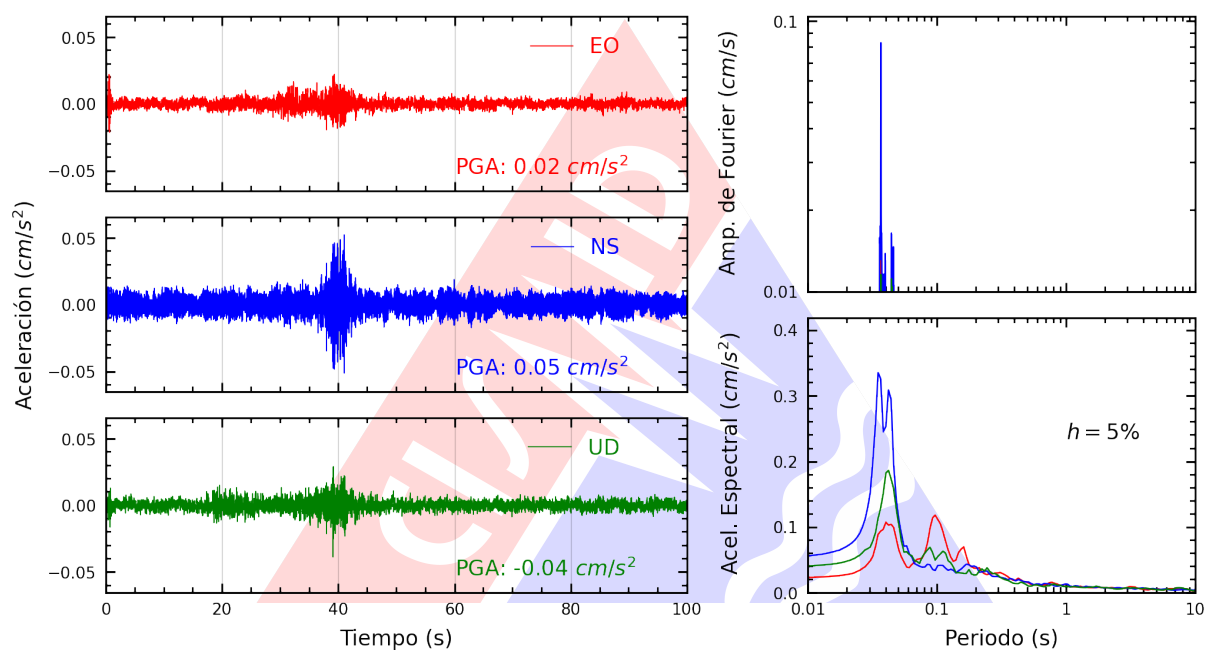
Figura A.3: Registros tiempo-historia, espectros de Fourier y de respuesta en las direcciones EO, NS y vertical de la estación UNJ. Sismo de Cutervo, Cutervo - Cajamarca del 2025-05-02, 14:37:05 (Hora local)
