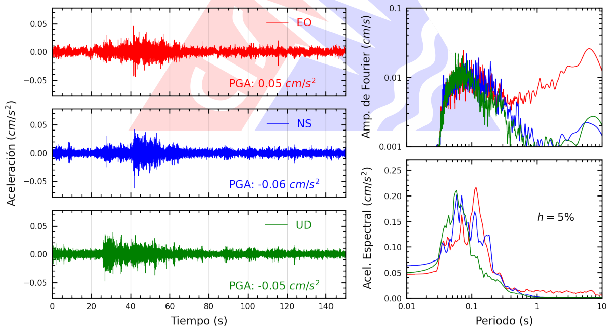
Figura A.2: Registros tiempo-historia, espectros de Fourier y de respuesta en las direcciones EO, NS y vertical de la estación SCCHI. Sismo de Cutervo, Cutervo - Cajamarca del 2025-05-02, 14:37:05 (Hora local)
