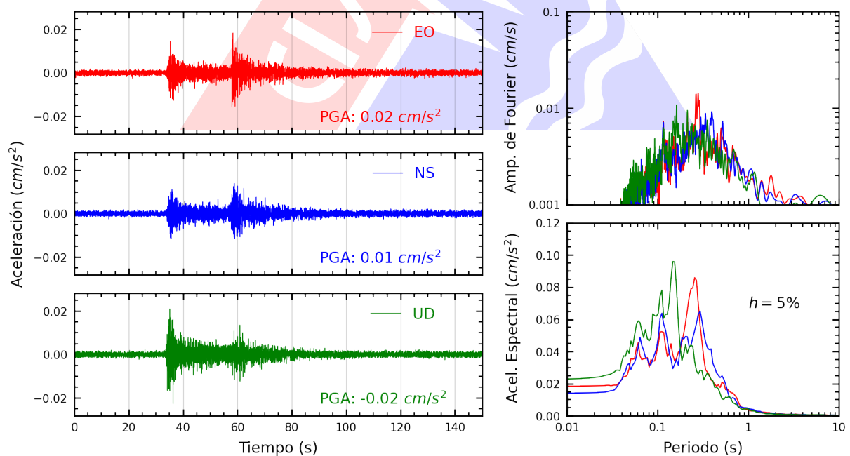
Figura A.4: Registros tiempo-historia, espectros de Fourier y de respuesta en las direcciones EO, NS y vertical de la estación UNCP. Sismo de Huancabamba, Oxapampa - Pasco del 2025-05-03, 03:21:30 (Hora local)
