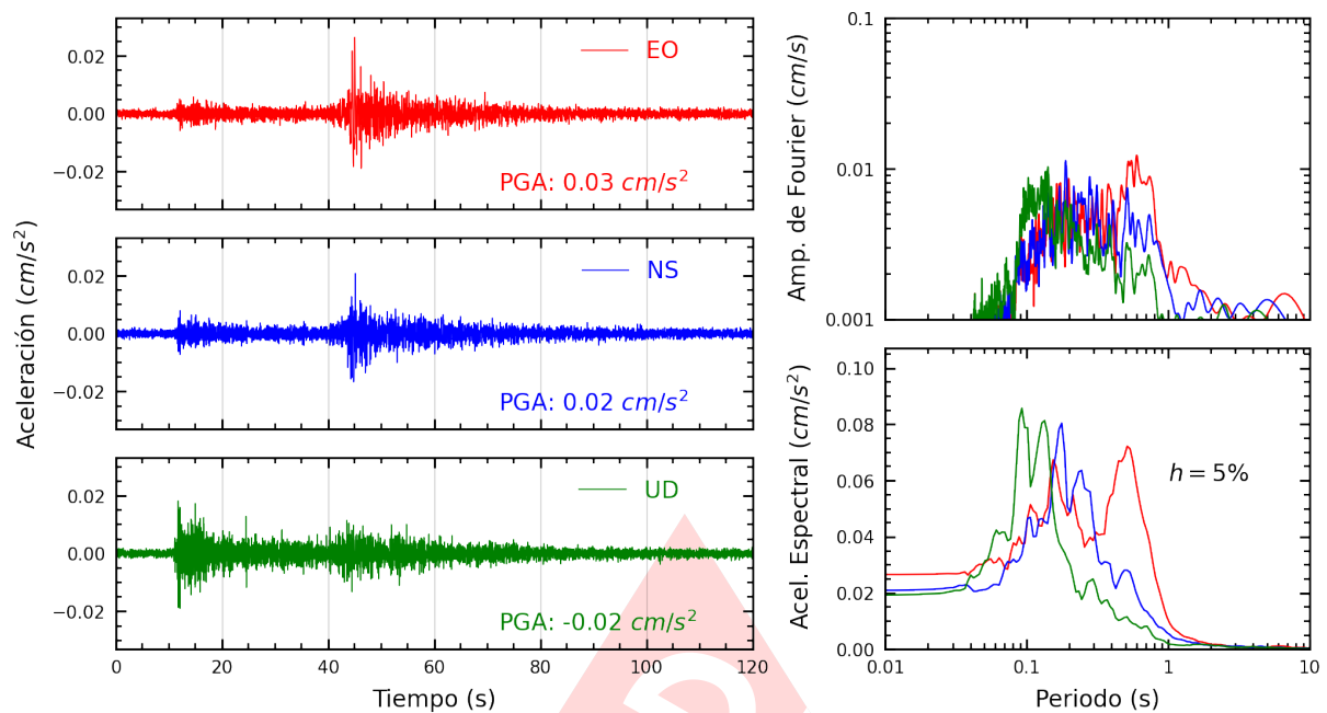
Figura A.3: Registros tiempo-historia, espectros de Fourier y de respuesta en las direcciones EO, NS y vertical de la estación UNIA. Sismo de Huancabamba, Oxapampa - Pasco del 2025-05-03, 03:21:30 (Hora local)
