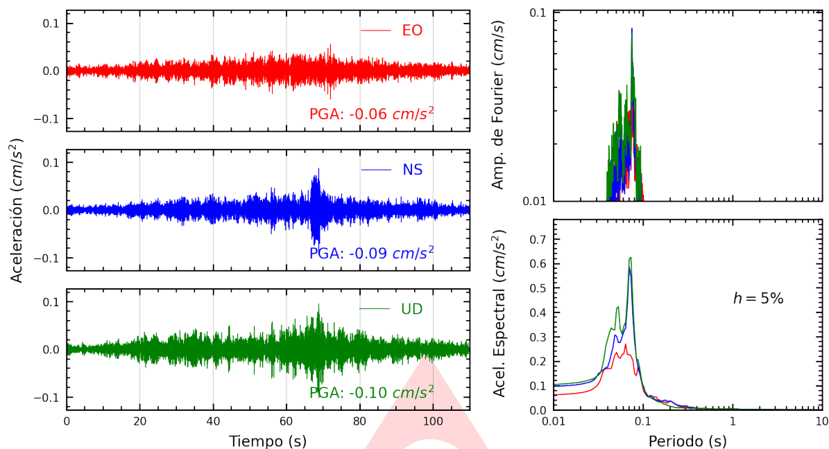
Figura A.1: Registros tiempo-historia, espectros de Fourier y de respuesta en las direcciones EO, NS y vertical de la estación ASIA. Sismo de Huancabamba, Oxapampa - Pasco del 2025-05-03, 03:21:30 (Hora local)
