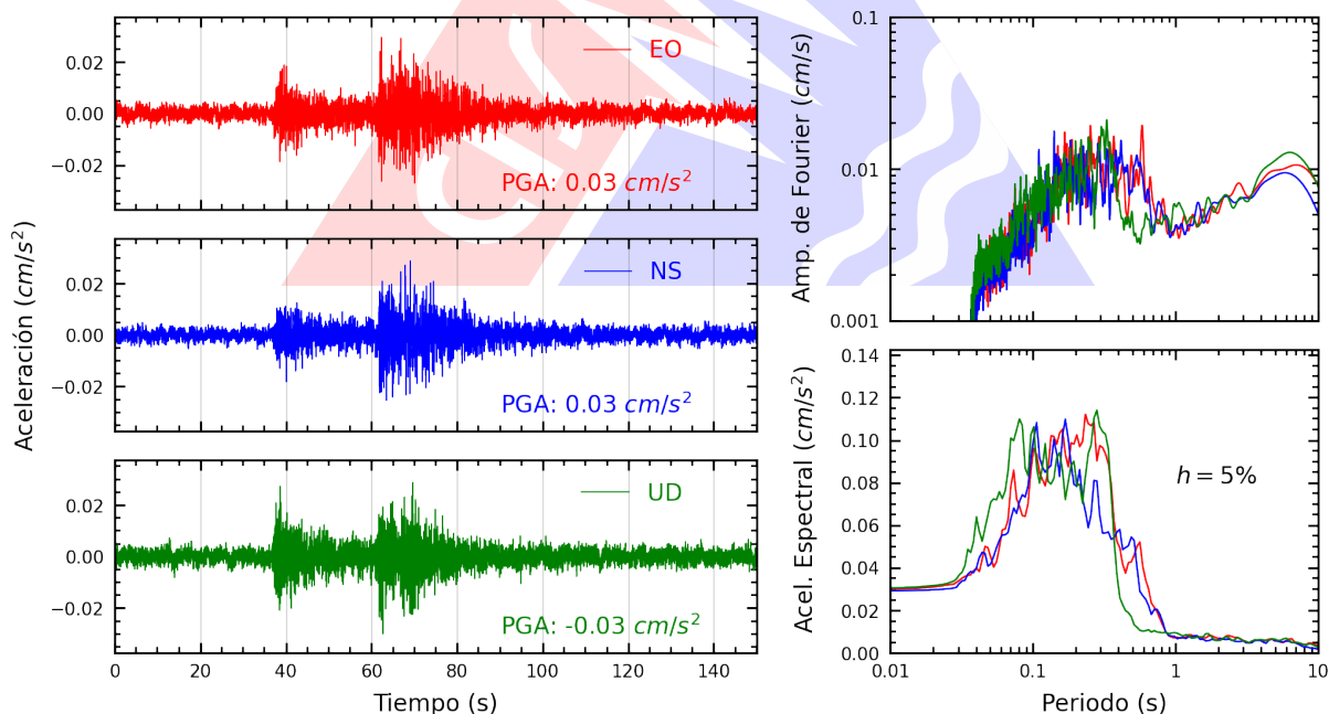
Figura A.2: Registros tiempo-historia, espectros de Fourier y de respuesta en las direcciones EO, NS y vertical de la estación CARAL. Sismo de Huancabamba, Oxapampa - Pasco del 2025-05-03, 03:21:30 (Hora local)
