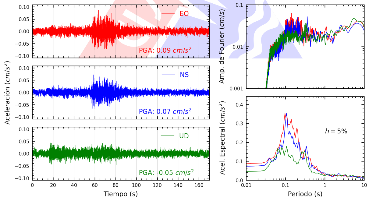
Figura A.4: Registros tiempo-historia, espectros de Fourier y de respuesta en las direcciones EO, NS y vertical de la estación UCVCH. Sismo de Zarumilla, Zarumilla - Tumbes del 2025-05-05, 04:17:19 (Hora local)
