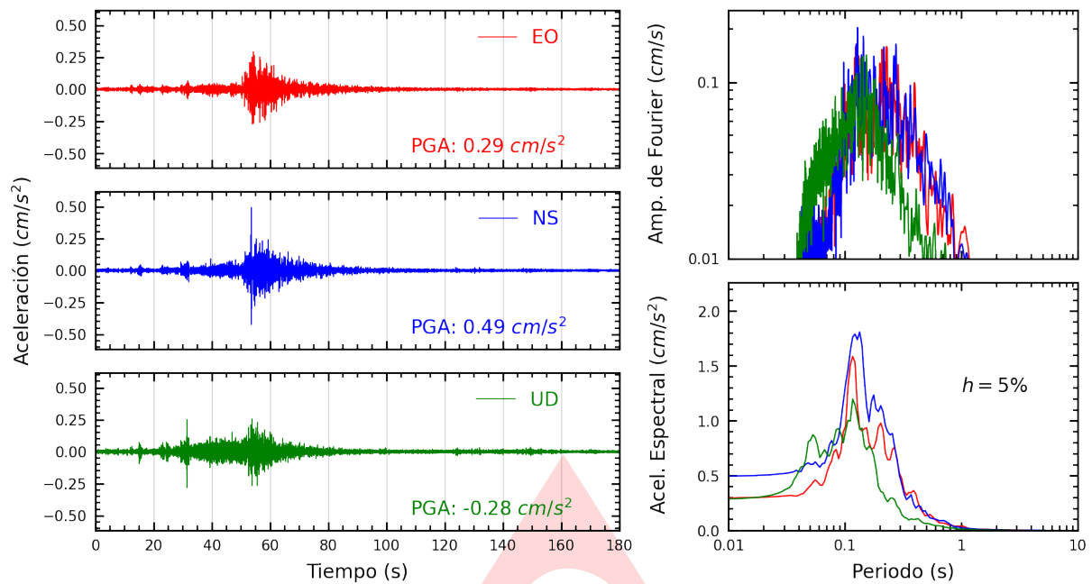
Figura A.1: Registros tiempo-historia, espectros de Fourier y de respuesta en las direcciones EO, NS y vertical de la estación UNP. Sismo de Zarumilla, Zarumilla - Tumbes del 2025-05-05, 04:17:19 (Hora local)
