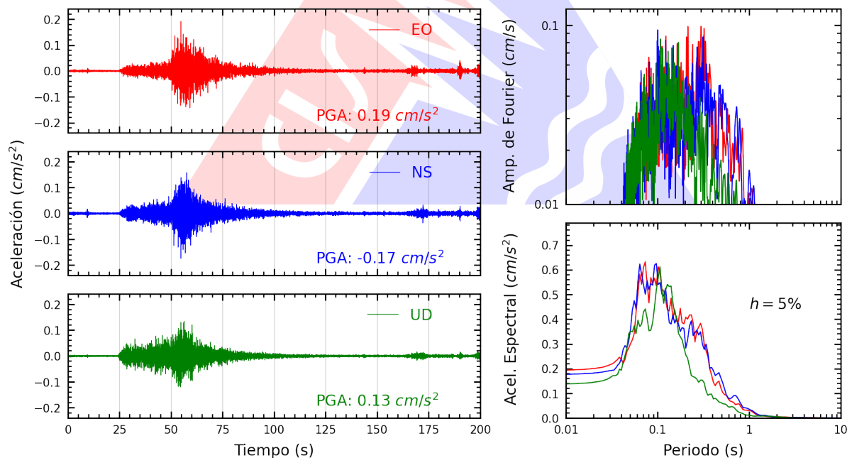
Figura A.2: Registros tiempo-historia, espectros de Fourier y de respuesta en las direcciones EO, NS y vertical de la estación UPAOP. Sismo de Zarumilla, Zarumilla - Tumbes del 2025-05-05, 04:17:19 (Hora local)
