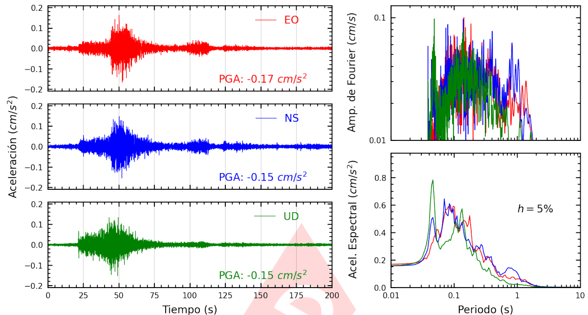
Figura A.3: Registros tiempo-historia, espectros de Fourier y de respuesta en las direcciones EO, NS y vertical de la estación UNF. Sismo de Zarumilla, Zarumilla - Tumbes del 2025-05-05, 04:17:19 (Hora local)
