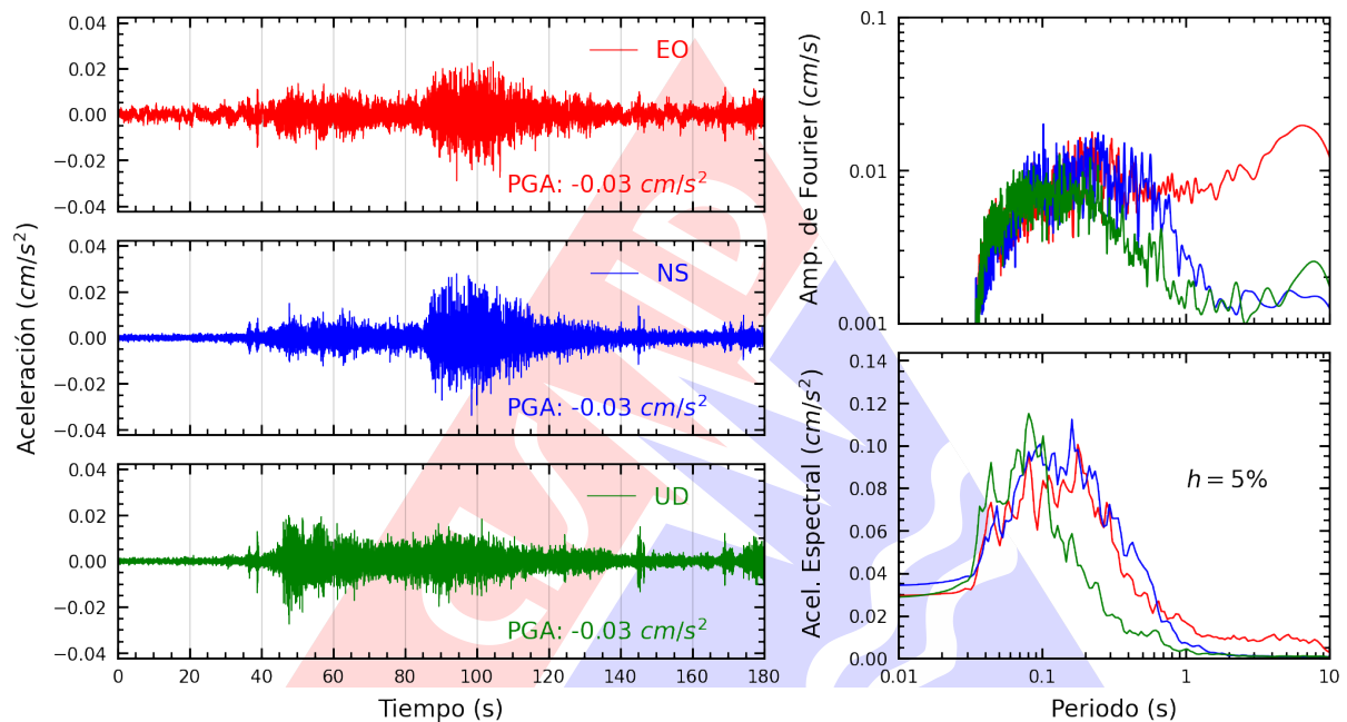
Figura A.5: Registros tiempo-historia, espectros de Fourier y de respuesta en las direcciones EO, NS y vertical de la estación SCCHI. Sismo de Zarumilla, Zarumilla - Tumbes del 2025-05-05, 04:17:19 (Hora local)
