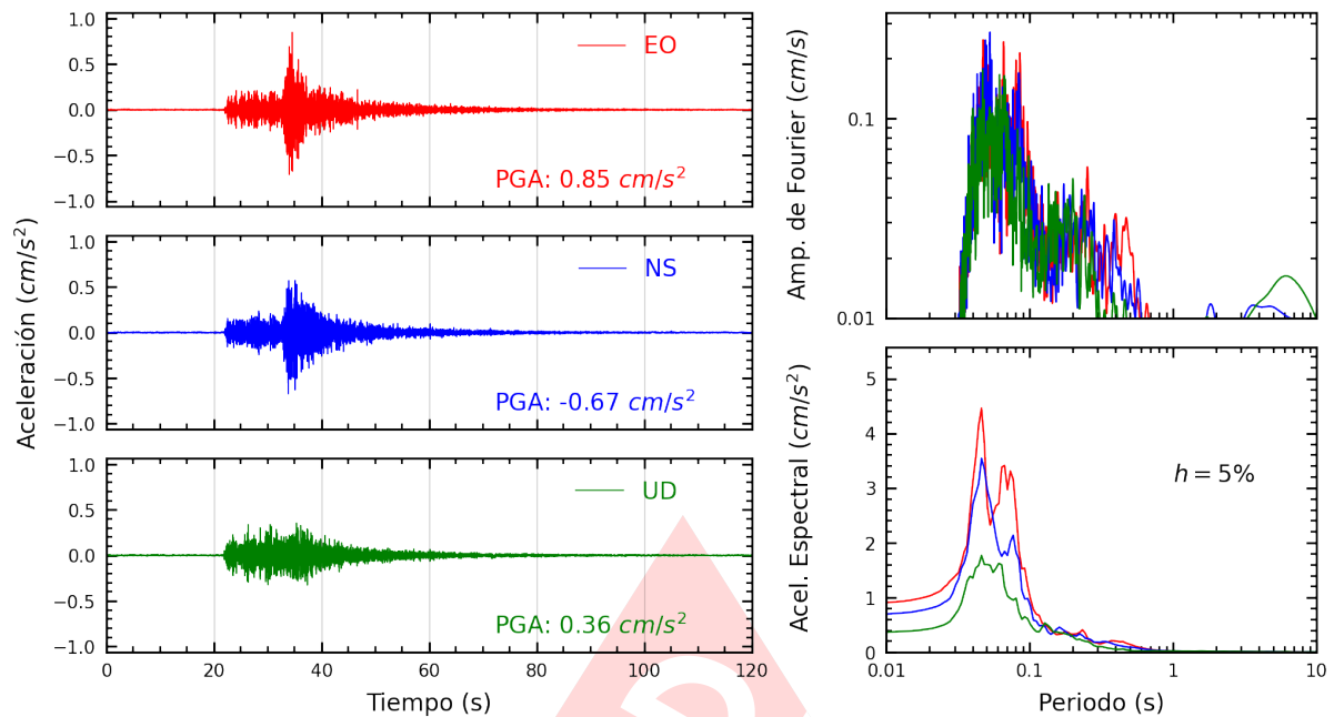
Figura A.5: Registros tiempo-historia, espectros de Fourier y de respuesta en las direcciones EO, NS y vertical de la estación CREY. Sismo de Locumba, Jorge Basadre - Tacna del 2025-05-07, 03:06:37 (Hora local)
