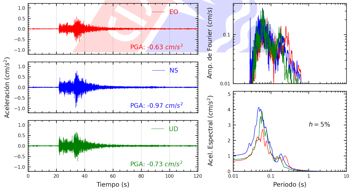
Figura A.4: Registros tiempo-historia, espectros de Fourier y de respuesta en las direcciones EO, NS y vertical de la estación UJBG4. Sismo de Locumba, Jorge Basadre - Tacna del 2025-05-07, 03:06:37 (Hora local)
