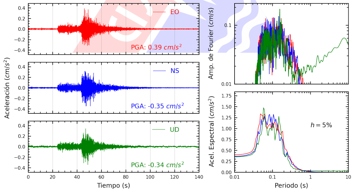
Figura A.6: Registros tiempo-historia, espectros de Fourier y de respuesta en las direcciones EO, NS y vertical de la estación SCARQ. Sismo de Locumba, Jorge Basadre - Tacna del 2025-05-07, 03:06:37 (Hora local)
