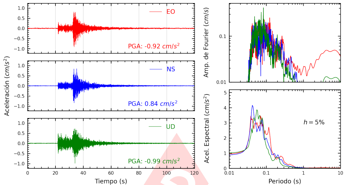
Figura A.3: Registros tiempo-historia, espectros de Fourier y de respuesta en las direcciones EO, NS y vertical de la estación UJBG3. Sismo de Locumba, Jorge Basadre - Tacna del 2025-05-07, 03:06:37 (Hora local)
