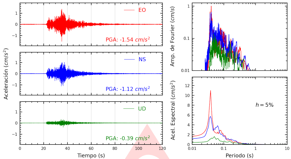
Figura A.1: Registros tiempo-historia, espectros de Fourier y de respuesta en las direcciones EO, NS y vertical de la estación UNAM. Sismo de Locumba, Jorge Basadre - Tacna del 2025-05-07, 03:06:37 (Hora local)
