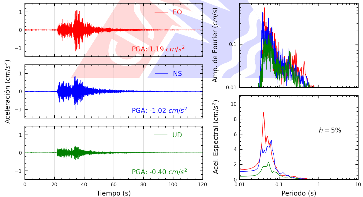
Figura A.2: Registros tiempo-historia, espectros de Fourier y de respuesta en las direcciones EO, NS y vertical de la estación UPTAC. Sismo de Locumba, Jorge Basadre - Tacna del 2025-05-07, 03:06:37 (Hora local)
