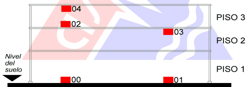
Figura 4: Distribución de sensores en la estructura monitoreada
