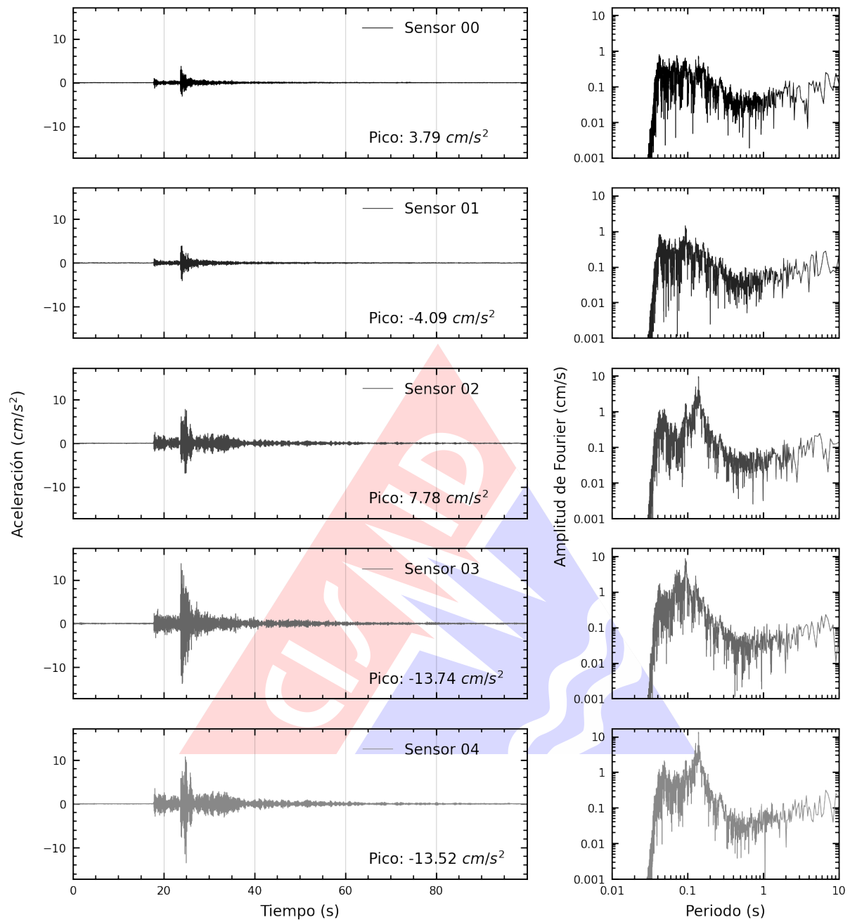
Figura A.1: Registros tiempo-historia y espectros de Fourier en la dirección EW de la estructura Centro de Observación para la Ingeniería Sísmica del CISMID-FIC-UNI. Sismo de Provincia Constitucional del Callao , Callao - Lima del 2025-05-07, 09:44:57 (Hora local)
