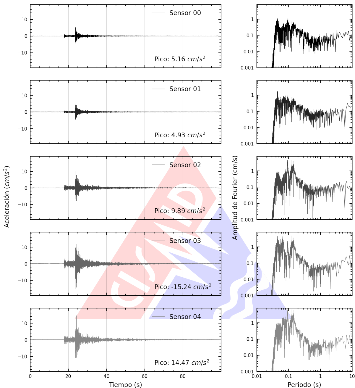
Figura A.2: Registros tiempo-historia y espectros de Fourier en la dirección NS de la estructura Centro de Observación para la Ingeniería Sísmica del CISMID-FIC-UNI. Sismo de Provincia Constitucional del Callao , Callao - Lima del 2025-05-07, 09:44:57 (Hora local)
