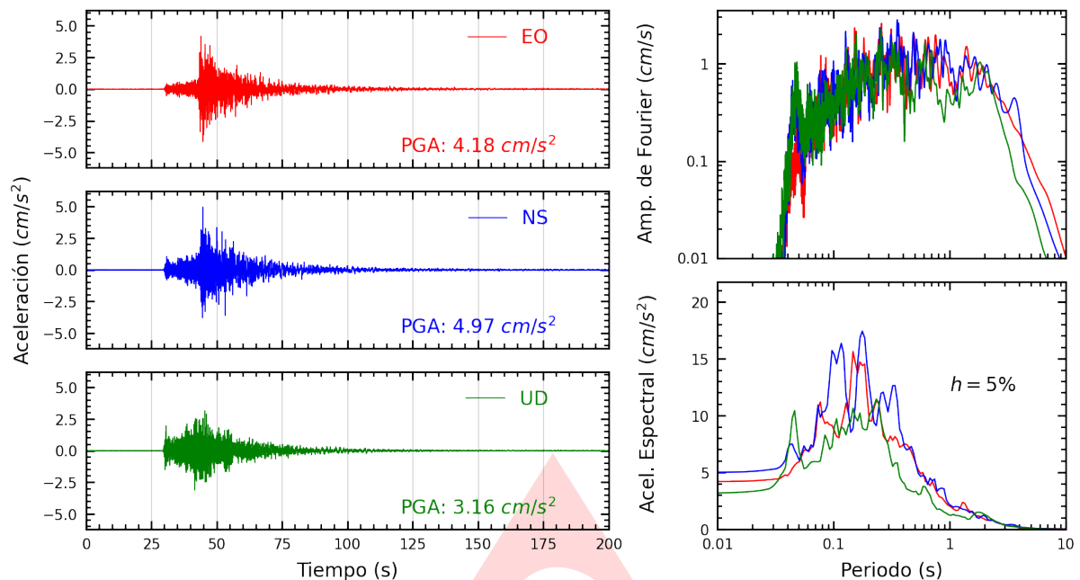
Figura A.1: Registros tiempo-historia, espectros de Fourier y de respuesta en las direcciones EO, NS y vertical de la estación UNF. Sismo de Zorritos, Contralmirante Villar - Tumbes del 2025-05-08, 06:22:39 (Hora local)
