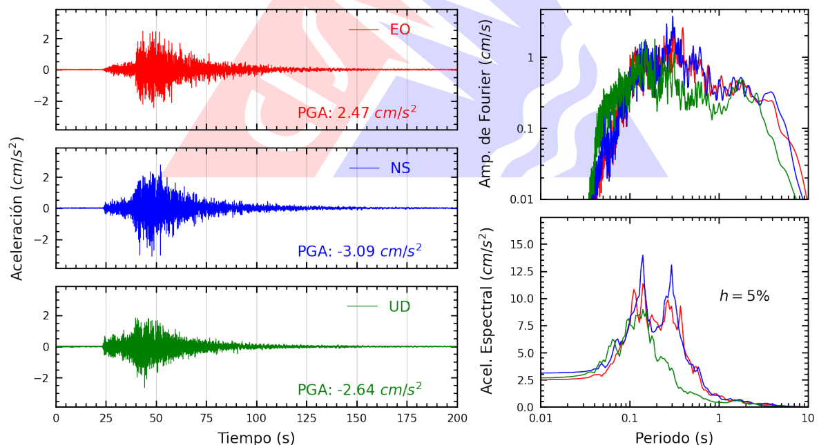
Figura A.2: Registros tiempo-historia, espectros de Fourier y de respuesta en las direcciones EO, NS y vertical de la estación UNP. Sismo de Zorritos, Contralmirante Villar - Tumbes del 2025-05-08, 06:22:39 (Hora local)
