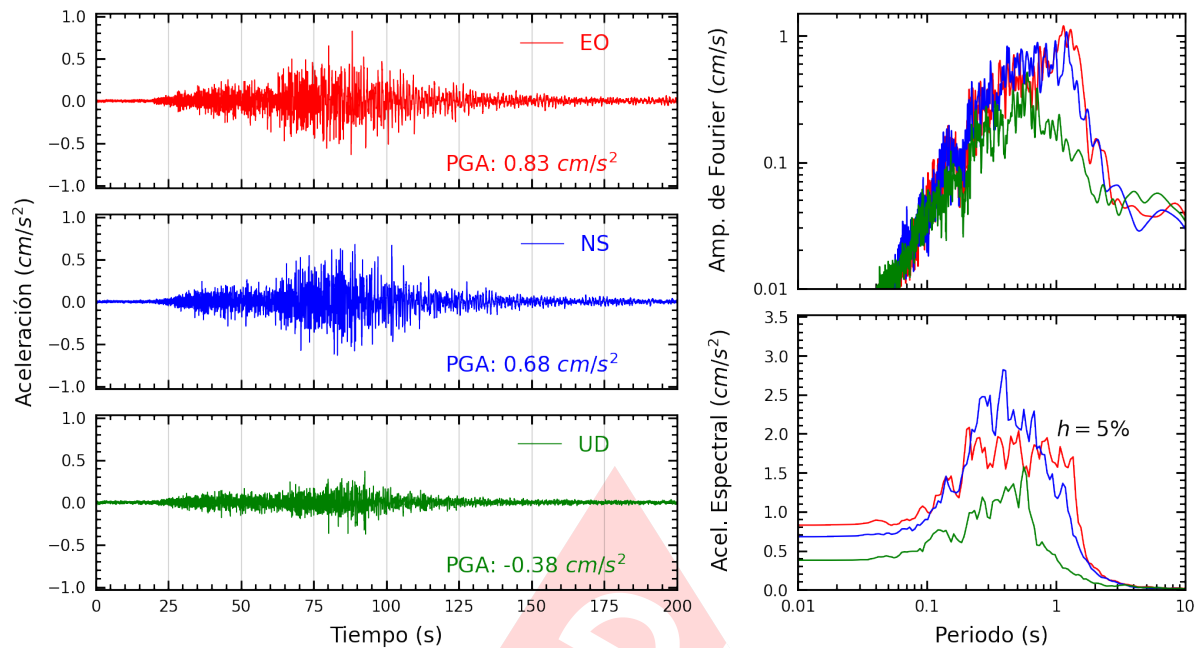
Figura A.5: Registros tiempo-historia, espectros de Fourier y de respuesta en las direcciones EO, NS y vertical de la estación UNTRM. Sismo de Zorritos, Contralmirante Villar - Tumbes del 2025-05-08, 06:22:39 (Hora local)
