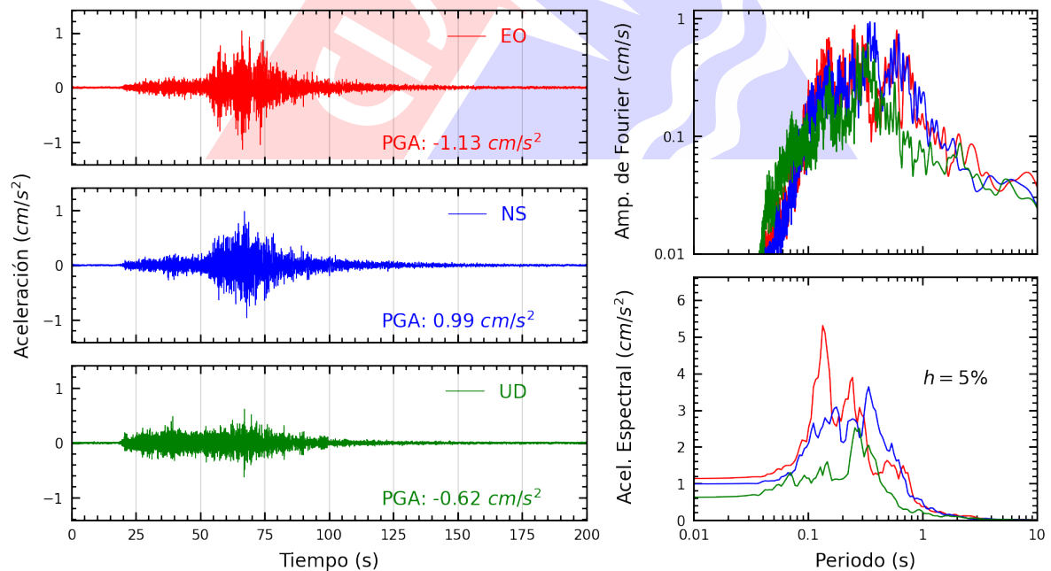
Figura A.4: Registros tiempo-historia, espectros de Fourier y de respuesta en las direcciones EO, NS y vertical de la estación UCVCH. Sismo de Zorritos, Contralmirante Villar - Tumbes del 2025-05-08, 06:22:39 (Hora local)
