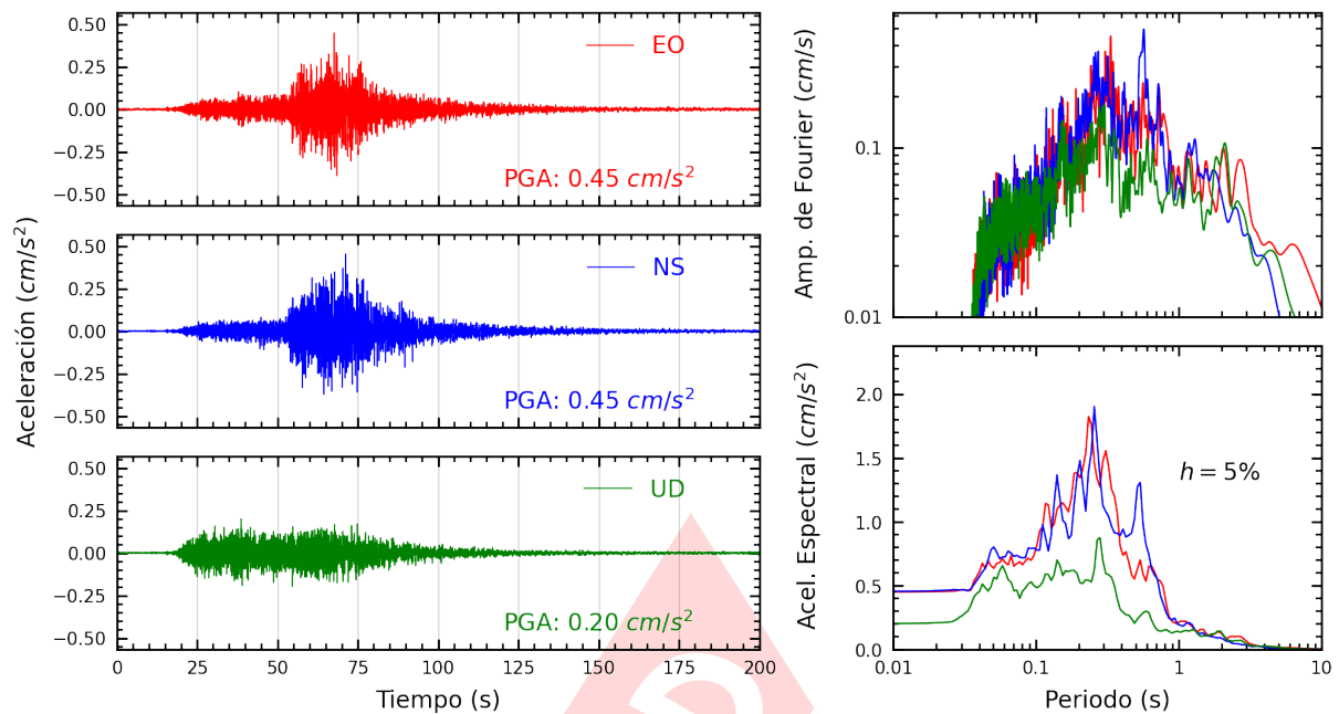
Figura A.7: Registros tiempo-historia, espectros de Fourier y de respuesta en las direcciones EO, NS y vertical de la estación SCCHI. Sismo de Zorritos, Contralmirante Villar - Tumbes del 2025-05-08, 06:22:39 (Hora local)
