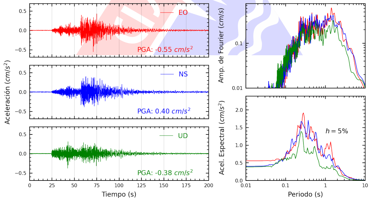
Figura A.6: Registros tiempo-historia, espectros de Fourier y de respuesta en las direcciones EO, NS y vertical de la estación UNJ. Sismo de Zorritos, Contralmirante Villar - Tumbes del 2025-05-08, 06:22:39 (Hora local)
