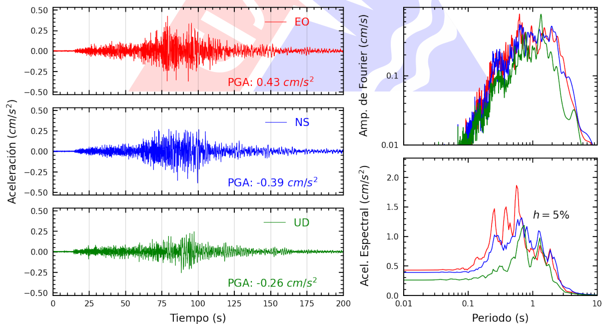
Figura A.8: Registros tiempo-historia, espectros de Fourier y de respuesta en las direcciones EO, NS y vertical de la estación UNC. Sismo de Zorritos, Contralmirante Villar - Tumbes del 2025-05-08, 06:22:39 (Hora local)
