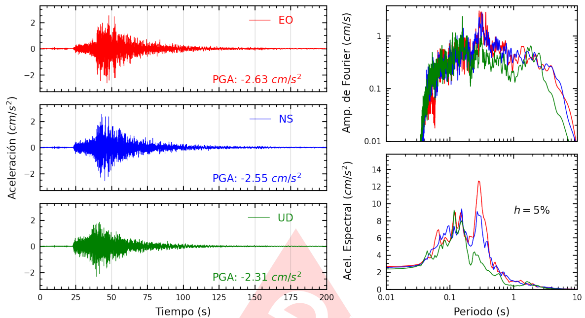
Figura A.3: Registros tiempo-historia, espectros de Fourier y de respuesta en las direcciones EO, NS y vertical de la estación UPAOP. Sismo de Zorritos, Contralmirante Villar - Tumbes del 2025-05-08, 06:22:39 (Hora local)
