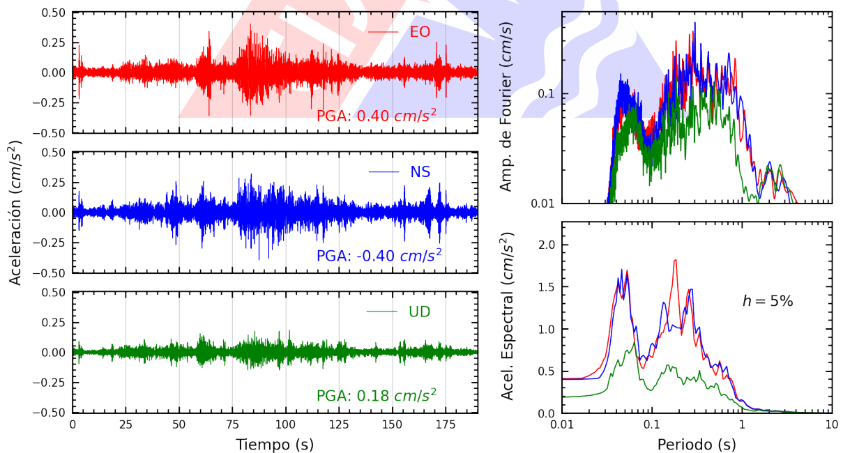
Figura A.8: Registros tiempo-historia, espectros de Fourier y de respuesta en las direcciones EO, NS y vertical de la estación BRIS2. Sismo de Chala, Caraveli - Arequipa del 2025-05-09, 22:34:08 (Hora local)
