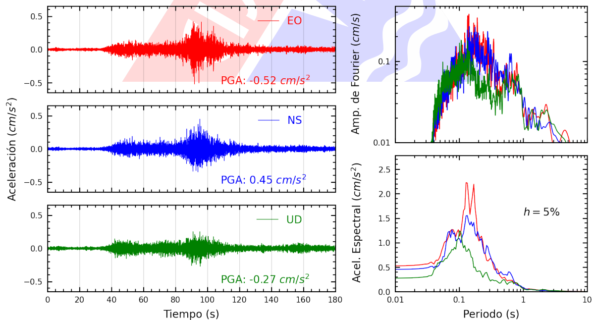
Figura A.6: Registros tiempo-historia, espectros de Fourier y de respuesta en las direcciones EO, NS y vertical de la estación ASIA. Sismo de Chala, Caraveli - Arequipa del 2025-05-09, 22:34:08 (Hora local)
