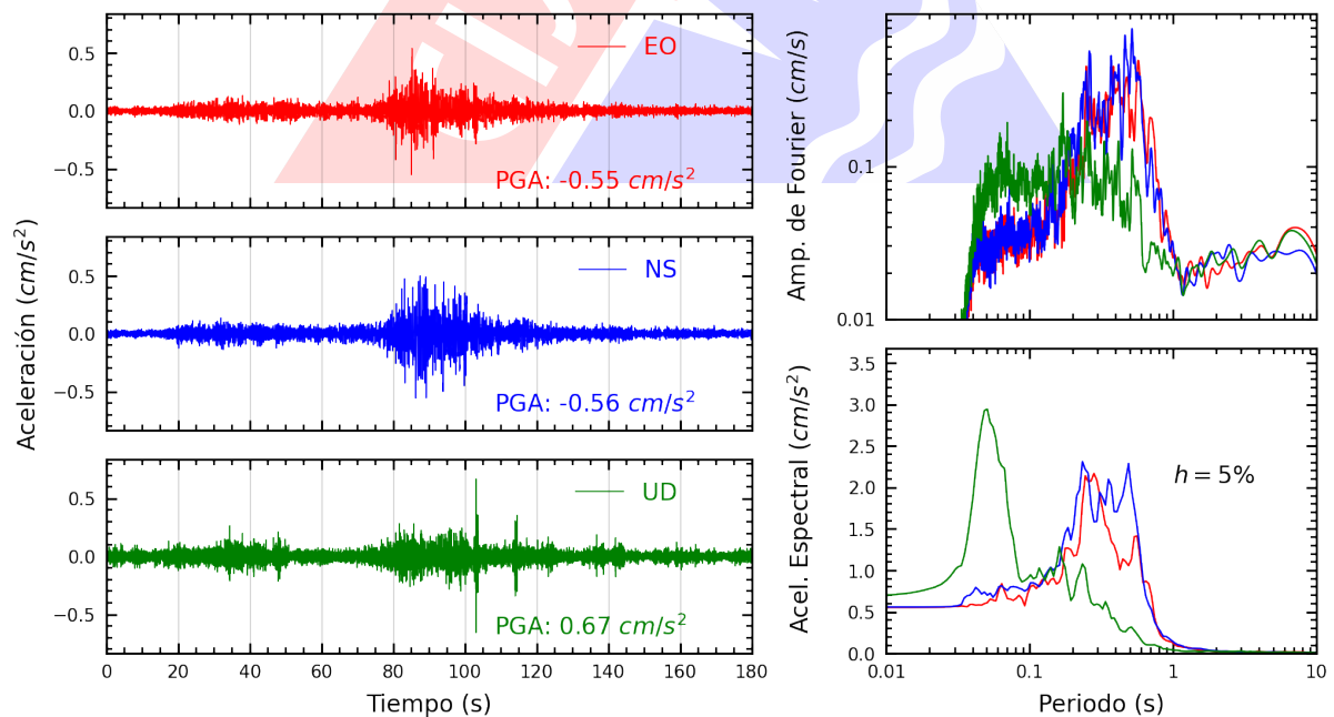
Figura A.4: Registros tiempo-historia, espectros de Fourier y de respuesta en las direcciones EO, NS y vertical de la estación MDPP. Sismo de Chala, Caraveli - Arequipa del 2025-05-09, 22:34:08 (Hora local)
