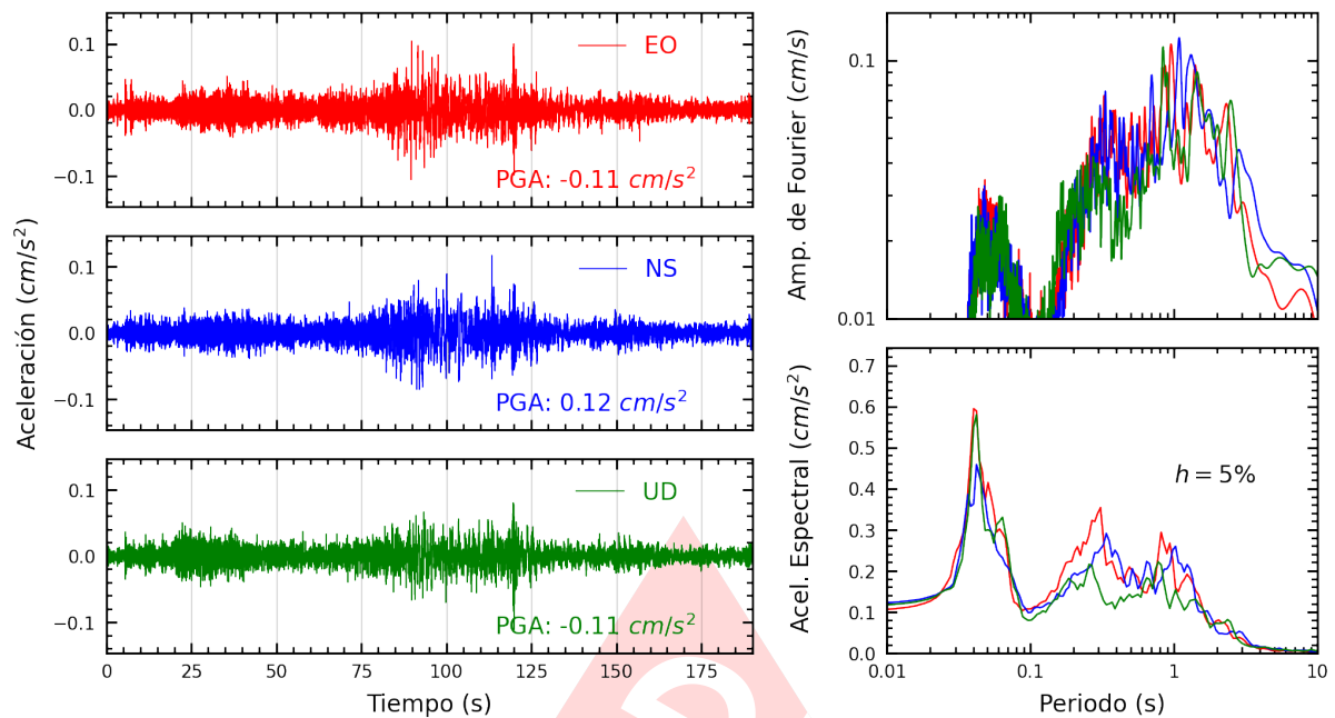
Figura A.25: Registros tiempo-historia, espectros de Fourier y de respuesta en las direcciones EO, NS y vertical de la estación CREY. Sismo de Chala, Caraveli - Arequipa del 2025-05-09, 22:34:08 (Hora local)
