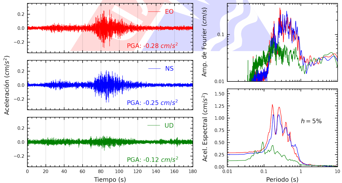
Figura A.12: Registros tiempo-historia, espectros de Fourier y de respuesta en las direcciones EO, NS y vertical de la estación ACAPU. Sismo de Chala, Caraveli - Arequipa del 2025-05-09, 22:34:08 (Hora local)
