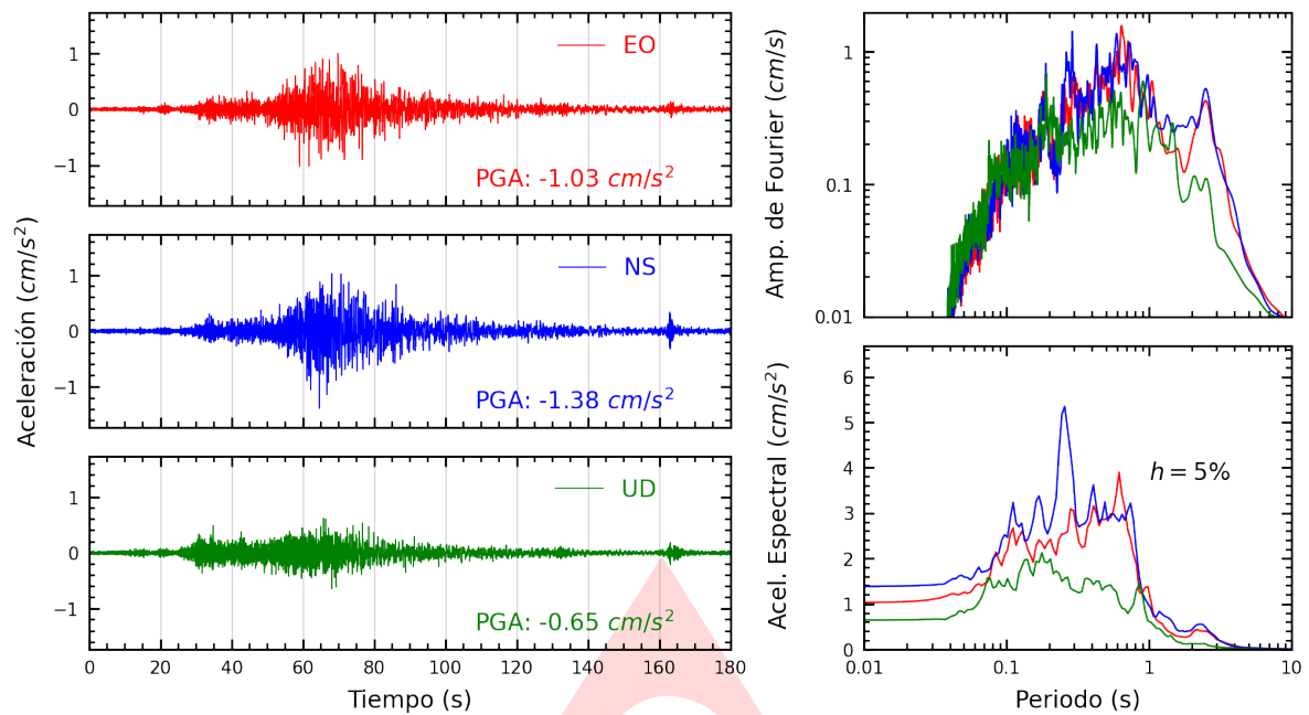
Figura A.1: Registros tiempo-historia, espectros de Fourier y de respuesta en las direcciones EO, NS y vertical de la estación UNICA. Sismo de Chala, Caraveli - Arequipa del 2025-05-09, 22:34:08 (Hora local)
