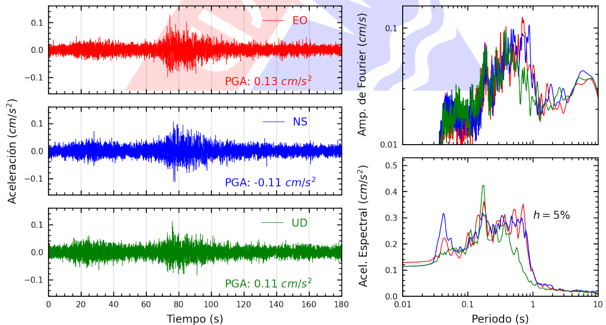
Figura A.24: Registros tiempo-historia, espectros de Fourier y de respuesta en las direcciones EO, NS y vertical de la estación UNFV. Sismo de Chala, Caraveli - Arequipa del 2025-05-09, 22:34:08 (Hora local)
