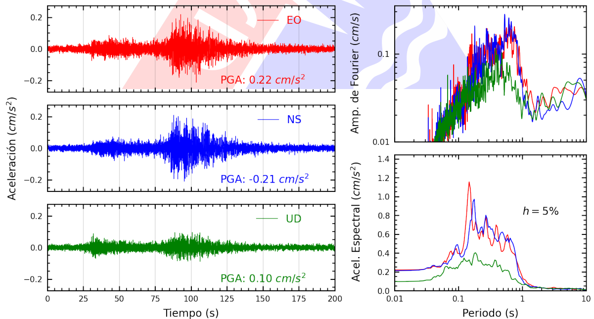
Figura A.16: Registros tiempo-historia, espectros de Fourier y de respuesta en las direcciones EO, NS y vertical de la estación USILP. Sismo de Chala, Caraveli - Arequipa del 2025-05-09, 22:34:08 (Hora local)
