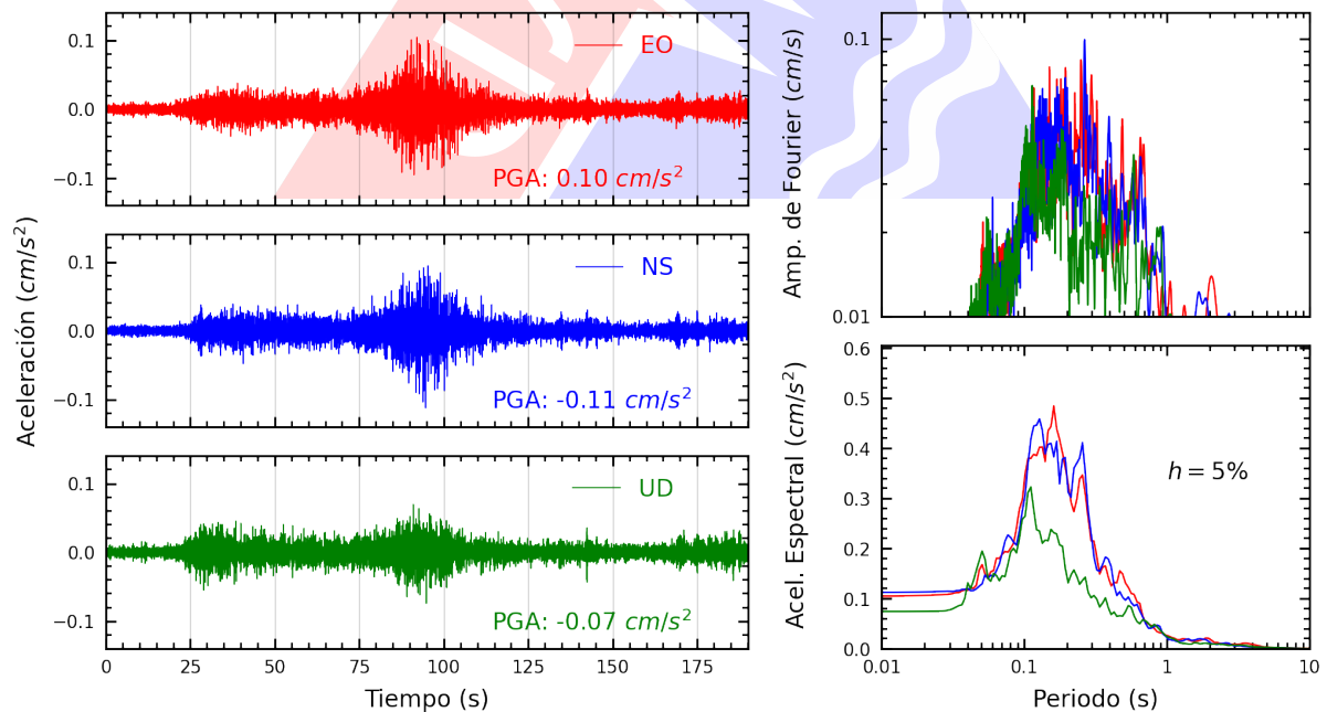
Figura A.26: Registros tiempo-historia, espectros de Fourier y de respuesta en las direcciones EO, NS y vertical de la estación JALV2. Sismo de Chala, Caraveli - Arequipa del 2025-05-09, 22:34:08 (Hora local)
