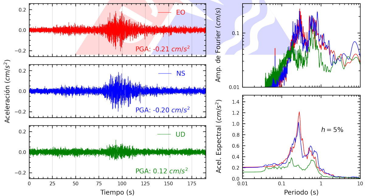
Figura A.18: Registros tiempo-historia, espectros de Fourier y de respuesta en las direcciones EO, NS y vertical de la estación DSMI. Sismo de Chala, Caraveli - Arequipa del 2025-05-09, 22:34:08 (Hora local)
