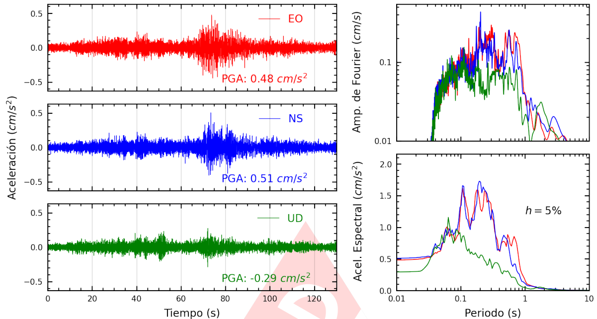
Figura A.7: Registros tiempo-historia, espectros de Fourier y de respuesta en las direcciones EO, NS y vertical de la estación SCCHO. Sismo de Chala, Caraveli - Arequipa del 2025-05-09, 22:34:08 (Hora local)
