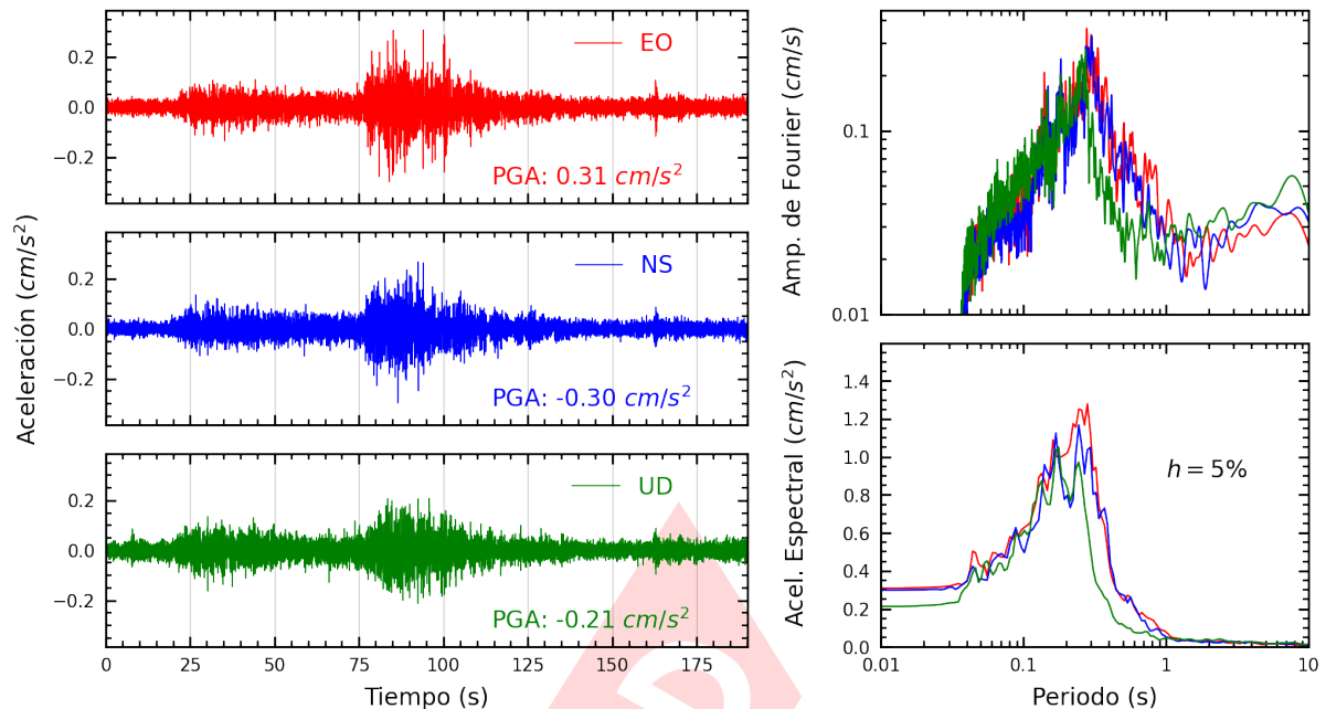
Figura A.9: Registros tiempo-historia, espectros de Fourier y de respuesta en las direcciones EO, NS y vertical de la estación SOVES. Sismo de Chala, Caraveli - Arequipa del 2025-05-09, 22:34:08 (Hora local)
