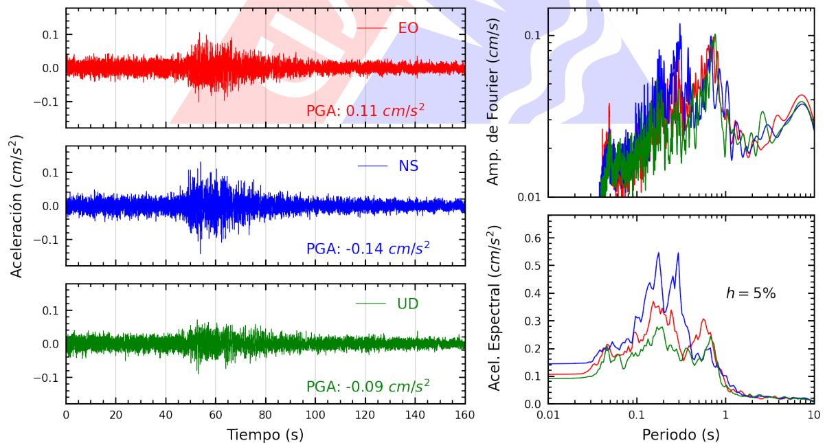
Figura A.22: Registros tiempo-historia, espectros de Fourier y de respuesta en las direcciones EO, NS y vertical de la estación SERVI. Sismo de Chala, Caraveli - Arequipa del 2025-05-09, 22:34:08 (Hora local)
