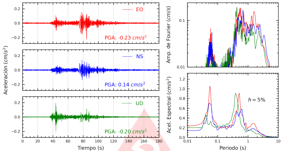
Figura A.13: Registros tiempo-historia, espectros de Fourier y de respuesta en las direcciones EO, NS y vertical de la estación UNMBA. Sismo de Chala, Caraveli - Arequipa del 2025-05-09, 22:34:08 (Hora local)
