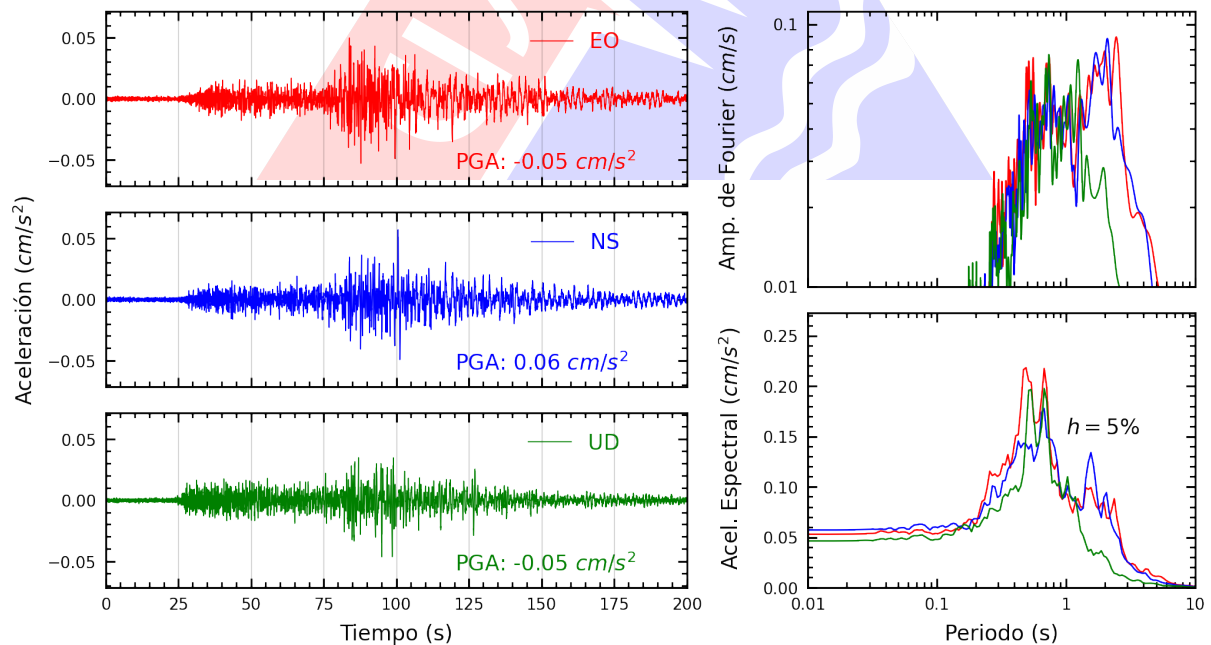
Figura A.30: Registros tiempo-historia, espectros de Fourier y de respuesta en las direcciones EO, NS y vertical de la estación UNCP. Sismo de Chala, Caraveli - Arequipa del 2025-05-09, 22:34:08 (Hora local)
