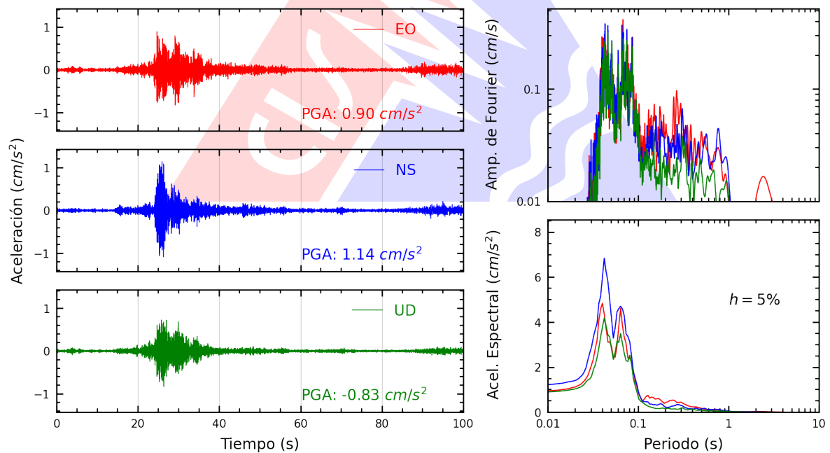
Figura A.2: Registros tiempo-historia, espectros de Fourier y de respuesta en las direcciones EO, NS y vertical de la estación PACHA. Sismo de Chala, Caraveli - Arequipa del 2025-05-09, 22:34:08 (Hora local)
