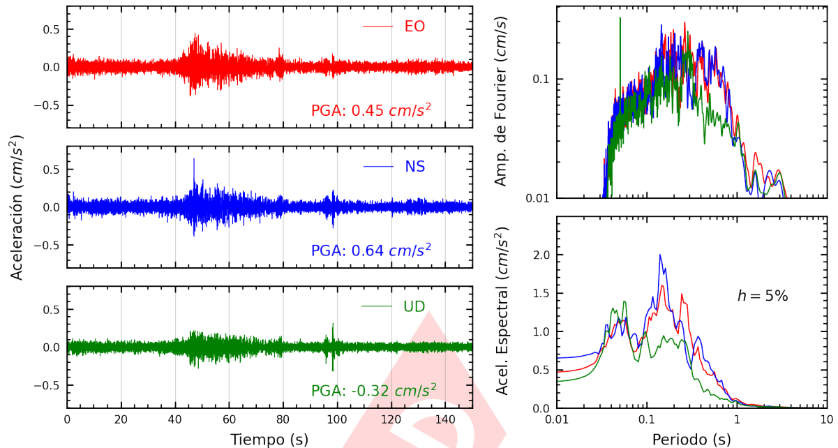
Figura A.5: Registros tiempo-historia, espectros de Fourier y de respuesta en las direcciones EO, NS y vertical de la estación PHER2. Sismo de Chala, Caraveli - Arequipa del 2025-05-09, 22:34:08 (Hora local)
