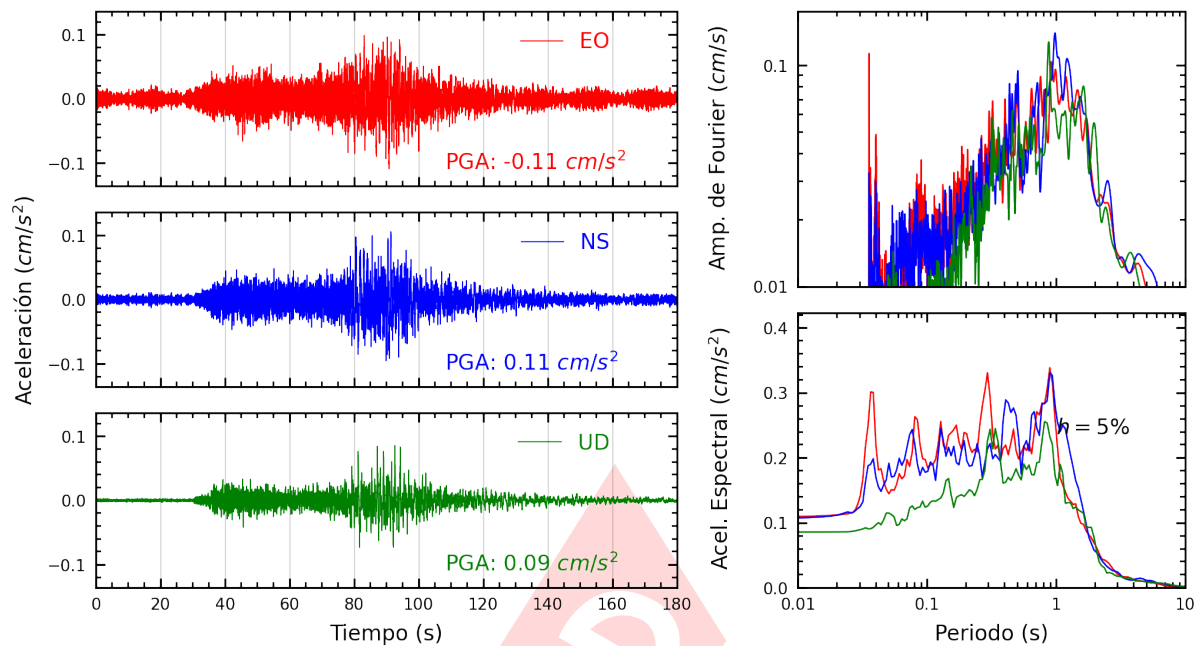
Figura A.27: Registros tiempo-historia, espectros de Fourier y de respuesta en las direcciones EO, NS y vertical de la estación UNAM. Sismo de Chala, Caraveli - Arequipa del 2025-05-09, 22:34:08 (Hora local)
