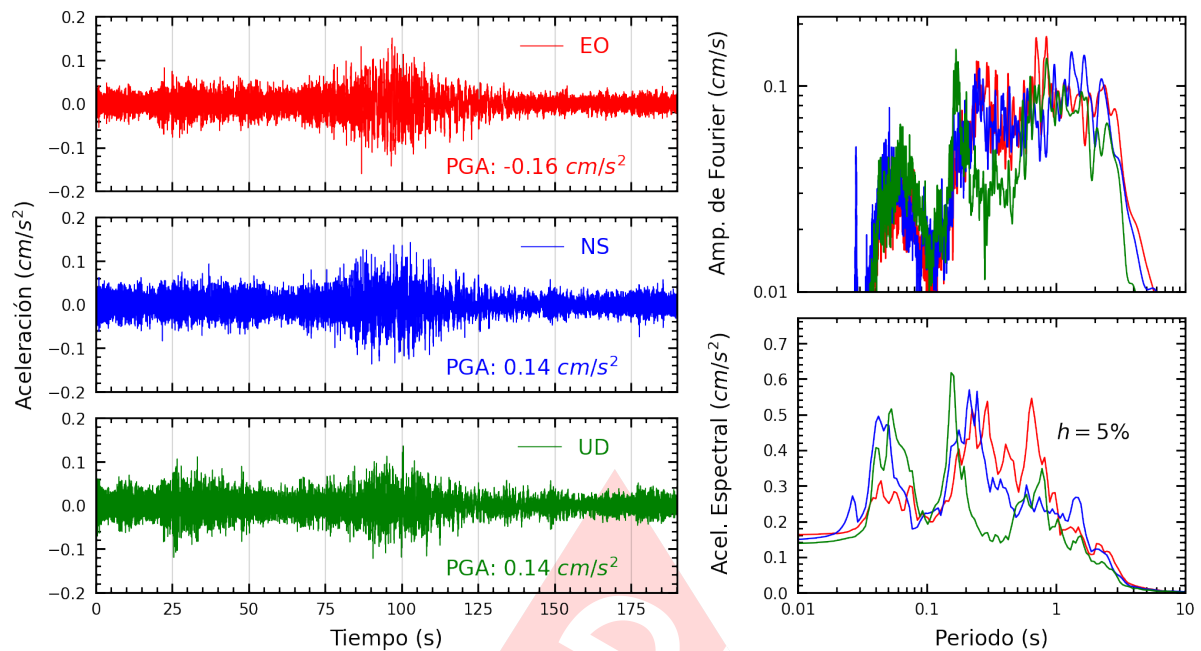
Figura A.21: Registros tiempo-historia, espectros de Fourier y de respuesta en las direcciones EO, NS y vertical de la estación UJBG4. Sismo de Chala, Caraveli - Arequipa del 2025-05-09, 22:34:08 (Hora local)
