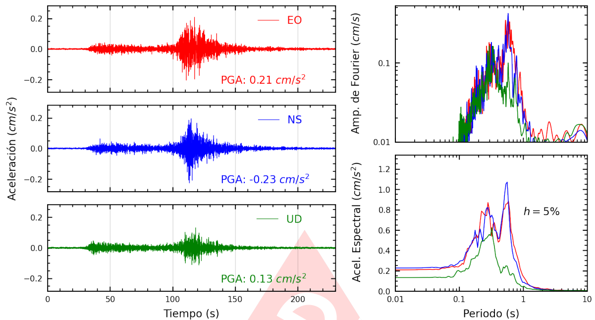
Figura A.15: Registros tiempo-historia, espectros de Fourier y de respuesta en las direcciones EO, NS y vertical de la estación CARAL. Sismo de Chala, Caraveli - Arequipa del 2025-05-09, 22:34:08 (Hora local)
