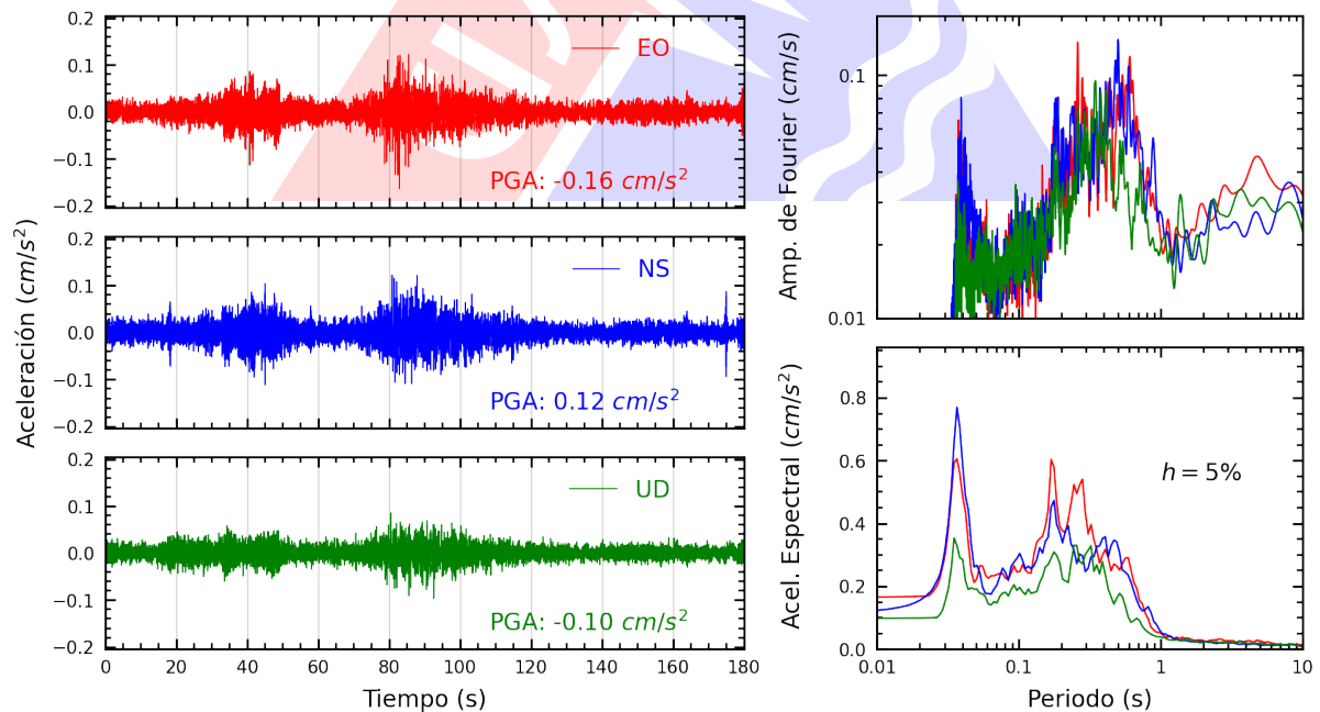
Figura A.20: Registros tiempo-historia, espectros de Fourier y de respuesta en las direcciones EO, NS y vertical de la estación COMAS. Sismo de Chala, Caraveli - Arequipa del 2025-05-09, 22:34:08 (Hora local)
