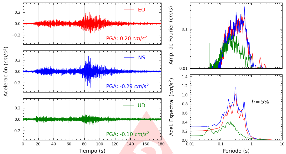
Figura A.11: Registros tiempo-historia, espectros de Fourier y de respuesta en las direcciones EO, NS y vertical de la estación VHAY2. Sismo de Chala, Caraveli - Arequipa del 2025-05-09, 22:34:08 (Hora local)
