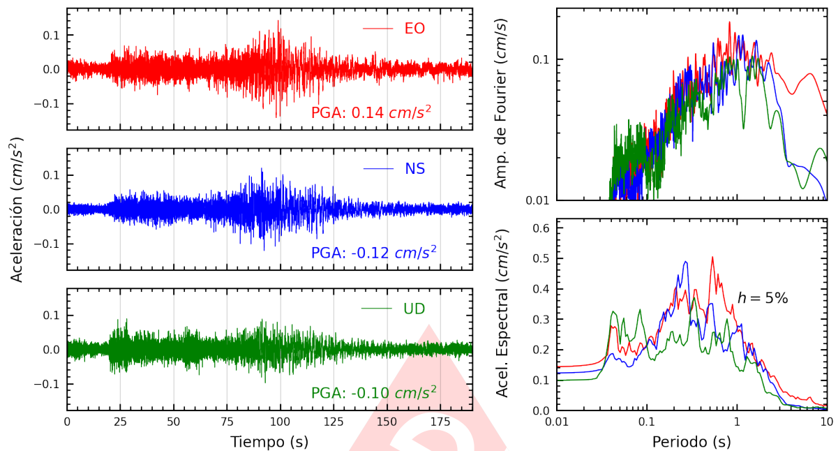
Figura A.23: Registros tiempo-historia, espectros de Fourier y de respuesta en las direcciones EO, NS y vertical de la estación UJBG3. Sismo de Chala, Caraveli - Arequipa del 2025-05-09, 22:34:08 (Hora local)
