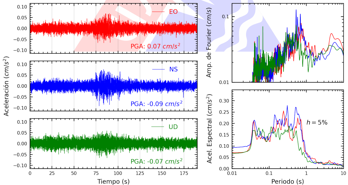
Figura A.28: Registros tiempo-historia, espectros de Fourier y de respuesta en las direcciones EO, NS y vertical de la estación BONDY. Sismo de Chala, Caraveli - Arequipa del 2025-05-09, 22:34:08 (Hora local)
