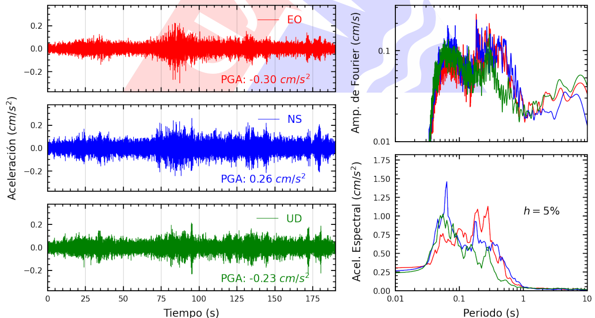
Figura A.10: Registros tiempo-historia, espectros de Fourier y de respuesta en las direcciones EO, NS y vertical de la estación SJLSC. Sismo de Chala, Caraveli - Arequipa del 2025-05-09, 22:34:08 (Hora local)
