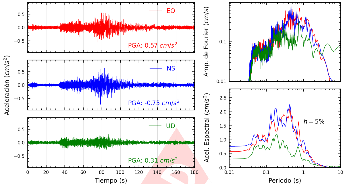
Figura A.3: Registros tiempo-historia, espectros de Fourier y de respuesta en las direcciones EO, NS y vertical de la estación SCARQ. Sismo de Chala, Caraveli - Arequipa del 2025-05-09, 22:34:08 (Hora local)
