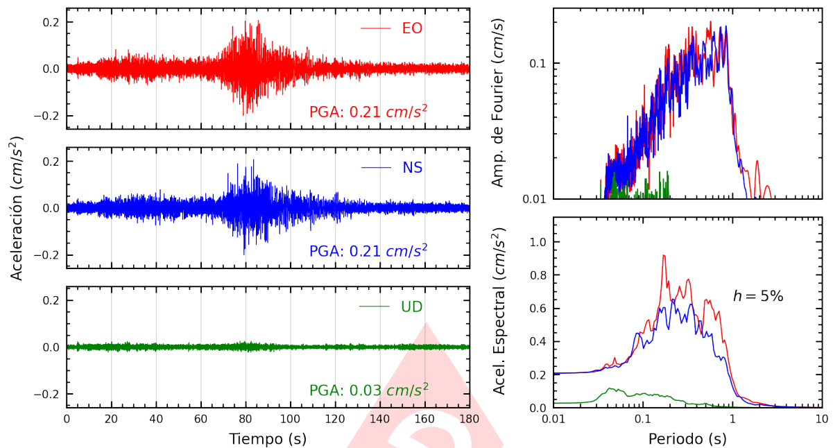
Figura A.17: Registros tiempo-historia, espectros de Fourier y de respuesta en las direcciones EO, NS y vertical de la estación UCVA2. Sismo de Chala, Caraveli - Arequipa del 2025-05-09, 22:34:08 (Hora local)
