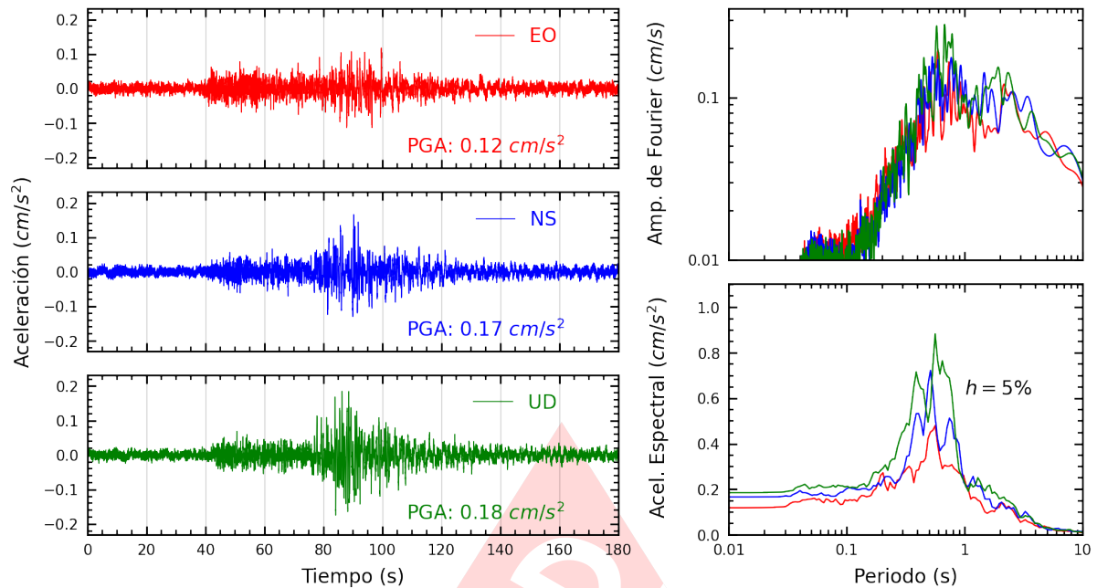
Figura A.19: Registros tiempo-historia, espectros de Fourier y de respuesta en las direcciones EO, NS y vertical de la estación UNSCH. Sismo de Chala, Caraveli - Arequipa del 2025-05-09, 22:34:08 (Hora local)
