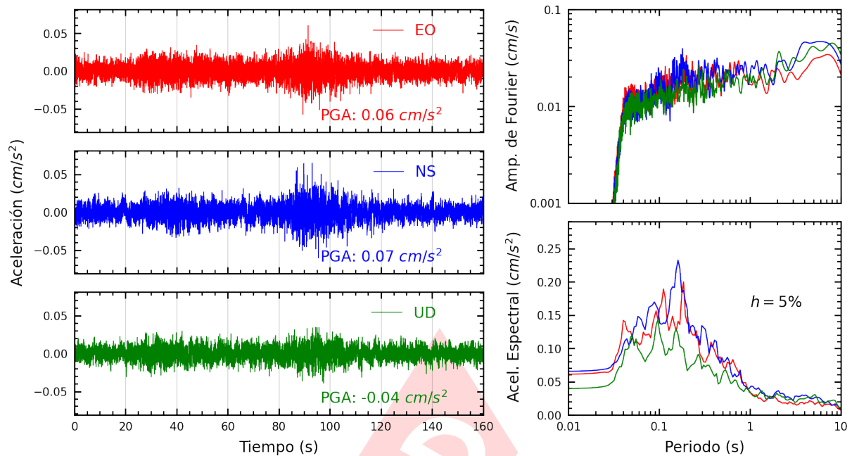
Figura A.29: Registros tiempo-historia, espectros de Fourier y de respuesta en las direcciones EO, NS y vertical de la estación UCSS. Sismo de Chala, Caraveli - Arequipa del 2025-05-09, 22:34:08 (Hora local)
