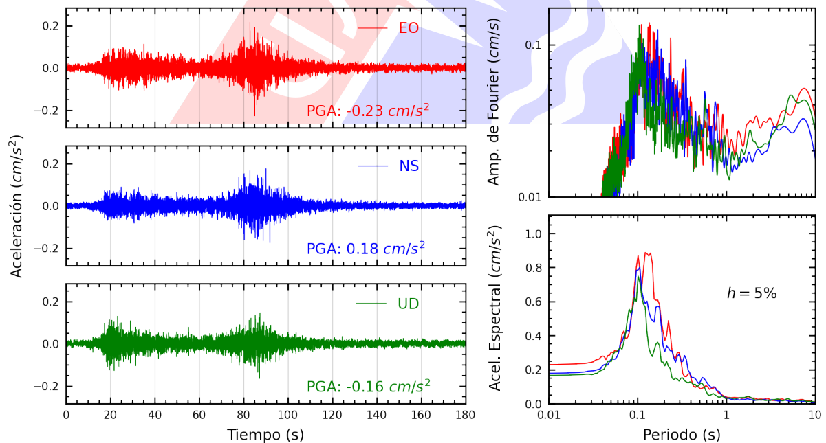
Figura A.14: Registros tiempo-historia, espectros de Fourier y de respuesta en las direcciones EO, NS y vertical de la estación AMORE. Sismo de Chala, Caraveli - Arequipa del 2025-05-09, 22:34:08 (Hora local)
