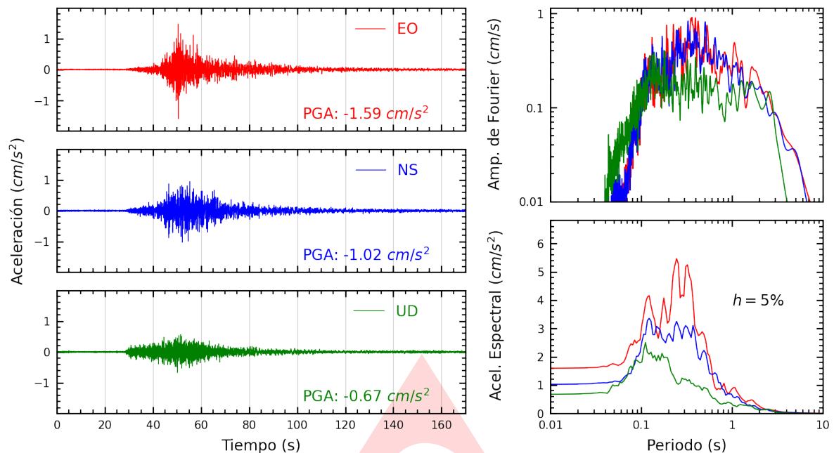
Figura A.1: Registros tiempo-historia, espectros de Fourier y de respuesta en las direcciones EO, NS y vertical de la estación UNP. Sismo de Mancora, Talara - Piura del 2025-05-10, 21:07:04 (Hora local)
