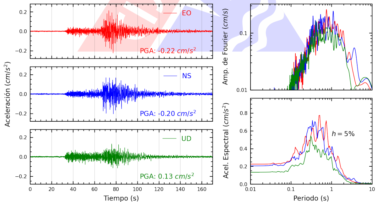
Figura A.6: Registros tiempo-historia, espectros de Fourier y de respuesta en las direcciones EO, NS y vertical de la estación UNJ. Sismo de Mancora, Talara - Piura del 2025-05-10, 21:07:04 (Hora local)
