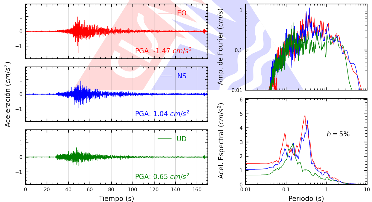
Figura A.2: Registros tiempo-historia, espectros de Fourier y de respuesta en las direcciones EO, NS y vertical de la estación UPAOP. Sismo de Mancora, Talara - Piura del 2025-05-10, 21:07:04 (Hora local)
