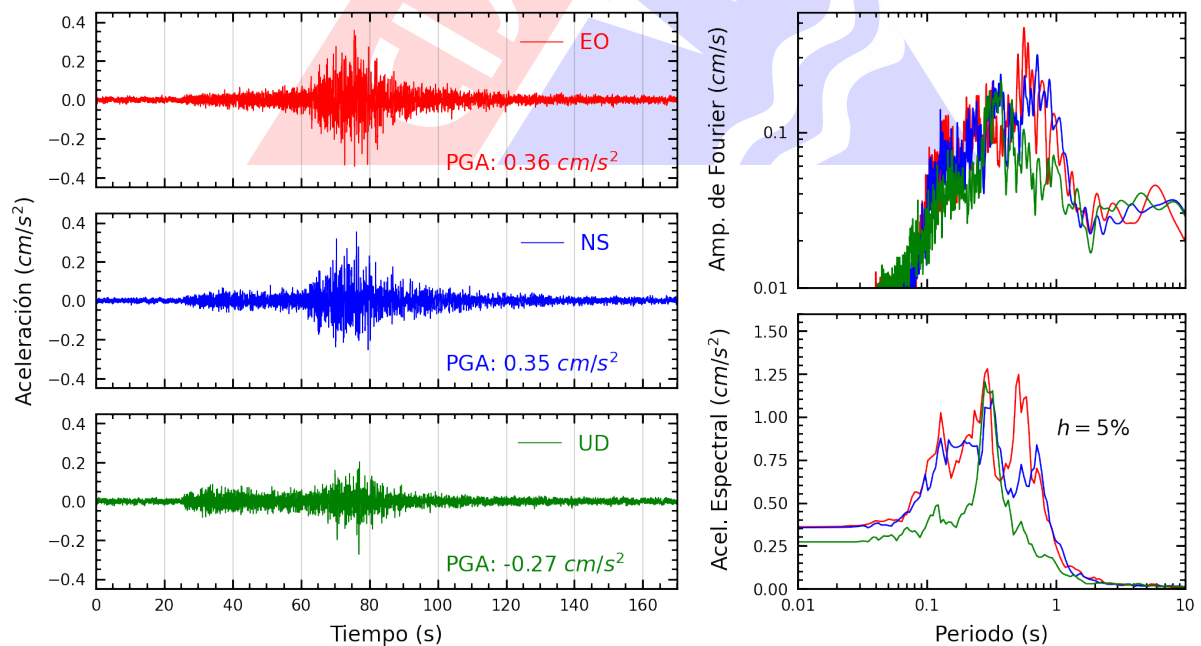
Figura A.4: Registros tiempo-historia, espectros de Fourier y de respuesta en las direcciones EO, NS y vertical de la estación UCVCH. Sismo de Mancora, Talara - Piura del 2025-05-10, 21:07:04 (Hora local)
