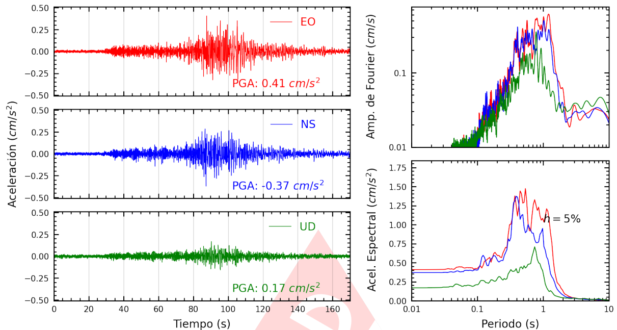
Figura A.3: Registros tiempo-historia, espectros de Fourier y de respuesta en las direcciones EO, NS y vertical de la estación UNTRM. Sismo de Mancora, Talara - Piura del 2025-05-10, 21:07:04 (Hora local)
