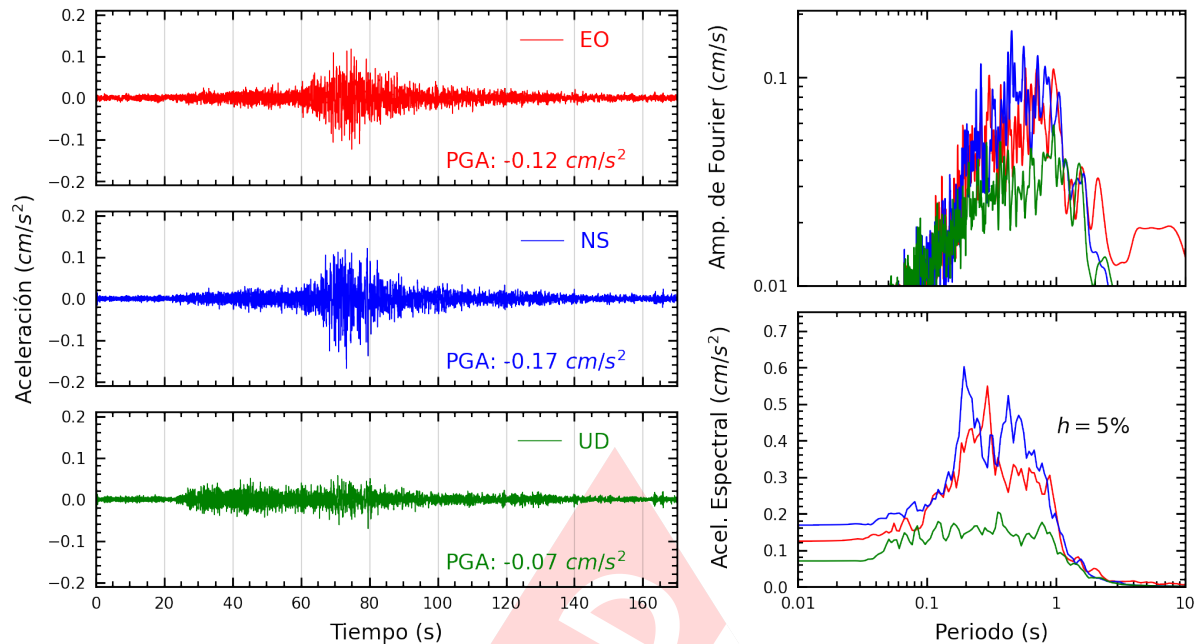
Figura A.7: Registros tiempo-historia, espectros de Fourier y de respuesta en las direcciones EO, NS y vertical de la estación SCCHL. Sismo de Mancora, Talara - Piura del 2025-05-10, 21:07:04 (Hora local)
