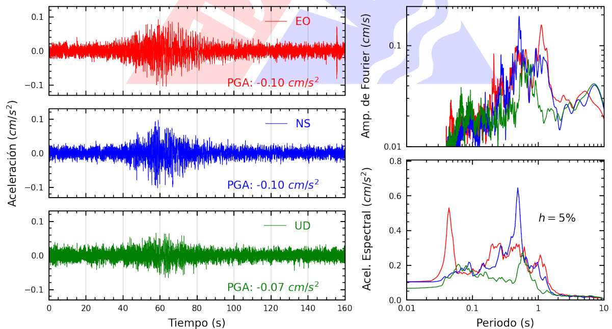
Figura A.8: Registros tiempo-historia, espectros de Fourier y de respuesta en las direcciones EO, NS y vertical de la estación UPAOT. Sismo de Mancora, Talara - Piura del 2025-05-10, 21:07:04 (Hora local)
