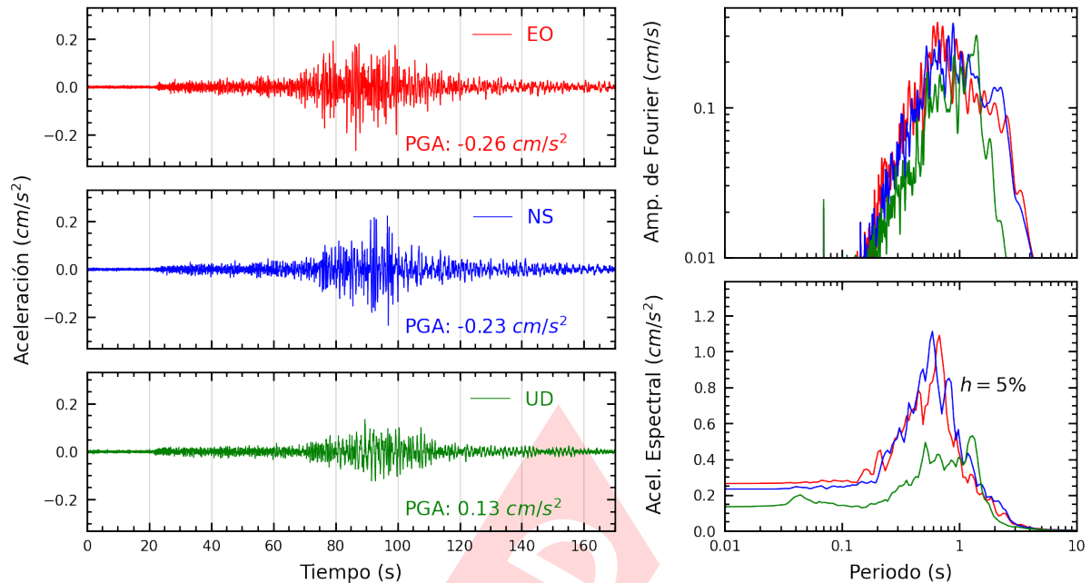
Figura A.5: Registros tiempo-historia, espectros de Fourier y de respuesta en las direcciones EO, NS y vertical de la estación UNC. Sismo de Mancora, Talara - Piura del 2025-05-10, 21:07:04 (Hora local)
