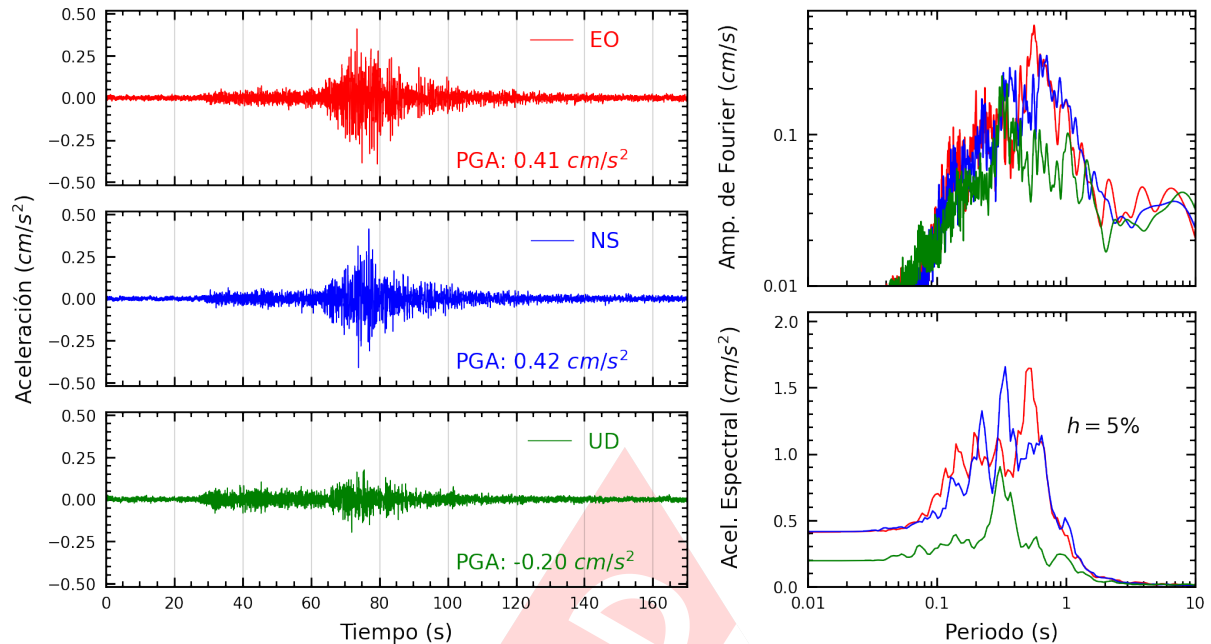
Figura A.5: Registros tiempo-historia, espectros de Fourier y de respuesta en las direcciones EO, NS y vertical de la estación UCVCH. Sismo de Mancora, Talara - Piura del 2025-05-11, 00:16:46 (Hora local)
