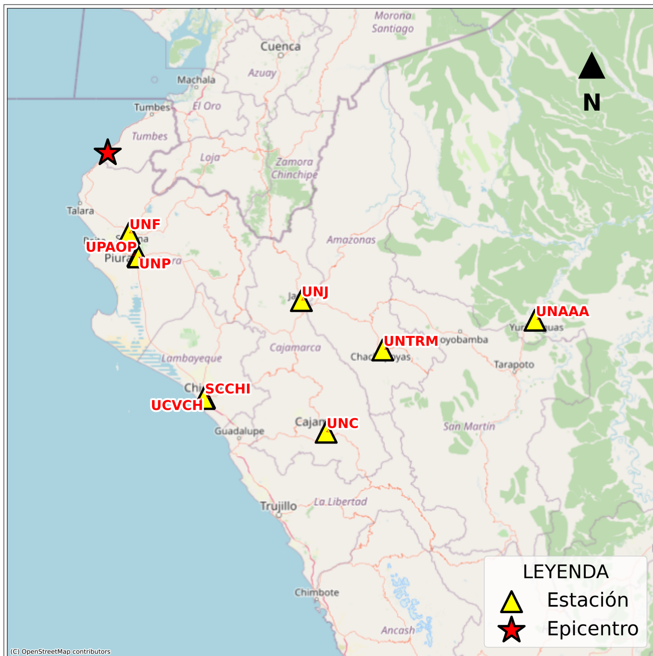
Figura 2: Mapa de ubicación de la(s) estación(es) acelerográfica(s) correspondiente(s) al Sismo de Mancora, Talara - Piura del 11 de mayo de 2025 a las 00:16:46 (hora local)
