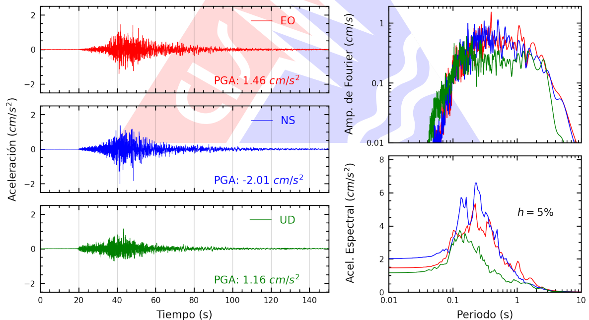
Figura A.2: Registros tiempo-historia, espectros de Fourier y de respuesta en las direcciones EO, NS y vertical de la estación UNP. Sismo de Mancora, Talara - Piura del 2025-05-11, 00:16:46 (Hora local)
