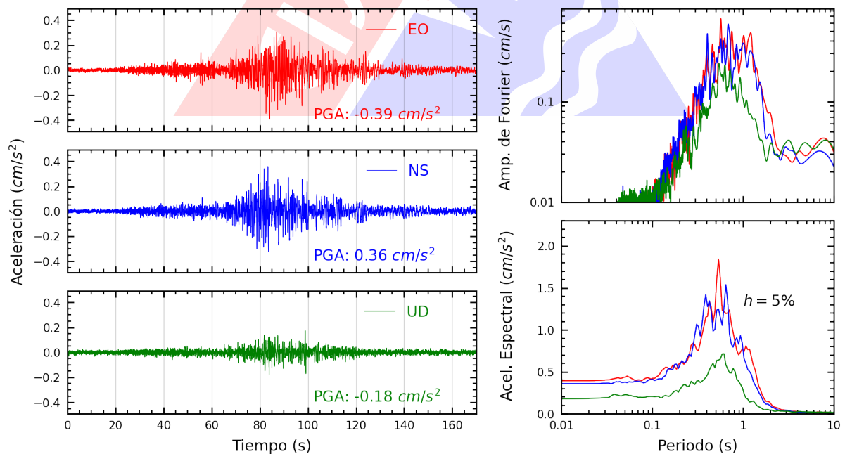
Figura A.6: Registros tiempo-historia, espectros de Fourier y de respuesta en las direcciones EO, NS y vertical de la estación UNTRM. Sismo de Mancora, Talara - Piura del 2025-05-11, 00:16:46 (Hora local)
