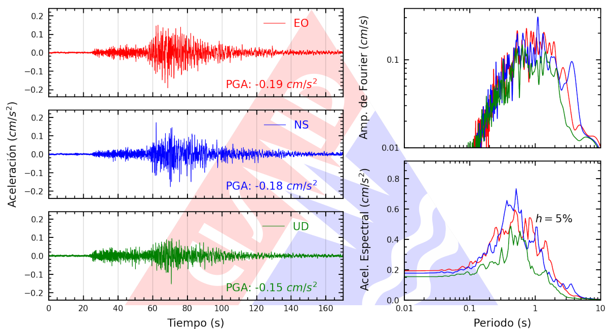
Figura A.9: Registros tiempo-historia, espectros de Fourier y de respuesta en las direcciones EO, NS y vertical de la estación UNJ. Sismo de Mancora, Talara - Piura del 2025-05-11, 00:16:46 (Hora local)
