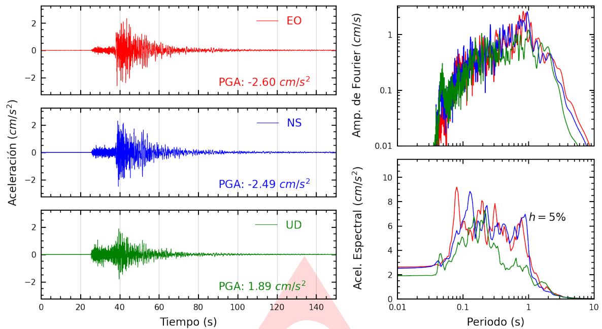
Figura A.1: Registros tiempo-historia, espectros de Fourier y de respuesta en las direcciones EO, NS y vertical de la estación UNF. Sismo de Mancora, Talara - Piura del 2025-05-11, 00:16:46 (Hora local)
