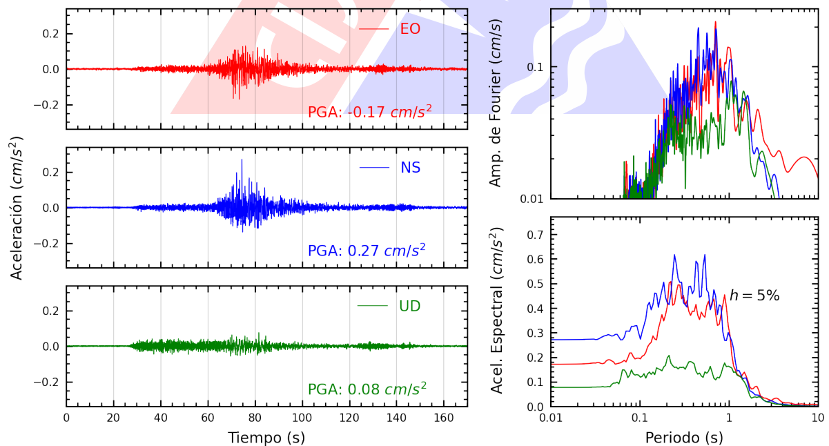
Figura A.8: Registros tiempo-historia, espectros de Fourier y de respuesta en las direcciones EO, NS y vertical de la estación SCCHL. Sismo de Mancora, Talara - Piura del 2025-05-11, 00:16:46 (Hora local)
