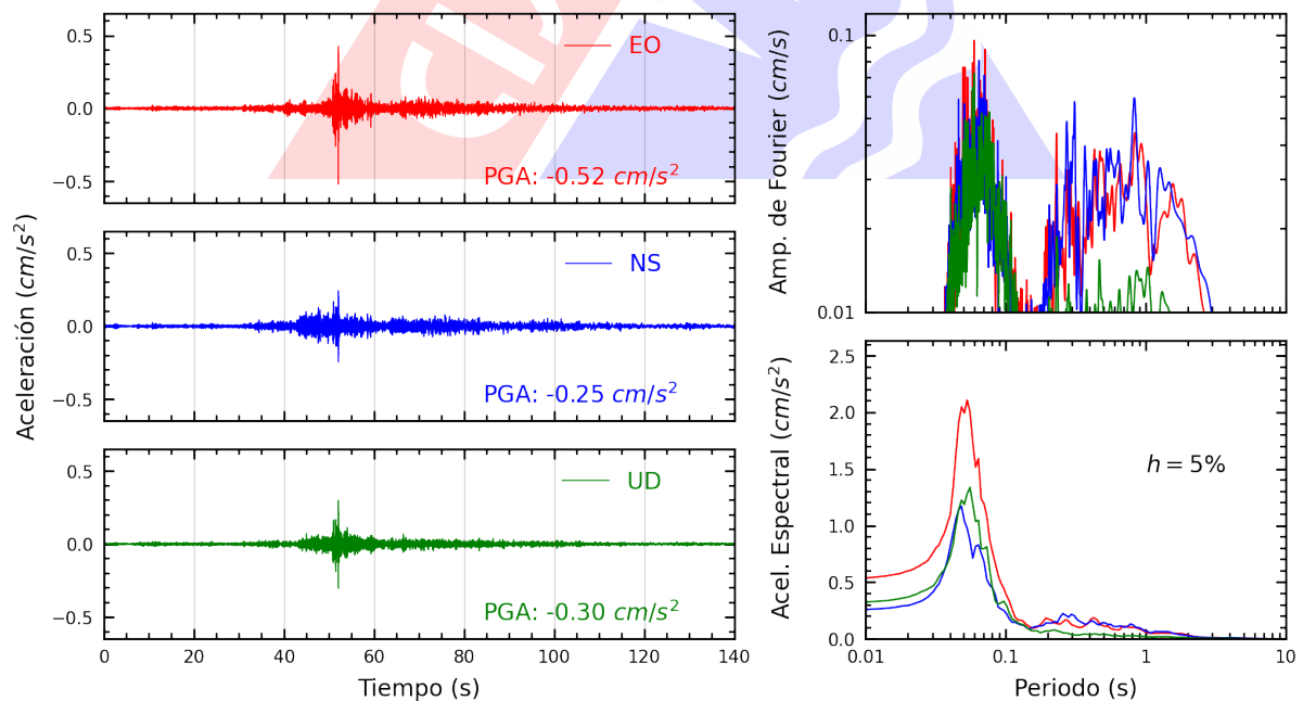
Figura A.4: Registros tiempo-historia, espectros de Fourier y de respuesta en las direcciones EO, NS y vertical de la estación UNAAA. Sismo de Mancora, Talara - Piura del 2025-05-11, 00:16:46 (Hora local)
