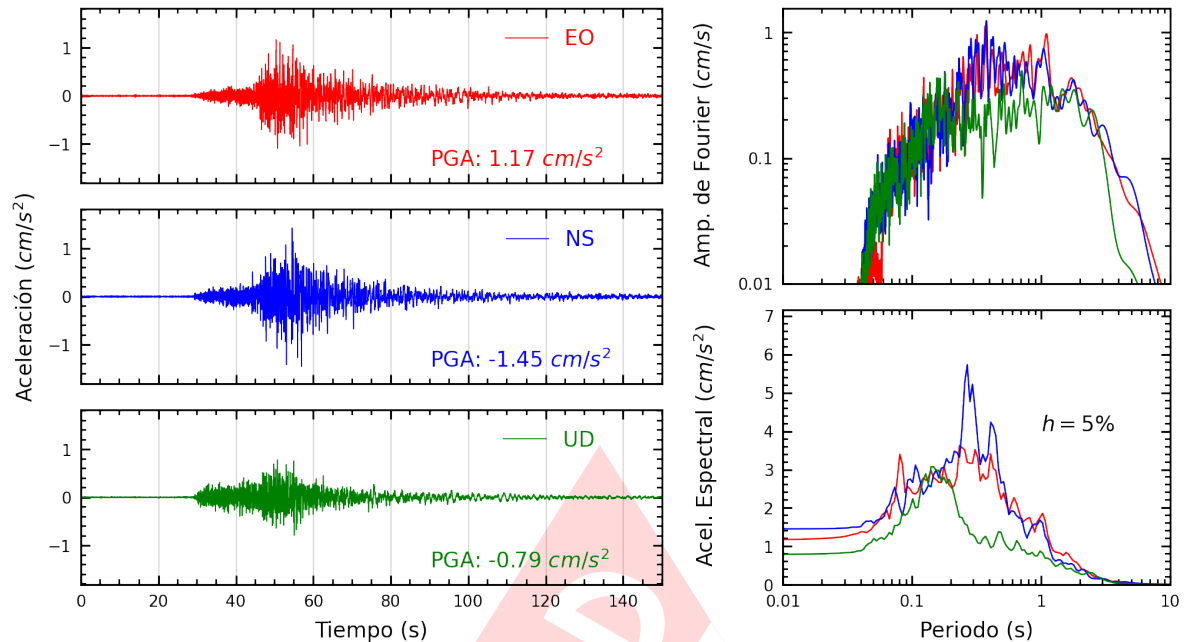
Figura A.3: Registros tiempo-historia, espectros de Fourier y de respuesta en las direcciones EO, NS y vertical de la estación UPAOP. Sismo de Mancora, Talara - Piura del 2025-05-11, 00:16:46 (Hora local)
