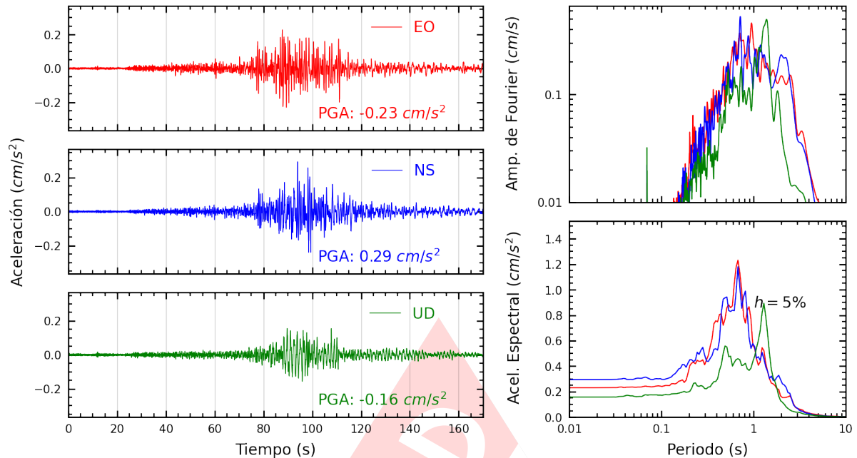
Figura A.7: Registros tiempo-historia, espectros de Fourier y de respuesta en las direcciones EO, NS y vertical de la estación UNC. Sismo de Mancora, Talara - Piura del 2025-05-11, 00:16:46 (Hora local)
