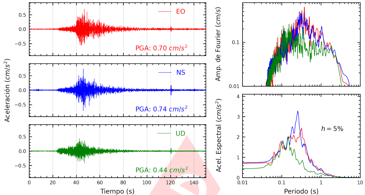
Figura A.3: Registros tiempo-historia, espectros de Fourier y de respuesta en las direcciones EO, NS y vertical de la estación UPAOP. Sismo de Mancora, Talara - Piura del 2025-05-11, 00:42:42 (Hora local)
