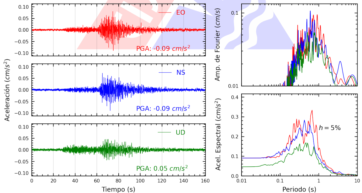
Figura A.8: Registros tiempo-historia, espectros de Fourier y de respuesta en las direcciones EO, NS y vertical de la estación UNJ. Sismo de Mancora, Talara - Piura del 2025-05-11, 00:42:42 (Hora local)
