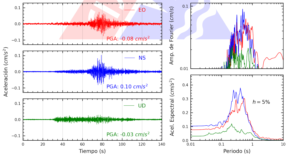
Figura A.6: Registros tiempo-historia, espectros de Fourier y de respuesta en las direcciones EO, NS y vertical de la estación SCCHI. Sismo de Mancora, Talara - Piura del 2025-05-11, 00:42:42 (Hora local)
