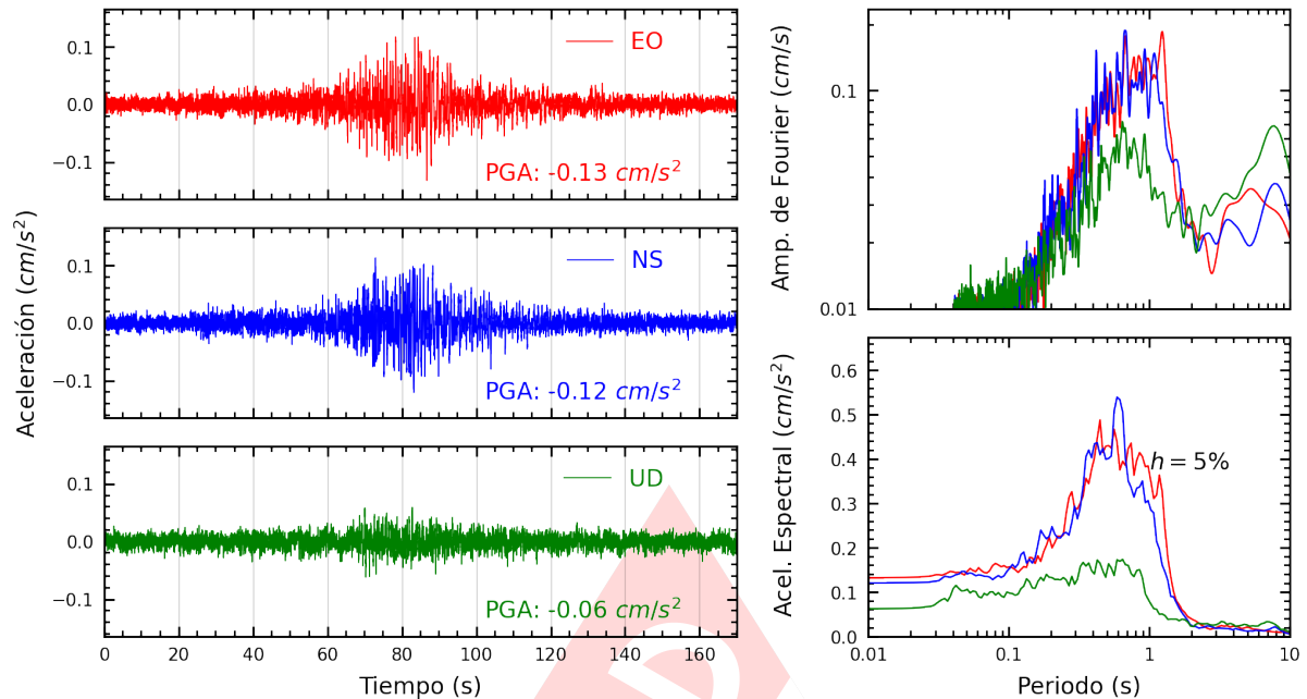
Figura A.5: Registros tiempo-historia, espectros de Fourier y de respuesta en las direcciones EO, NS y vertical de la estación UNTRM. Sismo de Mancora, Talara - Piura del 2025-05-11, 00:42:42 (Hora local)
