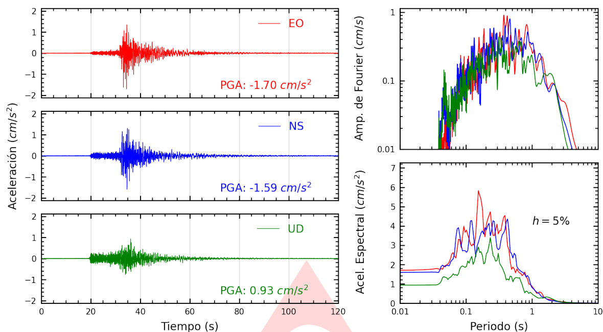
Figura A.1: Registros tiempo-historia, espectros de Fourier y de respuesta en las direcciones EO, NS y vertical de la estación UNF. Sismo de Mancora, Talara - Piura del 2025-05-11, 00:42:42 (Hora local)
