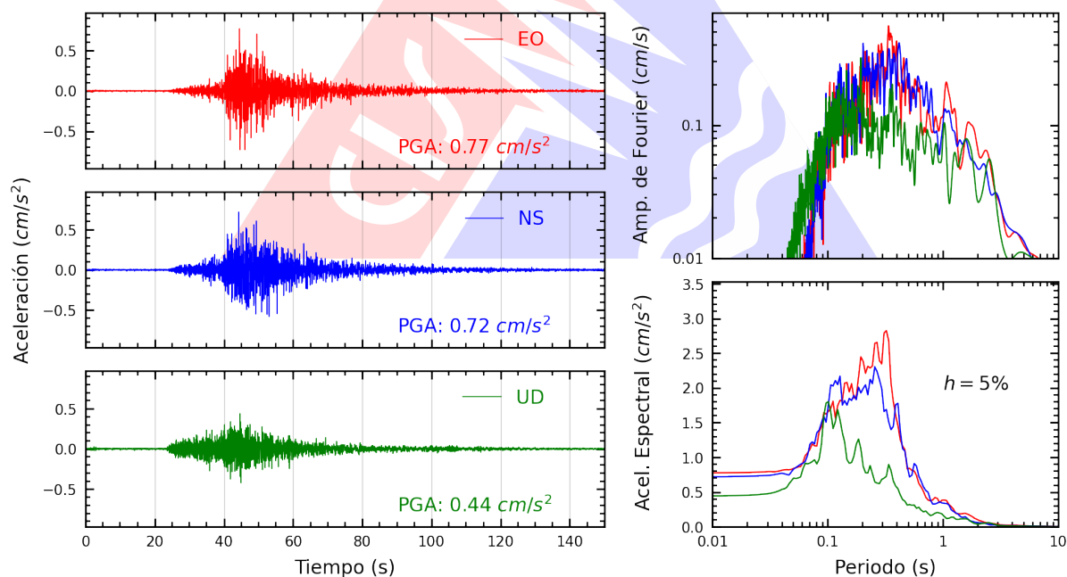
Figura A.2: Registros tiempo-historia, espectros de Fourier y de respuesta en las direcciones EO, NS y vertical de la estación UNP. Sismo de Mancora, Talara - Piura del 2025-05-11, 00:42:42 (Hora local)
