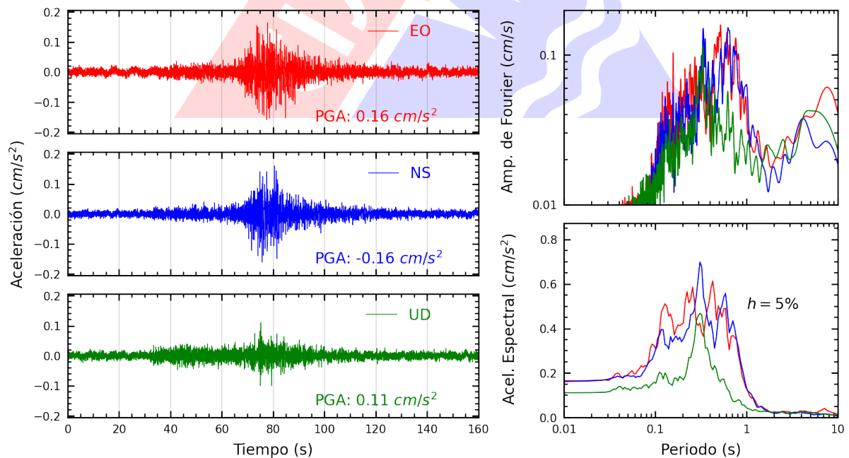
Figura A.4: Registros tiempo-historia, espectros de Fourier y de respuesta en las direcciones EO, NS y vertical de la estación UCVCH. Sismo de Mancora, Talara - Piura del 2025-05-11, 00:42:42 (Hora local)
