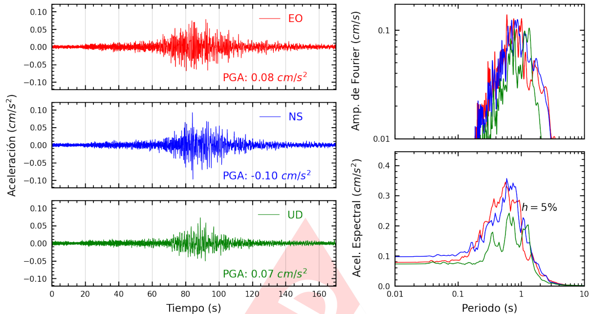
Figura A.7: Registros tiempo-historia, espectros de Fourier y de respuesta en las direcciones EO, NS y vertical de la estación UNC. Sismo de Mancora, Talara - Piura del 2025-05-11, 00:42:42 (Hora local)
