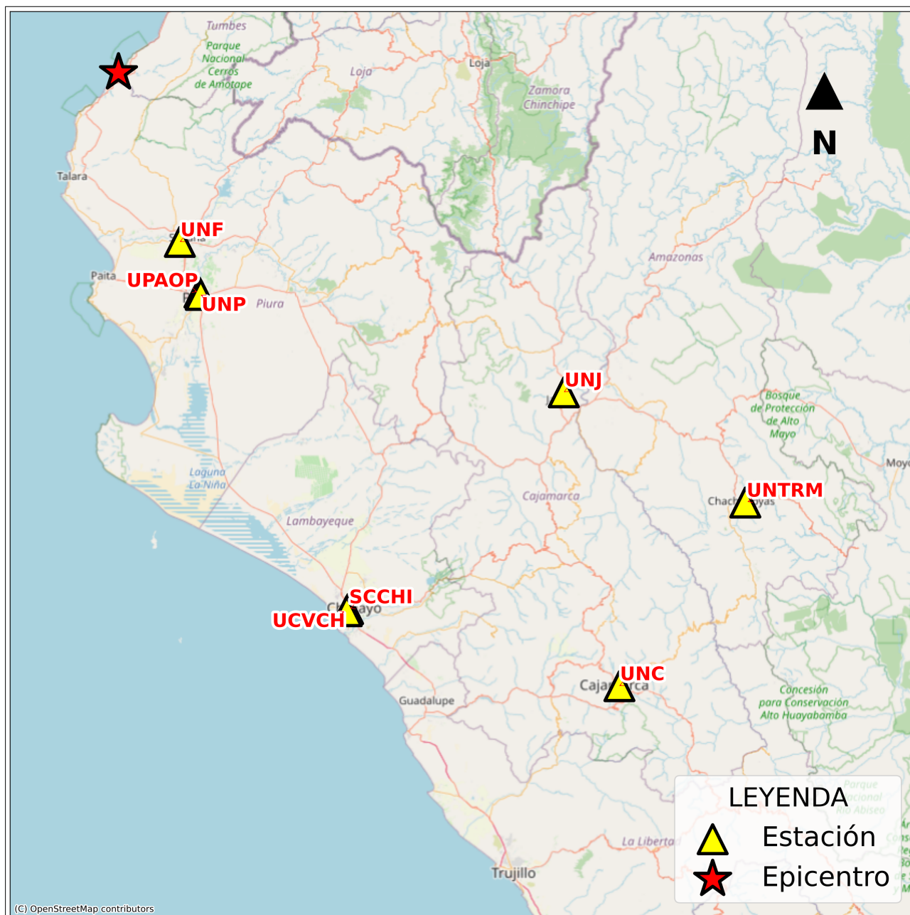
Figura 2: Mapa de ubicación de la(s) estación(es) acelerográfica(s) correspondiente(s) al Sismo de Mancora, Talara - Piura del 11 de mayo de 2025 a las 00:42:42 (hora local)
