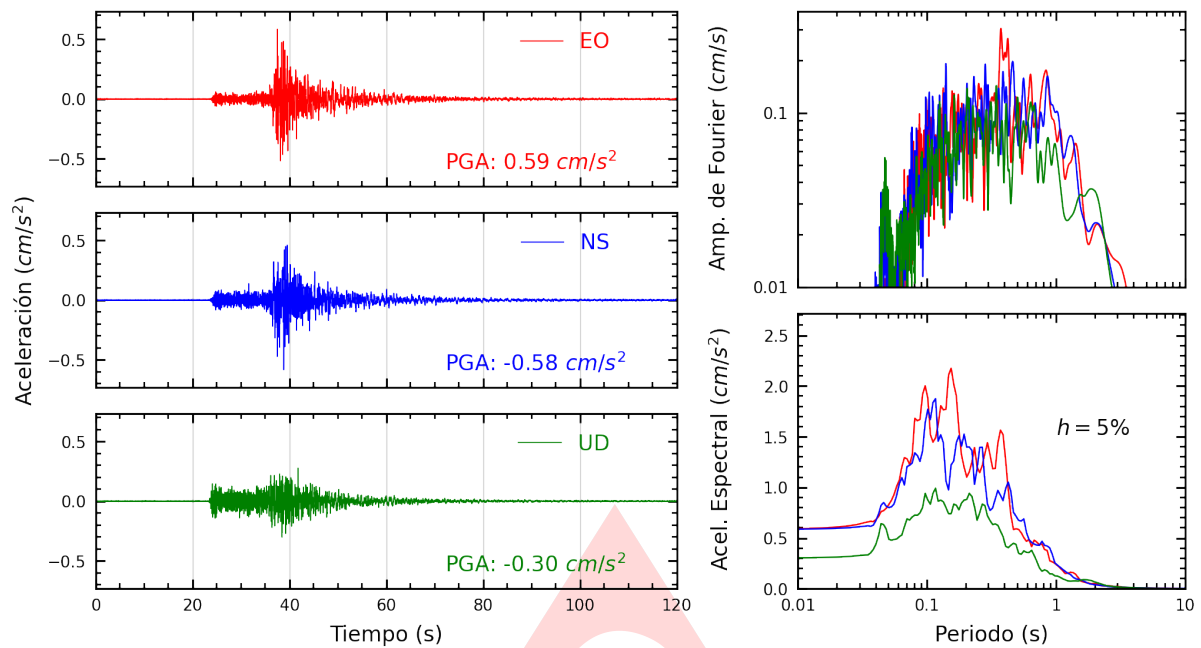
Figura A.1: Registros tiempo-historia, espectros de Fourier y de respuesta en las direcciones EO, NS y vertical de la estación UNF. Sismo de Mancora, Talara - Piura del 2025-05-11, 00:53:45 (Hora local)
