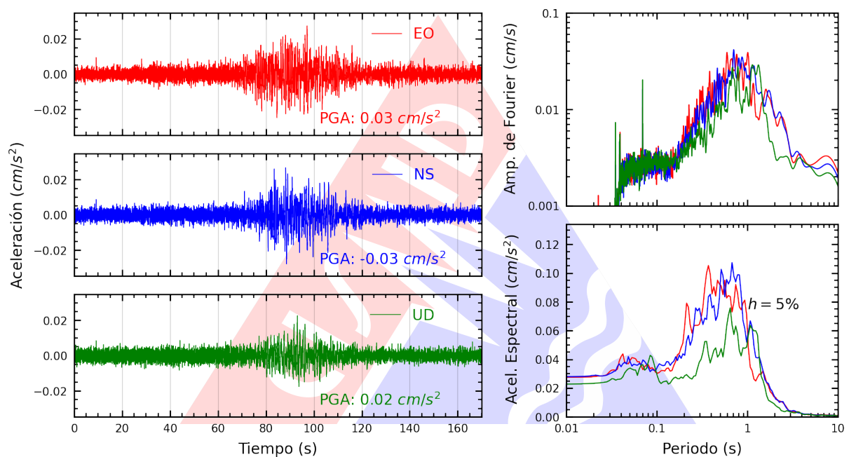
Figura A.7: Registros tiempo-historia, espectros de Fourier y de respuesta en las direcciones EO, NS y vertical de la estación UNC. Sismo de Mancora, Talara - Piura del 2025-05-11, 00:53:45 (Hora local)
