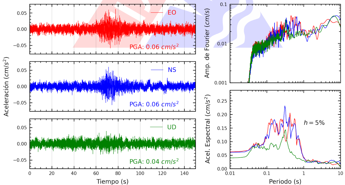
Figura A.4: Registros tiempo-historia, espectros de Fourier y de respuesta en las direcciones EO, NS y vertical de la estación UCVCH. Sismo de Mancora, Talara - Piura del 2025-05-11, 00:53:45 (Hora local)
