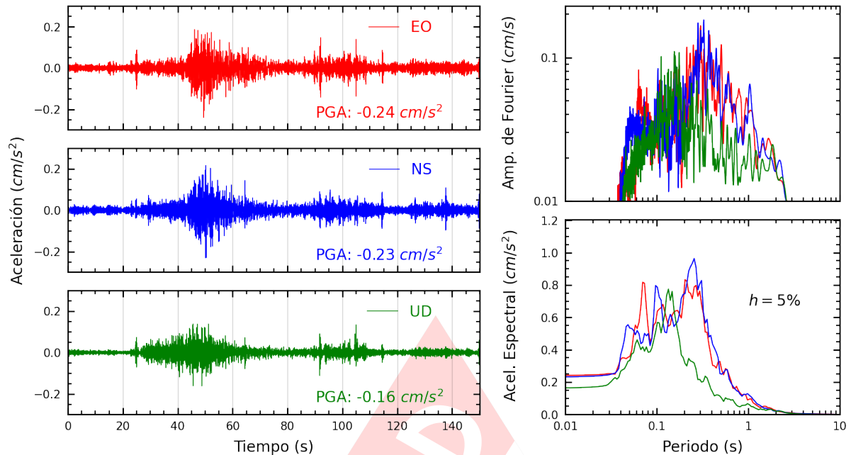
Figura A.3: Registros tiempo-historia, espectros de Fourier y de respuesta en las direcciones EO, NS y vertical de la estación UPAOP. Sismo de Mancora, Talara - Piura del 2025-05-11, 00:53:45 (Hora local)
