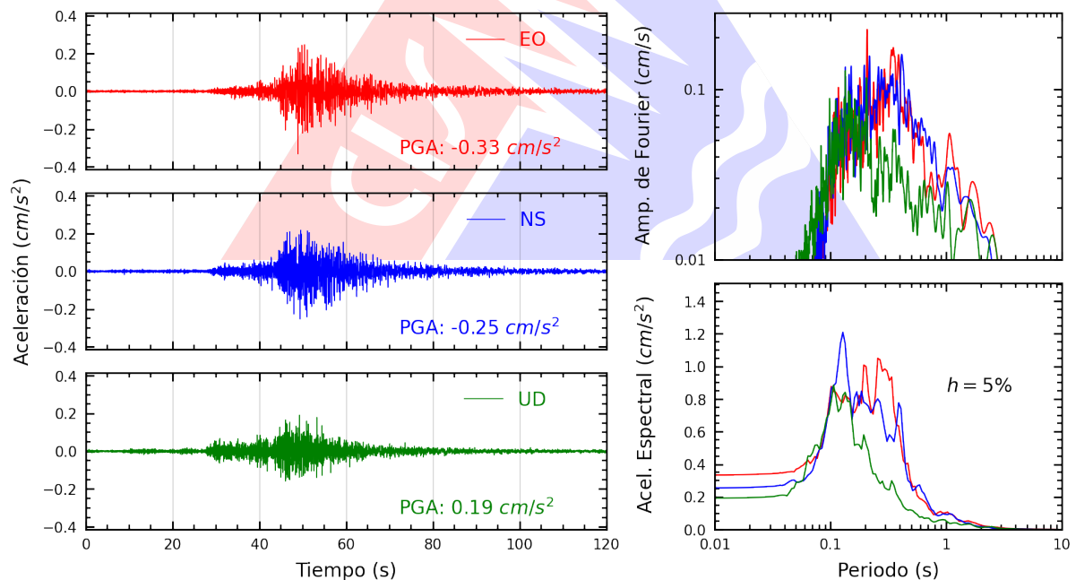
Figura A.2: Registros tiempo-historia, espectros de Fourier y de respuesta en las direcciones EO, NS y vertical de la estación UNP. Sismo de Mancora, Talara - Piura del 2025-05-11, 00:53:45 (Hora local)
