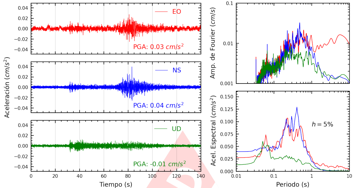
Figura A.5: Registros tiempo-historia, espectros de Fourier y de respuesta en las direcciones EO, NS y vertical de la estación SCCHI. Sismo de Mancora, Talara - Piura del 2025-05-11, 00:53:45 (Hora local)
