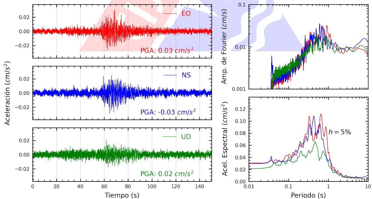
Figura A.6: Registros tiempo-historia, espectros de Fourier y de respuesta en las direcciones EO, NS y vertical de la estación UNJ. Sismo de Mancora, Talara - Piura del 2025-05-11, 00:53:45 (Hora local)
