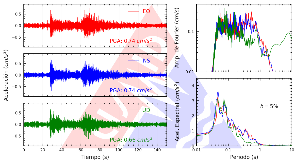
Figura A.5: Registros tiempo-historia, espectros de Fourier y de respuesta en las direcciones EO, NS y vertical de la estación SCARQ. Sismo de Calana, Tacna - Tacna del 2025-05-12, 09:57:51 (Hora local)
