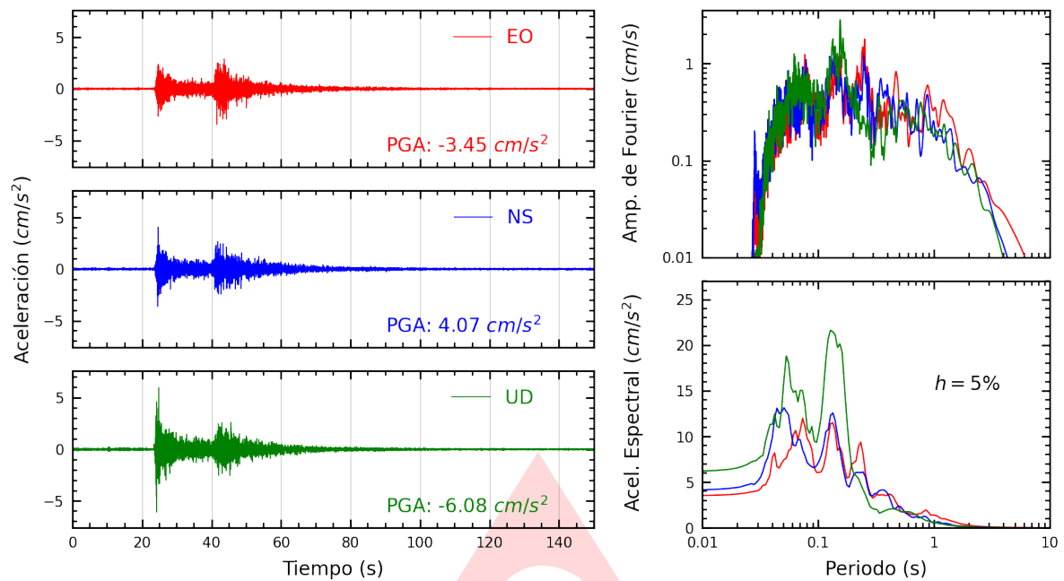
Figura A.1: Registros tiempo-historia, espectros de Fourier y de respuesta en las direcciones EO, NS y vertical de la estación UJBG4. Sismo de Calana, Tacna - Tacna del 2025-05-12, 09:57:51 (Hora local)
