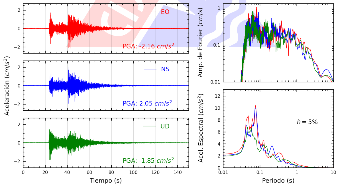
Figura A.4: Registros tiempo-historia, espectros de Fourier y de respuesta en las direcciones EO, NS y vertical de la estación CREY. Sismo de Calana, Tacna - Tacna del 2025-05-12, 09:57:51 (Hora local)
