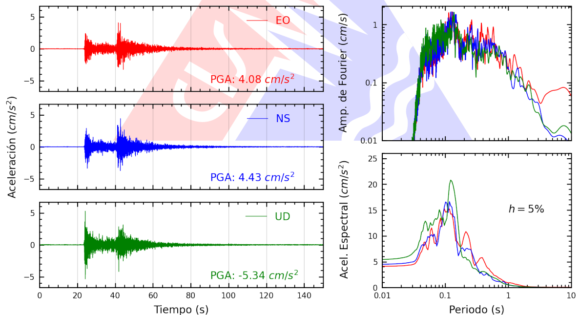
Figura A.2: Registros tiempo-historia, espectros de Fourier y de respuesta en las direcciones EO, NS y vertical de la estación UJBG3. Sismo de Calana, Tacna - Tacna del 2025-05-12, 09:57:51 (Hora local)
