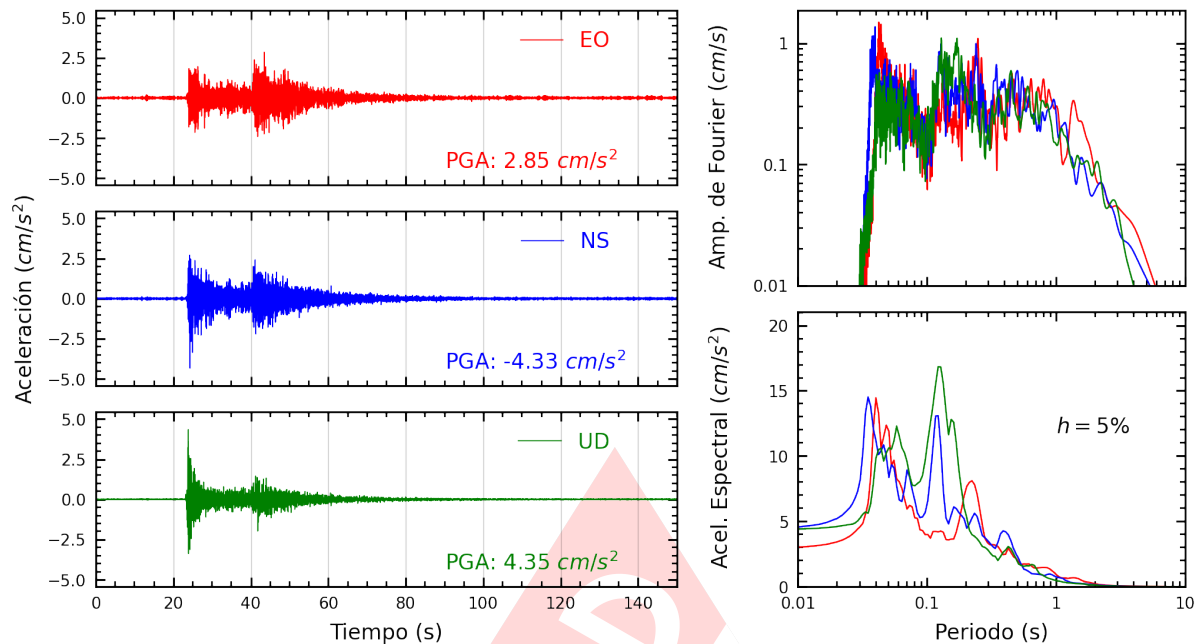
Figura A.3: Registros tiempo-historia, espectros de Fourier y de respuesta en las direcciones EO, NS y vertical de la estación UPTAC. Sismo de Calana, Tacna - Tacna del 2025-05-12, 09:57:51 (Hora local)
