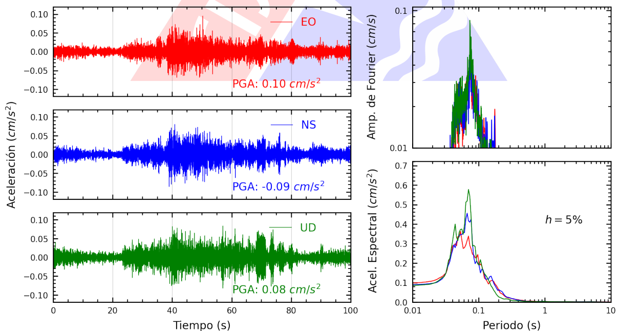
Figura A.40: Registros tiempo-historia, espectros de Fourier y de respuesta en las direcciones EO, NS y vertical de la estación ASIA. Sismo de Ancon, Lima - Lima del 2025-05-12, 11:53:20 (Hora local)
