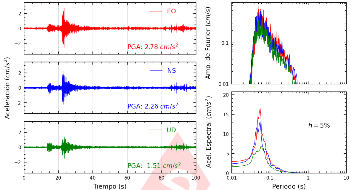
Figura A.3: Registros tiempo-historia, espectros de Fourier y de respuesta en las direcciones EO, NS y vertical de la estación UNTEL. Sismo de Ancon, Lima - Lima del 2025-05-12, 11:53:20 (Hora local)
