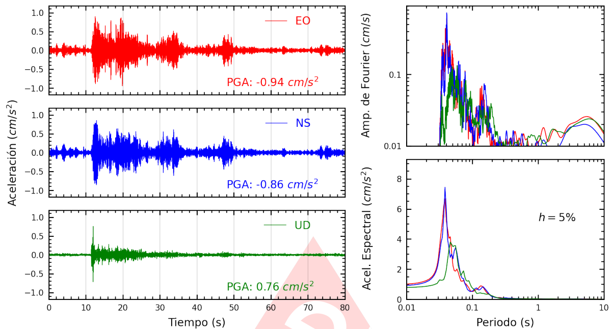
Figura A.23: Registros tiempo-historia, espectros de Fourier y de respuesta en las direcciones EO, NS y vertical de la estación DHNPE. Sismo de Ancon, Lima - Lima del 2025-05-12, 11:53:20 (Hora local)
