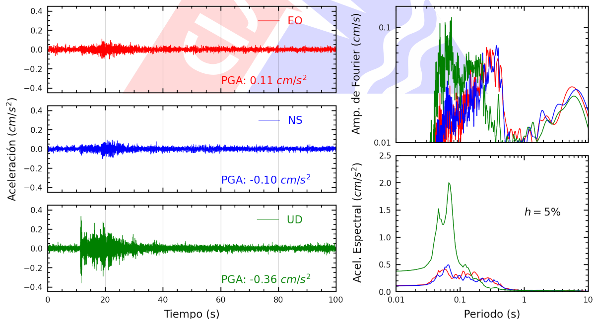
Figura A.34: Registros tiempo-historia, espectros de Fourier y de respuesta en las direcciones EO, NS y vertical de la estación ACAPU. Sismo de Ancon, Lima - Lima del 2025-05-12, 11:53:20 (Hora local)
