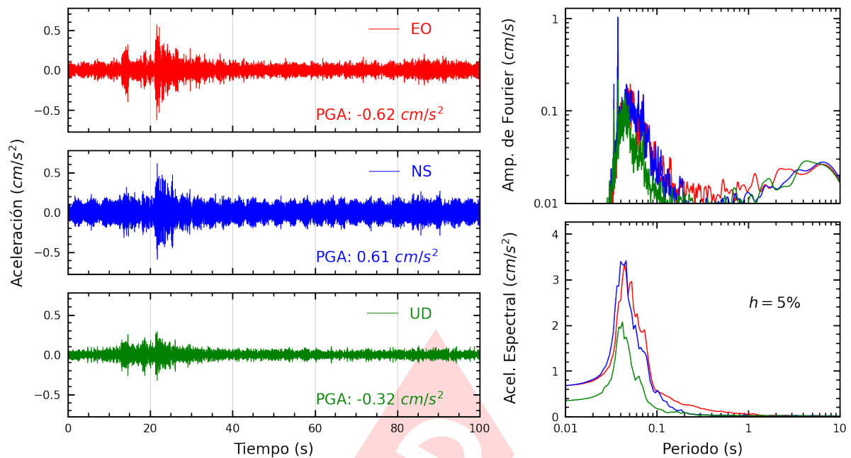
Figura A.29: Registros tiempo-historia, espectros de Fourier y de respuesta en las direcciones EO, NS y vertical de la estación UPCVI. Sismo de Ancon, Lima - Lima del 2025-05-12, 11:53:20 (Hora local)
