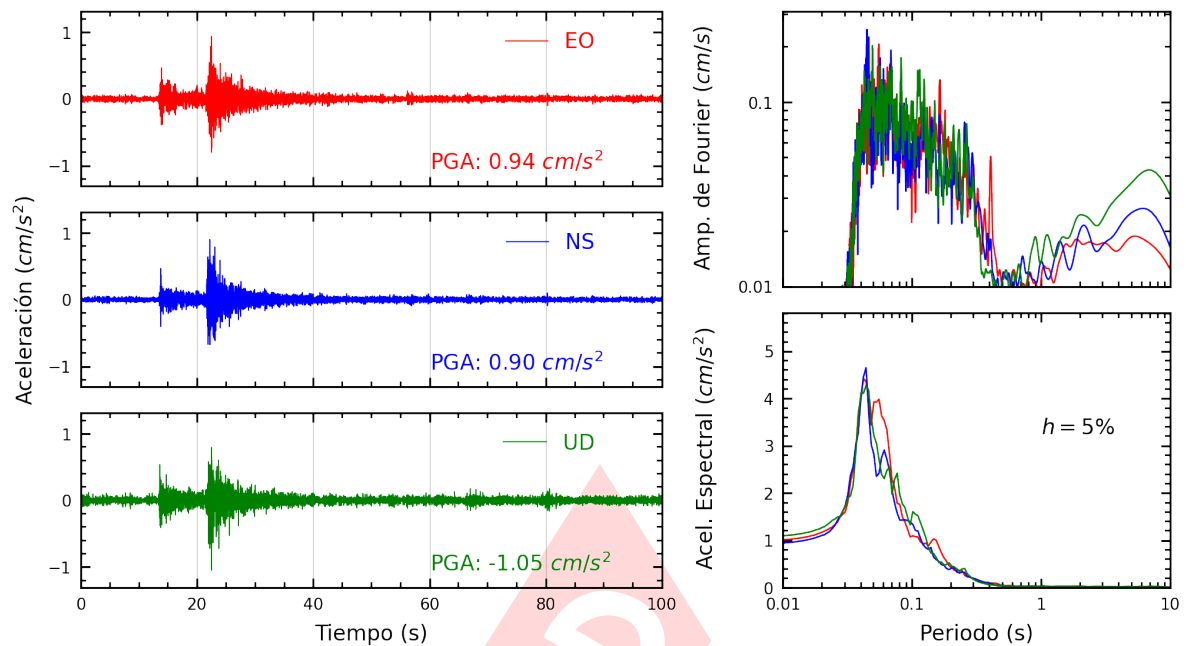
Figura A.21: Registros tiempo-historia, espectros de Fourier y de respuesta en las direcciones EO, NS y vertical de la estación SOVES. Sismo de Ancon, Lima - Lima del 2025-05-12, 11:53:20 (Hora local)
