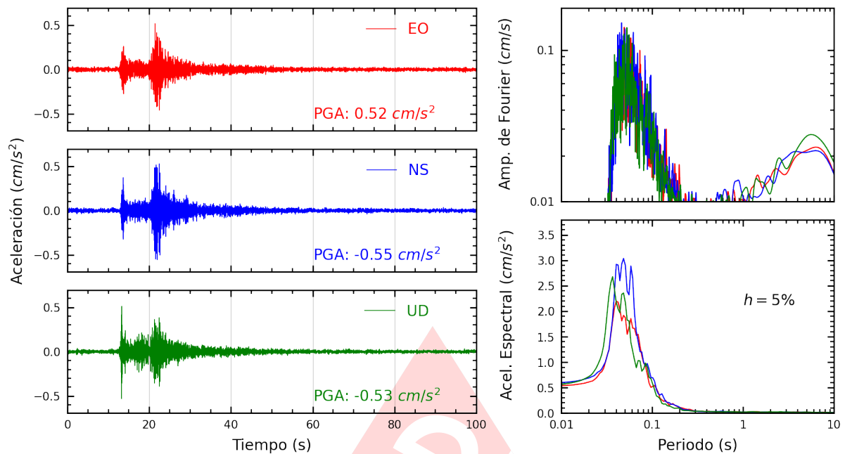
Figura A.31: Registros tiempo-historia, espectros de Fourier y de respuesta en las direcciones EO, NS y vertical de la estación SERVI. Sismo de Ancon, Lima - Lima del 2025-05-12, 11:53:20 (Hora local)
