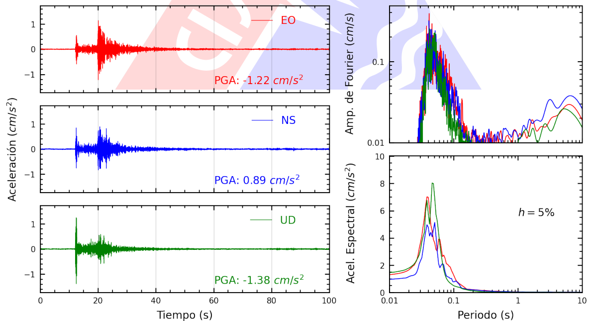
Figura A.14: Registros tiempo-historia, espectros de Fourier y de respuesta en las direcciones EO, NS y vertical de la estación SJLCE. Sismo de Ancon, Lima - Lima del 2025-05-12, 11:53:20 (Hora local)
