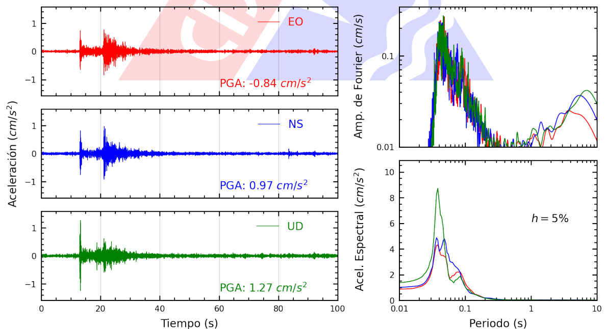
Figura A.16: Registros tiempo-historia, espectros de Fourier y de respuesta en las direcciones EO, NS y vertical de la estación USMP. Sismo de Ancon, Lima - Lima del 2025-05-12, 11:53:20 (Hora local)
