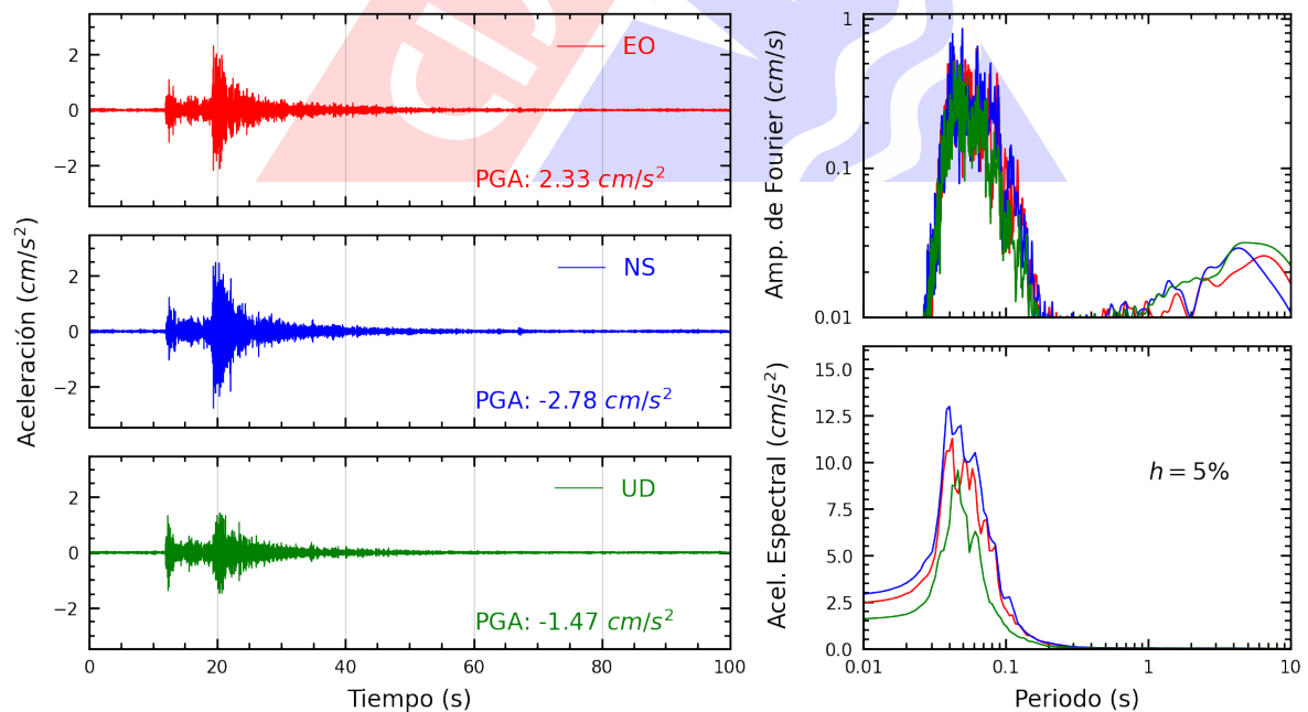
Figura A.4: Registros tiempo-historia, espectros de Fourier y de respuesta en las direcciones EO, NS y vertical de la estación JOSEO. Sismo de Ancon, Lima - Lima del 2025-05-12, 11:53:20 (Hora local)
