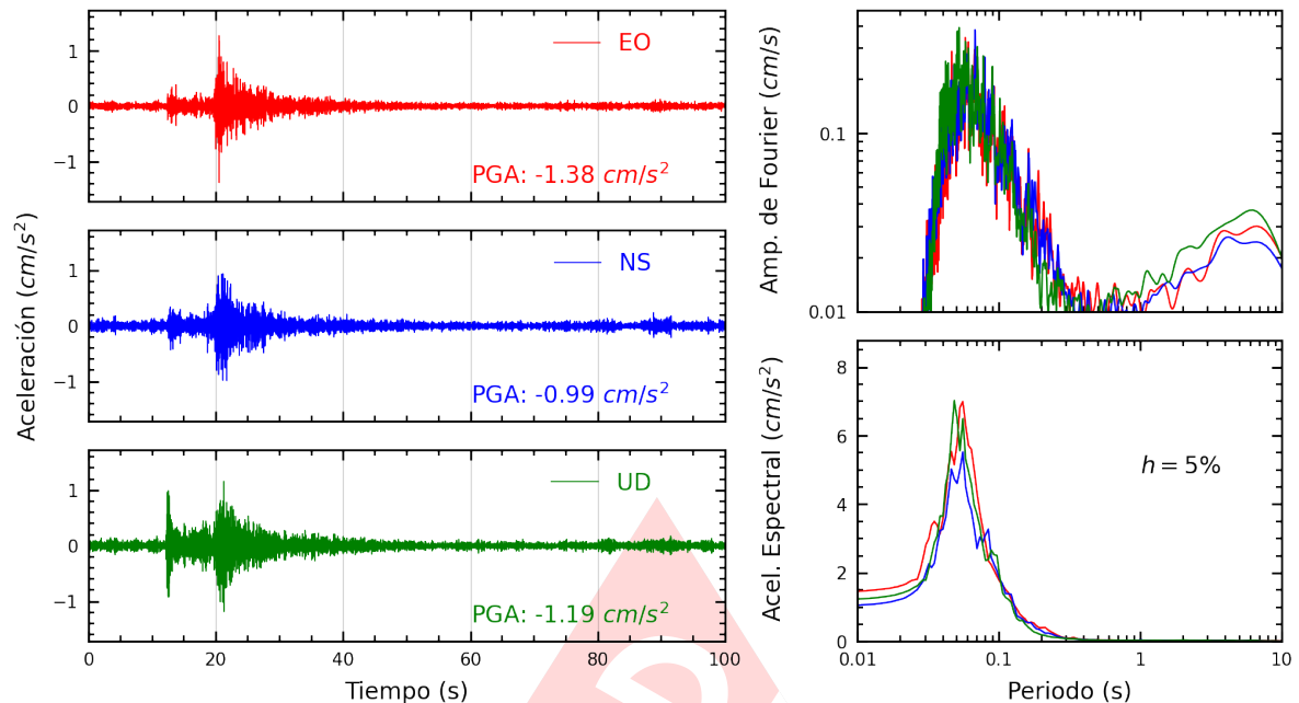
Figura A.15: Registros tiempo-historia, espectros de Fourier y de respuesta en las direcciones EO, NS y vertical de la estación SJLSC. Sismo de Ancon, Lima - Lima del 2025-05-12, 11:53:20 (Hora local)
