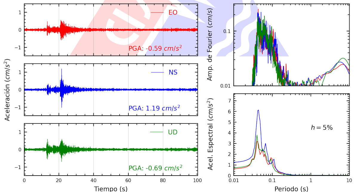
Figura A.18: Registros tiempo-historia, espectros de Fourier y de respuesta en las direcciones EO, NS y vertical de la estación URPPE. Sismo de Ancon, Lima - Lima del 2025-05-12, 11:53:20 (Hora local)
