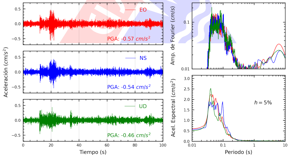
Figura A.30: Registros tiempo-historia, espectros de Fourier y de respuesta en las direcciones EO, NS y vertical de la estación MADRE. Sismo de Ancon, Lima - Lima del 2025-05-12, 11:53:20 (Hora local)
