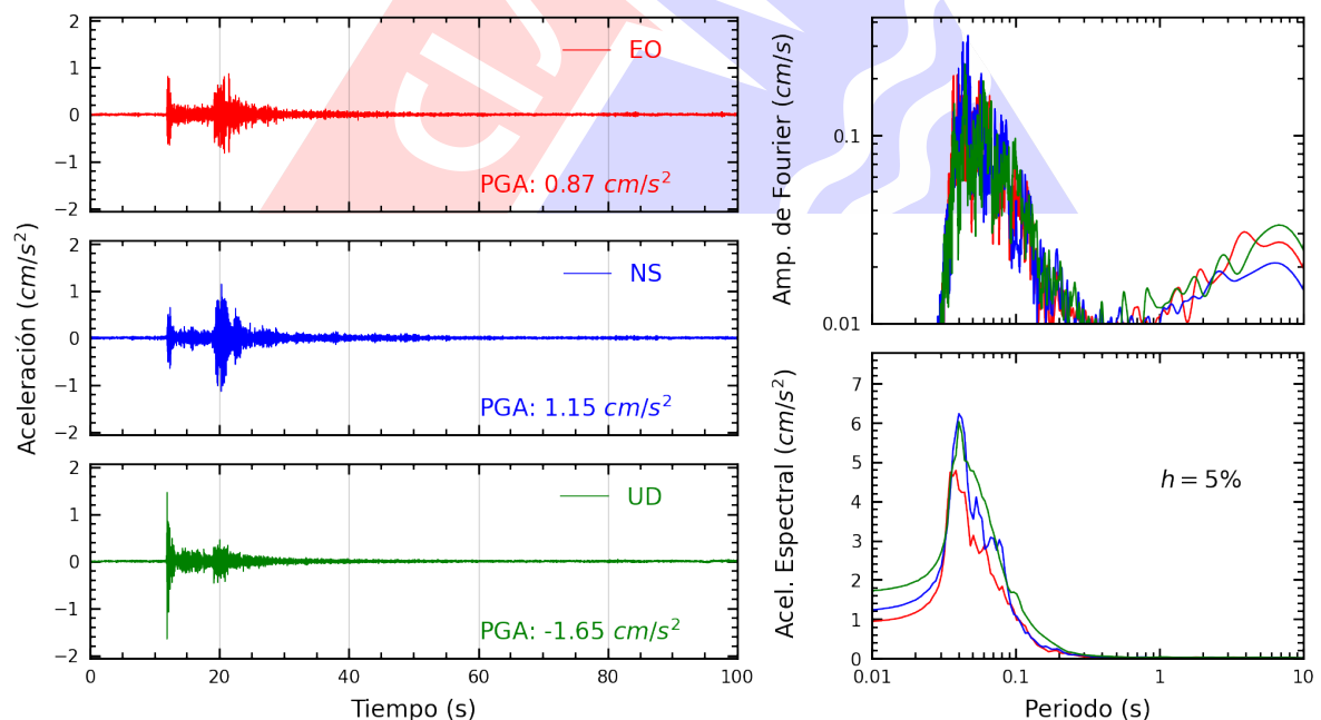
Figura A.10: Registros tiempo-historia, espectros de Fourier y de respuesta en las direcciones EO, NS y vertical de la estación COMAS. Sismo de Ancon, Lima - Lima del 2025-05-12, 11:53:20 (Hora local)
