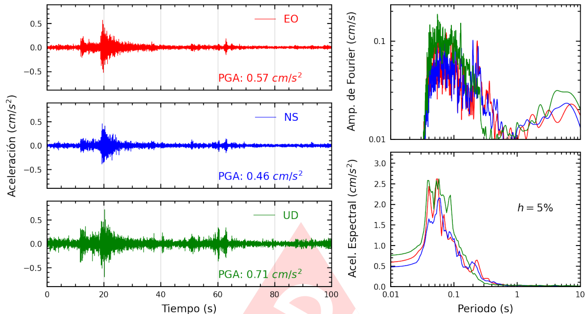
Figura A.25: Registros tiempo-historia, espectros de Fourier y de respuesta en las direcciones EO, NS y vertical de la estación MDPP. Sismo de Ancon, Lima - Lima del 2025-05-12, 11:53:20 (Hora local)
