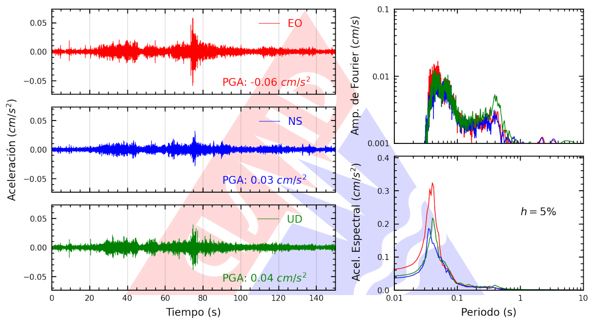
Figura A.41: Registros tiempo-historia, espectros de Fourier y de respuesta en las direcciones EO, NS y vertical de la estación UNCP. Sismo de Ancon, Lima - Lima del 2025-05-12, 11:53:20 (Hora local)
