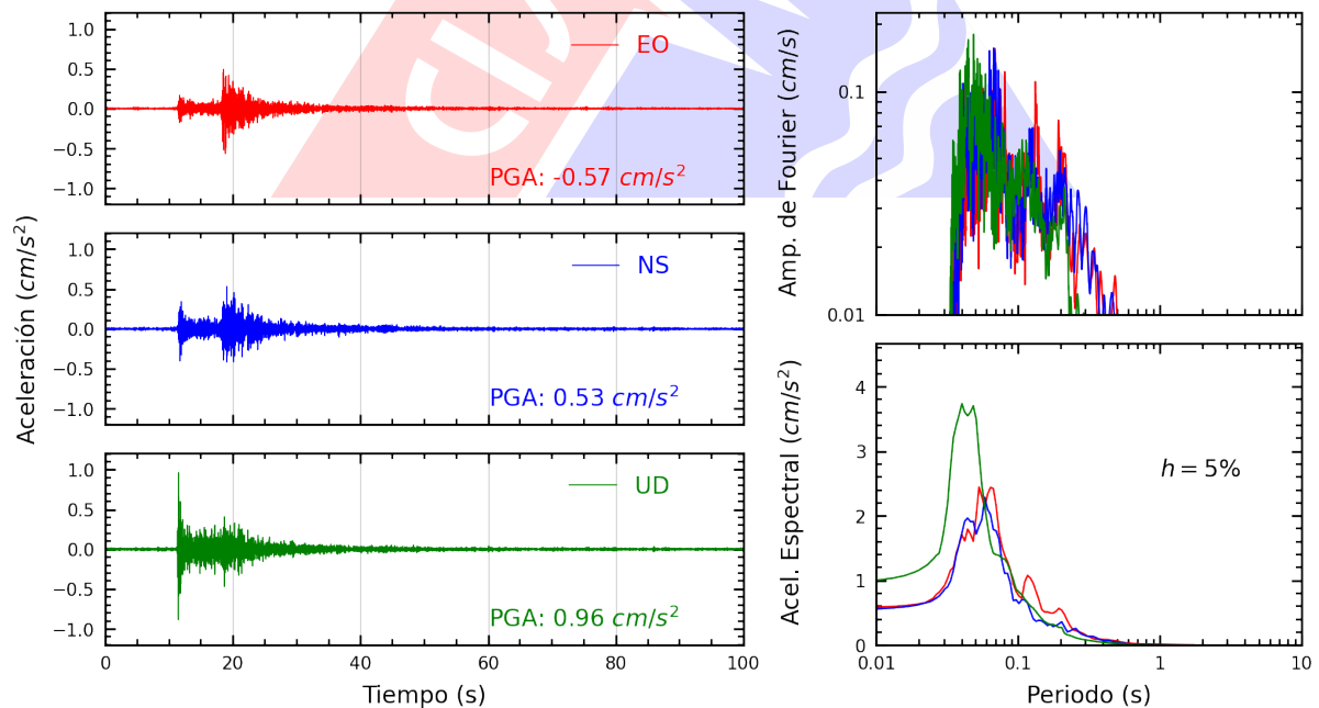
Figura A.22: Registros tiempo-historia, espectros de Fourier y de respuesta en las direcciones EO, NS y vertical de la estación VHAY2. Sismo de Ancon, Lima - Lima del 2025-05-12, 11:53:20 (Hora local)
