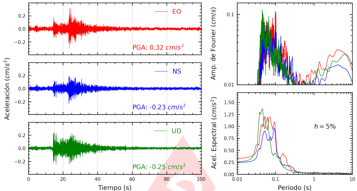
Figura A.35: Registros tiempo-historia, espectros de Fourier y de respuesta en las direcciones EO, NS y vertical de la estación USILP. Sismo de Ancon, Lima - Lima del 2025-05-12, 11:53:20 (Hora local)
