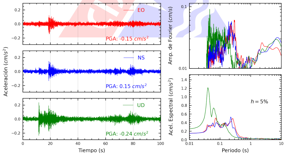
Figura A.38: Registros tiempo-historia, espectros de Fourier y de respuesta en las direcciones EO, NS y vertical de la estación DSMI. Sismo de Ancon, Lima - Lima del 2025-05-12, 11:53:20 (Hora local)
