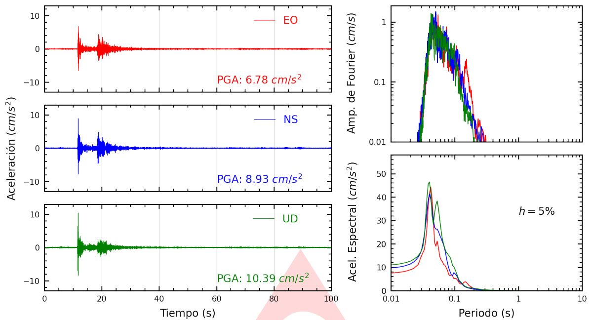
Figura A.1: Registros tiempo-historia, espectros de Fourier y de respuesta en las direcciones EO, NS y vertical de la estación SROS2. Sismo de Ancon, Lima - Lima del 2025-05-12, 11:53:20 (Hora local)
