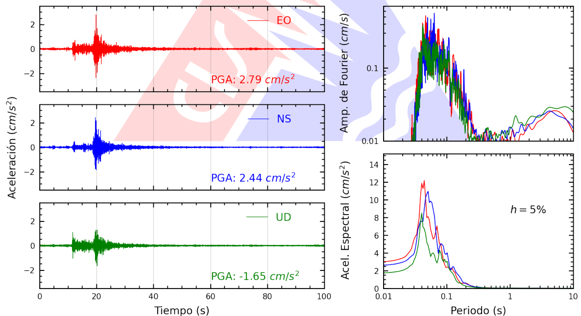
Figura A.2: Registros tiempo-historia, espectros de Fourier y de respuesta en las direcciones EO, NS y vertical de la estación INDEP. Sismo de Ancon, Lima - Lima del 2025-05-12, 11:53:20 (Hora local)
