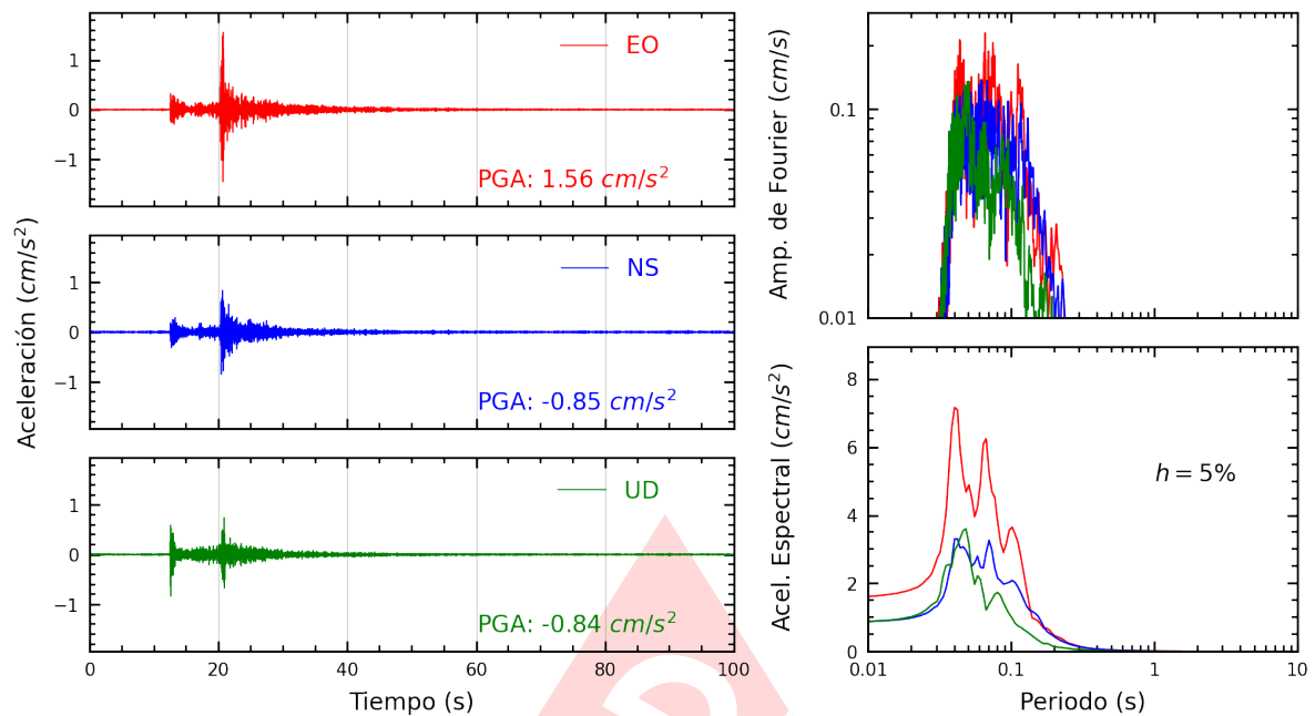
Figura A.11: Registros tiempo-historia, espectros de Fourier y de respuesta en las direcciones EO, NS y vertical de la estación ATARJ. Sismo de Ancon, Lima - Lima del 2025-05-12, 11:53:20 (Hora local)
