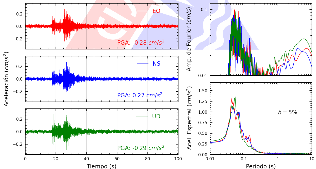
Figura A.36: Registros tiempo-historia, espectros de Fourier y de respuesta en las direcciones EO, NS y vertical de la estación UNMSM. Sismo de Ancon, Lima - Lima del 2025-05-12, 11:53:20 (Hora local)
