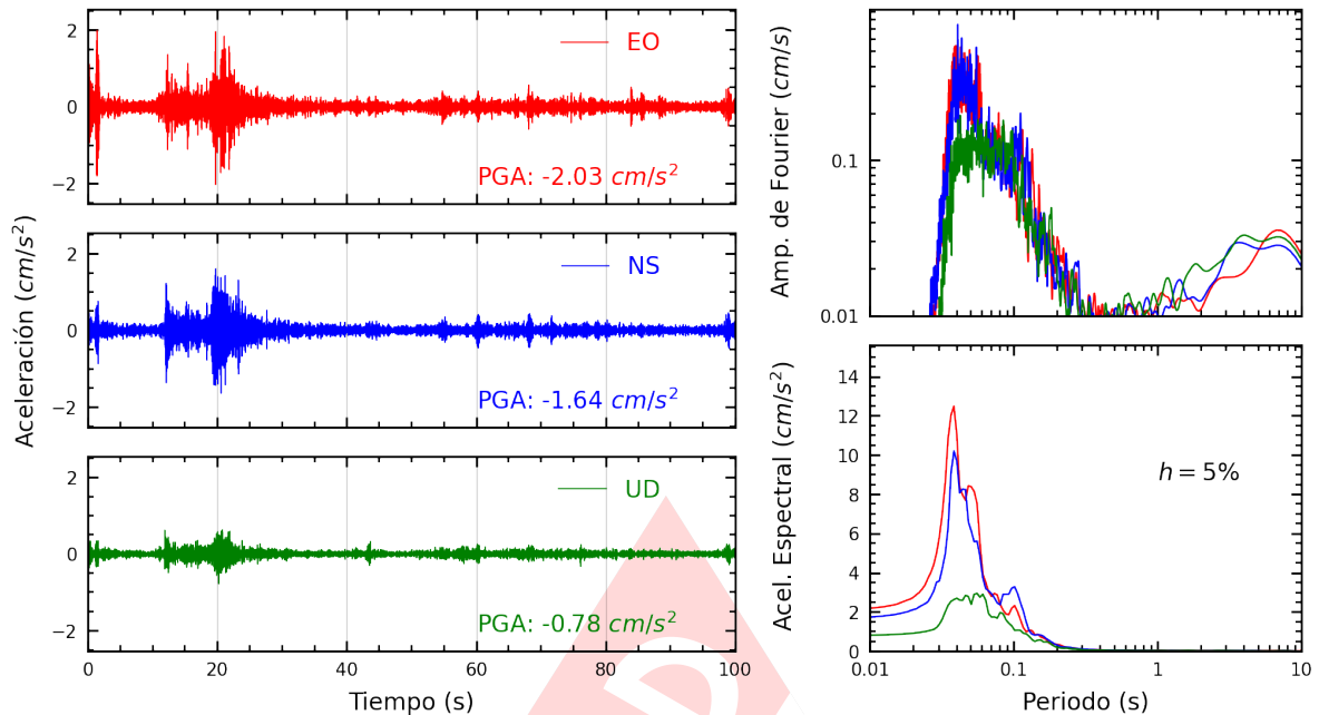
Figura A.7: Registros tiempo-historia, espectros de Fourier y de respuesta en las direcciones EO, NS y vertical de la estación OLIVO. Sismo de Ancon, Lima - Lima del 2025-05-12, 11:53:20 (Hora local)
