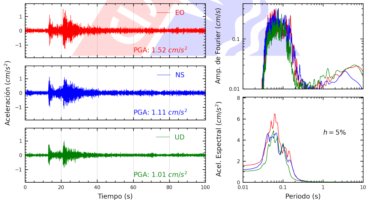
Figura A.12: Registros tiempo-historia, espectros de Fourier y de respuesta en las direcciones EO, NS y vertical de la estación USILM. Sismo de Ancon, Lima - Lima del 2025-05-12, 11:53:20 (Hora local)
