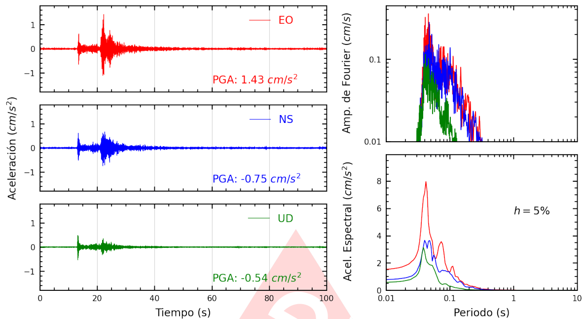
Figura A.13: Registros tiempo-historia, espectros de Fourier y de respuesta en las direcciones EO, NS y vertical de la estación UCVA2. Sismo de Ancon, Lima - Lima del 2025-05-12, 11:53:20 (Hora local)
