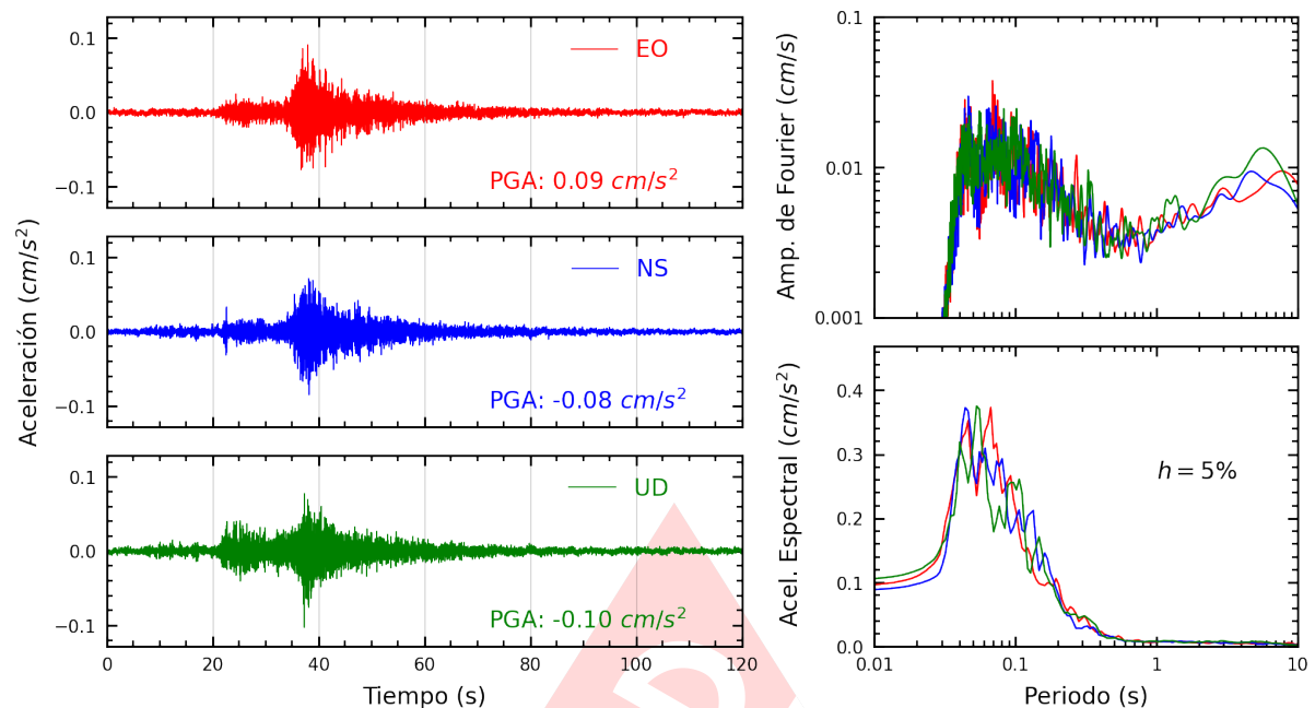
Figura A.39: Registros tiempo-historia, espectros de Fourier y de respuesta en las direcciones EO, NS y vertical de la estación CARAL. Sismo de Ancon, Lima - Lima del 2025-05-12, 11:53:20 (Hora local)
