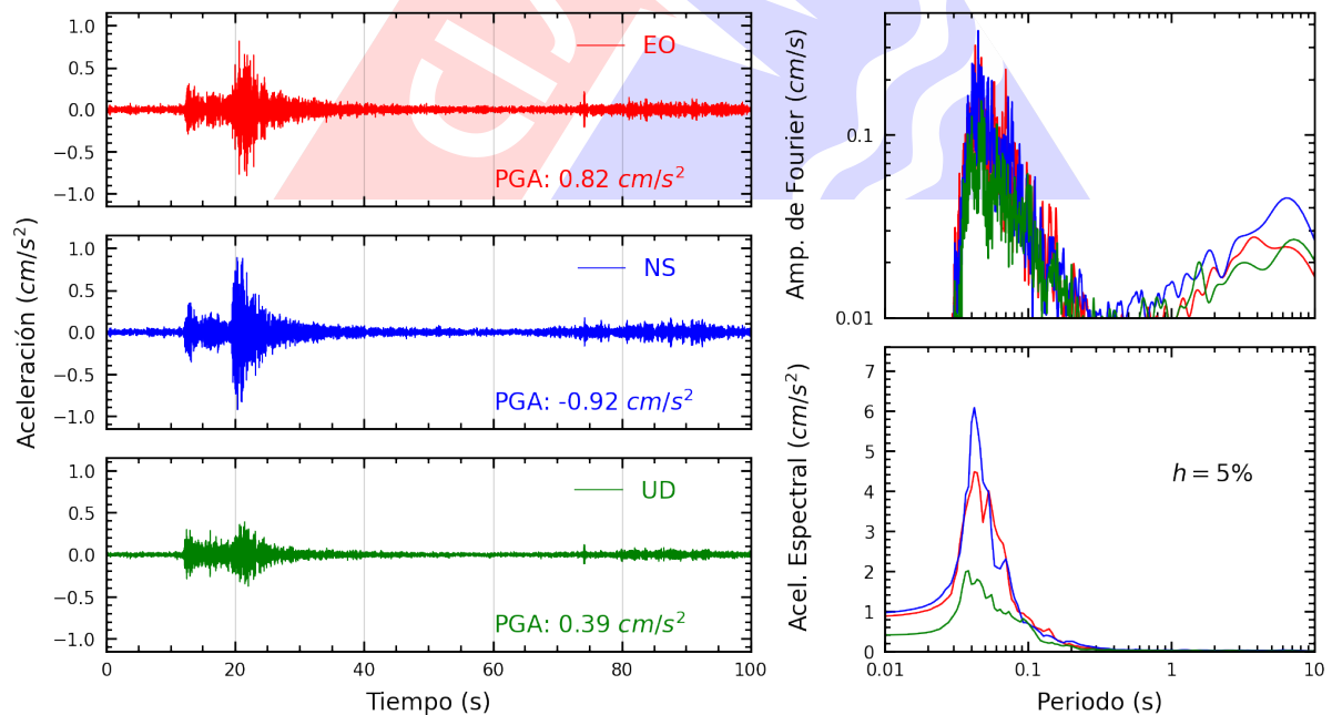
Figura A.24: Registros tiempo-historia, espectros de Fourier y de respuesta en las direcciones EO, NS y vertical de la estación CEPRE. Sismo de Ancon, Lima - Lima del 2025-05-12, 11:53:20 (Hora local)
