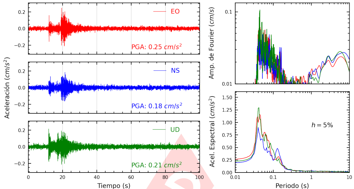
Figura A.37: Registros tiempo-historia, espectros de Fourier y de respuesta en las direcciones EO, NS y vertical de la estación BONDY. Sismo de Ancon, Lima - Lima del 2025-05-12, 11:53:20 (Hora local)
