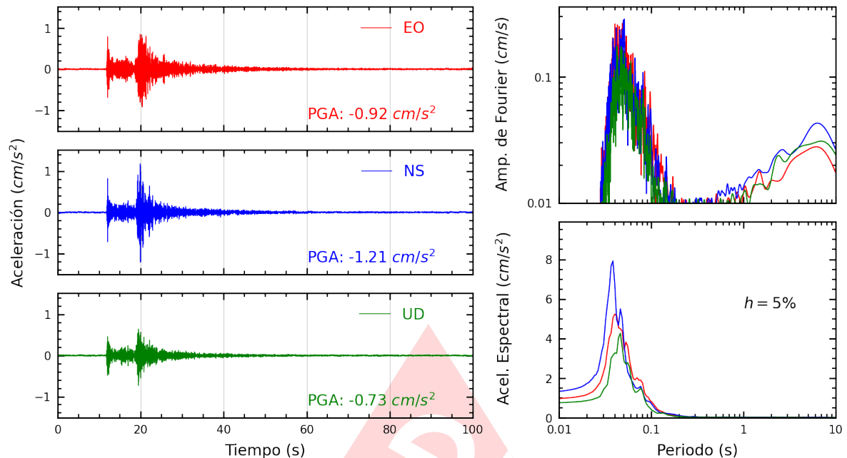
Figura A.17: Registros tiempo-historia, espectros de Fourier y de respuesta en las direcciones EO, NS y vertical de la estación UCSS. Sismo de Ancon, Lima - Lima del 2025-05-12, 11:53:20 (Hora local)
