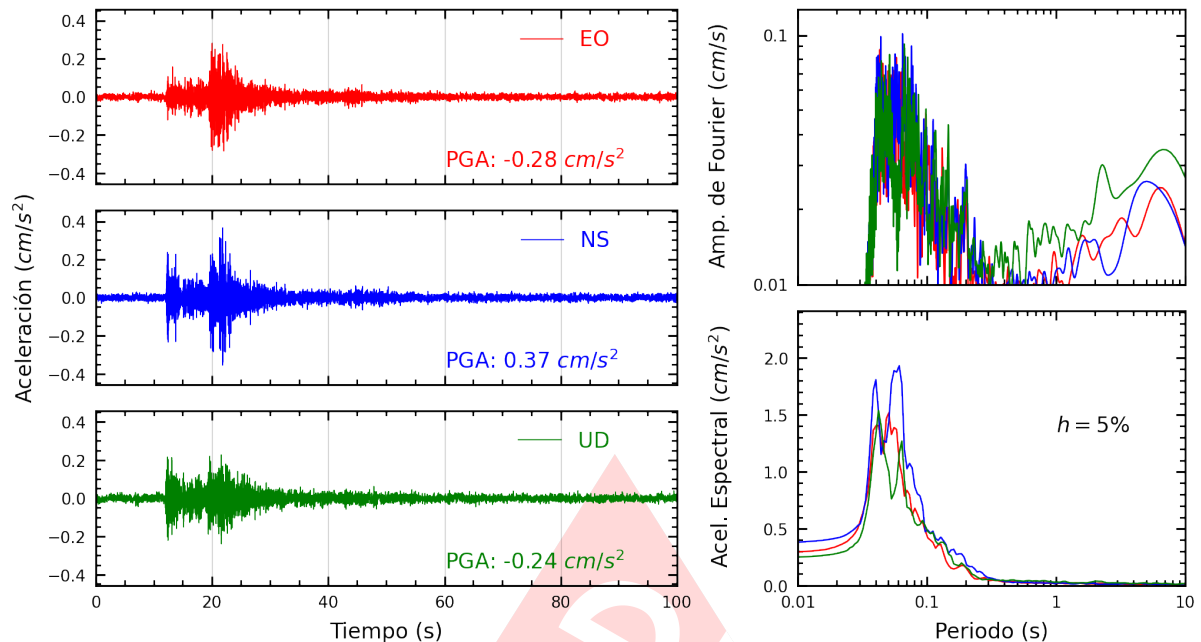
Figura A.33: Registros tiempo-historia, espectros de Fourier y de respuesta en las direcciones EO, NS y vertical de la estación UNFV. Sismo de Ancon, Lima - Lima del 2025-05-12, 11:53:20 (Hora local)
