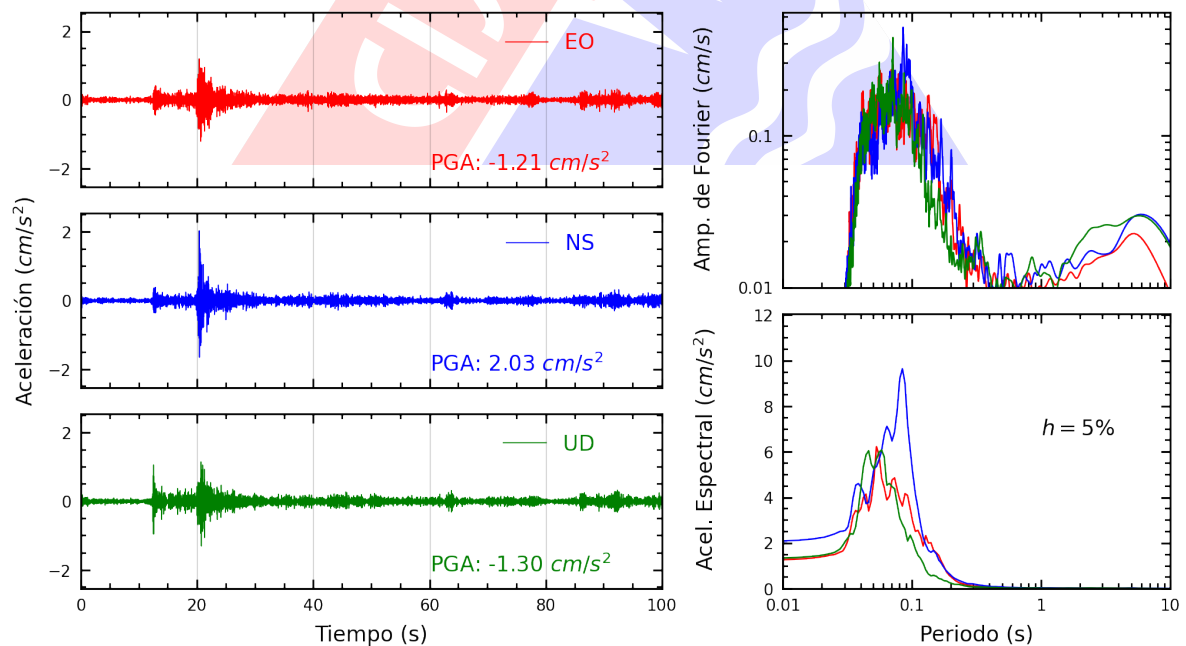
Figura A.6: Registros tiempo-historia, espectros de Fourier y de respuesta en las direcciones EO, NS y vertical de la estación SJLSV. Sismo de Ancon, Lima - Lima del 2025-05-12, 11:53:20 (Hora local)
