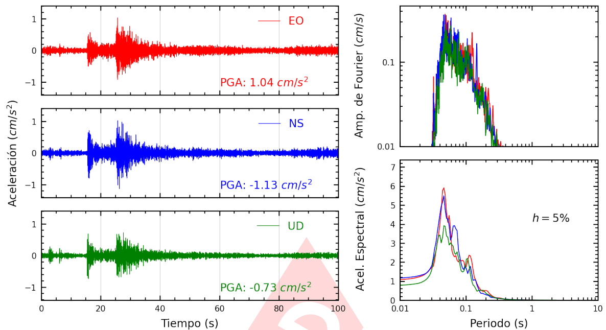
Figura A.19: Registros tiempo-historia, espectros de Fourier y de respuesta en las direcciones EO, NS y vertical de la estación PHER2. Sismo de Ancon, Lima - Lima del 2025-05-12, 11:53:20 (Hora local)
