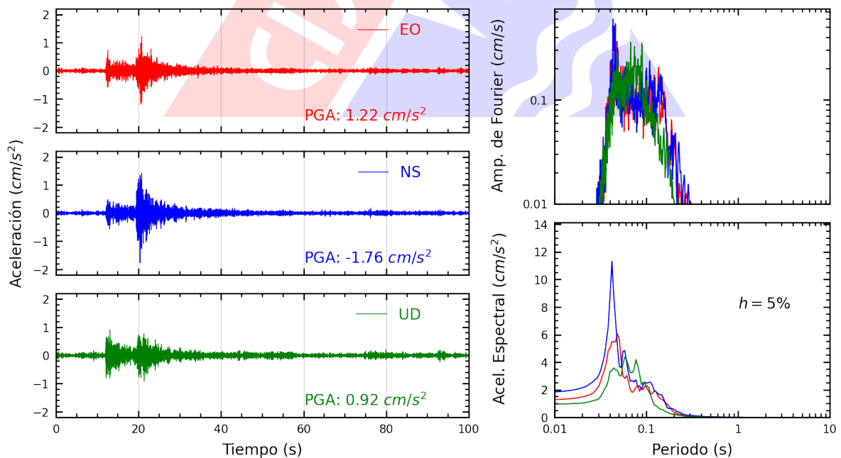
Figura A.8: Registros tiempo-historia, espectros de Fourier y de respuesta en las direcciones EO, NS y vertical de la estación CARA2. Sismo de Ancon, Lima - Lima del 2025-05-12, 11:53:20 (Hora local)
