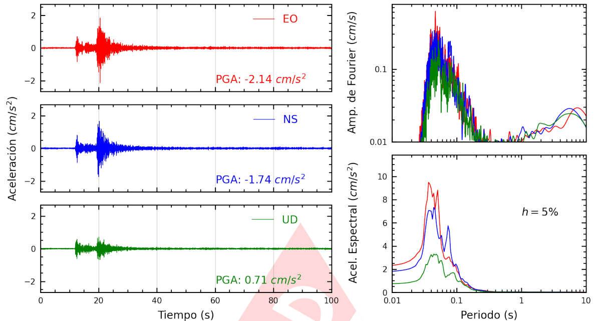
Figura A.5: Registros tiempo-historia, espectros de Fourier y de respuesta en las direcciones EO, NS y vertical de la estación FICPE. Sismo de Ancon, Lima - Lima del 2025-05-12, 11:53:20 (Hora local)
