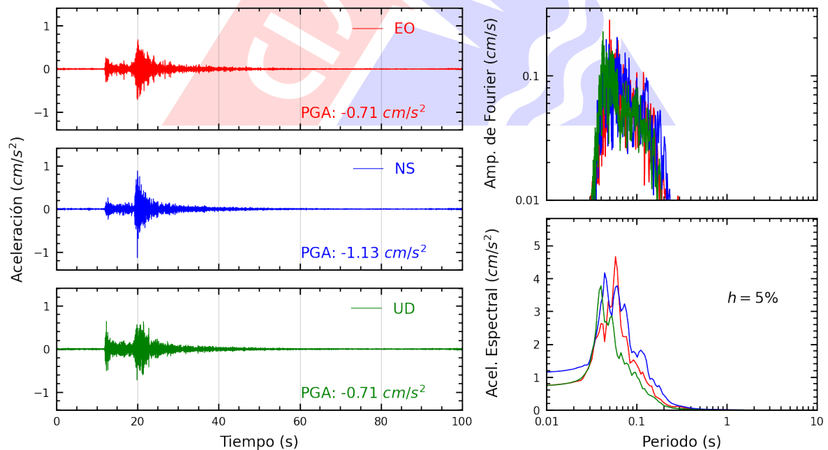
Figura A.20: Registros tiempo-historia, espectros de Fourier y de respuesta en las direcciones EO, NS y vertical de la estación JALV2. Sismo de Ancon, Lima - Lima del 2025-05-12, 11:53:20 (Hora local)
