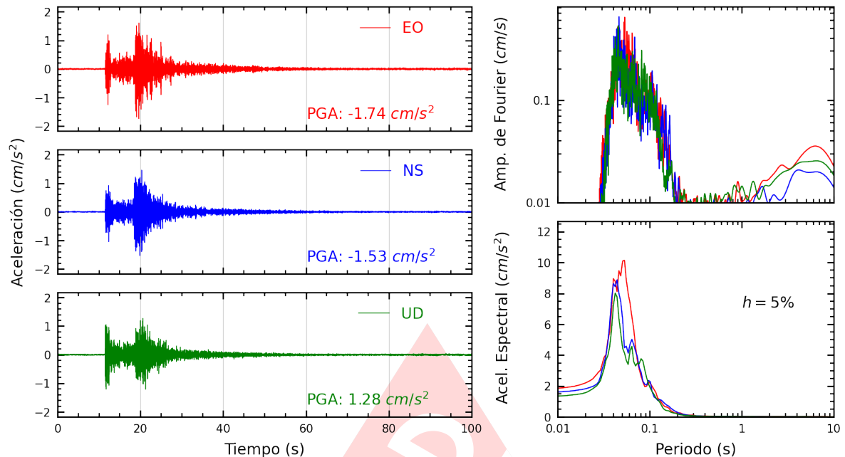
Figura A.9: Registros tiempo-historia, espectros de Fourier y de respuesta en las direcciones EO, NS y vertical de la estación AMORE. Sismo de Ancon, Lima - Lima del 2025-05-12, 11:53:20 (Hora local)
