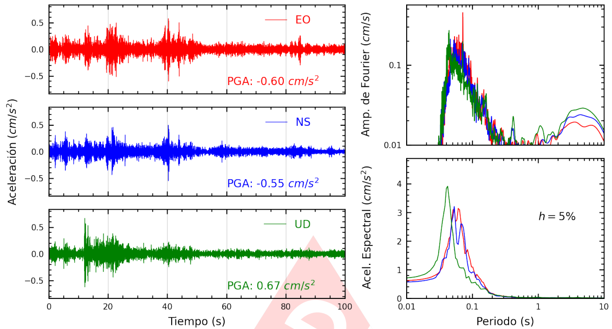
Figura A.27: Registros tiempo-historia, espectros de Fourier y de respuesta en las direcciones EO, NS y vertical de la estación UPCSM. Sismo de Ancon, Lima - Lima del 2025-05-12, 11:53:20 (Hora local)
