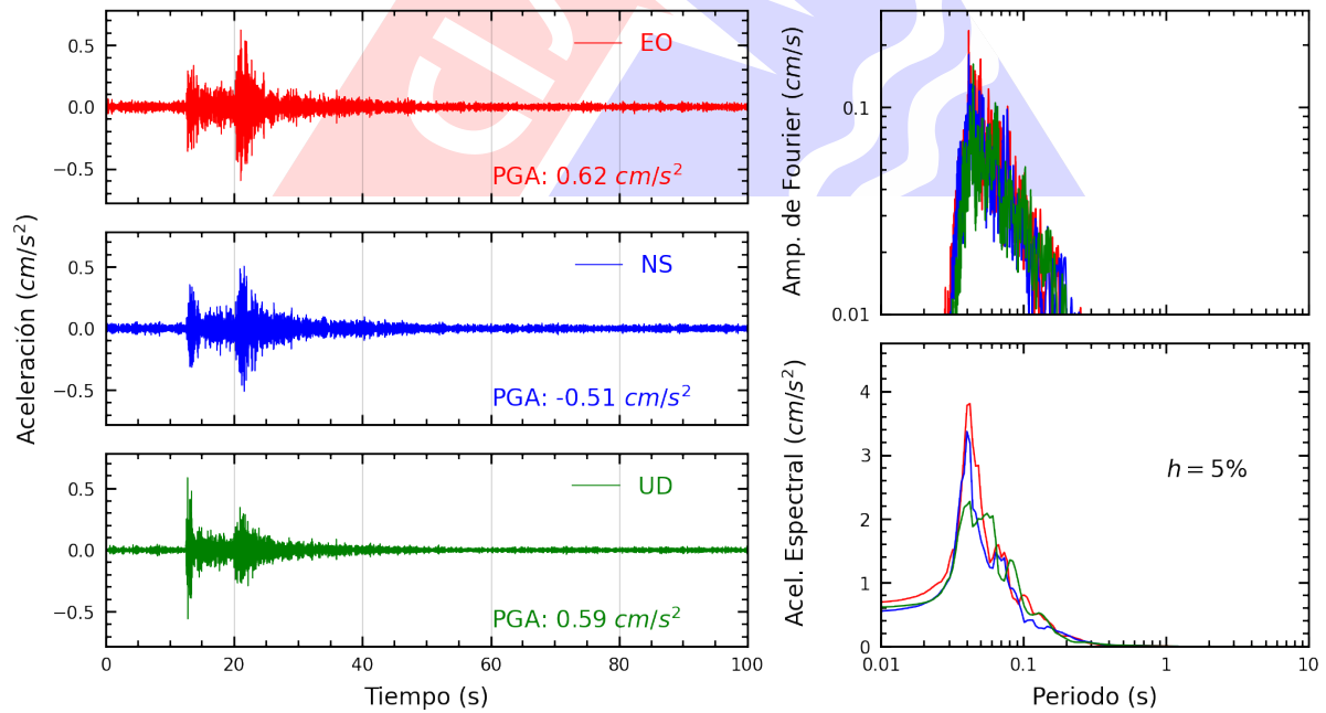
Figura A.28: Registros tiempo-historia, espectros de Fourier y de respuesta en las direcciones EO, NS y vertical de la estación BORJA. Sismo de Ancon, Lima - Lima del 2025-05-12, 11:53:20 (Hora local)
