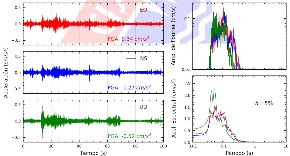
Figura A.32: Registros tiempo-historia, espectros de Fourier y de respuesta en las direcciones EO, NS y vertical de la estación SCCHO. Sismo de Ancon, Lima - Lima del 2025-05-12, 11:53:20 (Hora local)
