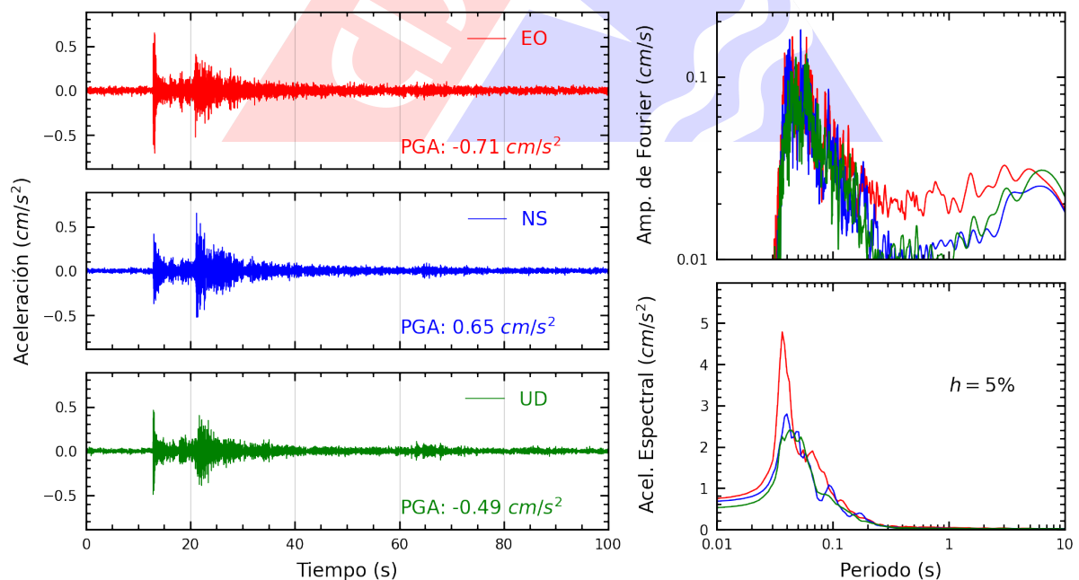
Figura A.26: Registros tiempo-historia, espectros de Fourier y de respuesta en las direcciones EO, NS y vertical de la estación IMCA. Sismo de Ancon, Lima - Lima del 2025-05-12, 11:53:20 (Hora local)
