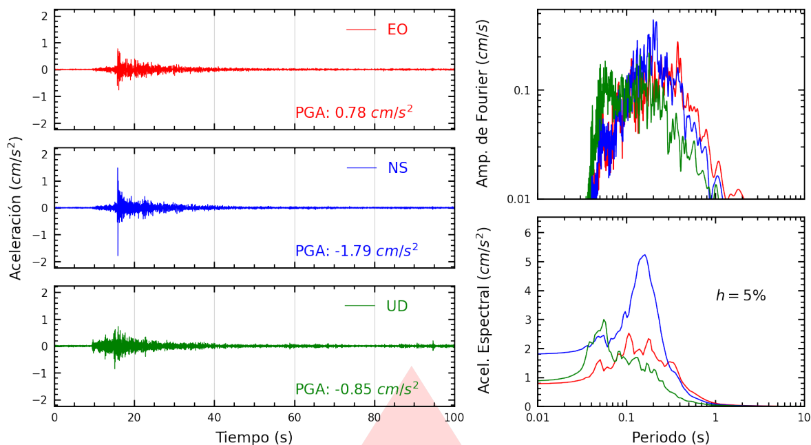
Figura A.1: Registros tiempo-historia, espectros de Fourier y de respuesta en las direcciones EO, NS y vertical de la estación UNP. Sismo de Sullana, Sullana - Piura del 2025-05-15, 08:03:00 (Hora local)
