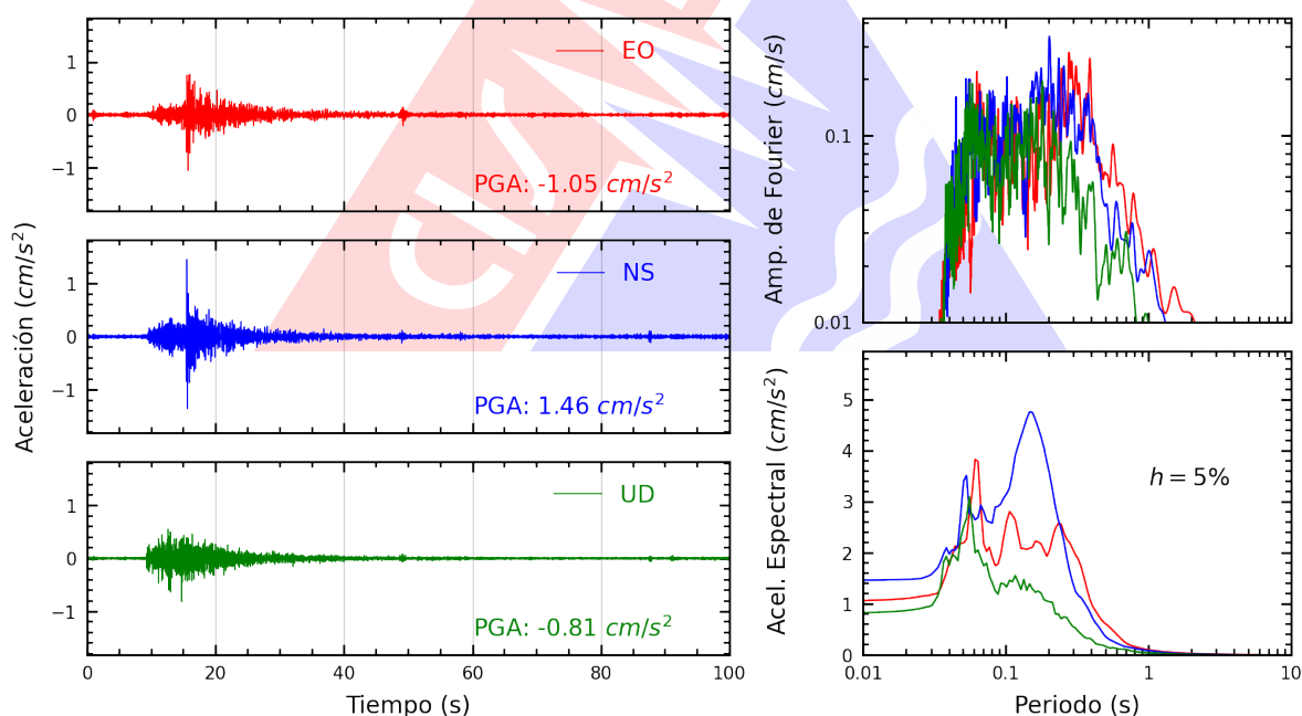
Figura A.2: Registros tiempo-historia, espectros de Fourier y de respuesta en las direcciones EO, NS y vertical de la estación UPAOP. Sismo de Sullana, Sullana - Piura del 2025-05-15, 08:03:00 (Hora local)
