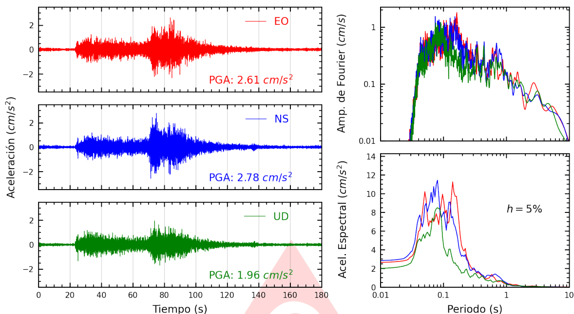
Figura A.13: Registros tiempo-historia, espectros de Fourier y de respuesta en las direcciones EO, NS y vertical de la estación SROS2. Sismo de Puquío, Lucanas - Ayacucho del 2025-05-17, 05:22:14 (Hora local)
