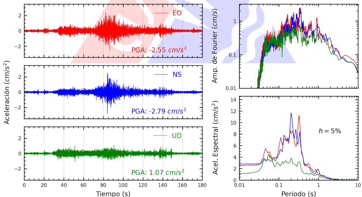
Figura A.12: Registros tiempo-historia, espectros de Fourier y de respuesta en las direcciones EO, NS y vertical de la estación SOBAR. Sismo de Puquio, Lucanas - Ayacucho del 2025-05-17, 05:22:14 (Hora local)
