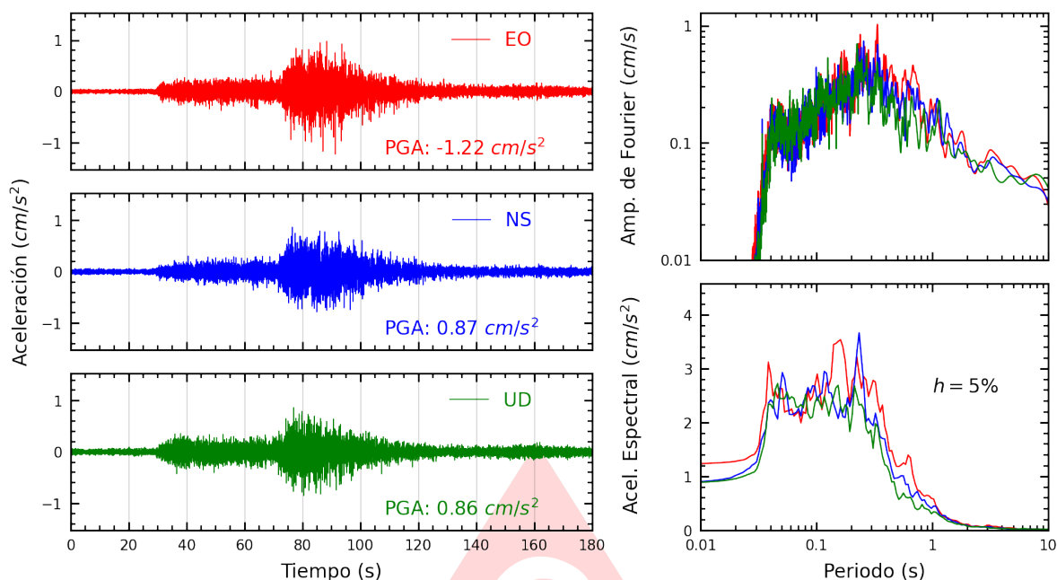
Figura A.37: Registros tiempo-historia, espectros de Fourier y de respuesta en las direcciones EO, NS y vertical de la estación USMP. Sismo de Puquio, Lucanas - Ayacucho del 2025-05-17, 05:22:14 (Hora local)
