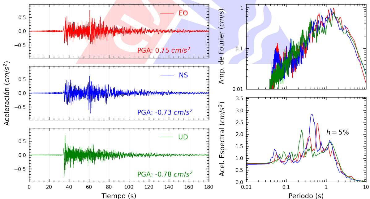
Figura A.48: Registros tiempo-historia, espectros de Fourier y de respuesta en las direcciones EO, NS y vertical de la estación UNMBA. Sismo de Puquio, Lucanas - Ayacucho del 2025-05-17, 05:22:14 (Hora local)
