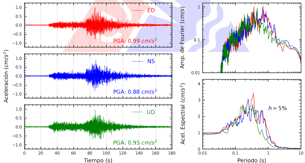
Figura A.42: Registros tiempo-historia, espectros de Fourier y de respuesta en las direcciones EO, NS y vertical de la estación UNFV. Sismo de Puquío, Lucanas - Ayacucho del 2025-05-17, 05:22:14 (Hora local)
