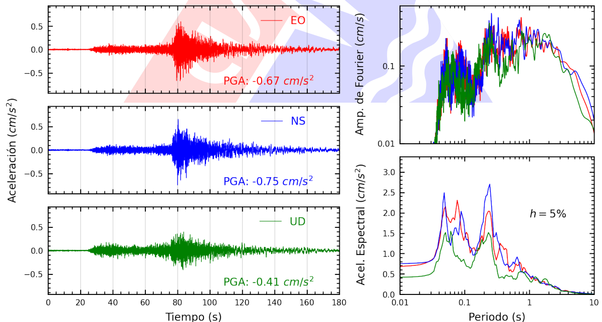
Figura A.50: Registros tiempo-historia, espectros de Fourier y de respuesta en las direcciones EO, NS y vertical de la estación CREY. Sismo de Puquío, Lucanas - Ayacucho del 2025-05-17, 05:22:14 (Hora local)
