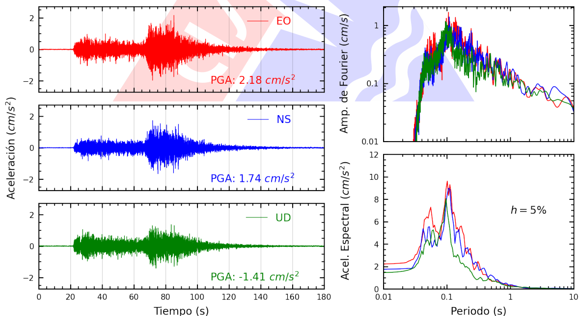
Figura A.18: Registros tiempo-historia, espectros de Fourier y de respuesta en las direcciones EO, NS y vertical de la estación AMORE. Sismo de Puquio, Lucanas - Ayacucho del 2025-05-17, 05:22:14 (Hora local)
