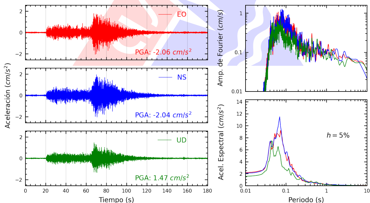
Figura A.22: Registros tiempo-historia, espectros de Fourier y de respuesta en las direcciones EO, NS y vertical de la estación JOSEO. Sismo de Puquío, Lucanas - Ayacucho del 2025-05-17, 05:22:14 (Hora local)
