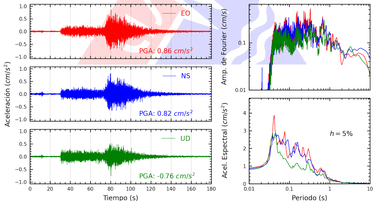
Figura A.46: Registros tiempo-historia, espectros de Fourier y de respuesta en las direcciones EO, NS y vertical de la estación SJLCE. Sismo de Puquío, Lucanas - Ayacucho del 2025-05-17, 05:22:14 (Hora local)
