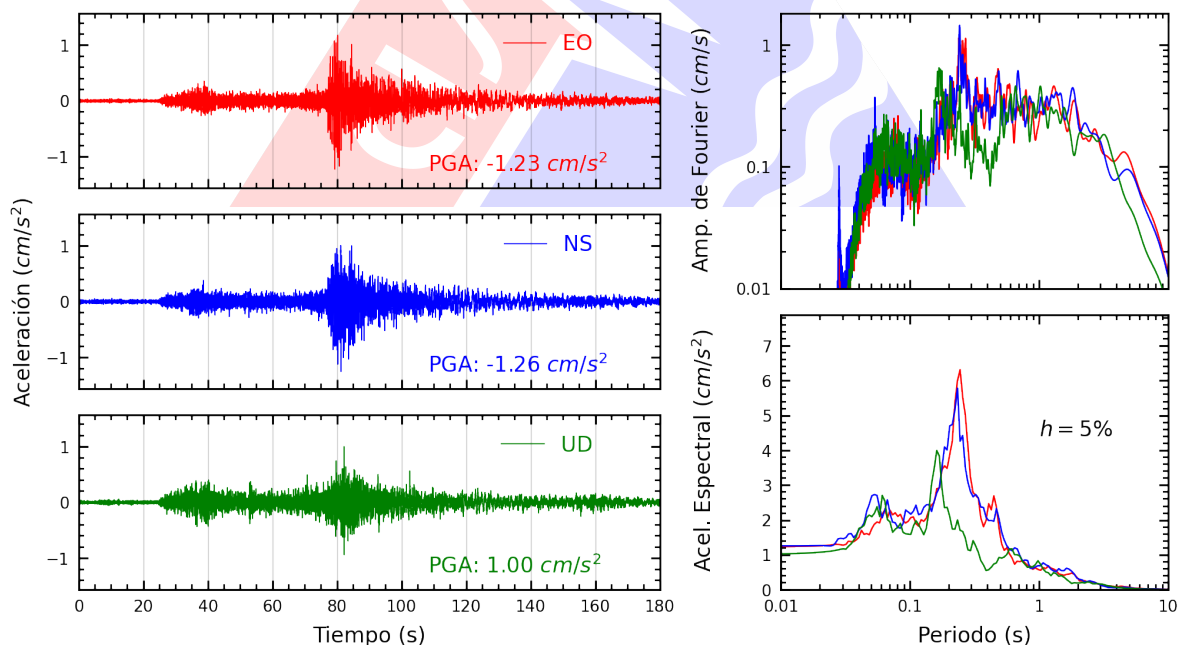
Figura A.36: Registros tiempo-historia, espectros de Fourier y de respuesta en las direcciones EO, NS y vertical de la estación UJBG4. Sismo de Puquio, Lucanas - Ayacucho del 2025-05-17, 05:22:14 (Hora local)
