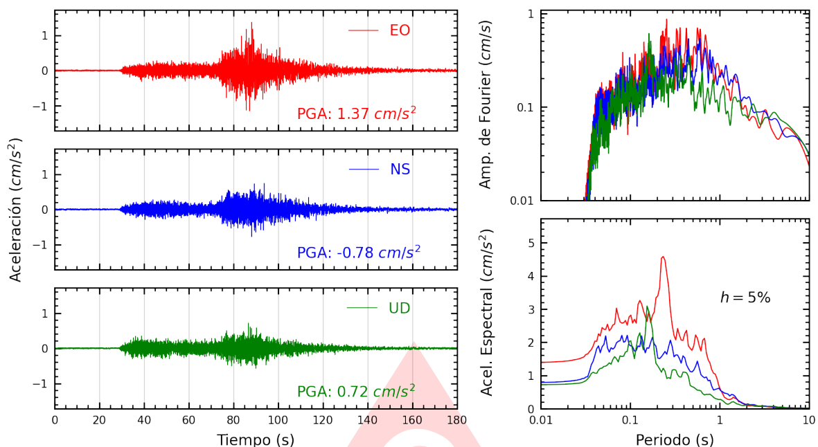
Figura A.33: Registros tiempo-historia, espectros de Fourier y de respuesta en las direcciones EO, NS y vertical de la estación CEPRE. Sismo de Puquio, Lucanas - Ayacucho del 2025-05-17, 05:22:14 (Hora local)
