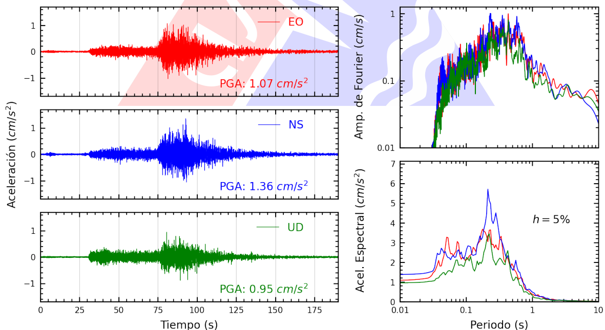
Figura A.34: Registros tiempo-historia, espectros de Fourier y de respuesta en las direcciones EO, NS y vertical de la estación COMAS. Sismo de Puquio, Lucanas - Ayacucho del 2025-05-17, 05:22:14 (Hora local)
