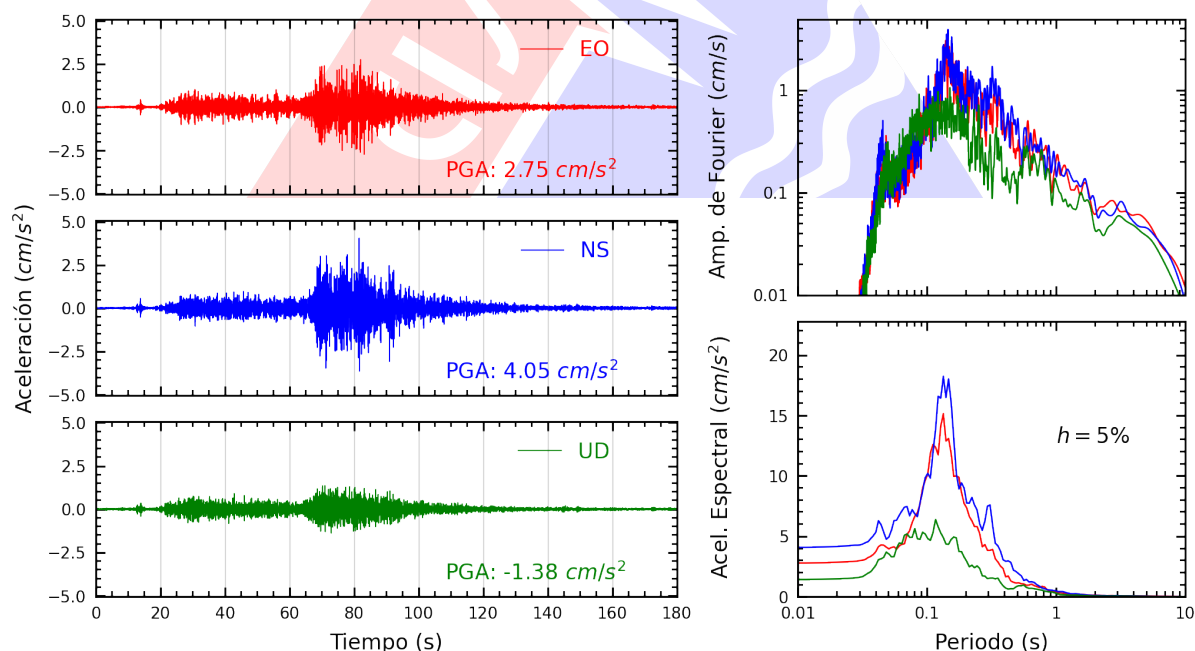
Figura A.4: Registros tiempo-historia, espectros de Fourier y de respuesta en las direcciones EO, NS y vertical de la estación CARA2. Sismo de Puquio, Lucanas - Ayacucho del 2025-05-17, 05:22:14 (Hora local)
