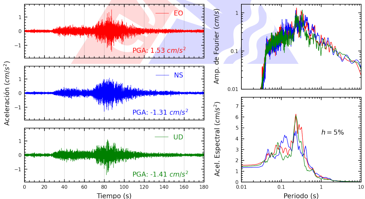
Figura A.30: Registros tiempo-historia, espectros de Fourier y de respuesta en las direcciones EO, NS y vertical de la estación URPPE. Sismo de Puquio, Lucanas - Ayacucho del 2025-05-17, 05:22:14 (Hora local)
