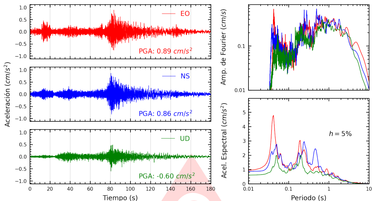
Figura A.45: Registros tiempo-historia, espectros de Fourier y de respuesta en las direcciones EO, NS y vertical de la estación UPTAC. Sismo de Puquío, Lucanas - Ayacucho del 2025-05-17, 05:22:14 (Hora local)
