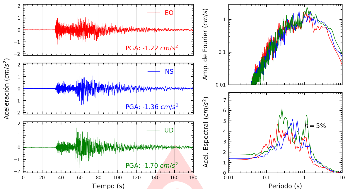
Figura A.25: Registros tiempo-historia, espectros de Fourier y de respuesta en las direcciones EO, NS y vertical de la estación UNSCH. Sismo de Puquio, Lucanas - Ayacucho del 2025-05-17, 05:22:14 (Hora local)
