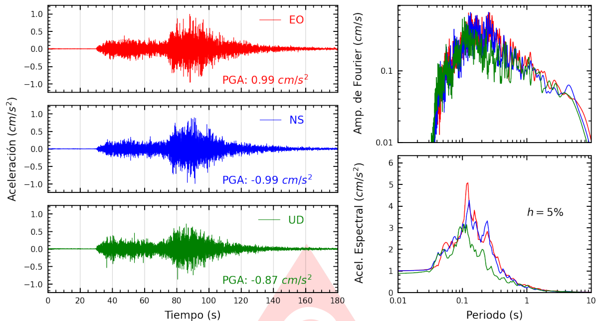
Figura A.41: Registros tiempo-historia, espectros de Fourier y de respuesta en las direcciones EO, NS y vertical de la estación JALV2. Sismo de Puquío, Lucanas - Ayacucho del 2025-05-17, 05:22:14 (Hora local)
