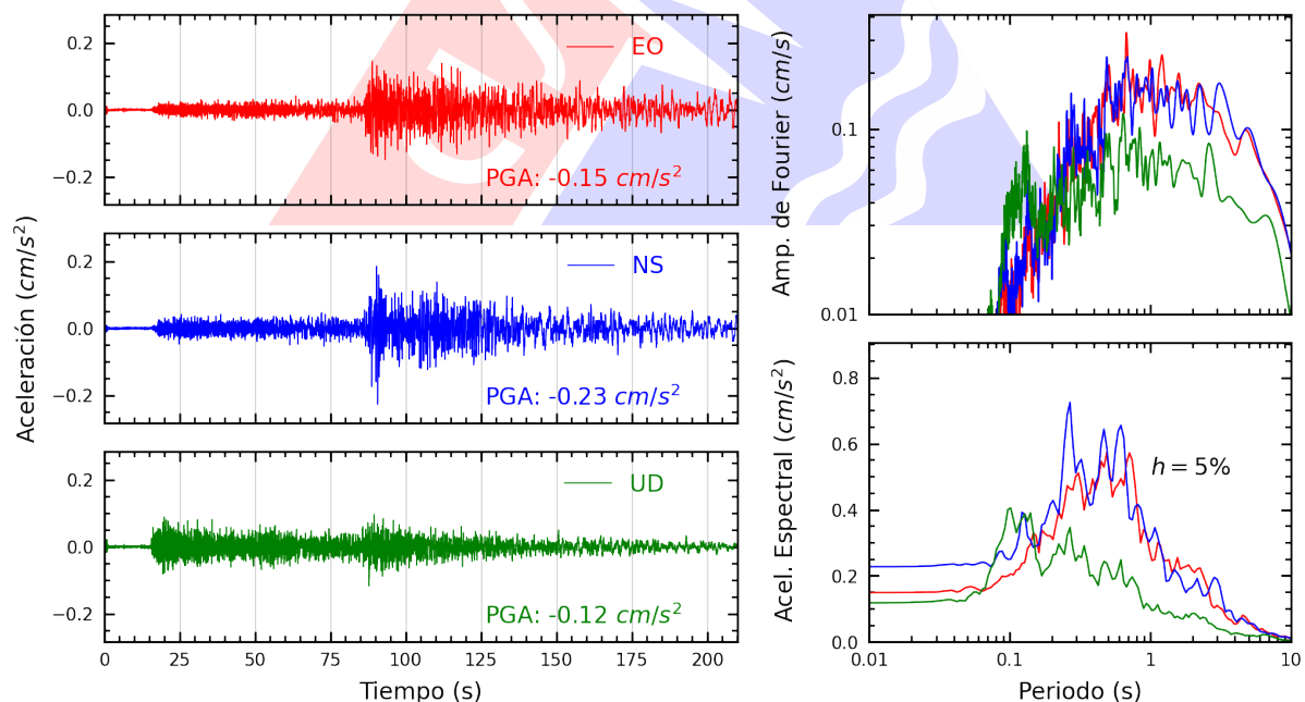
Figura A.52: Registros tiempo-historia, espectros de Fourier y de respuesta en las direcciones EO, NS y vertical de la estación UNIA. Sismo de Puquio, Lucanas - Ayacucho del 2025-05-17, 05:22:14 (Hora local)
