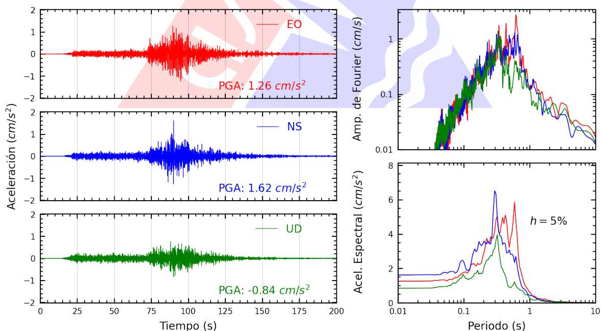
Figura A.28: Registros tiempo-historia, espectros de Fourier y de respuesta en las direcciones EO, NS y vertical de la estación CARAL. Sismo de Puquio, Lucanas - Ayacucho del 2025-05-17, 05:22:14 (Hora local)
