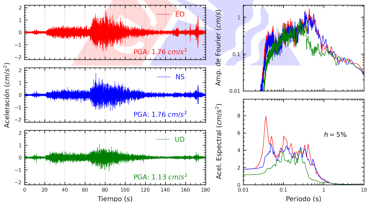
Figura A.24: Registros tiempo-historia, espectros de Fourier y de respuesta en las direcciones EO, NS y vertical de la estación OLIVO. Sismo de Puquio, Lucanas - Ayacucho del 2025-05-17, 05:22:14 (Hora local)
