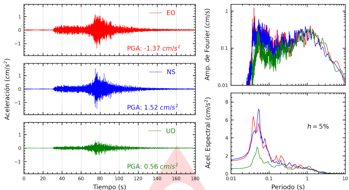
Figura A.31: Registros tiempo-historia, espectros de Fourier y de respuesta en las direcciones EO, NS y vertical de la estación UNAM. Sismo de Puquio, Lucanas - Ayacucho del 2025-05-17, 05:22:14 (Hora local)
