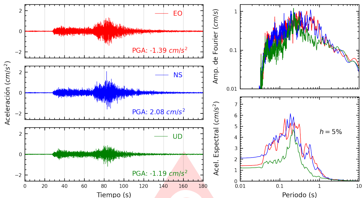
Figura A.21: Registros tiempo-historia, espectros de Fourier y de respuesta en las direcciones EO, NS y vertical de la estación UPCVI. Sismo de Puquío, Lucanas - Ayacucho del 2025-05-17, 05:22:14 (Hora local)
