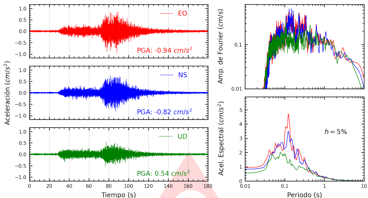
Figura A.43: Registros tiempo-historia, espectros de Fourier y de respuesta en las direcciones EO, NS y vertical de la estación ATARJ. Sismo de Puquio, Lucanas - Ayacucho del 2025-05-17, 05:22:14 (Hora local)
