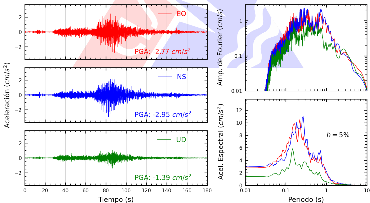
Figura A.10: Registros tiempo-historia, espectros de Fourier y de respuesta en las direcciones EO, NS y vertical de la estación BRIS2. Sismo de Puquío, Lucanas - Ayacucho del 2025-05-17, 05:22:14 (Hora local)
