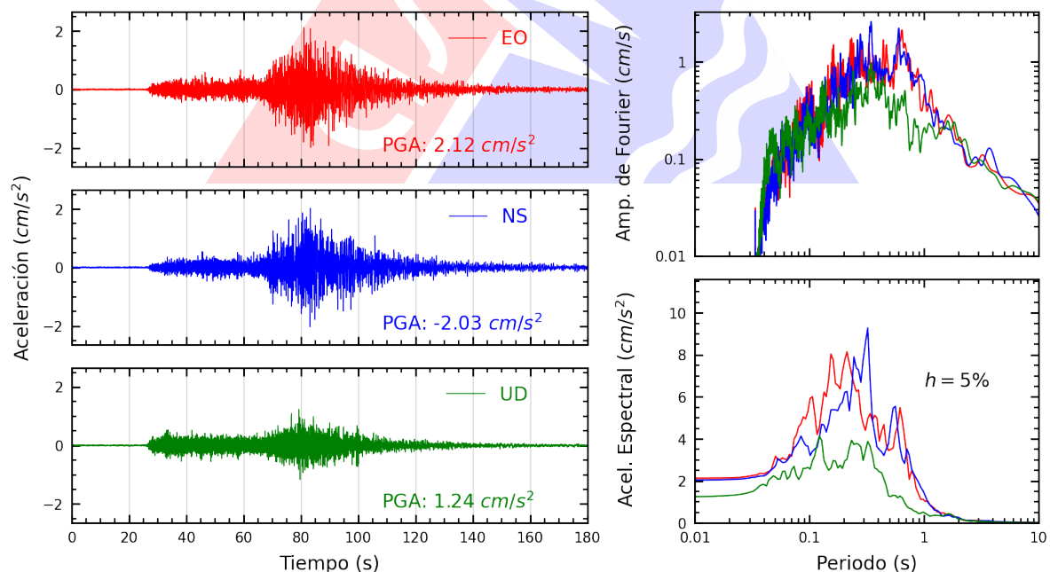
Figura A.20: Registros tiempo-historia, espectros de Fourier y de respuesta en las direcciones EO, NS y vertical de la estación USILP. Sismo de Puquio, Lucanas - Ayacucho del 2025-05-17, 05:22:14 (Hora local)
