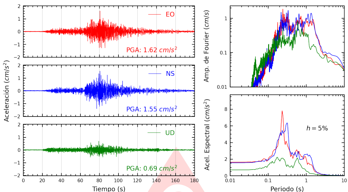
Figura A.27: Registros tiempo-historia, espectros de Fourier y de respuesta en las direcciones EO, NS y vertical de la estación DSML. Sismo de Puquio, Lucanas - Ayacucho del 2025-05-17, 05:22:14 (Hora local)
