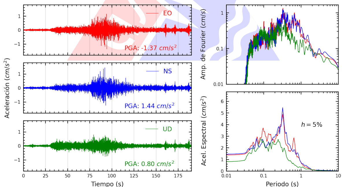
Figura A.32: Registros tiempo-historia, espectros de Fourier y de respuesta en las direcciones EO, NS y vertical de la estación MADRE. Sismo de Puquio, Lucanas - Ayacucho del 2025-05-17, 05:22:14 (Hora local)
