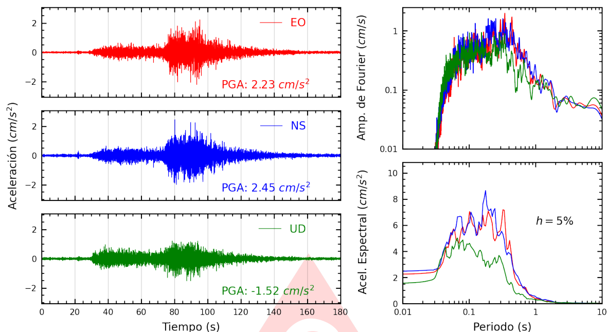
Figura A.15: Registros tiempo-historia, espectros de Fourier y de respuesta en las direcciones EO, NS y vertical de la estación SJLSC. Sismo de Puquio, Lucanas - Ayacucho del 2025-05-17, 05:22:14 (Hora local)
