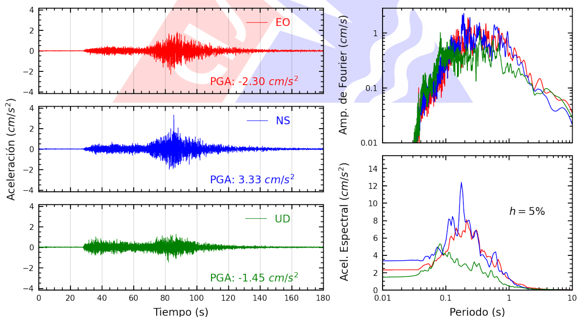
Figura A.8: Registros tiempo-historia, espectros de Fourier y de respuesta en las direcciones EO, NS y vertical de la estación SOCHO. Sismo de Puquío, Lucanas - Ayacucho del 2025-05-17, 05:22:14 (Hora local)
