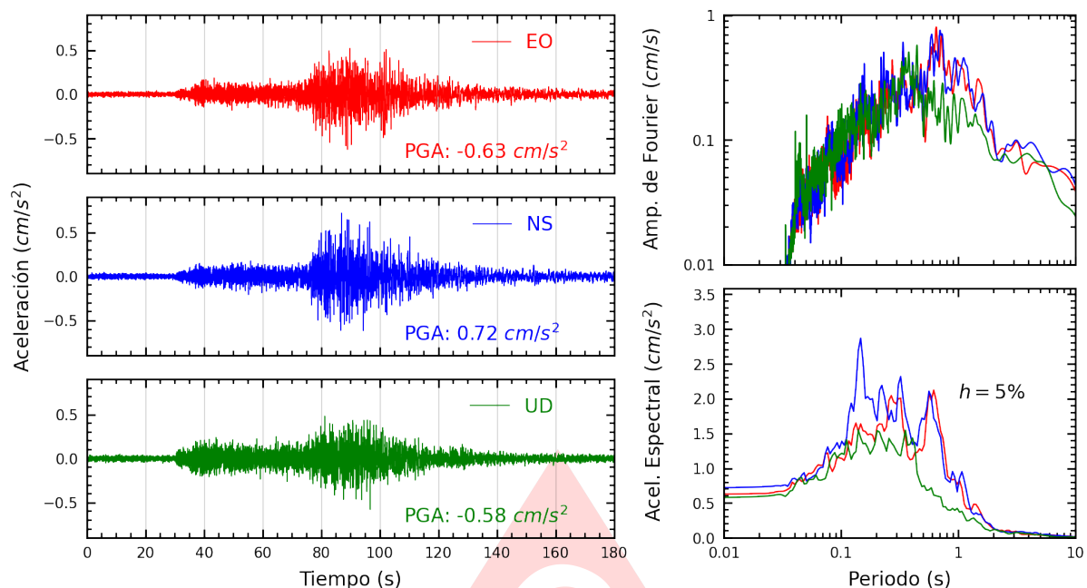
Figura A.51: Registros tiempo-historia, espectros de Fourier y de respuesta en las direcciones EO, NS y vertical de la estación BONDY. Sismo de Puquio, Lucanas - Ayacucho del 2025-05-17, 05:22:14 (Hora local)
