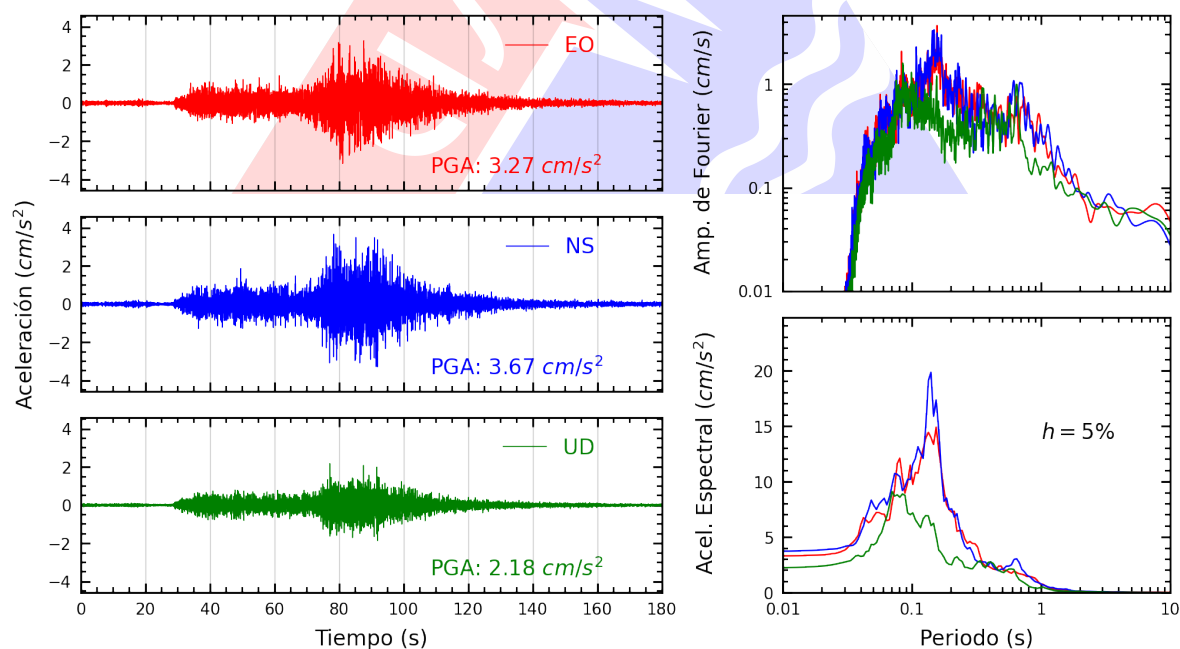
Figura A.6: Registros tiempo-historia, espectros de Fourier y de respuesta en las direcciones EO, NS y vertical de la estación USILM. Sismo de Puquio, Lucanas - Ayacucho del 2025-05-17, 05:22:14 (Hora local)
