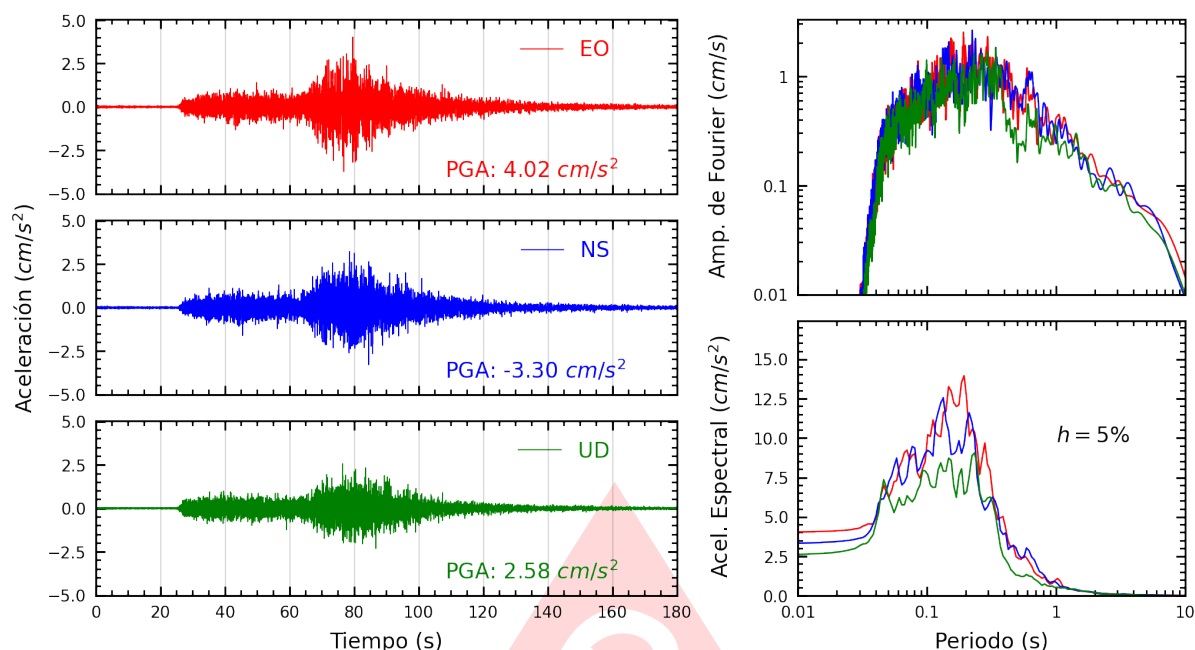
Figura A.5: Registros tiempo-historia, espectros de Fourier y de respuesta en las direcciones EO, NS y vertical de la estación PHER2. Sismo de Puquio, Lucanas - Ayacucho del 2025-05-17, 05:22:14 (Hora local)
