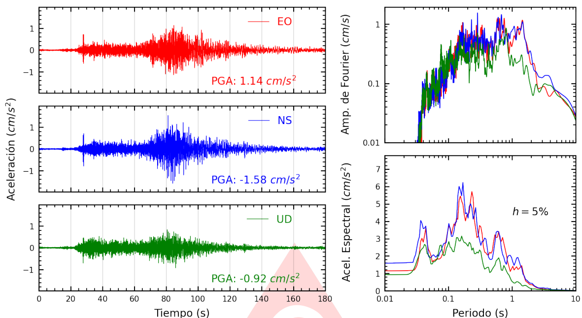
Figura A.29: Registros tiempo-historia, espectros de Fourier y de respuesta en las direcciones EO, NS y vertical de la estación PRADO. Sismo de Puquio, Lucanas - Ayacucho del 2025-05-17, 05:22:14 (Hora local)
