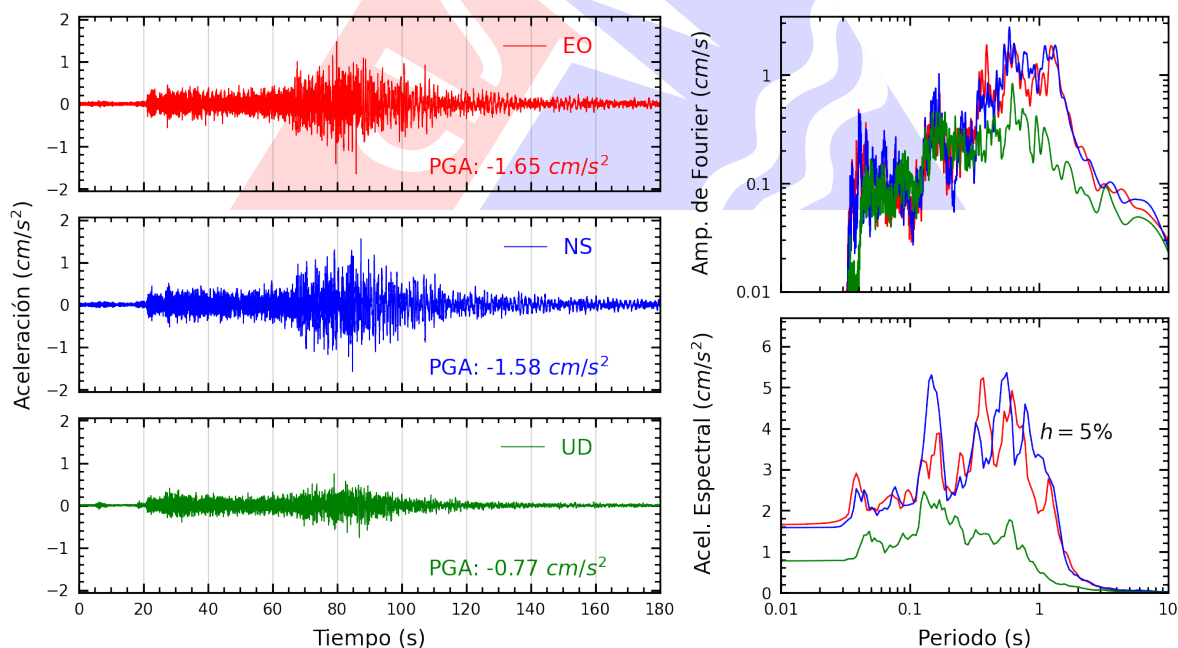
Figura A.26: Registros tiempo-historia, espectros de Fourier y de respuesta en las direcciones EO, NS y vertical de la estación DHNPE. Sismo de Puquio, Lucanas - Ayacucho del 2025-05-17, 05:22:14 (Hora local)
