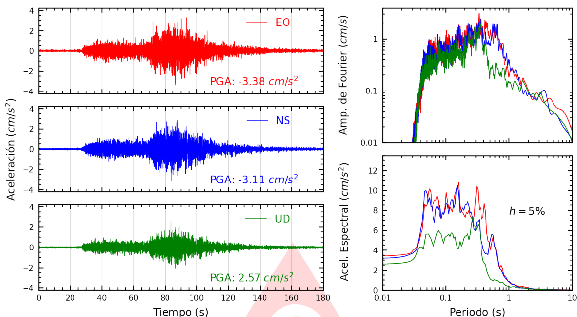
Figura A.7: Registros tiempo-historia, espectros de Fourier y de respuesta en las direcciones EO, NS y vertical de la estación UNTEL. Sismo de Puquío, Lucanas - Ayacucho del 2025-05-17, 05:22:14 (Hora local)
