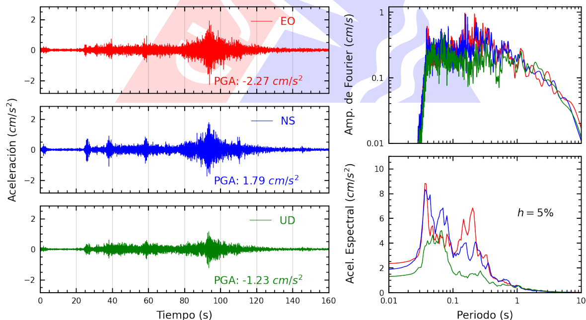
Figura A.16: Registros tiempo-historia, espectros de Fourier y de respuesta en las direcciones EO, NS y vertical de la estación PACHA. Sismo de Puquio, Lucanas - Ayacucho del 2025-05-17, 05:22:14 (Hora local)
