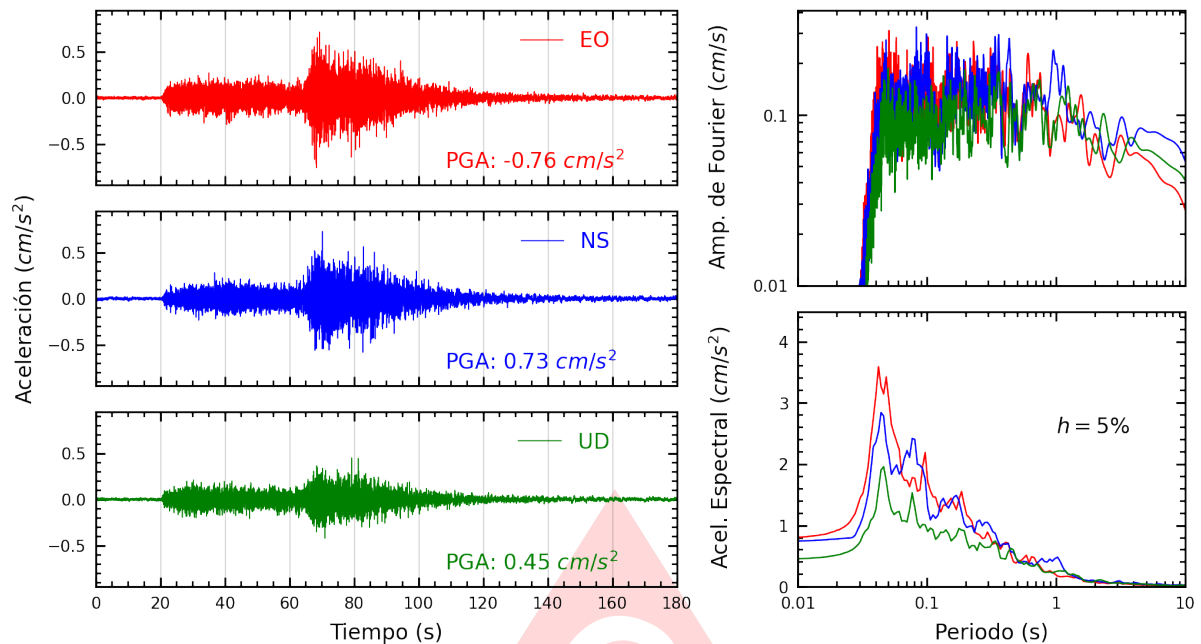
Figura A.49: Registros tiempo-historia, espectros de Fourier y de respuesta en las direcciones EO, NS y vertical de la estación UCSS. Sismo de Puquío, Lucanas - Ayacucho del 2025-05-17, 05:22:14 (Hora local)
