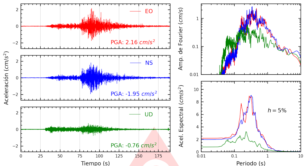
Figura A.19: Registros tiempo-historia, espectros de Fourier y de respuesta en las direcciones EO, NS y vertical de la estación ACAPU. Sismo de Puquio, Lucanas - Ayacucho del 2025-05-17, 05:22:14 (Hora local)
