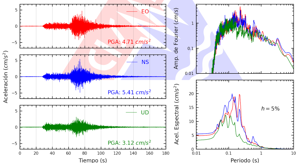
Figura A.2: Registros tiempo-historia, espectros de Fourier y de respuesta en las direcciones EO, NS y vertical de la estación ASIA. Sismo de Puquío, Lucanas - Ayacucho del 2025-05-17, 05:22:14 (Hora local)
