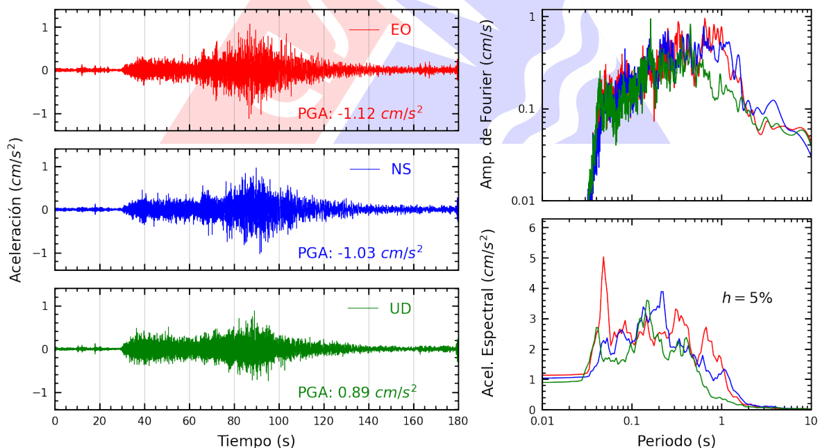
Figura A.40: Registros tiempo-historia, espectros de Fourier y de respuesta en las direcciones EO, NS y vertical de la estación UPCS. Sismo de Puquio, Lucanas - Ayacucho del 2025-05-17, 05:22:14 (Hora local)
