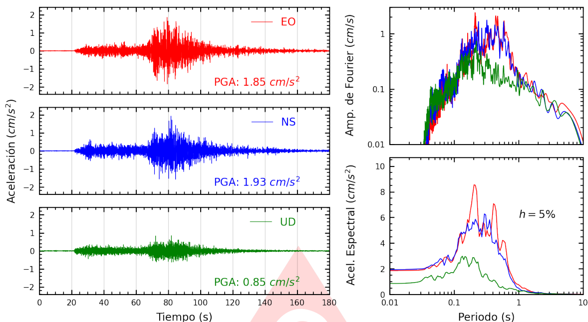
Figura A.23: Registros tiempo-historia, espectros de Fourier y de respuesta en las direcciones EO, NS y vertical de la estación VHAY2. Sismo de Puquio, Lucanas - Ayacucho del 2025-05-17, 05:22:14 (Hora local)
