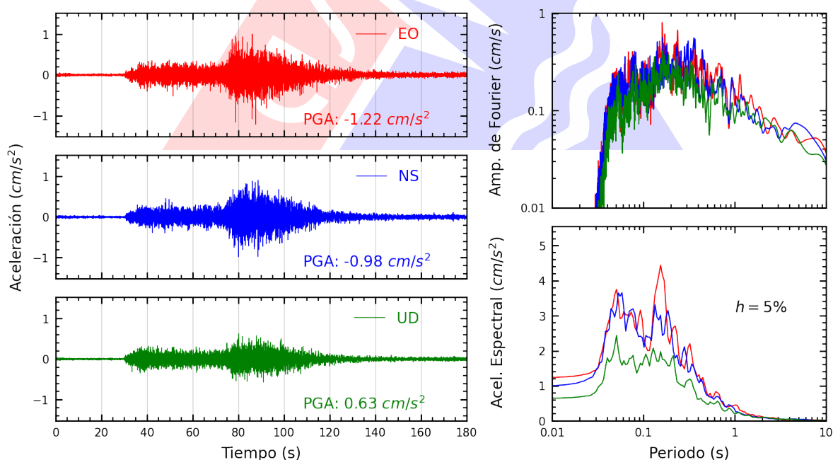
Figura A.38: Registros tiempo-historia, espectros de Fourier y de respuesta en las direcciones EO, NS y vertical de la estación FICPE. Sismo de Puquio, Lucanas - Ayacucho del 2025-05-17, 05:22:14 (Hora local)
