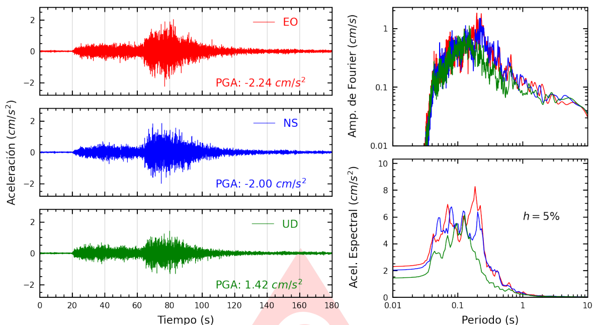
Figura A.17: Registros tiempo-historia, espectros de Fourier y de respuesta en las direcciones EO, NS y vertical de la estación INDEP. Sismo de Puquio, Lucanas - Ayacucho del 2025-05-17, 05:22:14 (Hora local)
