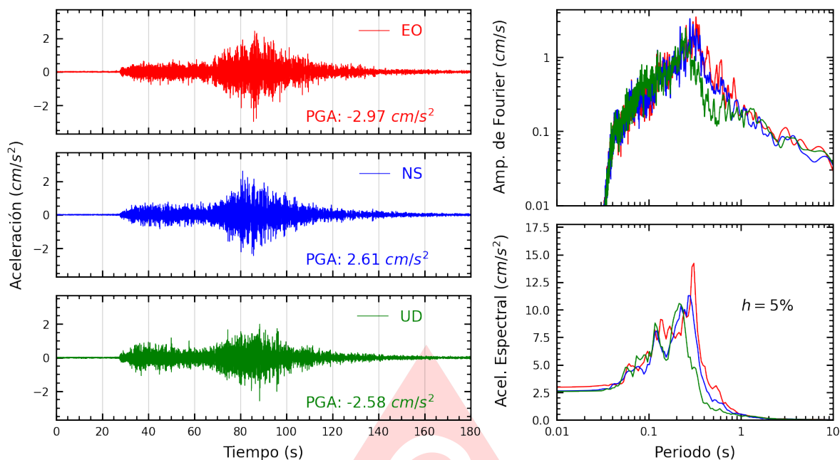
Figura A.9: Registros tiempo-historia, espectros de Fourier y de respuesta en las direcciones EO, NS y vertical de la estación SOVES. Sismo de Puquío, Lucanas - Ayacucho del 2025-05-17, 05:22:14 (Hora local)
