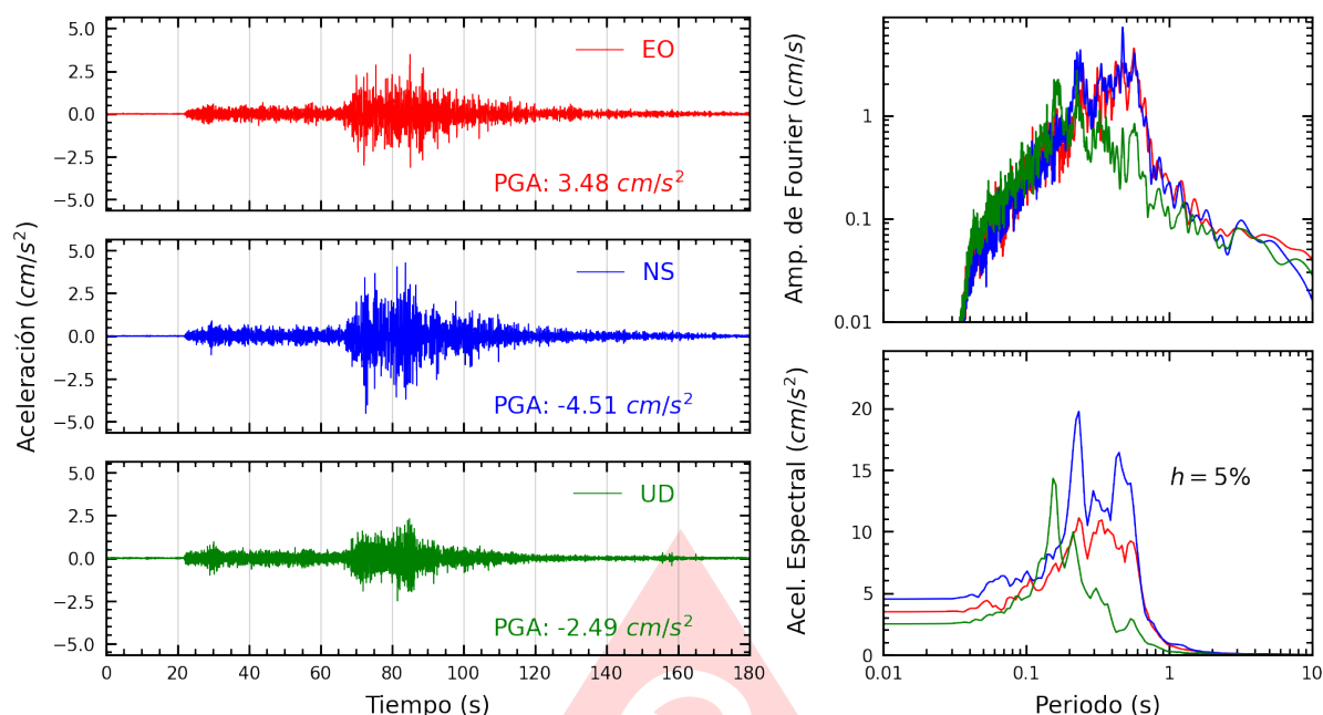
Figura A.3: Registros tiempo-historia, espectros de Fourier y de respuesta en las direcciones EO, NS y vertical de la estación MDPP. Sismo de Puquio, Lucanas - Ayacucho del 2025-05-17, 05:22:14 (Hora local)
