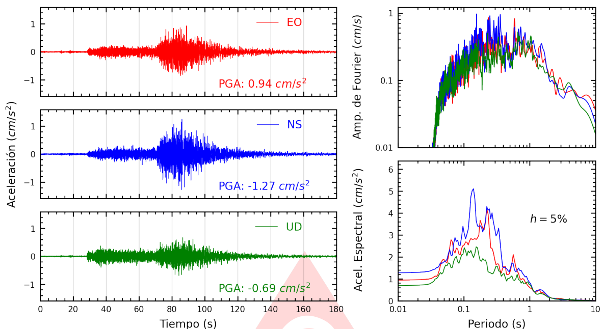
Figura A.35: Registros tiempo-historia, espectros de Fourier y de respuesta en las direcciones EO, NS y vertical de la estación SERVI. Sismo de Puquio, Lucanas - Ayacucho del 2025-05-17, 05:22:14 (Hora local)
