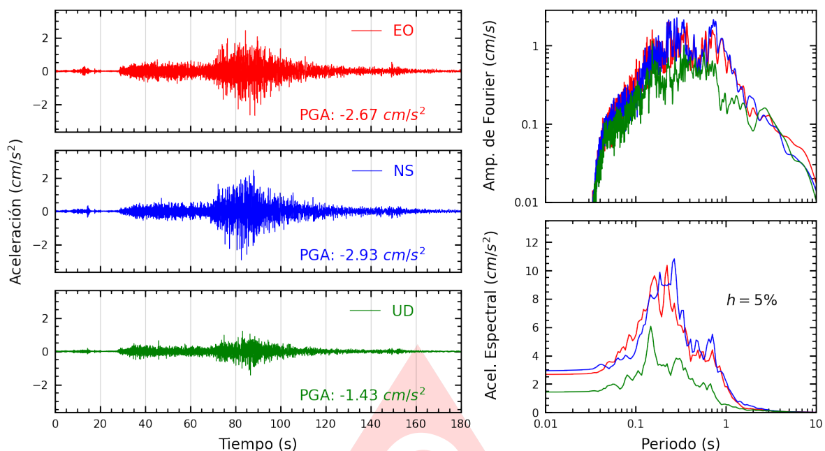
Figura A.11: Registros tiempo-historia, espectros de Fourier y de respuesta en las direcciones EO, NS y vertical de la estación BRISA. Sismo de Puquio, Lucanas - Ayacucho del 2025-05-17, 05:22:14 (Hora local)
