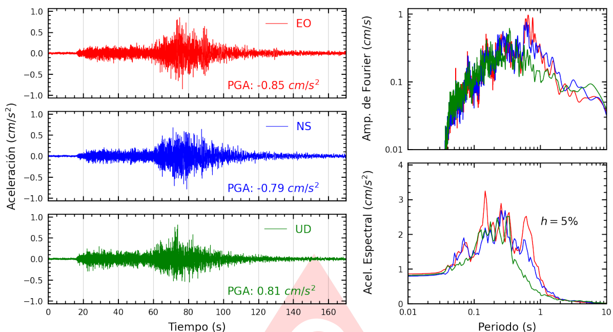
Figura A.47: Registros tiempo-historia, espectros de Fourier y de respuesta en las direcciones EO, NS y vertical de la estación UNMSM. Sismo de Puquio, Lucanas - Ayacucho del 2025-05-17, 05:22:14 (Hora local)
