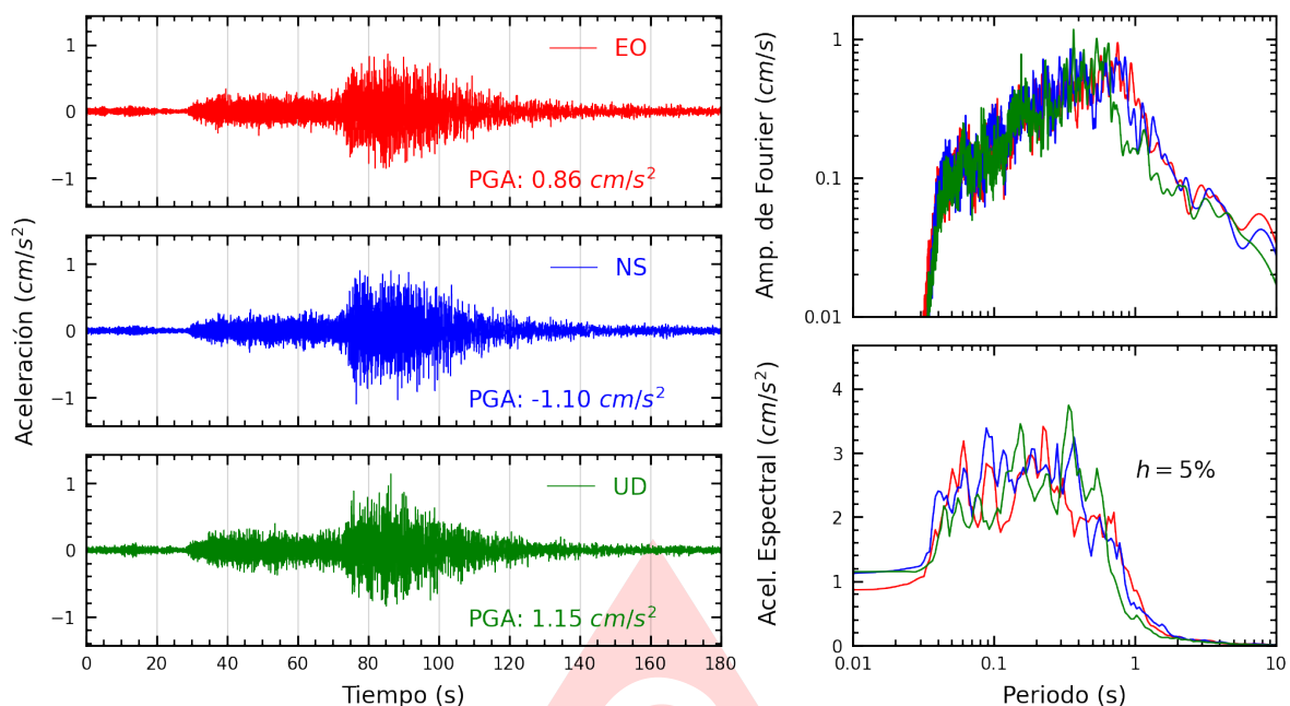
Figura A.39: Registros tiempo-historia, espectros de Fourier y de respuesta en las direcciones EO, NS y vertical de la estación IMCA. Sismo de Puquio, Lucanas - Ayacucho del 2025-05-17, 05:22:14 (Hora local)
