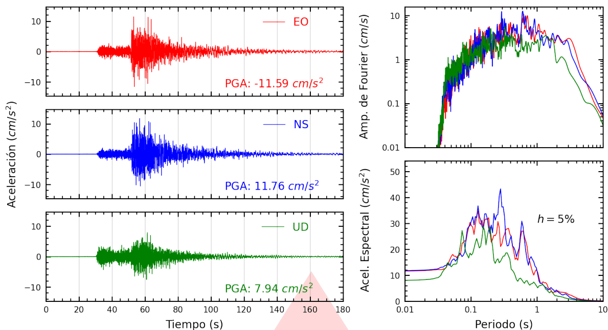
Figura A.1: Registros tiempo-historia, espectros de Fourier y de respuesta en las direcciones EO, NS y vertical de la estación UNICA. Sismo de Puquío, Lucanas - Ayacucho del 2025-05-17, 05:22:14 (Hora local)
