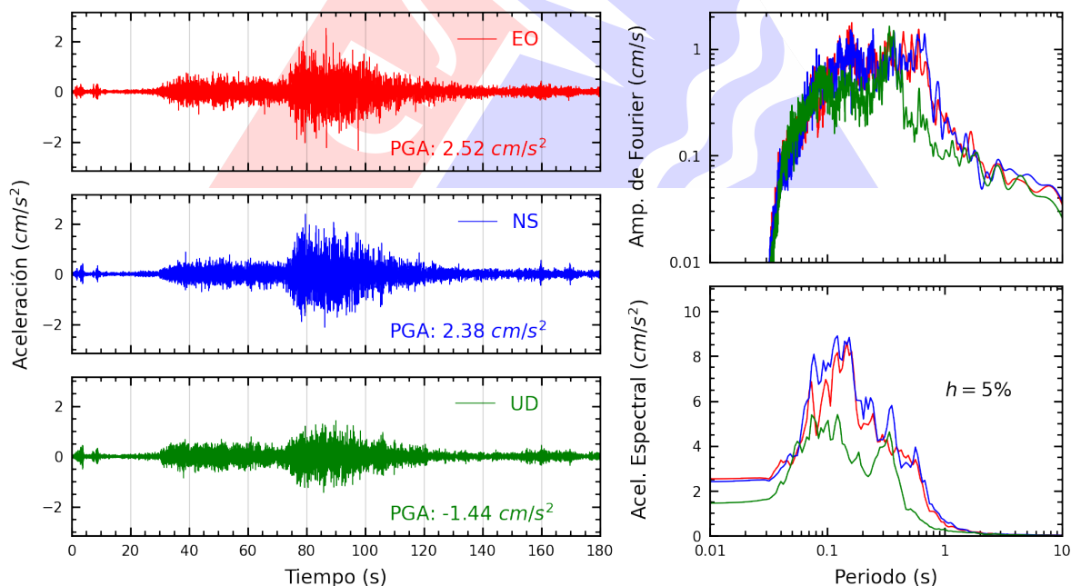
Figura A.14: Registros tiempo-historia, espectros de Fourier y de respuesta en las direcciones EO, NS y vertical de la estación SJLSV. Sismo de Puquío, Lucanas - Ayacucho del 2025-05-17, 05:22:14 (Hora local)
