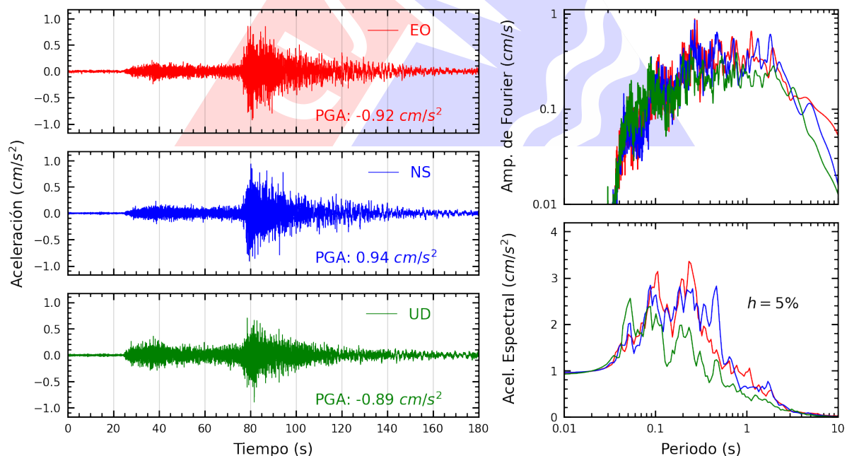
Figura A.44: Registros tiempo-historia, espectros de Fourier y de respuesta en las direcciones EO, NS y vertical de la estación UJBG3. Sismo de Puquio, Lucanas - Ayacucho del 2025-05-17, 05:22:14 (Hora local)
