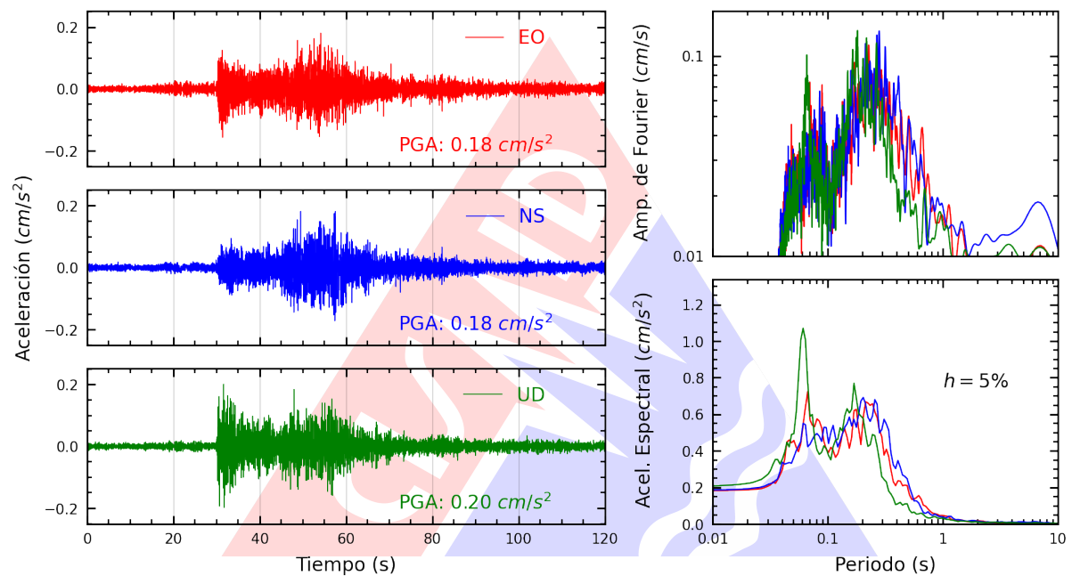
Figura A.5: Registros tiempo-historia, espectros de Fourier y de respuesta en las direcciones EO, NS y vertical de la estación CREY. Sismo de Ilo, Ilo - Moquegua del 2025-05-18, 18:57:57 (Hora local)
