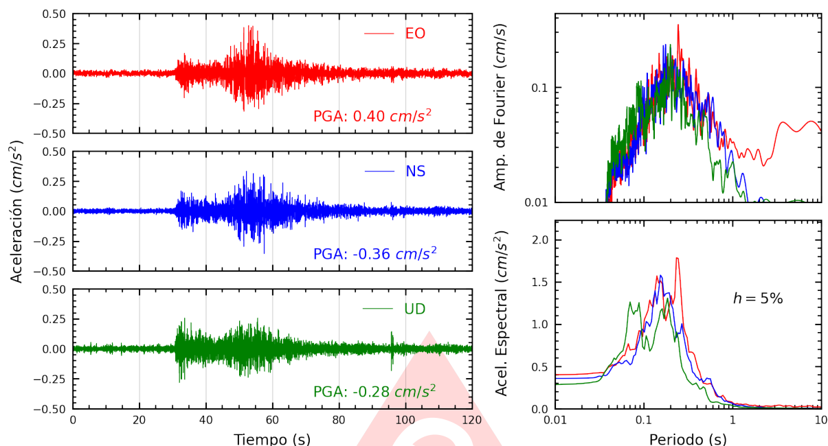
Figura A.3: Registros tiempo-historia, espectros de Fourier y de respuesta en las direcciones EO, NS y vertical de la estación UJBG3. Sismo de Ilo, Ilo - Moquegua del 2025-05-18, 18:57:57 (Hora local)
