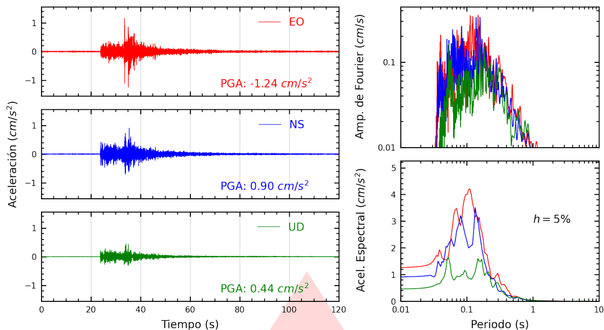
Figura A.1: Registros tiempo-historia, espectros de Fourier y de respuesta en las direcciones EO, NS y vertical de la estación UNAM. Sismo de Ilo, Ilo - Moquegua del 2025-05-18, 18:57:57 (Hora local)
