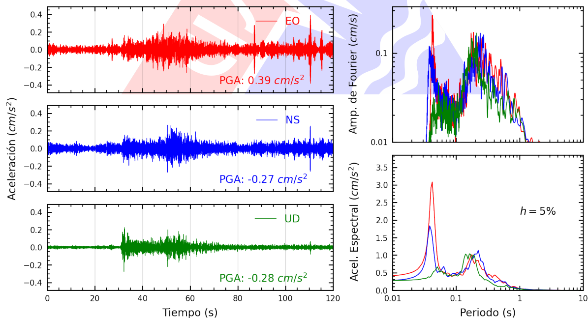
Figura A.4: Registros tiempo-historia, espectros de Fourier y de respuesta en las direcciones EO, NS y vertical de la estación UPTAC. Sismo de Ilo, Ilo - Moquegua del 2025-05-18, 18:57:57 (Hora local)
