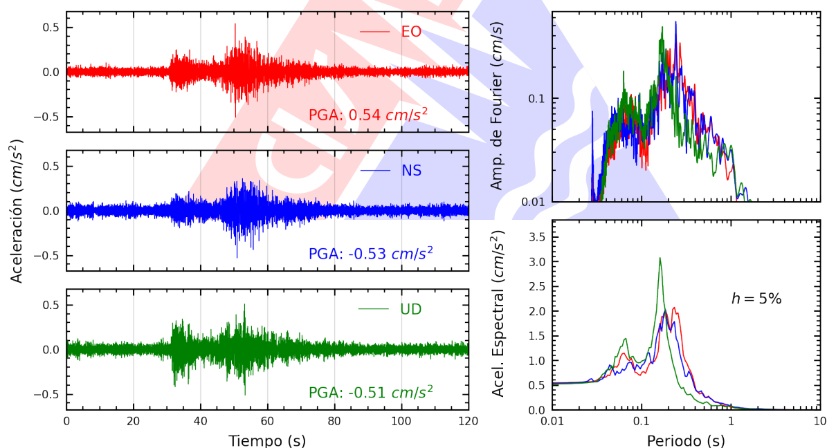
Figura A.2: Registros tiempo-historia, espectros de Fourier y de respuesta en las direcciones EO, NS y vertical de la estación UJBG4. Sismo de Ilo, Ilo - Moquegua del 2025-05-18, 18:57:57 (Hora local)
