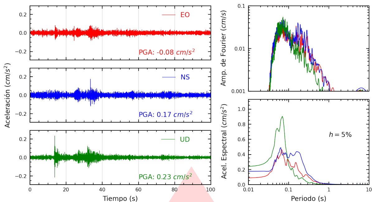
Figura A.1: Registros tiempo-historia, espectros de Fourier y de respuesta en las direcciones EO, NS y vertical de la estación UNAAA. Sismo de Barranca, Datem del Marañón - Loreto del 2025-05-19, 20:43:34 (Hora local)
