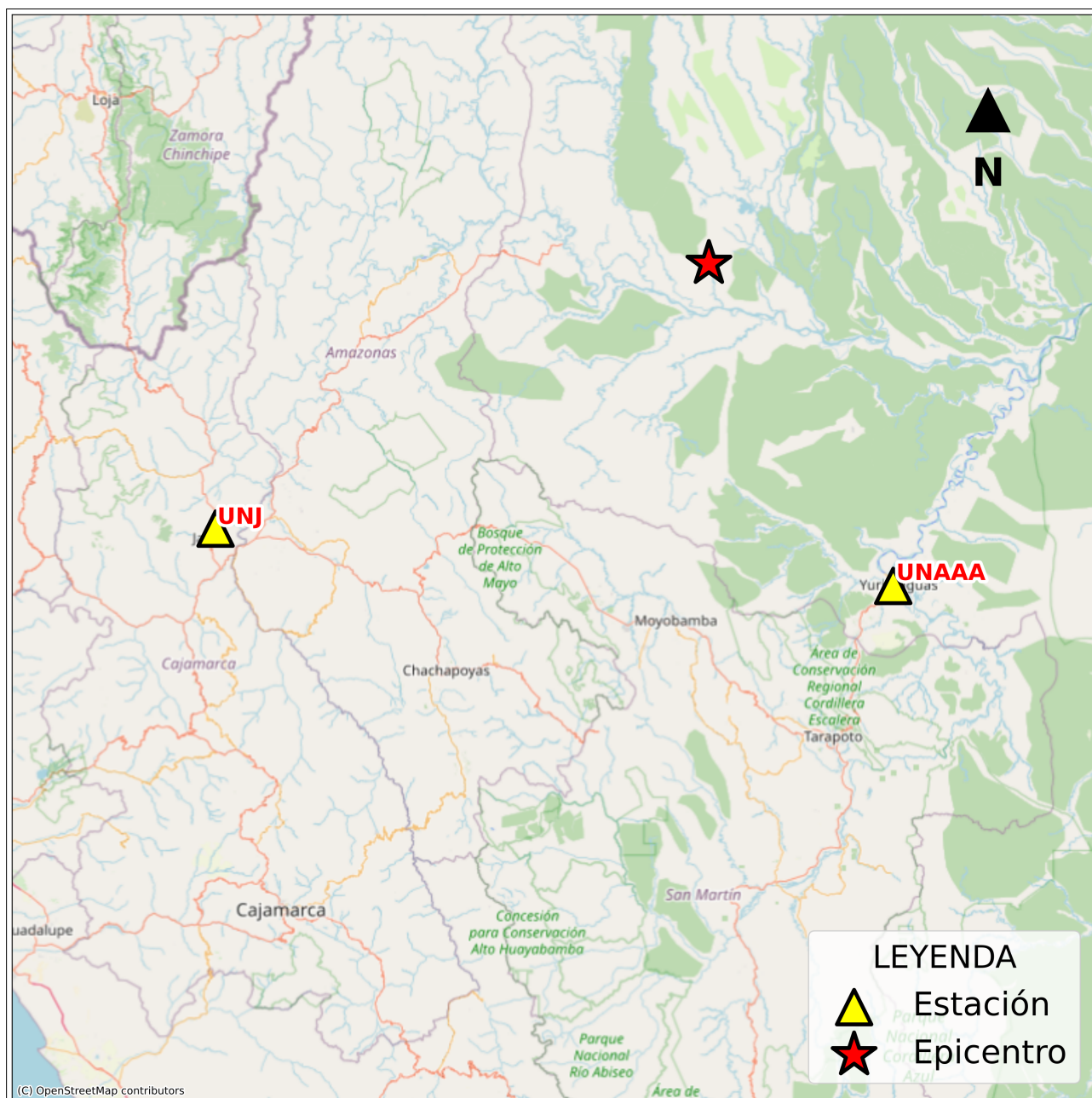
Figura 2: Mapa de ubicación de la(s) estación(es) acelerográfica(s) correspondiente(s) al Sismo de Barranca, Datem del Marañón - Loreto del 19 de mayo de 2025 a las 20:43:34 (hora local)
