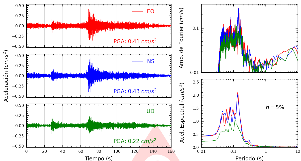
Figura A.17: Registros tiempo-historia, espectros de Fourier y de respuesta en las direcciones EO, NS y vertical de la estación FICPE. Sismo de Chimbote, Santa - Ancash del 2025-05-22, 06:13:11 (Hora local)
