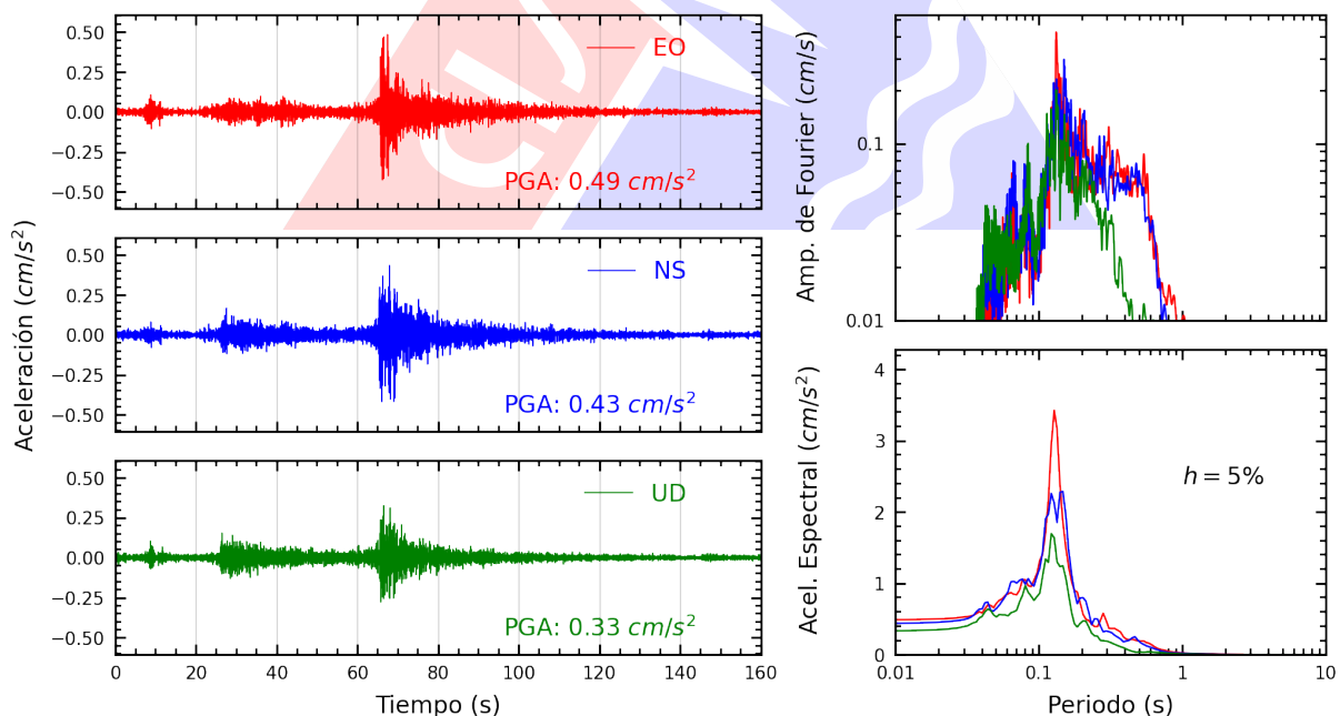
Figura A.14: Registros tiempo-historia, espectros de Fourier y de respuesta en las direcciones EO, NS y vertical de la estación VHAY2. Sismo de Chimbote, Santa - Ancash del 2025-05-22, 06:13:11 (Hora local)
