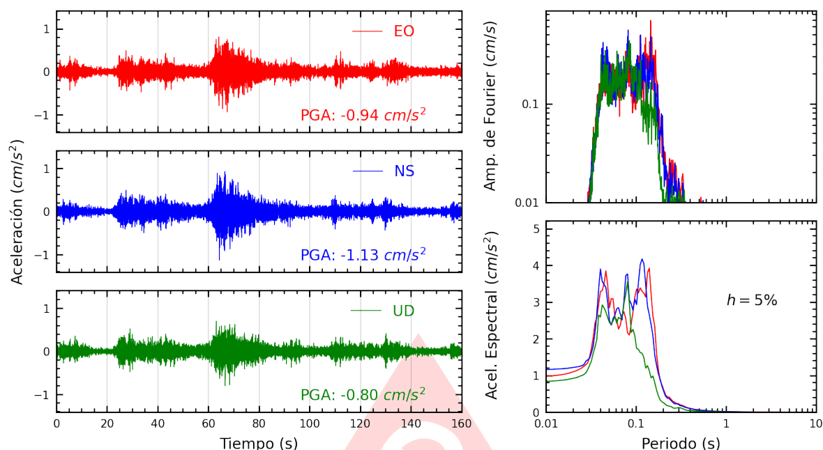
Figura A.5: Registros tiempo-historia, espectros de Fourier y de respuesta en las direcciones EO, NS y vertical de la estación SROS2. Sismo de Chimbote, Santa - Ancash del 2025-05-22, 06:13:11 (Hora local)
