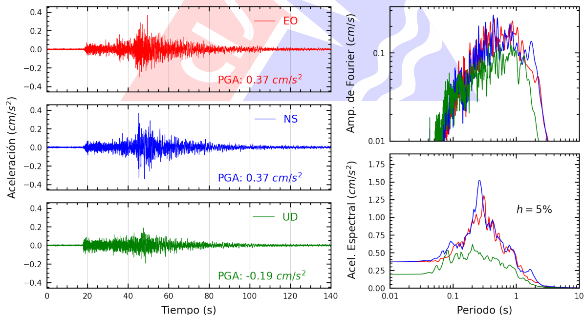
Figura A.20: Registros tiempo-historia, espectros de Fourier y de respuesta en las direcciones EO, NS y vertical de la estación UNC. Sismo de Chimbote, Santa - Ancash del 2025-05-22, 06:13:11 (Hora local)
