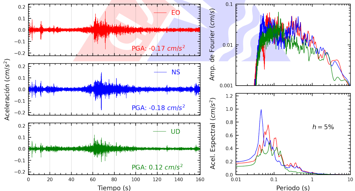
Figura A.34: Registros tiempo-historia, espectros de Fourier y de respuesta en las direcciones EO, NS y vertical de la estación UPAOP. Sismo de Chimbote, Santa - Ancash del 2025-05-22, 06:13:11 (Hora local)
