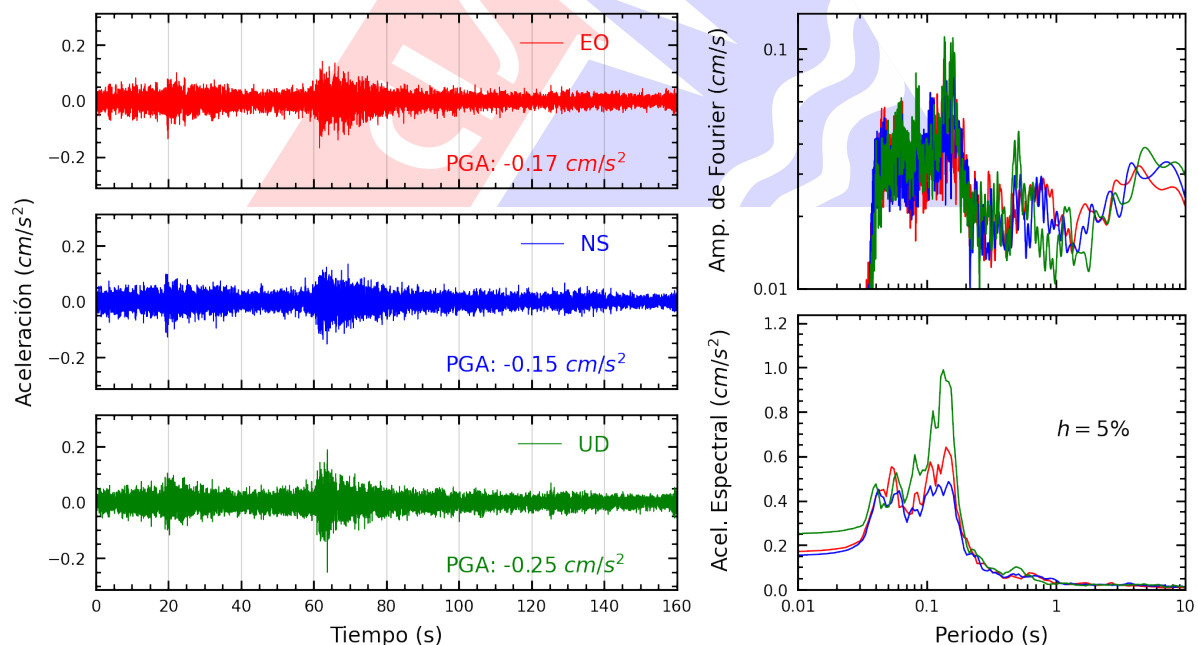
Figura A.26: Registros tiempo-historia, espectros de Fourier y de respuesta en las direcciones EO, NS y vertical de la estación IMCA. Sismo de Chimbote, Santa - Ancash del 2025-05-22, 06:13:11 (Hora local)
