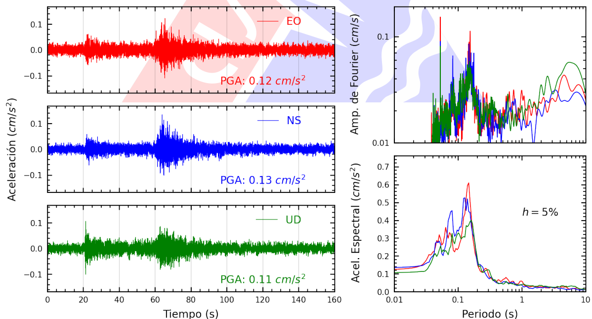
Figura A.36: Registros tiempo-historia, espectros de Fourier y de respuesta en las direcciones EO, NS y vertical de la estación UNMSM. Sismo de Chimbote, Santa - Ancash del 2025-05-22, 06:13:11 (Hora local)
