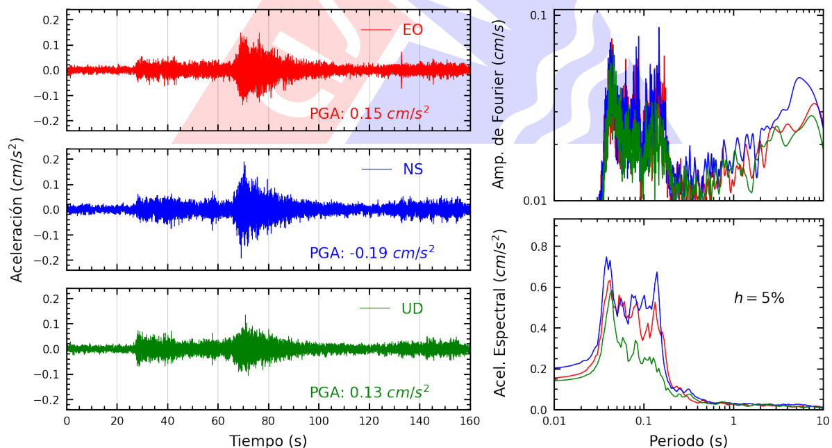
Figura A.32: Registros tiempo-historia, espectros de Fourier y de respuesta en las direcciones EO, NS y vertical de la estación SJLCE. Sismo de Chimbote, Santa - Ancash del 2025-05-22, 06:13:11 (Hora local)
