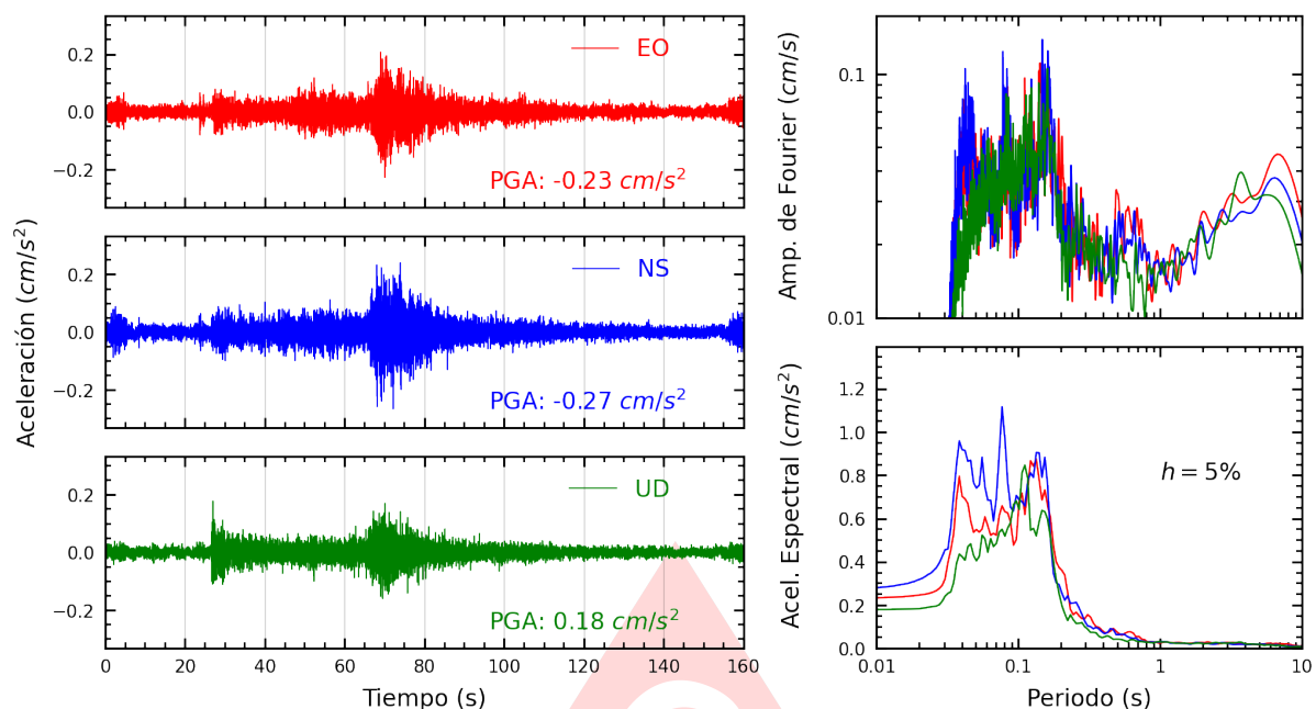
Figura A.23: Registros tiempo-historia, espectros de Fourier y de respuesta en las direcciones EO, NS y vertical de la estación COMAS. Sismo de Chimbote, Santa - Ancash del 2025-05-22, 06:13:11 (Hora local)
