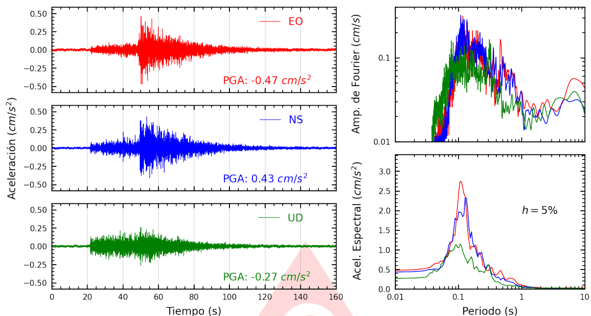
Figura A.15: Registros tiempo-historia, espectros de Fourier y de respuesta en las direcciones EO, NS y vertical de la estación UCVCH. Sismo de Chimbote, Santa - Ancash del 2025-05-22, 06:13:11 (Hora local)
