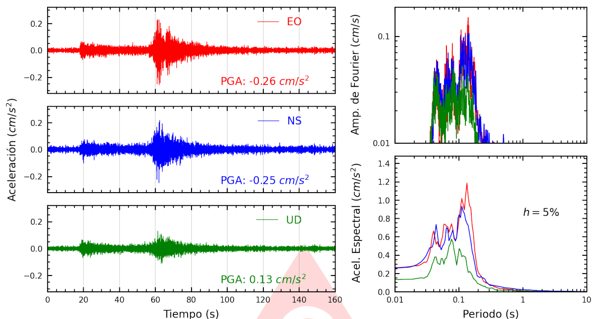
Figura A.25: Registros tiempo-historia, espectros de Fourier y de respuesta en las direcciones EO, NS y vertical de la estación ATARJ. Sismo de Chimbote, Santa - Ancash del 2025-05-22, 06:13:11 (Hora local)
