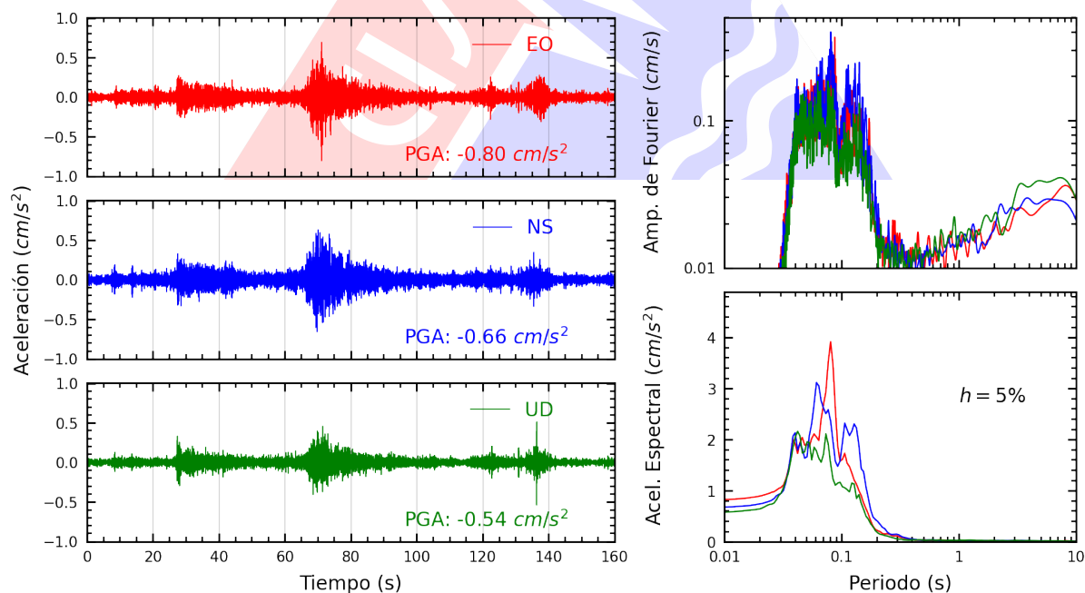
Figura A.8: Registros tiempo-historia, espectros de Fourier y de respuesta en las direcciones EO, NS y vertical de la estación JOSEO. Sismo de Chimbote, Santa - Ancash del 2025-05-22, 06:13:11 (Hora local)
