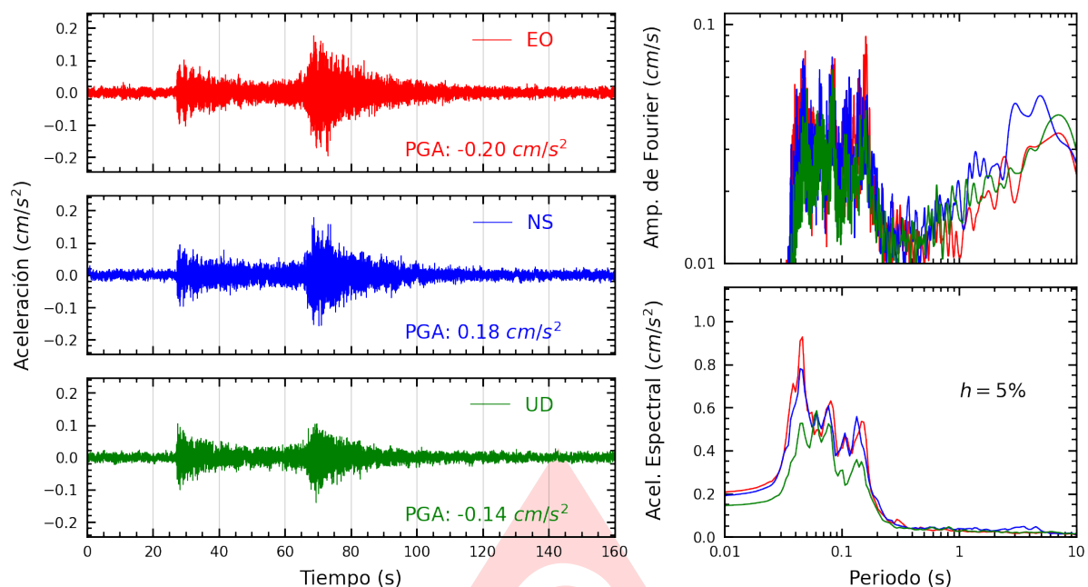
Figura A.31: Registros tiempo-historia, espectros de Fourier y de respuesta en las direcciones EO, NS y vertical de la estación UCSS. Sismo de Chimbote, Santa - Ancash del 2025-05-22, 06:13:11 (Hora local)
