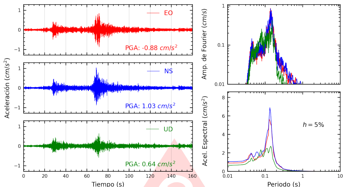
Figura A.7: Registros tiempo-historia, espectros de Fourier y de respuesta en las direcciones EO, NS y vertical de la estación CARA2. Sismo de Chimbote, Santa - Ancash del 2025-05-22, 06:13:11 (Hora local)
