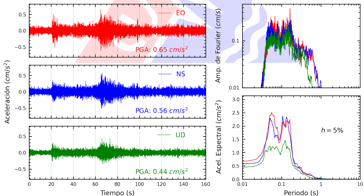
Figura A.12: Registros tiempo-historia, espectros de Fourier y de respuesta en las direcciones EO, NS y vertical de la estación UNTEL. Sismo de Chimbote, Santa - Ancash del 2025-05-22, 06:13:11 (Hora local)
