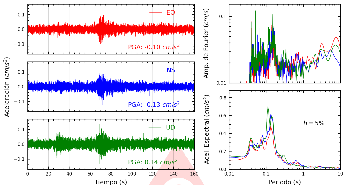
Figura A.35: Registros tiempo-historia, espectros de Fourier y de respuesta en las direcciones EO, NS y vertical de la estación BONDY. Sismo de Chimbote, Santa - Ancash del 2025-05-22, 06:13:11 (Hora local)
