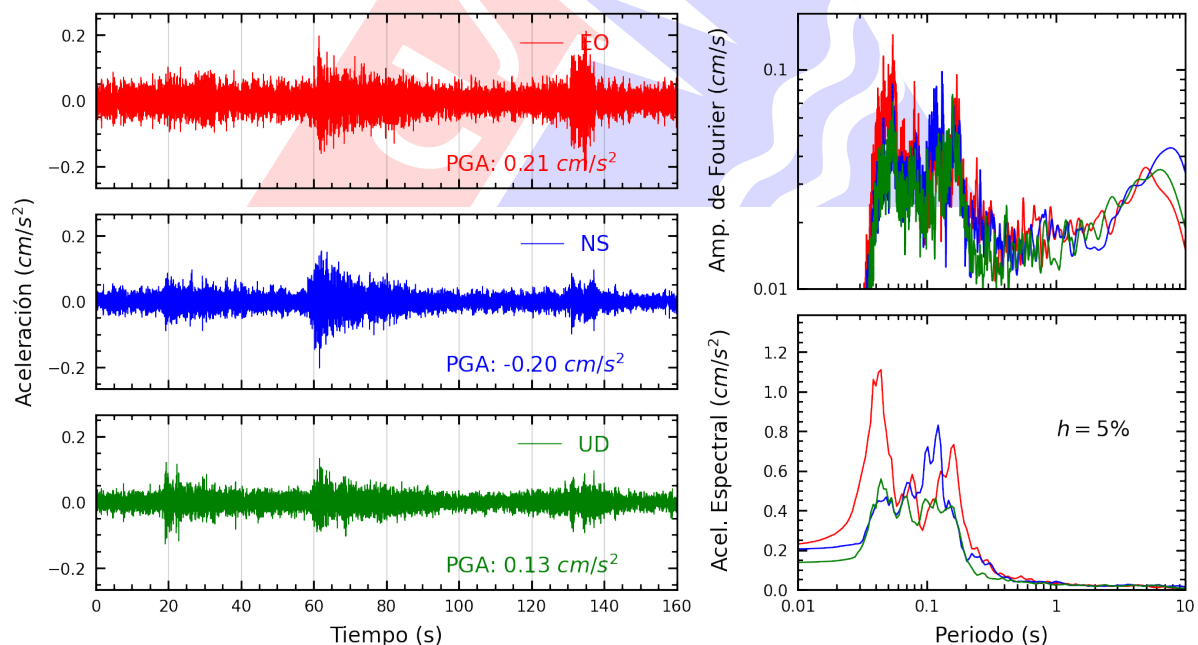
Figura A.28: Registros tiempo-historia, espectros de Fourier y de respuesta en las direcciones EO, NS y vertical de la estación INICT. Sismo de Chimbote, Santa - Ancash del 2025-05-22, 06:13:11 (Hora local)
