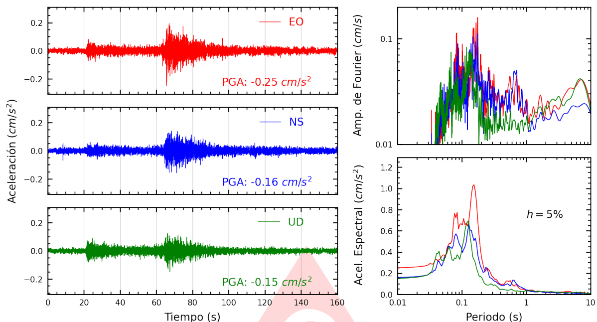
Figura A.27: Registros tiempo-historia, espectros de Fourier y de respuesta en las direcciones EO, NS y vertical de la estación USILP. Sismo de Chimbote, Santa - Ancash del 2025-05-22, 06:13:11 (Hora local)
