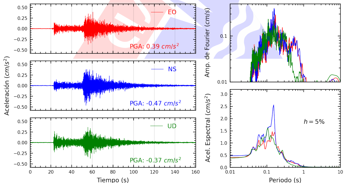
Figura A.16: Registros tiempo-historia, espectros de Fourier y de respuesta en las direcciones EO, NS y vertical de la estación CARAL. Sismo de Chimbote, Santa - Ancash del 2025-05-22, 06:13:11 (Hora local)
