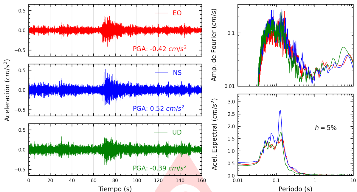
Figura A.13: Registros tiempo-historia, espectros de Fourier y de respuesta en las direcciones EO, NS y vertical de la estación SJLSC. Sismo de Chimbote, Santa - Ancash del 2025-05-22, 06:13:11 (Hora local)
