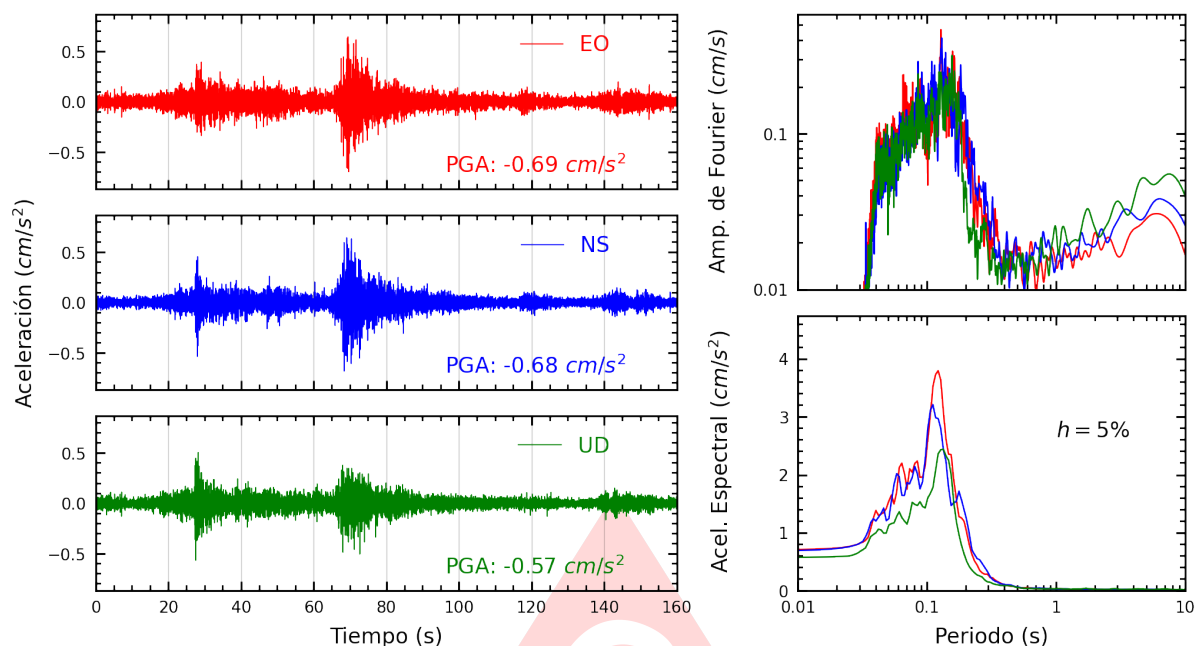
Figura A.11: Registros tiempo-historia, espectros de Fourier y de respuesta en las direcciones EO, NS y vertical de la estación INDEP. Sismo de Chimbote, Santa - Ancash del 2025-05-22, 06:13:11 (Hora local)
