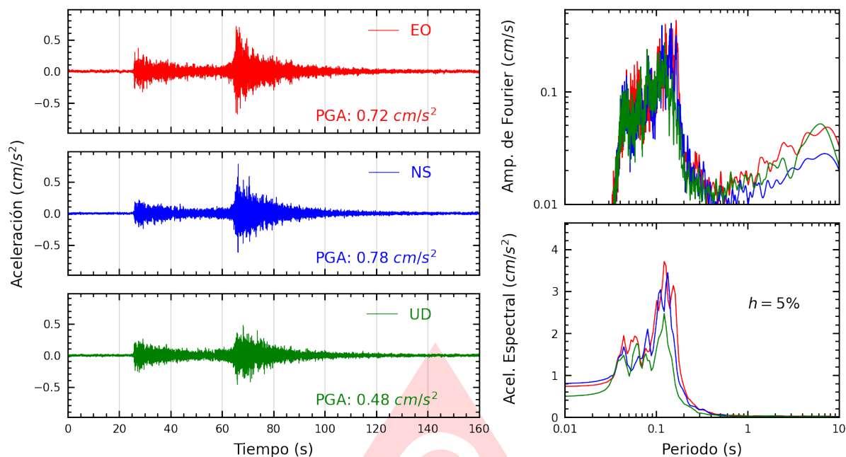
Figura A.9: Registros tiempo-historia, espectros de Fourier y de respuesta en las direcciones EO, NS y vertical de la estación AMORE. Sismo de Chimbote, Santa - Ancash del 2025-05-22, 06:13:11 (Hora local)
