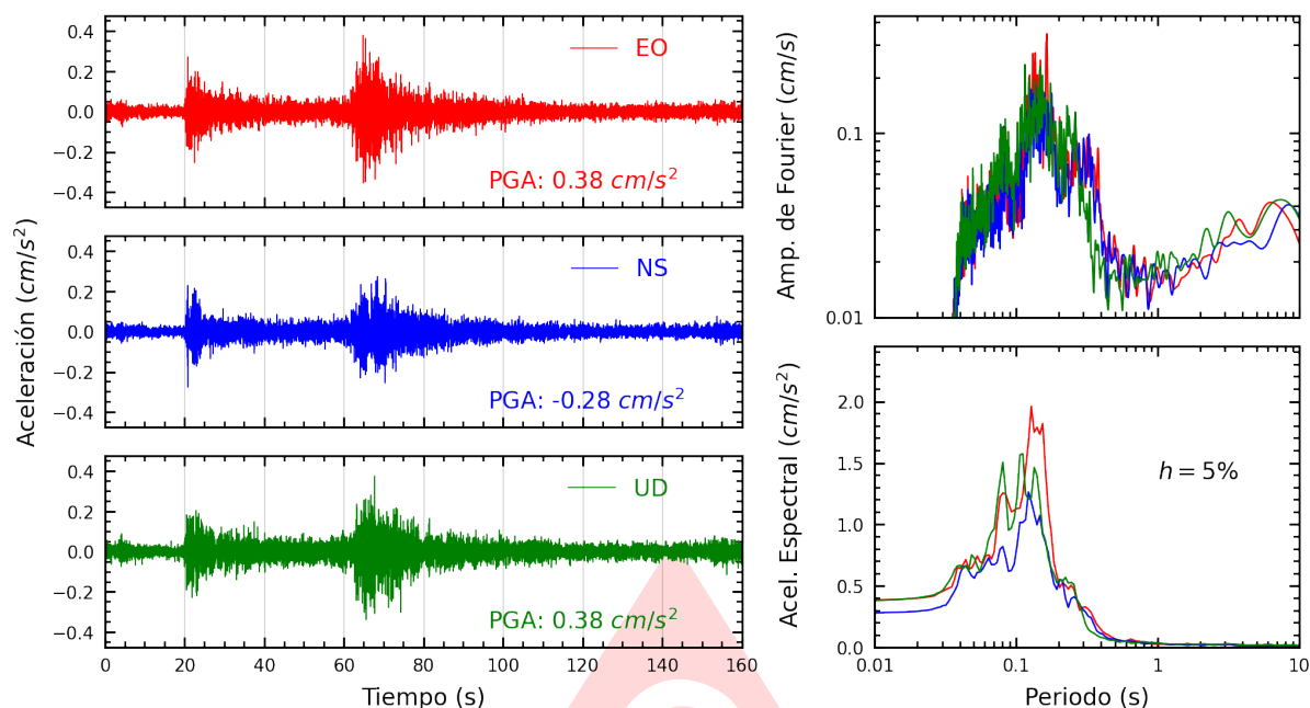
Figura A.19: Registros tiempo-historia, espectros de Fourier y de respuesta en las direcciones EO, NS y vertical de la estación SOVES. Sismo de Chimbote, Santa - Ancash del 2025-05-22, 06:13:11 (Hora local)
