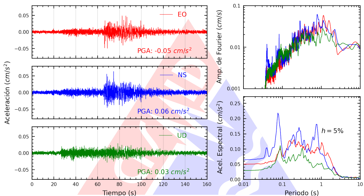
Figura A.37: Registros tiempo-historia, espectros de Fourier y de respuesta en las direcciones EO, NS y vertical de la estación UNJ. Sismo de Chimbote, Santa - Ancash del 2025-05-22, 06:13:11 (Hora local)
