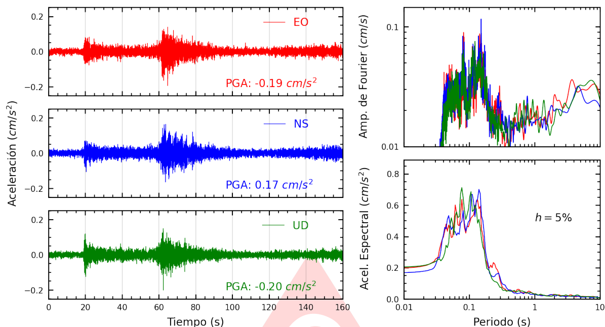
Figura A.29: Registros tiempo-historia, espectros de Fourier y de respuesta en las direcciones EO, NS y vertical de la estación SERVI. Sismo de Chimbote, Santa - Ancash del 2025-05-22, 06:13:11 (Hora local)
