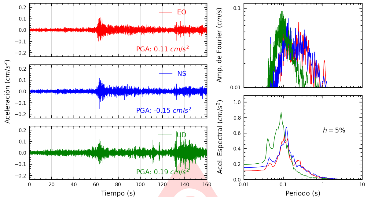
Figura A.33: Registros tiempo-historia, espectros de Fourier y de respuesta en las direcciones EO, NS y vertical de la estación UNP. Sismo de Chimbote, Santa - Ancash del 2025-05-22, 06:13:11 (Hora local)
