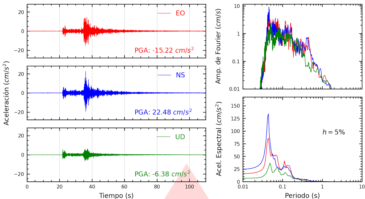
Figura A.1: Registros tiempo-historia, espectros de Fourier y de respuesta en las direcciones EO, NS y vertical de la estación SCTRU. Sismo de Chimbote, Santa - Ancash del 2025-05-22, 06:13:11 (Hora local)
