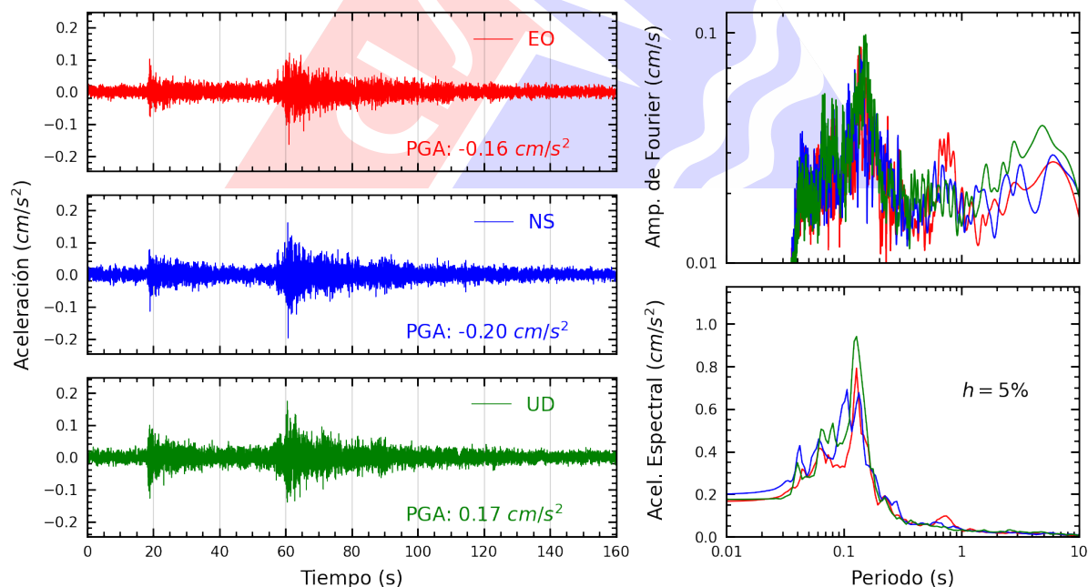
Figura A.30: Registros tiempo-historia, espectros de Fourier y de respuesta en las direcciones EO, NS y vertical de la estación UNFV. Sismo de Chimbote, Santa - Ancash del 2025-05-22, 06:13:11 (Hora local)
