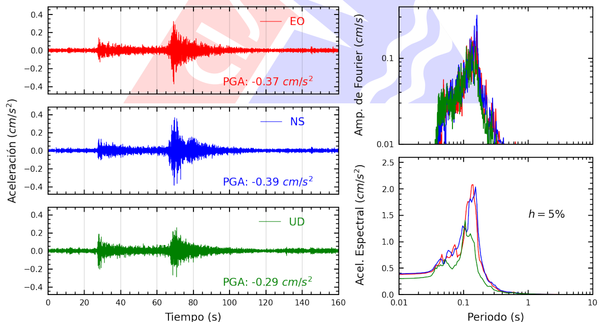
Figura A.18: Registros tiempo-historia, espectros de Fourier y de respuesta en las direcciones EO, NS y vertical de la estación JALV2. Sismo de Chimbote, Santa - Ancash del 2025-05-22, 06:13:11 (Hora local)
