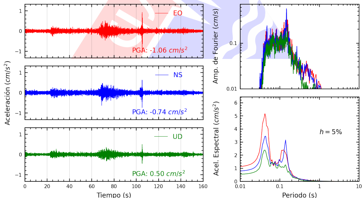
Figura A.6: Registros tiempo-historia, espectros de Fourier y de respuesta en las direcciones EO, NS y vertical de la estación PHER2. Sismo de Chimbote, Santa - Ancash del 2025-05-22, 06:13:11 (Hora local)
