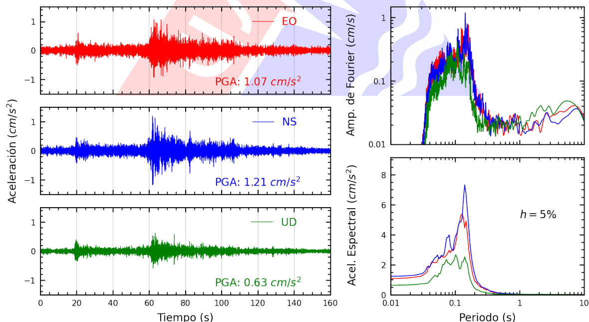
Figura A.4: Registros tiempo-historia, espectros de Fourier y de respuesta en las direcciones EO, NS y vertical de la estación USILM. Sismo de Chimbote, Santa - Ancash del 2025-05-22, 06:13:11 (Hora local)
