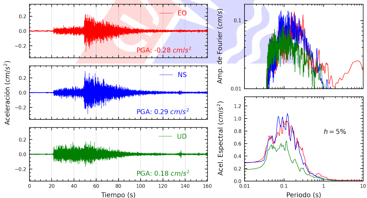
Figura A.22: Registros tiempo-historia, espectros de Fourier y de respuesta en las direcciones EO, NS y vertical de la estación SCCHI. Sismo de Chimbote, Santa - Ancash del 2025-05-22, 06:13:11 (Hora local)
