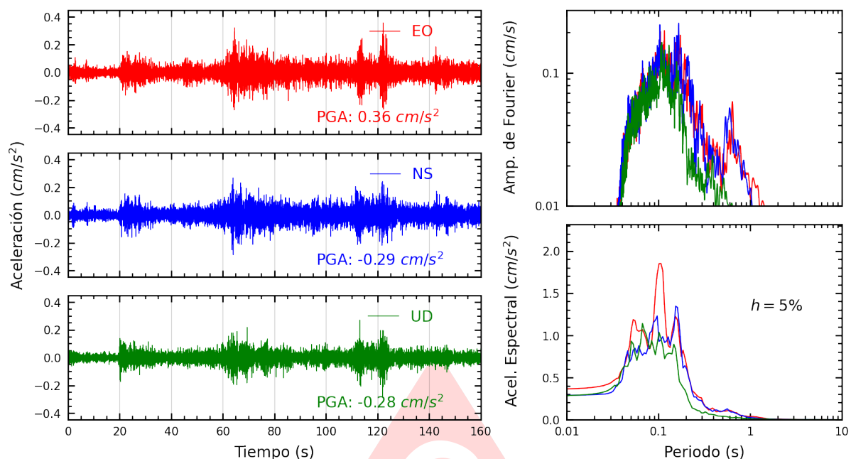
Figura A.21: Registros tiempo-historia, espectros de Fourier y de respuesta en las direcciones EO, NS y vertical de la estación SCCHO. Sismo de Chimbote, Santa - Ancash del 2025-05-22, 06:13:11 (Hora local)
