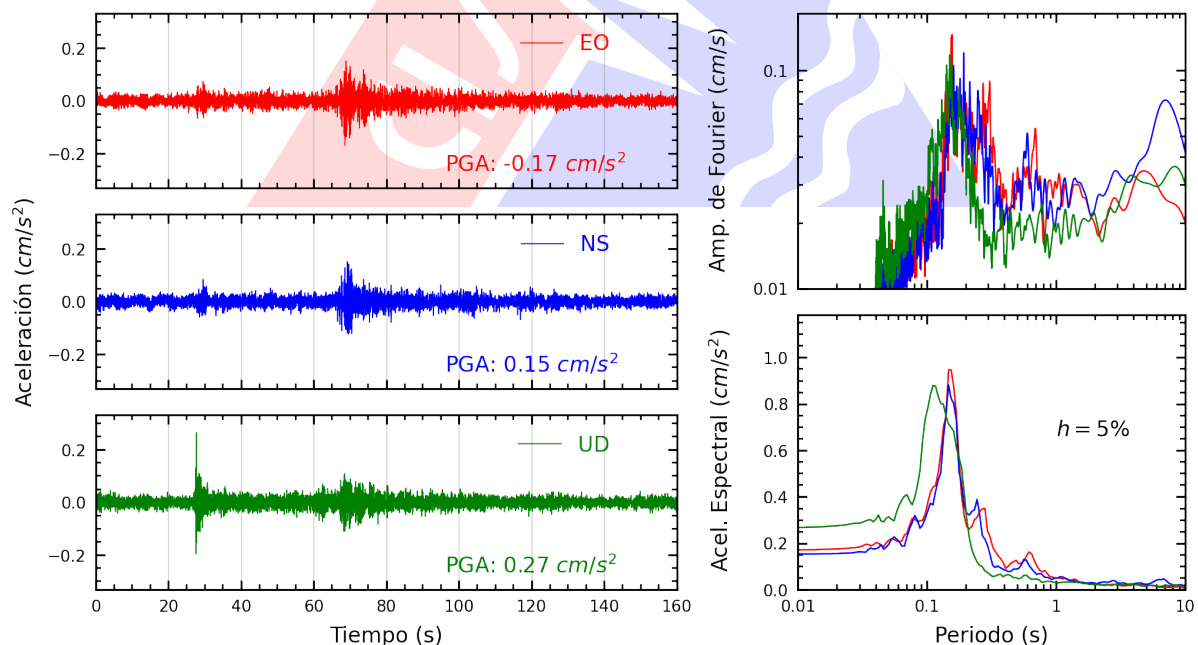
Figura A.24: Registros tiempo-historia, espectros de Fourier y de respuesta en las direcciones EO, NS y vertical de la estación DSMI. Sismo de Chimbote, Santa - Ancash del 2025-05-22, 06:13:11 (Hora local)
