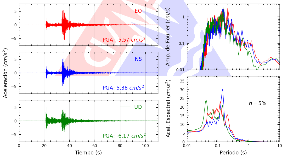
Figura A.2: Registros tiempo-historia, espectros de Fourier y de respuesta en las direcciones EO, NS y vertical de la estación UPAOT. Sismo de Chimbote, Santa - Ancash del 2025-05-22, 06:13:11 (Hora local)
