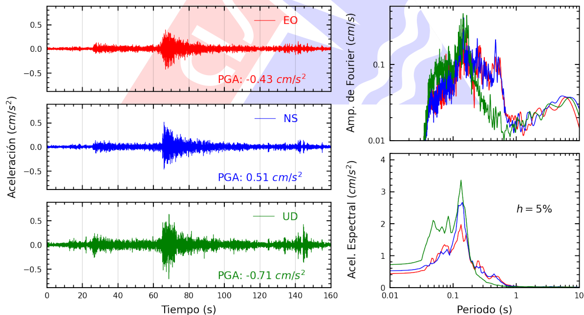
Figura A.10: Registros tiempo-historia, espectros de Fourier y de respuesta en las direcciones EO, NS y vertical de la estación MDPP. Sismo de Chimbote, Santa - Ancash del 2025-05-22, 06:13:11 (Hora local)
