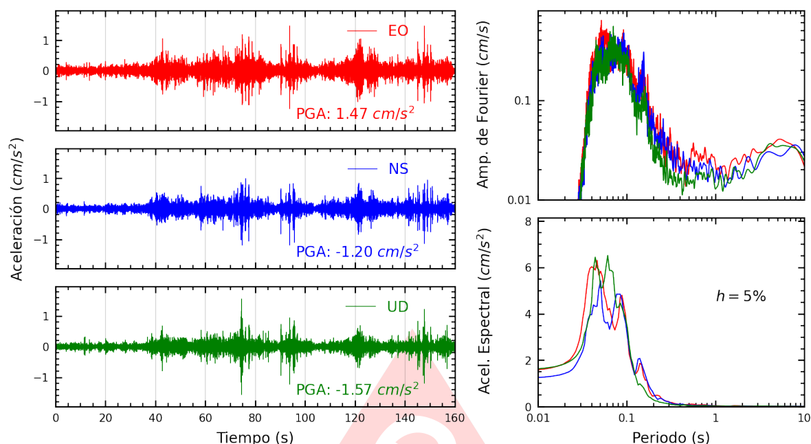
Figura A.3: Registros tiempo-historia, espectros de Fourier y de respuesta en las direcciones EO, NS y vertical de la estación SOBAR. Sismo de Chimbote, Santa - Ancash del 2025-05-22, 06:13:11 (Hora local)
