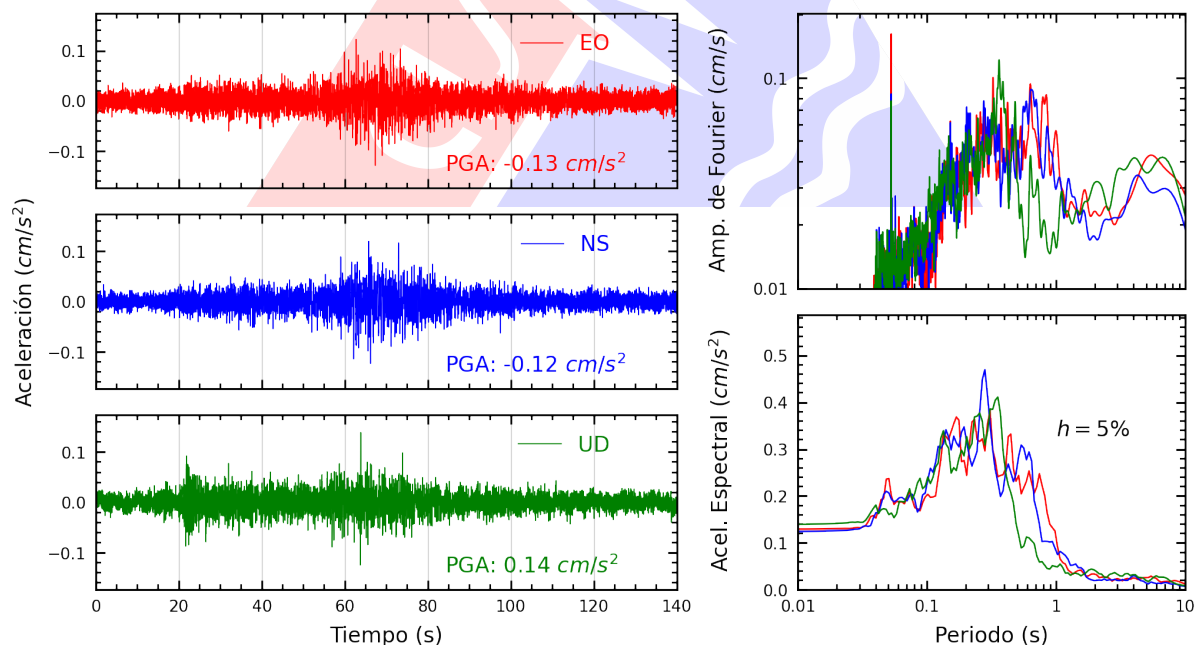
Figura A.18: Registros tiempo-historia, espectros de Fourier y de respuesta en las direcciones EO, NS y vertical de la estación UNMSM. Sismo de Puerto Inca, Puerto Inca - Huanuco del 2025-05-22, 14:57:39 (Hora local)
