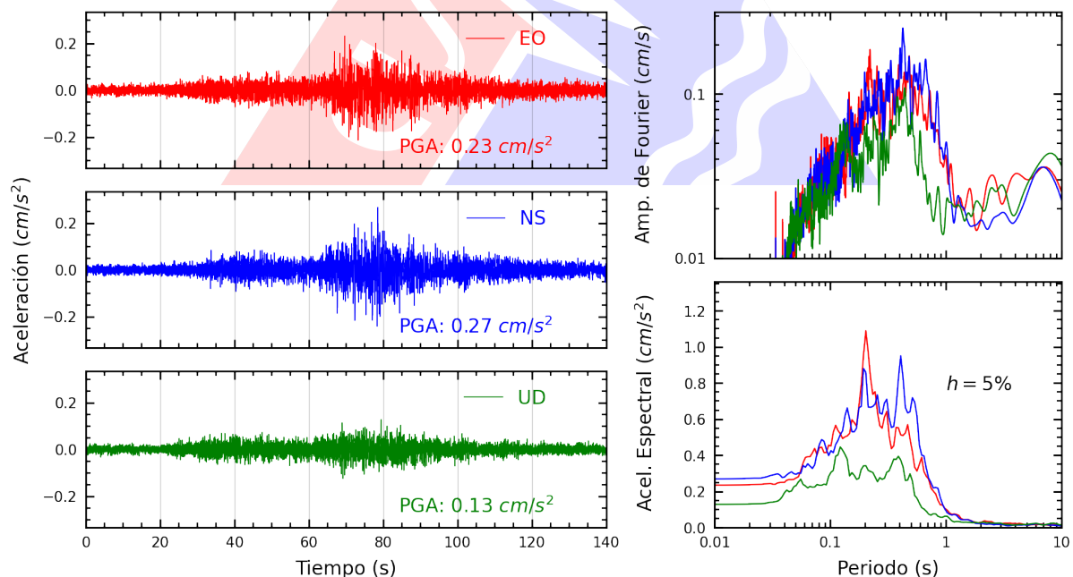
Figura A.12: Registros tiempo-historia, espectros de Fourier y de respuesta en las direcciones EO, NS y vertical de la estación USILP. Sismo de Puerto Inca, Puerto Inca - Huanuco del 2025-05-22, 14:57:39 (Hora local)
