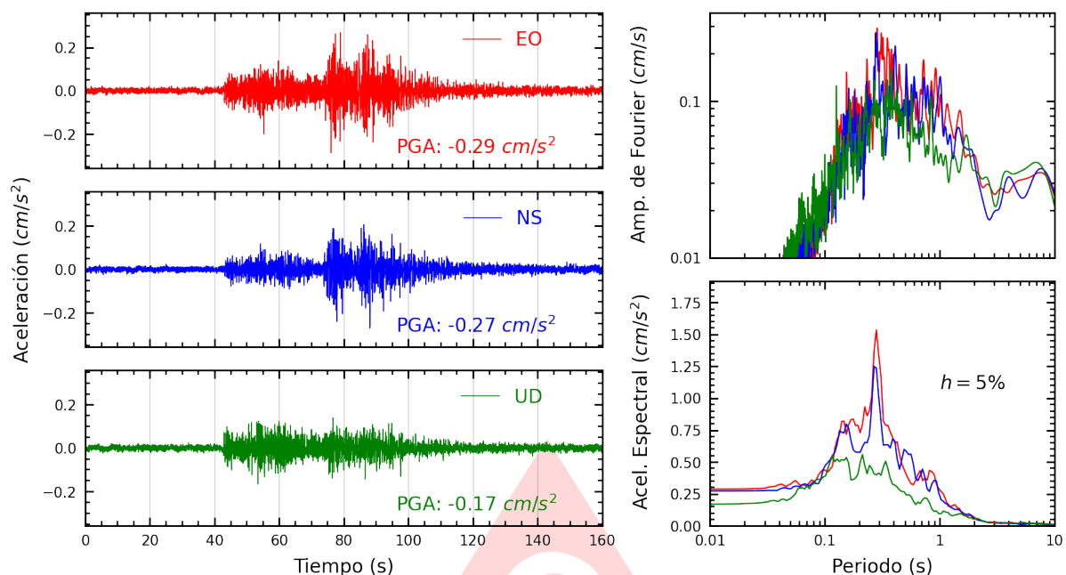
Figura A.11: Registros tiempo-historia, espectros de Fourier y de respuesta en las direcciones EO, NS y vertical de la estación UNASA. Sismo de Puerto Inca, Puerto Inca - Huanuco del 2025-05-22, 14:57:39 (Hora local)
