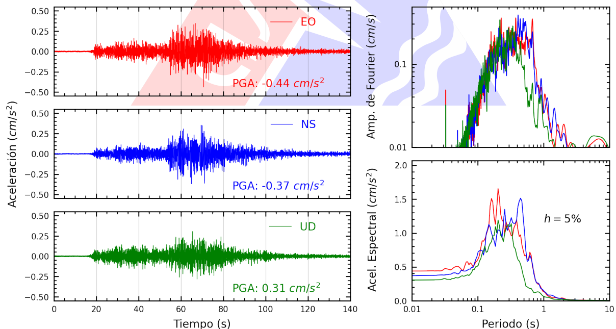
Figura A.6: Registros tiempo-historia, espectros de Fourier y de respuesta en las direcciones EO, NS y vertical de la estación CARAL. Sismo de Puerto Inca, Puerto Inca - Huanuco del 2025-05-22, 14:57:39 (Hora local)
