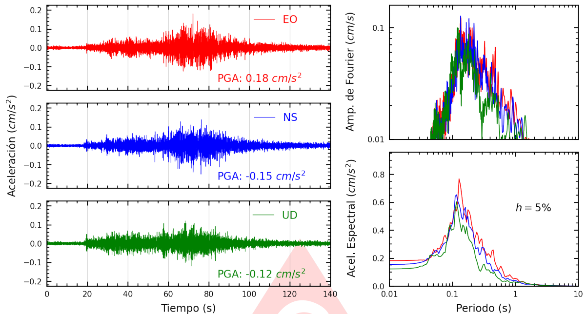
Figura A.15: Registros tiempo-historia, espectros de Fourier y de respuesta en las direcciones EO, NS y vertical de la estación JALV2. Sismo de Puerto Inca, Puerto Inca - Huanuco del 2025-05-22, 14:57:39 (Hora local)
