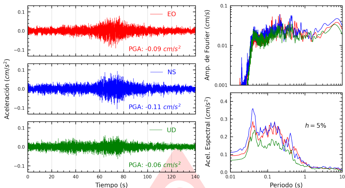
Figura A.19: Registros tiempo-historia, espectros de Fourier y de respuesta en las direcciones EO, NS y vertical de la estación SJLCE. Sismo de Puerto Inca, Puerto Inca - Huanuco del 2025-05-22, 14:57:39 (Hora local)
