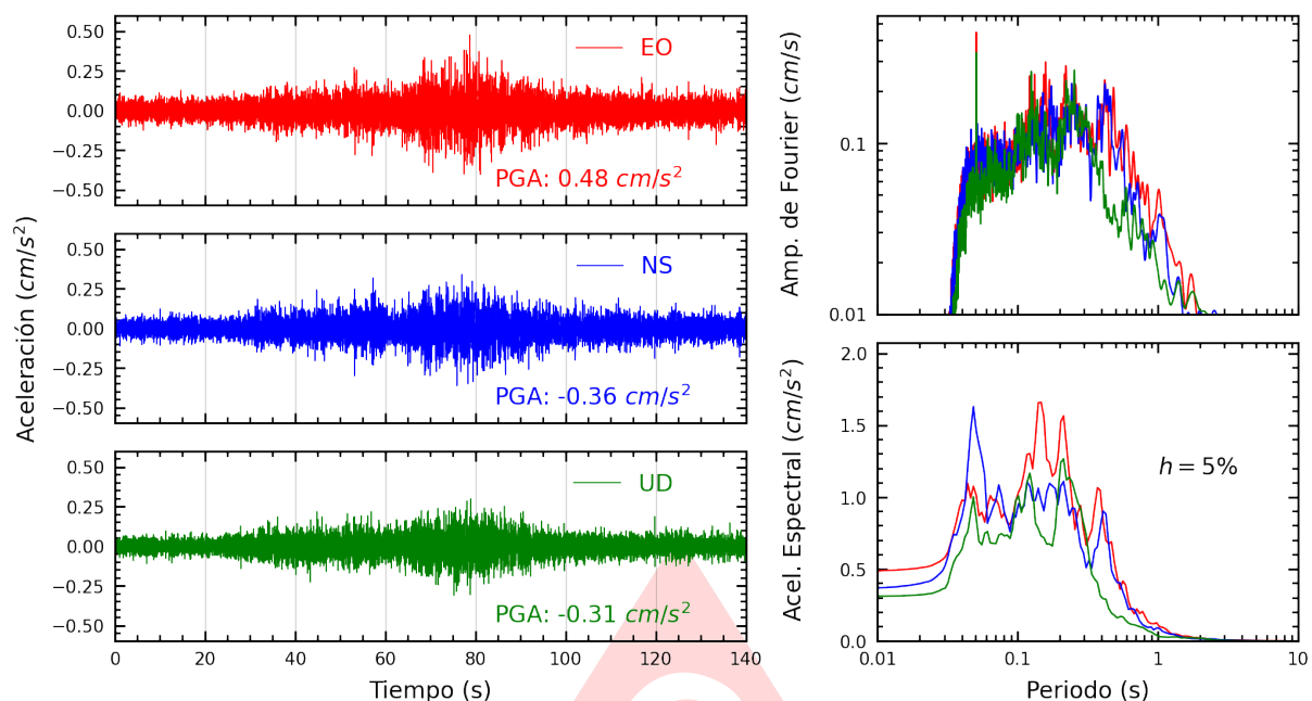
Figura A.5: Registros tiempo-historia, espectros de Fourier y de respuesta en las direcciones EO, NS y vertical de la estación PHER2. Sismo de Puerto Inca, Puerto Inca - Huanuco del 2025-05-22, 14:57:39 (Hora local)
