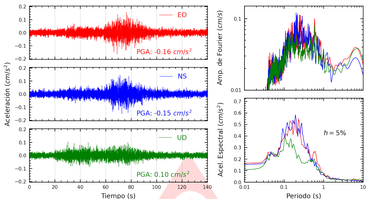
Figura A.17: Registros tiempo-historia, espectros de Fourier y de respuesta en las direcciones EO, NS y vertical de la estación SERVI. Sismo de Puerto Inca, Puerto Inca - Huanuco del 2025-05-22, 14:57:39 (Hora local)
