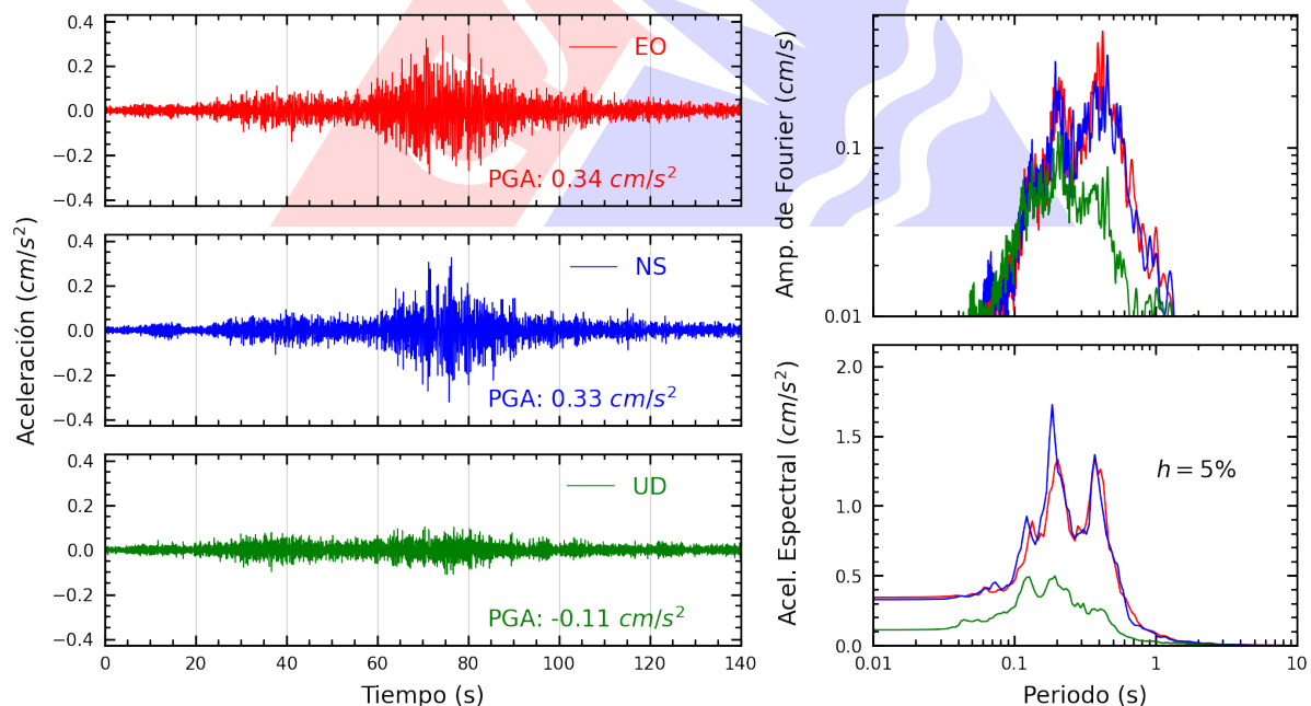
Figura A.8: Registros tiempo-historia, espectros de Fourier y de respuesta en las direcciones EO, NS y vertical de la estación VHAY2. Sismo de Puerto Inca, Puerto Inca - Huanuco del 2025-05-22, 14:57:39 (Hora local)
