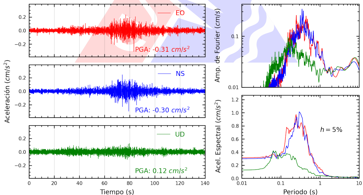
Figura A.10: Registros tiempo-historia, espectros de Fourier y de respuesta en las direcciones EO, NS y vertical de la estación ACAPU. Sismo de Puerto Inca, Puerto Inca - Huanuco del 2025-05-22, 14:57:39 (Hora local)
