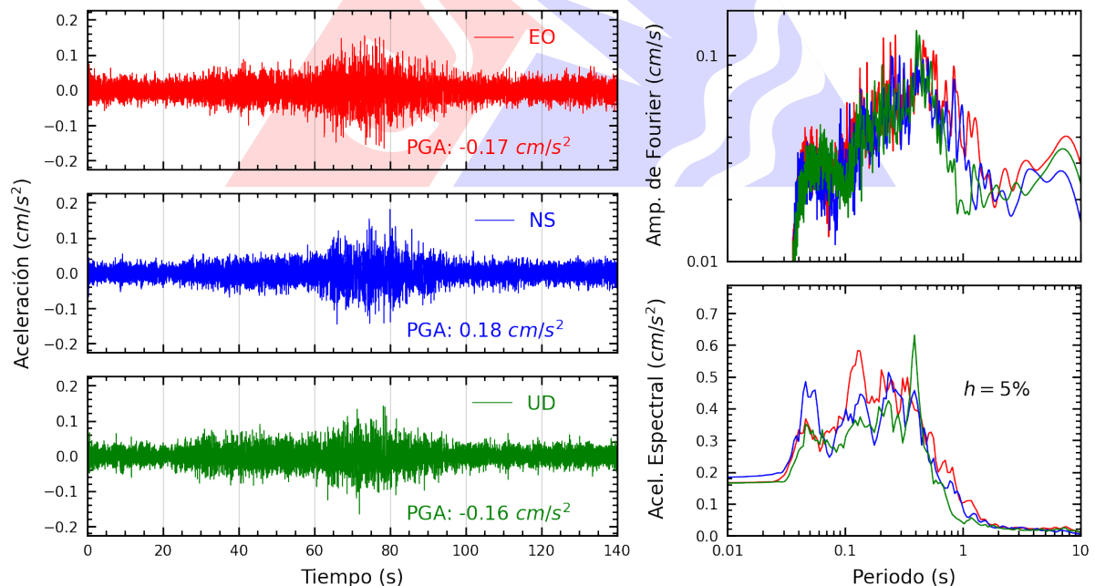
Figura A.16: Registros tiempo-historia, espectros de Fourier y de respuesta en las direcciones EO, NS y vertical de la estación IMCA. Sismo de Puerto Inca, Puerto Inca - Huanuco del 2025-05-22, 14:57:39 (Hora local)
