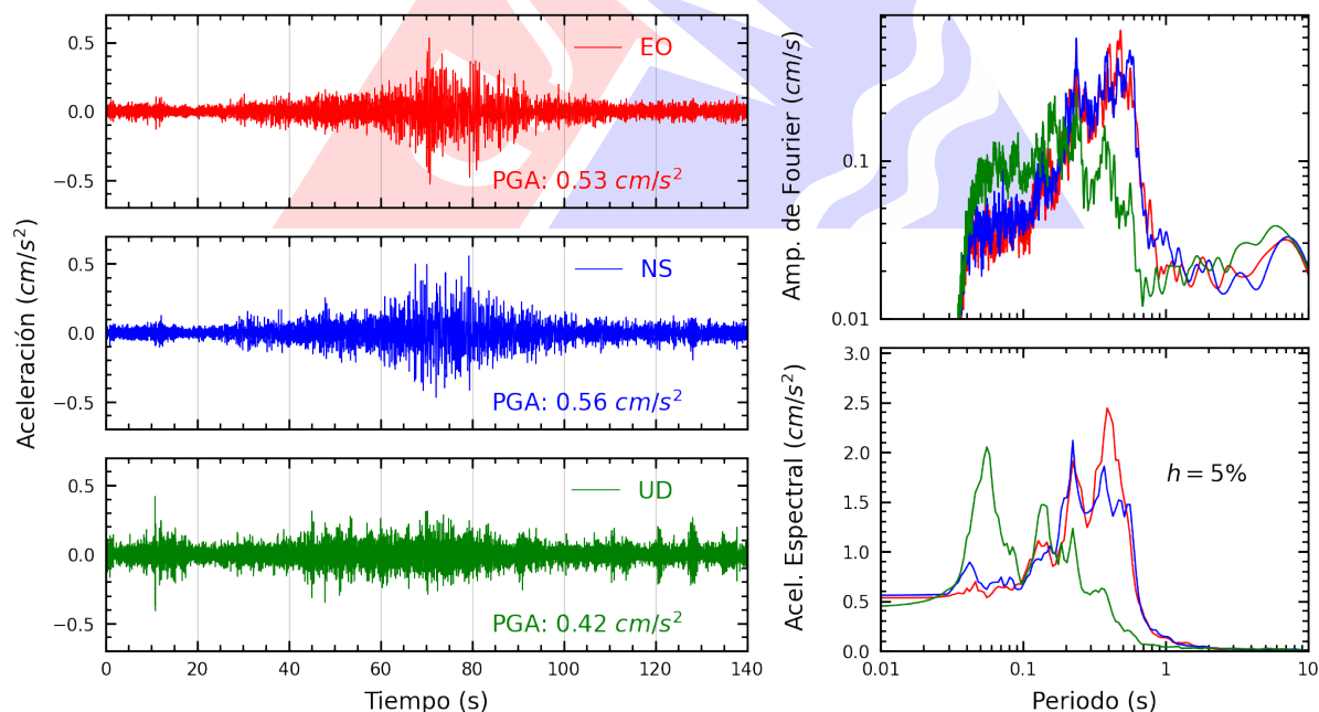
Figura A.4: Registros tiempo-historia, espectros de Fourier y de respuesta en las direcciones EO, NS y vertical de la estación MDPP. Sismo de Puerto Inca, Puerto Inca - Huanuco del 2025-05-22, 14:57:39 (Hora local)
