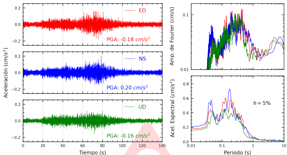
Figura A.13: Registros tiempo-historia, espectros de Fourier y de respuesta en las direcciones EO, NS y vertical de la estación COMAS. Sismo de Puerto Inca, Puerto Inca - Huanuco del 2025-05-22, 14:57:39 (Hora local)
