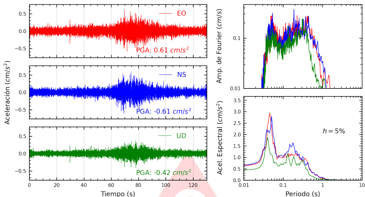
Figura A.3: Registros tiempo-historia, espectros de Fourier y de respuesta en las direcciones EO, NS y vertical de la estación UNTEL. Sismo de Puerto Inca, Puerto Inca - Huanuco del 2025-05-22, 14:57:39 (Hora local)
