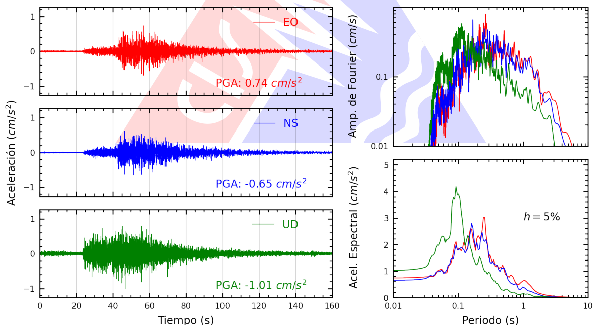
Figura A.2: Registros tiempo-historia, espectros de Fourier y de respuesta en las direcciones EO, NS y vertical de la estación SCPUC. Sismo de Puerto Inca, Puerto Inca - Huanuco del 2025-05-22, 14:57:39 (Hora local)
