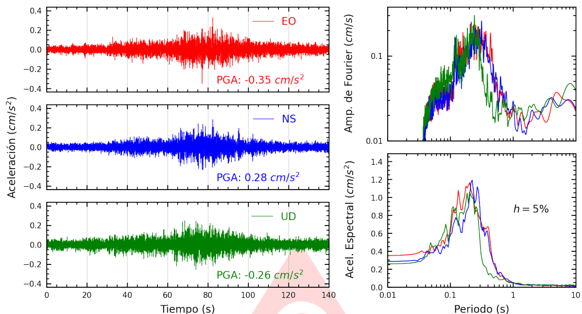
Figura A.7: Registros tiempo-historia, espectros de Fourier y de respuesta en las direcciones EO, NS y vertical de la estación SOVES. Sismo de Puerto Inca, Puerto Inca - Huanuco del 2025-05-22, 14:57:39 (Hora local)
