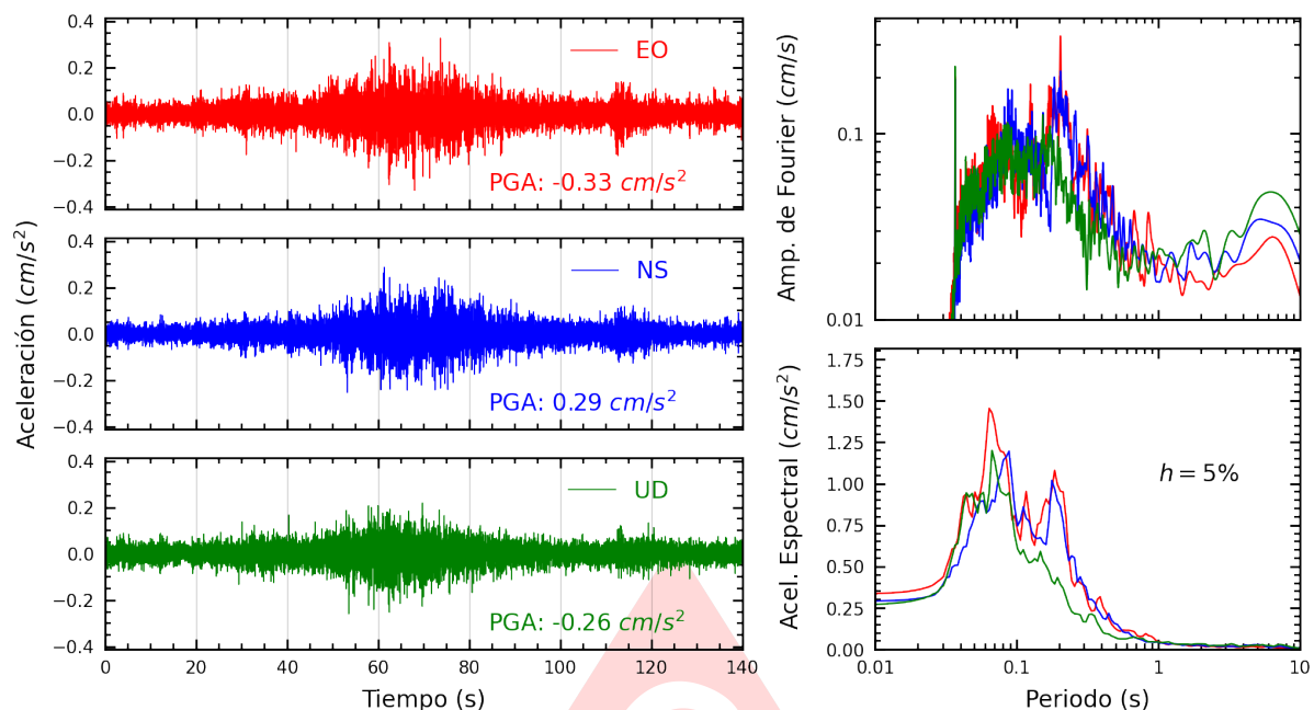
Figura A.9: Registros tiempo-historia, espectros de Fourier y de respuesta en las direcciones EO, NS y vertical de la estación INDEP. Sismo de Puerto Inca, Puerto Inca - Huanuco del 2025-05-22, 14:57:39 (Hora local)
