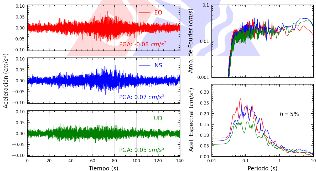
Figura A.20: Registros tiempo-historia, espectros de Fourier y de respuesta en las direcciones EO, NS y vertical de la estación UCSS. Sismo de Puerto Inca, Puerto Inca - Huanuco del 2025-05-22, 14:57:39 (Hora local)
