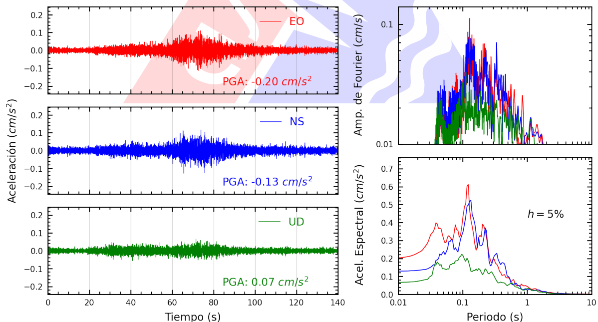
Figura A.14: Registros tiempo-historia, espectros de Fourier y de respuesta en las direcciones EO, NS y vertical de la estación ATARJ. Sismo de Puerto Inca, Puerto Inca - Huanuco del 2025-05-22, 14:57:39 (Hora local)
