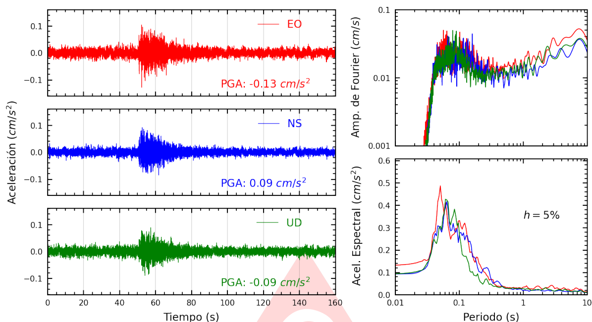
Figura A.7: Registros tiempo-historia, espectros de Fourier y de respuesta en las direcciones EO, NS y vertical de la estación AMORE. Sismo de Tocache Nuevo, Tocache - San Martín del 2025-05-23, 12:16:15 (Hora local)
