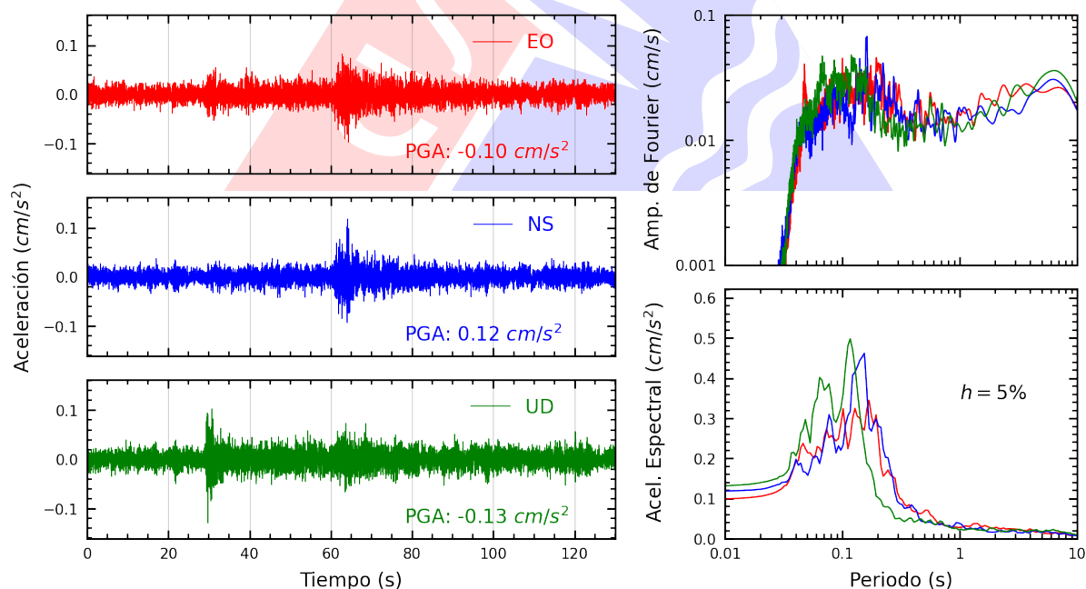
Figura A.6: Registros tiempo-historia, espectros de Fourier y de respuesta en las direcciones EO, NS y vertical de la estación UPAT. Sismo de Tocache Nuevo, Tocache - San Martin del 2025-05-23, 12:16:15 (Hora local)
