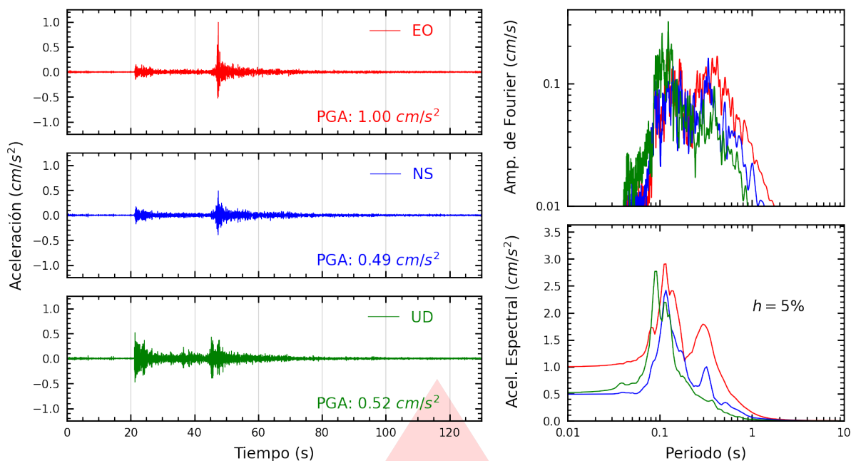
Figura A.1: Registros tiempo-historia, espectros de Fourier y de respuesta en las direcciones EO, NS y vertical de la estación UNIA. Sismo de Tocache Nuevo, Tocache - San Martin del 2025-05-23, 12:16:15 (Hora local)
