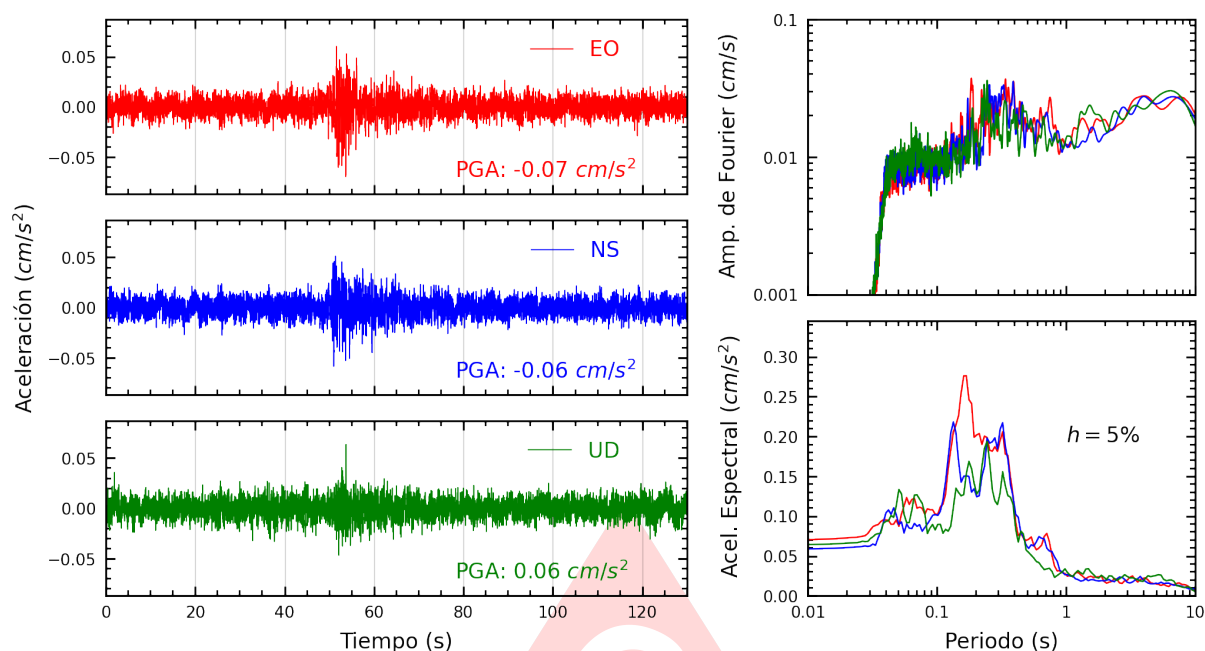
Figura A.9: Registros tiempo-historia, espectros de Fourier y de respuesta en las direcciones EO, NS y vertical de la estación UNASA. Sismo de Tocache Nuevo, Tocache - San Martin del 2025-05-23, 12:16:15 (Hora local)
