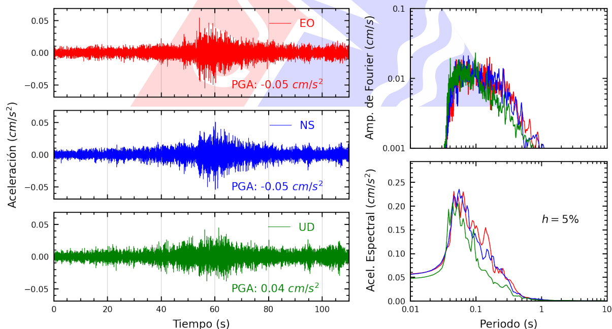
Figura A.10: Registros tiempo-historia, espectros de Fourier y de respuesta en las direcciones EO, NS y vertical de la estación JALV2. Sismo de Tocache Nuevo, Tocache - San Martin del 2025-05-23, 12:16:15 (Hora local)
