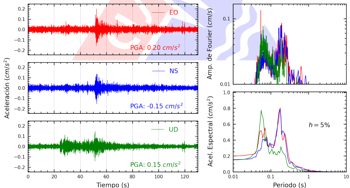
Figura A.4: Registros tiempo-historia, espectros de Fourier y de respuesta en las direcciones EO, NS y vertical de la estación UNAAA. Sismo de Tocache Nuevo, Tocache - San Martín del 2025-05-23, 12:16:15 (Hora local)
