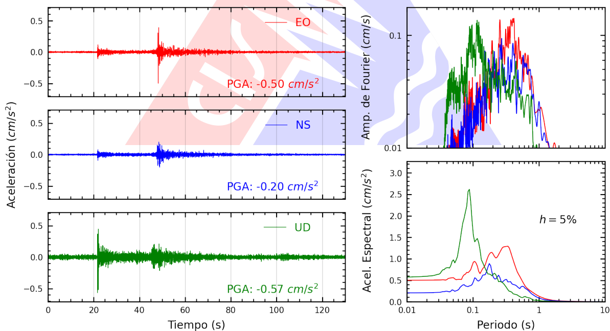
Figura A.2: Registros tiempo-historia, espectros de Fourier y de respuesta en las direcciones EO, NS y vertical de la estación SCPUC. Sismo de Tocache Nuevo, Tocache - San Martin del 2025-05-23, 12:16:15 (Hora local)
