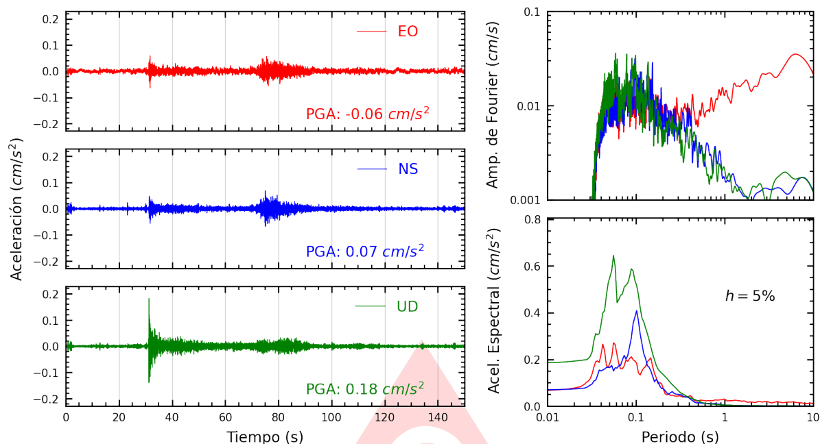
Figura A.5: Registros tiempo-historia, espectros de Fourier y de respuesta en las direcciones EO, NS y vertical de la estación SCCHI. Sismo de Tocache Nuevo, Tocache - San Martin del 2025-05-23, 12:16:15 (Hora local)
