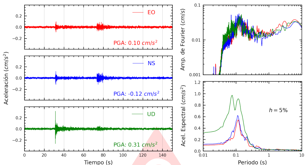
Figura A.3: Registros tiempo-historia, espectros de Fourier y de respuesta en las direcciones EO, NS y vertical de la estación UCVCH. Sismo de Tocache Nuevo, Tocache - San Martín del 2025-05-23, 12:16:15 (Hora local)
