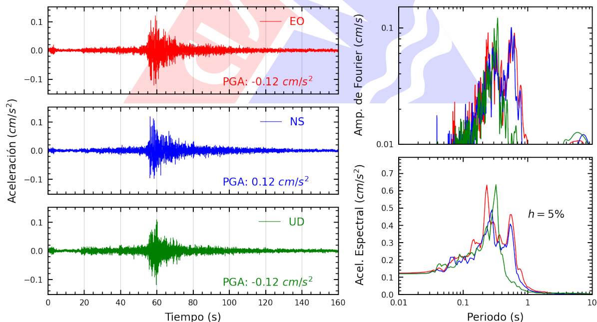
Figura A.8: Registros tiempo-historia, espectros de Fourier y de respuesta en las direcciones EO, NS y vertical de la estación CARAL. Sismo de Tocache Nuevo, Tocache - San Martín del 2025-05-23, 12:16:15 (Hora local)
