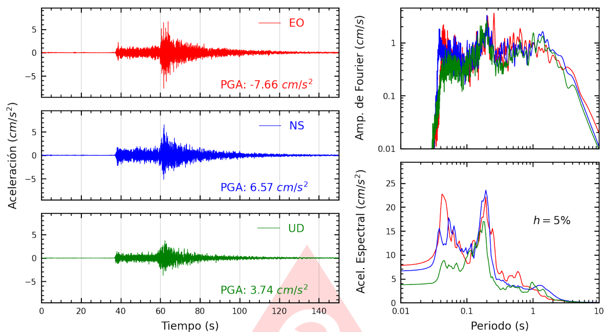
Figura A.3: Registros tiempo-historia, espectros de Fourier y de respuesta en las direcciones EO, NS y vertical de la estación UPTAC. Sismo de Tacna, Tacna - Tacna del 2025-05-25, 22:50:26 (Hora local)
