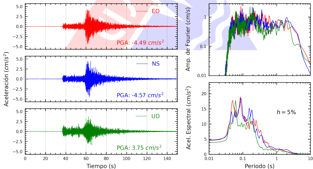
Figura A.4: Registros tiempo-historia, espectros de Fourier y de respuesta en las direcciones EO, NS y vertical de la estación CREY. Sismo de Tacna, Tacna - Tacna del 2025-05-25, 22:50:26 (Hora local)
