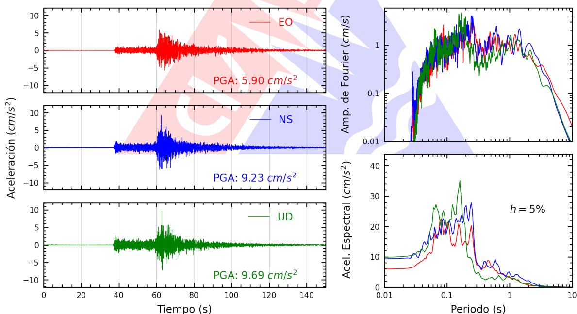
Figura A.2: Registros tiempo-historia, espectros de Fourier y de respuesta en las direcciones EO, NS y vertical de la estación UJBG4. Sismo de Tacna, Tacna - Tacna del 2025-05-25, 22:50:26 (Hora local)
