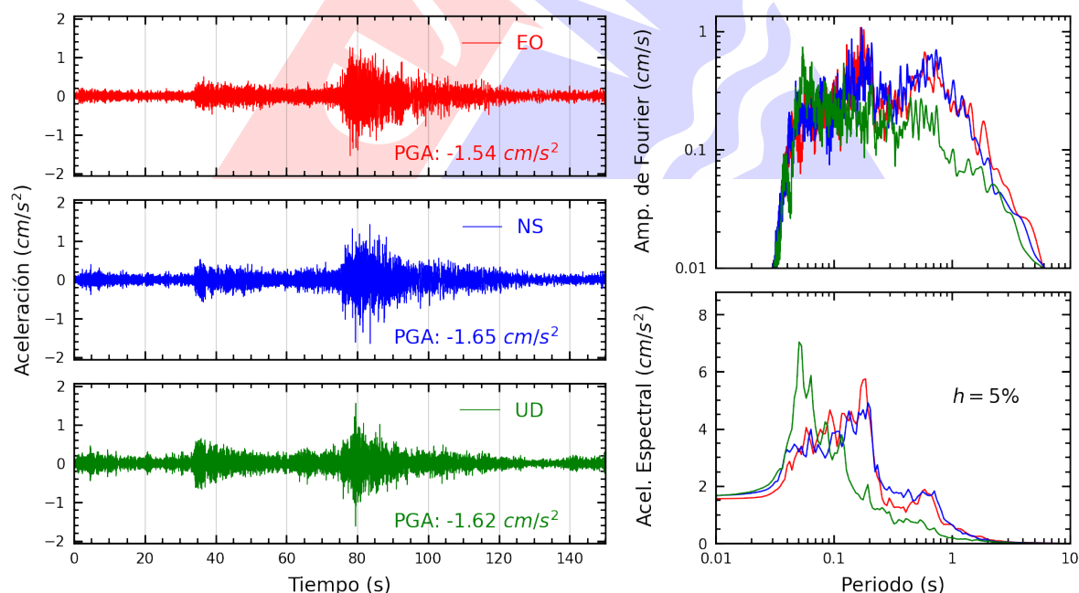
Figura A.6: Registros tiempo-historia, espectros de Fourier y de respuesta en las direcciones EO, NS y vertical de la estación SCAR2. Sismo de Tacna, Tacna - Tacna del 2025-05-25, 22:50:26 (Hora local)
