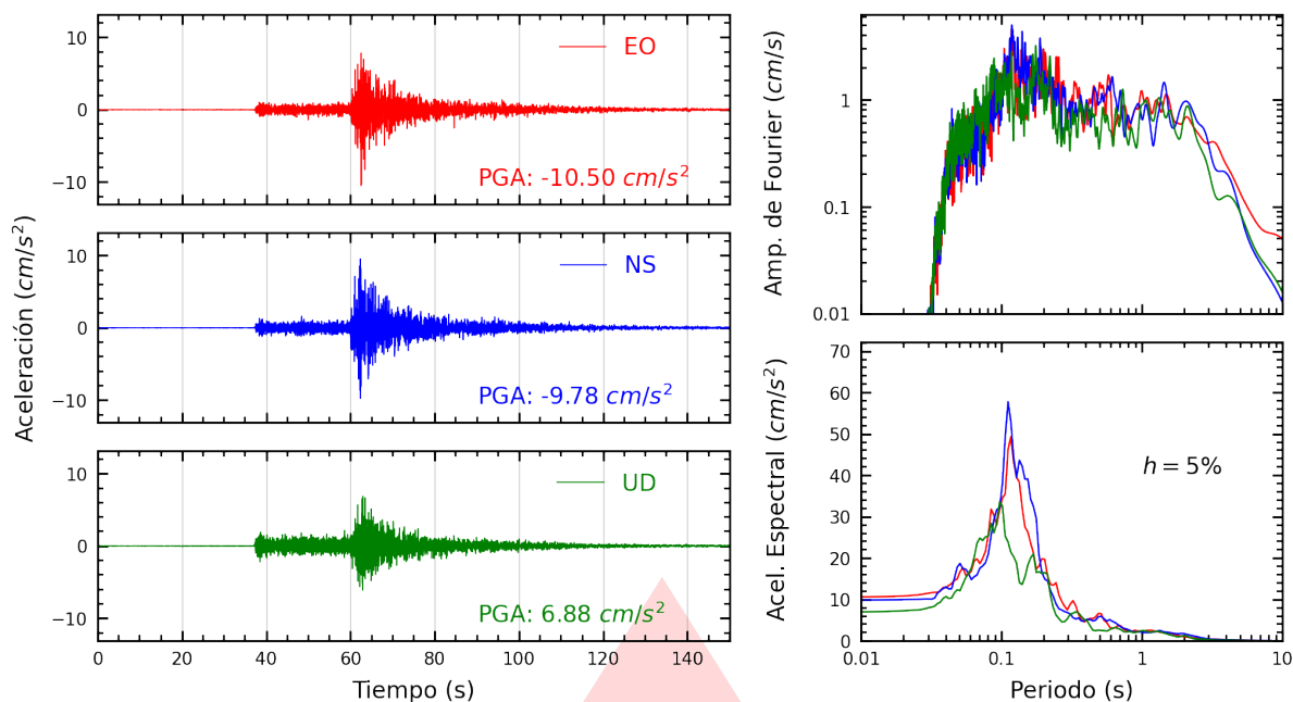
Figura A.1: Registros tiempo-historia, espectros de Fourier y de respuesta en las direcciones EO, NS y vertical de la estación UJBG3. Sismo de Tacna, Tacna - Tacna del 2025-05-25, 22:50:26 (Hora local)
