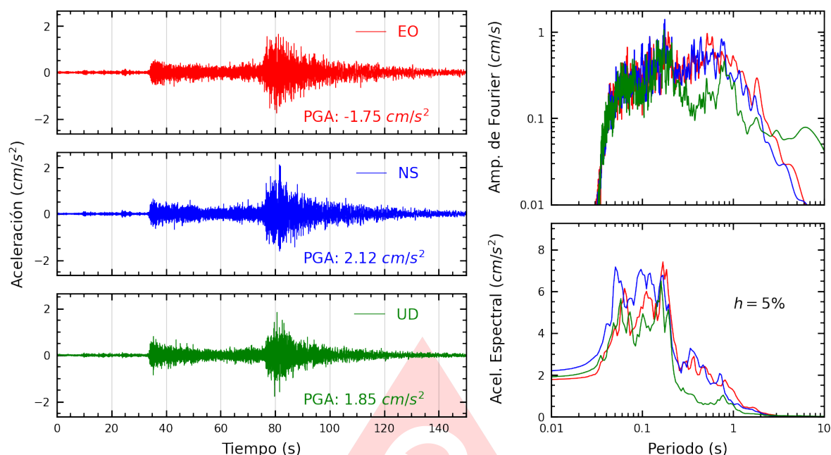
Figura A.5: Registros tiempo-historia, espectros de Fourier y de respuesta en las direcciones EO, NS y vertical de la estación SCARQ. Sismo de Tacna, Tacna - Tacna del 2025-05-25, 22:50:26 (Hora local)
